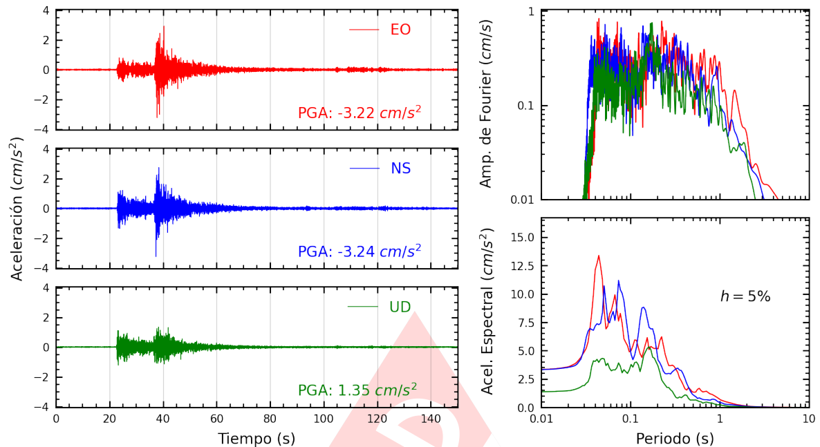
Figura A.3: Registros tiempo-historia, espectros de Fourier y de respuesta en las direcciones EO, NS y vertical de la estación UPTAC. Sismo de Calana, Tacna - Tacna del 2025-02-01, 15:27:24 (Hora local)
