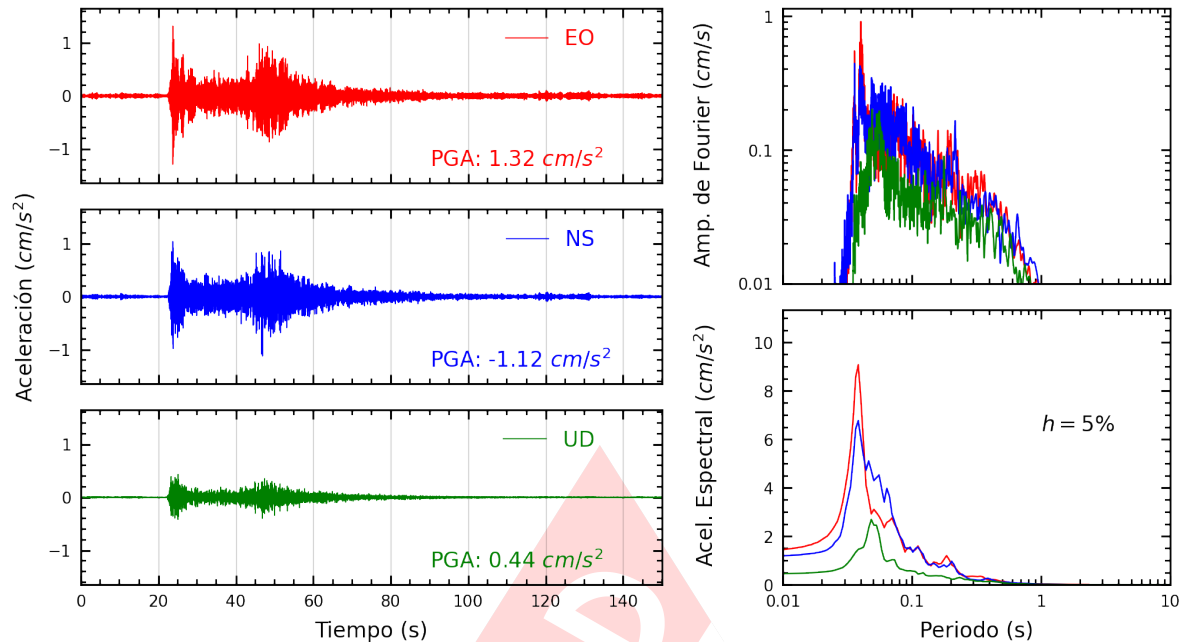
Figura A.5: Registros tiempo-historia, espectros de Fourier y de respuesta en las direcciones EO, NS y vertical de la estación UNAM. Sismo de Calana, Tacna - Tacna del 2025-02-01, 15:27:24 (Hora local)
