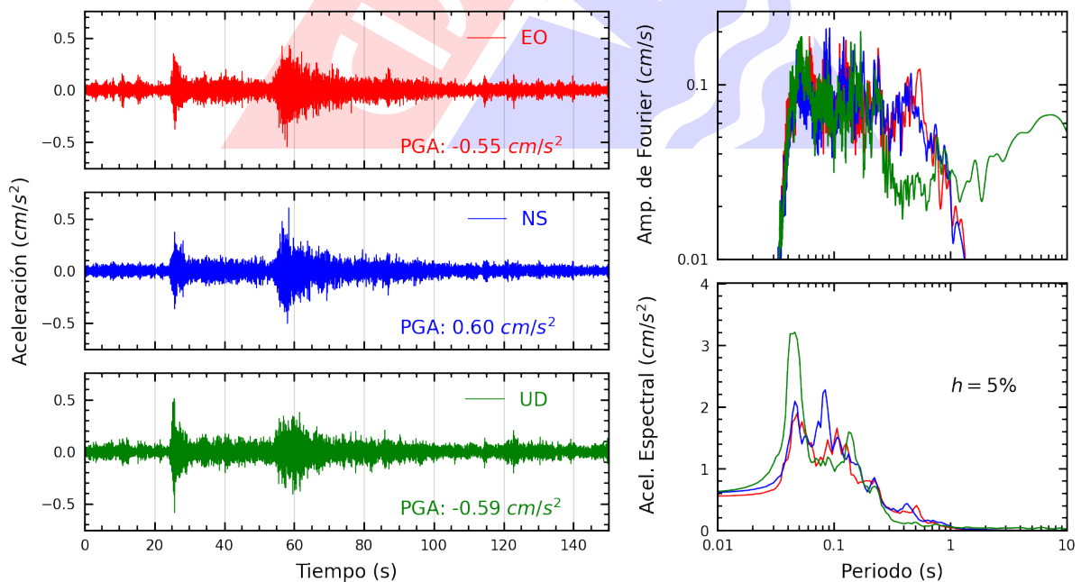
Figura A.6: Registros tiempo-historia, espectros de Fourier y de respuesta en las direcciones EO, NS y vertical de la estación SCARQ. Sismo de Calana, Tacna - Tacna del 2025-02-01, 15:27:24 (Hora local)
