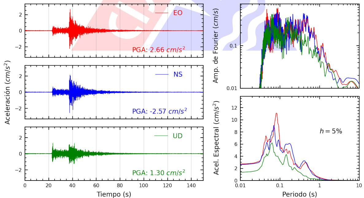
Figura A.4: Registros tiempo-historia, espectros de Fourier y de respuesta en las direcciones EO, NS y vertical de la estación CREY. Sismo de Calana, Tacna - Tacna del 2025-02-01, 15:27:24 (Hora local)
