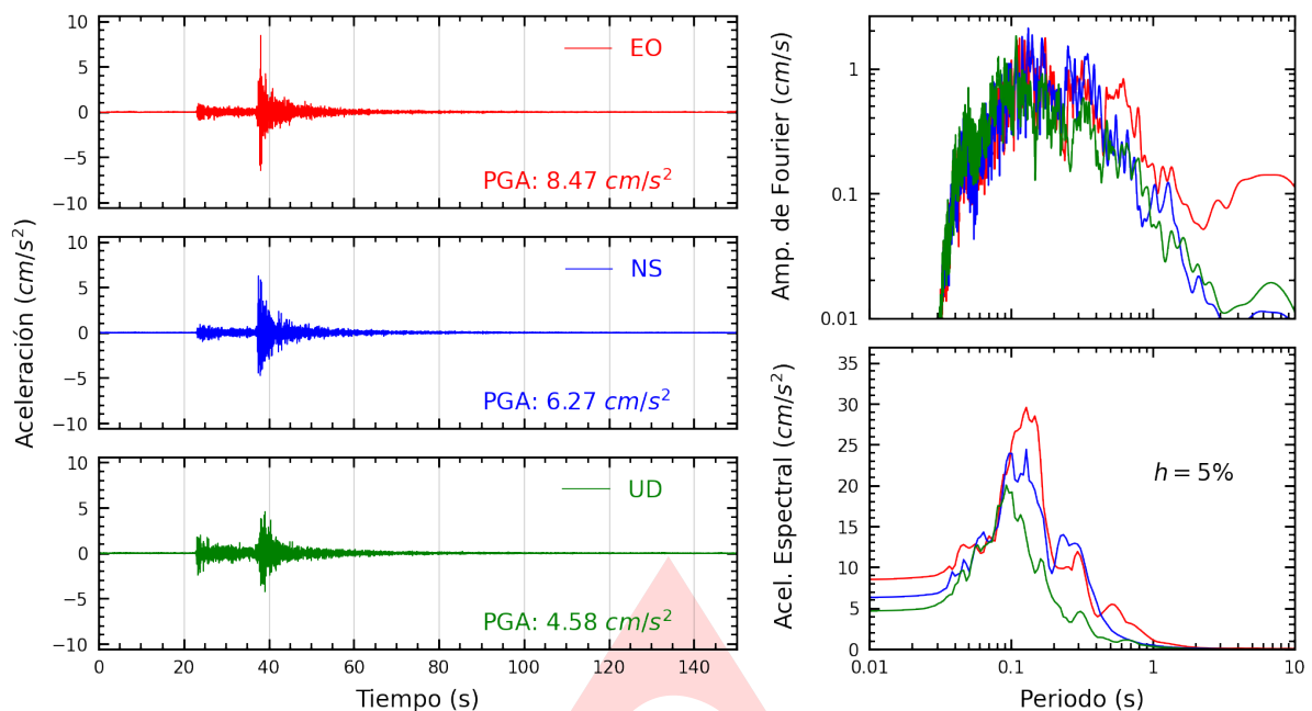
Figura A.1: Registros tiempo-historia, espectros de Fourier y de respuesta en las direcciones EO, NS y vertical de la estación UJBG3. Sismo de Calana, Tacna - Tacna del 2025-02-01, 15:27:24 (Hora local)
