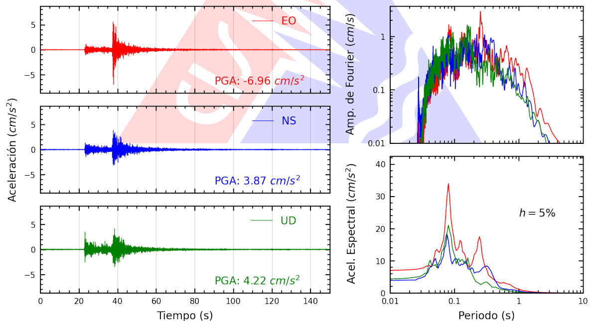
Figura A.2: Registros tiempo-historia, espectros de Fourier y de respuesta en las direcciones EO, NS y vertical de la estación UJBG4. Sismo de Calana, Tacna - Tacna del 2025-02-01, 15:27:24 (Hora local)
