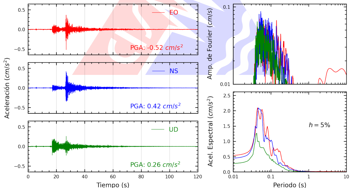
Figura A.2: Registros tiempo-historia, espectros de Fourier y de respuesta en las direcciones EO, NS y vertical de la estación SCCHI. Sismo de Olmos, Lambayeque - Lambayeque del 2025-02-02, 01:47:03 (Hora local)
