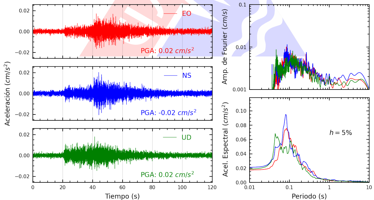
Figura A.6: Registros tiempo-historia, espectros de Fourier y de respuesta en las direcciones EO, NS y vertical de la estación UNF. Sismo de Olmos, Lambayeque - Lambayeque del 2025-02-02, 01:47:03 (Hora local)
