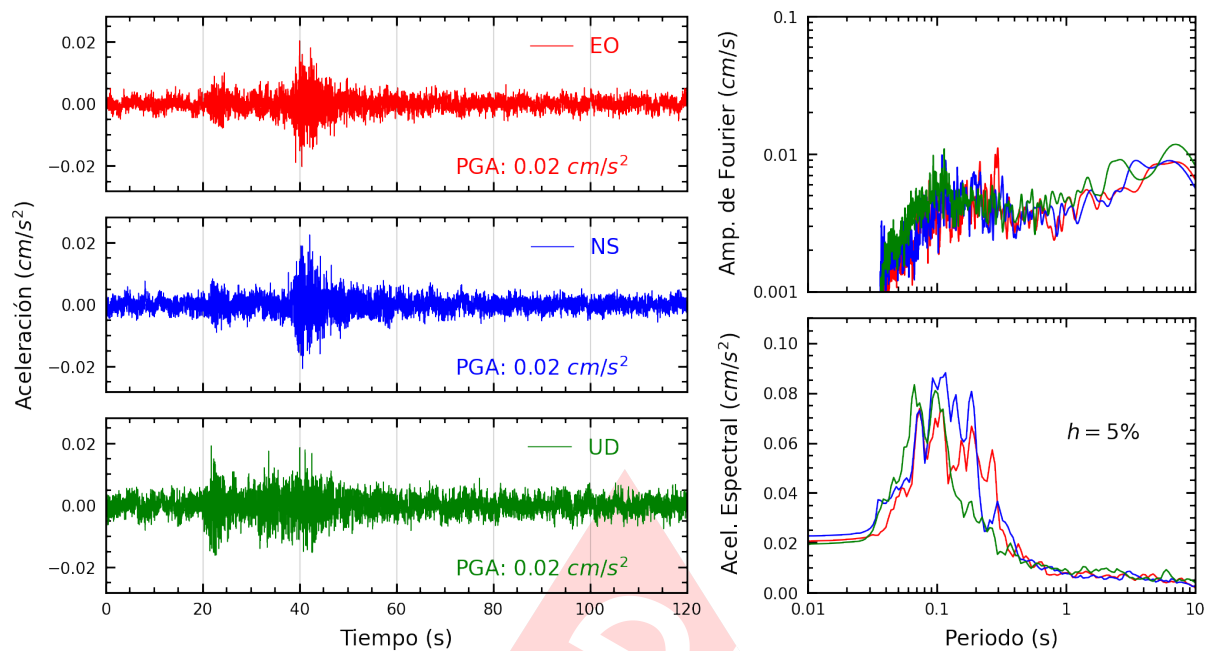
Figura A.5: Registros tiempo-historia, espectros de Fourier y de respuesta en las direcciones EO, NS y vertical de la estación UNJ. Sismo de Olmos, Lambayeque - Lambayeque del 2025-02-02, 01:47:03 (Hora local)
