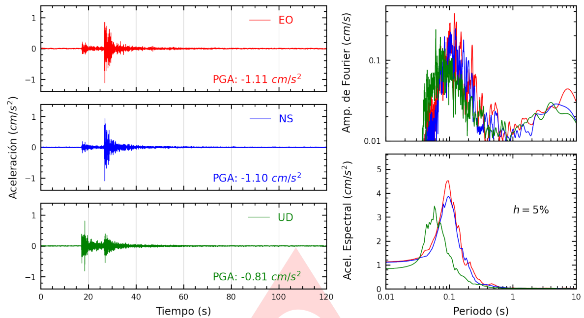
Figura A.1: Registros tiempo-historia, espectros de Fourier y de respuesta en las direcciones EO, NS y vertical de la estación UCVCH. Sismo de Olmos, Lambayeque - Lambayeque del 2025-02-02, 01:47:03 (Hora local)
