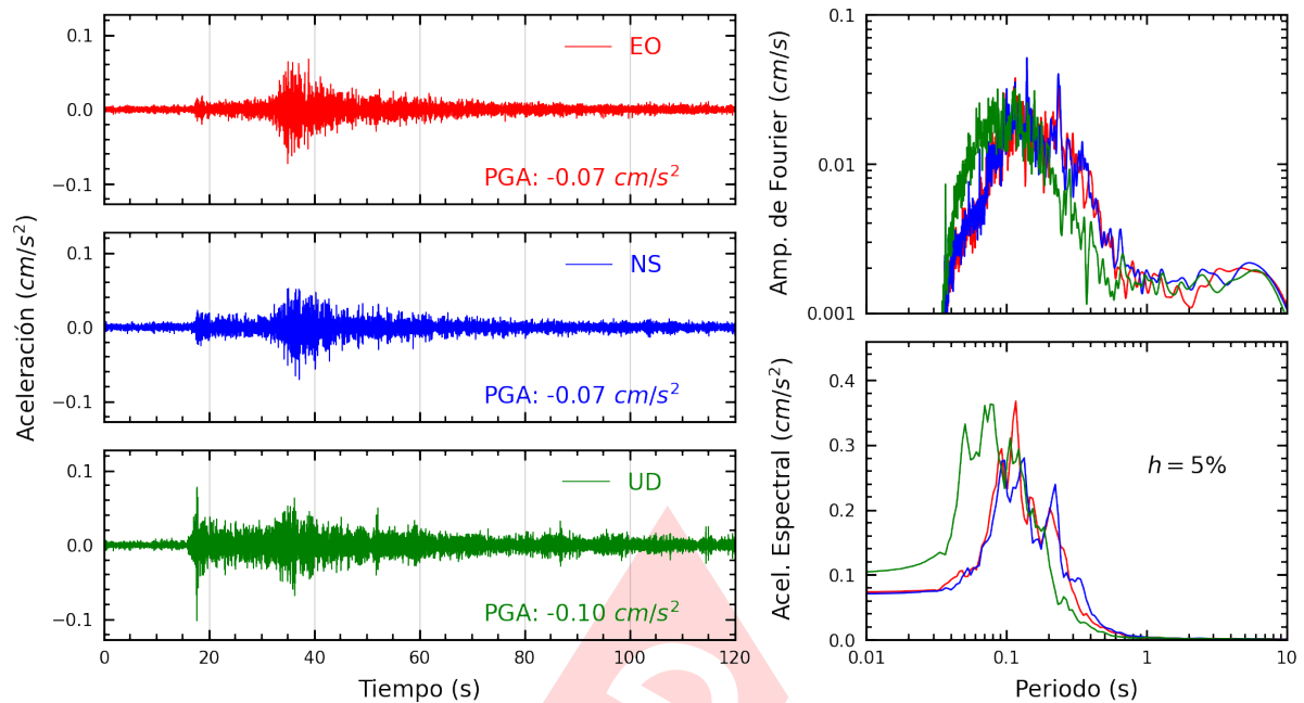
Figura A.3: Registros tiempo-historia, espectros de Fourier y de respuesta en las direcciones EO, NS y vertical de la estación UNP. Sismo de Olmos, Lambayeque - Lambayeque del 2025-02-02, 01:47:03 (Hora local)
