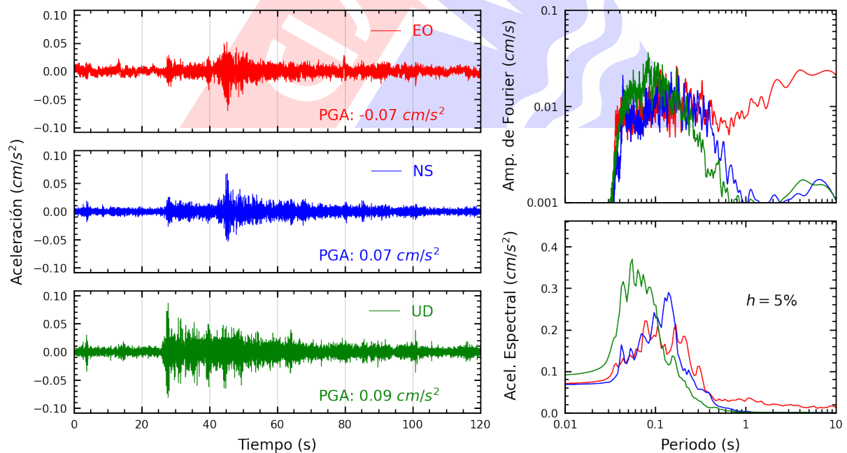
Figura A.4: Registros tiempo-historia, espectros de Fourier y de respuesta en las direcciones EO, NS y vertical de la estación SCPIU. Sismo de Olmos, Lambayeque - Lambayeque del 2025-02-02, 01:47:03 (Hora local)
