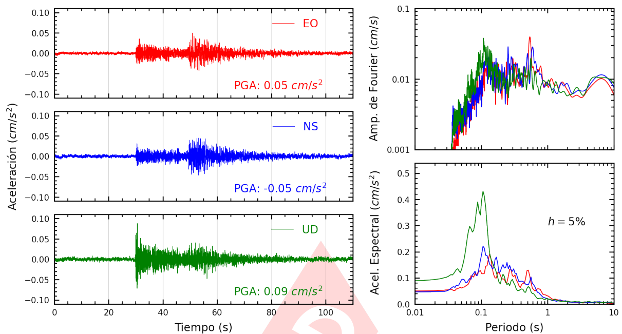
Figura A.3: Registros tiempo-historia, espectros de Fourier y de respuesta en las direcciones EO, NS y vertical de la estación UNJ. Sismo de Nueva Cajamarca, Rioja - San Martín del 2025-02-04, 04:12:02 (Hora local)
