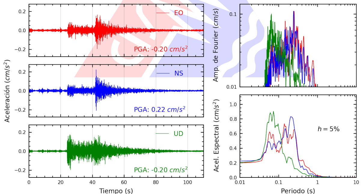
Figura A.2: Registros tiempo-historia, espectros de Fourier y de respuesta en las direcciones EO, NS y vertical de la estación UNAAA. Sismo de Nueva Cajamarca, Rioja - San Martín del 2025-02-04, 04:12:02 (Hora local)
