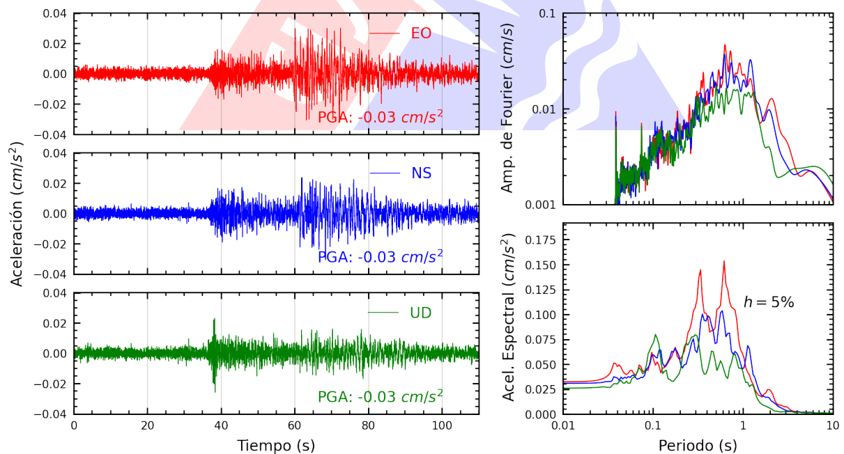
Figura A.4: Registros tiempo-historia, espectros de Fourier y de respuesta en las direcciones EO, NS y vertical de la estación UNC. Sismo de Nueva Cajamarca, Rioja - San Martín del 2025-02-04, 04:12:02 (Hora local)
