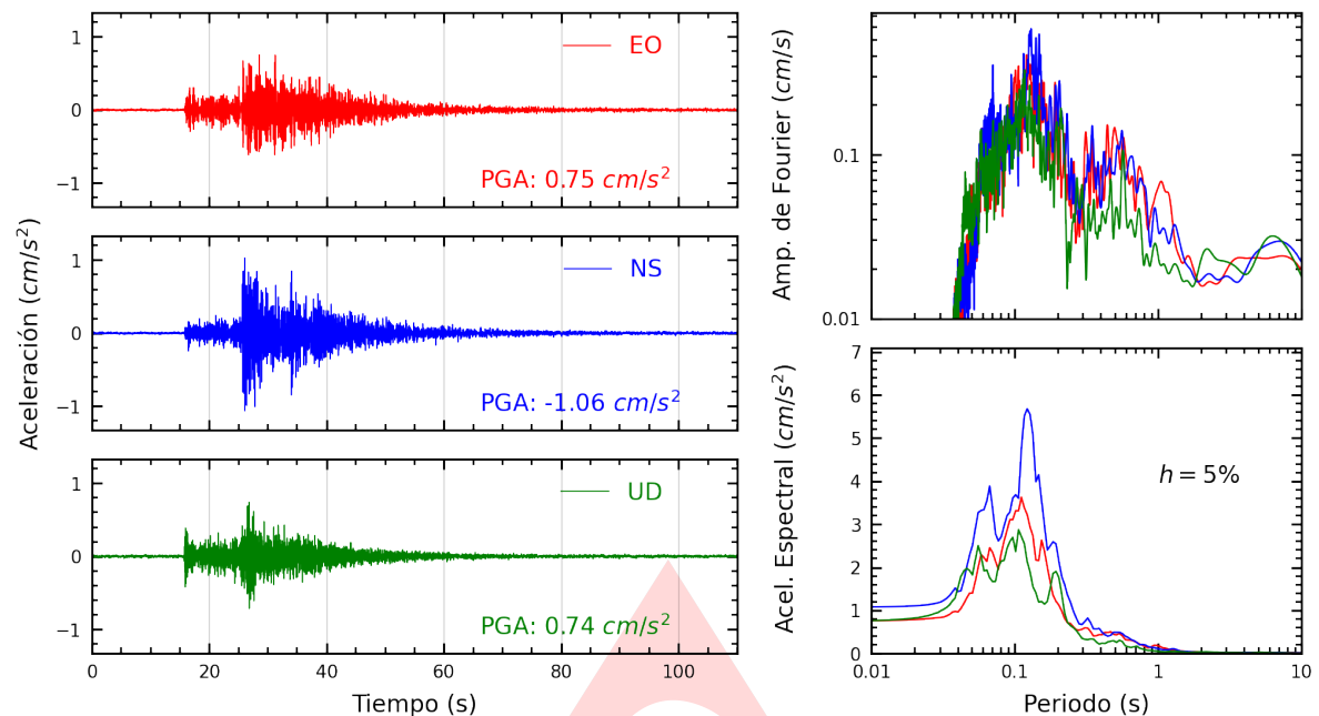
Figura A.1: Registros tiempo-historia, espectros de Fourier y de respuesta en las direcciones EO, NS y vertical de la estación UNTRM. Sismo de Nueva Cajamarca, Rioja - San Martín del 2025-02-04, 04:12:02 (Hora local)
