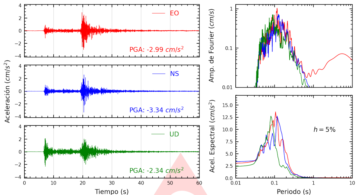
Figura A.1: Registros tiempo-historia, espectros de Fourier y de respuesta en las direcciones EO, NS y vertical de la estación UJBG3. Sismo de Calana, Tacna - Tacna del 2025-02-06, 01:02:58 (Hora local)
