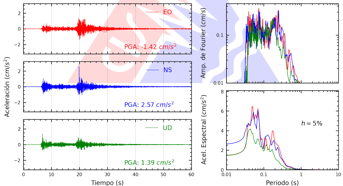
Figura A.2: Registros tiempo-historia, espectros de Fourier y de respuesta en las direcciones EO, NS y vertical de la estación UPTAC. Sismo de Calana, Tacna - Tacna del 2025-02-06, 01:02:58 (Hora local)
