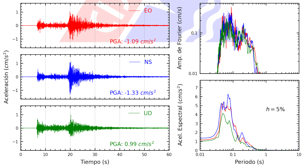
Figura A.4: Registros tiempo-historia, espectros de Fourier y de respuesta en las direcciones EO, NS y vertical de la estación CREY. Sismo de Calana, Tacna - Tacna del 2025-02-06, 01:02:58 (Hora local)
