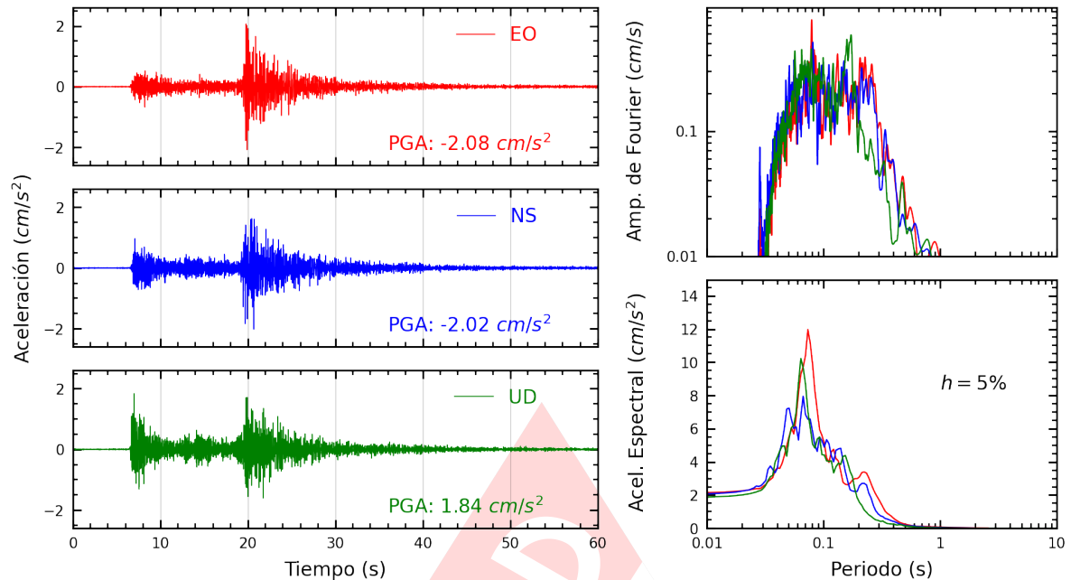
Figura A.3: Registros tiempo-historia, espectros de Fourier y de respuesta en las direcciones EO, NS y vertical de la estación UJBG4. Sismo de Calana, Tacna - Tacna del 2025-02-06, 01:02:58 (Hora local)
