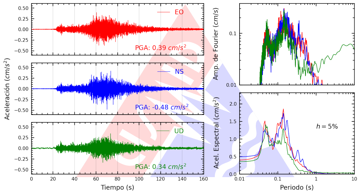
Figura A.7: Registros tiempo-historia, espectros de Fourier y de respuesta en las direcciones EO, NS y vertical de la estación SCARQ. Sismo de Puno, Puno - Puno del 2025-02-07, 02:24:44 (Hora local)
