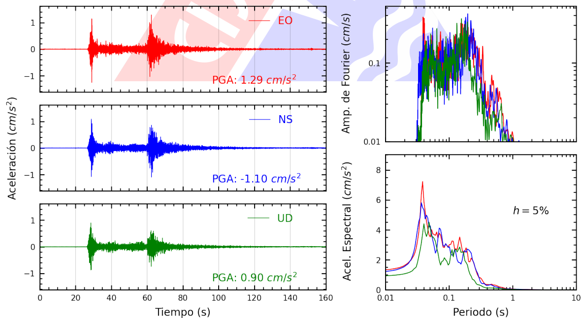
Figura A.4: Registros tiempo-historia, espectros de Fourier y de respuesta en las direcciones EO, NS y vertical de la estación UPTAC. Sismo de Puno, Puno - Puno del 2025-02-07, 02:24:44 (Hora local)
