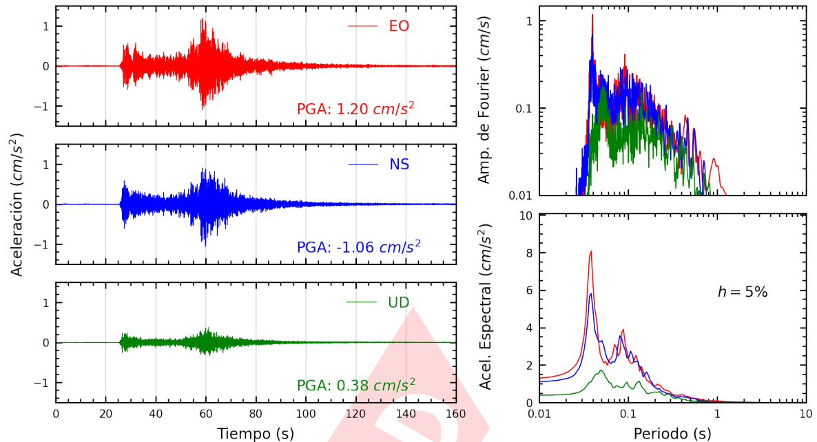
Figura A.5: Registros tiempo-historia, espectros de Fourier y de respuesta en las direcciones EO, NS y vertical de la estación UNAM. Sismo de Puno, Puno - Puno del 2025-02-07, 02:24:44 (Hora local)
