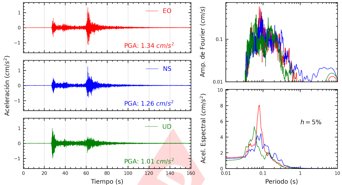
Figura A.3: Registros tiempo-historia, espectros de Fourier y de respuesta en las direcciones EO, NS y vertical de la estación CREY. Sismo de Puno, Puno - Puno del 2025-02-07, 02:24:44 (Hora local)
