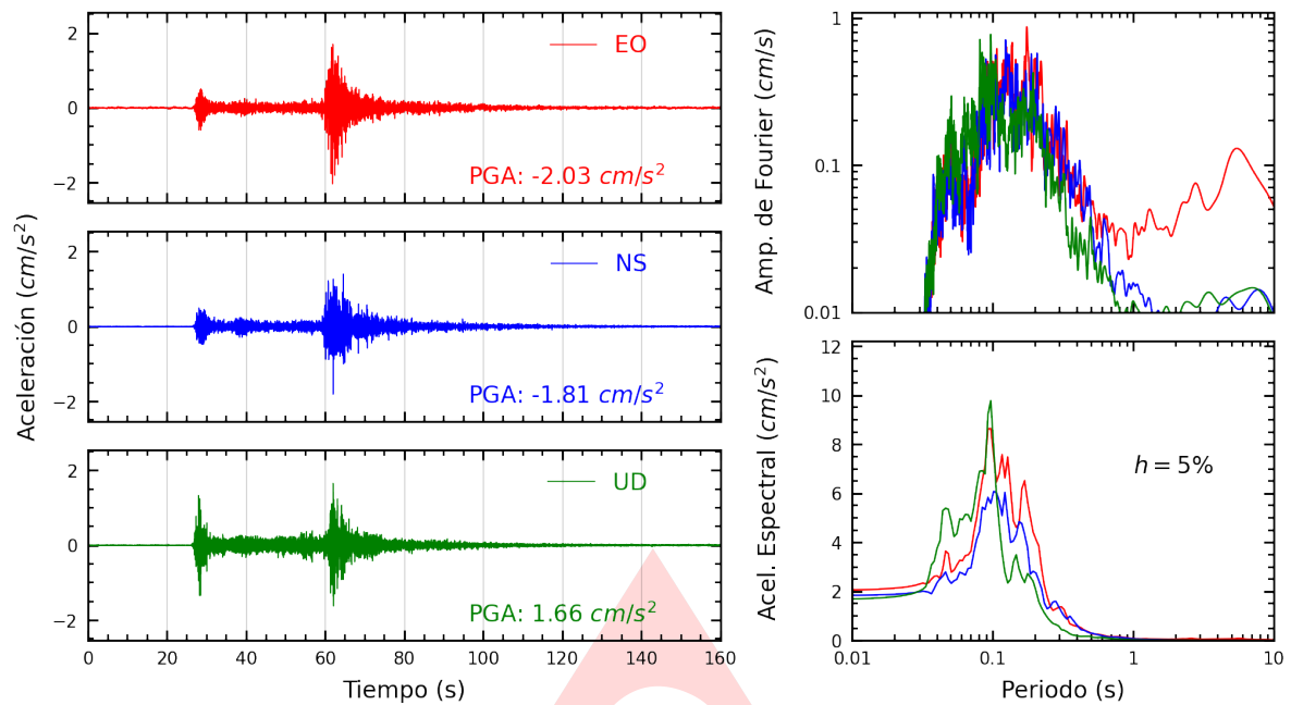
Figura A.1: Registros tiempo-historia, espectros de Fourier y de respuesta en las direcciones EO, NS y vertical de la estación UJBG3. Sismo de Puno, Puno - Puno del 2025-02-07, 02:24:44 (Hora local)
