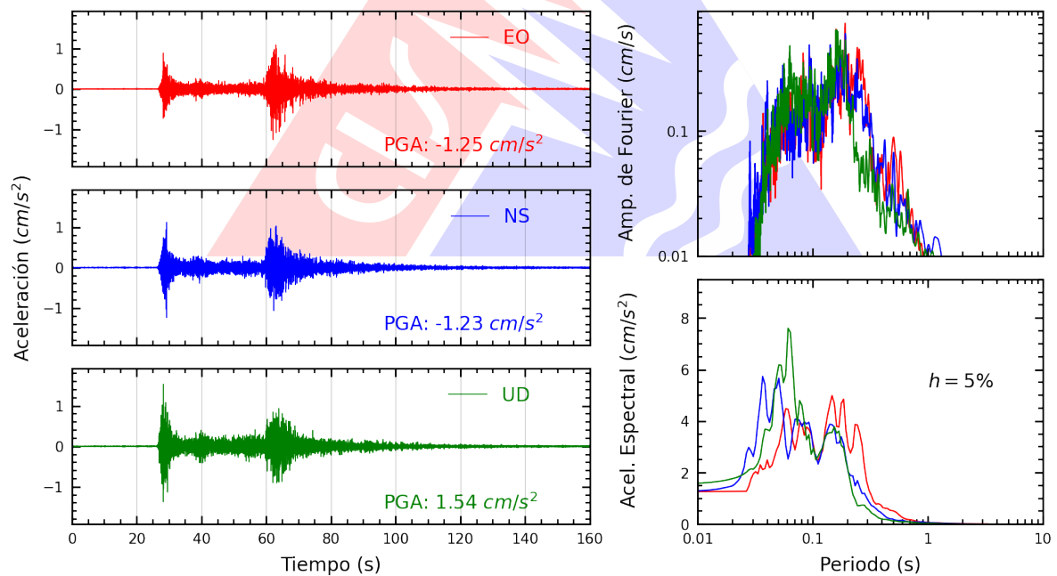
Figura A.2: Registros tiempo-historia, espectros de Fourier y de respuesta en las direcciones EO, NS y vertical de la estación UJBG4. Sismo de Puno, Puno - Puno del 2025-02-07, 02:24:44 (Hora local)
