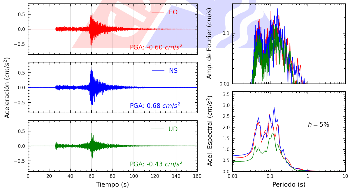
Figura A.6: Registros tiempo-historia, espectros de Fourier y de respuesta en las direcciones EO, NS y vertical de la estación UNSA2. Sismo de Puno, Puno - Puno del 2025-02-07, 02:24:44 (Hora local)
