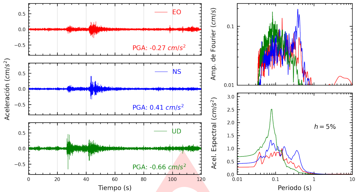
Figura A.1: Registros tiempo-historia, espectros de Fourier y de respuesta en las direcciones EO, NS y vertical de la estación SCPIU. Sismo de Ayabaca, Ayabaca - Piura del 2025-02-08, 09:12:54 (Hora local)
