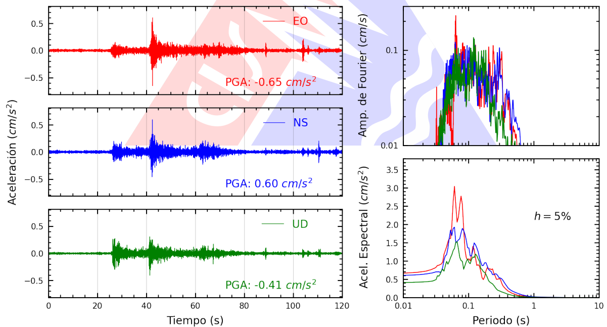
Figura A.2: Registros tiempo-historia, espectros de Fourier y de respuesta en las direcciones EO, NS y vertical de la estación UPAOP. Sismo de Ayabaca, Ayabaca - Piura del 2025-02-08, 09:12:54 (Hora local)
