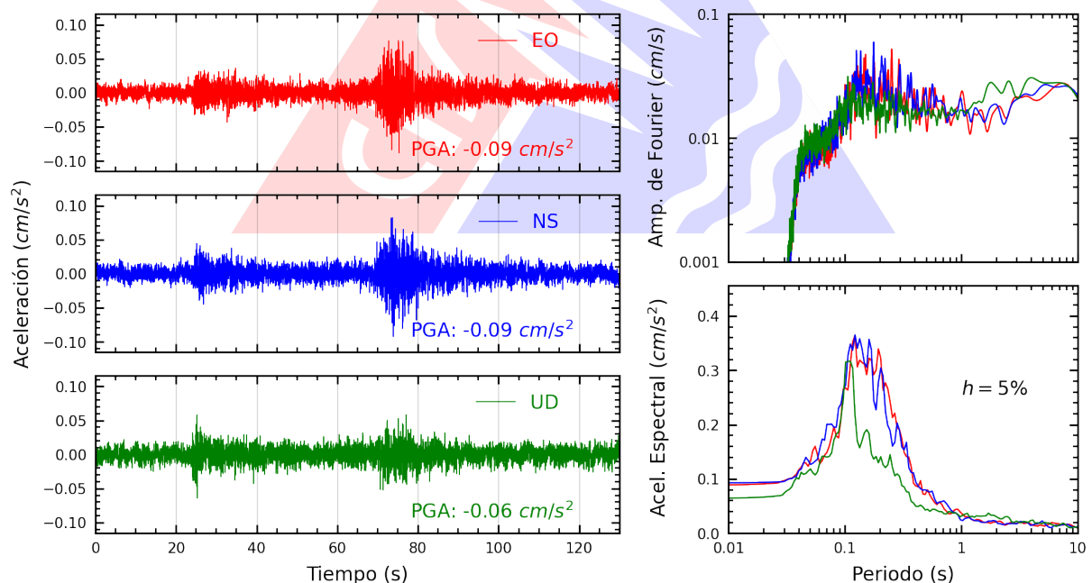
Figura A.2: Registros tiempo-historia, espectros de Fourier y de respuesta en las direcciones EO, NS y vertical de la estación UNTRM. Sismo de Pastaza, Datem del Marañón - Loreto del 2025-02-09, 00:41:59 (Hora local)
