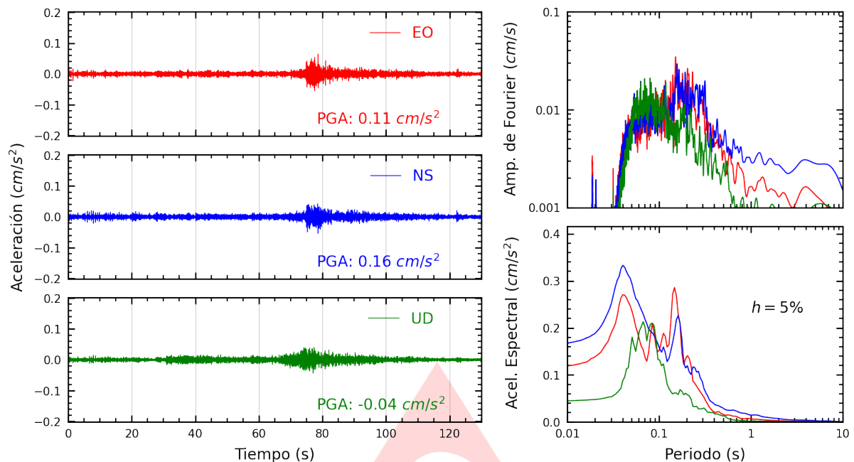
Figura A.1: Registros tiempo-historia, espectros de Fourier y de respuesta en las direcciones EO, NS y vertical de la estación UNAAA. Sismo de Pastaza, Datem del Marañón - Loreto del 2025-02-09, 00:41:59 (Hora local)
