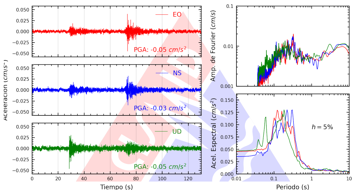
Figura A.3: Registros tiempo-historia, espectros de Fourier y de respuesta en las direcciones EO, NS y vertical de la estación UNJ. Sismo de Pastaza, Datem del Marañón - Loreto del 2025-02-09, 00:41:59 (Hora local)
