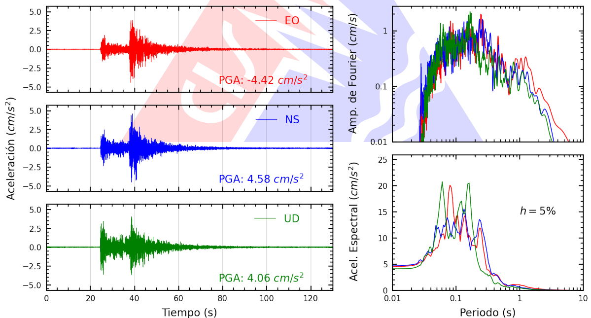
Figura A.2: Registros tiempo-historia, espectros de Fourier y de respuesta en las direcciones EO, NS y vertical de la estación UJBG4. Sismo de Tacna, Tacna - Tacna del 2025-02-10, 21:00:27 (Hora local)
