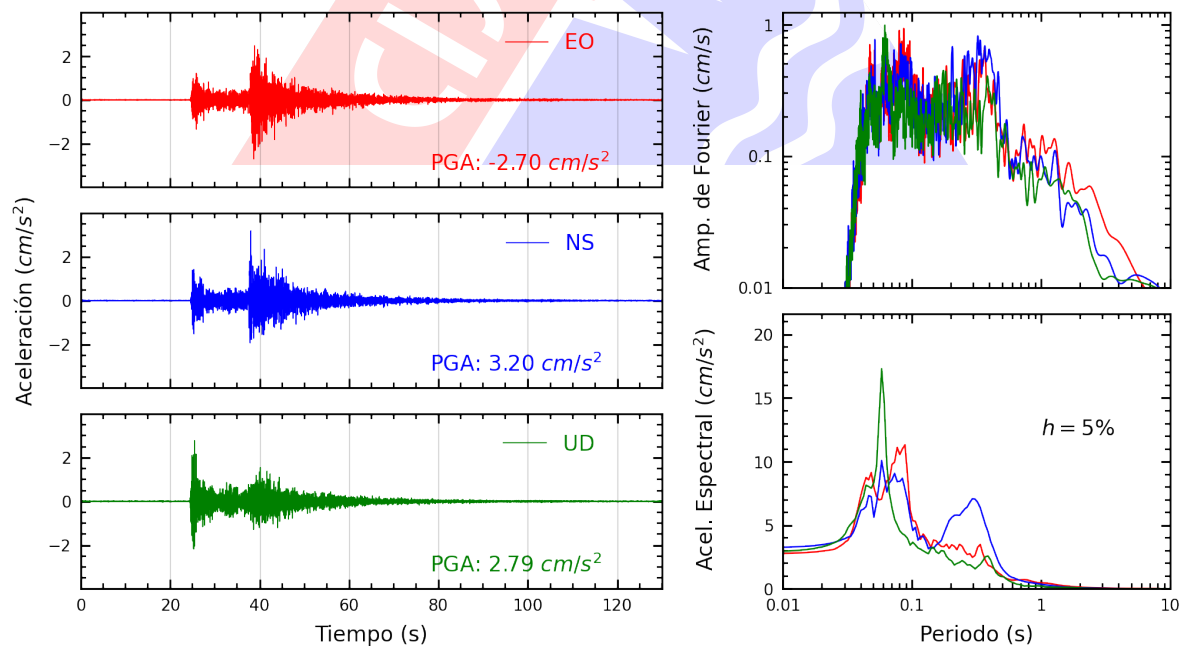
Figura A.4: Registros tiempo-historia, espectros de Fourier y de respuesta en las direcciones EO, NS y vertical de la estación CREY. Sismo de Tacna, Tacna - Tacna del 2025-02-10, 21:00:27 (Hora local)
