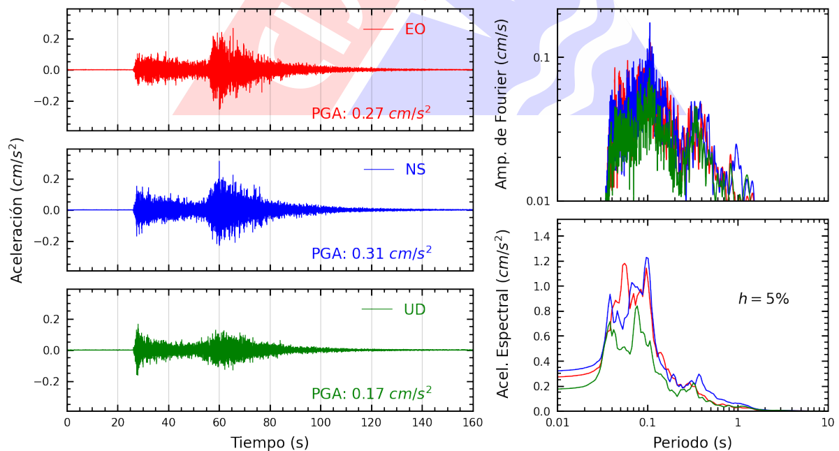
Figura A.6: Registros tiempo-historia, espectros de Fourier y de respuesta en las direcciones EO, NS y vertical de la estación UNSA2. Sismo de Tacna, Tacna - Tacna del 2025-02-10, 21:00:27 (Hora local)
