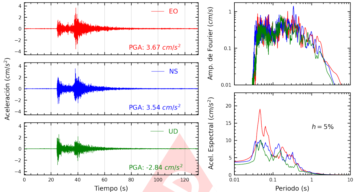
Figura A.3: Registros tiempo-historia, espectros de Fourier y de respuesta en las direcciones EO, NS y vertical de la estación UPTAC. Sismo de Tacna, Tacna - Tacna del 2025-02-10, 21:00:27 (Hora local)
