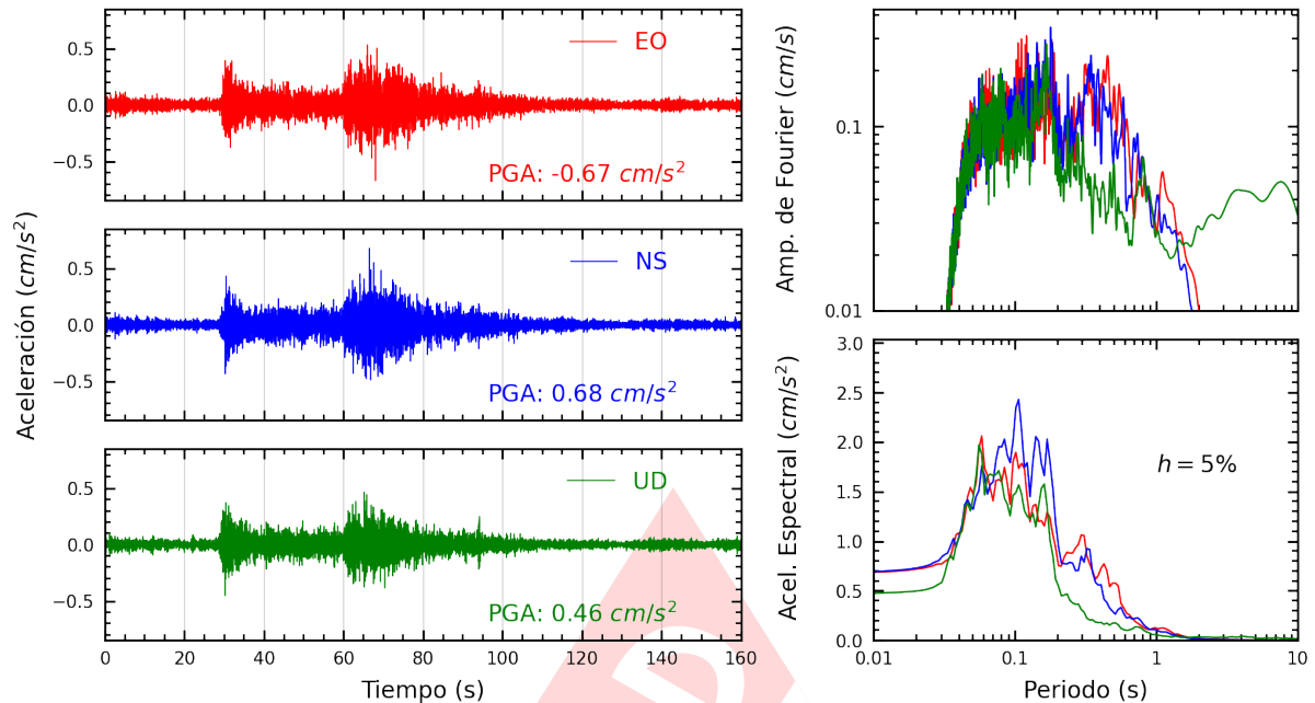
Figura A.5: Registros tiempo-historia, espectros de Fourier y de respuesta en las direcciones EO, NS y vertical de la estación SCARQ. Sismo de Tacna, Tacna - Tacna del 2025-02-10, 21:00:27 (Hora local)
