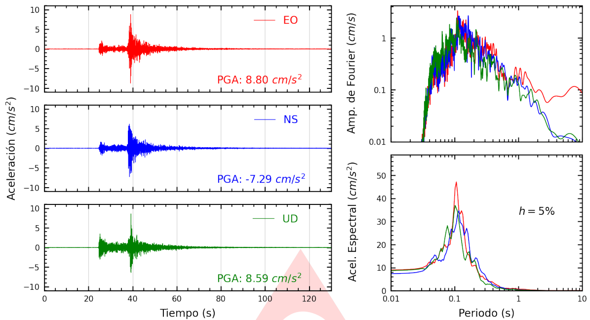
Figura A.1: Registros tiempo-historia, espectros de Fourier y de respuesta en las direcciones EO, NS y vertical de la estación UJBG3. Sismo de Tacna, Tacna - Tacna del 2025-02-10, 21:00:27 (Hora local)
