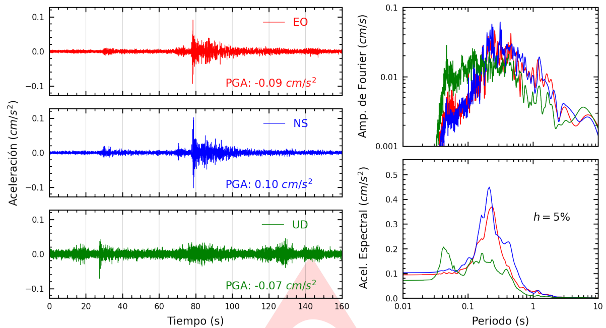
Figura A.1: Registros tiempo-historia, espectros de Fourier y de respuesta en las direcciones EO, NS y vertical de la estación SCPUC. Sismo de Fitzcarrald, Manu - Madre De Dios del 2025-02-11, 22:26:33 (Hora local)
