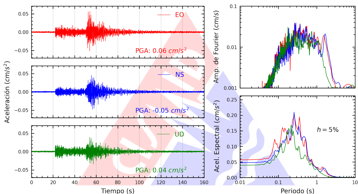
Figura A.3: Registros tiempo-historia, espectros de Fourier y de respuesta en las direcciones EO, NS y vertical de la estación UNCP. Sismo de Fitzcarrald, Manu - Madre De Dios del 2025-02-11, 22:26:33 (Hora local)
