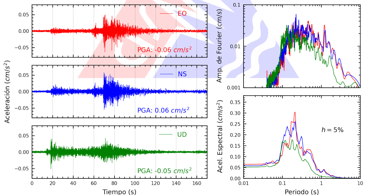
Figura A.2: Registros tiempo-historia, espectros de Fourier y de respuesta en las direcciones EO, NS y vertical de la estación UNIA. Sismo de Fitzcarrald, Manu - Madre De Dios del 2025-02-11, 22:26:33 (Hora local)
