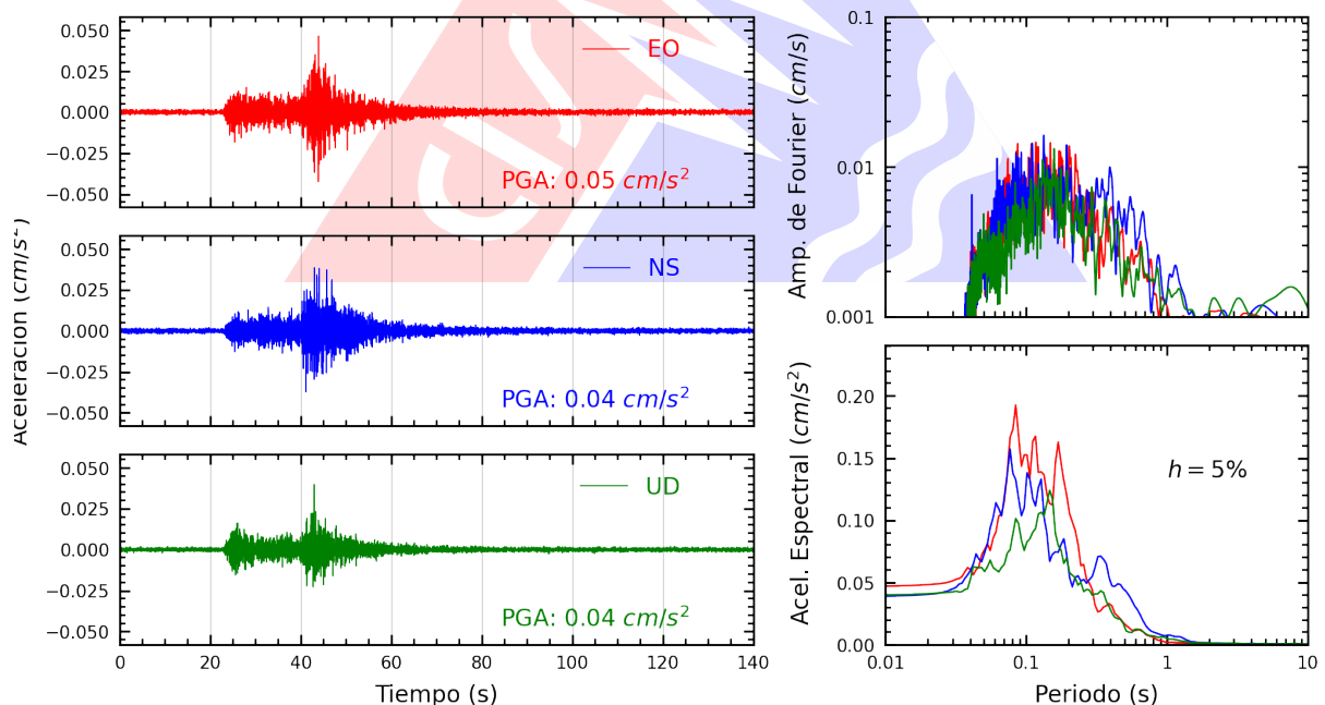
Figura A.2: Registros tiempo-historia, espectros de Fourier y de respuesta en las direcciones EO, NS y vertical de la estación UNSA2. Sismo de Cabanaconde, Caylloma - Arequipa del 2025-02-12, 01:32:08 (Hora local)
