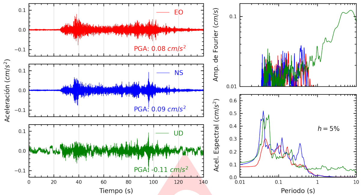
Figura A.1: Registros tiempo-historia, espectros de Fourier y de respuesta en las direcciones EO, NS y vertical de la estación SCARQ. Sismo de Cabanaconde, Caylloma - Arequipa del 2025-02-12, 01:32:08 (Hora local)
