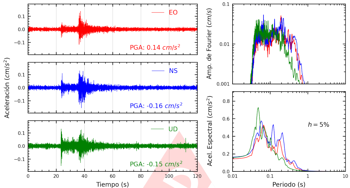
Figura A.5: Registros tiempo-historia, espectros de Fourier y de respuesta en las direcciones EO, NS y vertical de la estación VHAY2. Sismo de Huacho, Huaura - Lima del 2025-02-12, 07:48:24 (Hora local)
