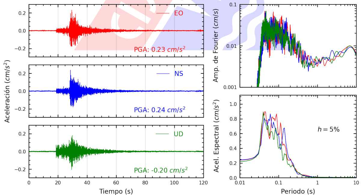
Figura A.4: Registros tiempo-historia, espectros de Fourier y de respuesta en las direcciones EO, NS y vertical de la estación CARAL. Sismo de Huacho, Huaura - Lima del 2025-02-12, 07:48:24 (Hora local)
