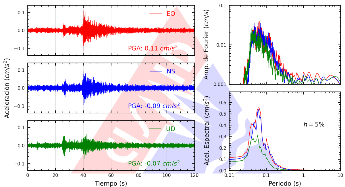
Figura A.7: Registros tiempo-historia, espectros de Fourier y de respuesta en las direcciones EO, NS y vertical de la estación ATARJ. Sismo de Huacho, Huaura - Lima del 2025-02-12, 07:48:24 (Hora local)
