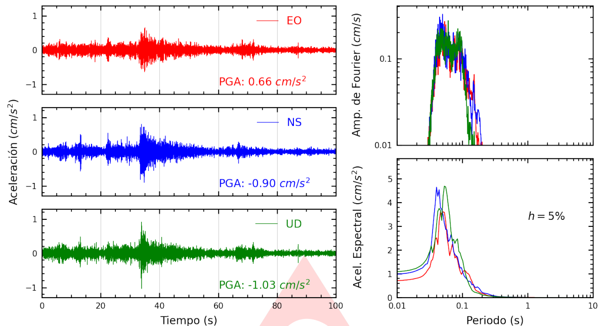
Figura A.1: Registros tiempo-historia, espectros de Fourier y de respuesta en las direcciones EO, NS y vertical de la estación SROS2. Sismo de Huacho, Huaura - Lima del 2025-02-12, 07:48:24 (Hora local)
