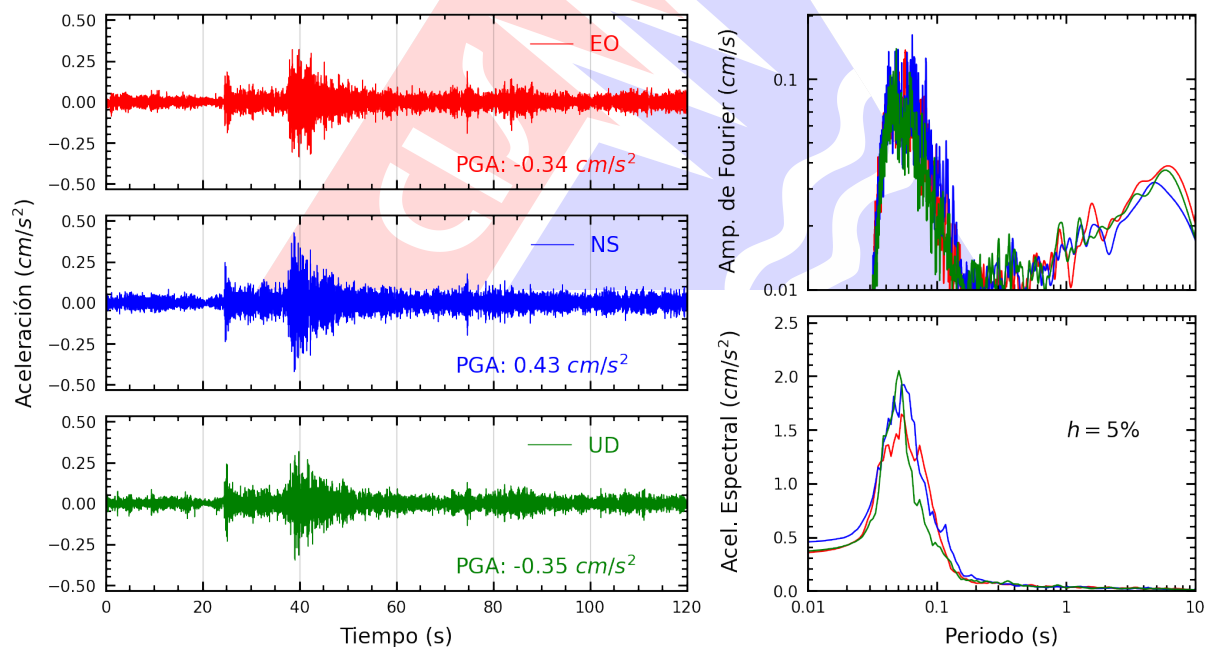
Figura A.2: Registros tiempo-historia, espectros de Fourier y de respuesta en las direcciones EO, NS y vertical de la estación JOSEO. Sismo de Huacho, Huaura - Lima del 2025-02-12, 07:48:24 (Hora local)
