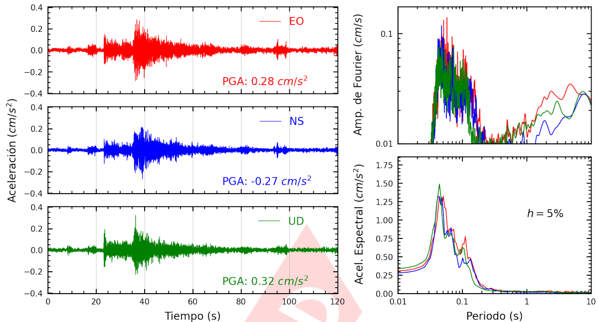
Figura A.3: Registros tiempo-historia, espectros de Fourier y de respuesta en las direcciones EO, NS y vertical de la estación AMORE. Sismo de Huacho, Huaura - Lima del 2025-02-12, 07:48:24 (Hora local)
