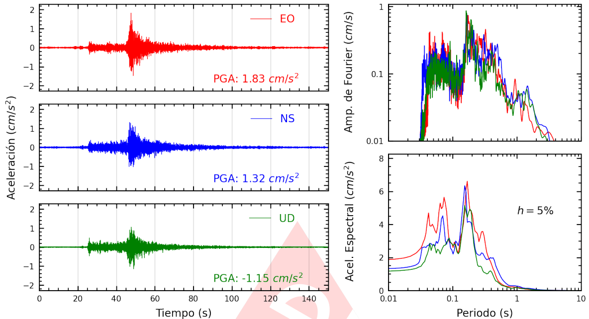
Figura A.3: Registros tiempo-historia, espectros de Fourier y de respuesta en las direcciones EO, NS y vertical de la estación UPTAC. Sismo de Tacna, Tacna - Tacna del 2025-02-16, 16:00:56 (Hora local)
