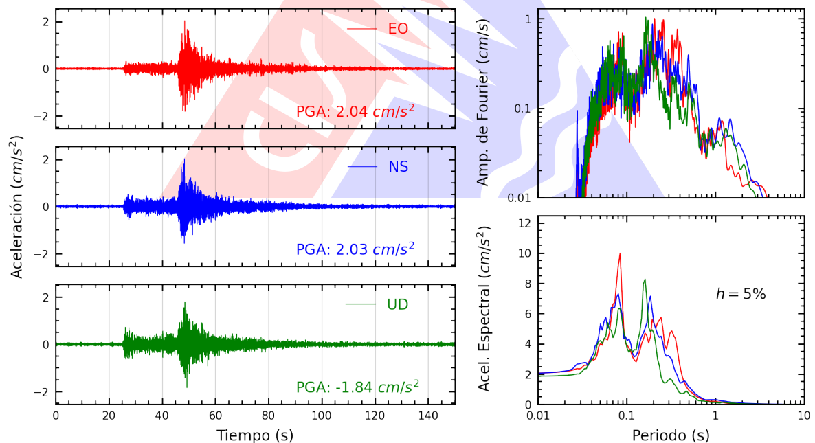
Figura A.2: Registros tiempo-historia, espectros de Fourier y de respuesta en las direcciones EO, NS y vertical de la estación UJBG4. Sismo de Tacna, Tacna - Tacna del 2025-02-16, 16:00:56 (Hora local)
