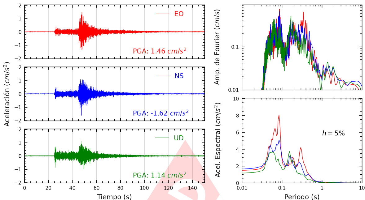
Figura A.5: Registros tiempo-historia, espectros de Fourier y de respuesta en las direcciones EO, NS y vertical de la estación CREY. Sismo de Tacna, Tacna - Tacna del 2025-02-16, 16:00:56 (Hora local)
