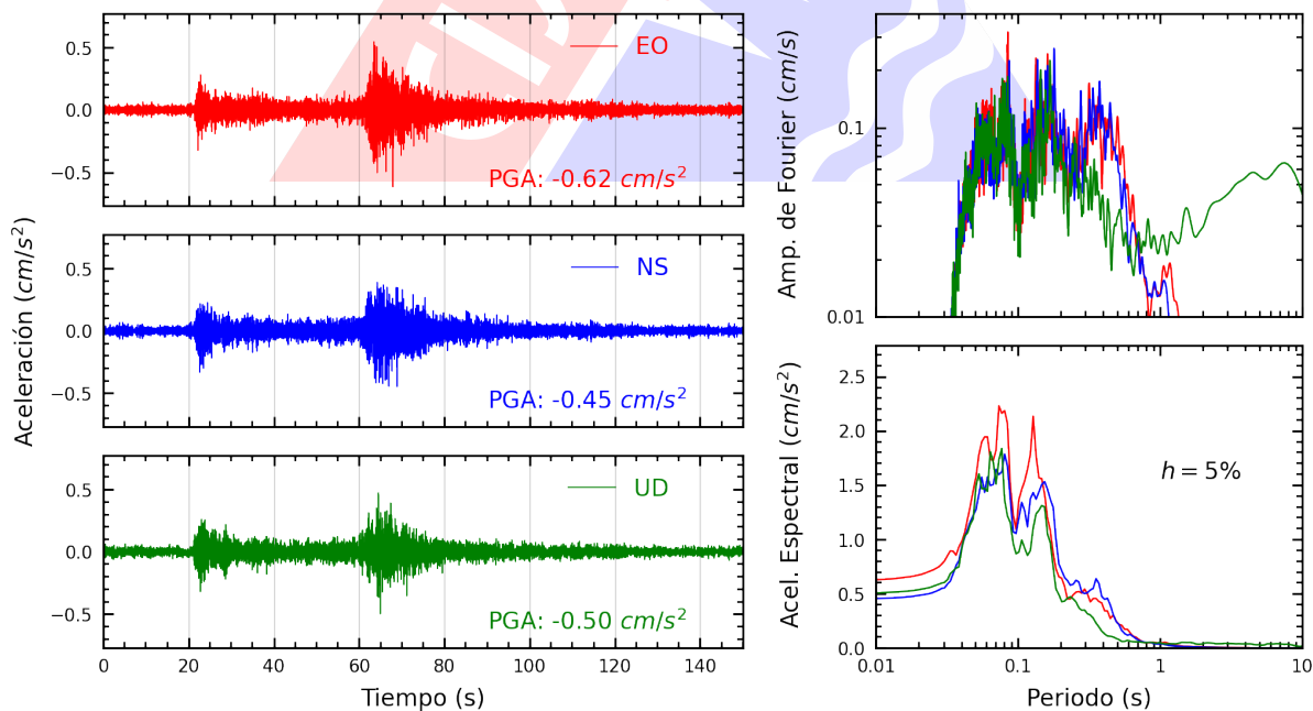
Figura A.6: Registros tiempo-historia, espectros de Fourier y de respuesta en las direcciones EO, NS y vertical de la estación SCARQ. Sismo de Tacna, Tacna - Tacna del 2025-02-16, 16:00:56 (Hora local)
