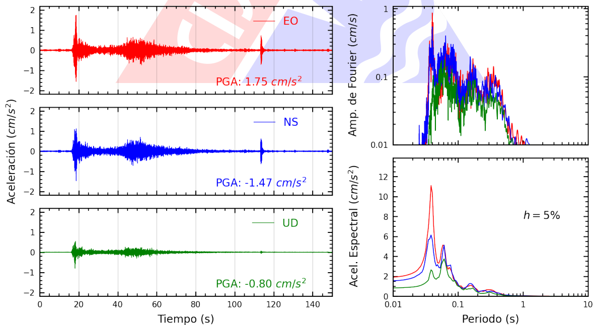
Figura A.4: Registros tiempo-historia, espectros de Fourier y de respuesta en las direcciones EO, NS y vertical de la estación UNAM. Sismo de Tacna, Tacna - Tacna del 2025-02-16, 16:00:56 (Hora local)
