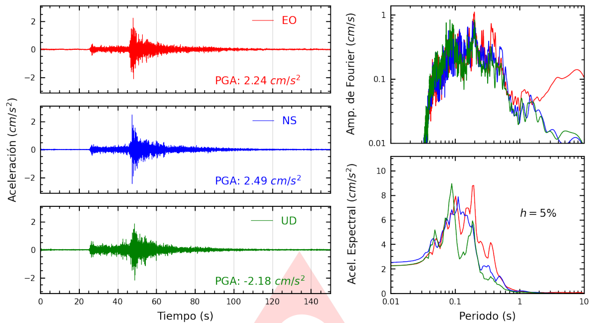
Figura A.1: Registros tiempo-historia, espectros de Fourier y de respuesta en las direcciones EO, NS y vertical de la estación UJBG3. Sismo de Tacna, Tacna - Tacna del 2025-02-16, 16:00:56 (Hora local)
