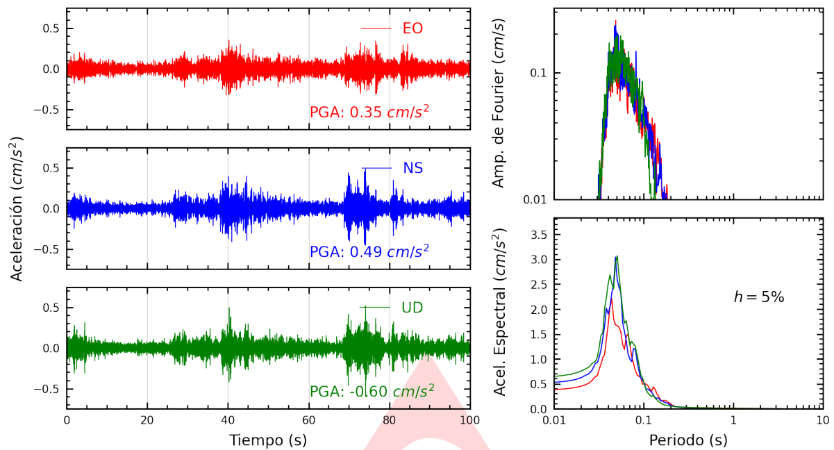
Figura A.1: Registros tiempo-historia, espectros de Fourier y de respuesta en las direcciones EO, NS y vertical de la estación SROS2. Sismo de Huacho, Huaura - Lima del 2025-02-16, 21:13:18 (Hora local)
