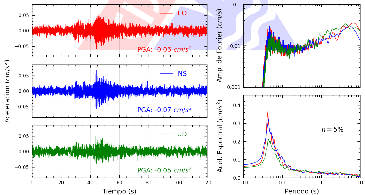
Figura A.4: Registros tiempo-historia, espectros de Fourier y de respuesta en las direcciones EO, NS y vertical de la estación UCSS. Sismo de Huacho, Huaura - Lima del 2025-02-16, 21:13:18 (Hora local)
