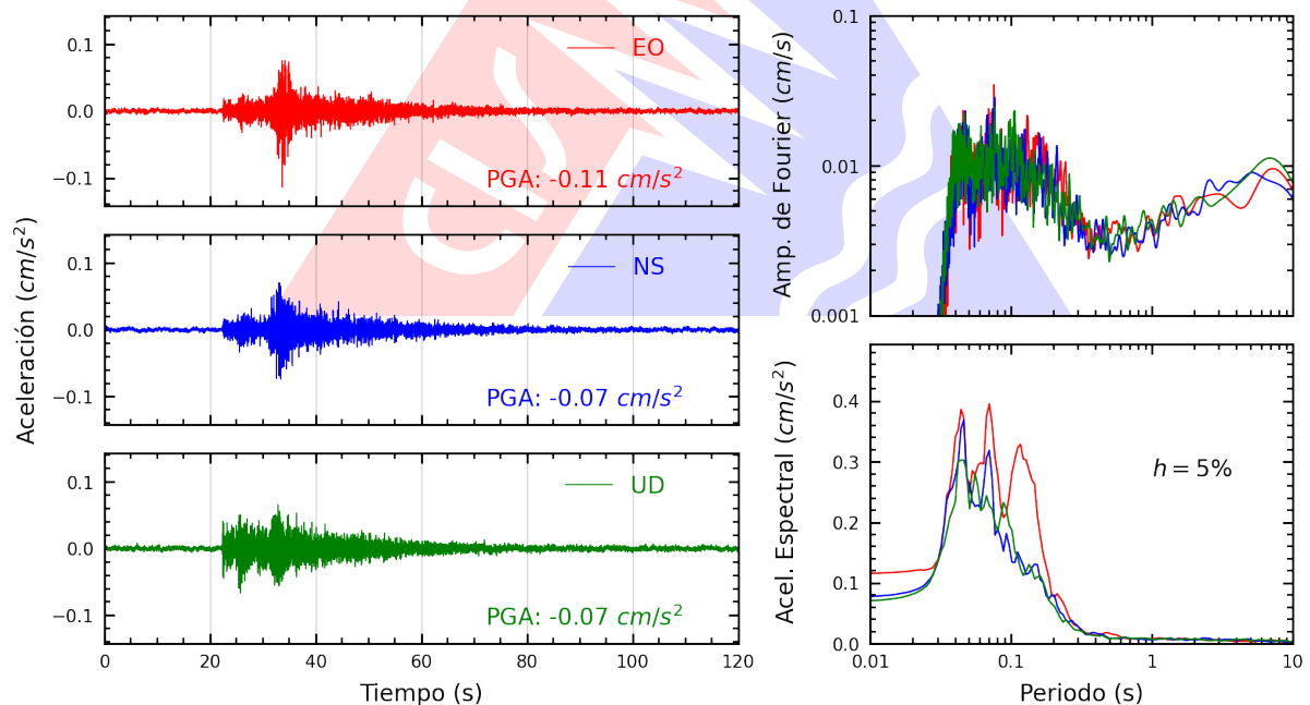
Figura A.2: Registros tiempo-historia, espectros de Fourier y de respuesta en las direcciones EO, NS y vertical de la estación CARAL. Sismo de Huacho, Huaura - Lima del 2025-02-16, 21:13:18 (Hora local)
