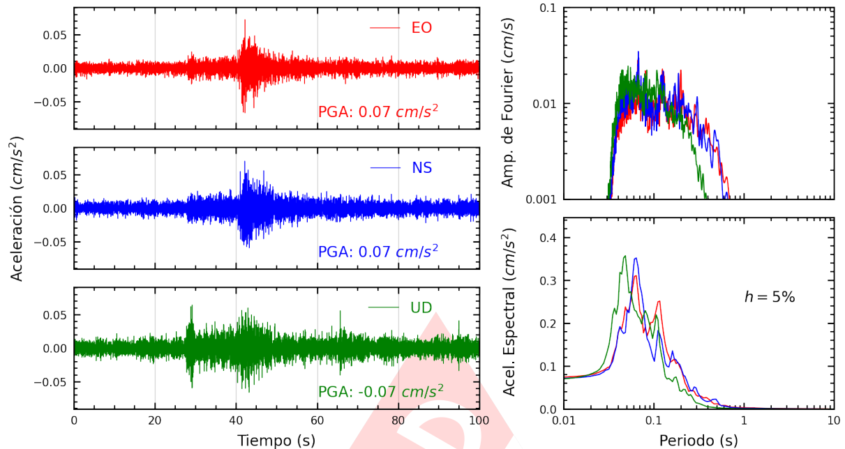
Figura A.3: Registros tiempo-historia, espectros de Fourier y de respuesta en las direcciones EO, NS y vertical de la estación VHAY2. Sismo de Huacho, Huaura - Lima del 2025-02-16, 21:13:18 (Hora local)
