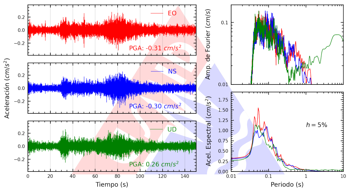
Figura A.7: Registros tiempo-historia, espectros de Fourier y de respuesta en las direcciones EO, NS y vertical de la estación SCARQ. Sismo de Ilave, El Collao - Puno del 2025-02-17, 11:34:09 (Hora local)
