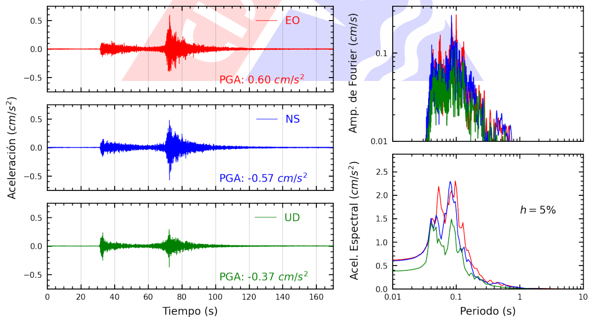
Figura A.4: Registros tiempo-historia, espectros de Fourier y de respuesta en las direcciones EO, NS y vertical de la estación UNSA2. Sismo de Ilave, El Collao - Puno del 2025-02-17, 11:34:09 (Hora local)
