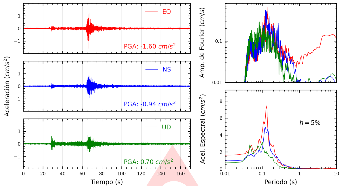
Figura A.1: Registros tiempo-historia, espectros de Fourier y de respuesta en las direcciones EO, NS y vertical de la estación UJBG3. Sismo de Ilave, El Collao - Puno del 2025-02-17, 11:34:09 (Hora local)
