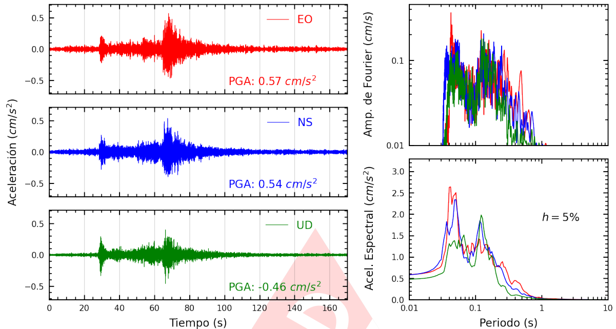
Figura A.5: Registros tiempo-historia, espectros de Fourier y de respuesta en las direcciones EO, NS y vertical de la estación UPTAC. Sismo de Ilave, El Collao - Puno del 2025-02-17, 11:34:09 (Hora local)
