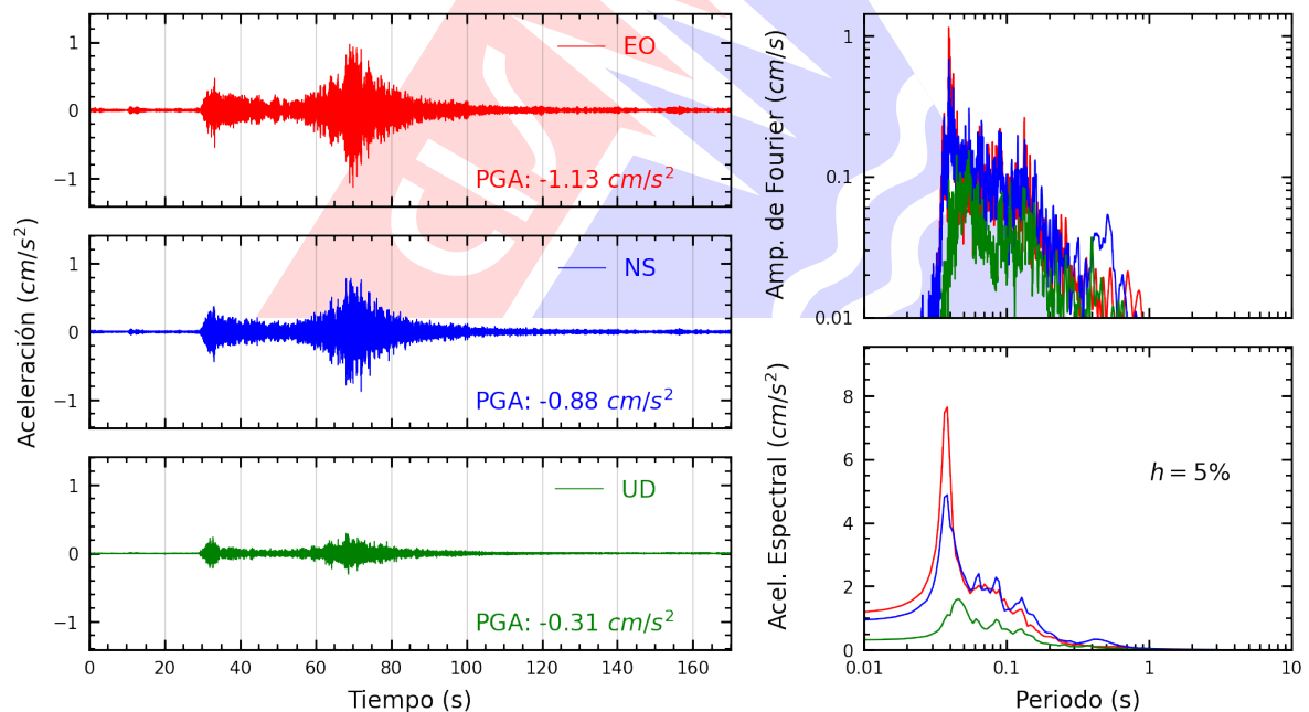
Figura A.2: Registros tiempo-historia, espectros de Fourier y de respuesta en las direcciones EO, NS y vertical de la estación UNAM. Sismo de Ilave, El Collao - Puno del 2025-02-17, 11:34:09 (Hora local)
