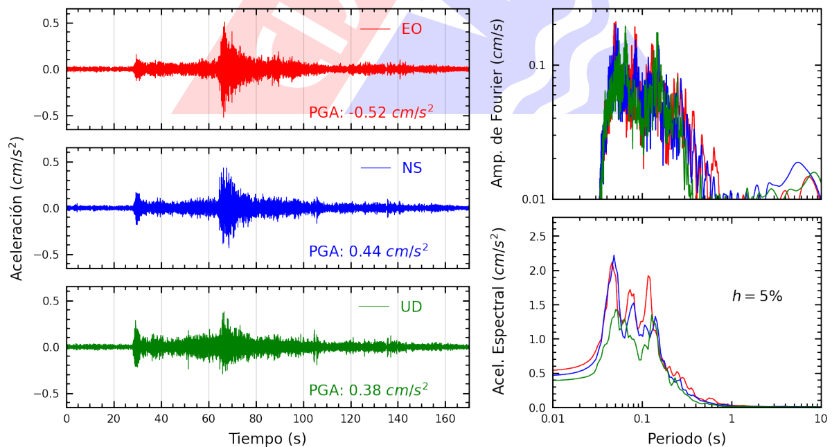
Figura A.6: Registros tiempo-historia, espectros de Fourier y de respuesta en las direcciones EO, NS y vertical de la estación CREY. Sismo de Ilave, El Collao - Puno del 2025-02-17, 11:34:09 (Hora local)
