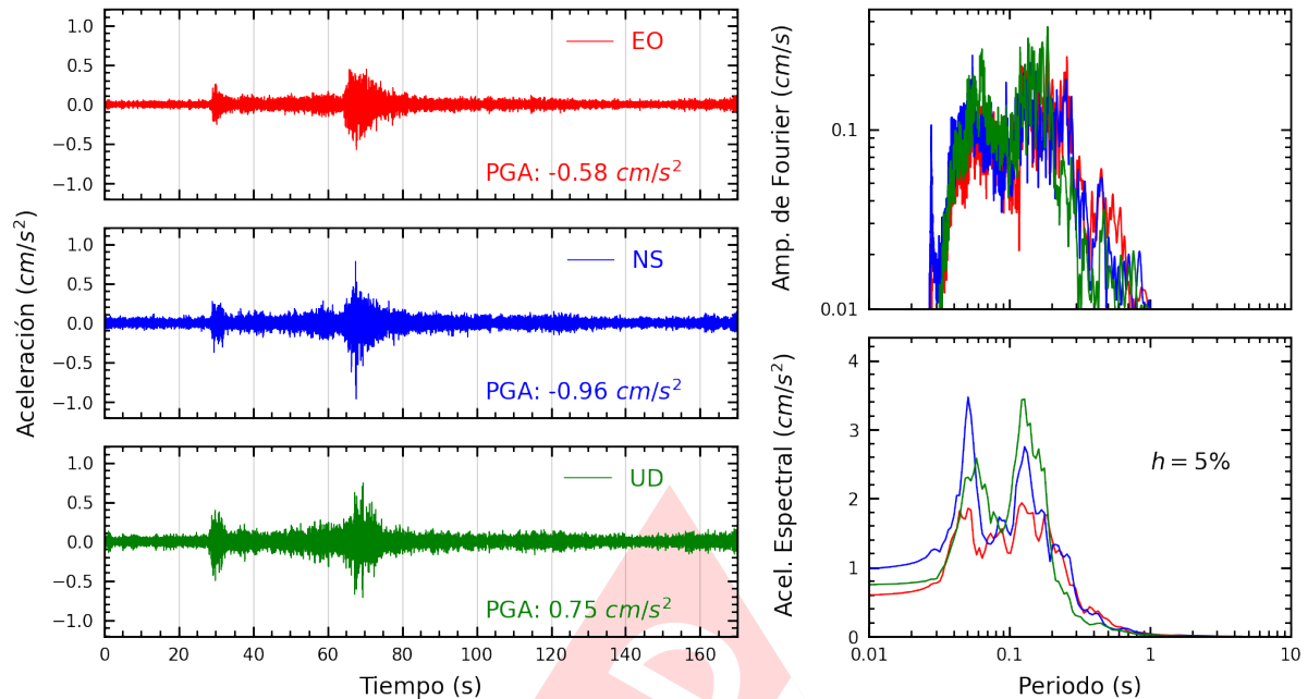
Figura A.3: Registros tiempo-historia, espectros de Fourier y de respuesta en las direcciones EO, NS y vertical de la estación UJBG4. Sismo de Ilave, El Collao - Puno del 2025-02-17, 11:34:09 (Hora local)
