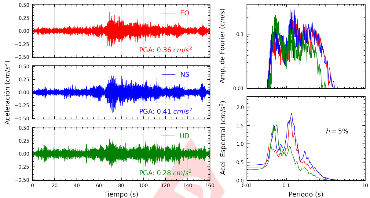
Figura A.7: Registros tiempo-historia, espectros de Fourier y de respuesta en las direcciones EO, NS y vertical de la estación SCAR2. Sismo de Tacna, Tacna - Tacna del 2025-02-20, 01:22:05 (Hora local)
