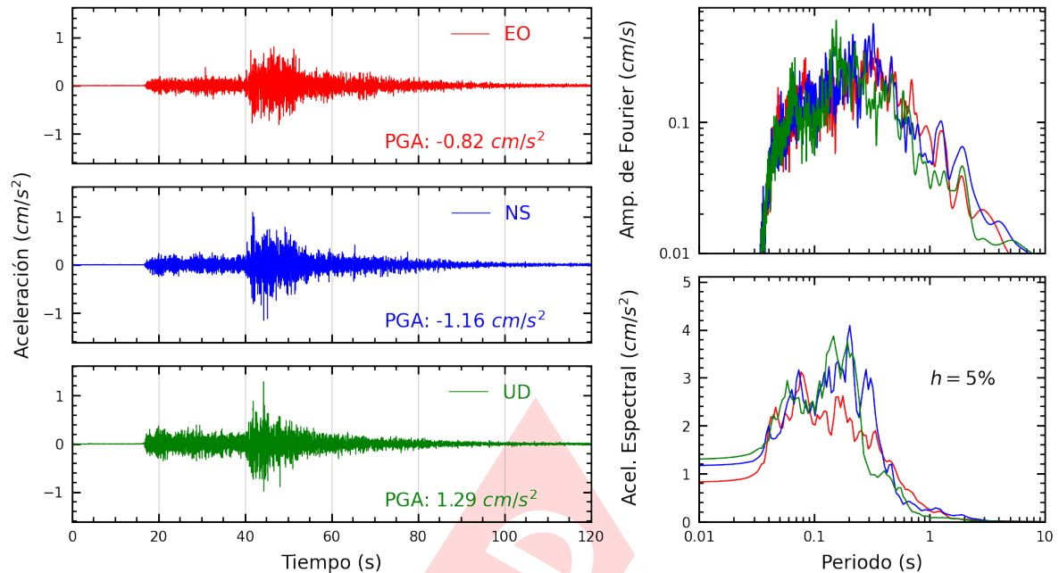
Figura A.3: Registros tiempo-historia, espectros de Fourier y de respuesta en las direcciones EO, NS y vertical de la estación CREY. Sismo de Tacna, Tacna - Tacna del 2025-02-20, 01:22:05 (Hora local)
