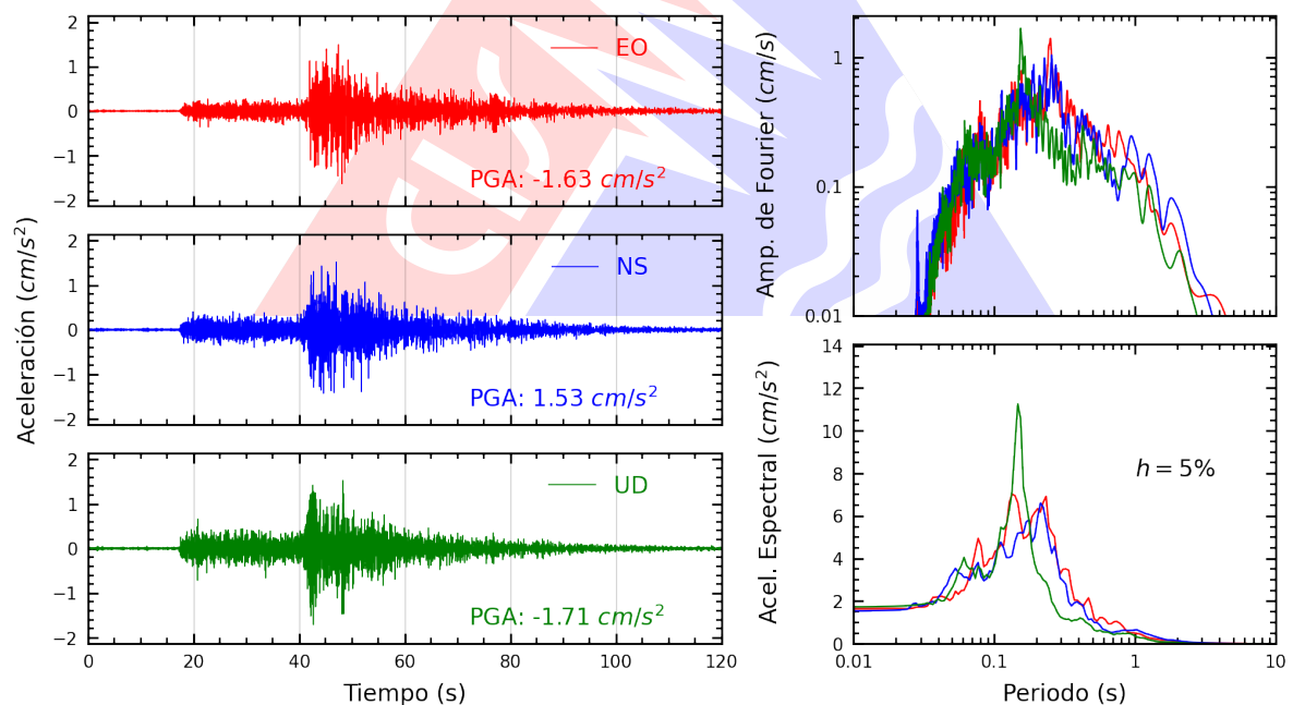
Figura A.2: Registros tiempo-historia, espectros de Fourier y de respuesta en las direcciones EO, NS y vertical de la estación UJBG4. Sismo de Tacna, Tacna - Tacna del 2025-02-20, 01:22:05 (Hora local)
