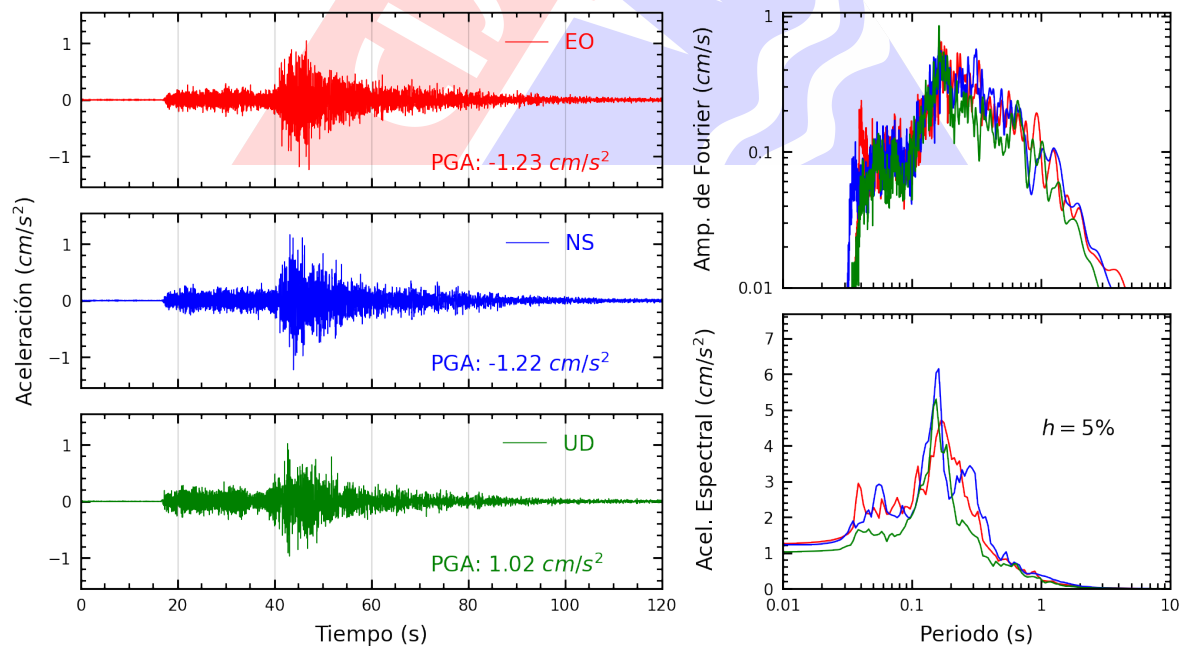
Figura A.4: Registros tiempo-historia, espectros de Fourier y de respuesta en las direcciones EO, NS y vertical de la estación UPTAC. Sismo de Tacna, Tacna - Tacna del 2025-02-20, 01:22:05 (Hora local)
