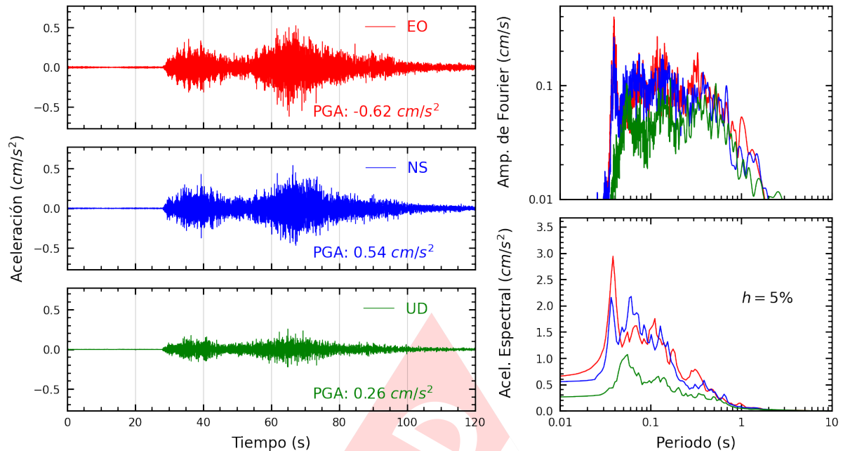
Figura A.5: Registros tiempo-historia, espectros de Fourier y de respuesta en las direcciones EO, NS y vertical de la estación UNAM. Sismo de Tacna, Tacna - Tacna del 2025-02-20, 01:22:05 (Hora local)
