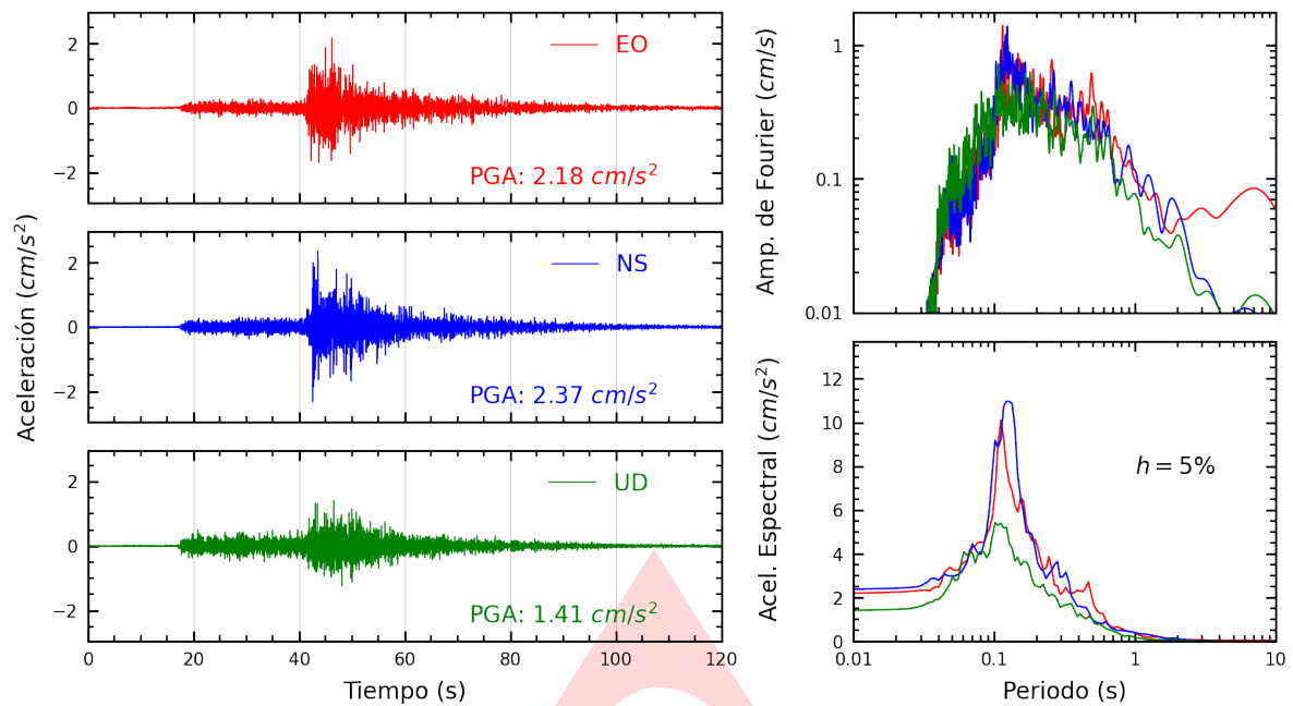
Figura A.1: Registros tiempo-historia, espectros de Fourier y de respuesta en las direcciones EO, NS y vertical de la estación UJBG3. Sismo de Tacna, Tacna - Tacna del 2025-02-20, 01:22:05 (Hora local)
