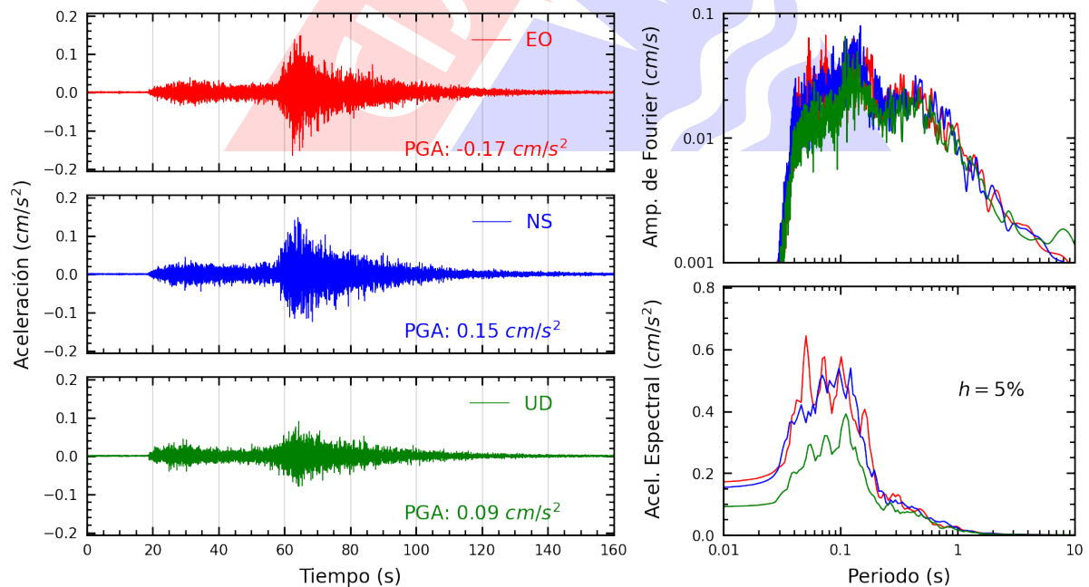
Figura A.8: Registros tiempo-historia, espectros de Fourier y de respuesta en las direcciones EO, NS y vertical de la estación UNSA2. Sismo de Tacna, Tacna - Tacna del 2025-02-20, 01:22:05 (Hora local)
