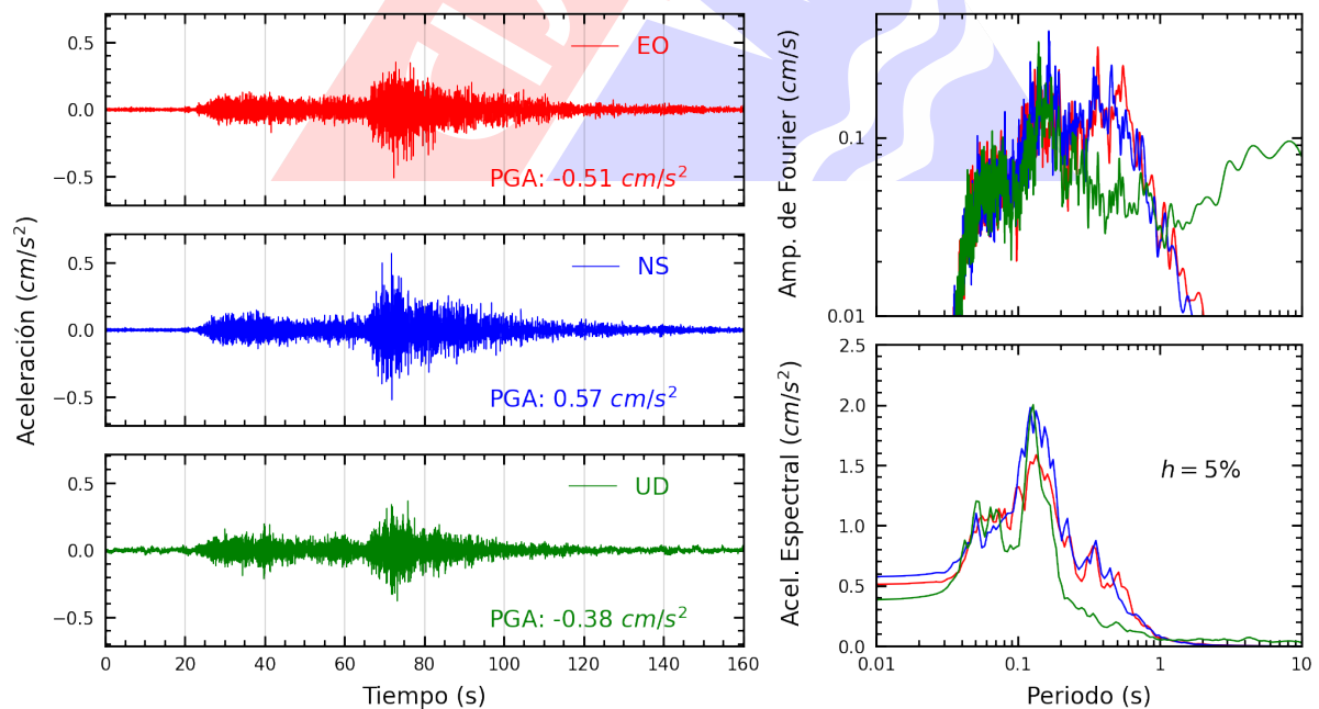
Figura A.6: Registros tiempo-historia, espectros de Fourier y de respuesta en las direcciones EO, NS y vertical de la estación SCARQ. Sismo de Tacna, Tacna - Tacna del 2025-02-20, 01:22:05 (Hora local)
