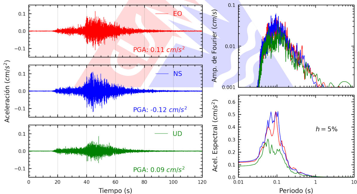
Figura A.2: Registros tiempo-historia, espectros de Fourier y de respuesta en las direcciones EO, NS y vertical de la estación UNSA2. Sismo de Atico, Caraveli - Arequipa del 2025-02-20, 03:51:07 (Hora local)
