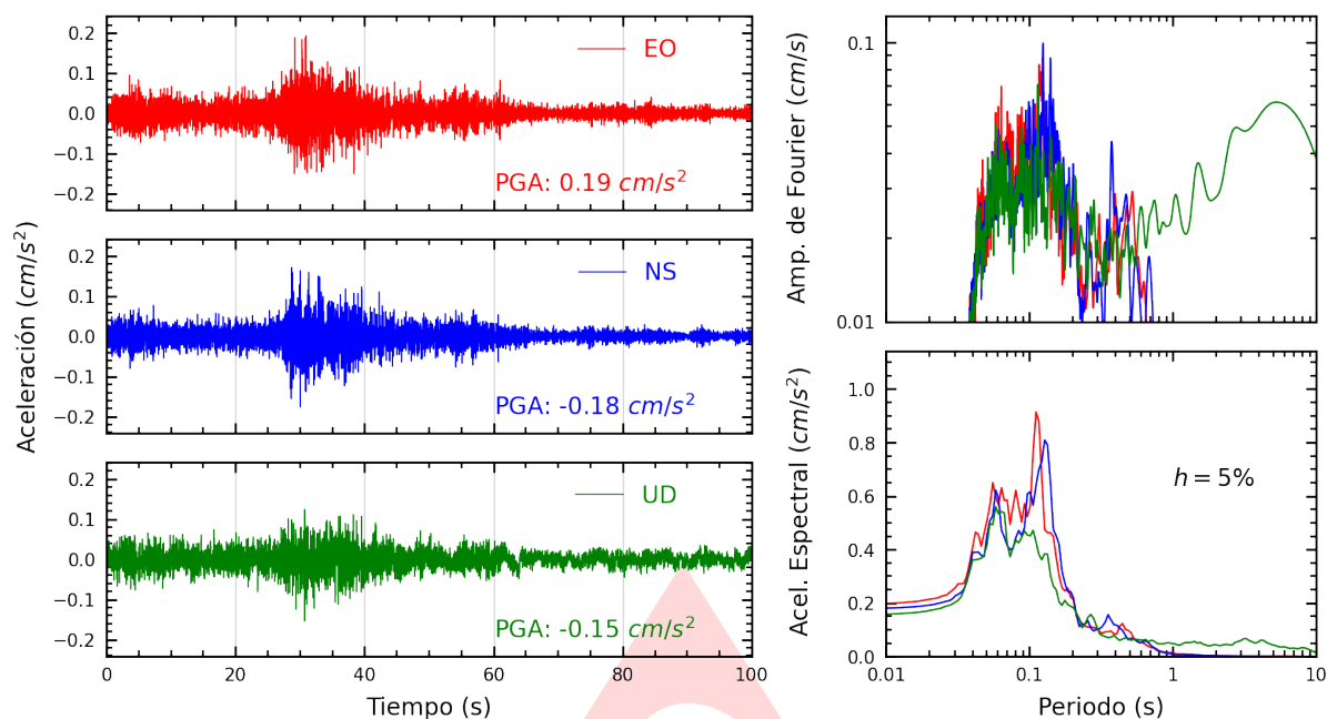
Figura A.1: Registros tiempo-historia, espectros de Fourier y de respuesta en las direcciones EO, NS y vertical de la estación SCARQ. Sismo de Atico, Caraveli - Arequipa del 2025-02-20, 03:51:07 (Hora local)
