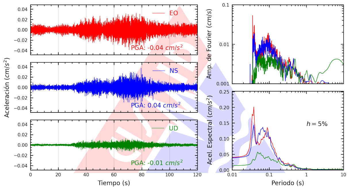
Figura A.3: Registros tiempo-historia, espectros de Fourier y de respuesta en las direcciones EO, NS y vertical de la estación UNAM. Sismo de Atico, Caraveli - Arequipa del 2025-02-20, 03:51:07 (Hora local)
