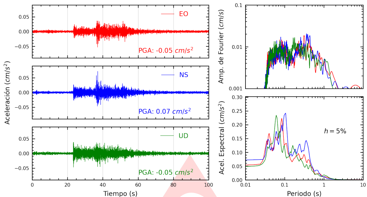
Figura A.1: Registros tiempo-historia, espectros de Fourier y de respuesta en las direcciones EO, NS y vertical de la estación UNCP. Sismo de Satipo, Satipo - Junin del 2025-02-25, 08:00:46 (Hora local)
