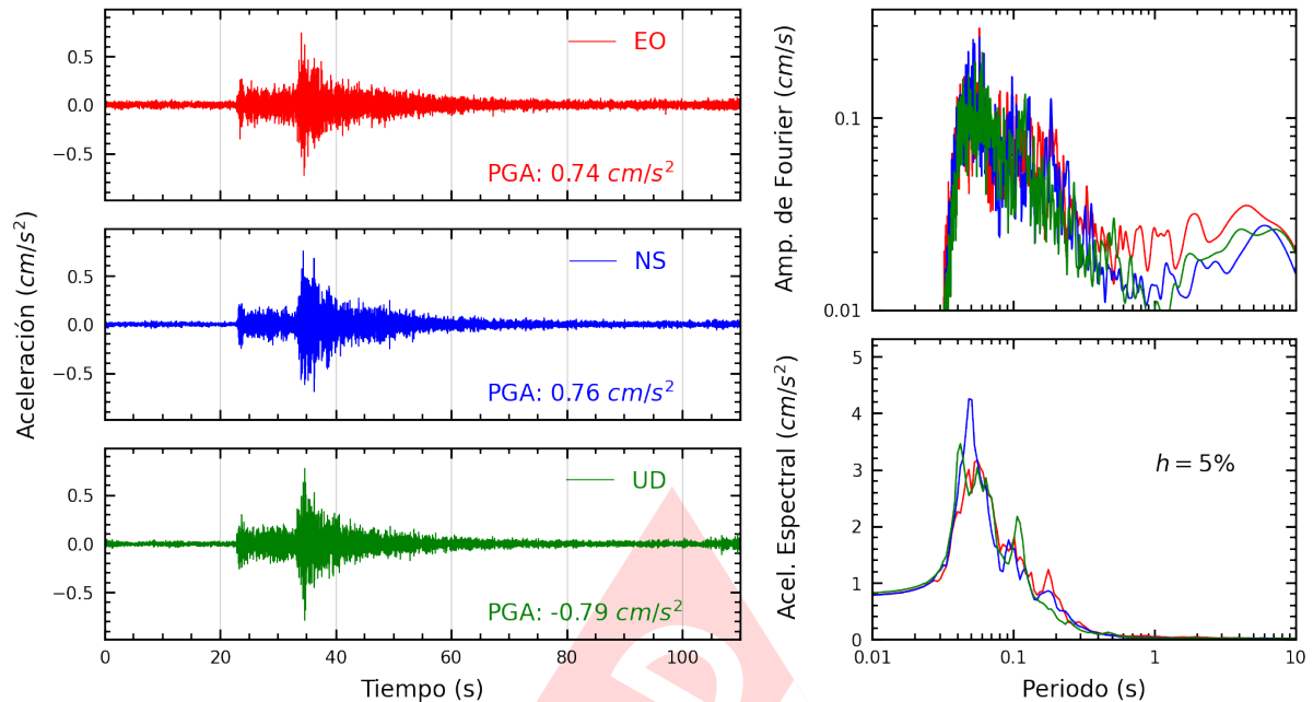
Figura A.31: Registros tiempo-historia, espectros de Fourier y de respuesta en las direcciones EO, NS y vertical de la estación IMCA. Sismo de Ancon, Lima - Lima del 2025-02-26, 23:48:47 (Hora local)
