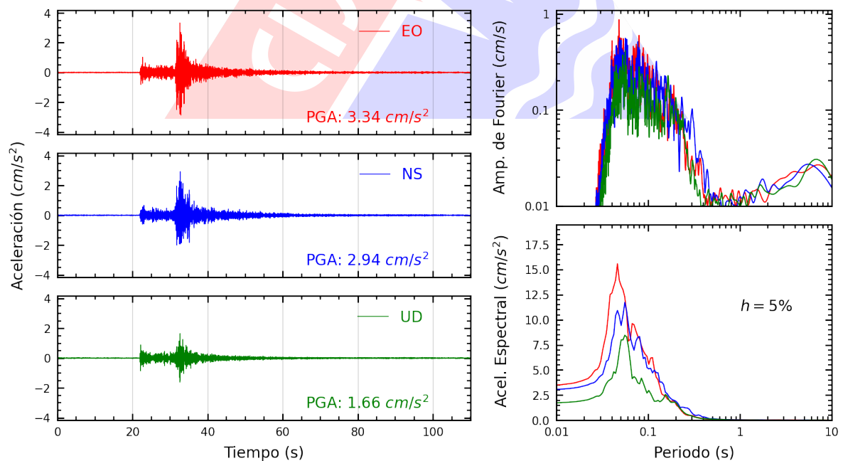
Figura A.8: Registros tiempo-historia, espectros de Fourier y de respuesta en las direcciones EO, NS y vertical de la estación FICPE. Sismo de Ancon, Lima - Lima del 2025-02-26, 23:48:47 (Hora local)
