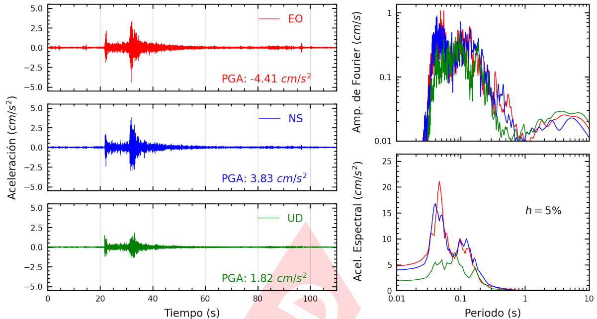
Figura A.5: Registros tiempo-historia, espectros de Fourier y de respuesta en las direcciones EO, NS y vertical de la estación OLIVO. Sismo de Ancon, Lima - Lima del 2025-02-26, 23:48:47 (Hora local)
