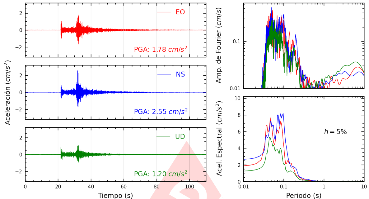
Figura A.11: Registros tiempo-historia, espectros de Fourier y de respuesta en las direcciones EO, NS y vertical de la estación UCSS. Sismo de Ancon, Lima - Lima del 2025-02-26, 23:48:47 (Hora local)
