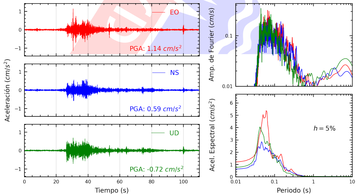
Figura A.22: Registros tiempo-historia, espectros de Fourier y de respuesta en las direcciones EO, NS y vertical de la estación PRADO. Sismo de Ancon, Lima - Lima del 2025-02-26, 23:48:47 (Hora local)
