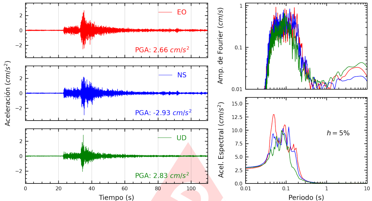
Figura A.9: Registros tiempo-historia, espectros de Fourier y de respuesta en las direcciones EO, NS y vertical de la estación USILM. Sismo de Ancon, Lima - Lima del 2025-02-26, 23:48:47 (Hora local)
