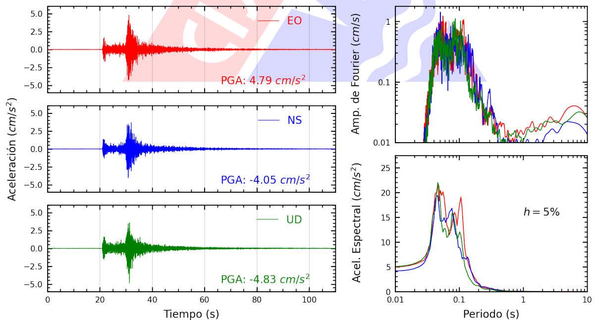
Figura A.4: Registros tiempo-historia, espectros de Fourier y de respuesta en las direcciones EO, NS y vertical de la estación AMORE. Sismo de Ancon, Lima - Lima del 2025-02-26, 23:48:47 (Hora local)
