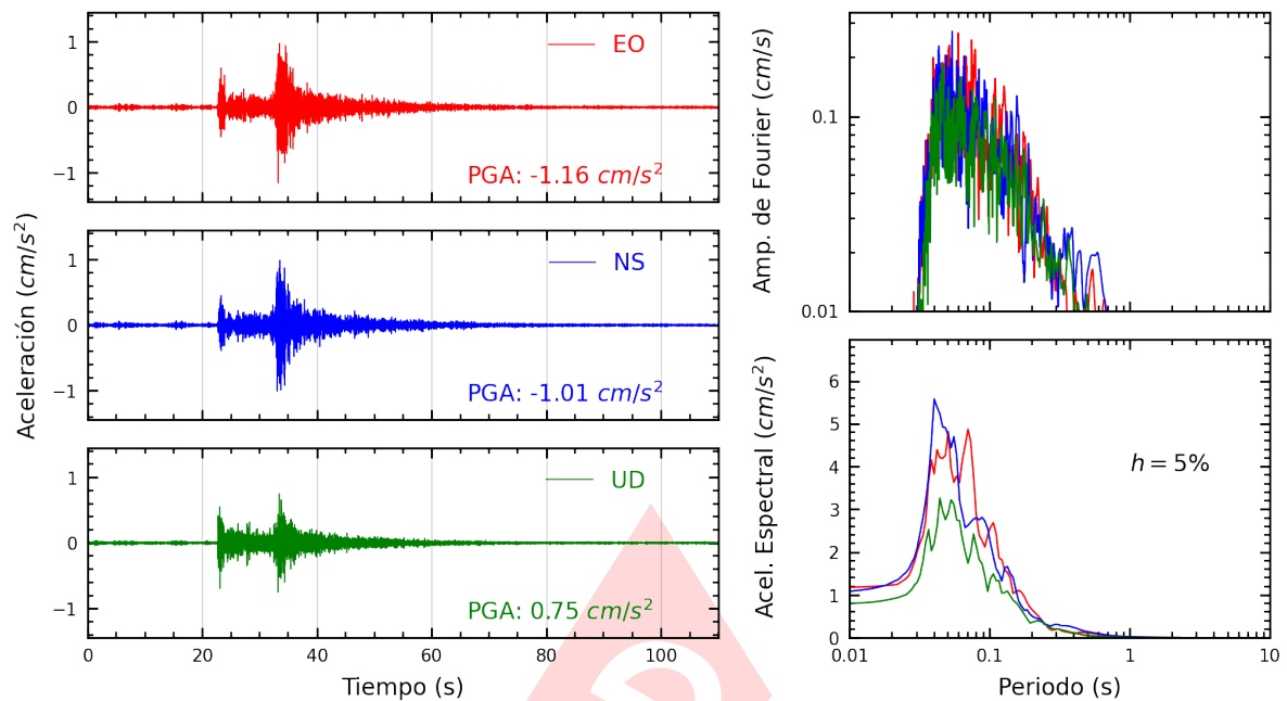
Figura A.21: Registros tiempo-historia, espectros de Fourier y de respuesta en las direcciones EO, NS y vertical de la estación BORJA. Sismo de Ancon, Lima - Lima del 2025-02-26, 23:48:47 (Hora local)
