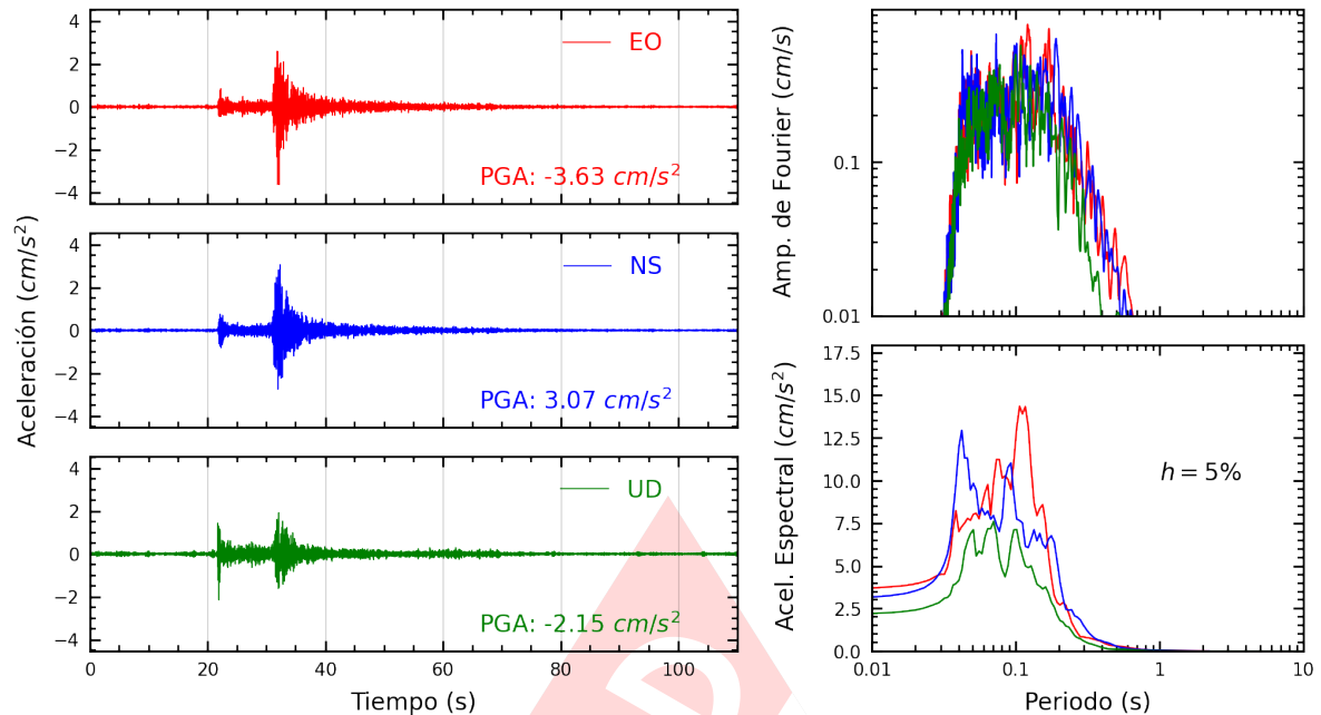
Figura A.7: Registros tiempo-historia, espectros de Fourier y de respuesta en las direcciones EO, NS y vertical de la estación SCOLI. Sismo de Ancon, Lima - Lima del 2025-02-26, 23:48:47 (Hora local)
