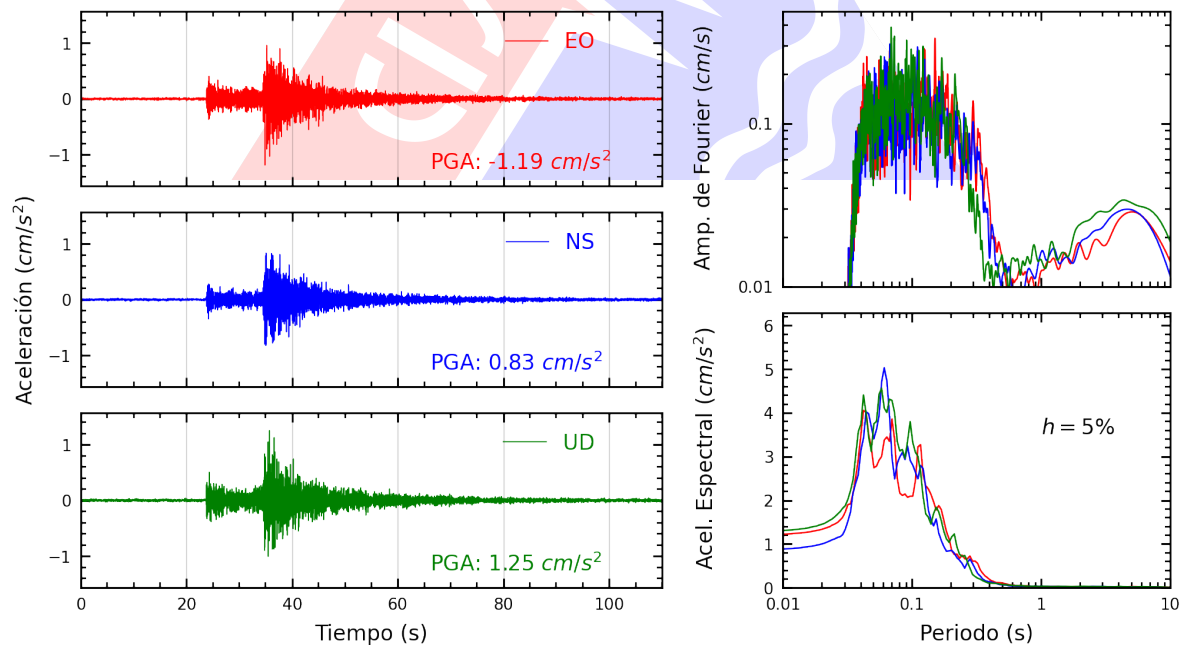
Figura A.20: Registros tiempo-historia, espectros de Fourier y de respuesta en las direcciones EO, NS y vertical de la estación SOVES. Sismo de Ancon, Lima - Lima del 2025-02-26, 23:48:47 (Hora local)
