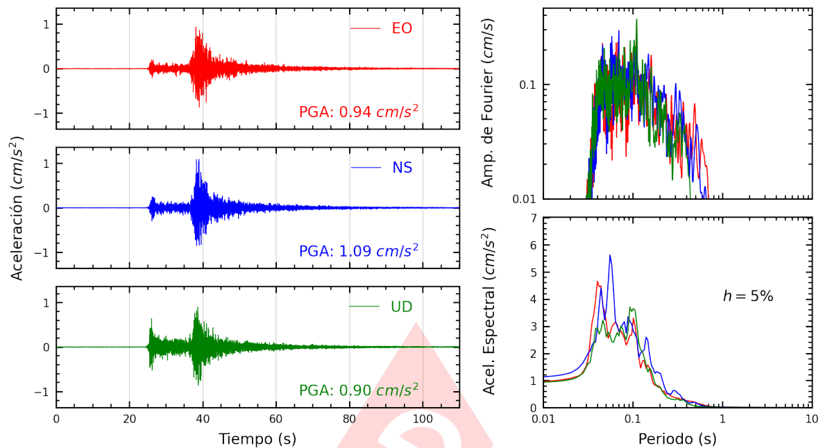
Figura A.23: Registros tiempo-historia, espectros de Fourier y de respuesta en las direcciones EO, NS y vertical de la estación CARAL. Sismo de Ancon, Lima - Lima del 2025-02-26, 23:48:47 (Hora local)
