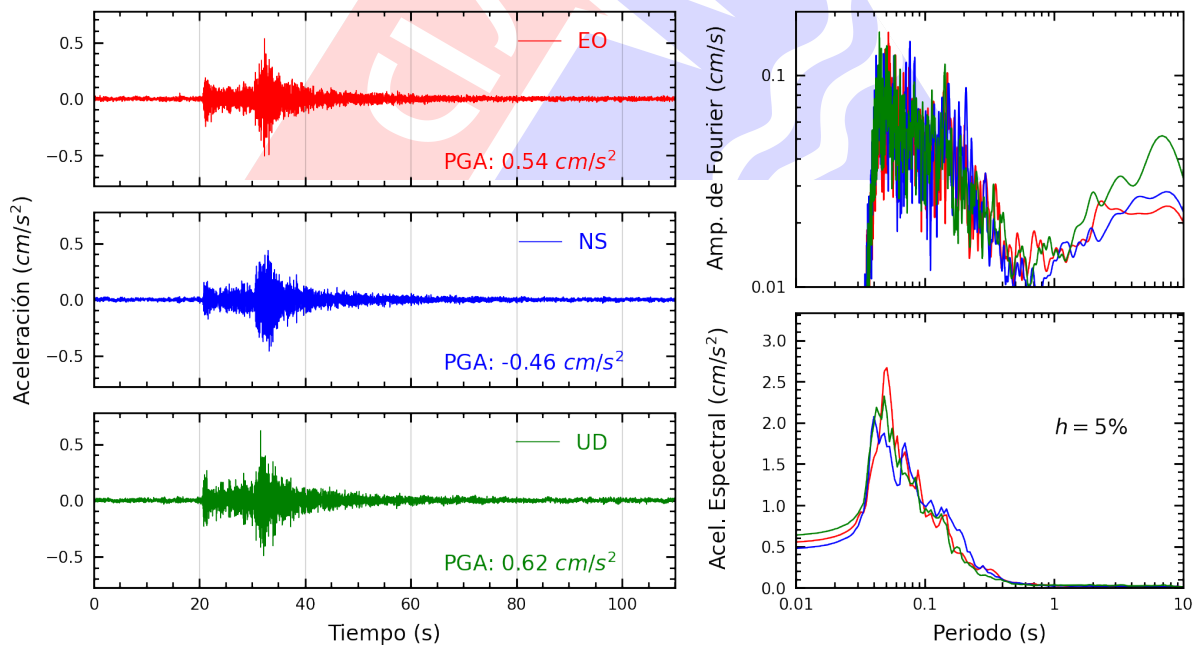
Figura A.34: Registros tiempo-historia, espectros de Fourier y de respuesta en las direcciones EO, NS y vertical de la estación UNMSM. Sismo de Ancon, Lima - Lima del 2025-02-26, 23:48:47 (Hora local)
