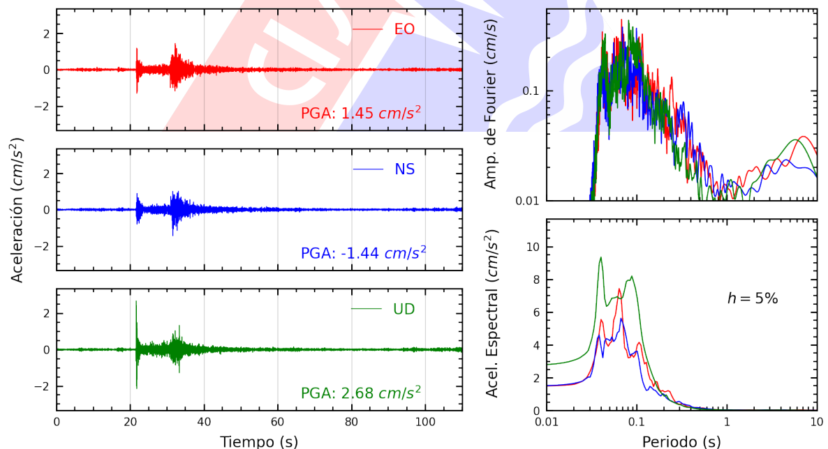
Figura A.10: Registros tiempo-historia, espectros de Fourier y de respuesta en las direcciones EO, NS y vertical de la estación MADRE. Sismo de Ancon, Lima - Lima del 2025-02-26, 23:48:47 (Hora local)
