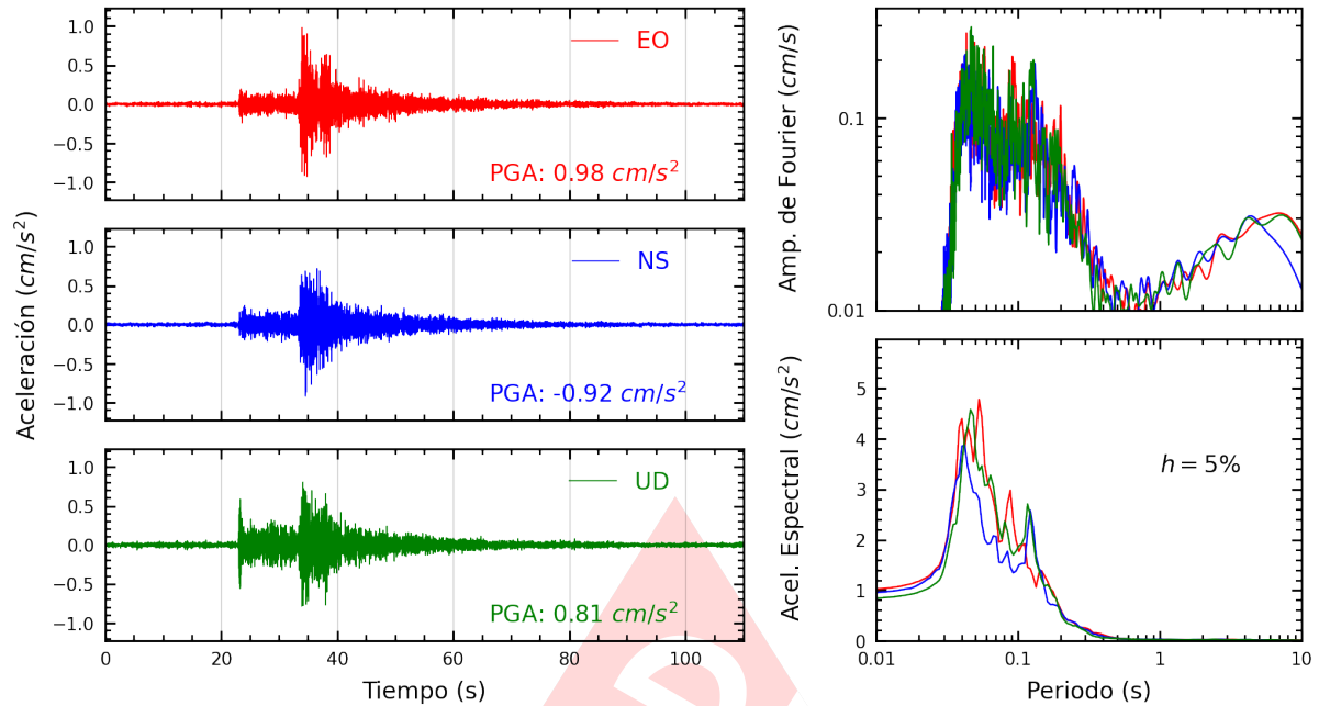
Figura A.27: Registros tiempo-historia, espectros de Fourier y de respuesta en las direcciones EO, NS y vertical de la estación USMP. Sismo de Ancon, Lima - Lima del 2025-02-26, 23:48:47 (Hora local)
