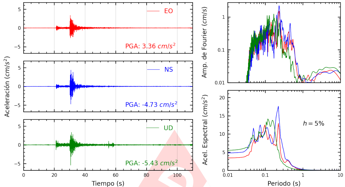
Figura A.3: Registros tiempo-historia, espectros de Fourier y de respuesta en las direcciones EO, NS y vertical de la estación MDPP. Sismo de Ancon, Lima - Lima del 2025-02-26, 23:48:47 (Hora local)
