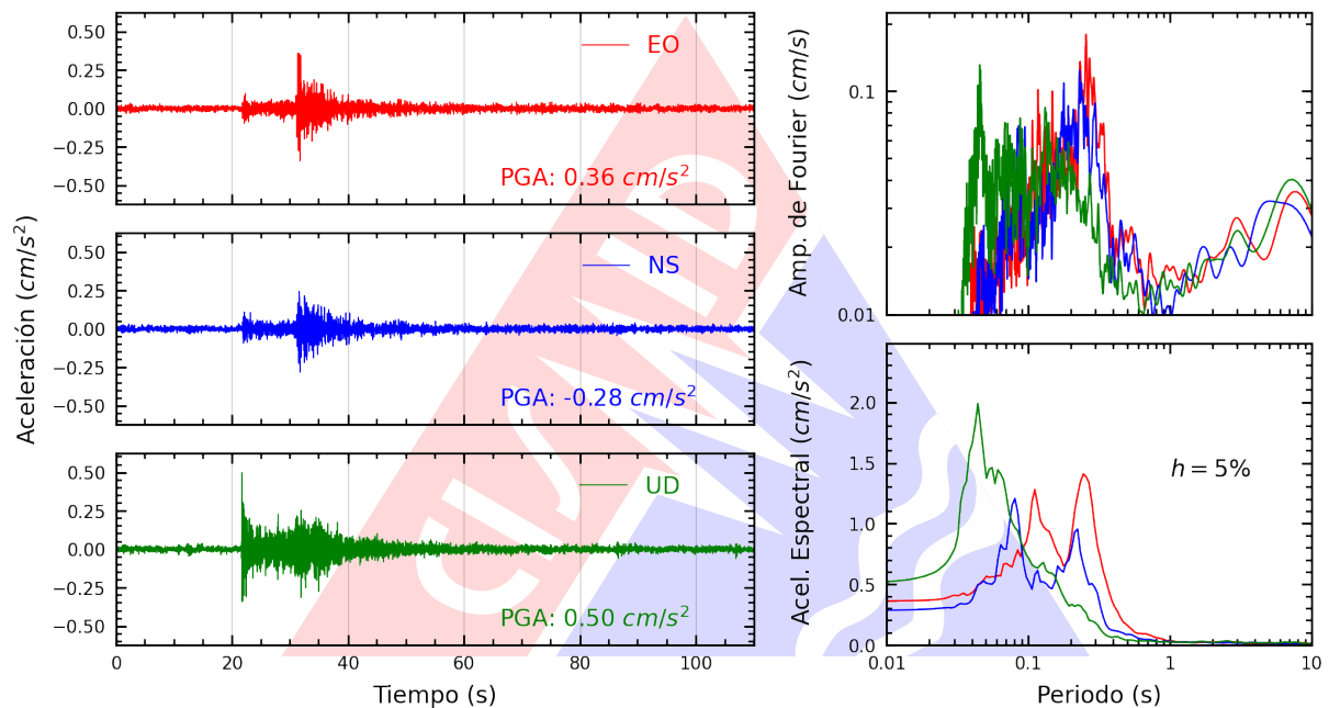
Figura A.37: Registros tiempo-historia, espectros de Fourier y de respuesta en las direcciones EO, NS y vertical de la estación DSMI. Sismo de Ancon, Lima - Lima del 2025-02-26, 23:48:47 (Hora local)
