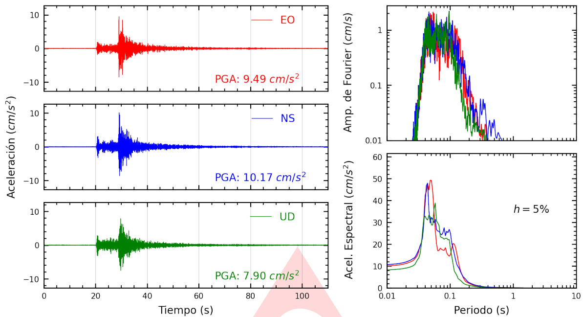
Figura A.1: Registros tiempo-historia, espectros de Fourier y de respuesta en las direcciones EO, NS y vertical de la estación SROS2. Sismo de Ancon, Lima - Lima del 2025-02-26, 23:48:47 (Hora local)
