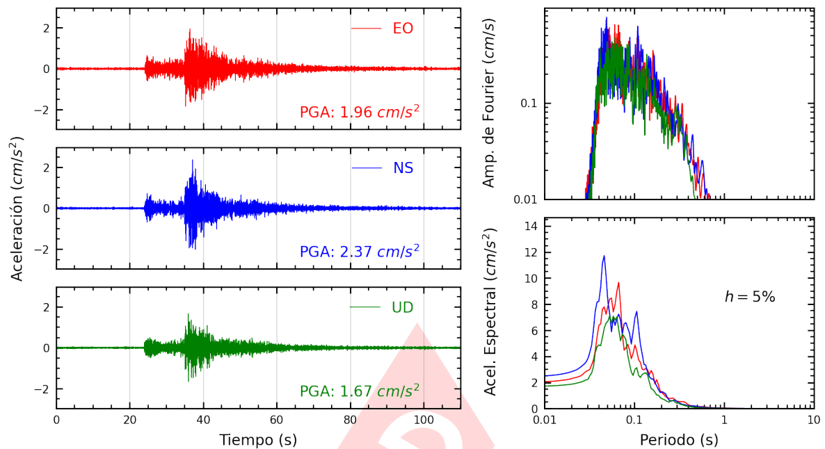
Figura A.13: Registros tiempo-historia, espectros de Fourier y de respuesta en las direcciones EO, NS y vertical de la estación UNTEL. Sismo de Ancon, Lima - Lima del 2025-02-26, 23:48:47 (Hora local)
