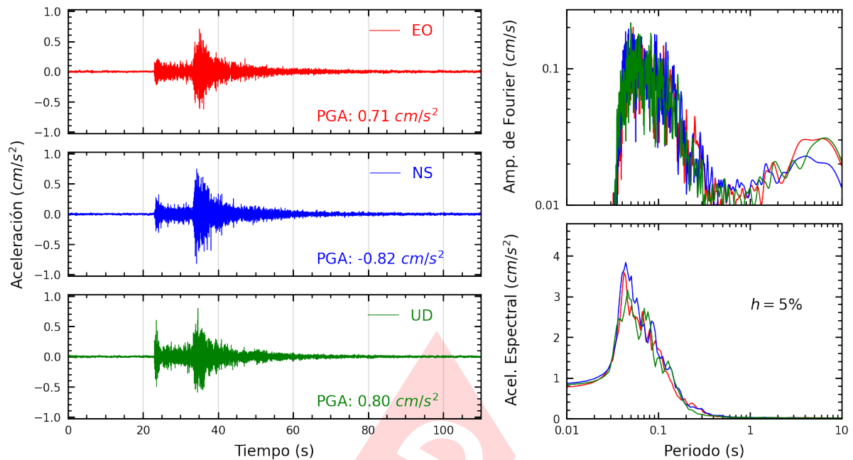
Figura A.29: Registros tiempo-historia, espectros de Fourier y de respuesta en las direcciones EO, NS y vertical de la estación SERVI. Sismo de Ancon, Lima - Lima del 2025-02-26, 23:48:47 (Hora local)
