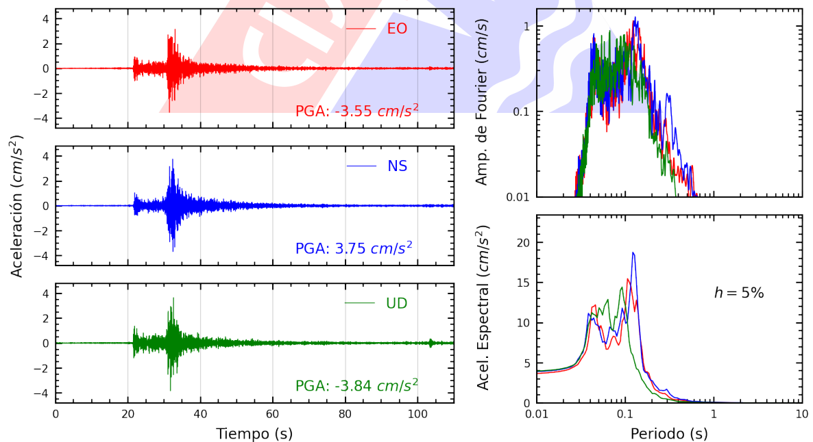
Figura A.6: Registros tiempo-historia, espectros de Fourier y de respuesta en las direcciones EO, NS y vertical de la estación CARA2. Sismo de Ancon, Lima - Lima del 2025-02-26, 23:48:47 (Hora local)
