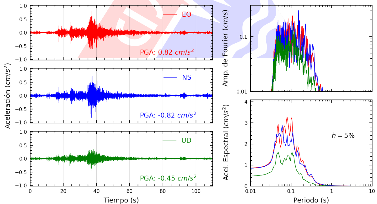
Figura A.30: Registros tiempo-historia, espectros de Fourier y de respuesta en las direcciones EO, NS y vertical de la estación BRISA. Sismo de Ancon, Lima - Lima del 2025-02-26, 23:48:47 (Hora local)
