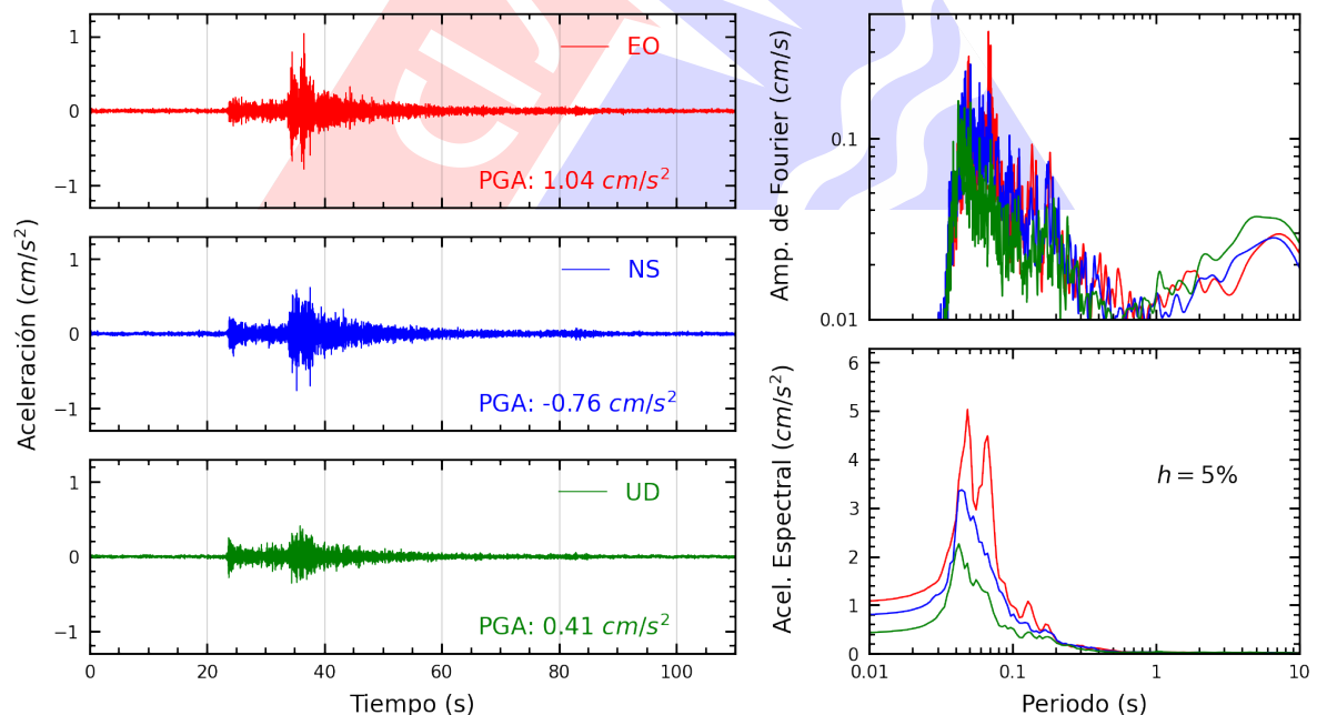
Figura A.26: Registros tiempo-historia, espectros de Fourier y de respuesta en las direcciones EO, NS y vertical de la estación UPCVI. Sismo de Ancon, Lima - Lima del 2025-02-26, 23:48:47 (Hora local)
