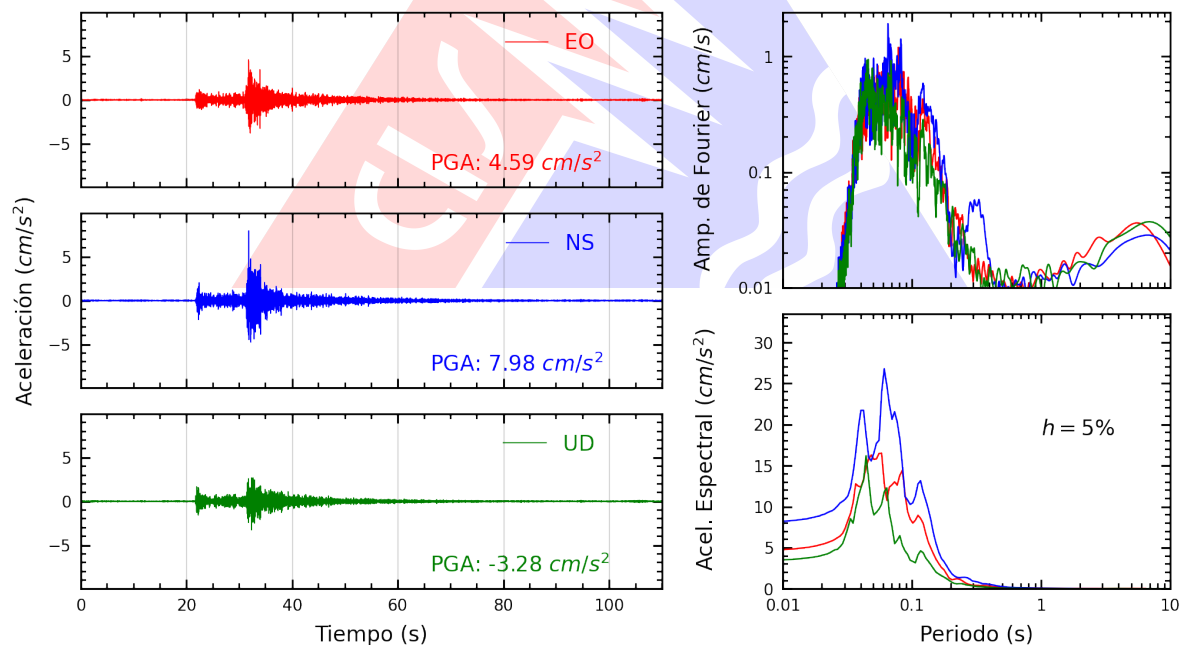
Figura A.2: Registros tiempo-historia, espectros de Fourier y de respuesta en las direcciones EO, NS y vertical de la estación JOSEO. Sismo de Ancon, Lima - Lima del 2025-02-26, 23:48:47 (Hora local)
