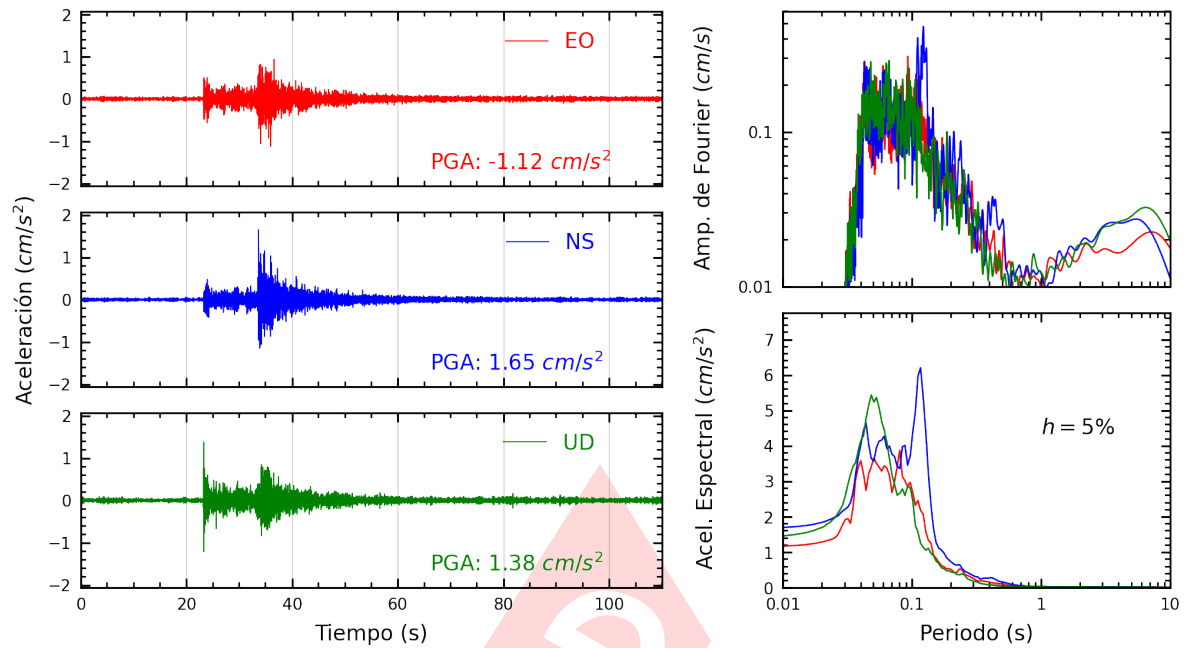
Figura A.15: Registros tiempo-historia, espectros de Fourier y de respuesta en las direcciones EO, NS y vertical de la estación URPPE. Sismo de Ancon, Lima - Lima del 2025-02-26, 23:48:47 (Hora local)
