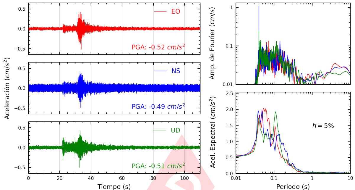
Figura A.35: Registros tiempo-historia, espectros de Fourier y de respuesta en las direcciones EO, NS y vertical de la estación BONDY. Sismo de Ancon, Lima - Lima del 2025-02-26, 23:48:47 (Hora local)
