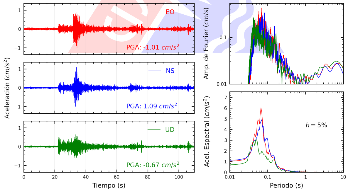
Figura A.24: Registros tiempo-historia, espectros de Fourier y de respuesta en las direcciones EO, NS y vertical de la estación UPCSM. Sismo de Ancon, Lima - Lima del 2025-02-26, 23:48:47 (Hora local)
