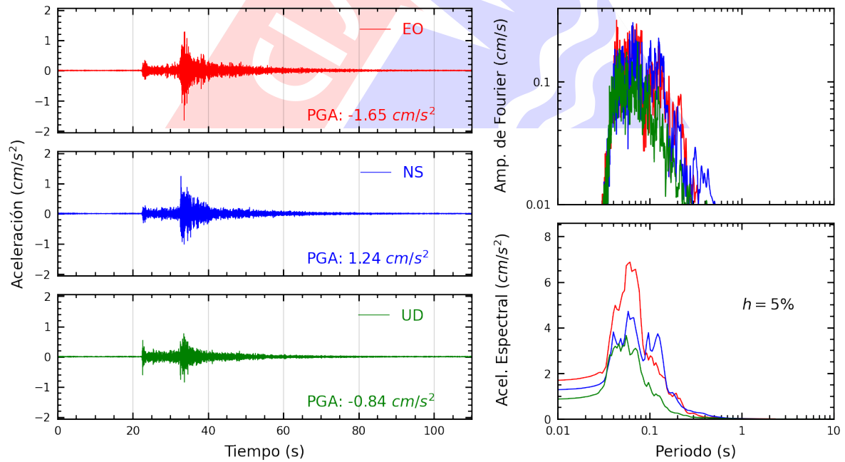
Figura A.16: Registros tiempo-historia, espectros de Fourier y de respuesta en las direcciones EO, NS y vertical de la estación ATARJ. Sismo de Ancon, Lima - Lima del 2025-02-26, 23:48:47 (Hora local)
