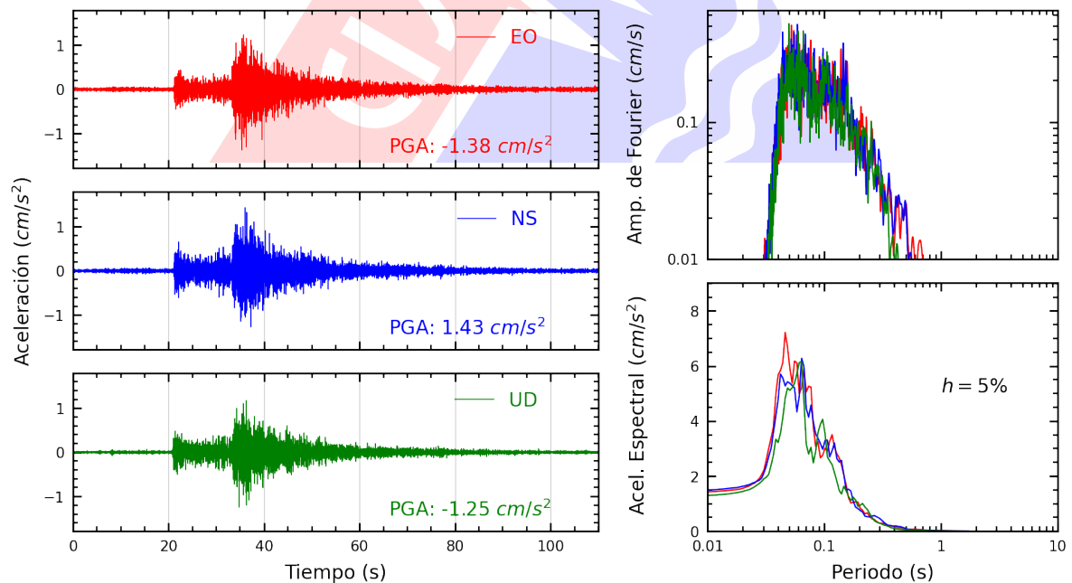
Figura A.18: Registros tiempo-historia, espectros de Fourier y de respuesta en las direcciones EO, NS y vertical de la estación PHER2. Sismo de Ancon, Lima - Lima del 2025-02-26, 23:48:47 (Hora local)
