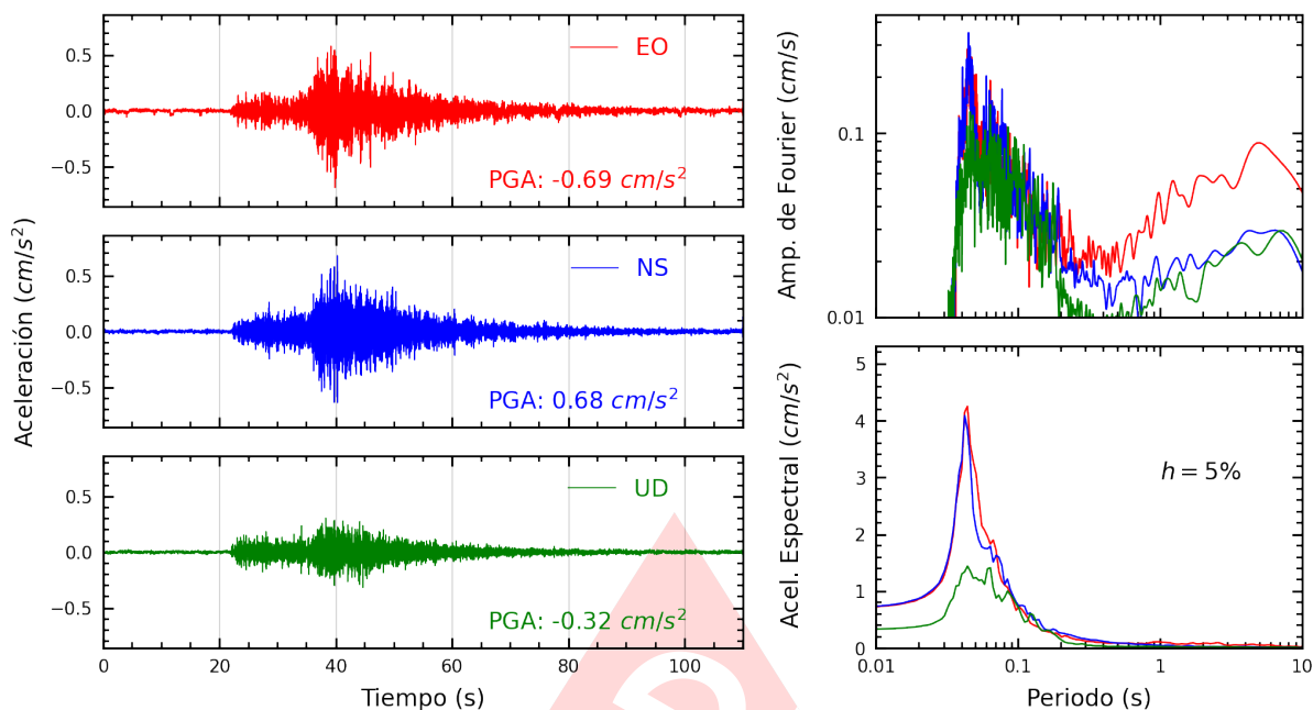
Figura A.33: Registros tiempo-historia, espectros de Fourier y de respuesta en las direcciones EO, NS y vertical de la estación UNAB. Sismo de Ancon, Lima - Lima del 2025-02-26, 23:48:47 (Hora local)
