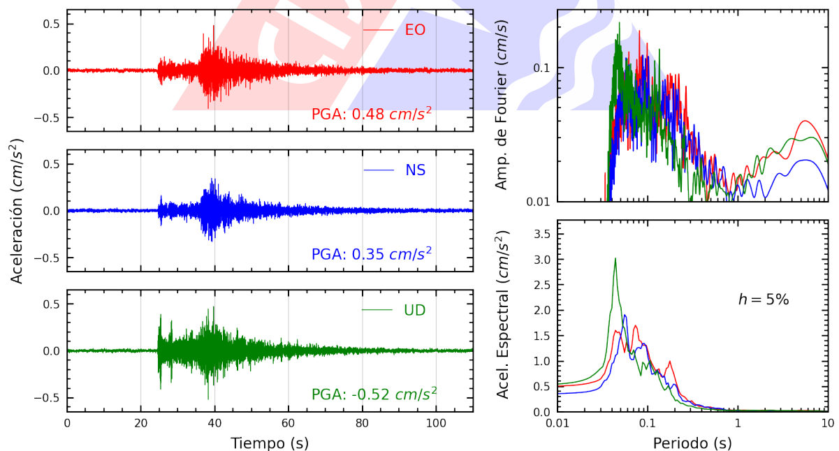
Figura A.36: Registros tiempo-historia, espectros de Fourier y de respuesta en las direcciones EO, NS y vertical de la estación USILP. Sismo de Ancon, Lima - Lima del 2025-02-26, 23:48:47 (Hora local)
