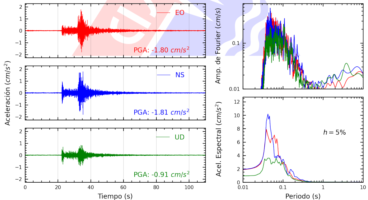
Figura A.14: Registros tiempo-historia, espectros de Fourier y de respuesta en las direcciones EO, NS y vertical de la estación CEPRE. Sismo de Ancon, Lima - Lima del 2025-02-26, 23:48:47 (Hora local)
