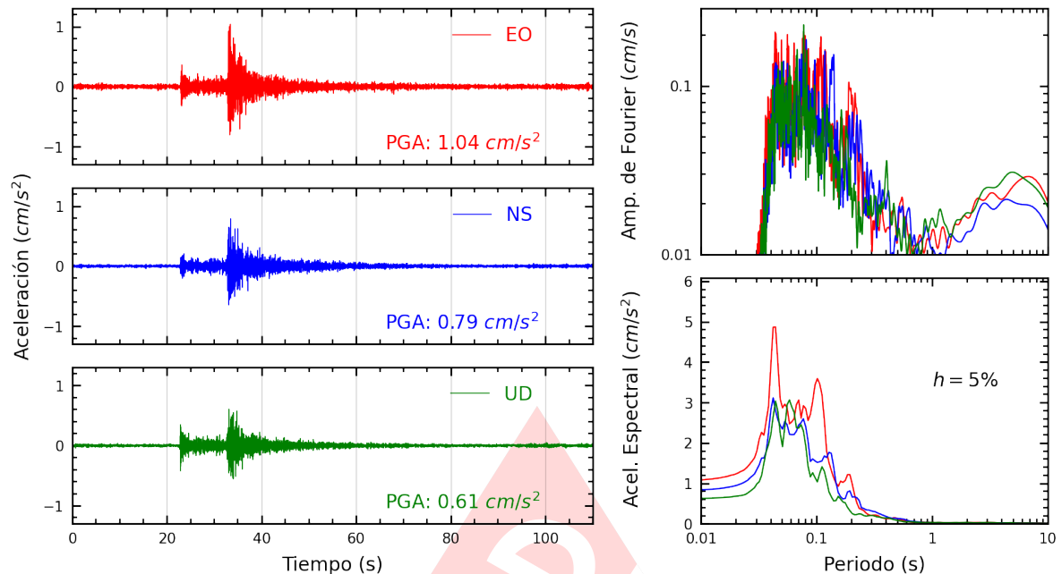
Figura A.25: Registros tiempo-historia, espectros de Fourier y de respuesta en las direcciones EO, NS y vertical de la estación INICT. Sismo de Ancon, Lima - Lima del 2025-02-26, 23:48:47 (Hora local)
