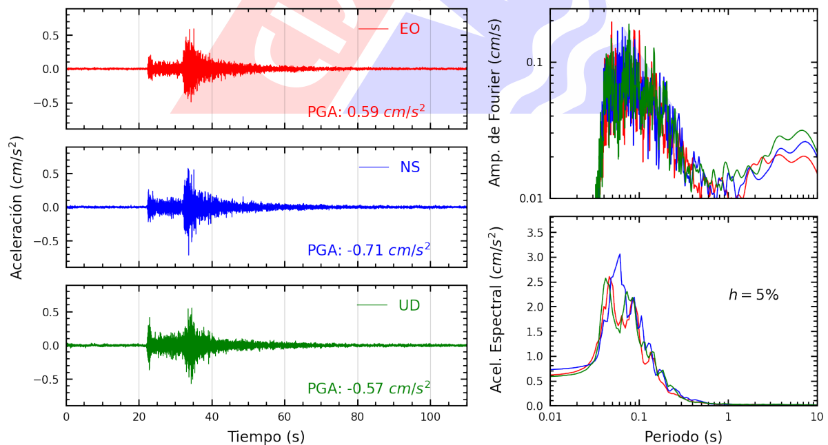
Figura A.32: Registros tiempo-historia, espectros de Fourier y de respuesta en las direcciones EO, NS y vertical de la estación UNFV. Sismo de Ancon, Lima - Lima del 2025-02-26, 23:48:47 (Hora local)
