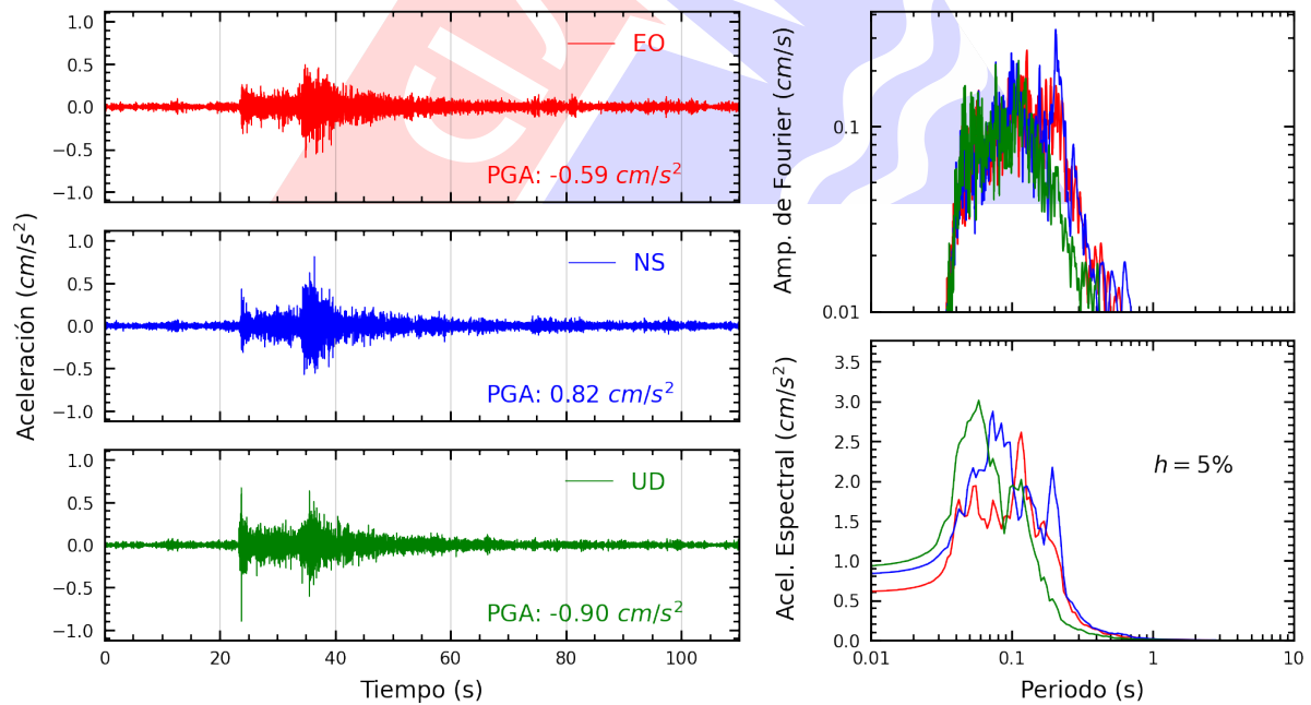
Figura A.28: Registros tiempo-historia, espectros de Fourier y de respuesta en las direcciones EO, NS y vertical de la estación SCCHO. Sismo de Ancon, Lima - Lima del 2025-02-26, 23:48:47 (Hora local)
