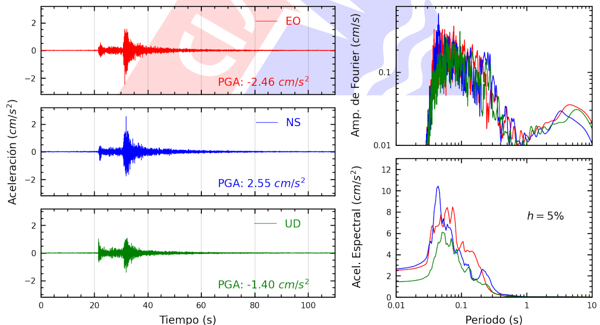
Figura A.12: Registros tiempo-historia, espectros de Fourier y de respuesta en las direcciones EO, NS y vertical de la estación COMAS. Sismo de Ancon, Lima - Lima del 2025-02-26, 23:48:47 (Hora local)
