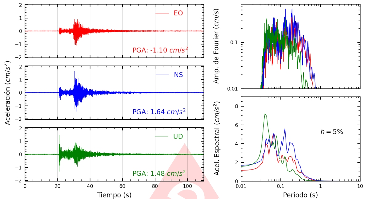
Figura A.17: Registros tiempo-historia, espectros de Fourier y de respuesta en las direcciones EO, NS y vertical de la estación VHAY2. Sismo de Ancon, Lima - Lima del 2025-02-26, 23:48:47 (Hora local)
