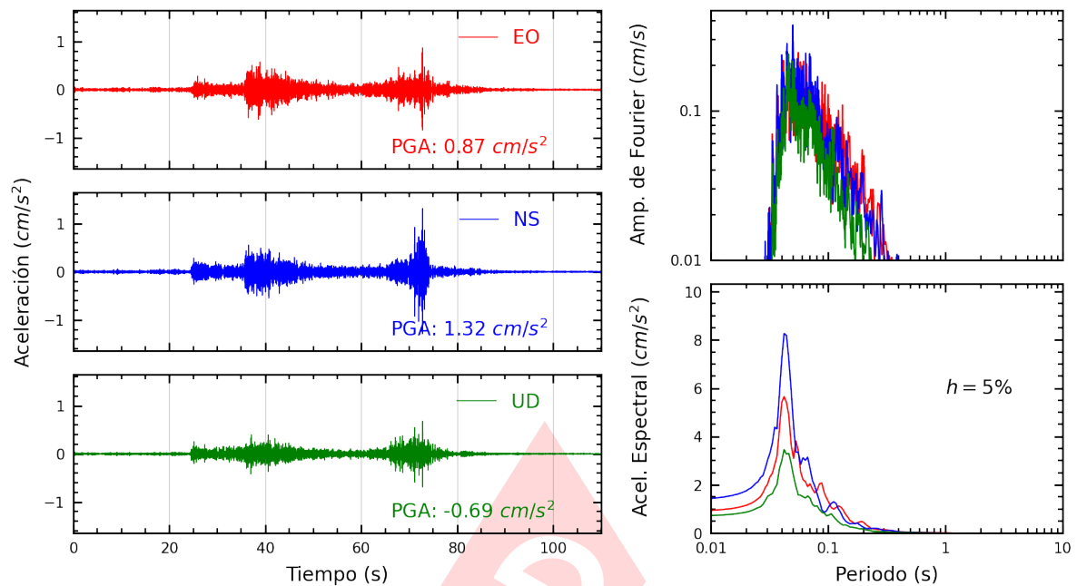
Figura A.19: Registros tiempo-historia, espectros de Fourier y de respuesta en las direcciones EO, NS y vertical de la estación PACHA. Sismo de Ancon, Lima - Lima del 2025-02-26, 23:48:47 (Hora local)
