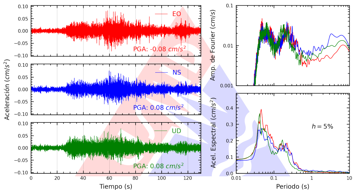
Figura A.7: Registros tiempo-historia, espectros de Fourier y de respuesta en las direcciones EO, NS y vertical de la estación CREY. Sismo de Quilca, Camana - Arequipa del 2025-02-27, 22:45:27 (Hora local)
