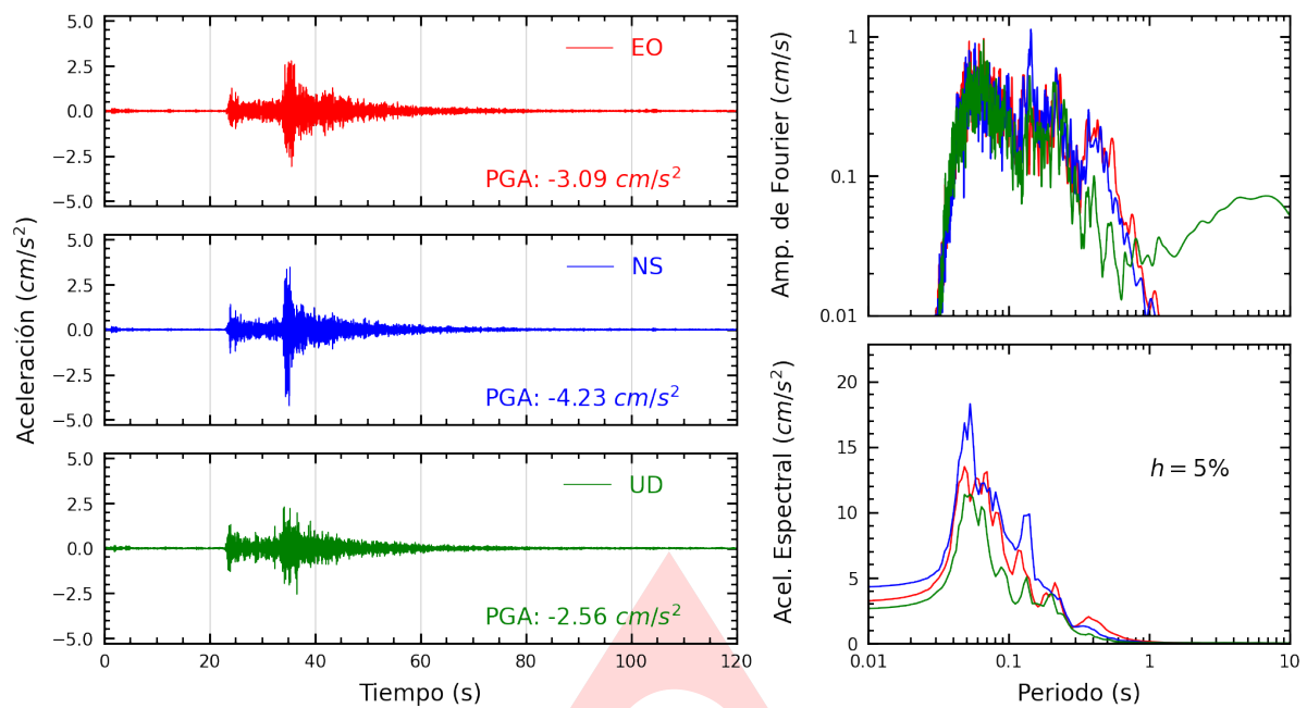
Figura A.1: Registros tiempo-historia, espectros de Fourier y de respuesta en las direcciones EO, NS y vertical de la estación SCARQ. Sismo de Quilca, Camana - Arequipa del 2025-02-27, 22:45:27 (Hora local)
