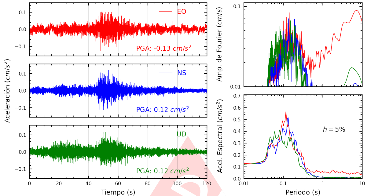
Figura A.5: Registros tiempo-historia, espectros de Fourier y de respuesta en las direcciones EO, NS y vertical de la estación UJBG3. Sismo de Quilca, Camana - Arequipa del 2025-02-27, 22:45:27 (Hora local)
