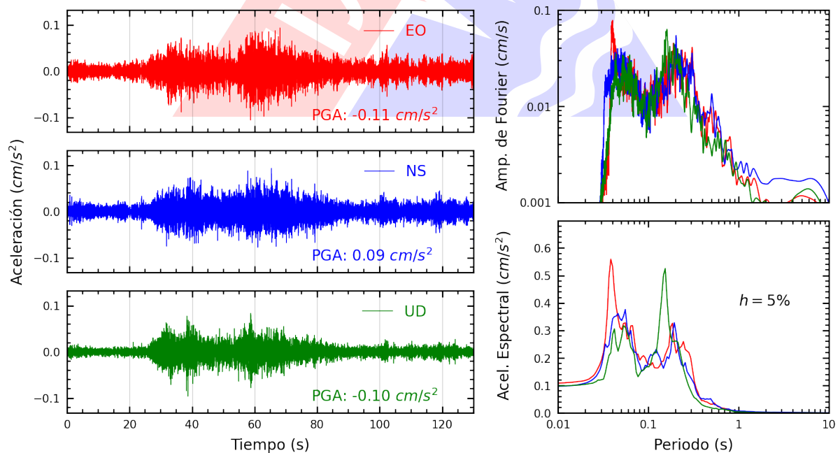
Figura A.6: Registros tiempo-historia, espectros de Fourier y de respuesta en las direcciones EO, NS y vertical de la estación UPTAC. Sismo de Quilca, Camana - Arequipa del 2025-02-27, 22:45:27 (Hora local)
