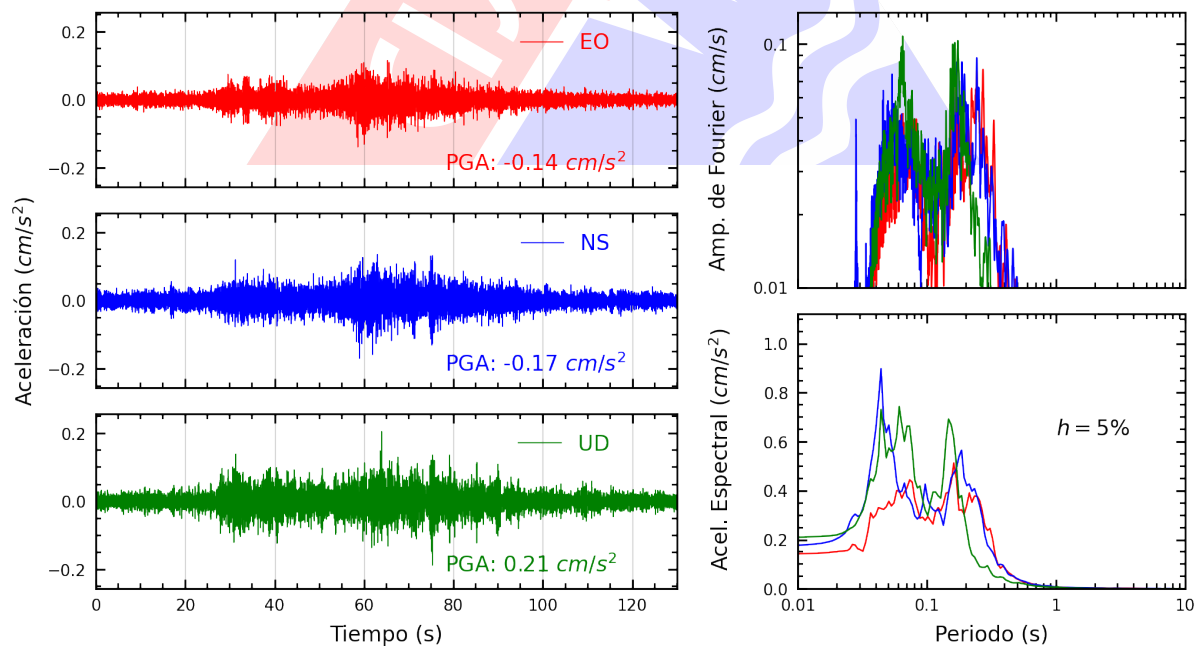
Figura A.4: Registros tiempo-historia, espectros de Fourier y de respuesta en las direcciones EO, NS y vertical de la estación UJBG4. Sismo de Quilca, Camana - Arequipa del 2025-02-27, 22:45:27 (Hora local)
