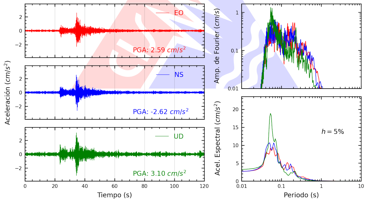
Figura A.2: Registros tiempo-historia, espectros de Fourier y de respuesta en las direcciones EO, NS y vertical de la estación SCAR2. Sismo de Quilca, Camana - Arequipa del 2025-02-27, 22:45:27 (Hora local)
