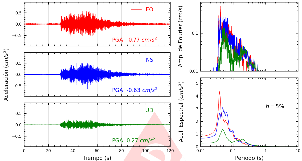
Figura A.3: Registros tiempo-historia, espectros de Fourier y de respuesta en las direcciones EO, NS y vertical de la estación UNAM. Sismo de Quilca, Camana - Arequipa del 2025-02-27, 22:45:27 (Hora local)
