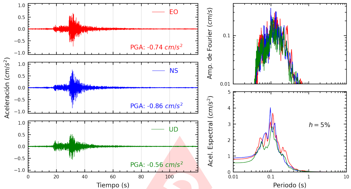
Figura A.23: Registros tiempo-historia, espectros de Fourier y de respuesta en las direcciones EO, NS y vertical de la estación JALV2. Sismo de Chilca, Cañete - Lima del 2024-10-22, 12:23:32 (Hora local)
