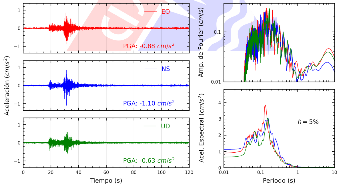
Figura A.18: Registros tiempo-historia, espectros de Fourier y de respuesta en las direcciones EO, NS y vertical de la estación IMCA. Sismo de Chilca, Cañete - Lima del 2024-10-22, 12:23:32 (Hora local)
