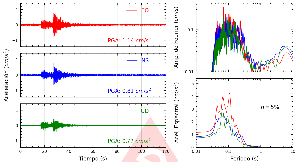
Figura A.17: Registros tiempo-historia, espectros de Fourier y de respuesta en las direcciones EO, NS y vertical de la estación CEPRE. Sismo de Chilca, Cañete - Lima del 2024-10-22, 12:23:32 (Hora local)
