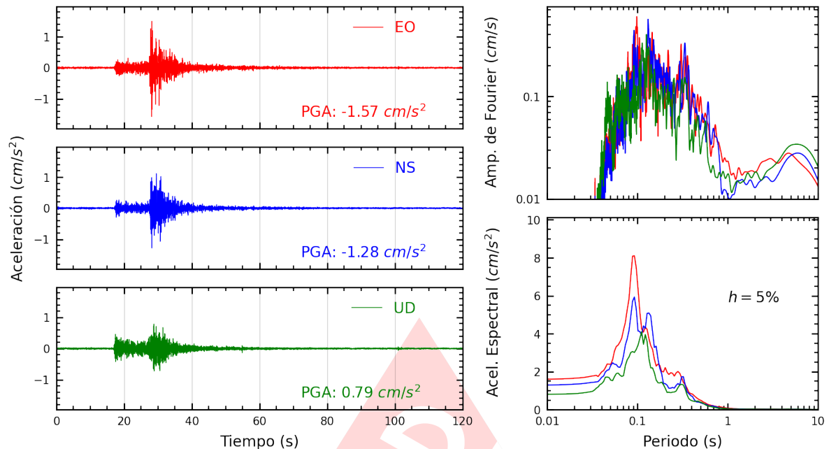
Figura A.9: Registros tiempo-historia, espectros de Fourier y de respuesta en las direcciones EO, NS y vertical de la estación USILP. Sismo de Chilca, Cañete - Lima del 2024-10-22, 12:23:32 (Hora local)
