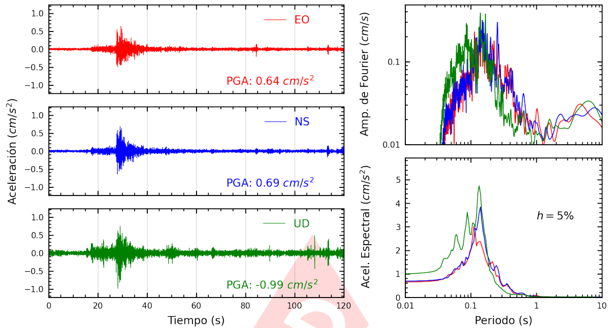
Figura A.19: Registros tiempo-historia, espectros de Fourier y de respuesta en las direcciones EO, NS y vertical de la estación RAMON. Sismo de Chilca, Cañete - Lima del 2024-10-22, 12:23:32 (Hora local)
