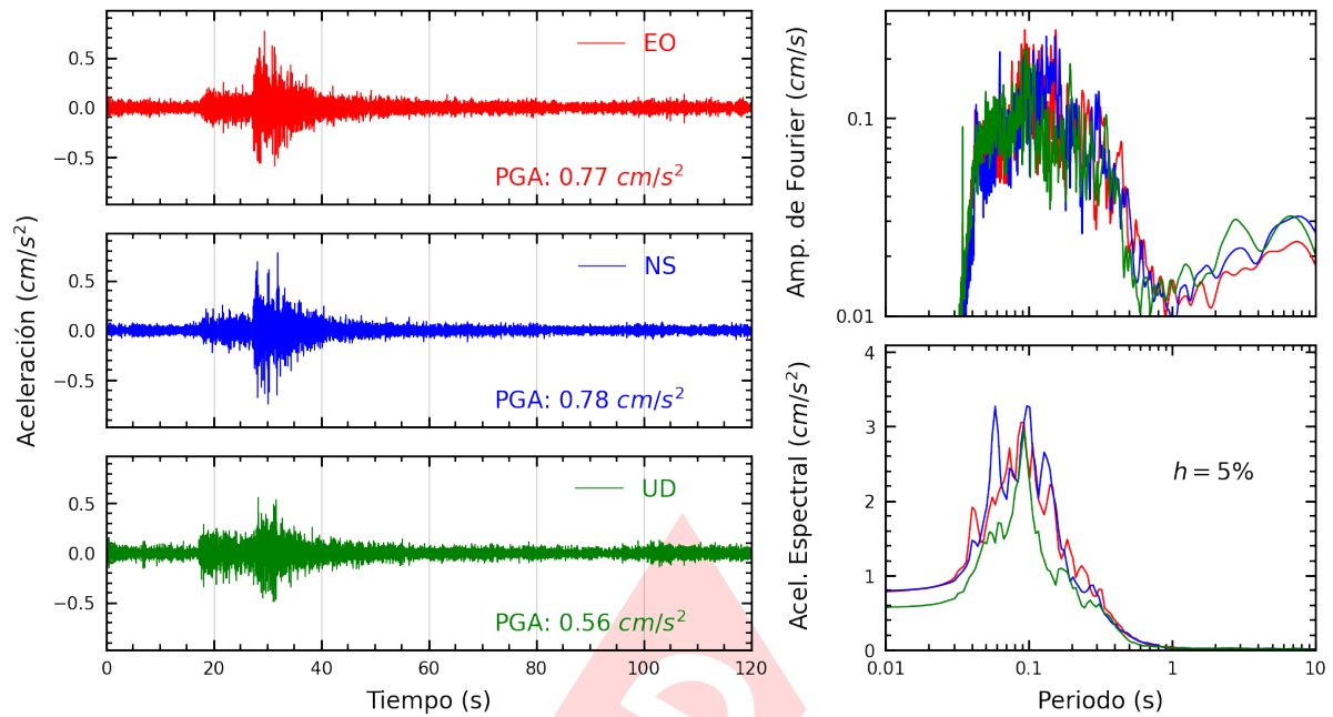
Figura A.25: Registros tiempo-historia, espectros de Fourier y de respuesta en las direcciones EO, NS y vertical de la estación URPPE. Sismo de Chilca, Cañete - Lima del 2024-10-22, 12:23:32 (Hora local)
