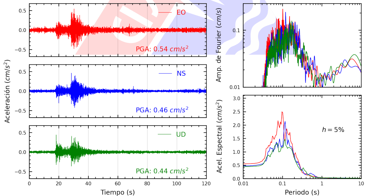
Figura A.28: Registros tiempo-historia, espectros de Fourier y de respuesta en las direcciones EO, NS y vertical de la estación INICT. Sismo de Chilca, Cañete - Lima del 2024-10-22, 12:23:32 (Hora local)
