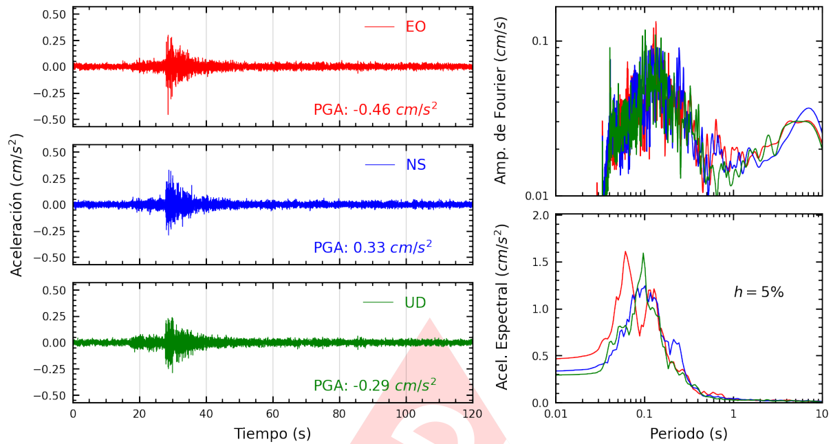
Figura A.29: Registros tiempo-historia, espectros de Fourier y de respuesta en las direcciones EO, NS y vertical de la estación BONDY. Sismo de Chilca, Cañete - Lima del 2024-10-22, 12:23:32 (Hora local)
