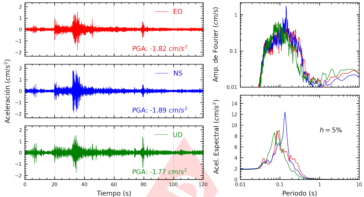
Figura A.5: Registros tiempo-historia, espectros de Fourier y de respuesta en las direcciones EO, NS y vertical de la estación CARAB. Sismo de Chilca, Cañete - Lima del 2024-10-22, 12:23:32 (Hora local)
