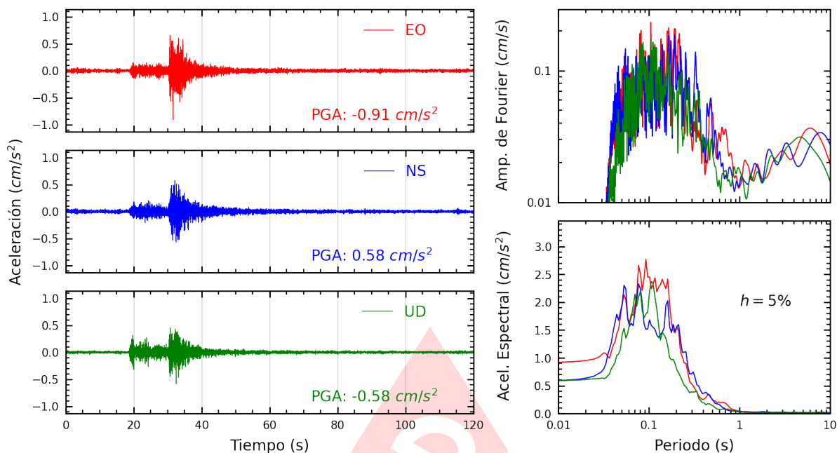
Figura A.21: Registros tiempo-historia, espectros de Fourier y de respuesta en las direcciones EO, NS y vertical de la estación COMAS. Sismo de Chilca, Cañete - Lima del 2024-10-22, 12:23:32 (Hora local)
