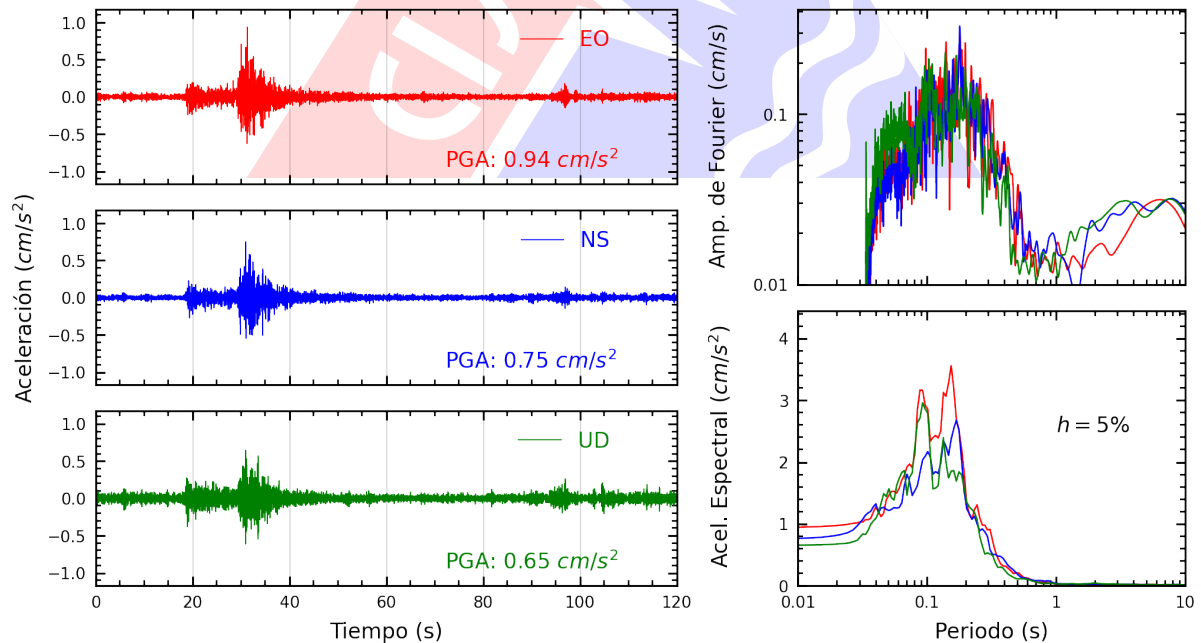
Figura A.20: Registros tiempo-historia, espectros de Fourier y de respuesta en las direcciones EO, NS y vertical de la estación USMP. Sismo de Chilca, Cañete - Lima del 2024-10-22, 12:23:32 (Hora local)
