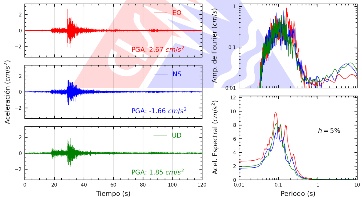
Figura A.2: Registros tiempo-historia, espectros de Fourier y de respuesta en las direcciones EO, NS y vertical de la estación INDEP. Sismo de Chilca, Cañete - Lima del 2024-10-22, 12:23:32 (Hora local)
