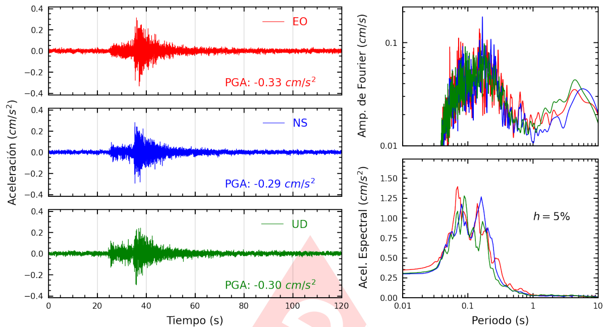
Figura A.33: Registros tiempo-historia, espectros de Fourier y de respuesta en las direcciones EO, NS y vertical de la estación UNMSM. Sismo de Chilca, Cañete - Lima del 2024-10-22, 12:23:32 (Hora local)
