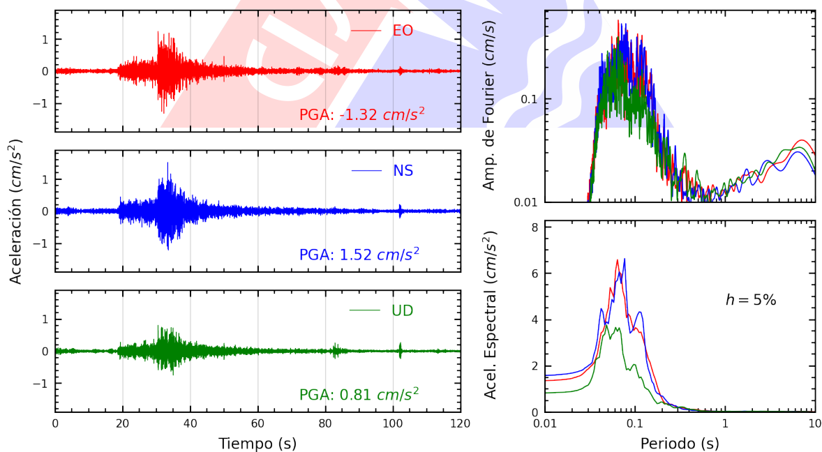
Figura A.12: Registros tiempo-historia, espectros de Fourier y de respuesta en las direcciones EO, NS y vertical de la estación JOSEO. Sismo de Chilca, Cañete - Lima del 2024-10-22, 12:23:32 (Hora local)
