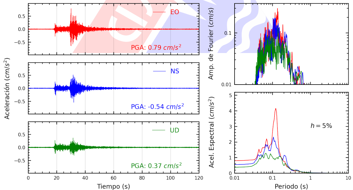
Figura A.24: Registros tiempo-historia, espectros de Fourier y de respuesta en las direcciones EO, NS y vertical de la estación ATARJ. Sismo de Chilca, Cañete - Lima del 2024-10-22, 12:23:32 (Hora local)
