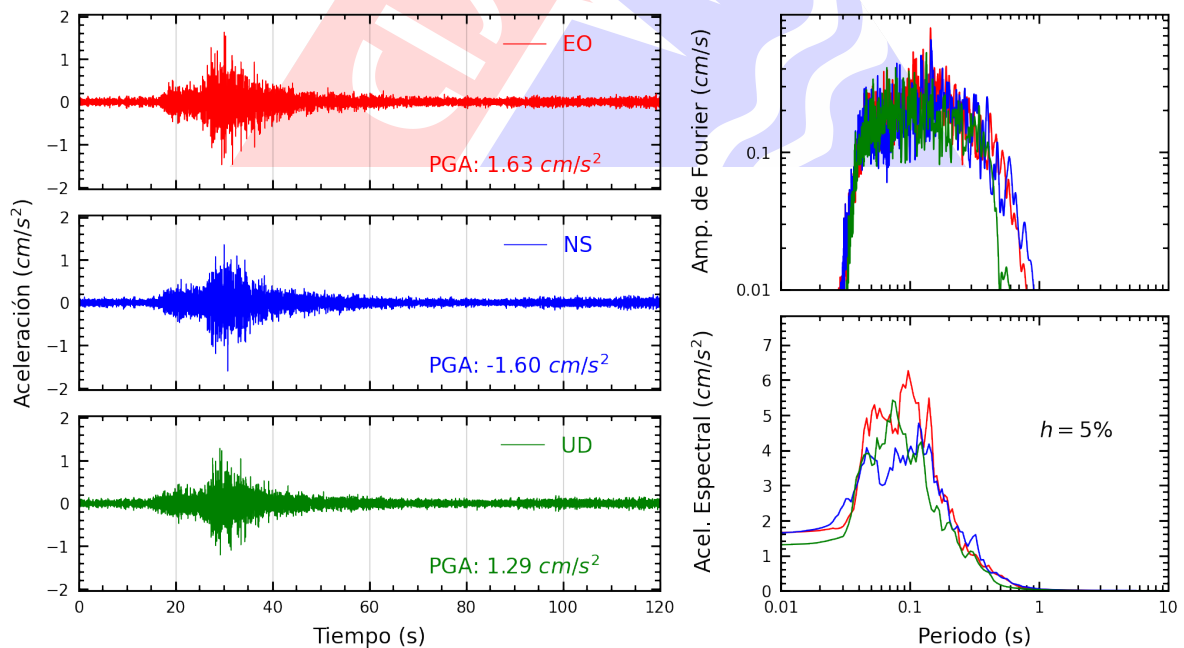
Figura A.8: Registros tiempo-historia, espectros de Fourier y de respuesta en las direcciones EO, NS y vertical de la estación UNTEL. Sismo de Chilca, Cañete - Lima del 2024-10-22, 12:23:32 (Hora local)
