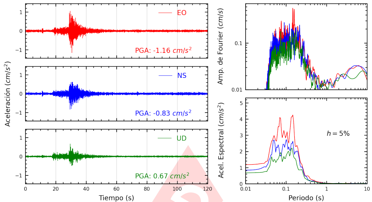
Figura A.15: Registros tiempo-historia, espectros de Fourier y de respuesta en las direcciones EO, NS y vertical de la estación FICPE. Sismo de Chilca, Cañete - Lima del 2024-10-22, 12:23:32 (Hora local)
