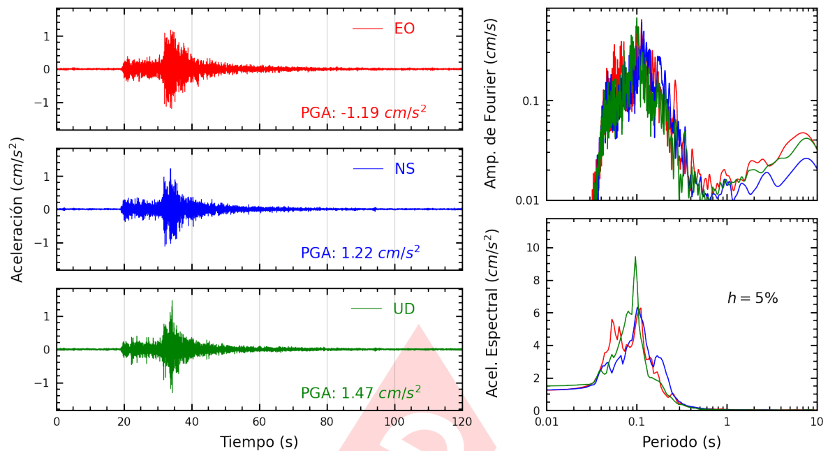
Figura A.13: Registros tiempo-historia, espectros de Fourier y de respuesta en las direcciones EO, NS y vertical de la estación AMORE. Sismo de Chilca, Cañete - Lima del 2024-10-22, 12:23:32 (Hora local)
