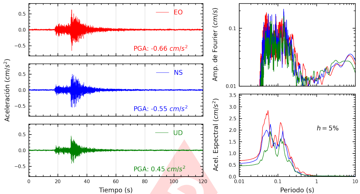
Figura A.27: Registros tiempo-historia, espectros de Fourier y de respuesta en las direcciones EO, NS y vertical de la estación UCSS. Sismo de Chilca, Cañete - Lima del 2024-10-22, 12:23:32 (Hora local)
