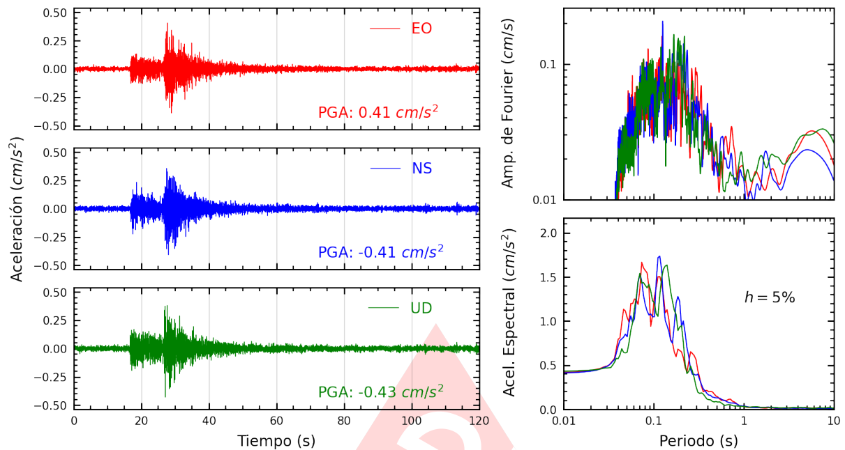
Figura A.31: Registros tiempo-historia, espectros de Fourier y de respuesta en las direcciones EO, NS y vertical de la estación UNFV. Sismo de Chilca, Cañete - Lima del 2024-10-22, 12:23:32 (Hora local)
