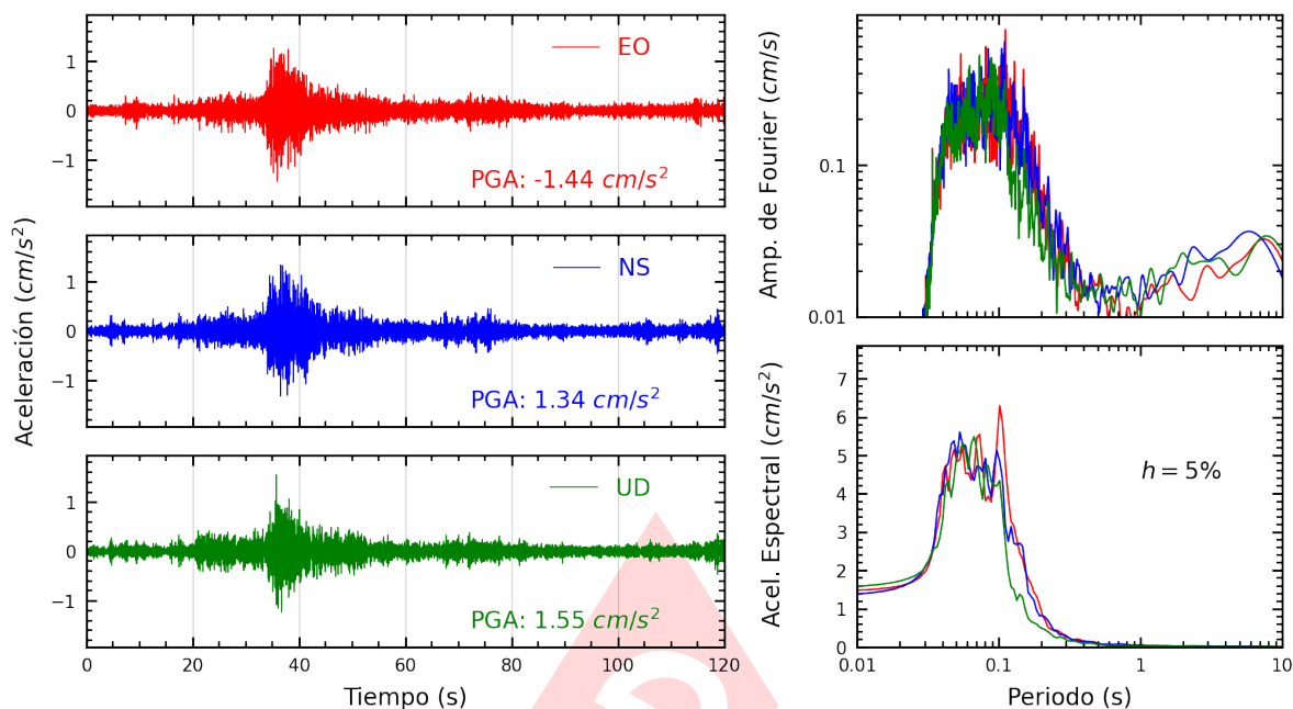
Figura A.11: Registros tiempo-historia, espectros de Fourier y de respuesta en las direcciones EO, NS y vertical de la estación SROSA. Sismo de Chilca, Cañete - Lima del 2024-10-22, 12:23:32 (Hora local)
