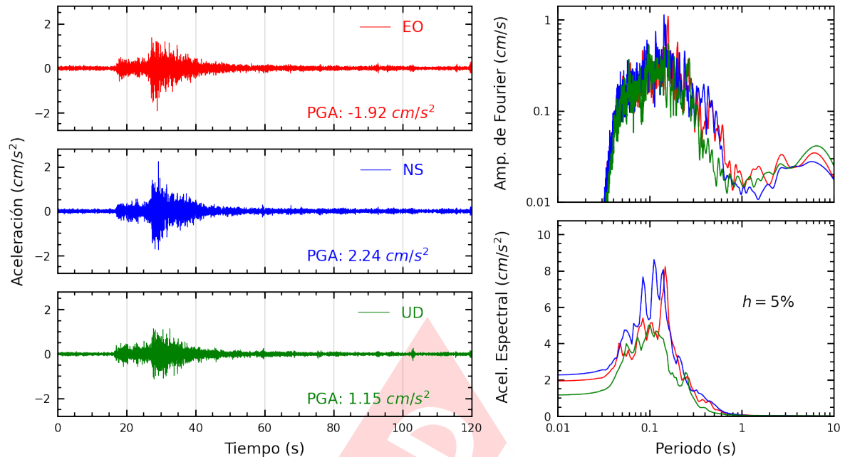
Figura A.3: Registros tiempo-historia, espectros de Fourier y de respuesta en las direcciones EO, NS y vertical de la estación PHERM. Sismo de Chilca, Cañete - Lima del 2024-10-22, 12:23:32 (Hora local)
