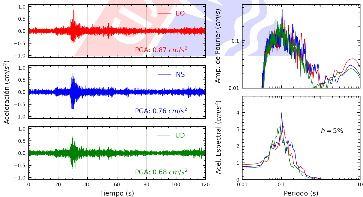
Figura A.22: Registros tiempo-historia, espectros de Fourier y de respuesta en las direcciones EO, NS y vertical de la estación MADRE. Sismo de Chilca, Cañete - Lima del 2024-10-22, 12:23:32 (Hora local)
