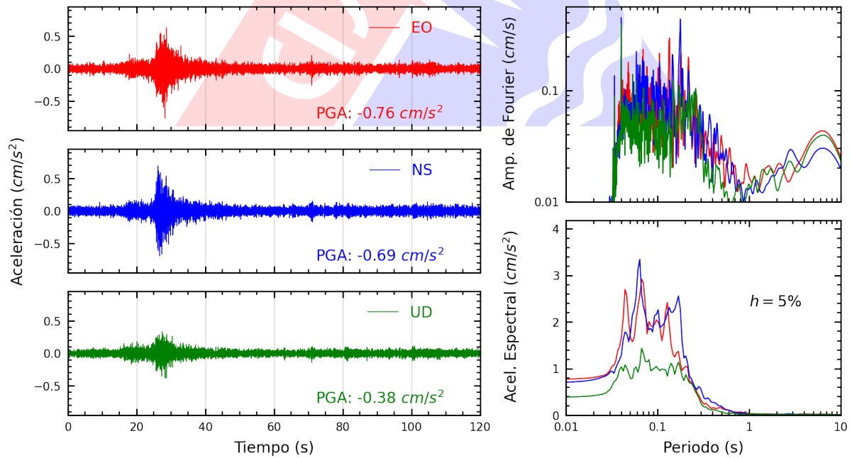
Figura A.26: Registros tiempo-historia, espectros de Fourier y de respuesta en las direcciones EO, NS y vertical de la estación UPCVI. Sismo de Chilca, Cañete - Lima del 2024-10-22, 12:23:32 (Hora local)
