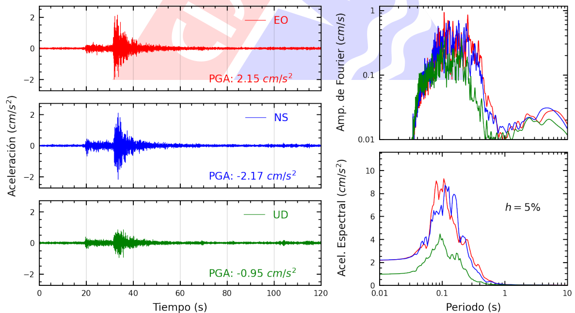
Figura A.4: Registros tiempo-historia, espectros de Fourier y de respuesta en las direcciones EO, NS y vertical de la estación DEFEN. Sismo de Chilca, Cañete - Lima del 2024-10-22, 12:23:32 (Hora local)
