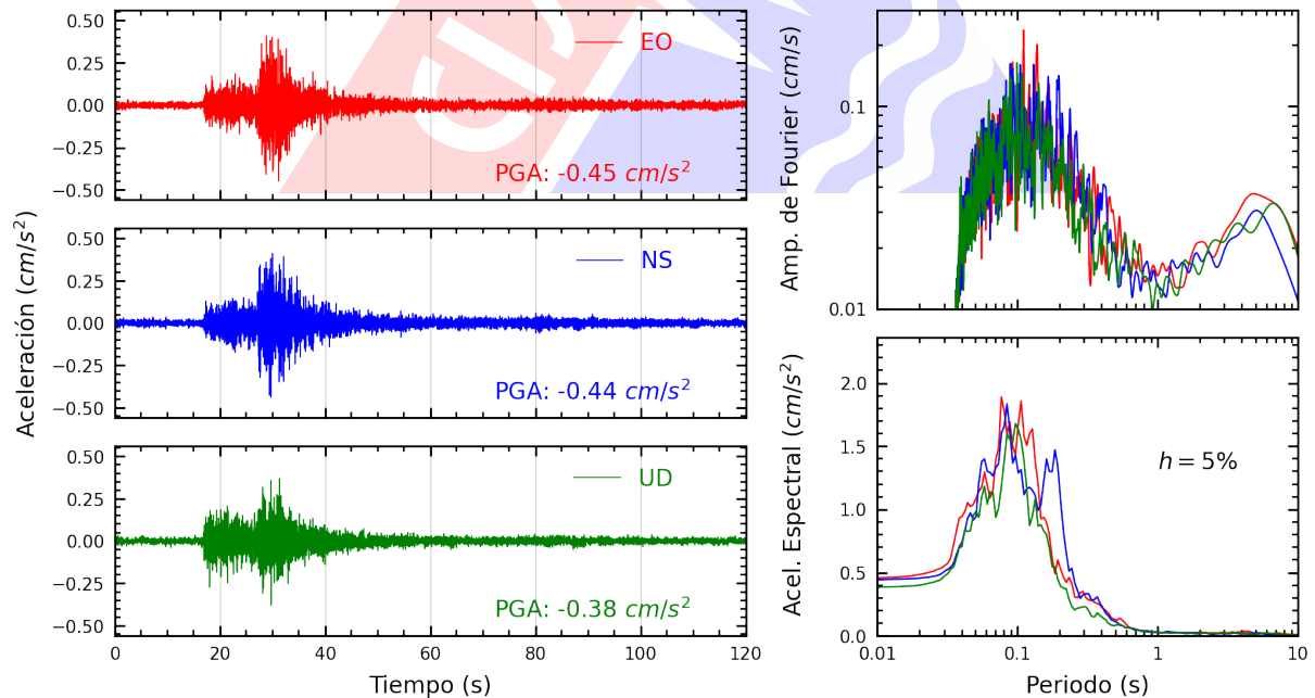
Figura A.30: Registros tiempo-historia, espectros de Fourier y de respuesta en las direcciones EO, NS y vertical de la estación SERVI. Sismo de Chilca, Cañete - Lima del 2024-10-22, 12:23:32 (Hora local)
