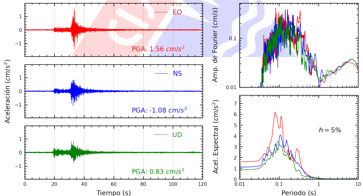
Figura A.10: Registros tiempo-historia, espectros de Fourier y de respuesta en las direcciones EO, NS y vertical de la estación UCVAT. Sismo de Chilca, Cañete - Lima del 2024-10-22, 12:23:32 (Hora local)
