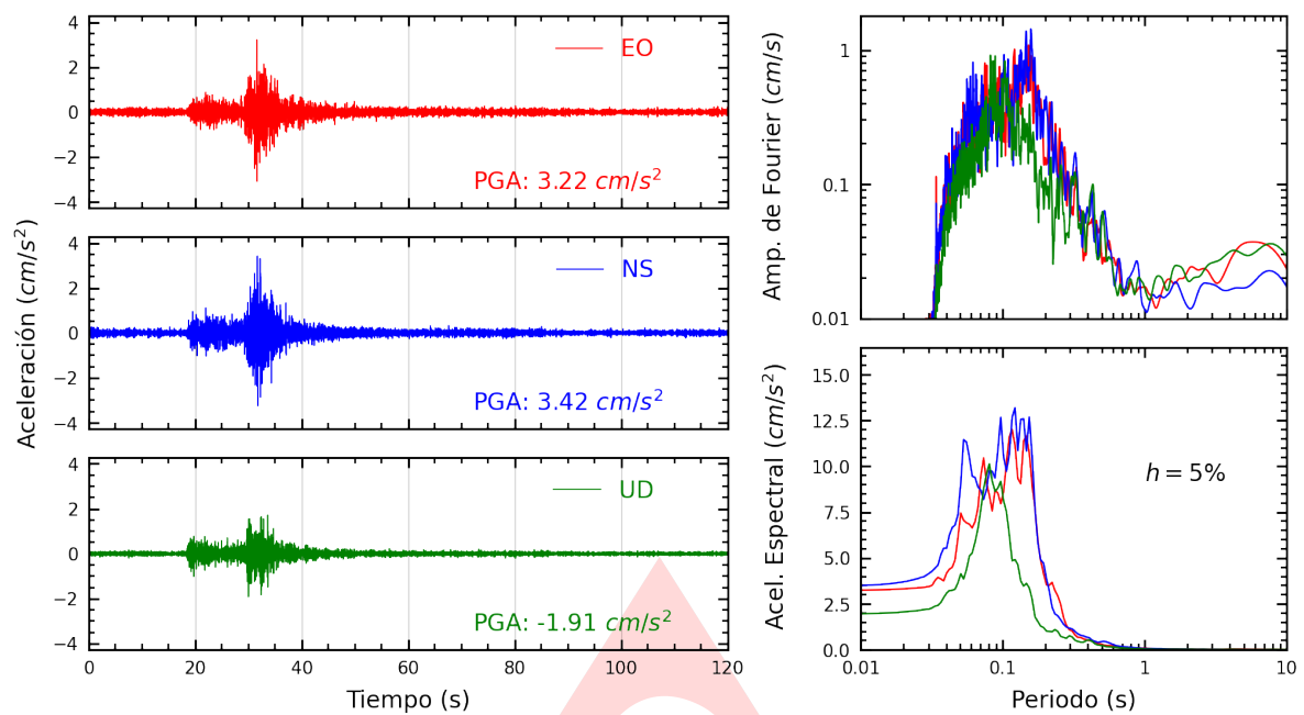
Figura A.1: Registros tiempo-historia, espectros de Fourier y de respuesta en las direcciones EO, NS y vertical de la estación USILM. Sismo de Chilca, Cañete - Lima del 2024-10-22, 12:23:32 (Hora local)
