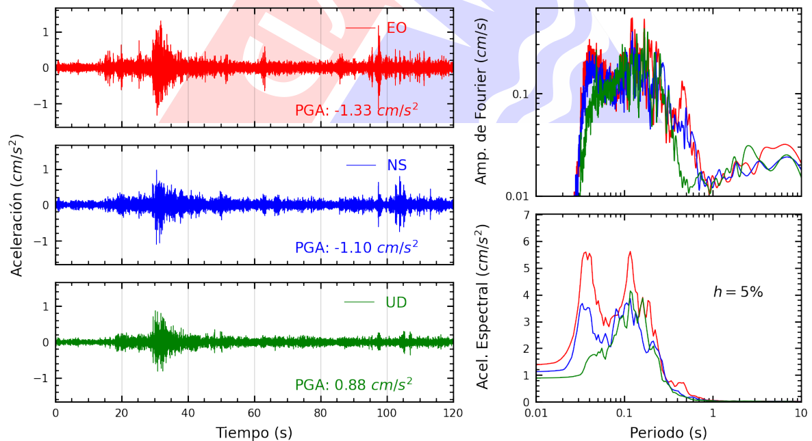
Figura A.14: Registros tiempo-historia, espectros de Fourier y de respuesta en las direcciones EO, NS y vertical de la estación OLIVO. Sismo de Chilca, Cañete - Lima del 2024-10-22, 12:23:32 (Hora local)
