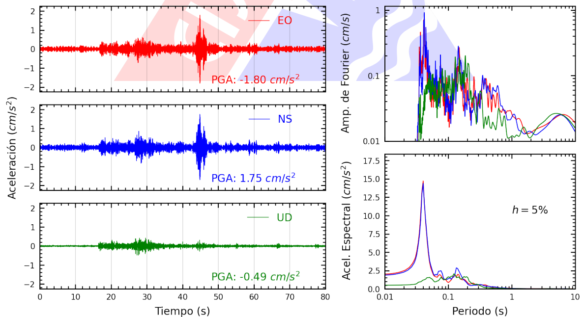
Figura A.6: Registros tiempo-historia, espectros de Fourier y de respuesta en las direcciones EO, NS y vertical de la estación DHNPE. Sismo de Chilca, Cañete - Lima del 2024-10-22, 12:23:32 (Hora local)
