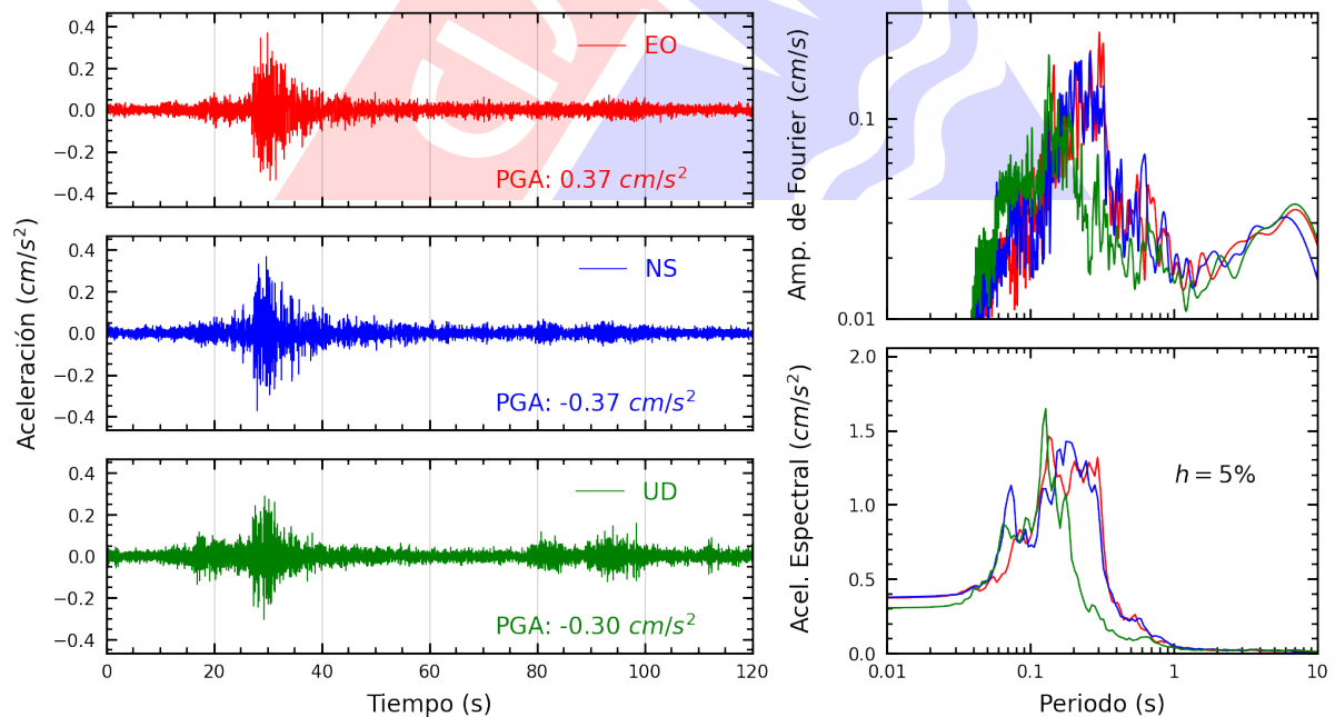
Figura A.32: Registros tiempo-historia, espectros de Fourier y de respuesta en las direcciones EO, NS y vertical de la estación DSMI. Sismo de Chilca, Cañete - Lima del 2024-10-22, 12:23:32 (Hora local)
