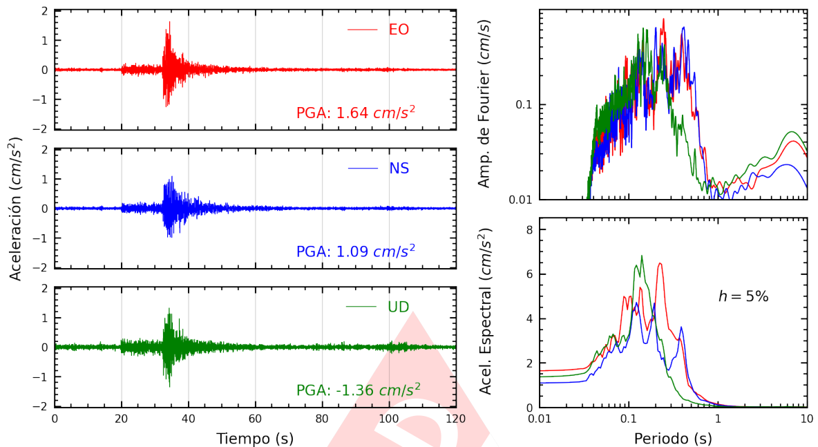
Figura A.7: Registros tiempo-historia, espectros de Fourier y de respuesta en las direcciones EO, NS y vertical de la estación MDPP. Sismo de Chilca, Cañete - Lima del 2024-10-22, 12:23:32 (Hora local)
