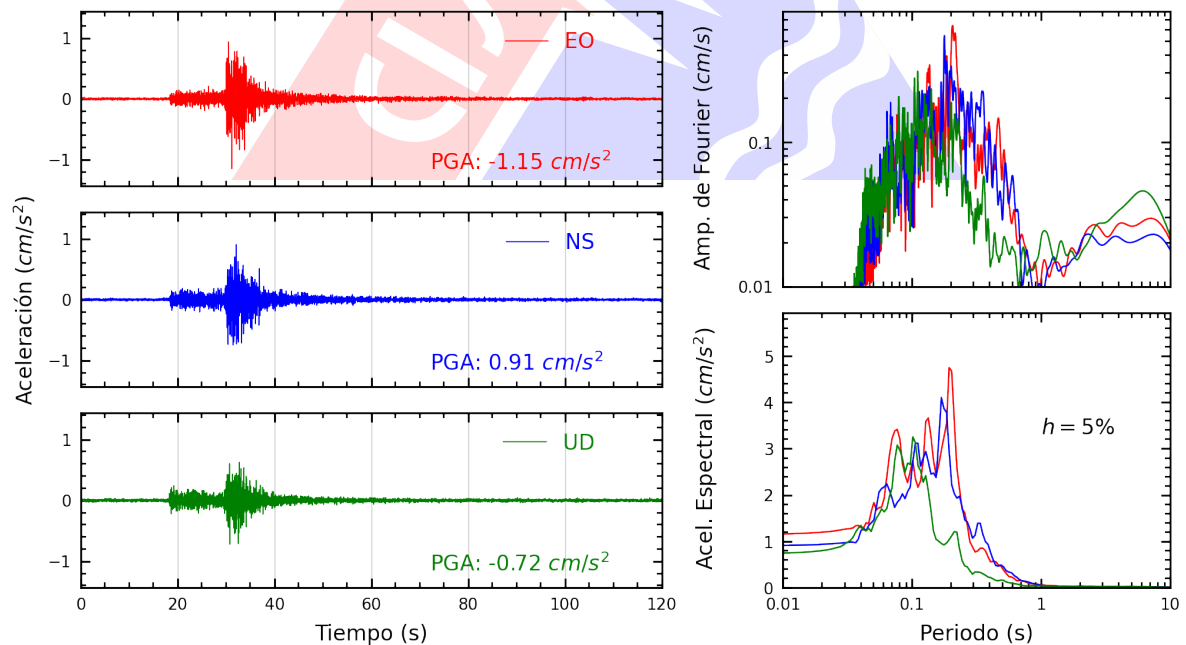
Figura A.16: Registros tiempo-historia, espectros de Fourier y de respuesta en las direcciones EO, NS y vertical de la estación VHAYA. Sismo de Chilca, Cañete - Lima del 2024-10-22, 12:23:32 (Hora local)
