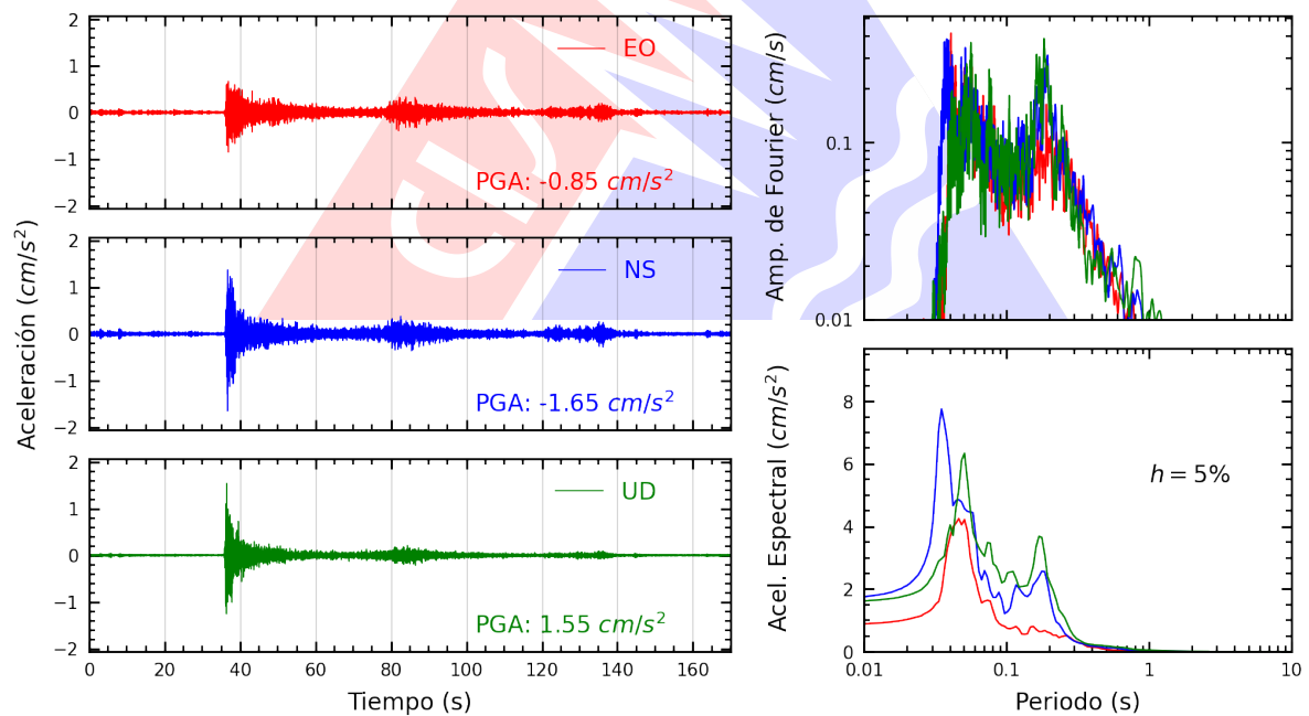
Figura A.2: Registros tiempo-historia, espectros de Fourier y de respuesta en las direcciones EO, NS y vertical de la estación UPTAC. Sismo de Calana, Tacna - Tacna del 2024-11-03, 16:18:39 (Hora local)
