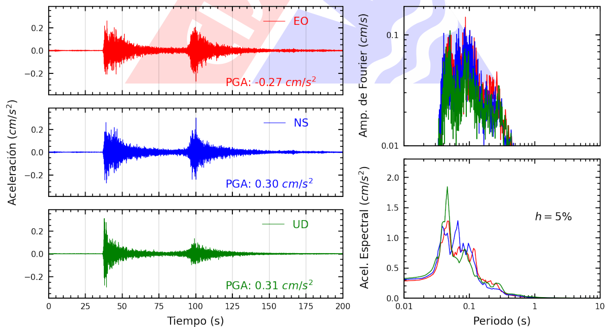
Figura A.6: Registros tiempo-historia, espectros de Fourier y de respuesta en las direcciones EO, NS y vertical de la estación UNSA2. Sismo de Calana, Tacna - Tacna del 2024-11-03, 16:18:39 (Hora local)
