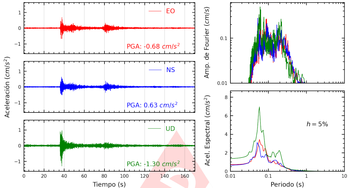
Figura A.3: Registros tiempo-historia, espectros de Fourier y de respuesta en las direcciones EO, NS y vertical de la estación UJBG2. Sismo de Calana, Tacna - Tacna del 2024-11-03, 16:18:39 (Hora local)
