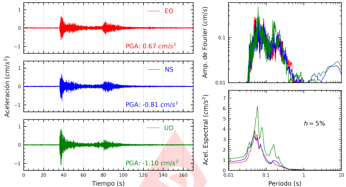
Figura A.5: Registros tiempo-historia, espectros de Fourier y de respuesta en las direcciones EO, NS y vertical de la estación CREY. Sismo de Calana, Tacna - Tacna del 2024-11-03, 16:18:39 (Hora local)
