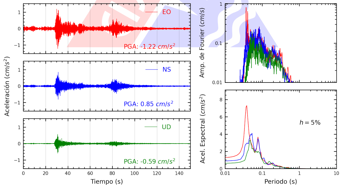
Figura A.4: Registros tiempo-historia, espectros de Fourier y de respuesta en las direcciones EO, NS y vertical de la estación UNAM. Sismo de Calana, Tacna - Tacna del 2024-11-03, 16:18:39 (Hora local)
