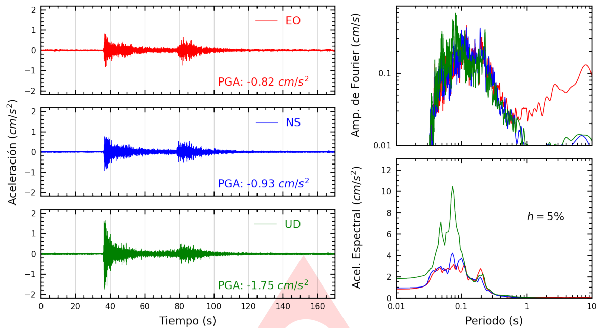
Figura A.1: Registros tiempo-historia, espectros de Fourier y de respuesta en las direcciones EO, NS y vertical de la estación UJBG3. Sismo de Calana, Tacna - Tacna del 2024-11-03, 16:18:39 (Hora local)
