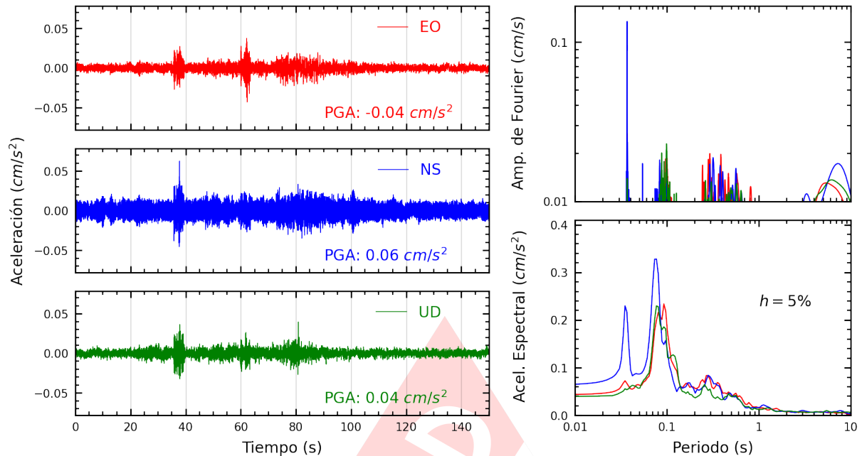
Figura A.5: Registros tiempo-historia, espectros de Fourier y de respuesta en las direcciones EO, NS y vertical de la estación UNJ. Sismo de Sullana, Sullana - Piura del 2024-12-31, 14:07:16 (Hora local)
