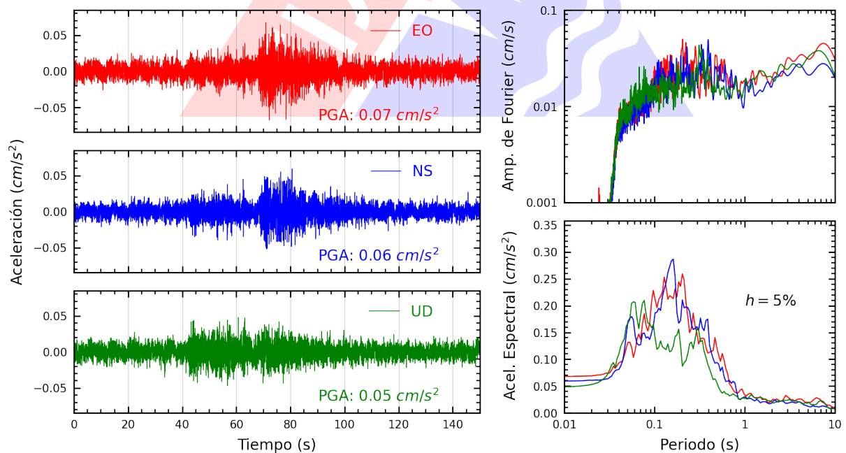
Figura A.4: Registros tiempo-historia, espectros de Fourier y de respuesta en las direcciones EO, NS y vertical de la estación UCVCH. Sismo de Sullana, Sullana - Piura del 2024-12-31, 14:07:16 (Hora local)
