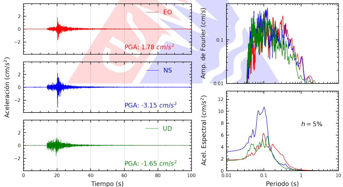
Figura A.2: Registros tiempo-historia, espectros de Fourier y de respuesta en las direcciones EO, NS y vertical de la estación UPAOP. Sismo de Sullana, Sullana - Piura del 2024-12-31, 14:07:16 (Hora local)
