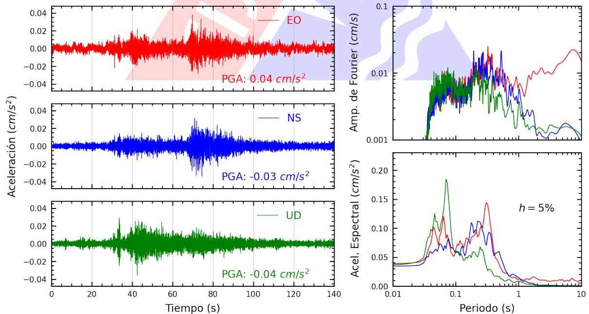
Figura A.6: Registros tiempo-historia, espectros de Fourier y de respuesta en las direcciones EO, NS y vertical de la estación SCCI. Sismo de Sullana, Sullana - Piura del 2024-12-31, 14:07:16 (Hora local)
