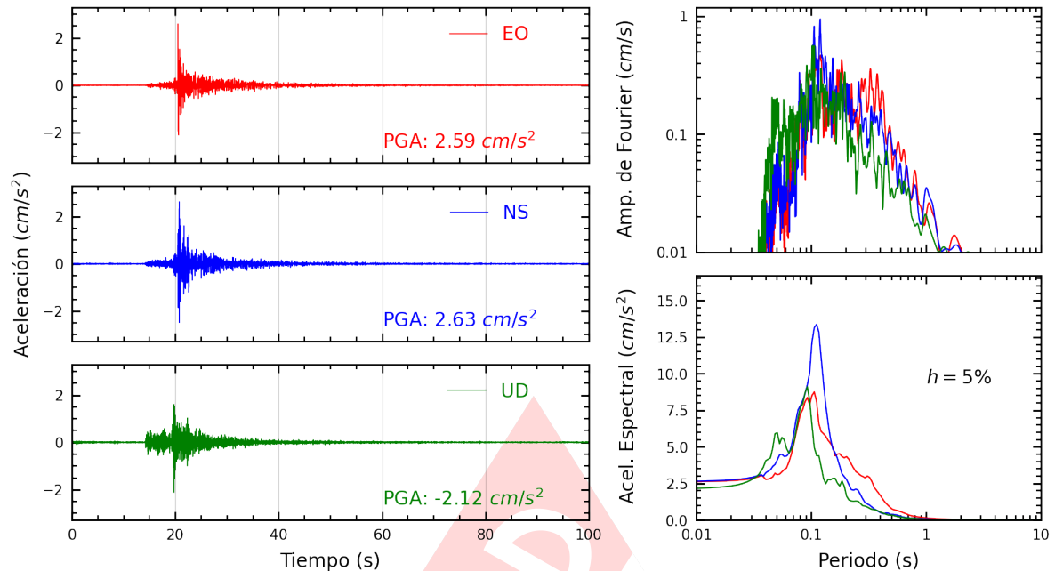
Figura A.3: Registros tiempo-historia, espectros de Fourier y de respuesta en las direcciones EO, NS y vertical de la estación UNP. Sismo de Sullana, Sullana - Piura del 2024-12-31, 14:07:16 (Hora local)
