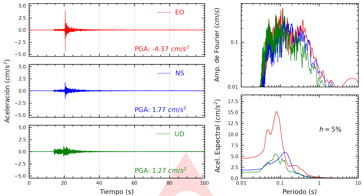
Figura A.1: Registros tiempo-historia, espectros de Fourier y de respuesta en las direcciones EO, NS y vertical de la estación SCPIU. Sismo de Sullana, Sullana - Piura del 2024-12-31, 14:07:16 (Hora local)
