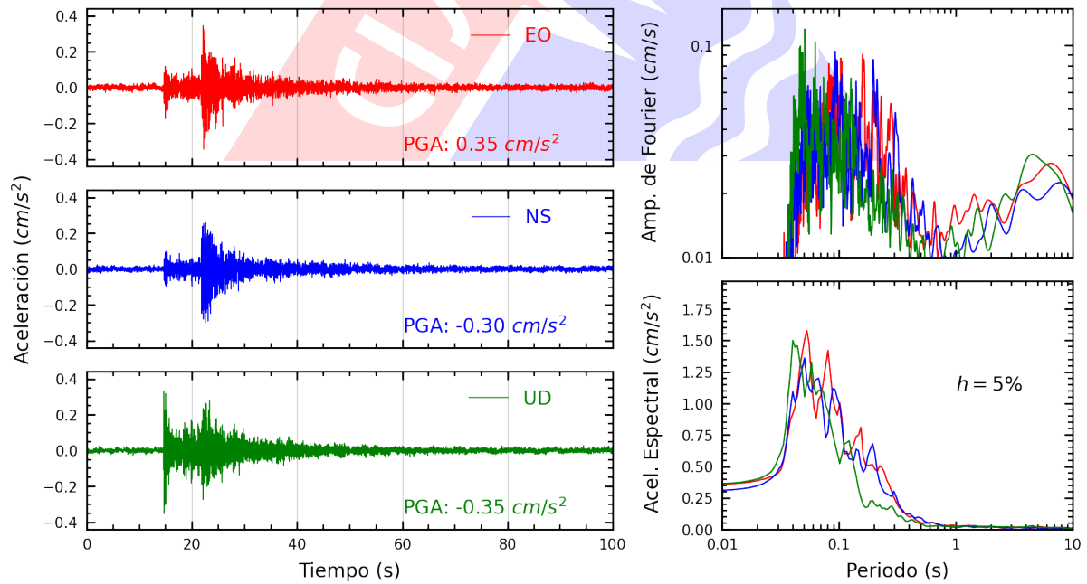
Figura A.22: Registros tiempo-historia, espectros de Fourier y de respuesta en las direcciones EO, NS y vertical de la estación USILP. Sismo de Chilca, Cañete - Lima del 2025-03-02, 07:36:43 (Hora local)
