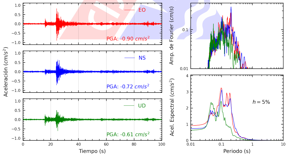
Figura A.6: Registros tiempo-historia, espectros de Fourier y de respuesta en las direcciones EO, NS y vertical de la estación SCCHO. Sismo de Chilca, Cañete - Lima del 2025-03-02, 07:36:43 (Hora local)
