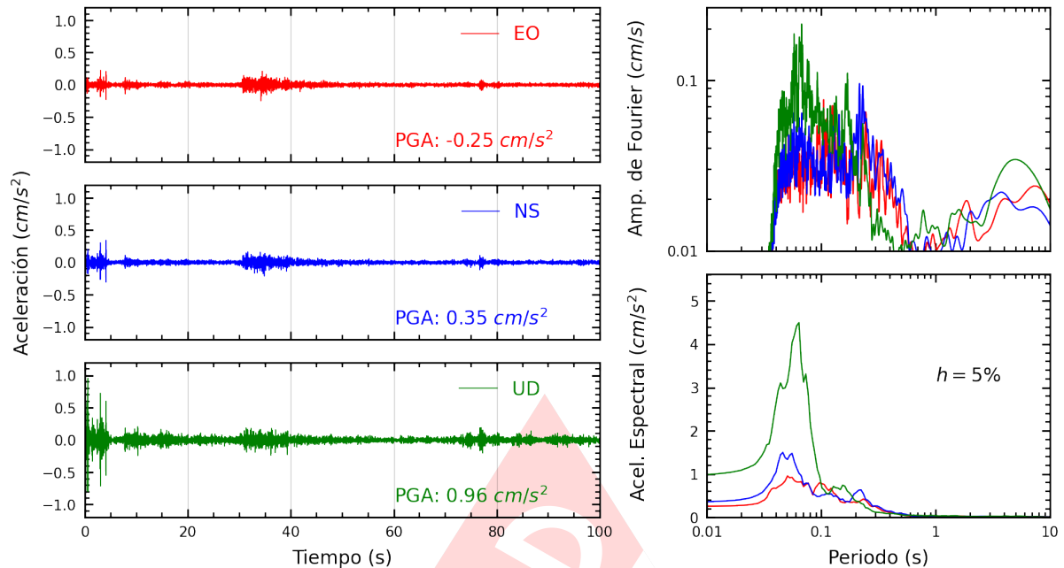
Figura A.5: Registros tiempo-historia, espectros de Fourier y de respuesta en las direcciones EO, NS y vertical de la estación MDPP. Sismo de Chilca, Cañete - Lima del 2025-03-02, 07:36:43 (Hora local)
