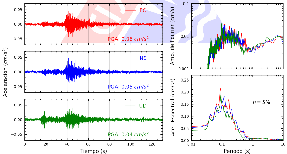
Figura A.32: Registros tiempo-historia, espectros de Fourier y de respuesta en las direcciones EO, NS y vertical de la estación CARAL. Sismo de Chilca, Cañete - Lima del 2025-03-02, 07:36:43 (Hora local)
