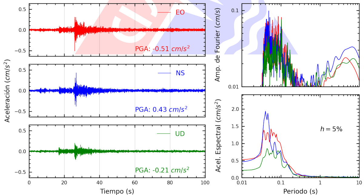
Figura A.16: Registros tiempo-historia, espectros de Fourier y de respuesta en las direcciones EO, NS y vertical de la estación CEPRE. Sismo de Chilca, Cañete - Lima del 2025-03-02, 07:36:43 (Hora local)
