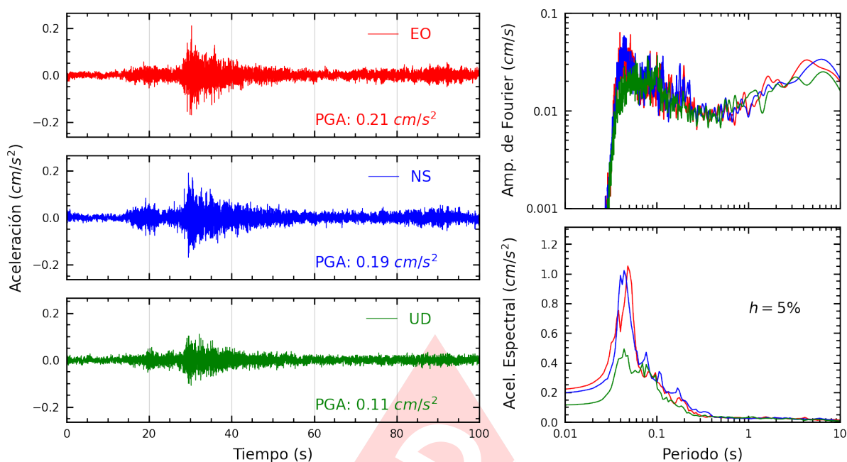
Figura A.25: Registros tiempo-historia, espectros de Fourier y de respuesta en las direcciones EO, NS y vertical de la estación COMAS. Sismo de Chilca, Cañete - Lima del 2025-03-02, 07:36:43 (Hora local)
