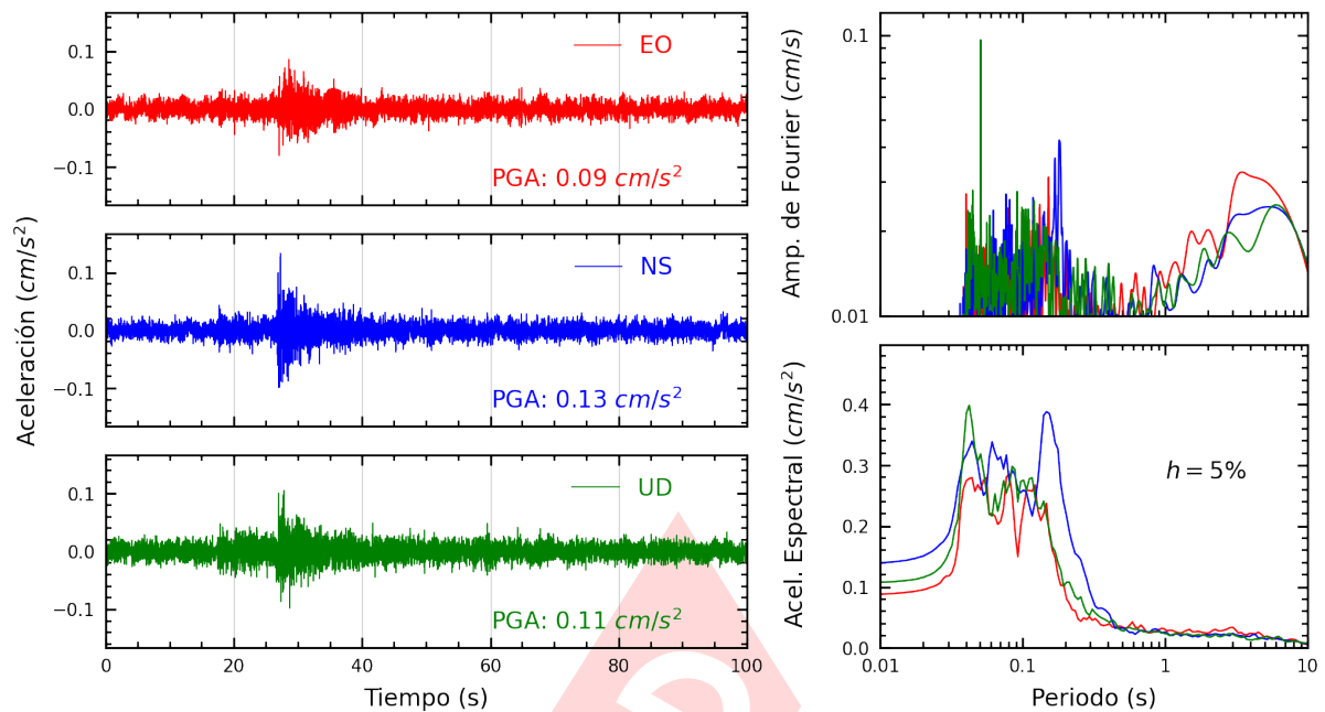
Figura A.31: Registros tiempo-historia, espectros de Fourier y de respuesta en las direcciones EO, NS y vertical de la estación BONDY. Sismo de Chilca, Cañete - Lima del 2025-03-02, 07:36:43 (Hora local)
