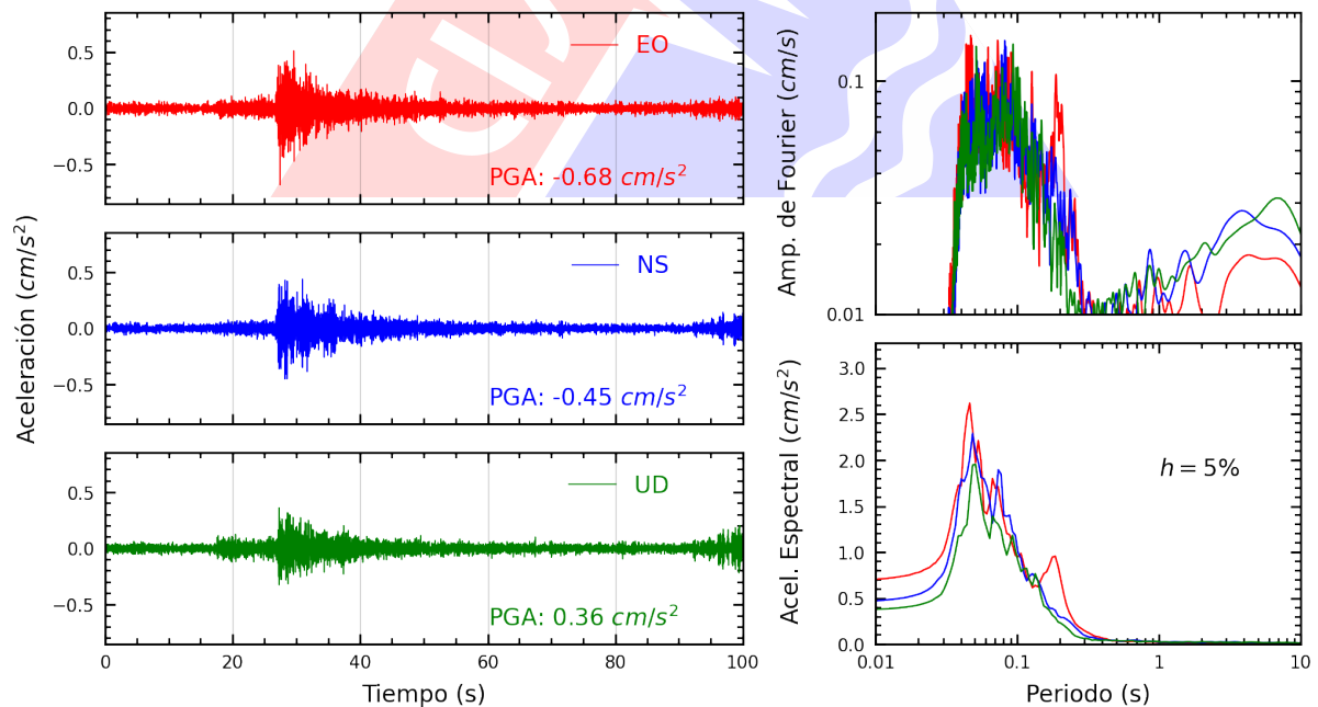
Figura A.12: Registros tiempo-historia, espectros de Fourier y de respuesta en las direcciones EO, NS y vertical de la estación INDEP. Sismo de Chilca, Cañete - Lima del 2025-03-02, 07:36:43 (Hora local)
