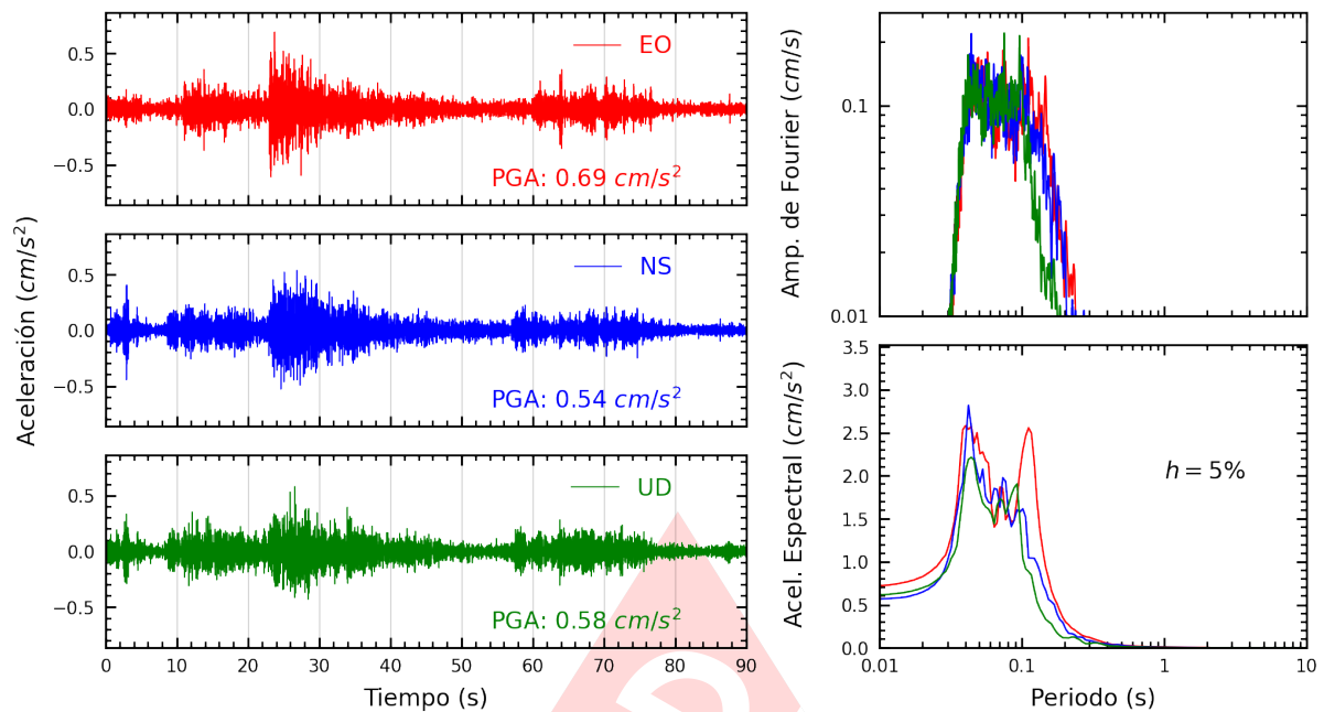
Figura A.11: Registros tiempo-historia, espectros de Fourier y de respuesta en las direcciones EO, NS y vertical de la estación SROS2. Sismo de Chilca, Cañete - Lima del 2025-03-02, 07:36:43 (Hora local)
