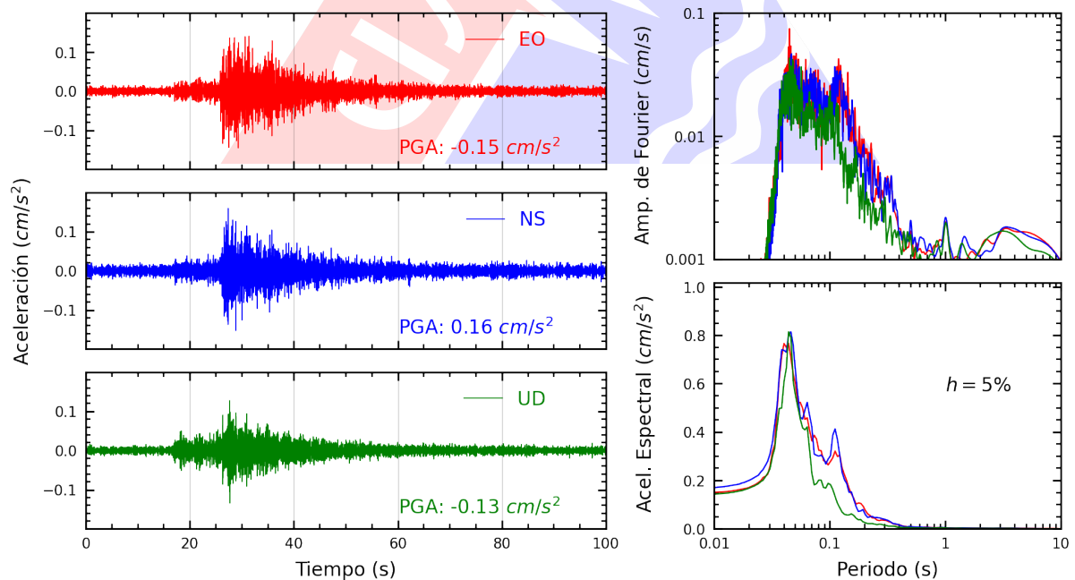
Figura A.30: Registros tiempo-historia, espectros de Fourier y de respuesta en las direcciones EO, NS y vertical de la estación ATARJ. Sismo de Chilca, Cañete - Lima del 2025-03-02, 07:36:43 (Hora local)
