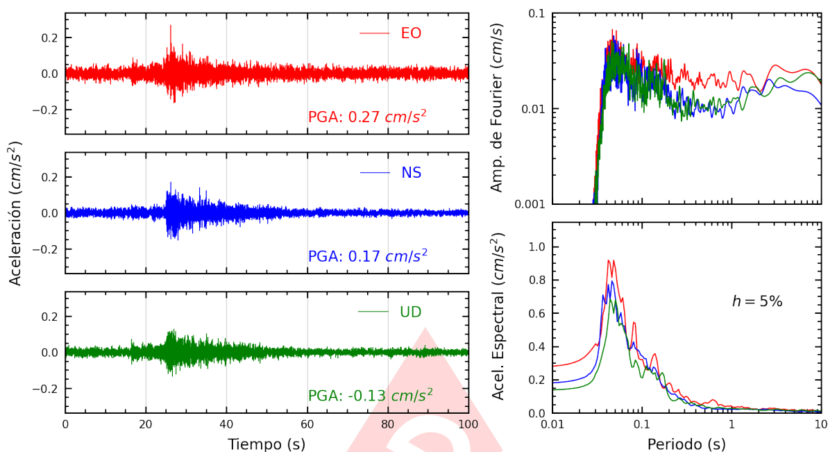
Figura A.23: Registros tiempo-historia, espectros de Fourier y de respuesta en las direcciones EO, NS y vertical de la estación IMCA. Sismo de Chilca, Cañete - Lima del 2025-03-02, 07:36:43 (Hora local)
