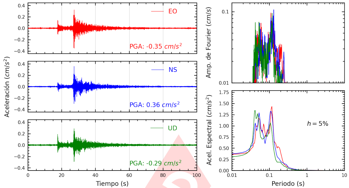
Figura A.21: Registros tiempo-historia, espectros de Fourier y de respuesta en las direcciones EO, NS y vertical de la estación JALV2. Sismo de Chilca, Cañete - Lima del 2025-03-02, 07:36:43 (Hora local)
