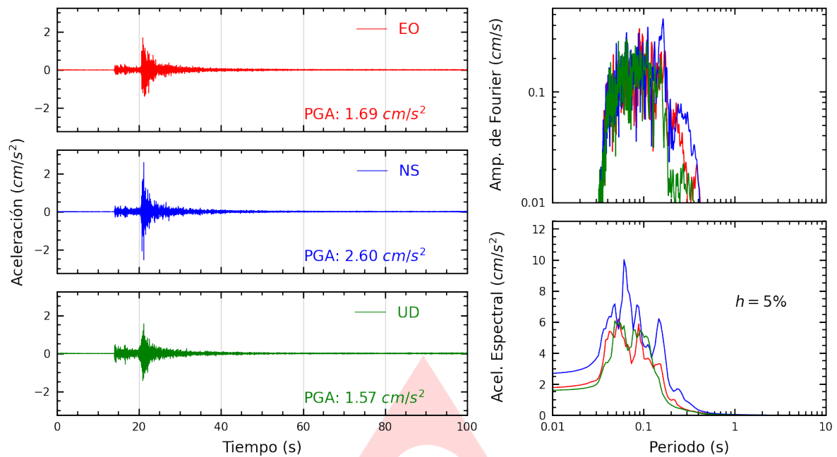
Figura A.1: Registros tiempo-historia, espectros de Fourier y de respuesta en las direcciones EO, NS y vertical de la estación ASIA. Sismo de Chilca, Cañete - Lima del 2025-03-02, 07:36:43 (Hora local)
