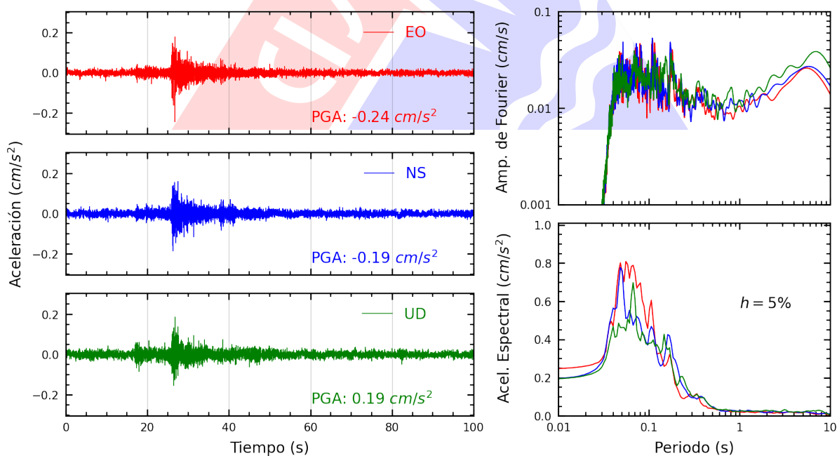
Figura A.24: Registros tiempo-historia, espectros de Fourier y de respuesta en las direcciones EO, NS y vertical de la estación UNFV. Sismo de Chilca, Cañete - Lima del 2025-03-02, 07:36:43 (Hora local)
