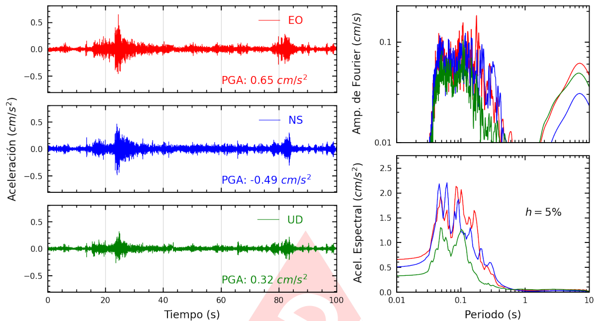
Figura A.13: Registros tiempo-historia, espectros de Fourier y de respuesta en las direcciones EO, NS y vertical de la estación BRISA. Sismo de Chilca, Cañete - Lima del 2025-03-02, 07:36:43 (Hora local)
