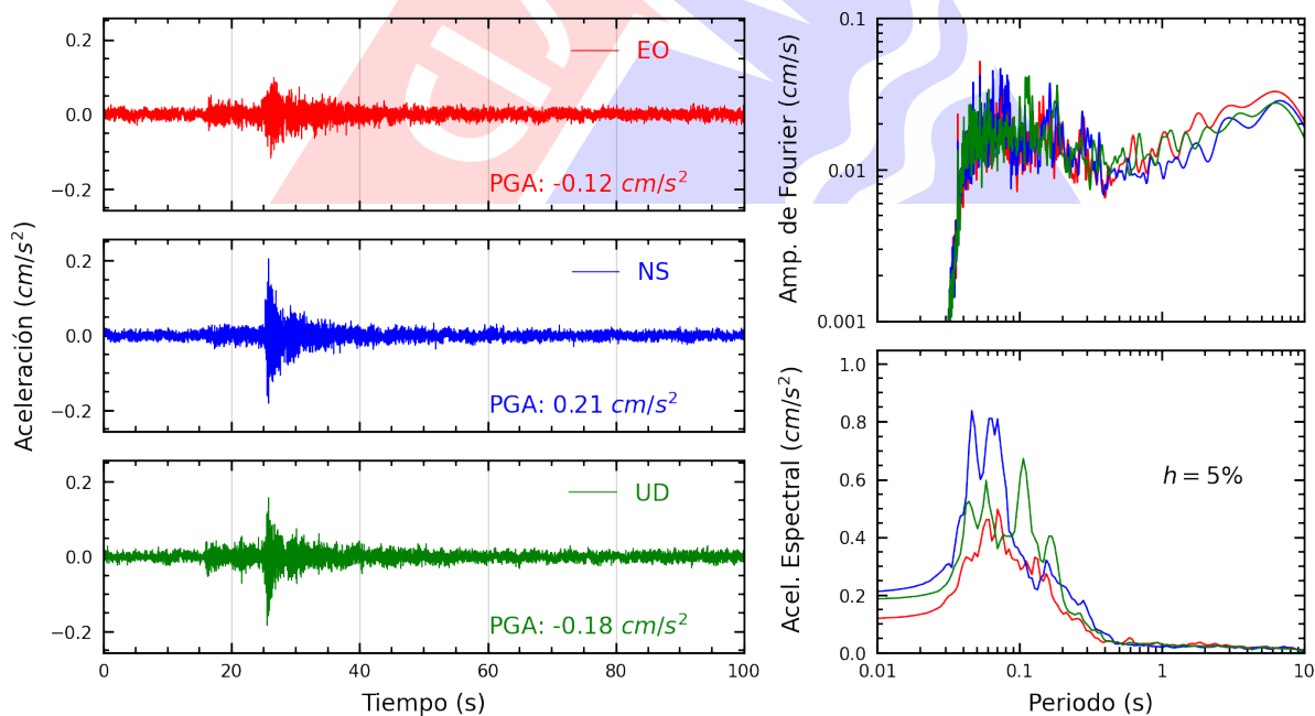
Figura A.26: Registros tiempo-historia, espectros de Fourier y de respuesta en las direcciones EO, NS y vertical de la estación UNMSM. Sismo de Chilca, Cañete - Lima del 2025-03-02, 07:36:43 (Hora local)
