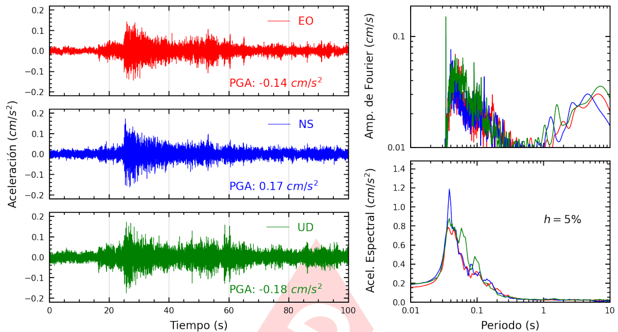
Figura A.29: Registros tiempo-historia, espectros de Fourier y de respuesta en las direcciones EO, NS y vertical de la estación USMP. Sismo de Chilca, Cañete - Lima del 2025-03-02, 07:36:43 (Hora local)
