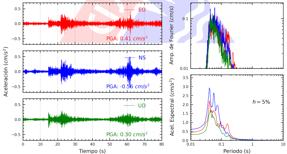
Figura A.14: Registros tiempo-historia, espectros de Fourier y de respuesta en las direcciones EO, NS y vertical de la estación PACHA. Sismo de Chilca, Cañete - Lima del 2025-03-02, 07:36:43 (Hora local)
