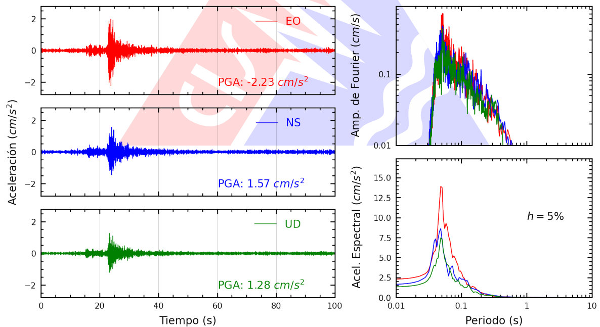
Figura A.2: Registros tiempo-historia, espectros de Fourier y de respuesta en las direcciones EO, NS y vertical de la estación UNTEL. Sismo de Chilca, Cañete - Lima del 2025-03-02, 07:36:43 (Hora local)
