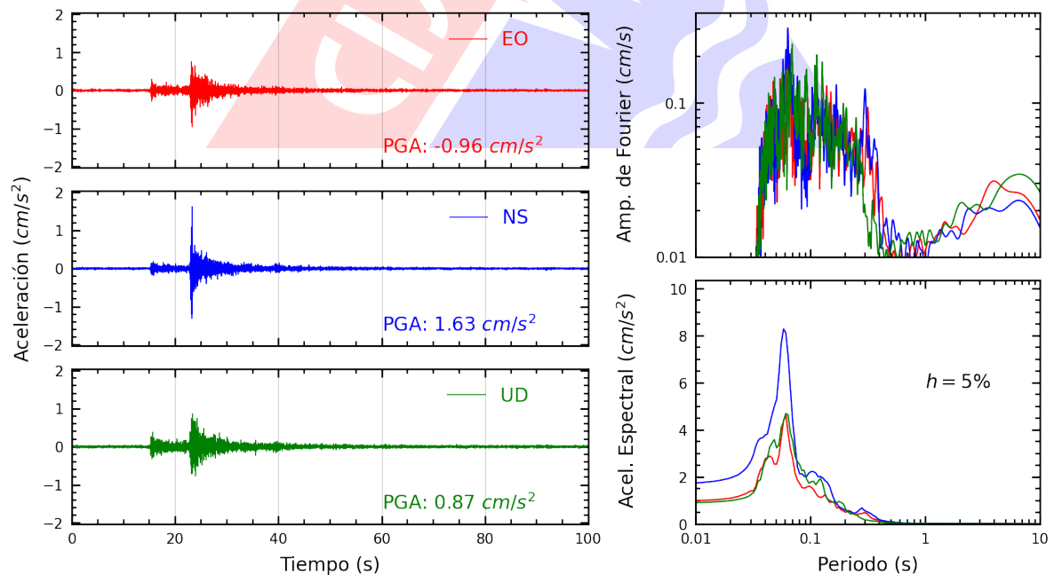
Figura A.4: Registros tiempo-historia, espectros de Fourier y de respuesta en las direcciones EO, NS y vertical de la estación SOVES. Sismo de Chilca, Cañete - Lima del 2025-03-02, 07:36:43 (Hora local)
