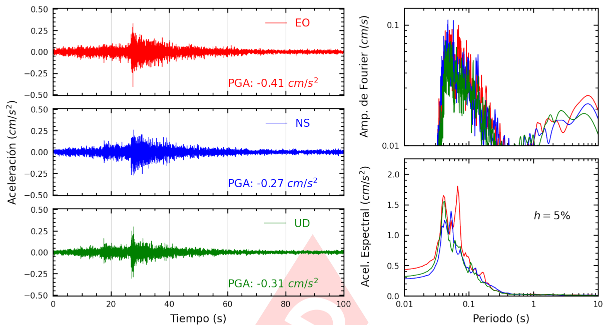
Figura A.19: Registros tiempo-historia, espectros de Fourier y de respuesta en las direcciones EO, NS y vertical de la estación FICPE. Sismo de Chilca, Cañete - Lima del 2025-03-02, 07:36:43 (Hora local)
