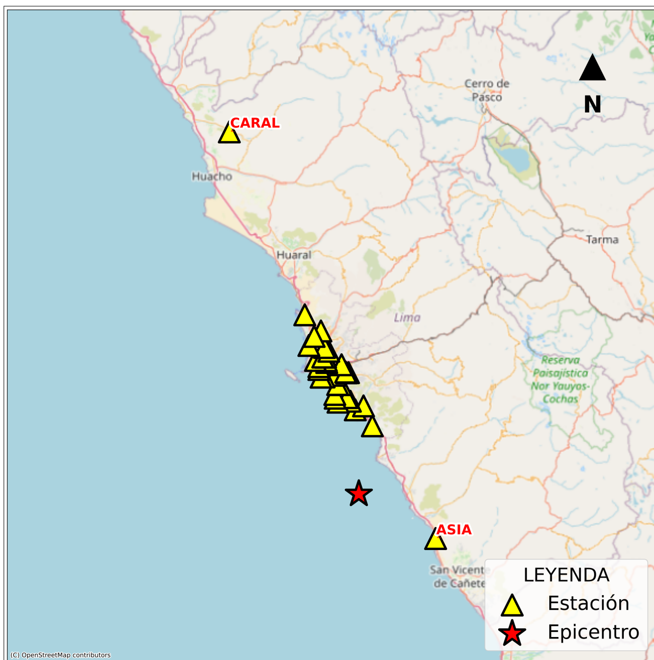
Figura 2: Mapa de ubicación de la(s) estación(es) acelerográfica(s) a nivel nacional correspondiente(s) al Sismo de Chilca, Cañete - Lima del 02 de marzo de 2025 a las 07:36:43 (hora local)
