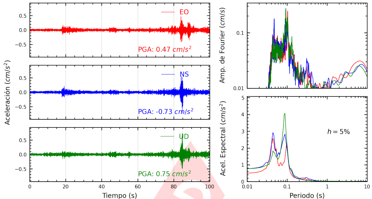
Figura A.9: Registros tiempo-historia, espectros de Fourier y de respuesta en las direcciones EO, NS y vertical de la estación MADRE. Sismo de Chilca, Cañete - Lima del 2025-03-02, 07:36:43 (Hora local)
