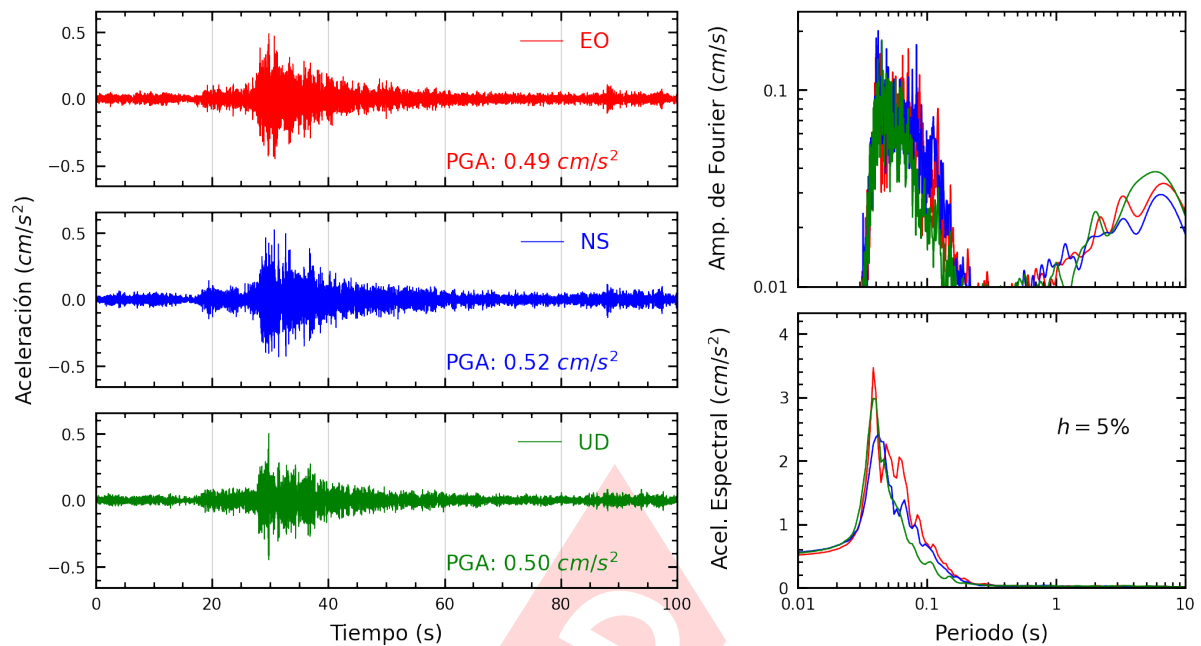
Figura A.15: Registros tiempo-historia, espectros de Fourier y de respuesta en las direcciones EO, NS y vertical de la estación JOSEO. Sismo de Chilca, Cañete - Lima del 2025-03-02, 07:36:43 (Hora local)
