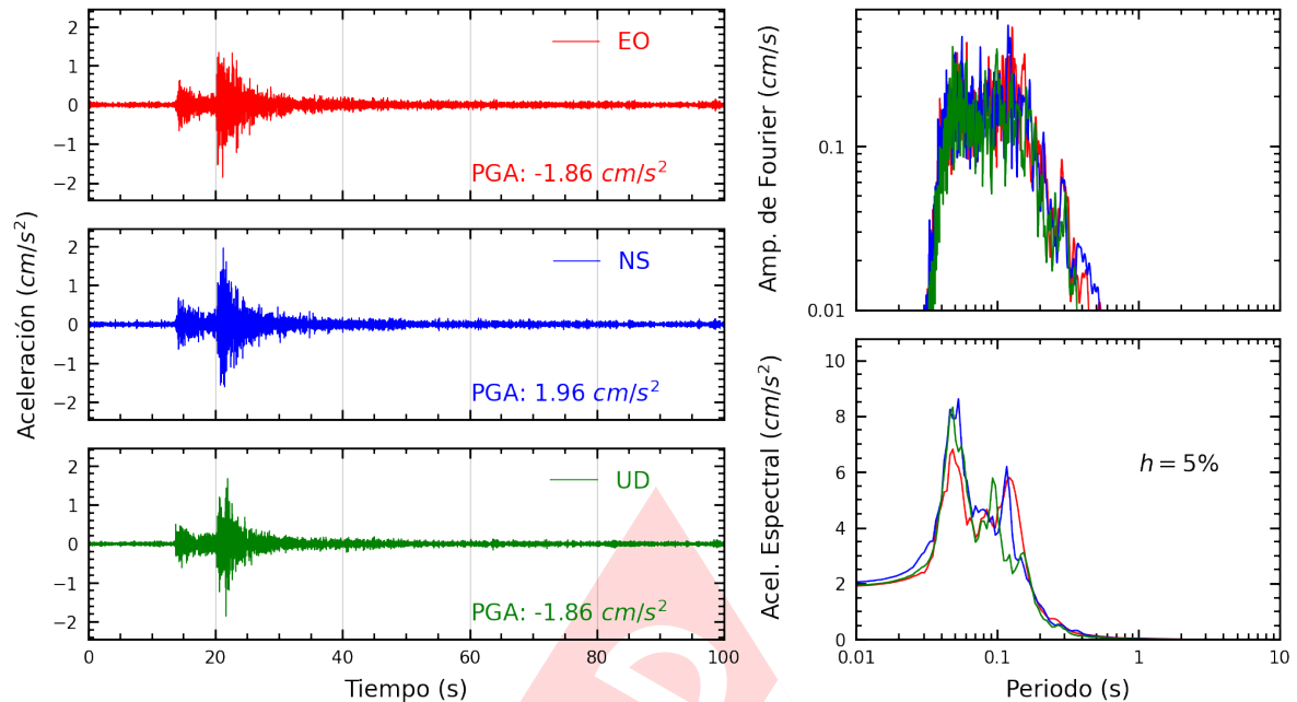
Figura A.3: Registros tiempo-historia, espectros de Fourier y de respuesta en las direcciones EO, NS y vertical de la estación PHER2. Sismo de Chilca, Cañete - Lima del 2025-03-02, 07:36:43 (Hora local)
