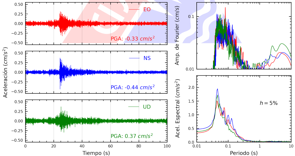
Figura A.18: Registros tiempo-historia, espectros de Fourier y de respuesta en las direcciones EO, NS y vertical de la estación URPPE. Sismo de Chilca, Cañete - Lima del 2025-03-02, 07:36:43 (Hora local)
