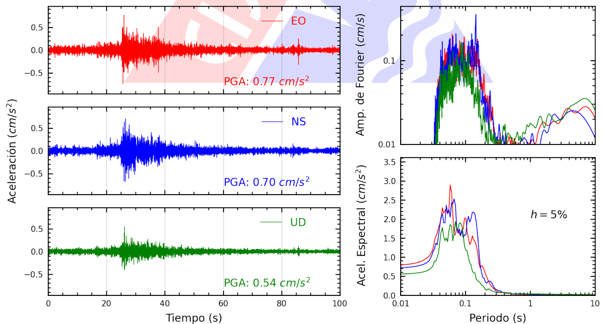
Figura A.8: Registros tiempo-historia, espectros de Fourier y de respuesta en las direcciones EO, NS y vertical de la estación USILM. Sismo de Chilca, Cañete - Lima del 2025-03-02, 07:36:43 (Hora local)
