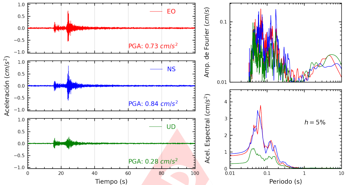
Figura A.7: Registros tiempo-historia, espectros de Fourier y de respuesta en las direcciones EO, NS y vertical de la estación UPCVI. Sismo de Chilca, Cañete - Lima del 2025-03-02, 07:36:43 (Hora local)
