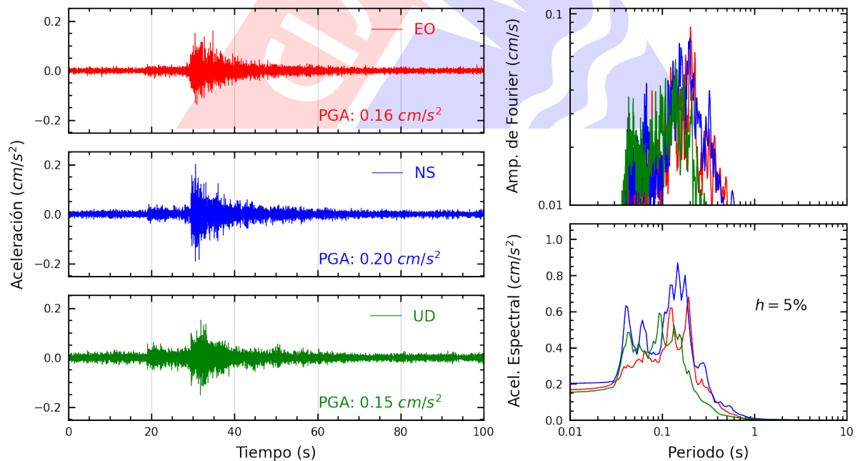
Figura A.28: Registros tiempo-historia, espectros de Fourier y de respuesta en las direcciones EO, NS y vertical de la estación VHAY2. Sismo de Chilca, Cañete - Lima del 2025-03-02, 07:36:43 (Hora local)
