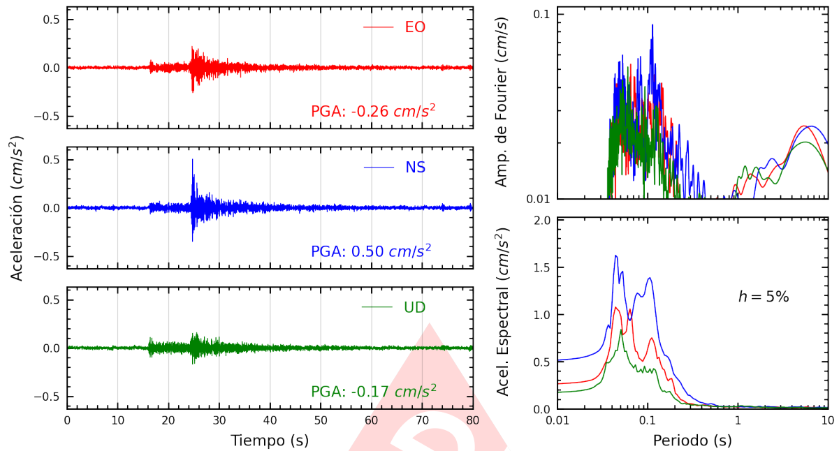
Figura A.17: Registros tiempo-historia, espectros de Fourier y de respuesta en las direcciones EO, NS y vertical de la estación SERVI. Sismo de Chilca, Cañete - Lima del 2025-03-02, 07:36:43 (Hora local)
