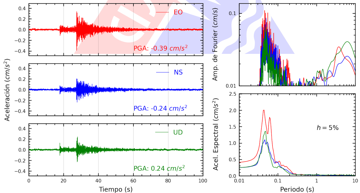
Figura A.20: Registros tiempo-historia, espectros de Fourier y de respuesta en las direcciones EO, NS y vertical de la estación UCSS. Sismo de Chilca, Cañete - Lima del 2025-03-02, 07:36:43 (Hora local)
