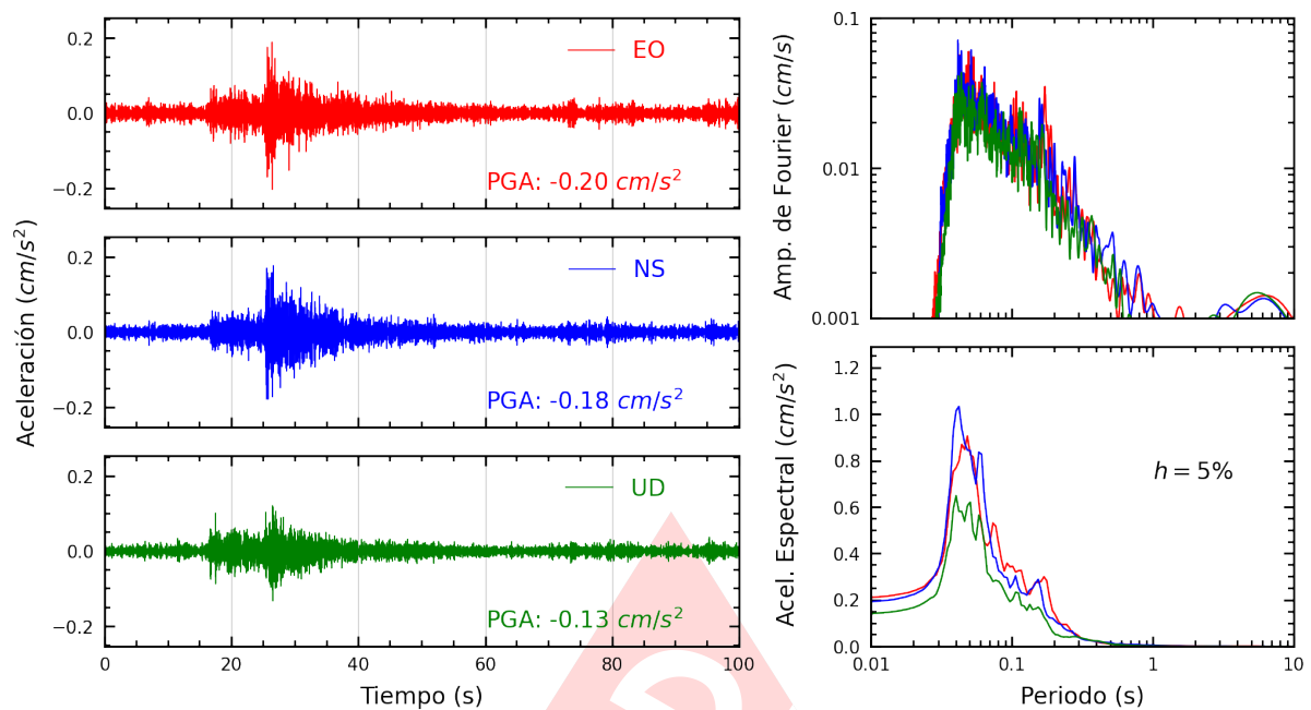
Figura A.27: Registros tiempo-historia, espectros de Fourier y de respuesta en las direcciones EO, NS y vertical de la estación BORJA. Sismo de Chilca, Cañete - Lima del 2025-03-02, 07:36:43 (Hora local)
