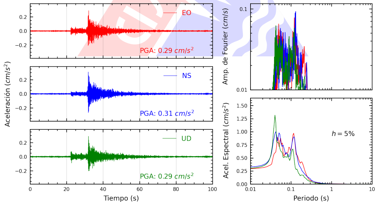
Figura A.20: Registros tiempo-historia, espectros de Fourier y de respuesta en las direcciones EO, NS y vertical de la estación JALV2. Sismo de Chilca, Cañete - Lima del 2025-03-02, 08:58:18 (Hora local)
