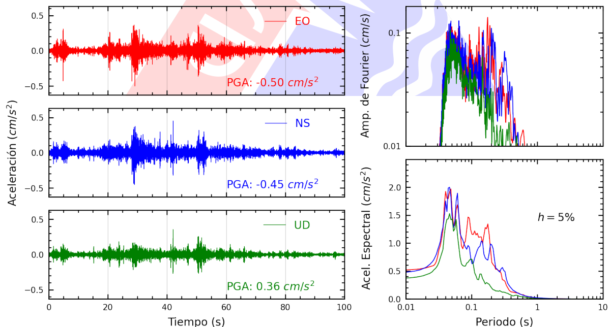
Figura A.10: Registros tiempo-historia, espectros de Fourier y de respuesta en las direcciones EO, NS y vertical de la estación BRISA. Sismo de Chilca, Cañete - Lima del 2025-03-02, 08:58:18 (Hora local)
