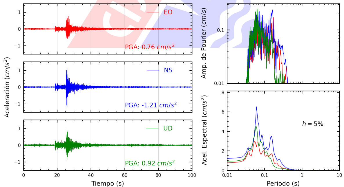
Figura A.4: Registros tiempo-historia, espectros de Fourier y de respuesta en las direcciones EO, NS y vertical de la estación ASIA. Sismo de Chilca, Cañete - Lima del 2025-03-02, 08:58:18 (Hora local)
