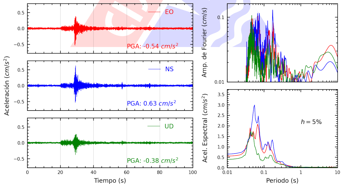
Figura A.8: Registros tiempo-historia, espectros de Fourier y de respuesta en las direcciones EO, NS y vertical de la estación UPCVI. Sismo de Chilca, Cañete - Lima del 2025-03-02, 08:58:18 (Hora local)
