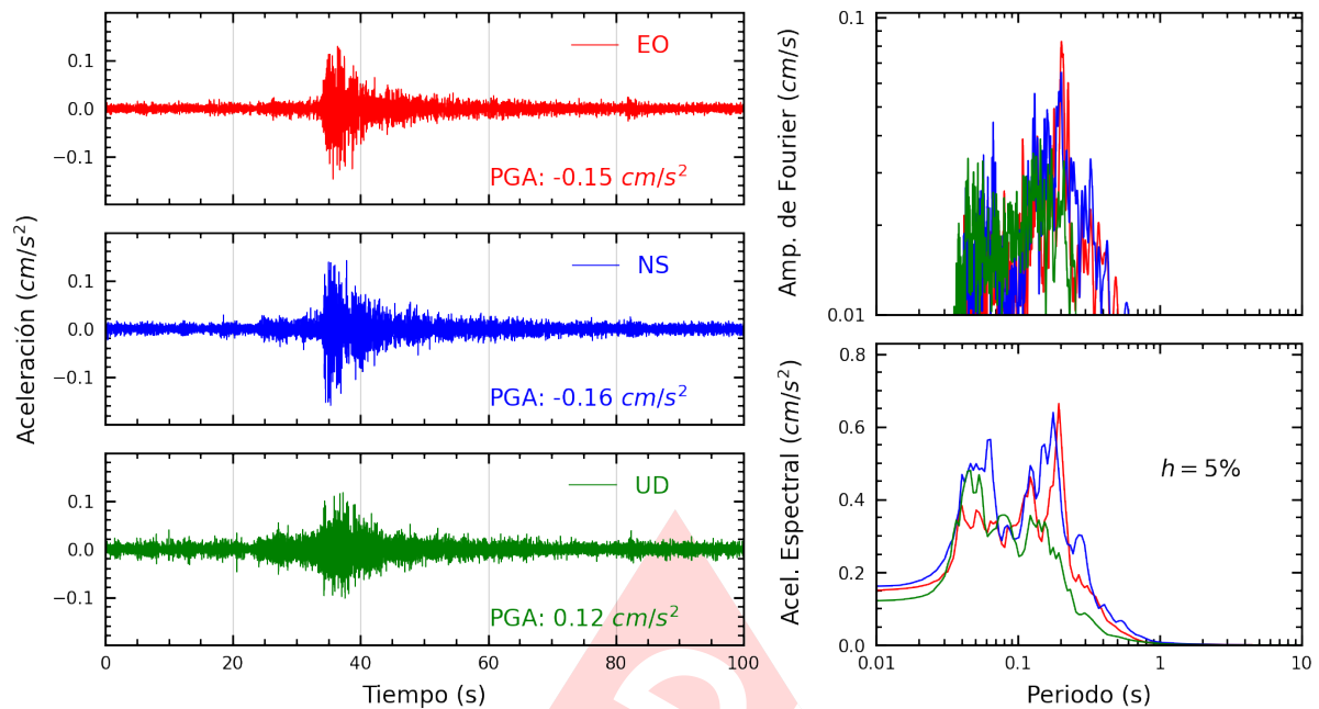
Figura A.29: Registros tiempo-historia, espectros de Fourier y de respuesta en las direcciones EO, NS y vertical de la estación VHAY2. Sismo de Chilca, Cañete - Lima del 2025-03-02, 08:58:18 (Hora local)
