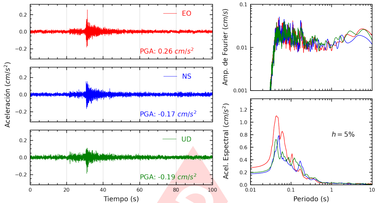
Figura A.21: Registros tiempo-historia, espectros de Fourier y de respuesta en las direcciones EO, NS y vertical de la estación UNFV. Sismo de Chilca, Cañete - Lima del 2025-03-02, 08:58:18 (Hora local)
