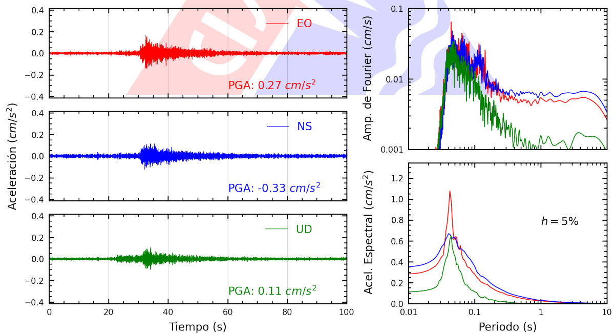
Figura A.18: Registros tiempo-historia, espectros de Fourier y de respuesta en las direcciones EO, NS y vertical de la estación ATARJ. Sismo de Chilca, Cañete - Lima del 2025-03-02, 08:58:18 (Hora local)
