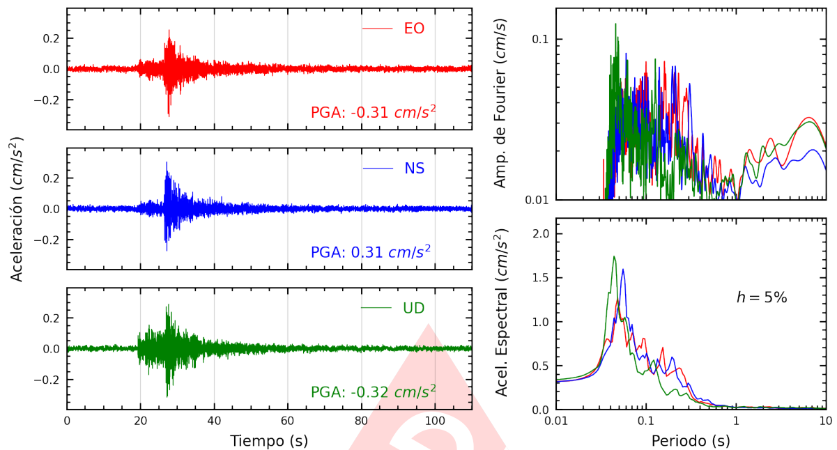
Figura A.19: Registros tiempo-historia, espectros de Fourier y de respuesta en las direcciones EO, NS y vertical de la estación USILP. Sismo de Chilca, Cañete - Lima del 2025-03-02, 08:58:18 (Hora local)
