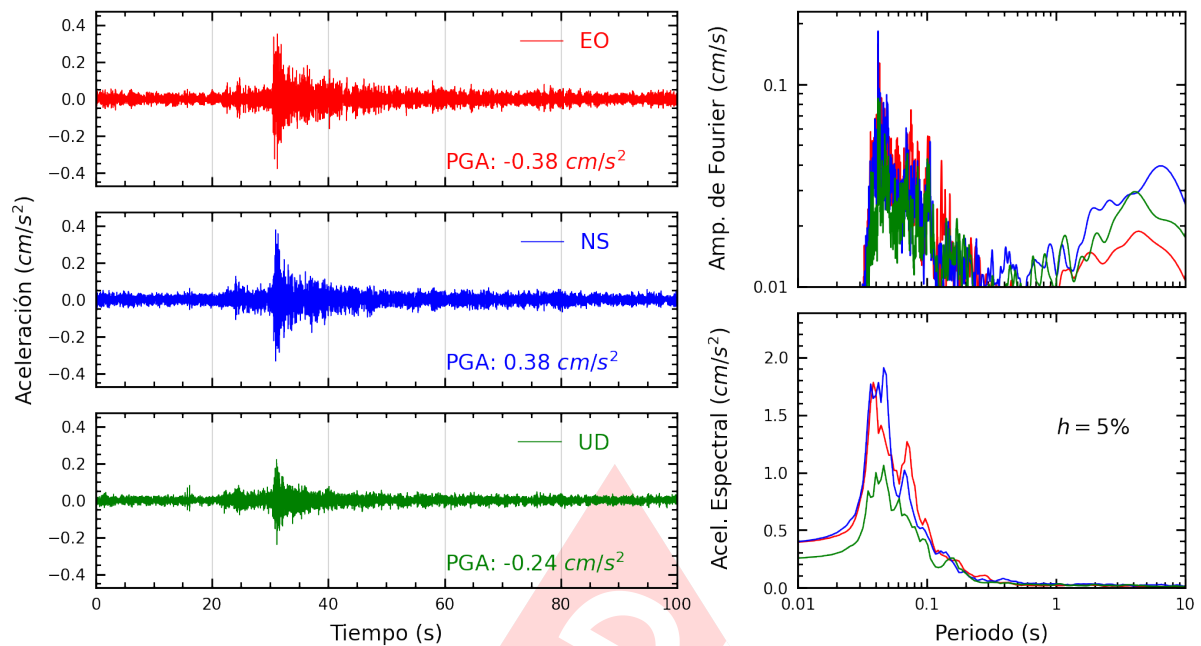
Figura A.15: Registros tiempo-historia, espectros de Fourier y de respuesta en las direcciones EO, NS y vertical de la estación CEPRE. Sismo de Chilca, Cañete - Lima del 2025-03-02, 08:58:18 (Hora local)
