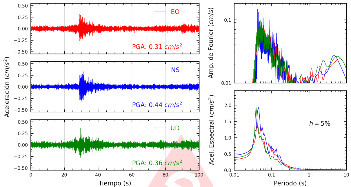
Figura A.13: Registros tiempo-historia, espectros de Fourier y de respuesta en las direcciones EO, NS y vertical de la estación URPPE. Sismo de Chilca, Cañete - Lima del 2025-03-02, 08:58:18 (Hora local)
