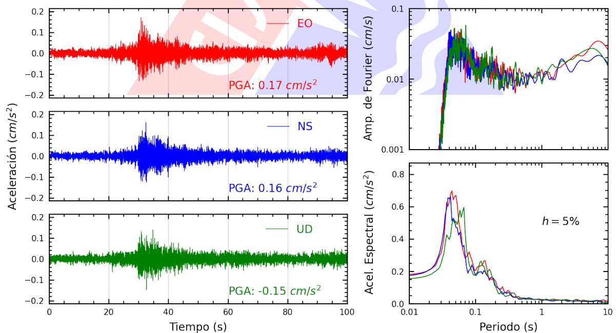
Figura A.26: Registros tiempo-historia, espectros de Fourier y de respuesta en las direcciones EO, NS y vertical de la estación IMCA. Sismo de Chilca, Cañete - Lima del 2025-03-02, 08:58:18 (Hora local)
