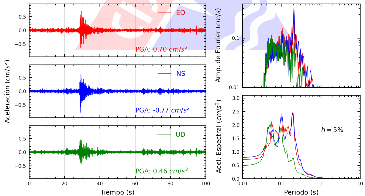
Figura A.6: Registros tiempo-historia, espectros de Fourier y de respuesta en las direcciones EO, NS y vertical de la estación SCCHO. Sismo de Chilca, Cañete - Lima del 2025-03-02, 08:58:18 (Hora local)
