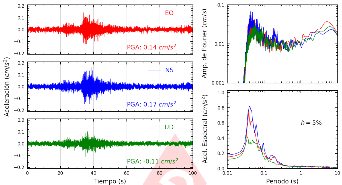
Figura A.27: Registros tiempo-historia, espectros de Fourier y de respuesta en las direcciones EO, NS y vertical de la estación COMAS. Sismo de Chilca, Cañete - Lima del 2025-03-02, 08:58:18 (Hora local)
