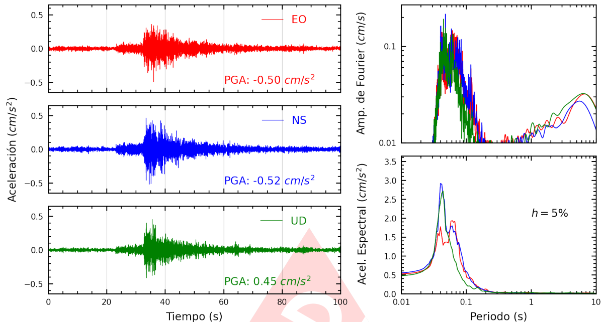
Figura A.9: Registros tiempo-historia, espectros de Fourier y de respuesta en las direcciones EO, NS y vertical de la estación JOSEO. Sismo de Chilca, Cañete - Lima del 2025-03-02, 08:58:18 (Hora local)
