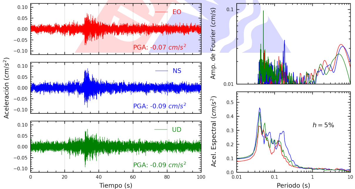
Figura A.30: Registros tiempo-historia, espectros de Fourier y de respuesta en las direcciones EO, NS y vertical de la estación BONDY. Sismo de Chilca, Cañete - Lima del 2025-03-02, 08:58:18 (Hora local)
