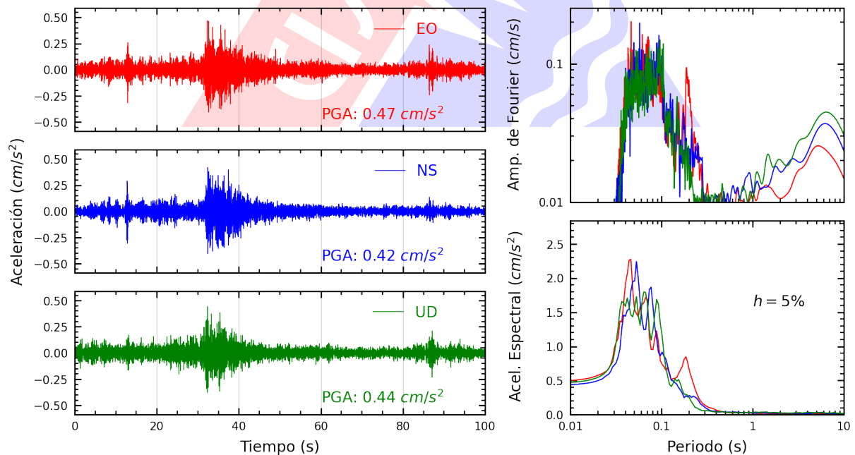
Figura A.12: Registros tiempo-historia, espectros de Fourier y de respuesta en las direcciones EO, NS y vertical de la estación INDEP. Sismo de Chilca, Cañete - Lima del 2025-03-02, 08:58:18 (Hora local)
