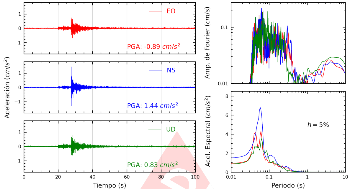
Figura A.3: Registros tiempo-historia, espectros de Fourier y de respuesta en las direcciones EO, NS y vertical de la estación SOVES. Sismo de Chilca, Cañete - Lima del 2025-03-02, 08:58:18 (Hora local)
