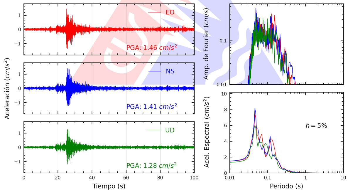
Figura A.2: Registros tiempo-historia, espectros de Fourier y de respuesta en las direcciones EO, NS y vertical de la estación PHER2. Sismo de Chilca, Cañete - Lima del 2025-03-02, 08:58:18 (Hora local)
