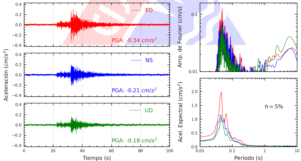
Figura A.16: Registros tiempo-historia, espectros de Fourier y de respuesta en las direcciones EO, NS y vertical de la estación UCSS. Sismo de Chilca, Cañete - Lima del 2025-03-02, 08:58:18 (Hora local)
