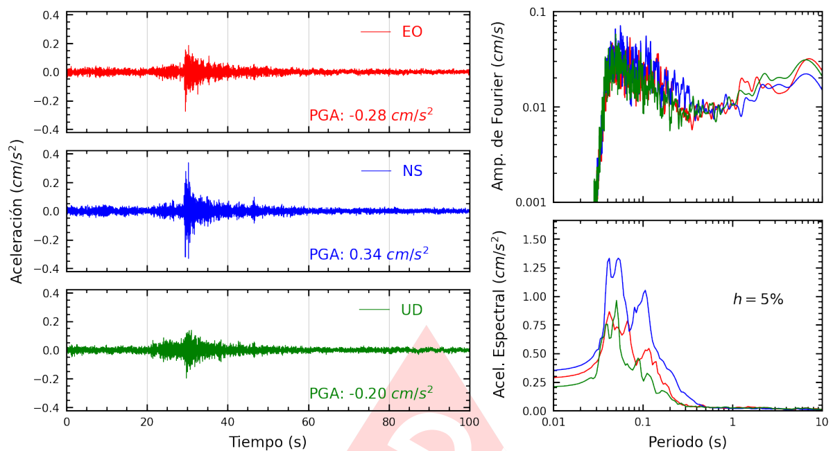
Figura A.17: Registros tiempo-historia, espectros de Fourier y de respuesta en las direcciones EO, NS y vertical de la estación SERVI. Sismo de Chilca, Cañete - Lima del 2025-03-02, 08:58:18 (Hora local)
