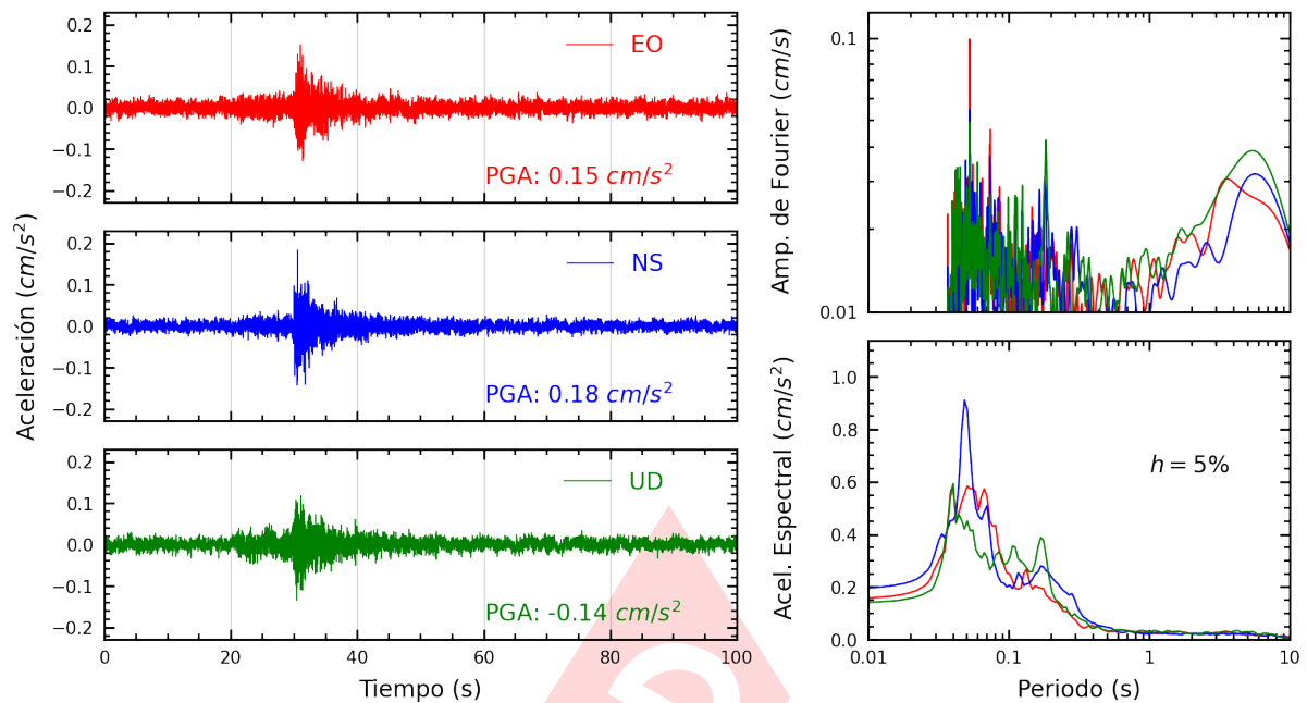
Figura A.25: Registros tiempo-historia, espectros de Fourier y de respuesta en las direcciones EO, NS y vertical de la estación UNMSM. Sismo de Chilca, Cañete - Lima del 2025-03-02, 08:58:18 (Hora local)
