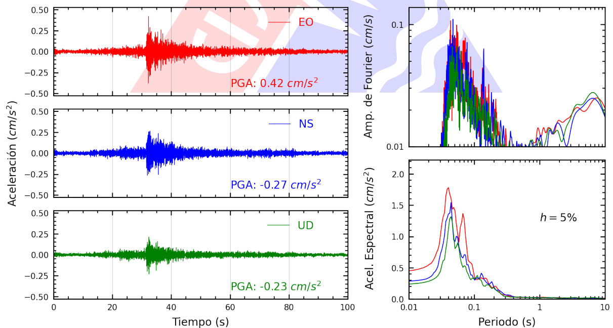
Figura A.14: Registros tiempo-historia, espectros de Fourier y de respuesta en las direcciones EO, NS y vertical de la estación FICPE. Sismo de Chilca, Cañete - Lima del 2025-03-02, 08:58:18 (Hora local)
