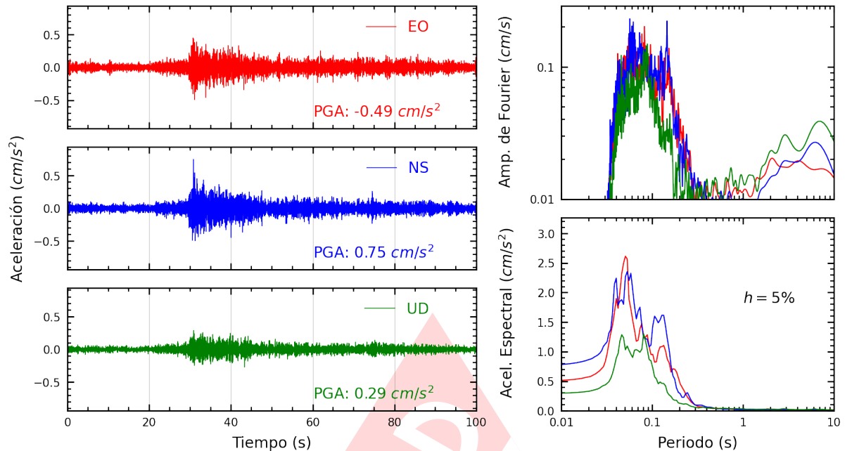
Figura A.7: Registros tiempo-historia, espectros de Fourier y de respuesta en las direcciones EO, NS y vertical de la estación USILM. Sismo de Chilca, Cañete - Lima del 2025-03-02, 08:58:18 (Hora local)
