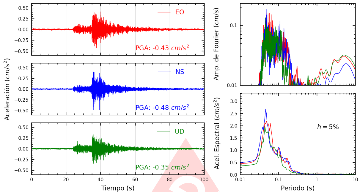
Figura A.11: Registros tiempo-historia, espectros de Fourier y de respuesta en las direcciones EO, NS y vertical de la estación AMORE. Sismo de Chilca, Cañete - Lima del 2025-03-02, 08:58:18 (Hora local)
