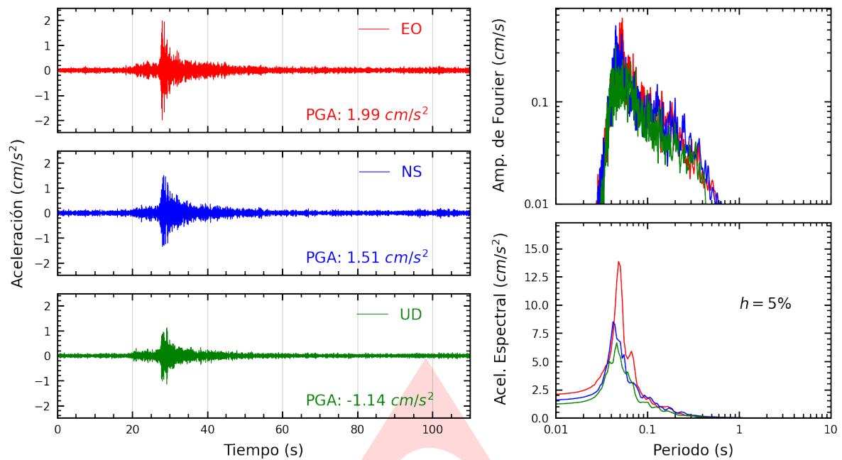
Figura A.1: Registros tiempo-historia, espectros de Fourier y de respuesta en las direcciones EO, NS y vertical de la estación UNTEL. Sismo de Chilca, Cañete - Lima del 2025-03-02, 08:58:18 (Hora local)
