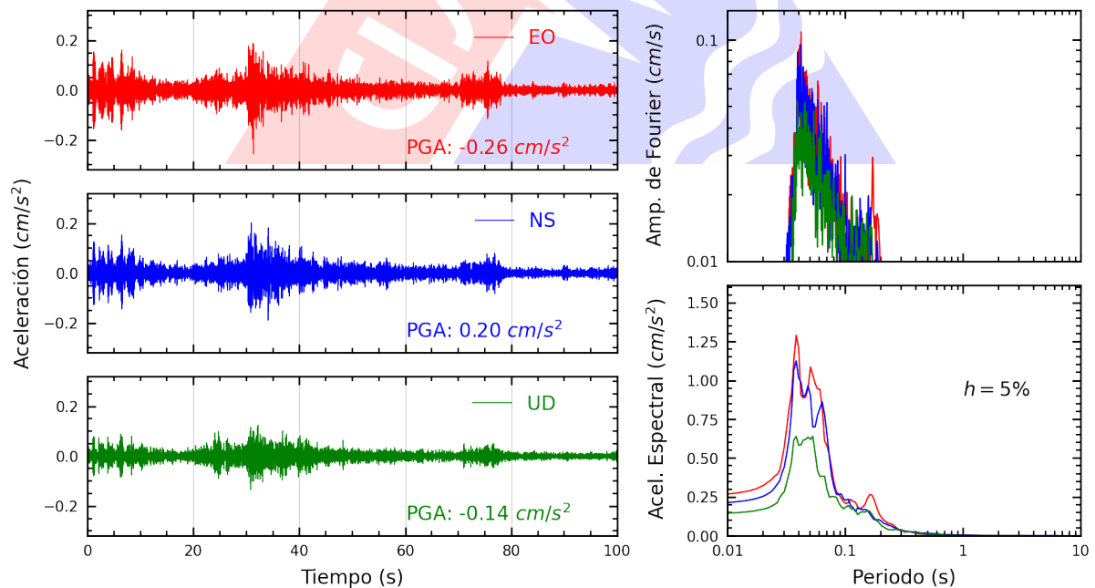
Figura A.22: Registros tiempo-historia, espectros de Fourier y de respuesta en las direcciones EO, NS y vertical de la estación BORJA. Sismo de Chilca, Cañete - Lima del 2025-03-02, 08:58:18 (Hora local)
