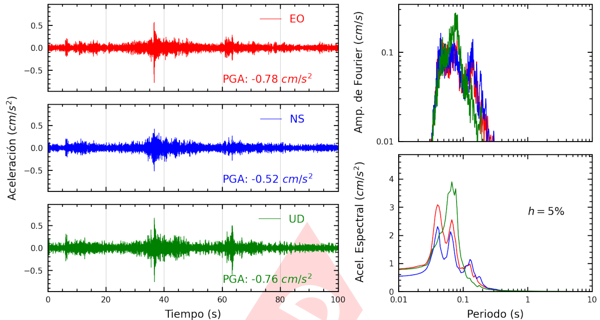
Figura A.5: Registros tiempo-historia, espectros de Fourier y de respuesta en las direcciones EO, NS y vertical de la estación CARA2. Sismo de Chilca, Cañete - Lima del 2025-03-02, 08:58:18 (Hora local)
