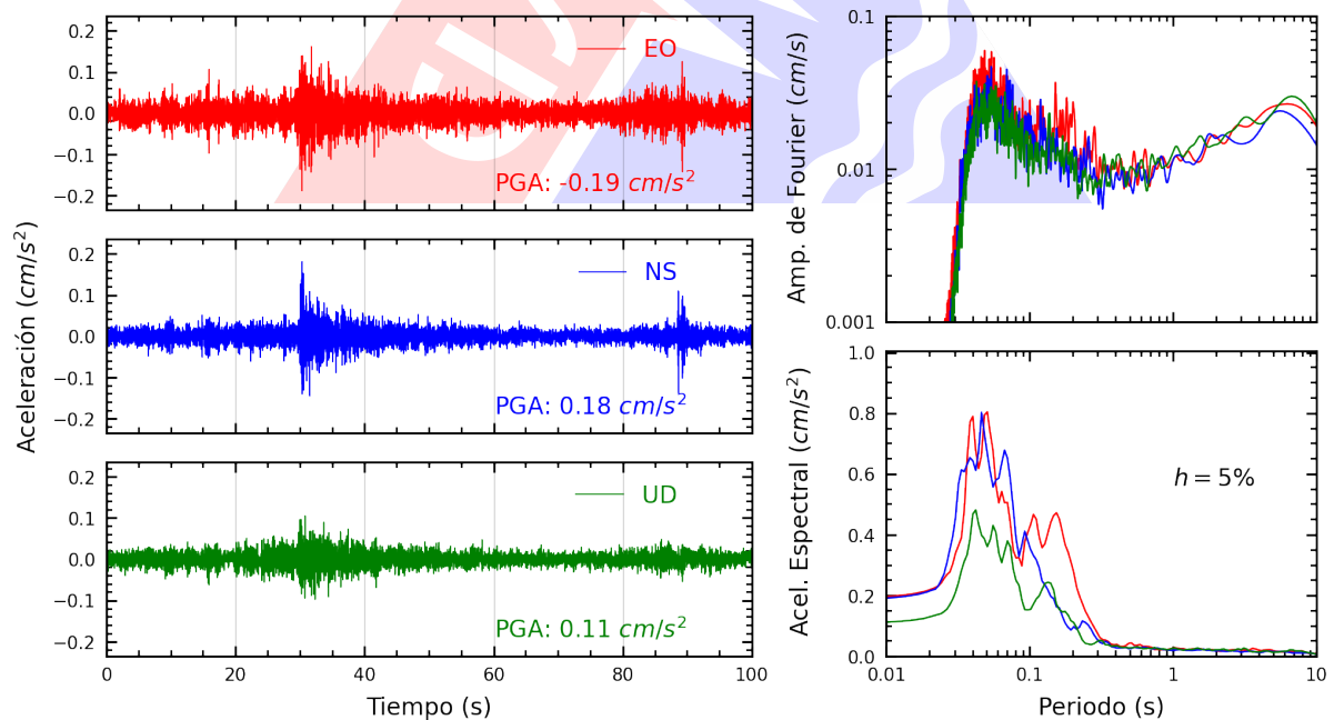
Figura A.24: Registros tiempo-historia, espectros de Fourier y de respuesta en las direcciones EO, NS y vertical de la estación INICT. Sismo de Chilca, Cañete - Lima del 2025-03-02, 08:58:18 (Hora local)
