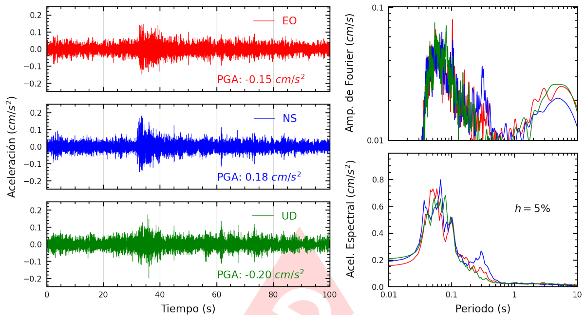
Figura A.23: Registros tiempo-historia, espectros de Fourier y de respuesta en las direcciones EO, NS y vertical de la estación MADRE. Sismo de Chilca, Cañete - Lima del 2025-03-02, 08:58:18 (Hora local)
