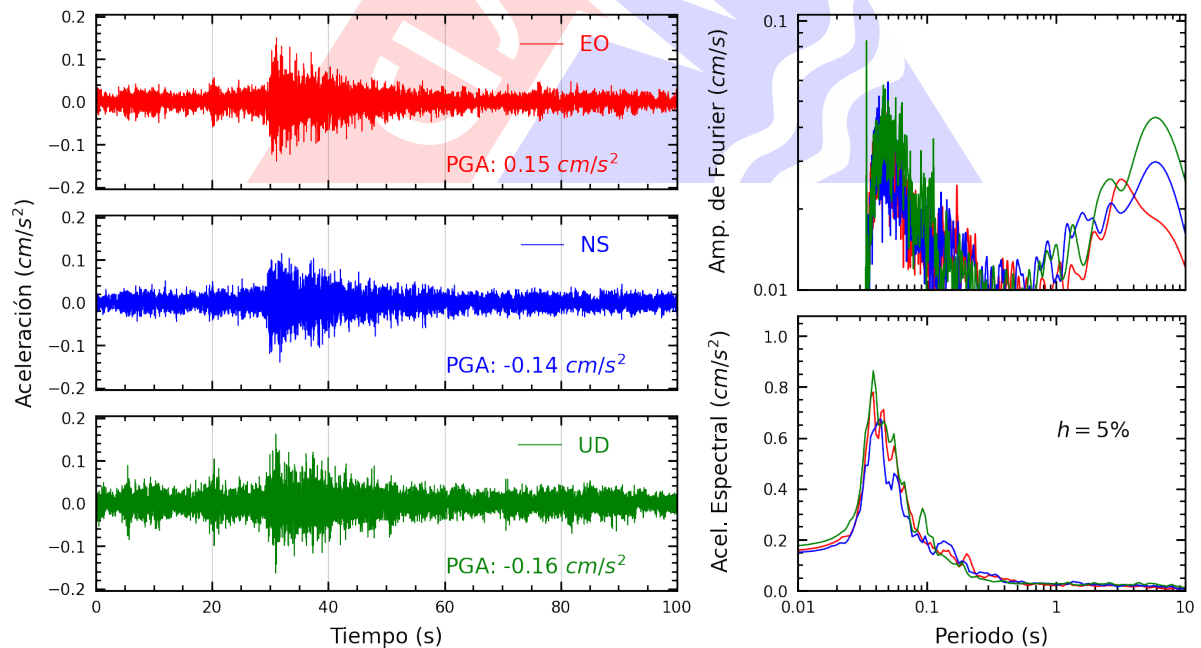
Figura A.28: Registros tiempo-historia, espectros de Fourier y de respuesta en las direcciones EO, NS y vertical de la estación USMP. Sismo de Chilca, Cañete - Lima del 2025-03-02, 08:58:18 (Hora local)
