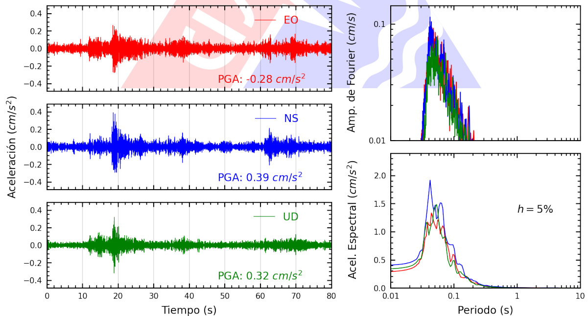
Figura A.18: Registros tiempo-historia, espectros de Fourier y de respuesta en las direcciones EO, NS y vertical de la estación BORJA. Sismo de Chilca, Cañete - Lima del 2025-03-03, 07:30:50 (Hora local)
