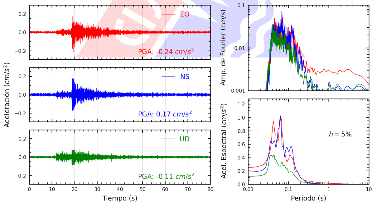
Figura A.26: Registros tiempo-historia, espectros de Fourier y de respuesta en las direcciones EO, NS y vertical de la estación ATARJ. Sismo de Chilca, Cañete - Lima del 2025-03-03, 07:30:50 (Hora local)
