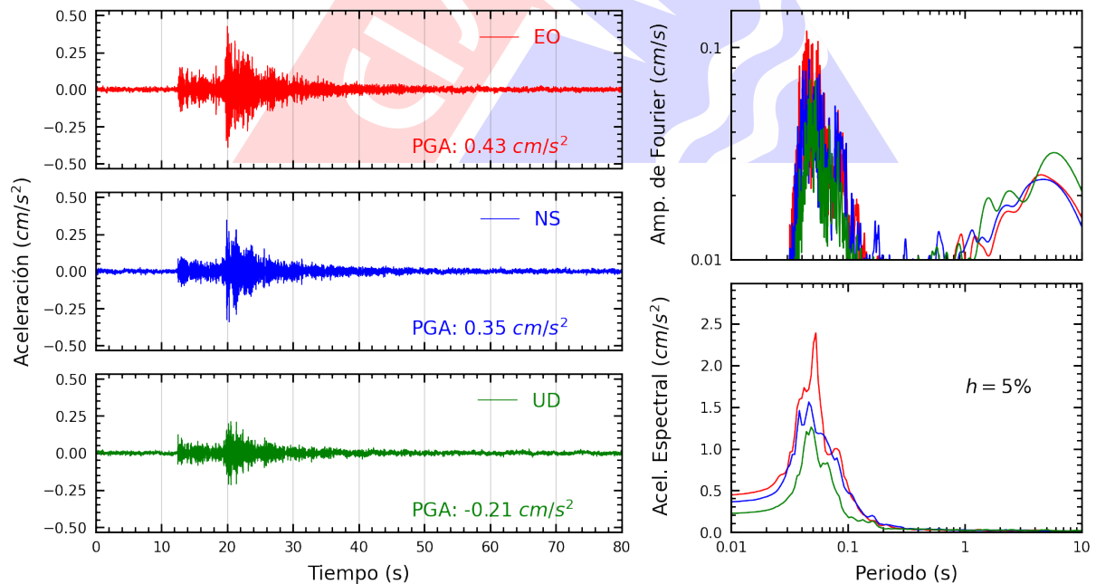
Figura A.16: Registros tiempo-historia, espectros de Fourier y de respuesta en las direcciones EO, NS y vertical de la estación UCSS. Sismo de Chilca, Cañete - Lima del 2025-03-03, 07:30:50 (Hora local)
