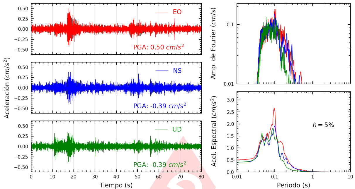
Figura A.13: Registros tiempo-historia, espectros de Fourier y de respuesta en las direcciones EO, NS y vertical de la estación SCCHO. Sismo de Chilca, Cañete - Lima del 2025-03-03, 07:30:50 (Hora local)
