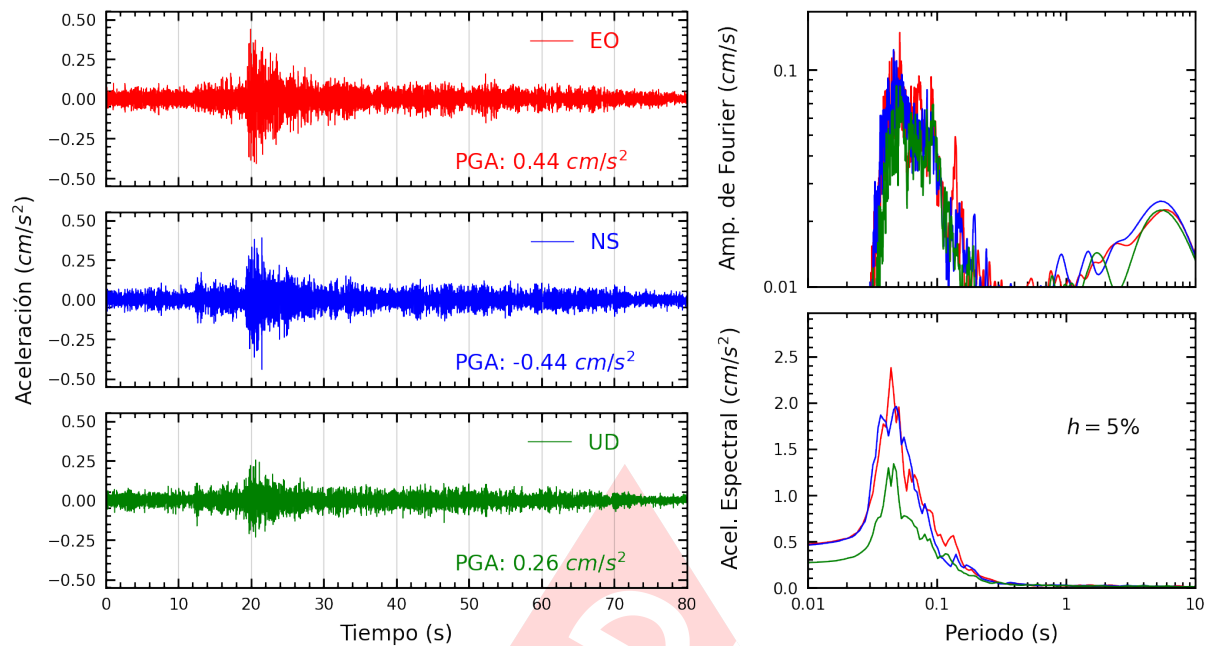
Figura A.15: Registros tiempo-historia, espectros de Fourier y de respuesta en las direcciones EO, NS y vertical de la estación FICPE. Sismo de Chilca, Cañete - Lima del 2025-03-03, 07:30:50 (Hora local)
