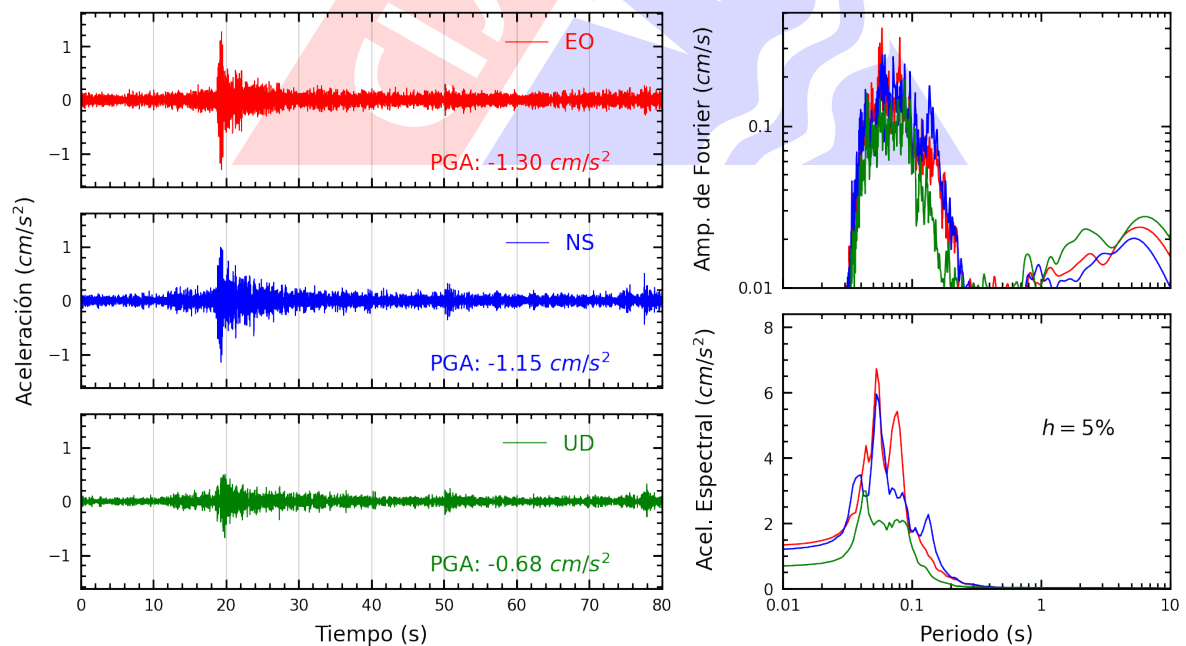
Figura A.4: Registros tiempo-historia, espectros de Fourier y de respuesta en las direcciones EO, NS y vertical de la estación USILM. Sismo de Chilca, Cañete - Lima del 2025-03-03, 07:30:50 (Hora local)
