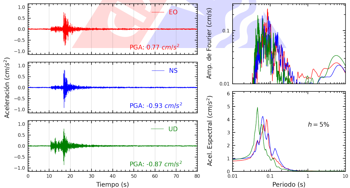
Figura A.8: Registros tiempo-historia, espectros de Fourier y de respuesta en las direcciones EO, NS y vertical de la estación USILP. Sismo de Chilca, Cañete - Lima del 2025-03-03, 07:30:50 (Hora local)
