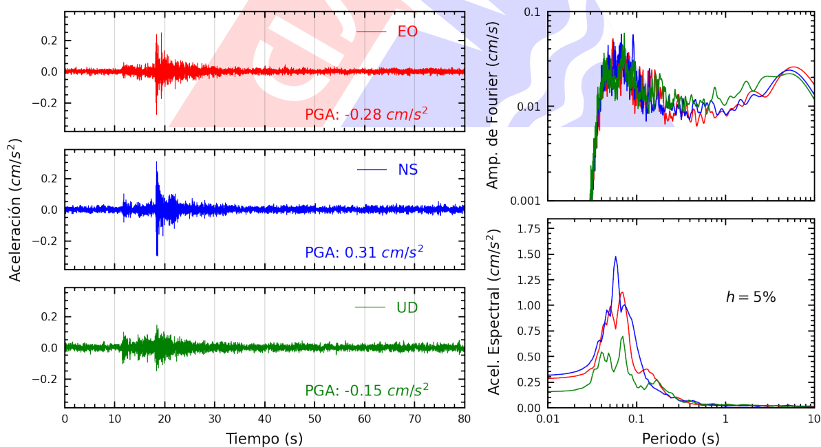
Figura A.20: Registros tiempo-historia, espectros de Fourier y de respuesta en las direcciones EO, NS y vertical de la estación UNFV. Sismo de Chilca, Cañete - Lima del 2025-03-03, 07:30:50 (Hora local)
