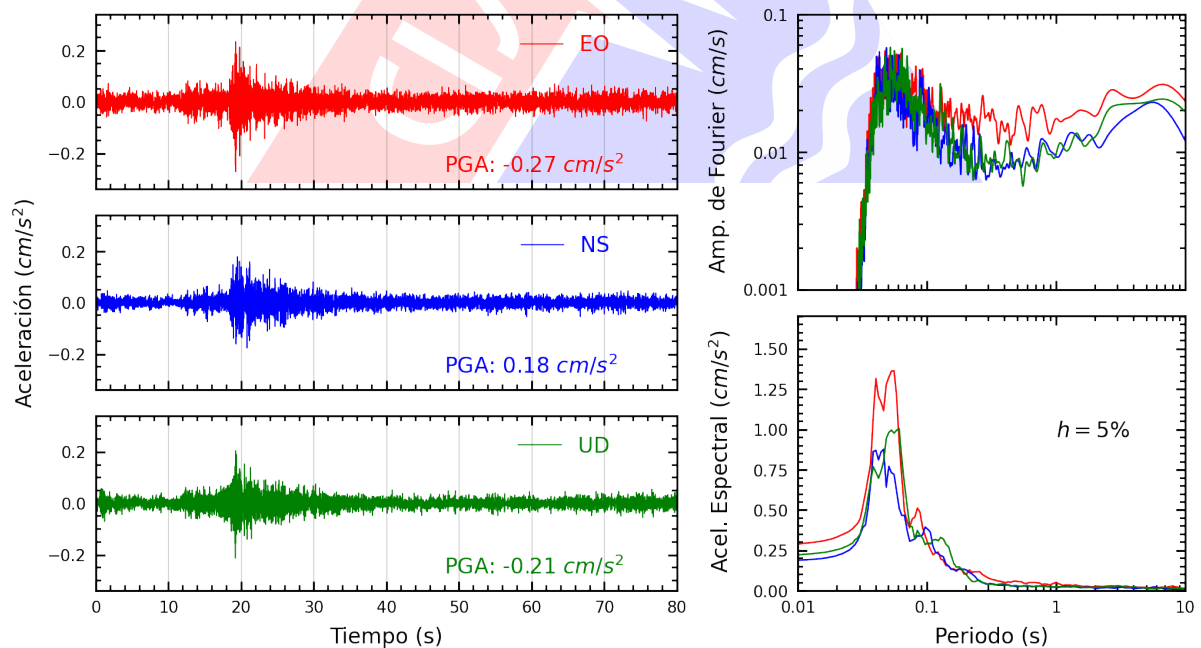
Figura A.24: Registros tiempo-historia, espectros de Fourier y de respuesta en las direcciones EO, NS y vertical de la estación IMCA. Sismo de Chilca, Cañete - Lima del 2025-03-03, 07:30:50 (Hora local)
