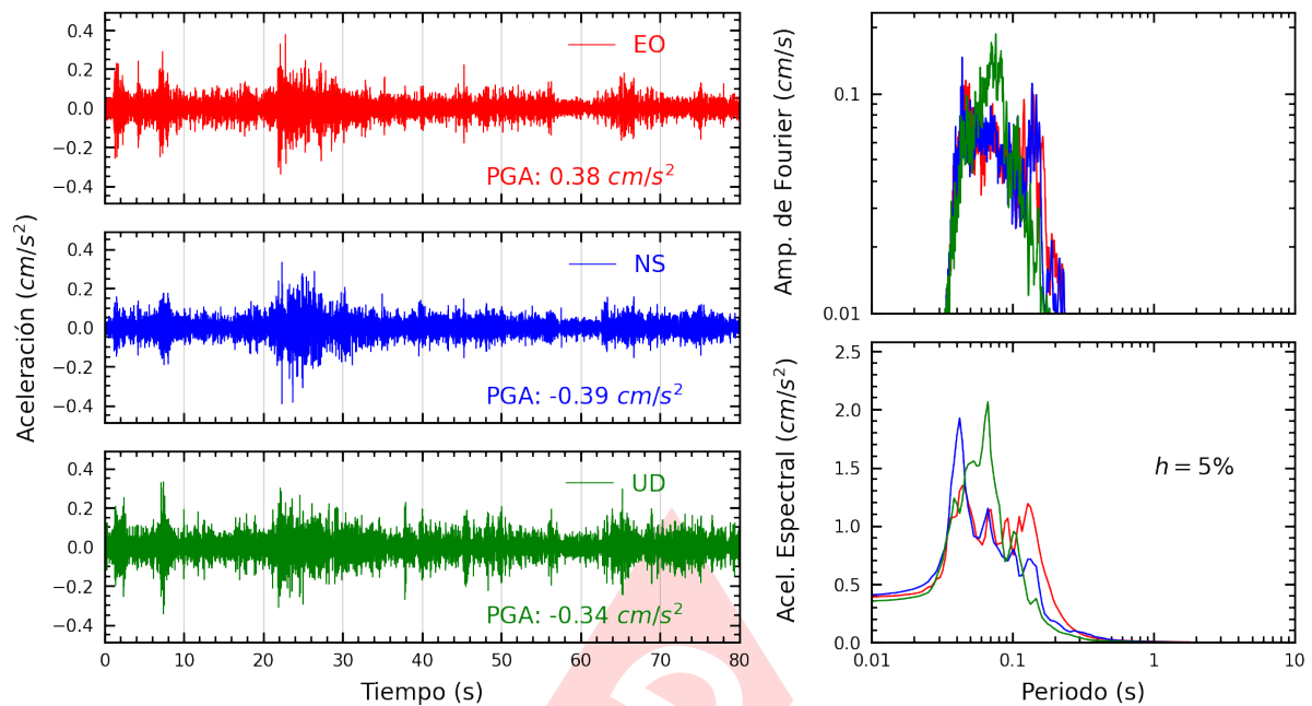
Figura A.17: Registros tiempo-historia, espectros de Fourier y de respuesta en las direcciones EO, NS y vertical de la estación CARA2. Sismo de Chilca, Cañete - Lima del 2025-03-03, 07:30:50 (Hora local)
