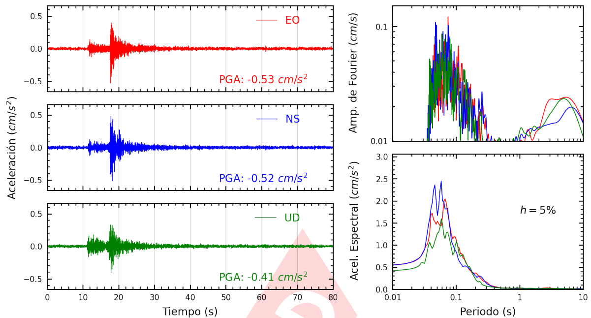
Figura A.11: Registros tiempo-historia, espectros de Fourier y de respuesta en las direcciones EO, NS y vertical de la estación SERVI. Sismo de Chilca, Cañete - Lima del 2025-03-03, 07:30:50 (Hora local)
