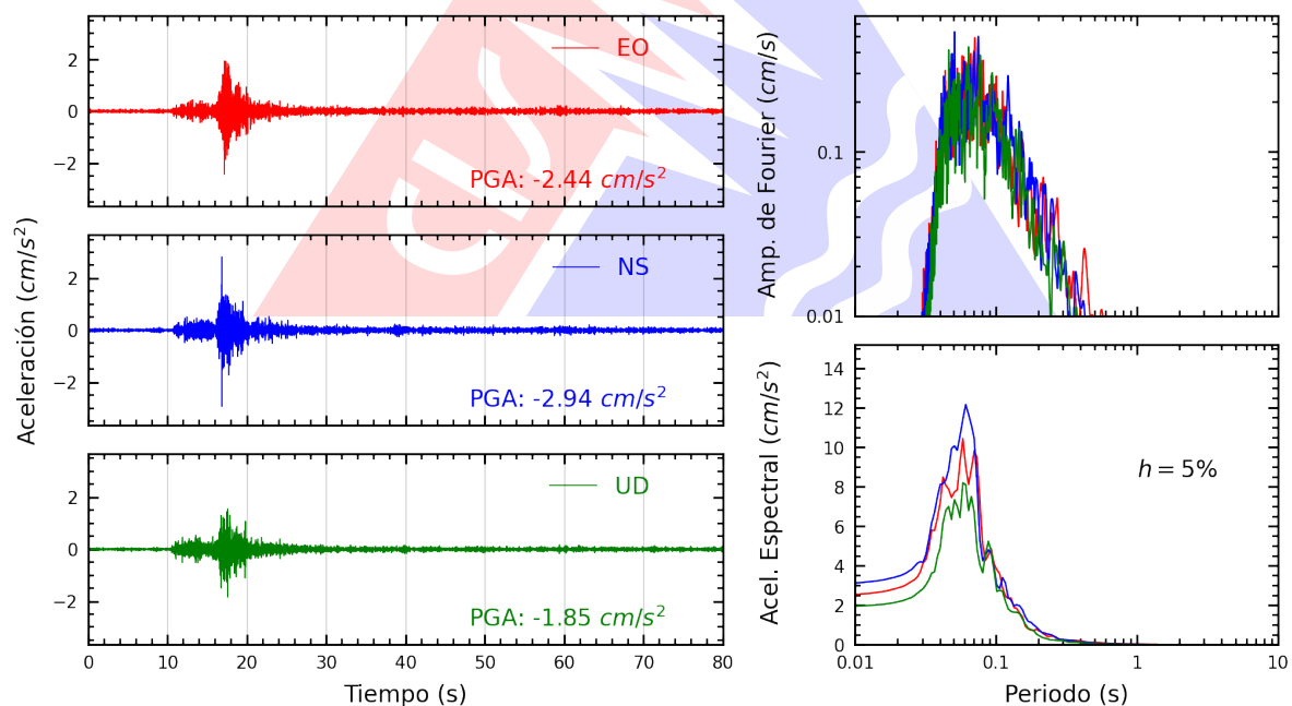
Figura A.2: Registros tiempo-historia, espectros de Fourier y de respuesta en las direcciones EO, NS y vertical de la estación PHER2. Sismo de Chilca, Cañete - Lima del 2025-03-03, 07:30:50 (Hora local)
