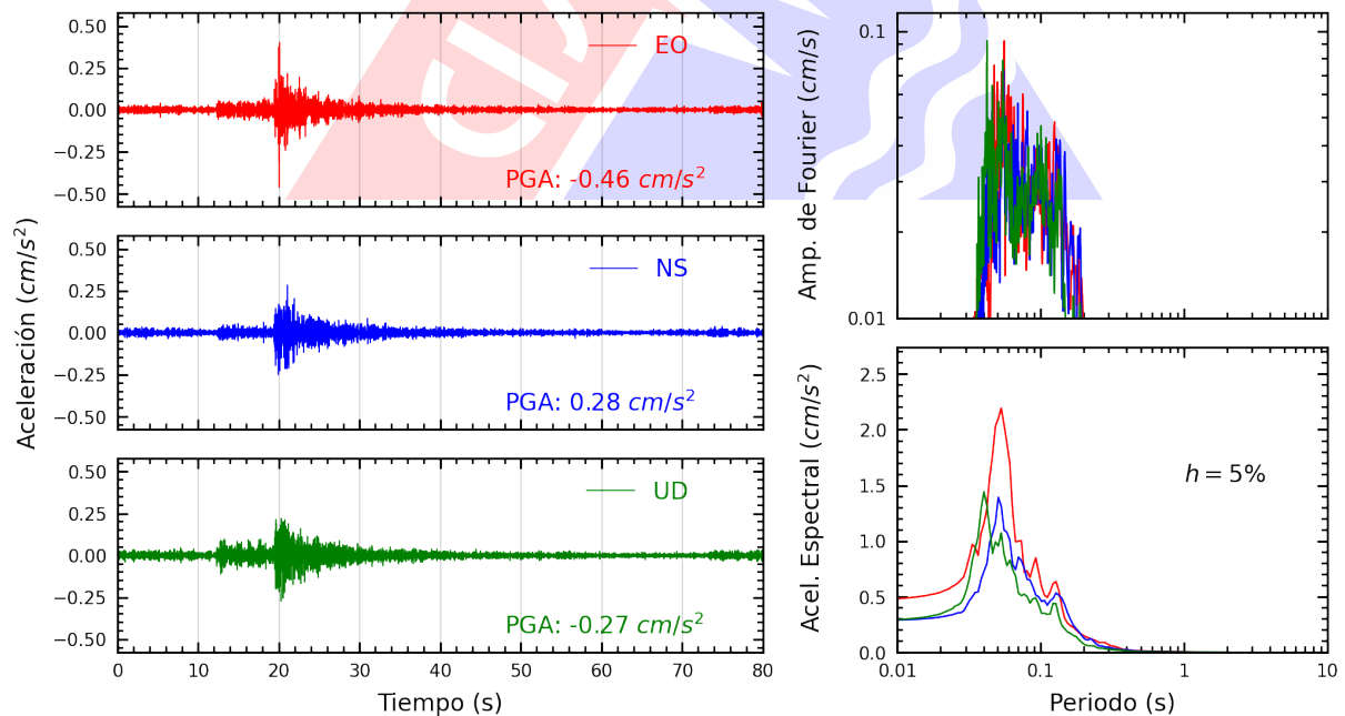
Figura A.14: Registros tiempo-historia, espectros de Fourier y de respuesta en las direcciones EO, NS y vertical de la estación JALV2. Sismo de Chilca, Cañete - Lima del 2025-03-03, 07:30:50 (Hora local)
