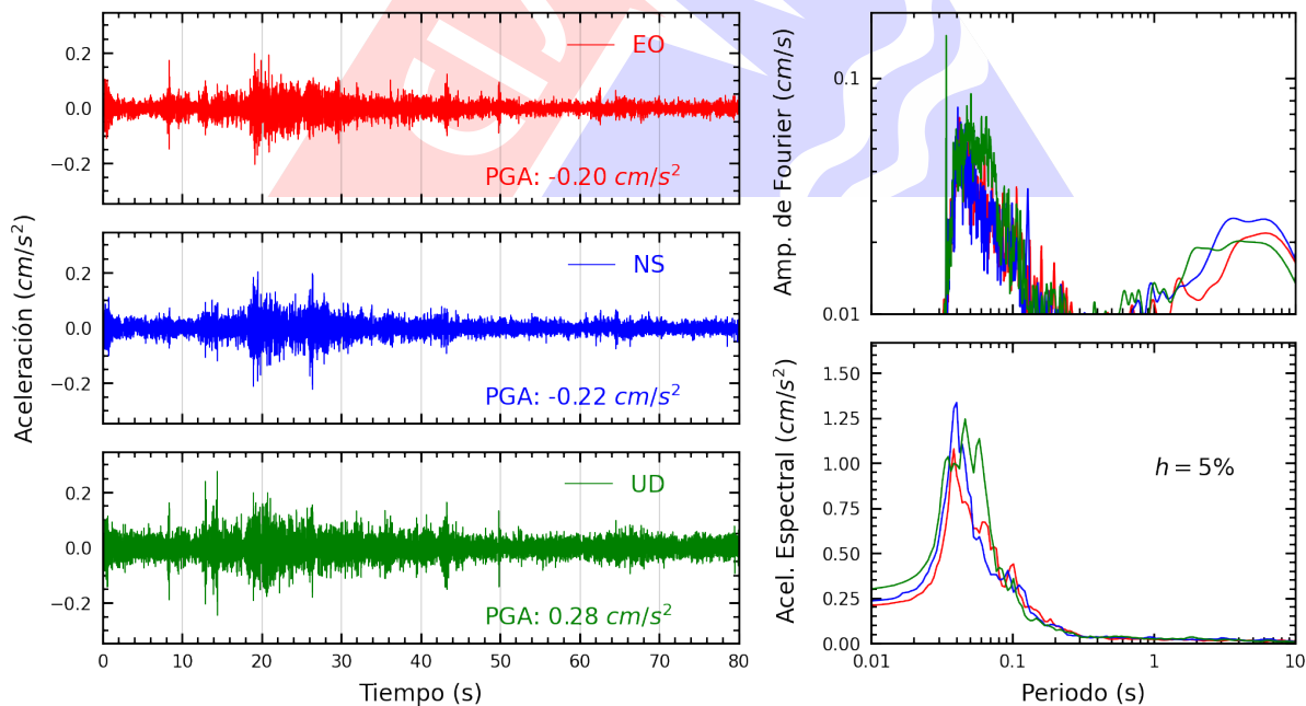
Figura A.22: Registros tiempo-historia, espectros de Fourier y de respuesta en las direcciones EO, NS y vertical de la estación USMP. Sismo de Chilca, Cañete - Lima del 2025-03-03, 07:30:50 (Hora local)
