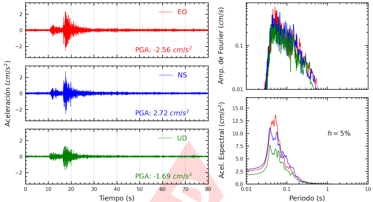
Figura A.3: Registros tiempo-historia, espectros de Fourier y de respuesta en las direcciones EO, NS y vertical de la estación UNTEL. Sismo de Chilca, Cañete - Lima del 2025-03-03, 07:30:50 (Hora local)
