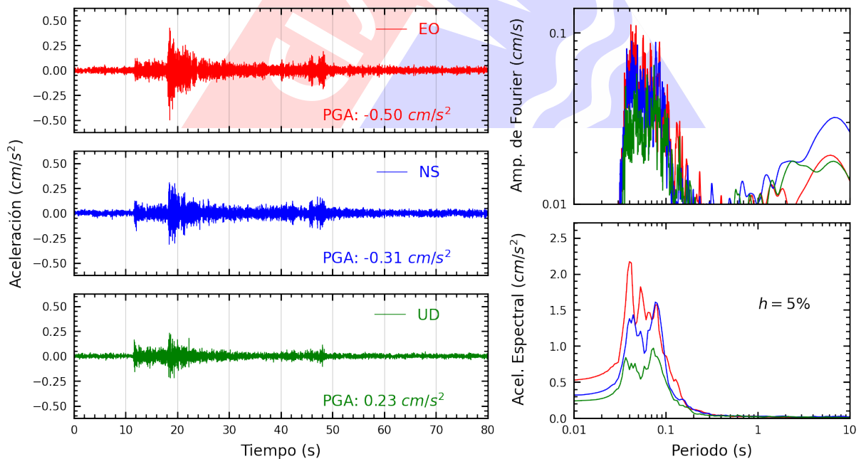
Figura A.12: Registros tiempo-historia, espectros de Fourier y de respuesta en las direcciones EO, NS y vertical de la estación CEPRE. Sismo de Chilca, Cañete - Lima del 2025-03-03, 07:30:50 (Hora local)
