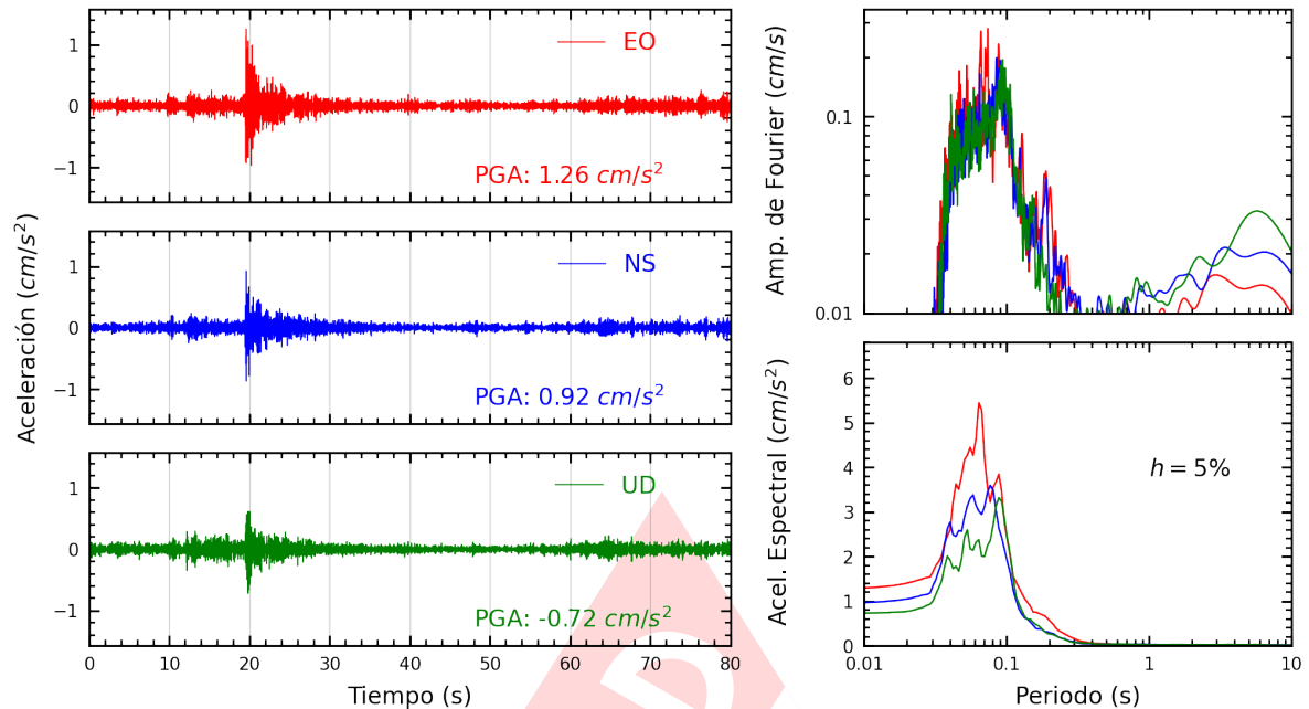
Figura A.5: Registros tiempo-historia, espectros de Fourier y de respuesta en las direcciones EO, NS y vertical de la estación INDEP. Sismo de Chilca, Cañete - Lima del 2025-03-03, 07:30:50 (Hora local)
