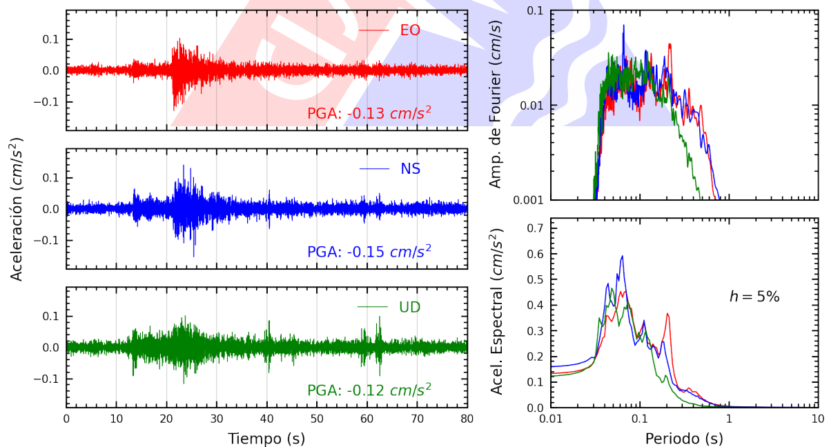
Figura A.28: Registros tiempo-historia, espectros de Fourier y de respuesta en las direcciones EO, NS y vertical de la estación VHAY2. Sismo de Chilca, Cañete - Lima del 2025-03-03, 07:30:50 (Hora local)
