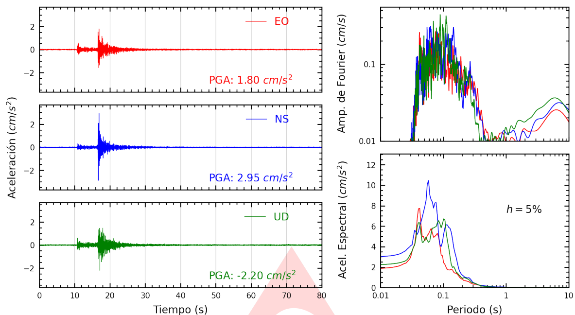
Figura A.1: Registros tiempo-historia, espectros de Fourier y de respuesta en las direcciones EO, NS y vertical de la estación SOVES. Sismo de Chilca, Cañete - Lima del 2025-03-03, 07:30:50 (Hora local)
