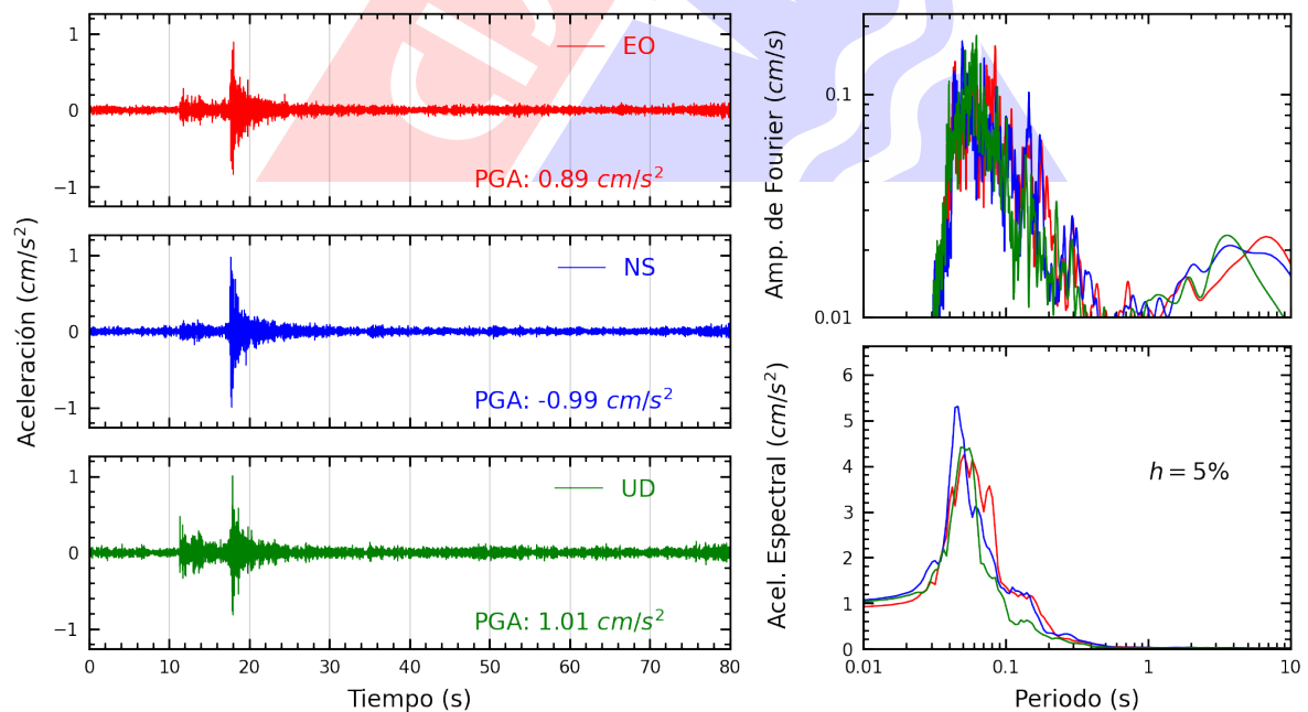
Figura A.6: Registros tiempo-historia, espectros de Fourier y de respuesta en las direcciones EO, NS y vertical de la estación URPE. Sismo de Chilca, Cañete - Lima del 2025-03-03, 07:30:50 (Hora local)
