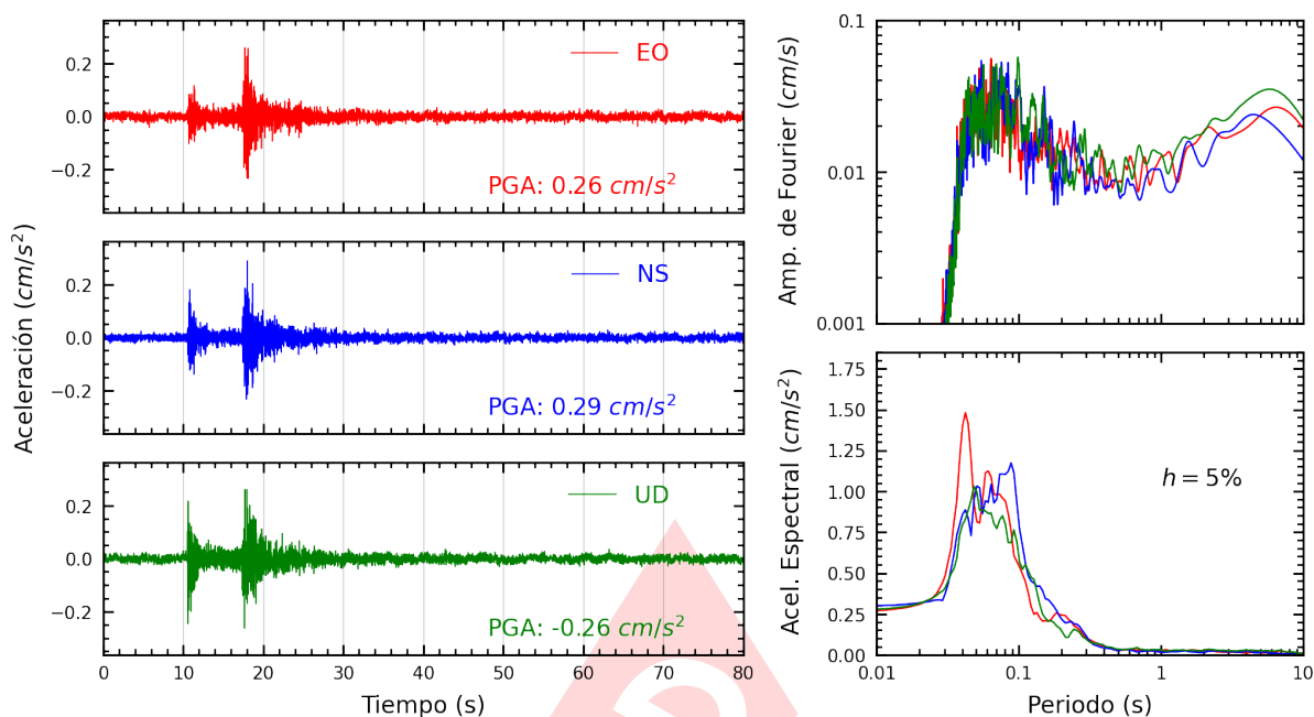
Figura A.21: Registros tiempo-historia, espectros de Fourier y de respuesta en las direcciones EO, NS y vertical de la estación UNMSM. Sismo de Chilca, Cañete - Lima del 2025-03-03, 07:30:50 (Hora local)
