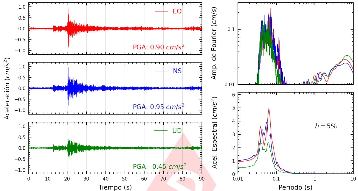
Figura A.7: Registros tiempo-historia, espectros de Fourier y de respuesta en las direcciones EO, NS y vertical de la estación JOSEO. Sismo de Chilca, Cañete - Lima del 2025-03-03, 07:30:50 (Hora local)
