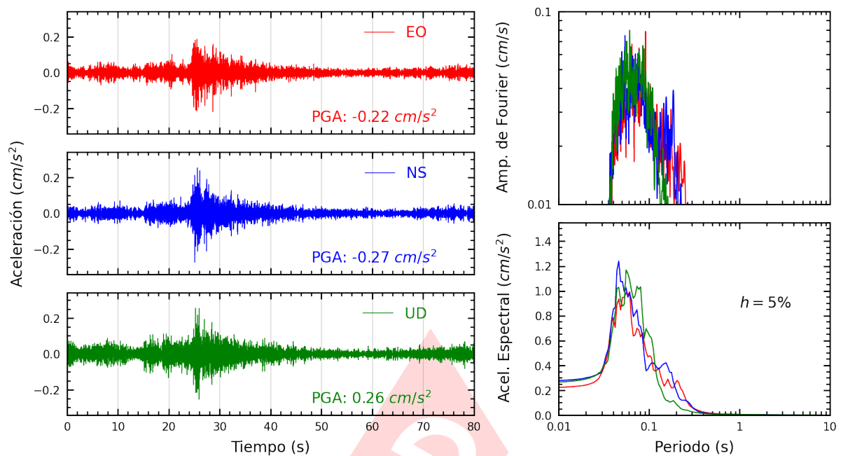
Figura A.23: Registros tiempo-historia, espectros de Fourier y de respuesta en las direcciones EO, NS y vertical de la estación ASIA. Sismo de Chilca, Cañete - Lima del 2025-03-03, 07:30:50 (Hora local)
