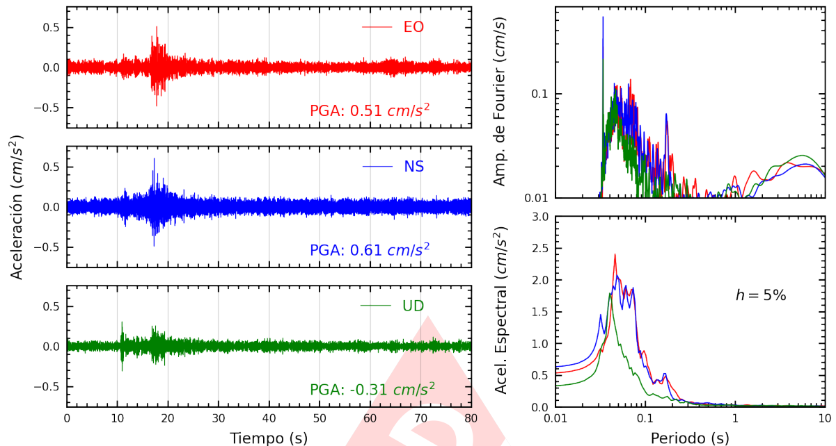
Figura A.9: Registros tiempo-historia, espectros de Fourier y de respuesta en las direcciones EO, NS y vertical de la estación UPCVI. Sismo de Chilca, Cañete - Lima del 2025-03-03, 07:30:50 (Hora local)
