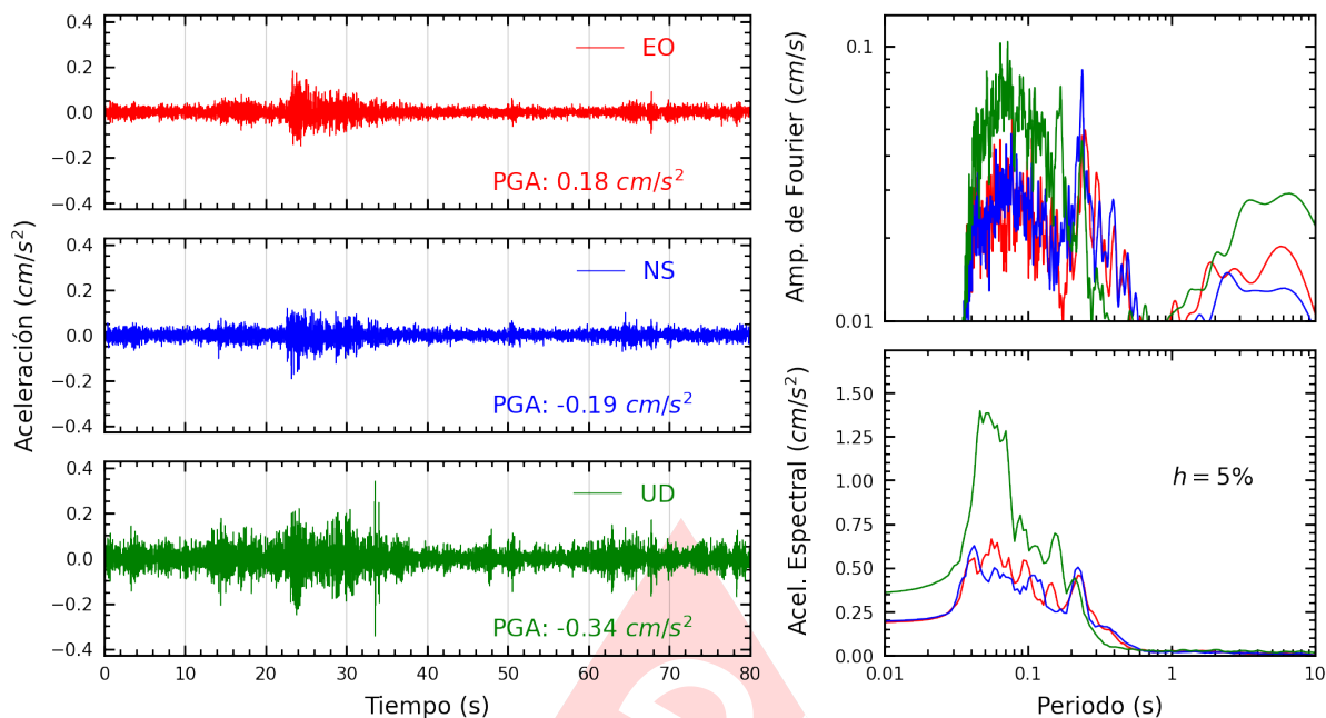
Figura A.19: Registros tiempo-historia, espectros de Fourier y de respuesta en las direcciones EO, NS y vertical de la estación MDPP. Sismo de Chilca, Cañete - Lima del 2025-03-03, 07:30:50 (Hora local)
