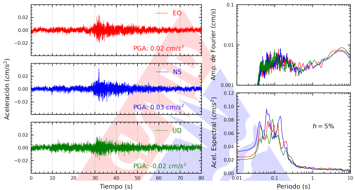
Figura A.29: Registros tiempo-historia, espectros de Fourier y de respuesta en las direcciones EO, NS y vertical de la estación CARAL. Sismo de Chilca, Cañete - Lima del 2025-03-03, 07:30:50 (Hora local)
