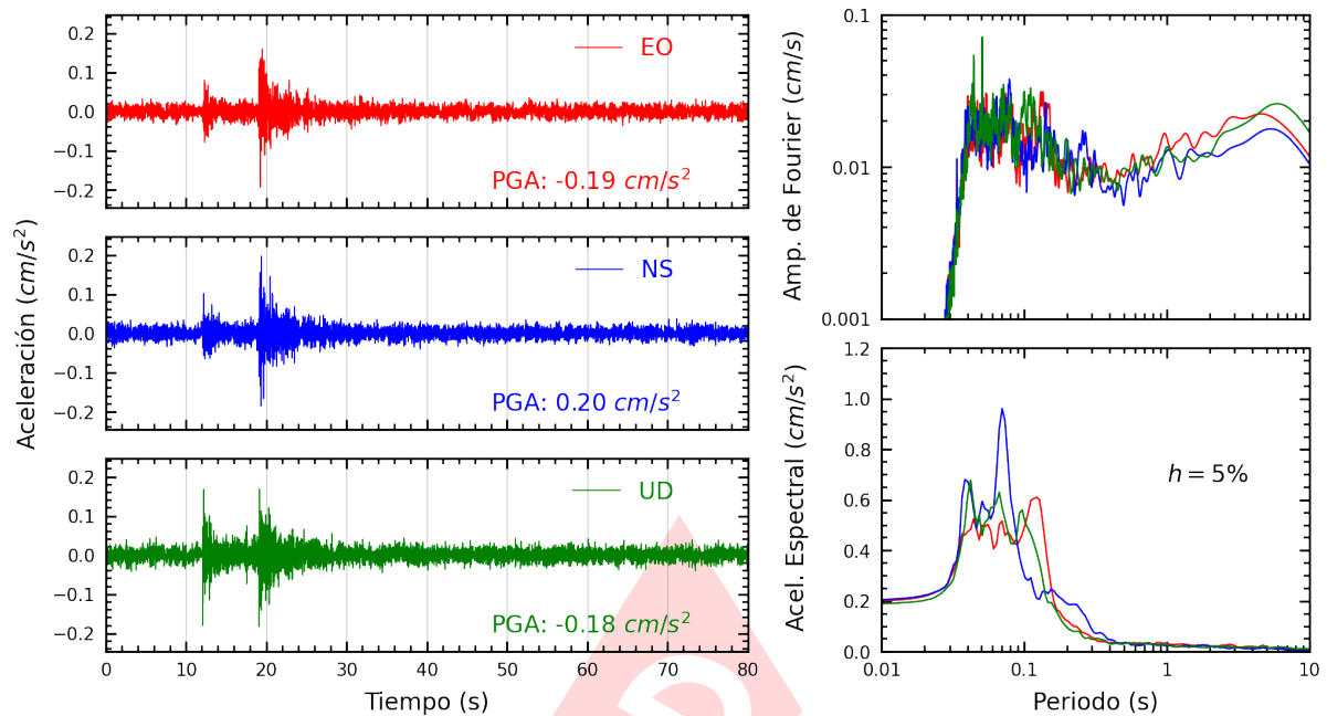
Figura A.27: Registros tiempo-historia, espectros de Fourier y de respuesta en las direcciones EO, NS y vertical de la estación BONDY. Sismo de Chilca, Cañete - Lima del 2025-03-03, 07:30:50 (Hora local)
