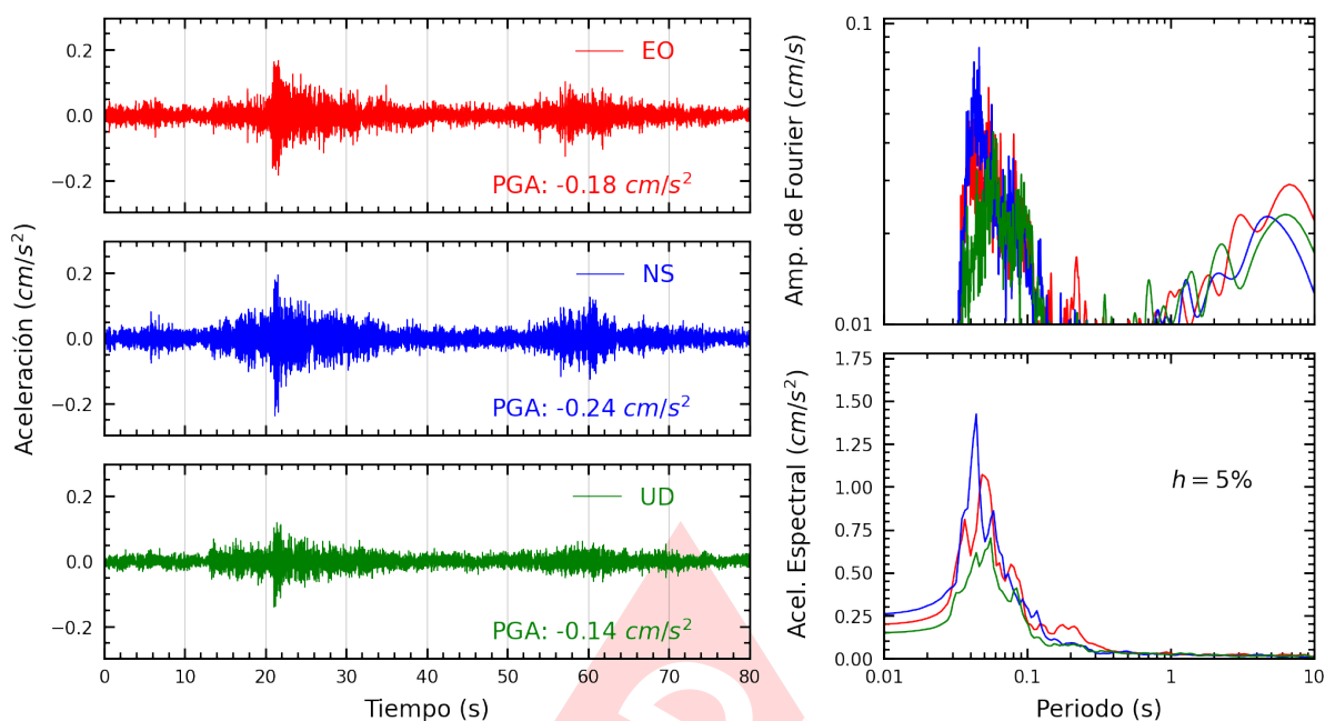
Figura A.25: Registros tiempo-historia, espectros de Fourier y de respuesta en las direcciones EO, NS y vertical de la estación COMAS. Sismo de Chilca, Cañete - Lima del 2025-03-03, 07:30:50 (Hora local)
