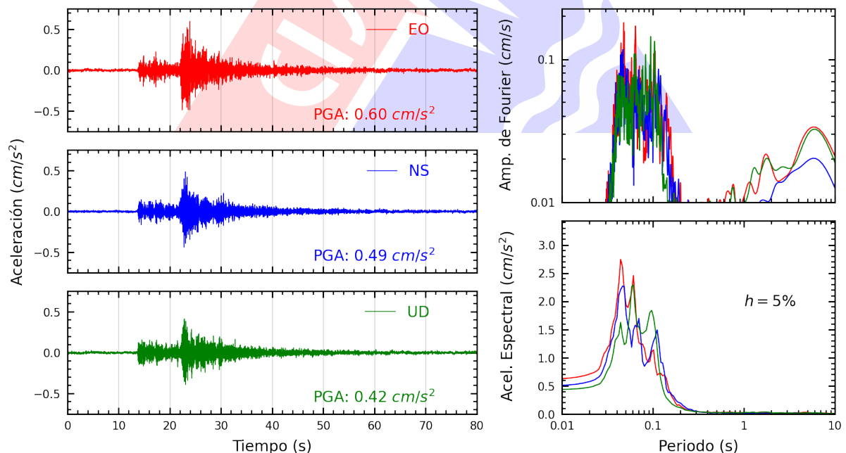
Figura A.10: Registros tiempo-historia, espectros de Fourier y de respuesta en las direcciones EO, NS y vertical de la estación AMORE. Sismo de Chilca, Cañete - Lima del 2025-03-03, 07:30:50 (Hora local)
