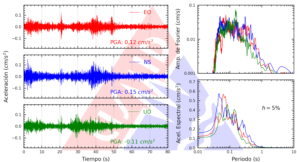
Figura A.3: Registros tiempo-historia, espectros de Fourier y de respuesta en las direcciones EO, NS y vertical de la estación UPAOP. Sismo de Talara, Talara - Piura del 2025-03-03, 13:11:08 (Hora local)
