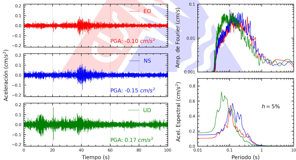
Figura A.2: Registros tiempo-historia, espectros de Fourier y de respuesta en las direcciones EO, NS y vertical de la estación UNP. Sismo de Talara, Talara - Piura del 2025-03-03, 13:11:08 (Hora local)
