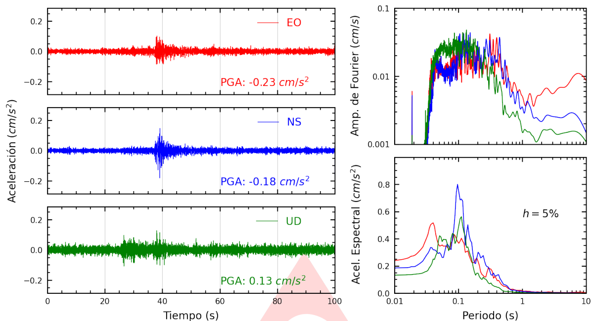
Figura A.1: Registros tiempo-historia, espectros de Fourier y de respuesta en las direcciones EO, NS y vertical de la estación SCPIU. Sismo de Talara, Talara - Piura del 2025-03-03, 13:11:08 (Hora local)
