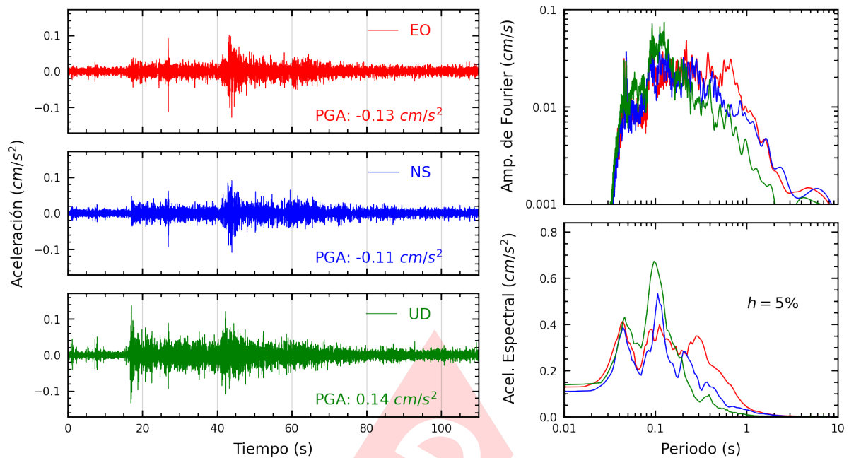
Figura A.5: Registros tiempo-historia, espectros de Fourier y de respuesta en las direcciones EO, NS y vertical de la estación UNIA. Sismo de Tingo Maria, Leoncio Prado - Huanuco del 2025-03-04, 08:22:02 (Hora local)
