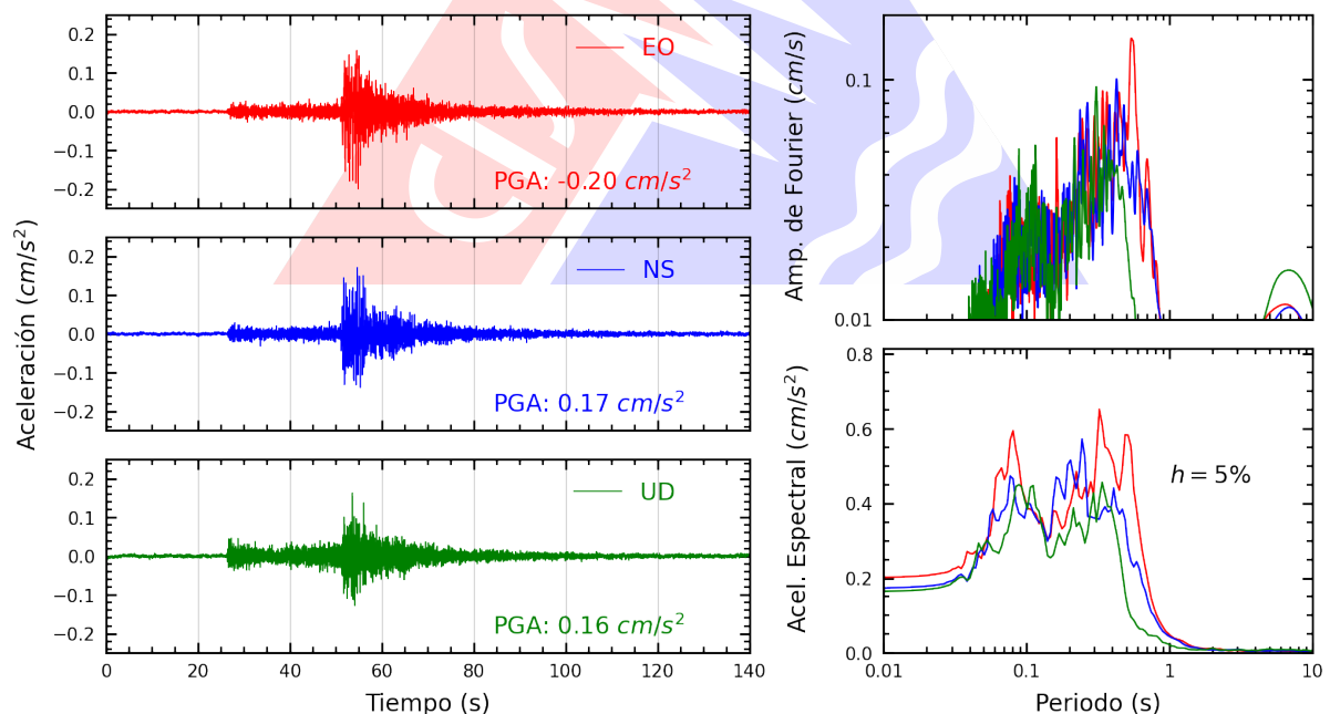
Figura A.2: Registros tiempo-historia, espectros de Fourier y de respuesta en las direcciones EO, NS y vertical de la estación CARAL. Sismo de Tingo Maria, Leoncio Prado - Huanuco del 2025-03-04, 08:22:02 (Hora local)
