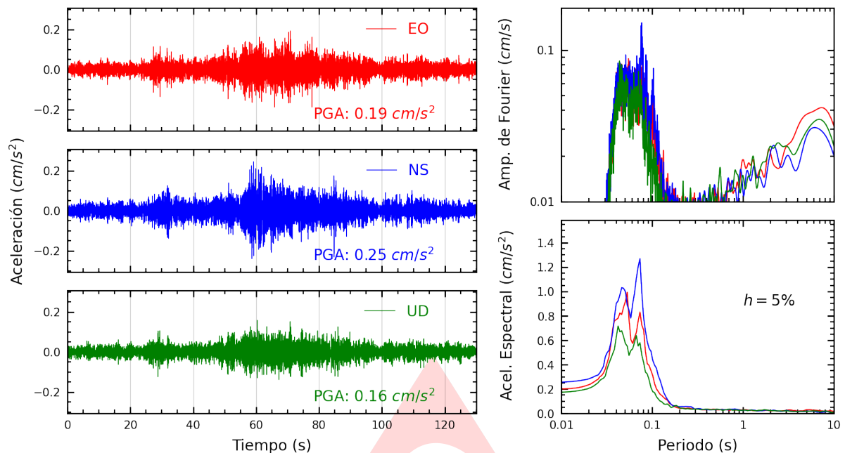
Figura A.1: Registros tiempo-historia, espectros de Fourier y de respuesta en las direcciones EO, NS y vertical de la estación JOSEO. Sismo de Tingo Maria, Leoncio Prado - Huanuco del 2025-03-04, 08:22:02 (Hora local)
