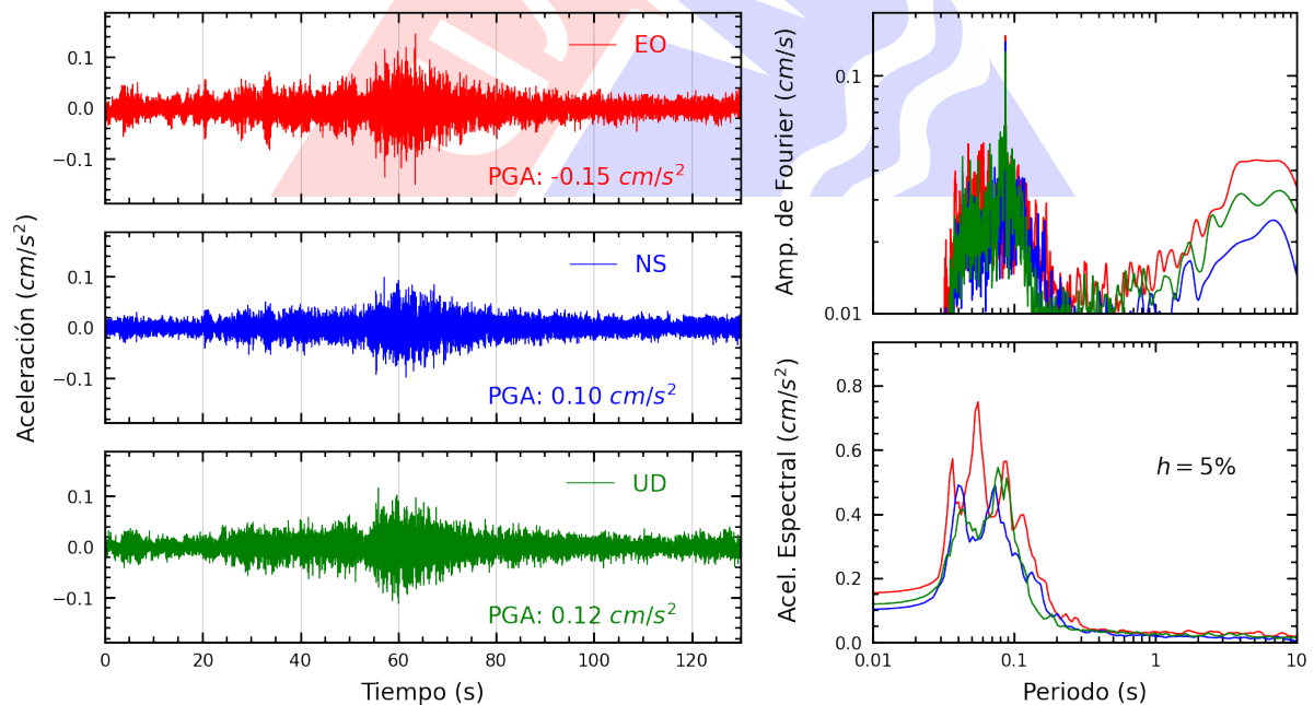
Figura A.4: Registros tiempo-historia, espectros de Fourier y de respuesta en las direcciones EO, NS y vertical de la estación AMORE. Sismo de Tingo Maria, Leoncio Prado - Huanuco del 2025-03-04, 08:22:02 (Hora local)
