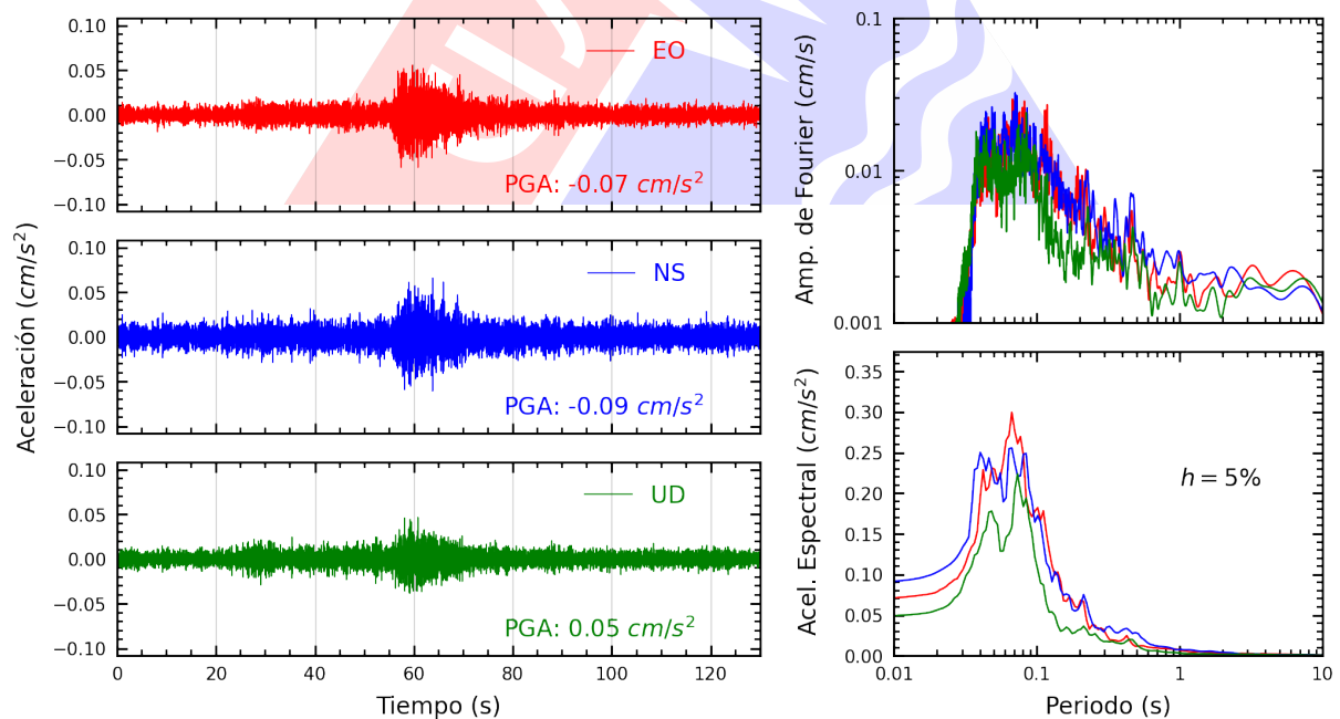
Figura A.6: Registros tiempo-historia, espectros de Fourier y de respuesta en las direcciones EO, NS y vertical de la estación ATARJ. Sismo de Tingo Maria, Leoncio Prado - Huanuco del 2025-03-04, 08:22:02 (Hora local)
