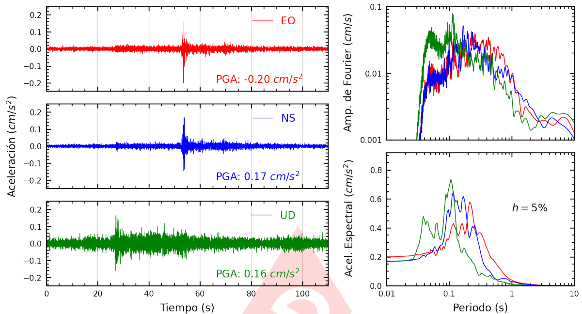
Figura A.3: Registros tiempo-historia, espectros de Fourier y de respuesta en las direcciones EO, NS y vertical de la estación SCPUC. Sismo de Tingo Maria, Leoncio Prado - Huanuco del 2025-03-04, 08:22:02 (Hora local)
