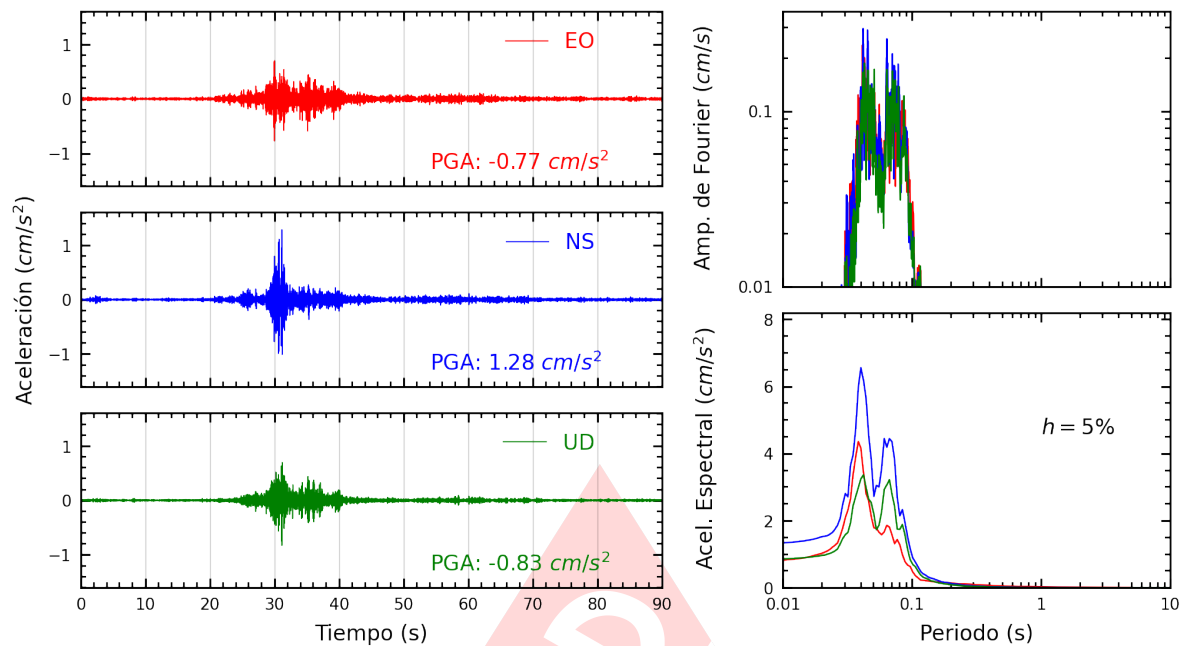
Figura A.3: Registros tiempo-historia, espectros de Fourier y de respuesta en las direcciones EO, NS y vertical de la estación PACHA. Sismo de Pucallpa, Coronel Portillo - Ucayali del 2025-03-05, 02:36:38 (Hora local)
