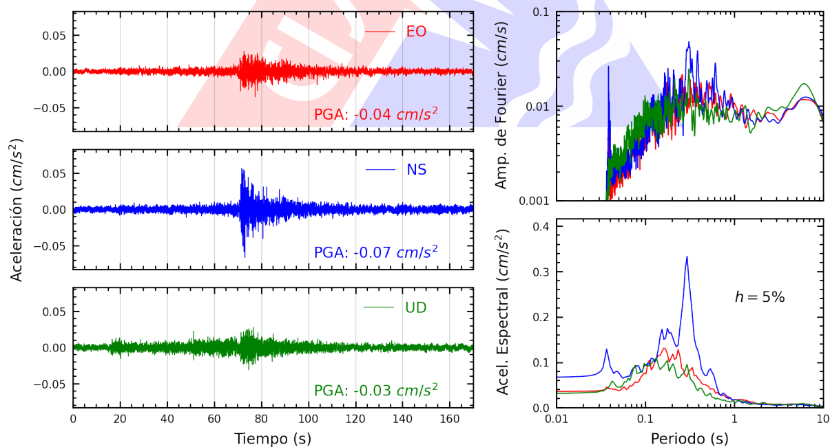
Figura A.12: Registros tiempo-historia, espectros de Fourier y de respuesta en las direcciones EO, NS y vertical de la estación UNJ. Sismo de Pucallpa, Coronel Portillo - Ucayali del 2025-03-05, 02:36:38 (Hora local)
