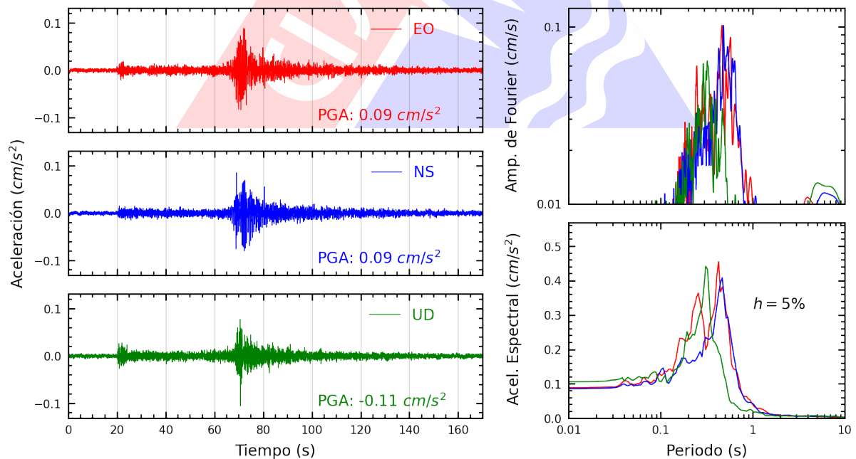
Figura A.10: Registros tiempo-historia, espectros de Fourier y de respuesta en las direcciones EO, NS y vertical de la estación CARAL. Sismo de Pucallpa, Coronel Portillo - Ucayali del 2025-03-05, 02:36:38 (Hora local)
