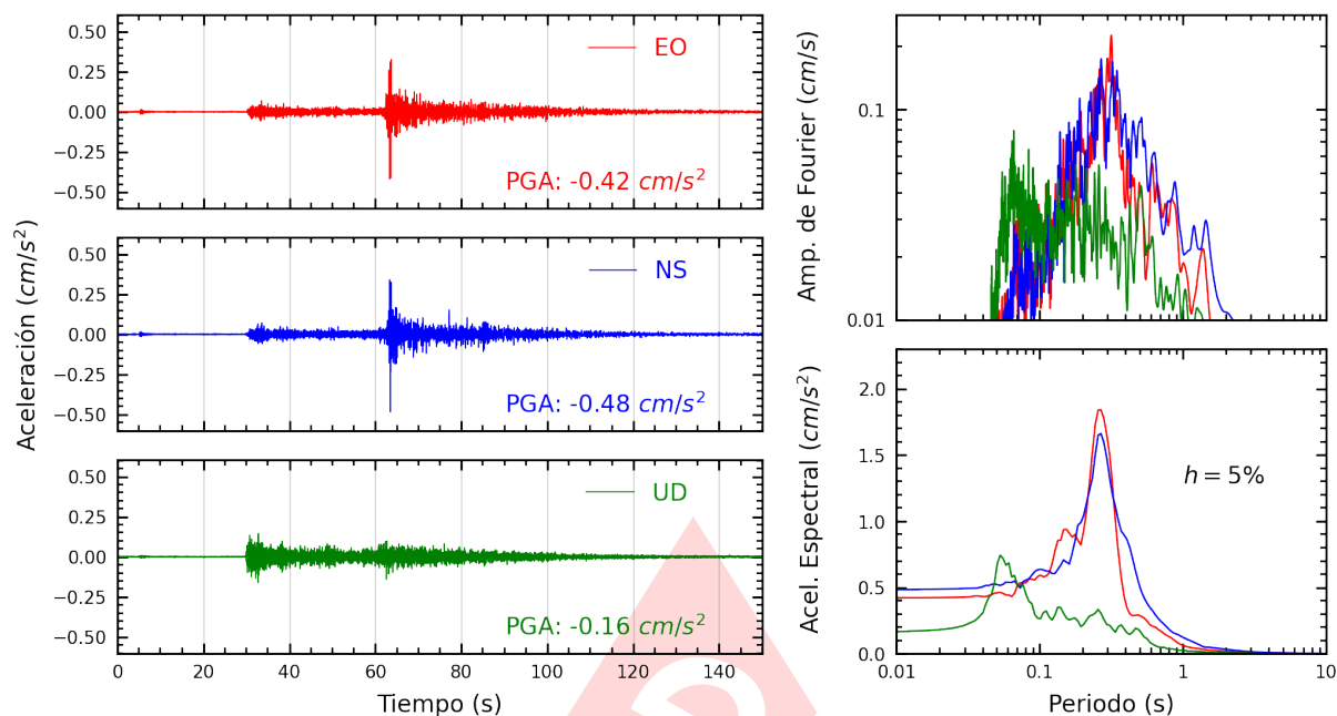
Figura A.5: Registros tiempo-historia, espectros de Fourier y de respuesta en las direcciones EO, NS y vertical de la estación UNAAA. Sismo de Pucallpa, Coronel Portillo - Ucayali del 2025-03-05, 02:36:38 (Hora local)
