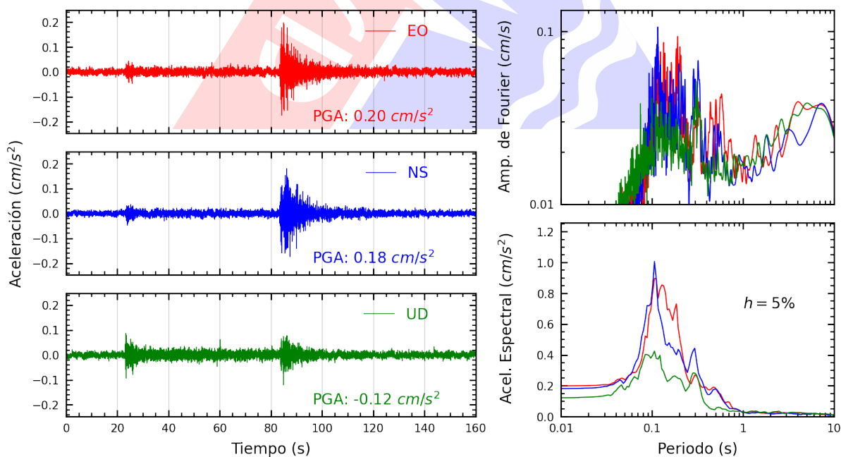
Figura A.6: Registros tiempo-historia, espectros de Fourier y de respuesta en las direcciones EO, NS y vertical de la estación UCVCH. Sismo de Pucallpa, Coronel Portillo - Ucayali del 2025-03-05, 02:36:38 (Hora local)
