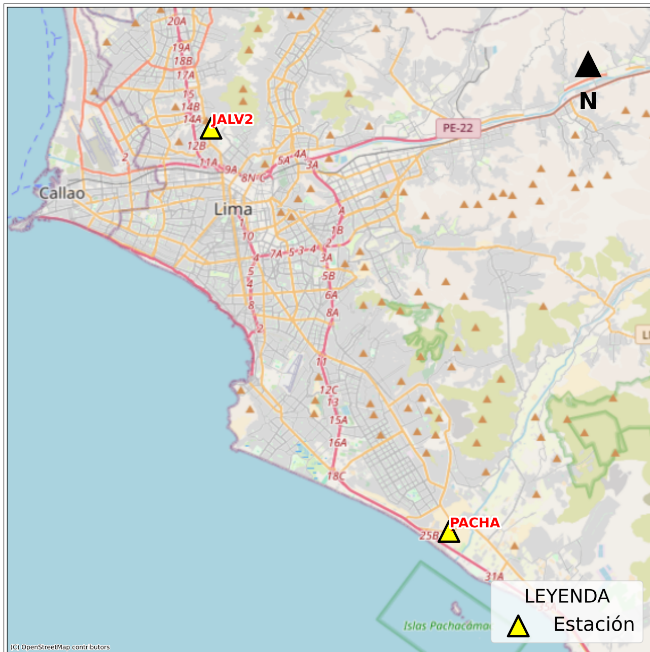
Figura 3: Mapa de ubicación de la(s) estación(es) acelerográfica(s) en Lima Metropolitana correspondiente(s) al Sismo de Pucallpa, Coronel Portillo - Ucayali del 05 de marzo de 2025 a las 02:36:38 (hora local)
