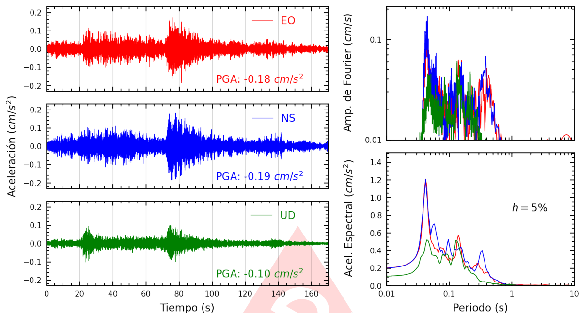
Figura A.7: Registros tiempo-historia, espectros de Fourier y de respuesta en las direcciones EO, NS y vertical de la estación SCTRU. Sismo de Pucallpa, Coronel Portillo - Ucayali del 2025-03-05, 02:36:38 (Hora local)
