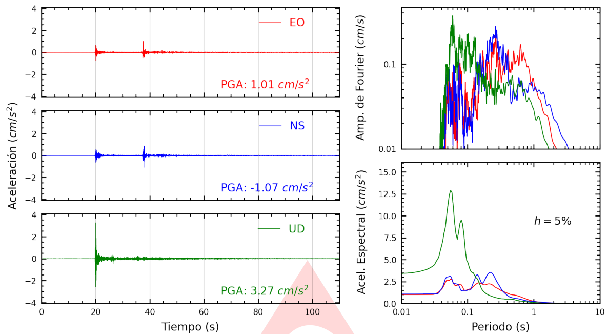
Figura A.1: Registros tiempo-historia, espectros de Fourier y de respuesta en las direcciones EO, NS y vertical de la estación SCPUC. Sismo de Pucallpa, Coronel Portillo - Ucayali del 2025-03-05, 02:36:38 (Hora local)
