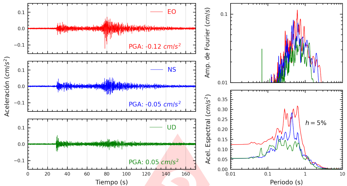
Figura A.9: Registros tiempo-historia, espectros de Fourier y de respuesta en las direcciones EO, NS y vertical de la estación UNC. Sismo de Pucallpa, Coronel Portillo - Ucayali del 2025-03-05, 02:36:38 (Hora local)
