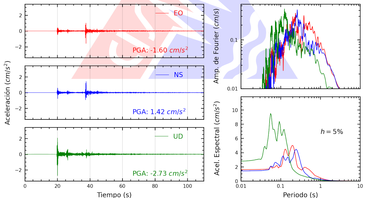
Figura A.2: Registros tiempo-historia, espectros de Fourier y de respuesta en las direcciones EO, NS y vertical de la estación UNIA. Sismo de Pucallpa, Coronel Portillo - Ucayali del 2025-03-05, 02:36:38 (Hora local)
