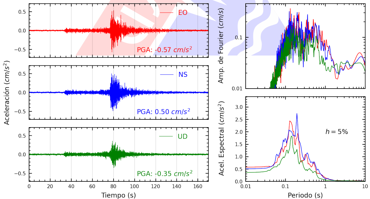
Figura A.4: Registros tiempo-historia, espectros de Fourier y de respuesta en las direcciones EO, NS y vertical de la estación UNTRM. Sismo de Pucallpa, Coronel Portillo - Ucayali del 2025-03-05, 02:36:38 (Hora local)
