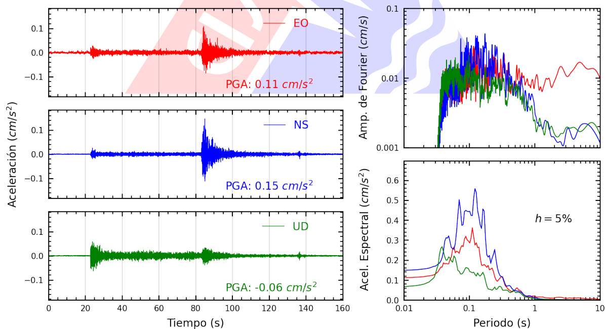
Figura A.8: Registros tiempo-historia, espectros de Fourier y de respuesta en las direcciones EO, NS y vertical de la estación SCCHI. Sismo de Pucallpa, Coronel Portillo - Ucayali del 2025-03-05, 02:36:38 (Hora local)
