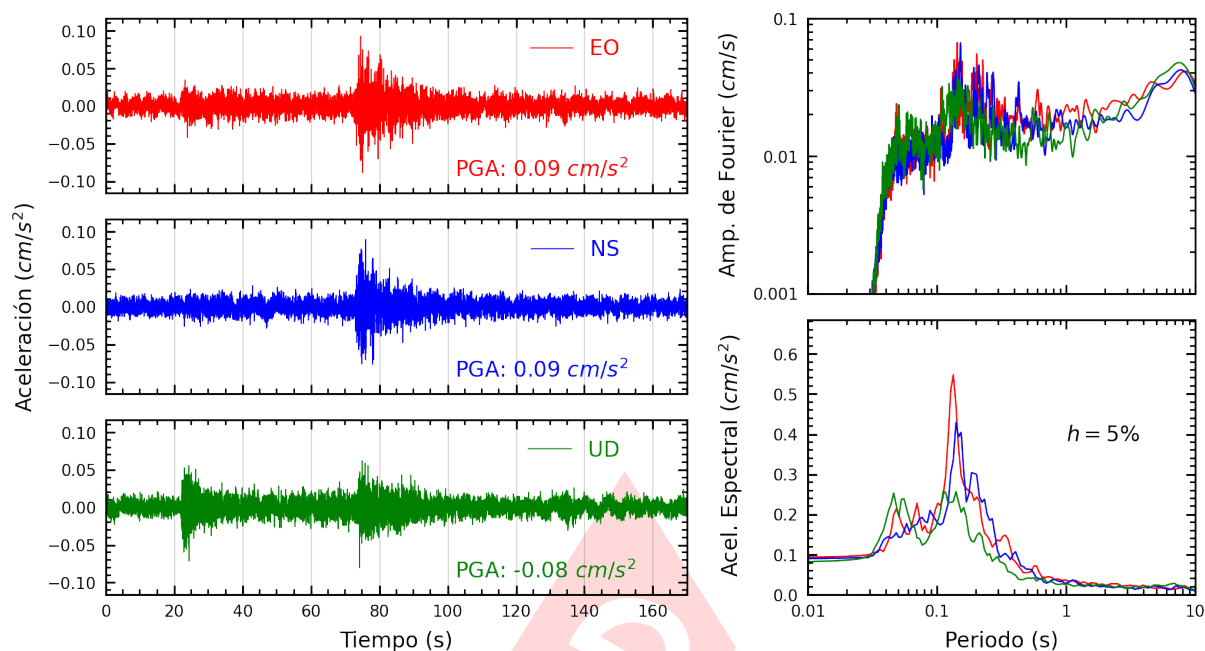
Figura A.11: Registros tiempo-historia, espectros de Fourier y de respuesta en las direcciones EO, NS y vertical de la estación UPAOT. Sismo de Pucallpa, Coronel Portillo - Ucayali del 2025-03-05, 02:36:38 (Hora local)
