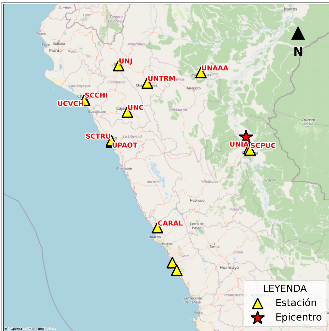
Figura 2: Mapa de ubicación de la(s) estación(es) acelerográfica(s) a nivel nacional correspondiente(s) al Sismo de Pucallpa, Coronel Portillo - Ucayali del 05 de marzo de 2025 a las 02:36:38 (hora local)
