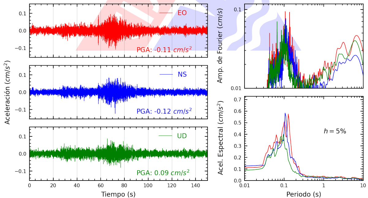
Figura A.4: Registros tiempo-historia, espectros de Fourier y de respuesta en las direcciones EO, NS y vertical de la estación AMORE. Sismo de Palpa, Palpa - Ica del 2025-03-05, 09:19:55 (Hora local)
