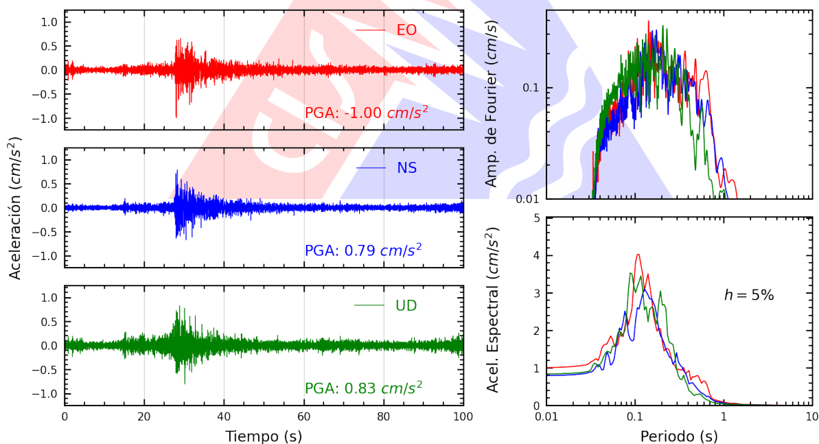
Figura A.2: Registros tiempo-historia, espectros de Fourier y de respuesta en las direcciones EO, NS y vertical de la estación SCICA. Sismo de Palpa, Palpa - Ica del 2025-03-05, 09:19:55 (Hora local)
