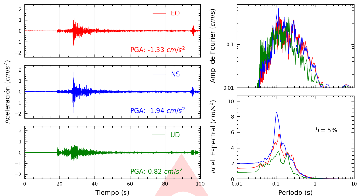
Figura A.1: Registros tiempo-historia, espectros de Fourier y de respuesta en las direcciones EO, NS y vertical de la estación UNICA. Sismo de Palpa, Palpa - Ica del 2025-03-05, 09:19:55 (Hora local)
