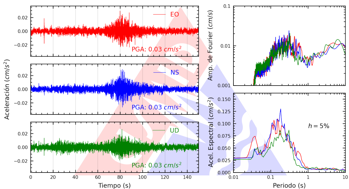
Figura A.5: Registros tiempo-historia, espectros de Fourier y de respuesta en las direcciones EO, NS y vertical de la estación CARAL. Sismo de Palpa, Palpa - Ica del 2025-03-05, 09:19:55 (Hora local)
