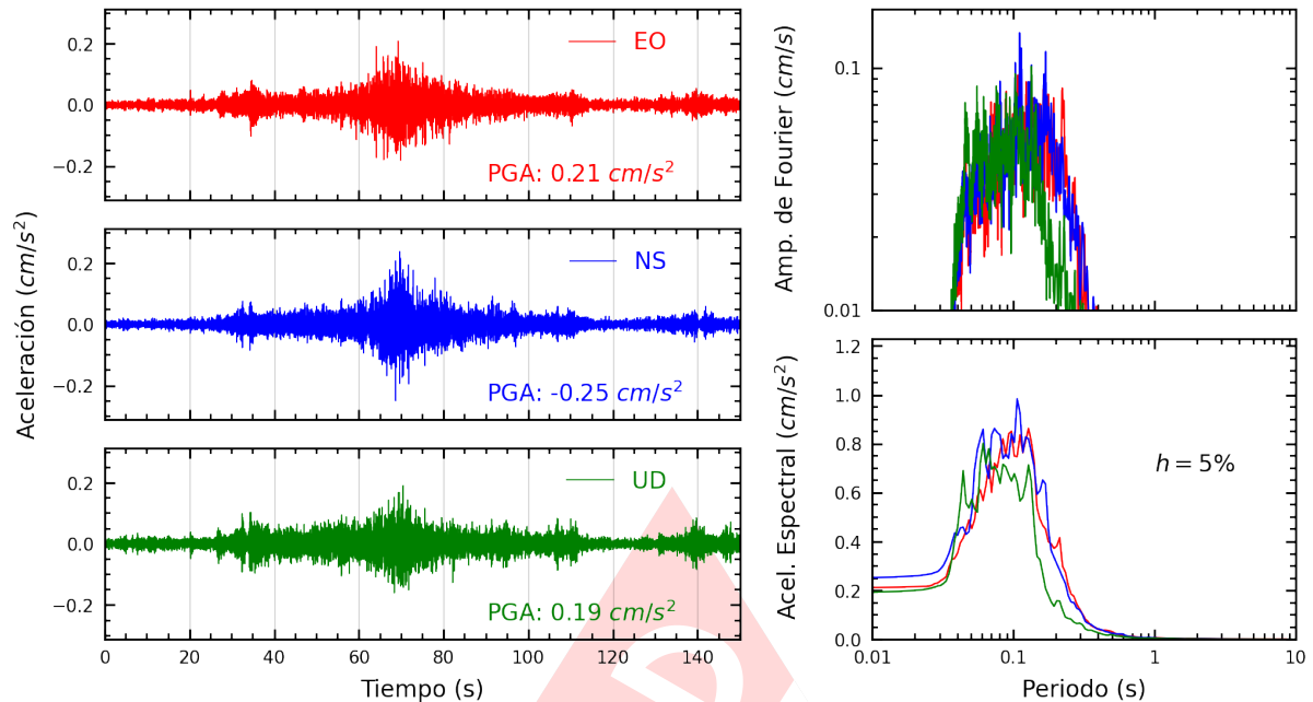
Figura A.3: Registros tiempo-historia, espectros de Fourier y de respuesta en las direcciones EO, NS y vertical de la estación ASIA. Sismo de Palpa, Palpa - Ica del 2025-03-05, 09:19:55 (Hora local)
