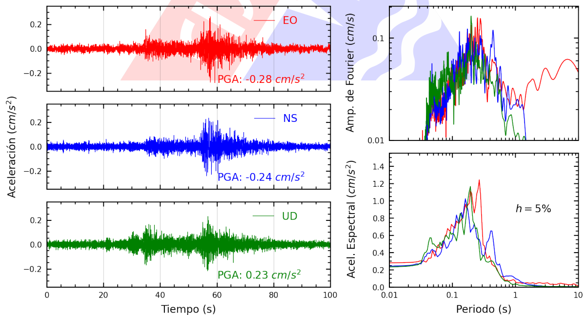
Figura A.6: Registros tiempo-historia, espectros de Fourier y de respuesta en las direcciones EO, NS y vertical de la estación UJB3. Sismo de Ilo, Ilo - Moquegua del 2025-03-06, 13:13:35 (Hora local)
