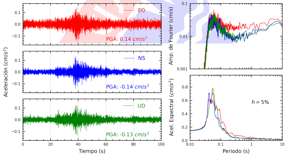
Figura A.30: Registros tiempo-historia, espectros de Fourier y de respuesta en las direcciones EO, NS y vertical de la estación IMCA. Sismo de Mala, Cañete - Lima del 2025-03-07, 22:47:44 (Hora local)
