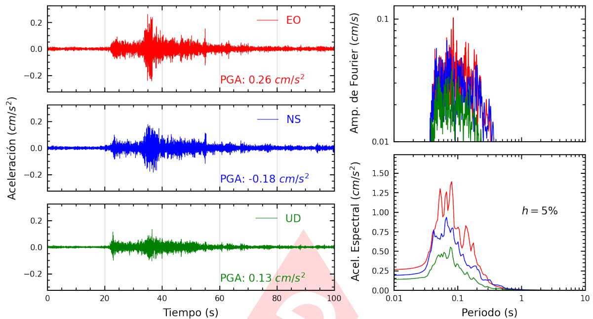
Figura A.23: Registros tiempo-historia, espectros de Fourier y de respuesta en las direcciones EO, NS y vertical de la estación BRISA. Sismo de Mala, Cañete - Lima del 2025-03-07, 22:47:44 (Hora local)
