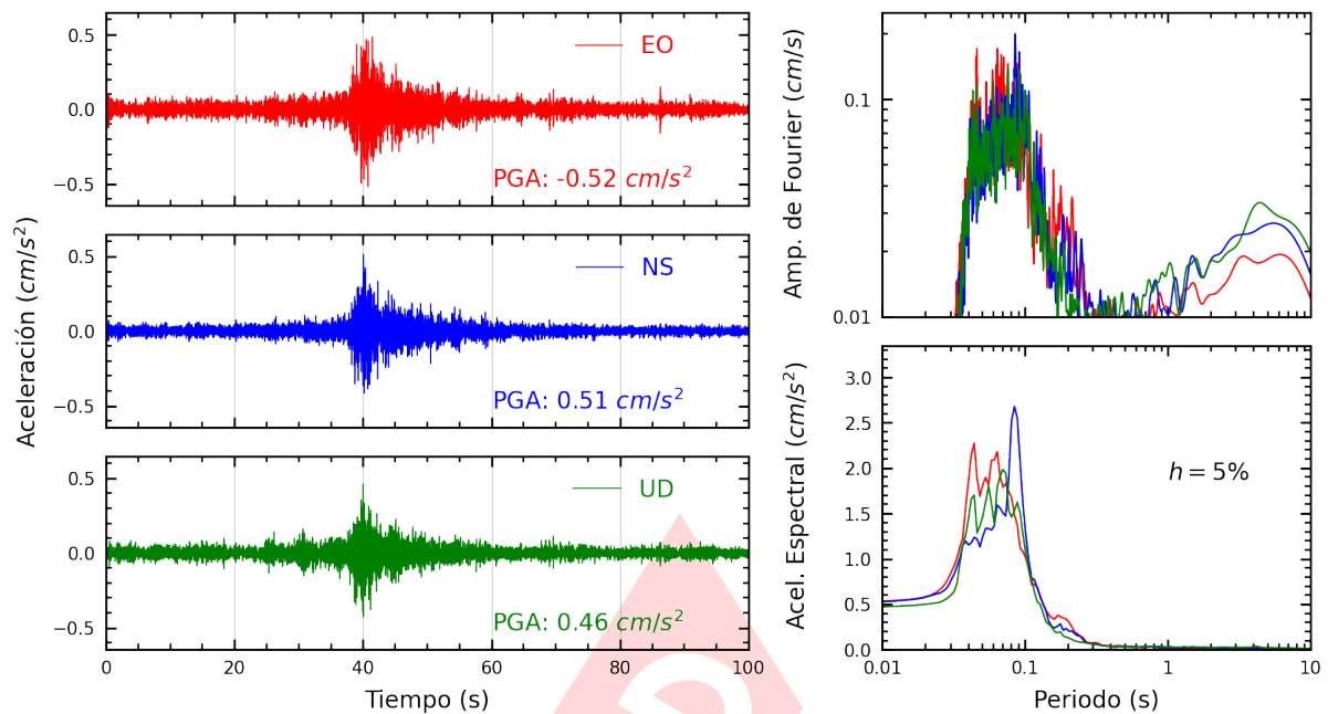
Figura A.11: Registros tiempo-historia, espectros de Fourier y de respuesta en las direcciones EO, NS y vertical de la estación INDEP. Sismo de Mala, Cañete - Lima del 2025-03-07, 22:47:44 (Hora local)
