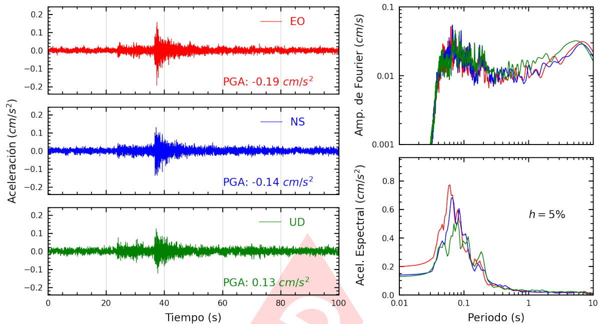
Figura A.27: Registros tiempo-historia, espectros de Fourier y de respuesta en las direcciones EO, NS y vertical de la estación UNFV. Sismo de Mala, Cañete - Lima del 2025-03-07, 22:47:44 (Hora local)
