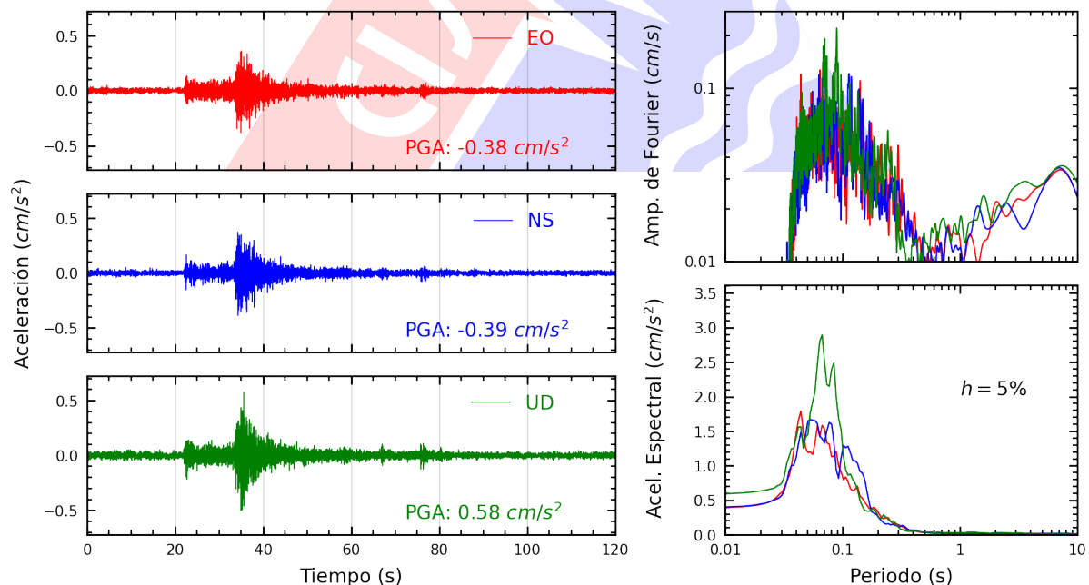
Figura A.10: Registros tiempo-historia, espectros de Fourier y de respuesta en las direcciones EO, NS y vertical de la estación SOVES. Sismo de Mala, Cañete - Lima del 2025-03-07, 22:47:44 (Hora local)
