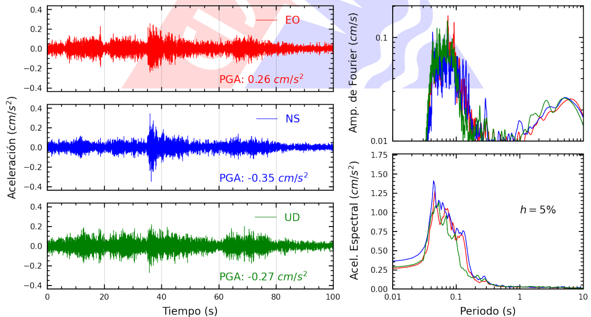
Figura A.16: Registros tiempo-historia, espectros de Fourier y de respuesta en las direcciones EO, NS y vertical de la estación URPE. Sismo de Mala, Cañete - Lima del 2025-03-07, 22:47:44 (Hora local)
