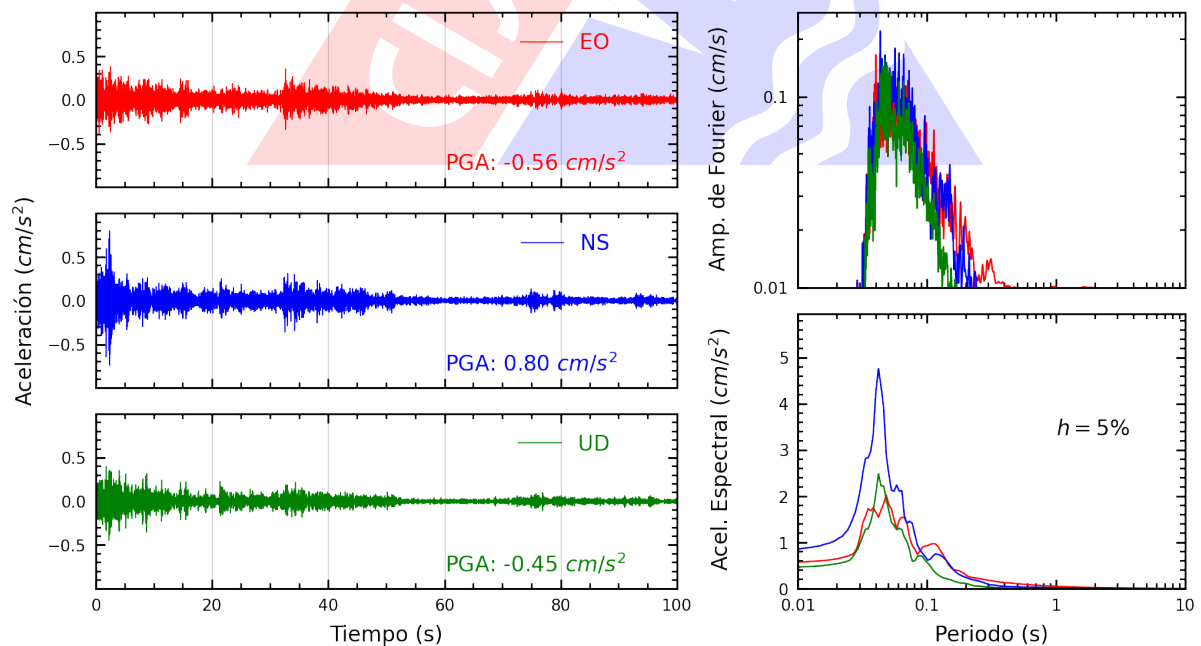
Figura A.6: Registros tiempo-historia, espectros de Fourier y de respuesta en las direcciones EO, NS y vertical de la estación PACHA. Sismo de Mala, Cañete - Lima del 2025-03-07, 22:47:44 (Hora local)
