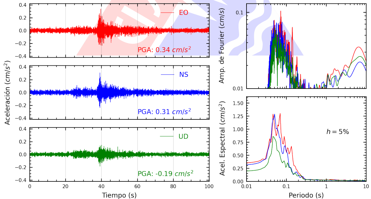
Figura A.18: Registros tiempo-historia, espectros de Fourier y de respuesta en las direcciones EO, NS y vertical de la estación FICPE. Sismo de Mala, Cañete - Lima del 2025-03-07, 22:47:44 (Hora local)
