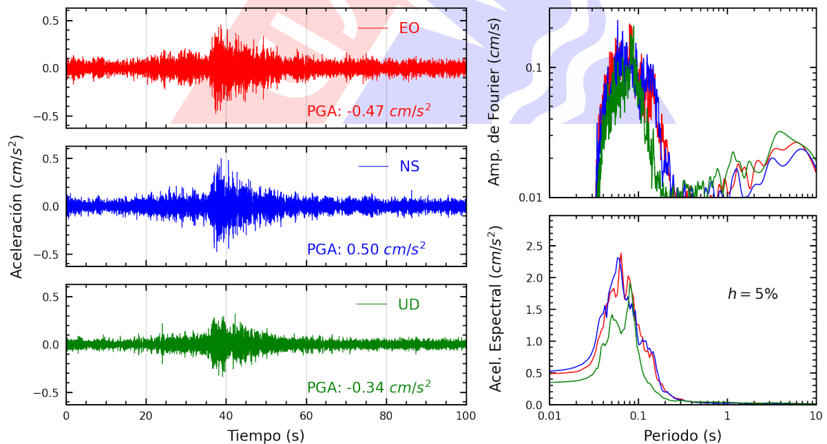
Figura A.12: Registros tiempo-historia, espectros de Fourier y de respuesta en las direcciones EO, NS y vertical de la estación USILM. Sismo de Mala, Cañete - Lima del 2025-03-07, 22:47:44 (Hora local)
