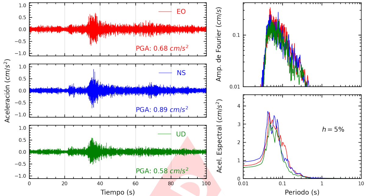
Figura A.5: Registros tiempo-historia, espectros de Fourier y de respuesta en las direcciones EO, NS y vertical de la estación UNTEL. Sismo de Mala, Cañete - Lima del 2025-03-07, 22:47:44 (Hora local)
