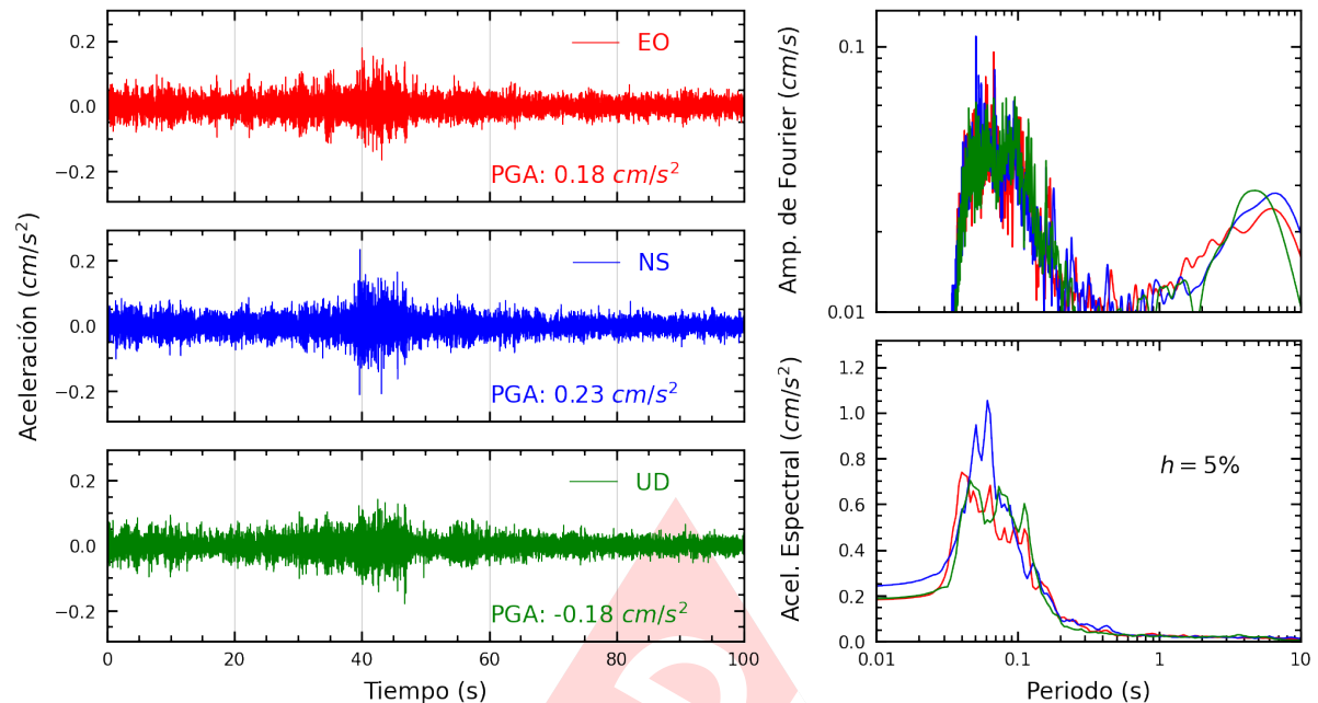
Figura A.25: Registros tiempo-historia, espectros de Fourier y de respuesta en las direcciones EO, NS y vertical de la estación MADRE. Sismo de Mala, Cañete - Lima del 2025-03-07, 22:47:44 (Hora local)
