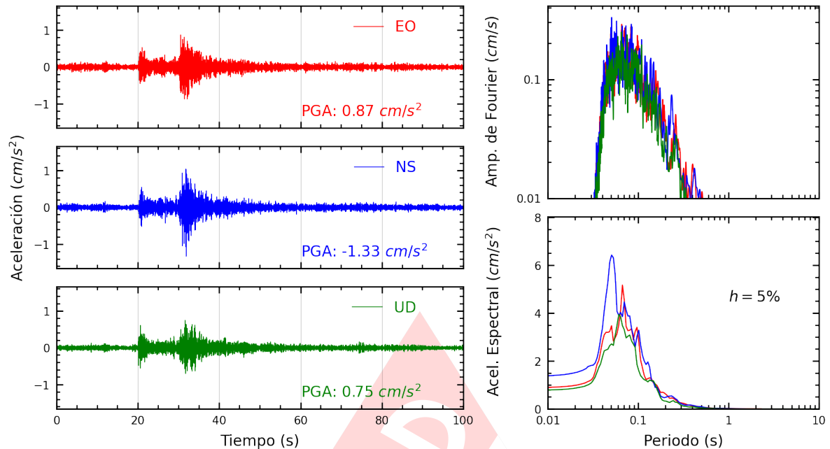
Figura A.3: Registros tiempo-historia, espectros de Fourier y de respuesta en las direcciones EO, NS y vertical de la estación PHER2. Sismo de Mala, Cañete - Lima del 2025-03-07, 22:47:44 (Hora local)
