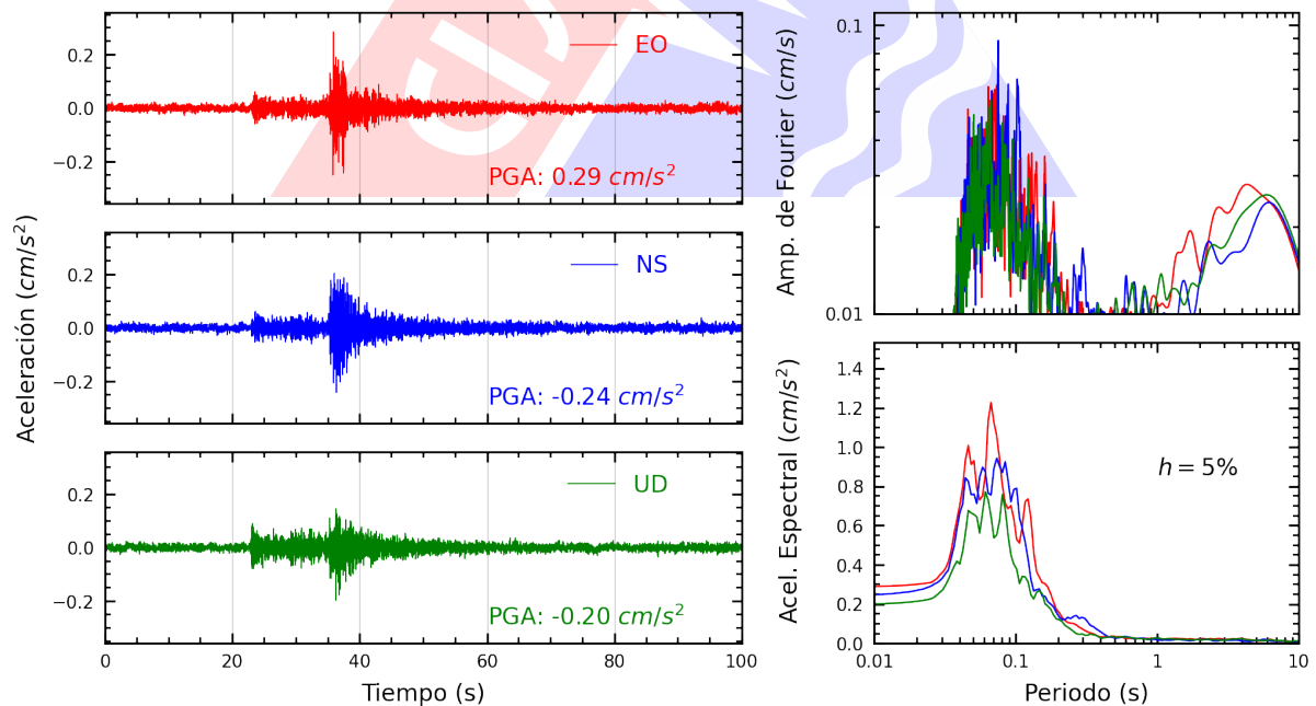
Figura A.20: Registros tiempo-historia, espectros de Fourier y de respuesta en las direcciones EO, NS y vertical de la estación SERVI. Sismo de Mala, Cañete - Lima del 2025-03-07, 22:47:44 (Hora local)
