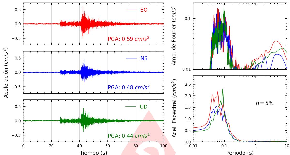
Figura A.9: Registros tiempo-historia, espectros de Fourier y de respuesta en las direcciones EO, NS y vertical de la estación AMORE. Sismo de Mala, Cañete - Lima del 2025-03-07, 22:47:44 (Hora local)
