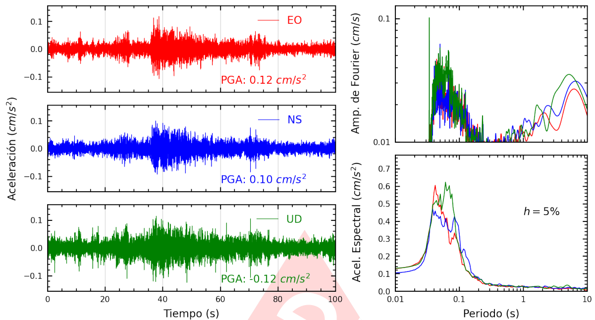
Figura A.31: Registros tiempo-historia, espectros de Fourier y de respuesta en las direcciones EO, NS y vertical de la estación USMP. Sismo de Mala, Cañete - Lima del 2025-03-07, 22:47:44 (Hora local)
