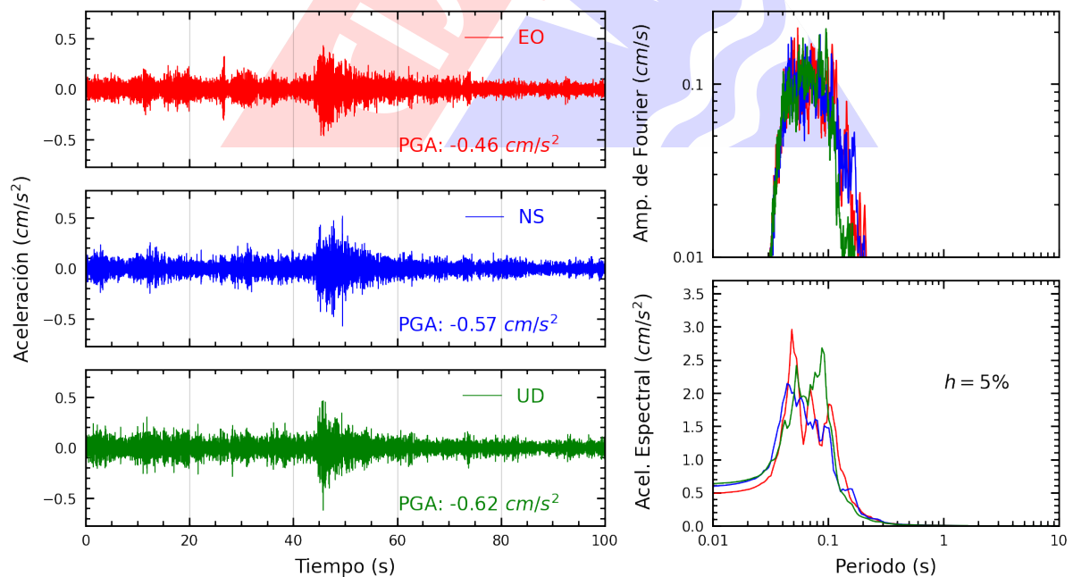
Figura A.8: Registros tiempo-historia, espectros de Fourier y de respuesta en las direcciones EO, NS y vertical de la estación SROS2. Sismo de Mala, Cañete - Lima del 2025-03-07, 22:47:44 (Hora local)
