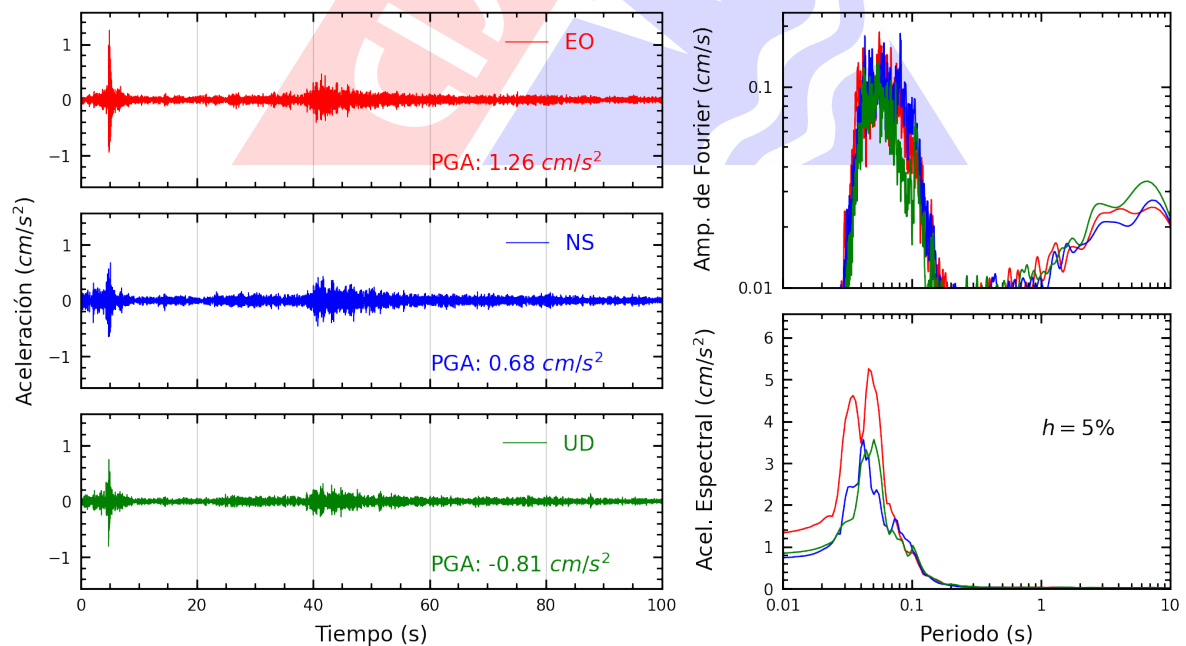
Figura A.4: Registros tiempo-historia, espectros de Fourier y de respuesta en las direcciones EO, NS y vertical de la estación JOSEO. Sismo de Mala, Cañete - Lima del 2025-03-07, 22:47:44 (Hora local)
