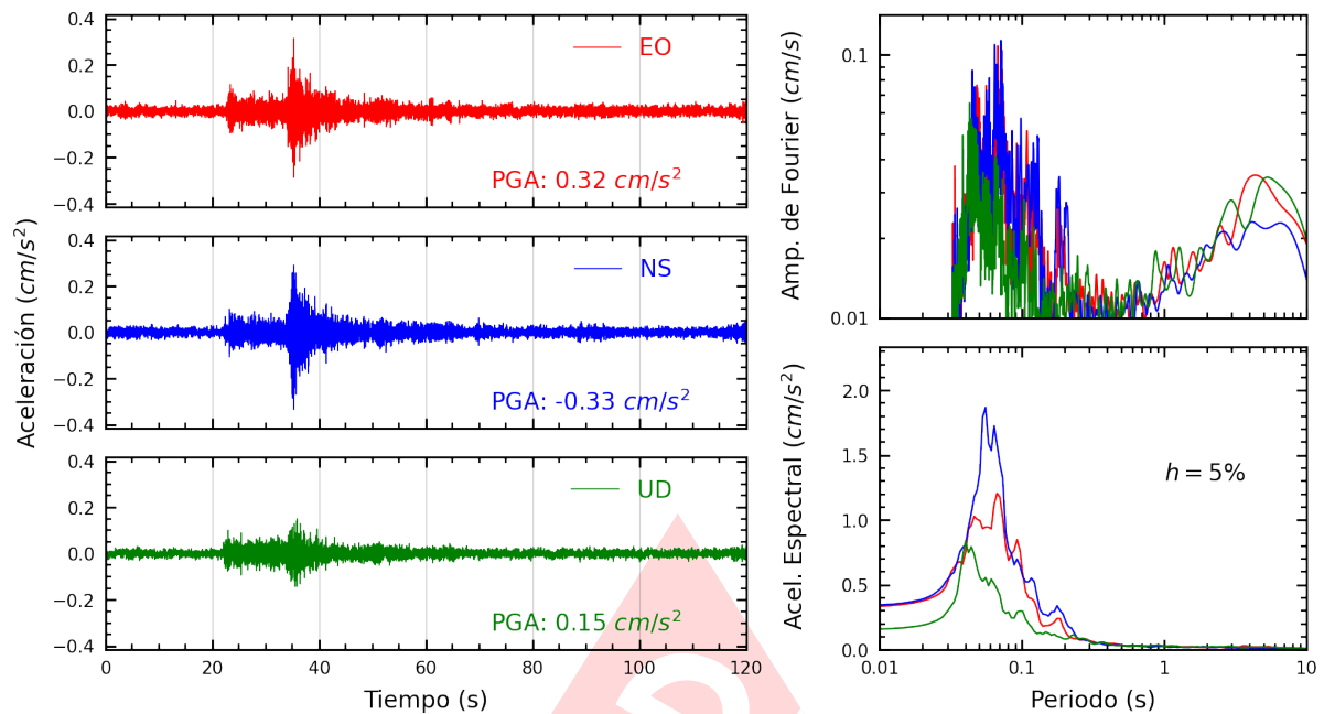
Figura A.19: Registros tiempo-historia, espectros de Fourier y de respuesta en las direcciones EO, NS y vertical de la estación UPCVI. Sismo de Mala, Cañete - Lima del 2025-03-07, 22:47:44 (Hora local)
