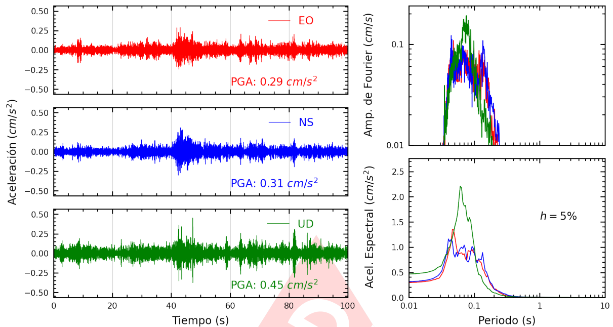
Figura A.13: Registros tiempo-historia, espectros de Fourier y de respuesta en las direcciones EO, NS y vertical de la estación CARA2. Sismo de Mala, Cañete - Lima del 2025-03-07, 22:47:44 (Hora local)
