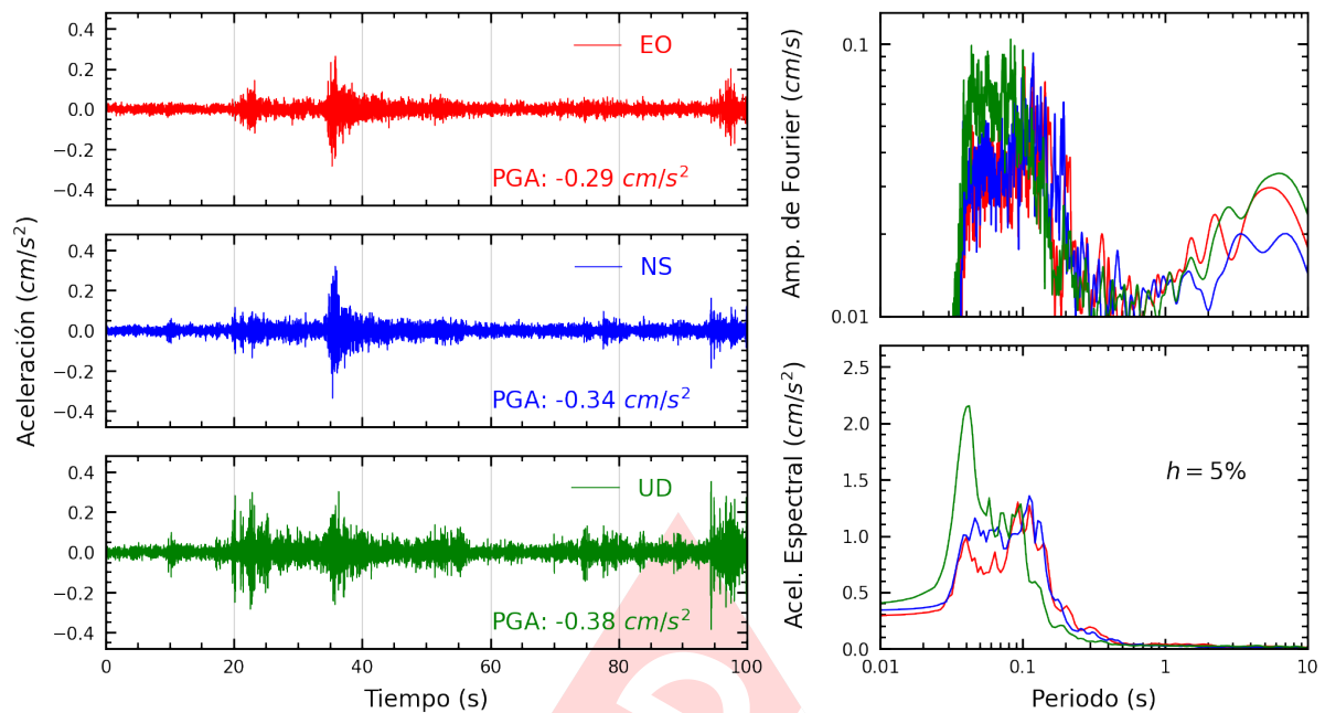
Figura A.15: Registros tiempo-historia, espectros de Fourier y de respuesta en las direcciones EO, NS y vertical de la estación SOCHO. Sismo de Mala, Cañete - Lima del 2025-03-07, 22:47:44 (Hora local)
