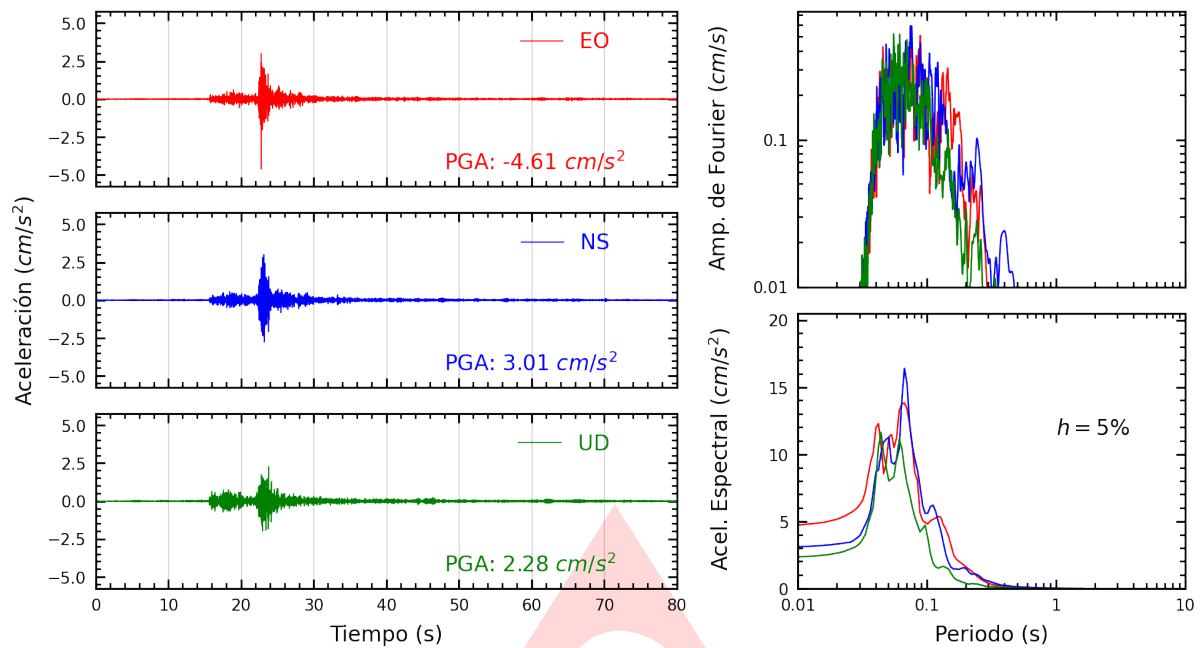
Figura A.1: Registros tiempo-historia, espectros de Fourier y de respuesta en las direcciones EO, NS y vertical de la estación ASIA. Sismo de Mala, Cañete - Lima del 2025-03-07, 22:47:44 (Hora local)
