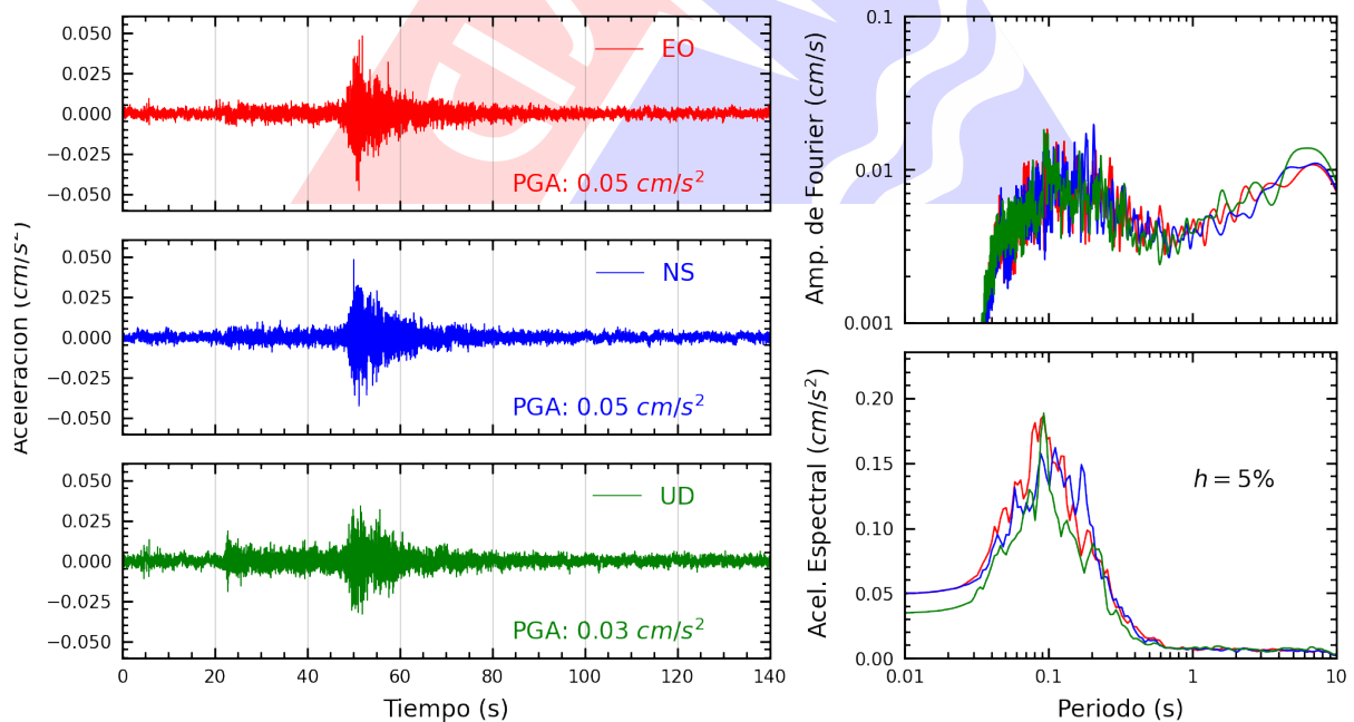
Figura A.32: Registros tiempo-historia, espectros de Fourier y de respuesta en las direcciones EO, NS y vertical de la estación CARAL. Sismo de Mala, Cañete - Lima del 2025-03-07, 22:47:44 (Hora local)
