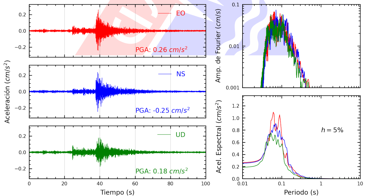
Figura A.24: Registros tiempo-historia, espectros de Fourier y de respuesta en las direcciones EO, NS y vertical de la estación JALV2. Sismo de Mala, Cañete - Lima del 2025-03-07, 22:47:44 (Hora local)
