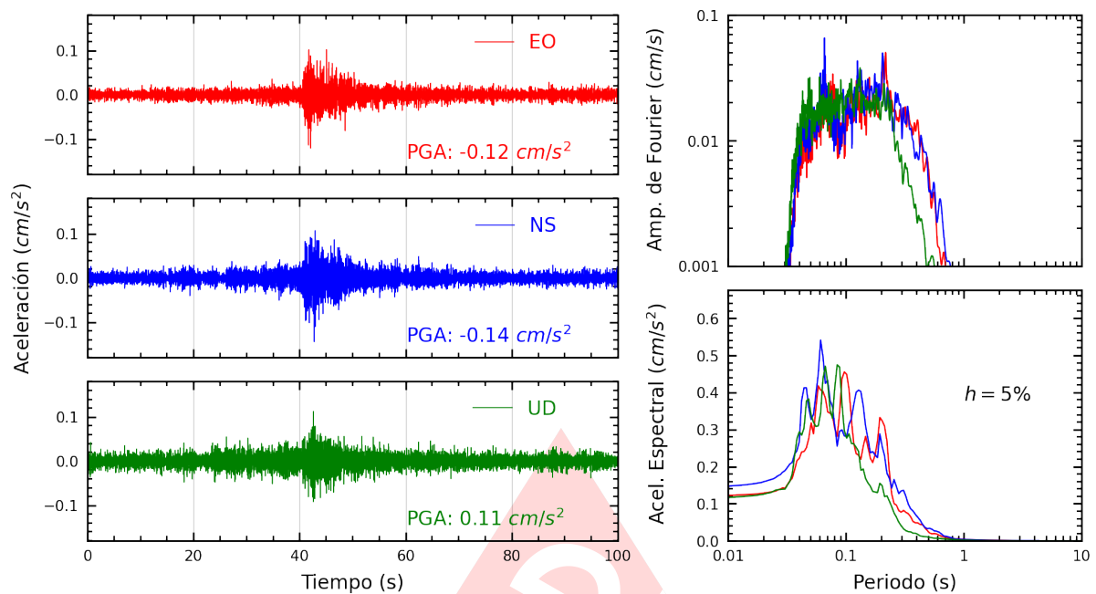
Figura A.29: Registros tiempo-historia, espectros de Fourier y de respuesta en las direcciones EO, NS y vertical de la estación VHAY2. Sismo de Mala, Cañete - Lima del 2025-03-07, 22:47:44 (Hora local)
