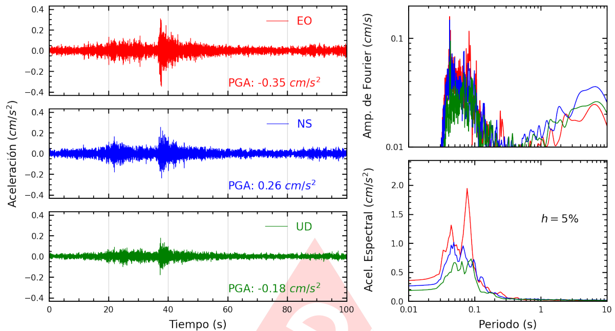
Figura A.17: Registros tiempo-historia, espectros de Fourier y de respuesta en las direcciones EO, NS y vertical de la estación CEPRE. Sismo de Mala, Cañete - Lima del 2025-03-07, 22:47:44 (Hora local)
