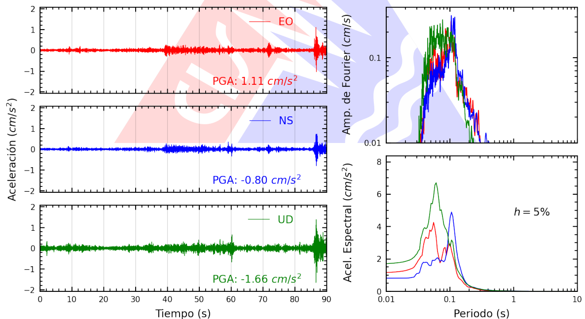
Figura A.2: Registros tiempo-historia, espectros de Fourier y de respuesta en las direcciones EO, NS y vertical de la estación SCOLI. Sismo de Mala, Cañete - Lima del 2025-03-07, 22:47:44 (Hora local)
