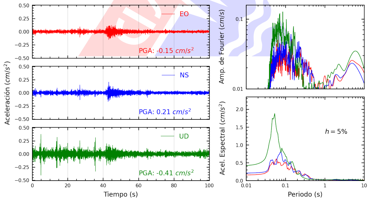
Figura A.14: Registros tiempo-historia, espectros de Fourier y de respuesta en las direcciones EO, NS y vertical de la estación MDPP. Sismo de Mala, Cañete - Lima del 2025-03-07, 22:47:44 (Hora local)
