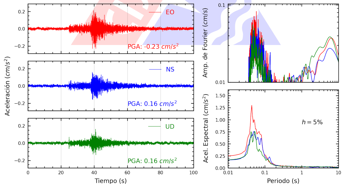
Figura A.26: Registros tiempo-historia, espectros de Fourier y de respuesta en las direcciones EO, NS y vertical de la estación UCSS. Sismo de Mala, Cañete - Lima del 2025-03-07, 22:47:44 (Hora local)
