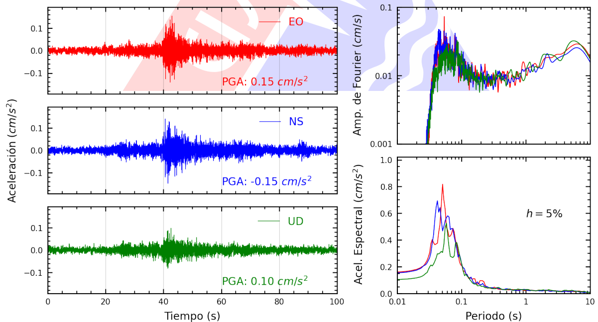
Figura A.28: Registros tiempo-historia, espectros de Fourier y de respuesta en las direcciones EO, NS y vertical de la estación COMAS. Sismo de Mala, Cañete - Lima del 2025-03-07, 22:47:44 (Hora local)
