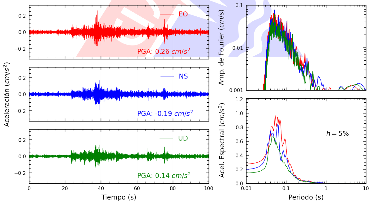
Figura A.22: Registros tiempo-historia, espectros de Fourier y de respuesta en las direcciones EO, NS y vertical de la estación BORJA. Sismo de Mala, Cañete - Lima del 2025-03-07, 22:47:44 (Hora local)
