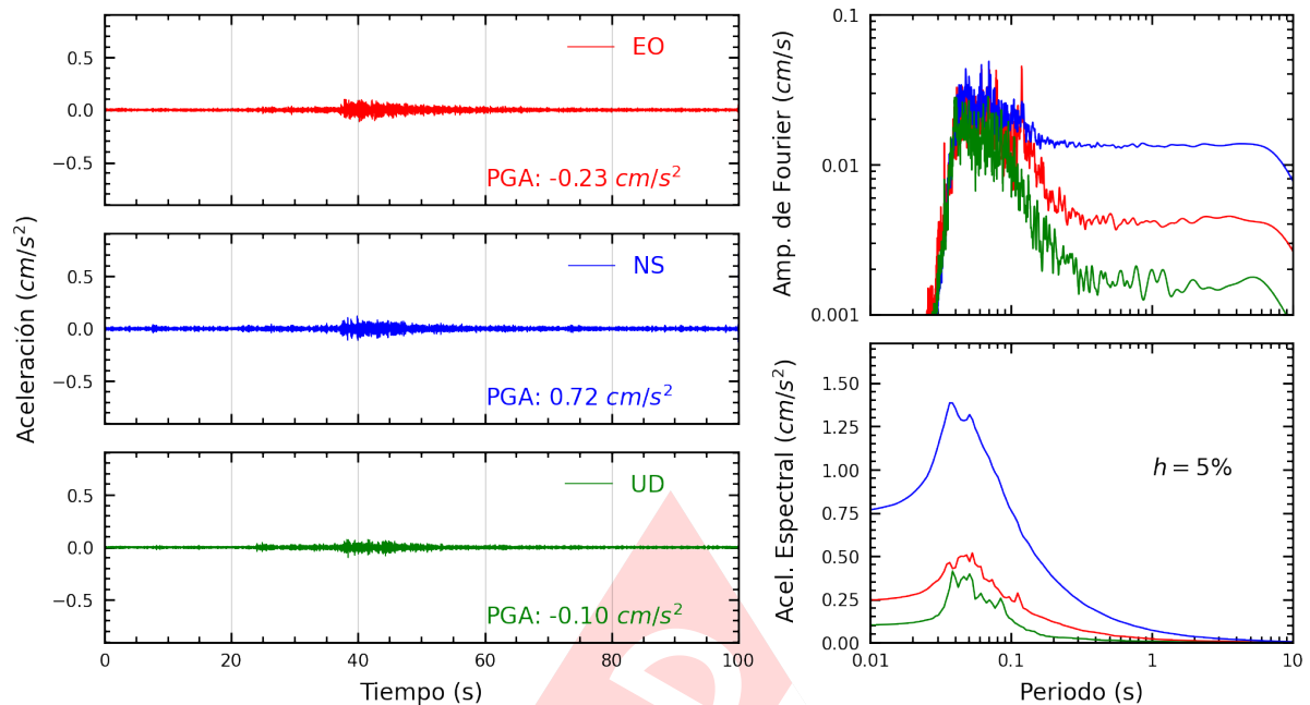
Figura A.7: Registros tiempo-historia, espectros de Fourier y de respuesta en las direcciones EO, NS y vertical de la estación ATARJ. Sismo de Mala, Cañete - Lima del 2025-03-07, 22:47:44 (Hora local)
