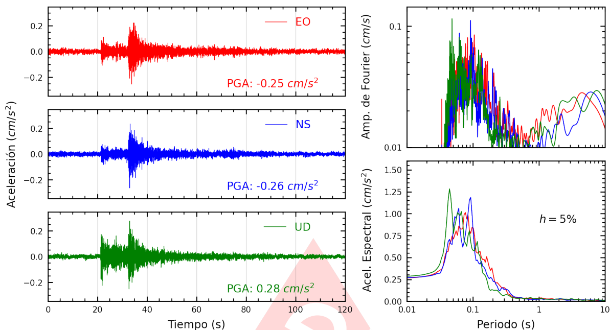
Figura A.21: Registros tiempo-historia, espectros de Fourier y de respuesta en las direcciones EO, NS y vertical de la estación USILP. Sismo de Mala, Cañete - Lima del 2025-03-07, 22:47:44 (Hora local)
