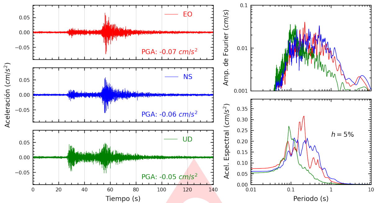
Figura A.1: Registros tiempo-historia, espectros de Fourier y de respuesta en las direcciones EO, NS y vertical de la estación UNIA. Sismo de Codo Del Pozuzo, Puerto Inca - Huanuco del 2025-03-08, 18:55:02 (Hora local)
