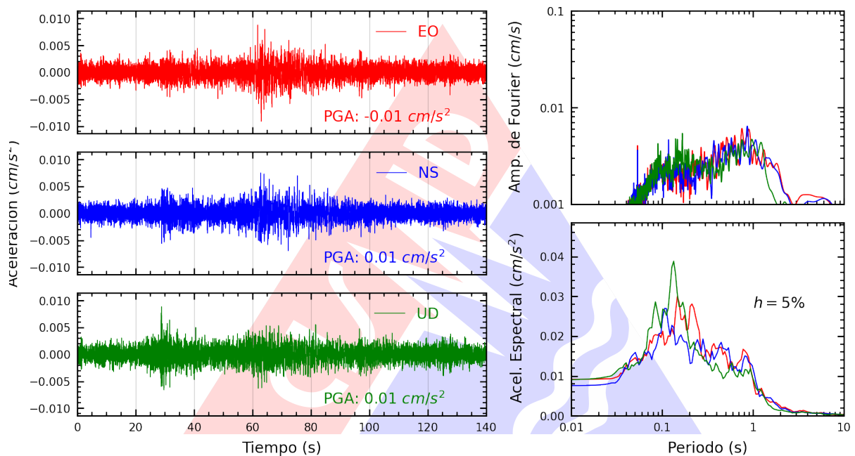
Figura A.3: Registros tiempo-historia, espectros de Fourier y de respuesta en las direcciones EO, NS y vertical de la estación UNCP. Sismo de Codo Del Pozuzo, Puerto Inca - Huanuco del 2025-03-08, 18:55:02 (Hora local)
