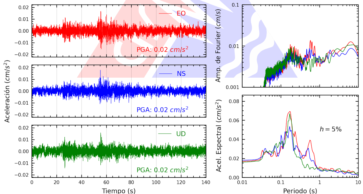
Figura A.2: Registros tiempo-historia, espectros de Fourier y de respuesta en las direcciones EO, NS y vertical de la estación CARAL. Sismo de Codo Del Pozuzo, Puerto Inca - Huanuco del 2025-03-08, 18:55:02 (Hora local)
