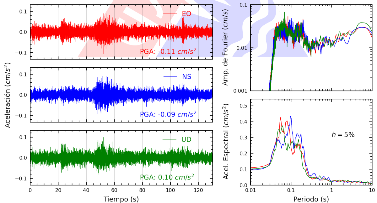
Figura A.12: Registros tiempo-historia, espectros de Fourier y de respuesta en las direcciones EO, NS y vertical de la estación IMCA. Sismo de Castrovirreyna, Castrovirreyna - Huancavelica del 2025-03-09, 11:49:49 (Hora local)
