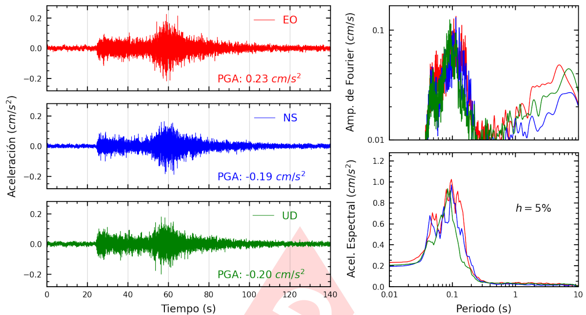
Figura A.7: Registros tiempo-historia, espectros de Fourier y de respuesta en las direcciones EO, NS y vertical de la estación AMORE. Sismo de Castrovirreyna, Castrovirreyna - Huancavelica del 2025-03-09, 11:49:49 (Hora local)
