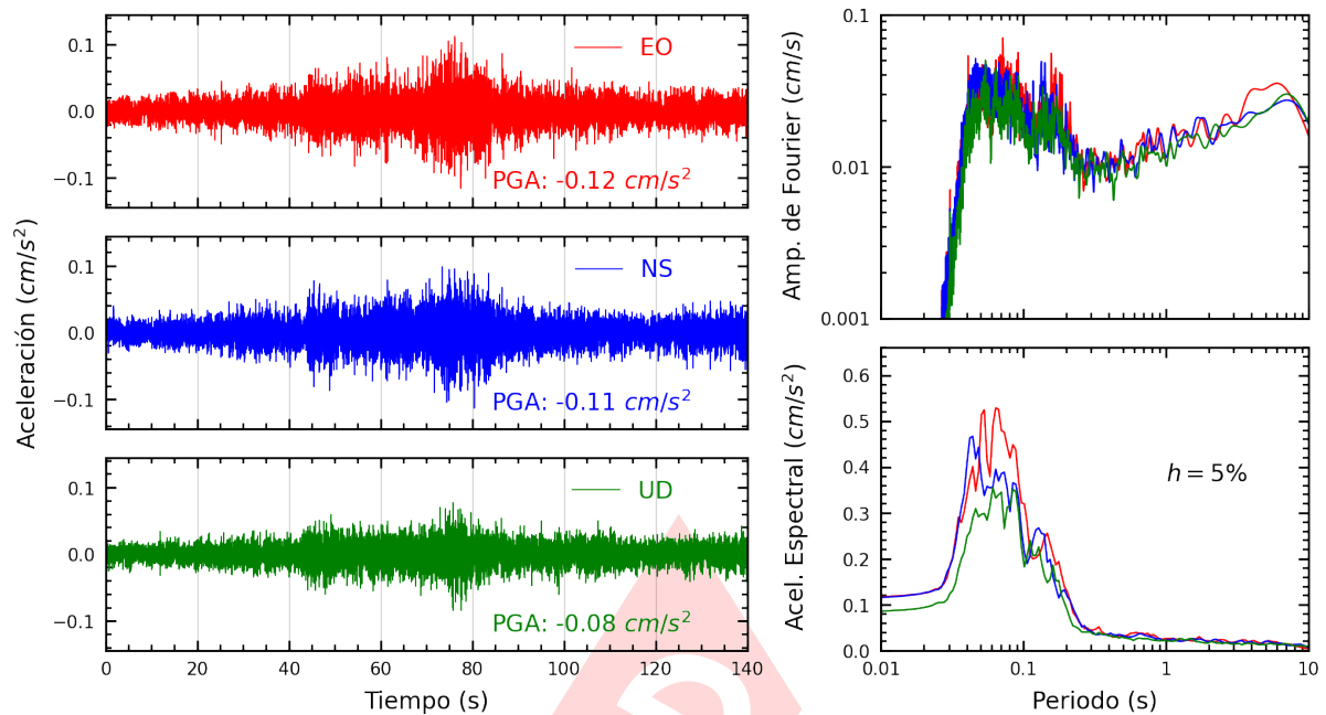
Figura A.11: Registros tiempo-historia, espectros de Fourier y de respuesta en las direcciones EO, NS y vertical de la estación FICPE. Sismo de Castrovirreyna, Castrovirreyna - Huancavelica del 2025-03-09, 11:49:49 (Hora local)
