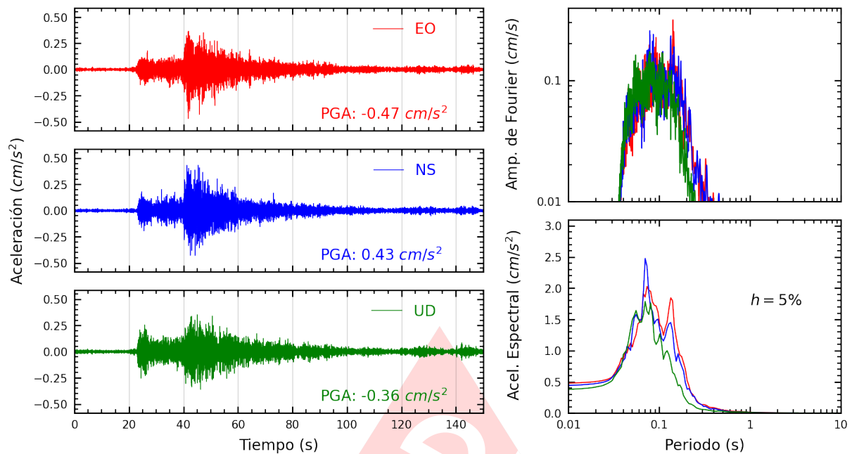
Figura A.3: Registros tiempo-historia, espectros de Fourier y de respuesta en las direcciones EO, NS y vertical de la estación ASIA. Sismo de Castrovirreyna, Castrovirreyna - Huancavelica del 2025-03-09, 11:49:49 (Hora local)
