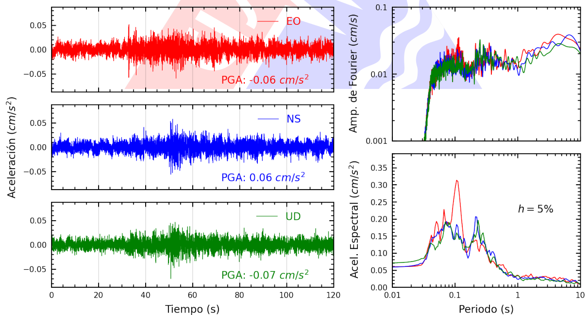
Figura A.16: Registros tiempo-historia, espectros de Fourier y de respuesta en las direcciones EO, NS y vertical de la estación UNSCH. Sismo de Castrovirreyna, Castrovirreyna - Huancavelica del 2025-03-09, 11:49:49 (Hora local)
