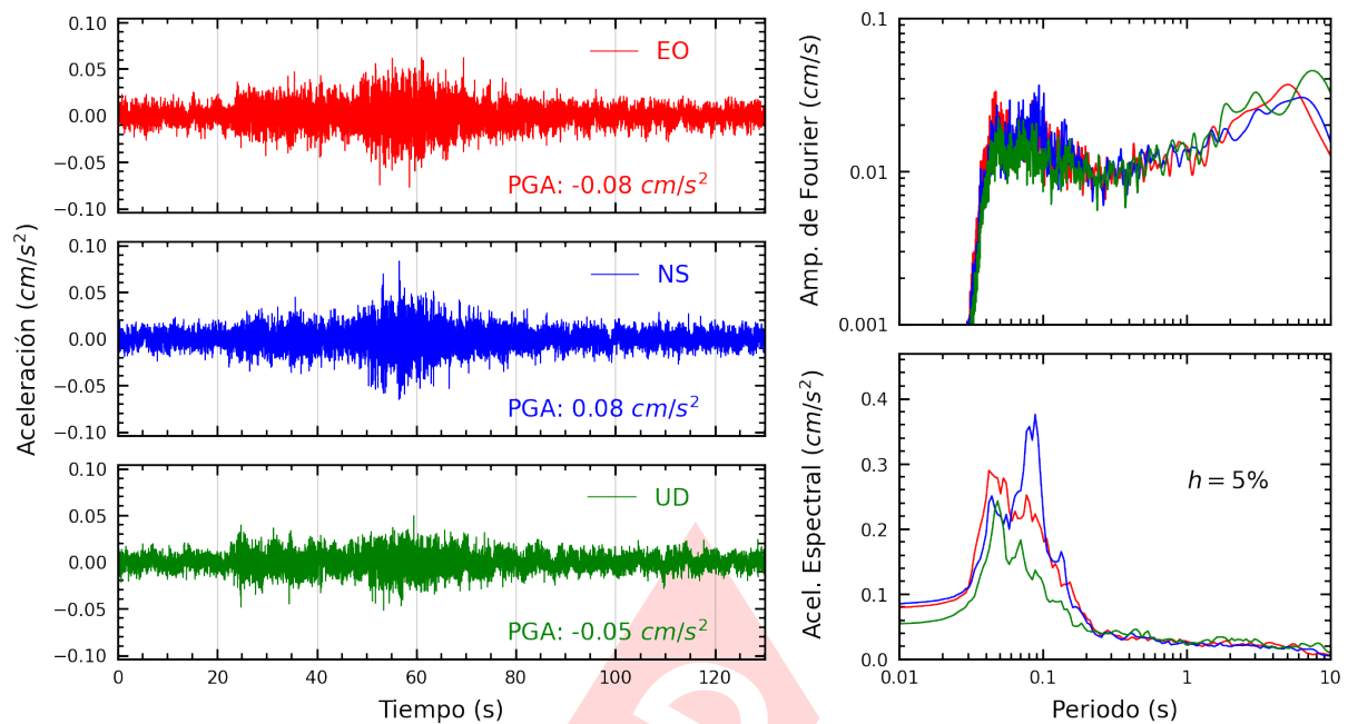
Figura A.15: Registros tiempo-historia, espectros de Fourier y de respuesta en las direcciones EO, NS y vertical de la estación UCSS. Sismo de Castrovirreyna, Castrovirreyna - Huancavelica del 2025-03-09, 11:49:49 (Hora local)
