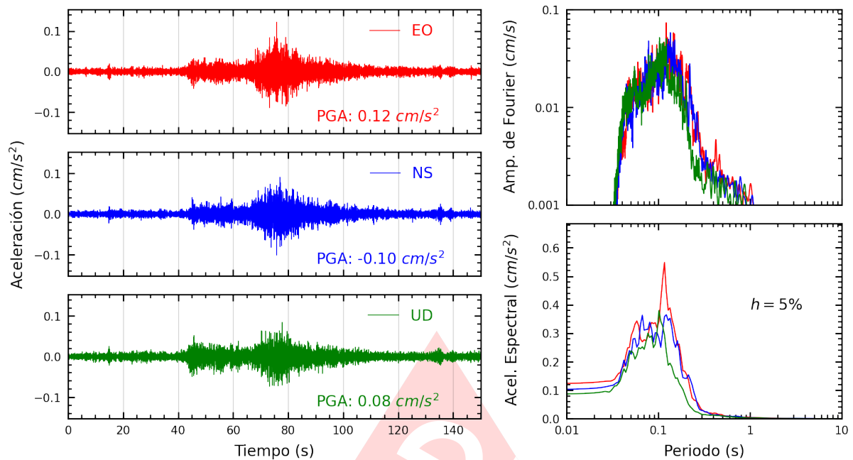
Figura A.9: Registros tiempo-historia, espectros de Fourier y de respuesta en las direcciones EO, NS y vertical de la estación JALV2. Sismo de Castrovirreyna, Castrovirreyna - Huancavelica del 2025-03-09, 11:49:49 (Hora local)
