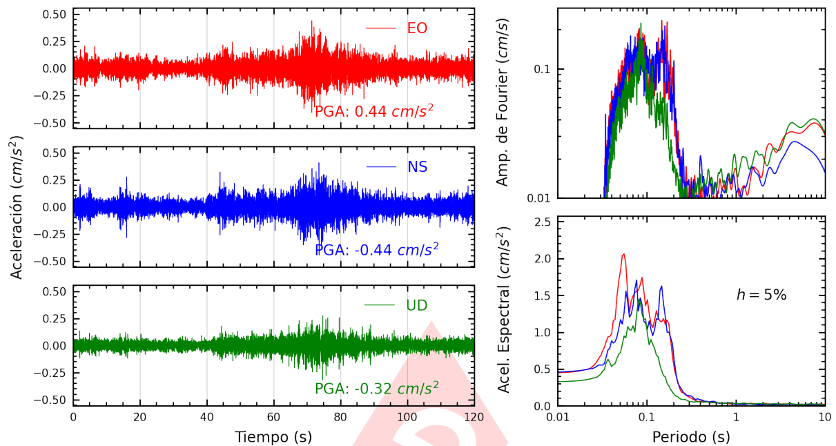
Figura A.5: Registros tiempo-historia, espectros de Fourier y de respuesta en las direcciones EO, NS y vertical de la estación USILM. Sismo de Castrovirreyna, Castrovirreyna - Huancavelica del 2025-03-09, 11:49:49 (Hora local)
