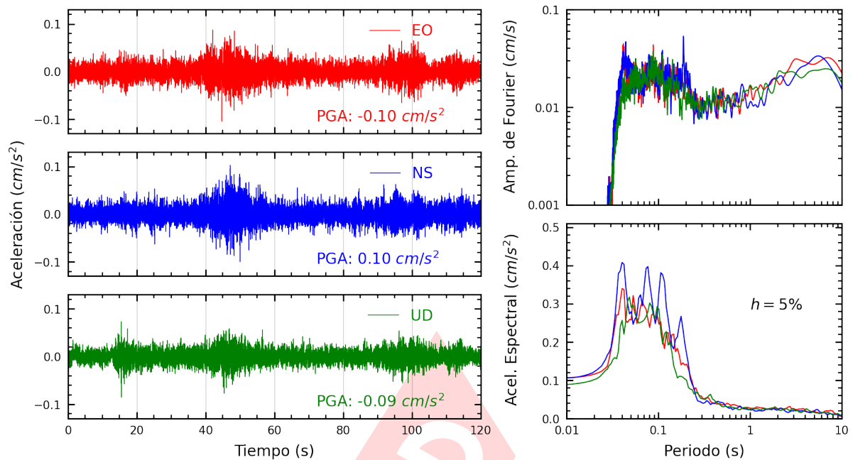
Figura A.13: Registros tiempo-historia, espectros de Fourier y de respuesta en las direcciones EO, NS y vertical de la estación COMAS. Sismo de Castrovirreyna, Castrovirreyna - Huancavelica del 2025-03-09, 11:49:49 (Hora local)
