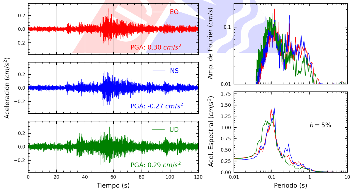
Figura A.6: Registros tiempo-historia, espectros de Fourier y de respuesta en las direcciones EO, NS y vertical de la estación UNICA. Sismo de Castrovirreyna, Castrovirreyna - Huancavelica del 2025-03-09, 11:49:49 (Hora local)
