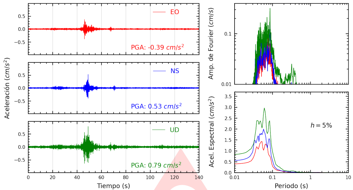
Figura A.1: Registros tiempo-historia, espectros de Fourier y de respuesta en las direcciones EO, NS y vertical de la estación SCCUS. Sismo de Castrovirreyna, Castrovirreyna - Huancavelica del 2025-03-09, 11:49:49 (Hora local)
