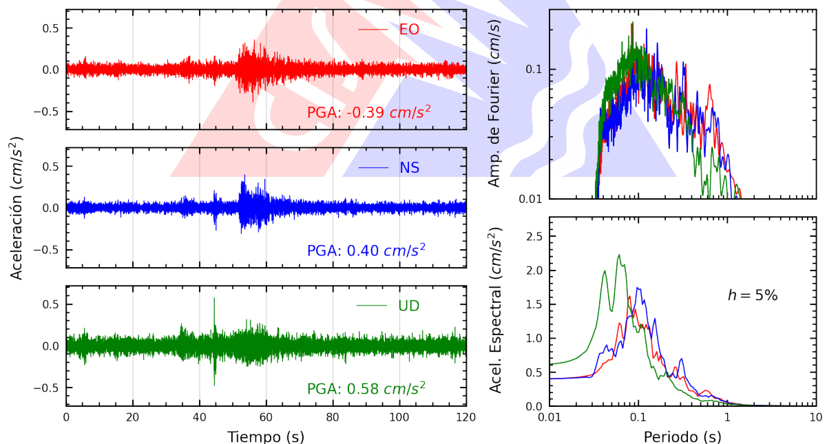
Figura A.2: Registros tiempo-historia, espectros de Fourier y de respuesta en las direcciones EO, NS y vertical de la estación SCICA. Sismo de Castrovirreyna, Castrovirreyna - Huancavelica del 2025-03-09, 11:49:49 (Hora local)
