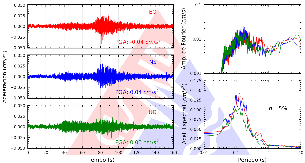
Figura A.17: Registros tiempo-historia, espectros de Fourier y de respuesta en las direcciones EO, NS y vertical de la estación CARAL. Sismo de Castrovirreyna, Castrovirreyna - Huancavelica del 2025-03-09, 11:49:49 (Hora local)
