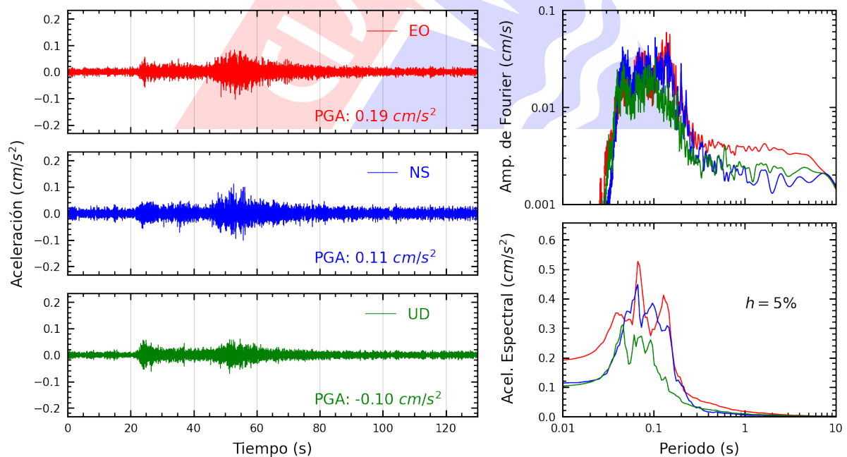
Figura A.8: Registros tiempo-historia, espectros de Fourier y de respuesta en las direcciones EO, NS y vertical de la estación ATARJ. Sismo de Castrovirreyna, Castrovirreyna - Huancavelica del 2025-03-09, 11:49:49 (Hora local)
