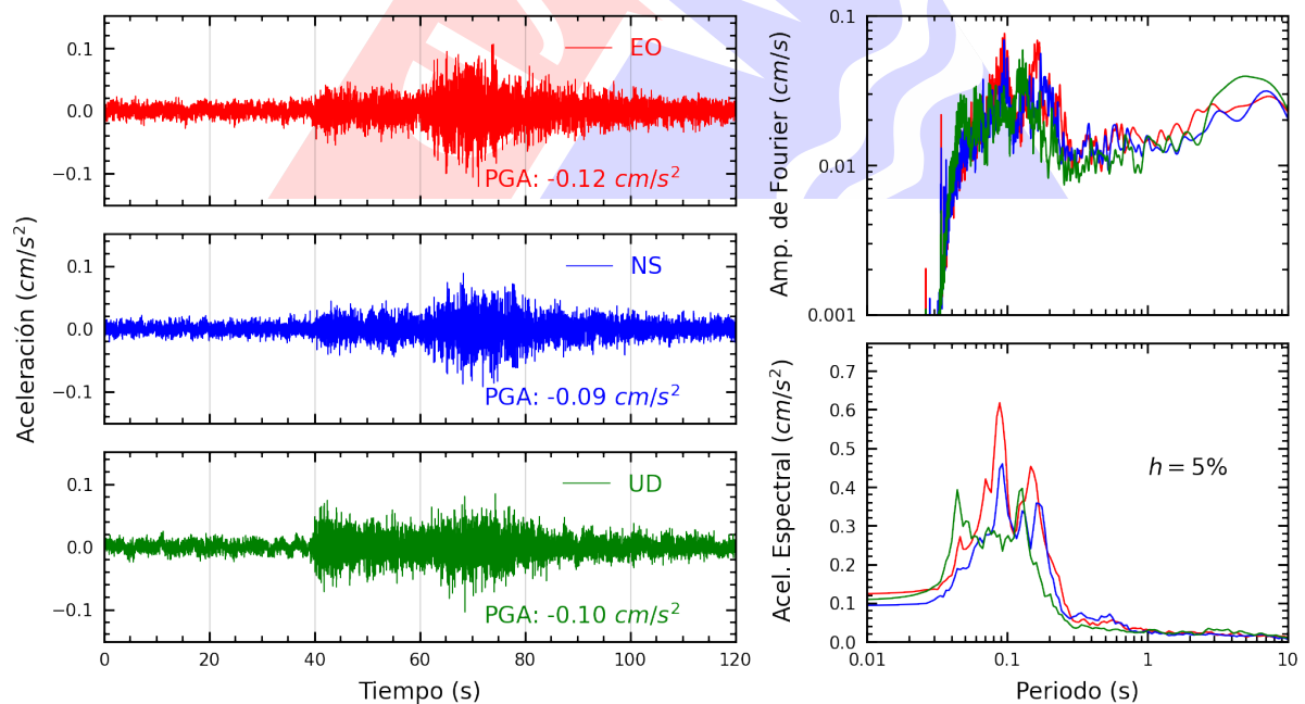
Figura A.10: Registros tiempo-historia, espectros de Fourier y de respuesta en las direcciones EO, NS y vertical de la estación USILP. Sismo de Castrovirreyna, Castrovirreyna - Huancavelica del 2025-03-09, 11:49:49 (Hora local)
