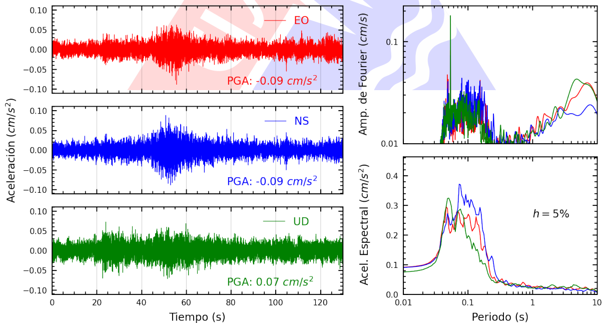
Figura A.14: Registros tiempo-historia, espectros de Fourier y de respuesta en las direcciones EO, NS y vertical de la estación SERVI. Sismo de Castrovirreyna, Castrovirreyna - Huancavelica del 2025-03-09, 11:49:49 (Hora local)
