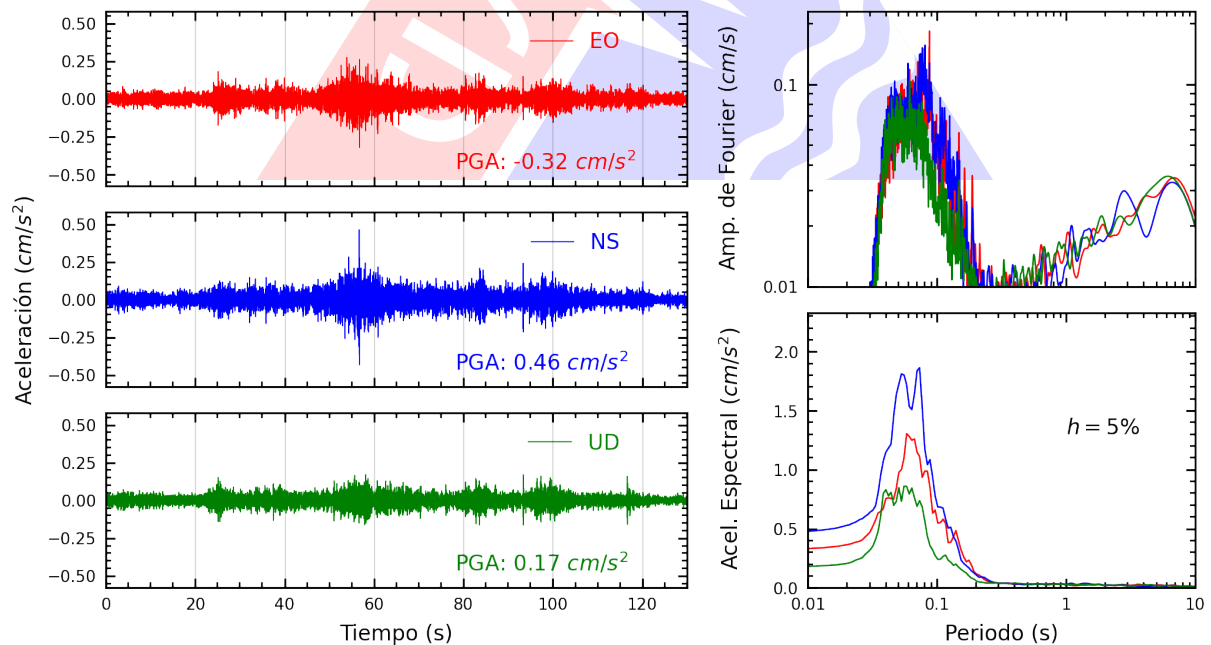
Figura A.4: Registros tiempo-historia, espectros de Fourier y de respuesta en las direcciones EO, NS y vertical de la estación JOSEO. Sismo de Castrovirreyna, Castrovirreyna - Huancavelica del 2025-03-09, 11:49:49 (Hora local)
