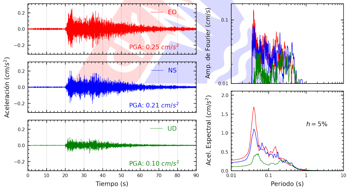
Figura A.2: Registros tiempo-historia, espectros de Fourier y de respuesta en las direcciones EO, NS y vertical de la estación UNAM. Sismo de Mollendo, Islay - Arequipa del 2025-03-13, 04:54:26 (Hora local)
