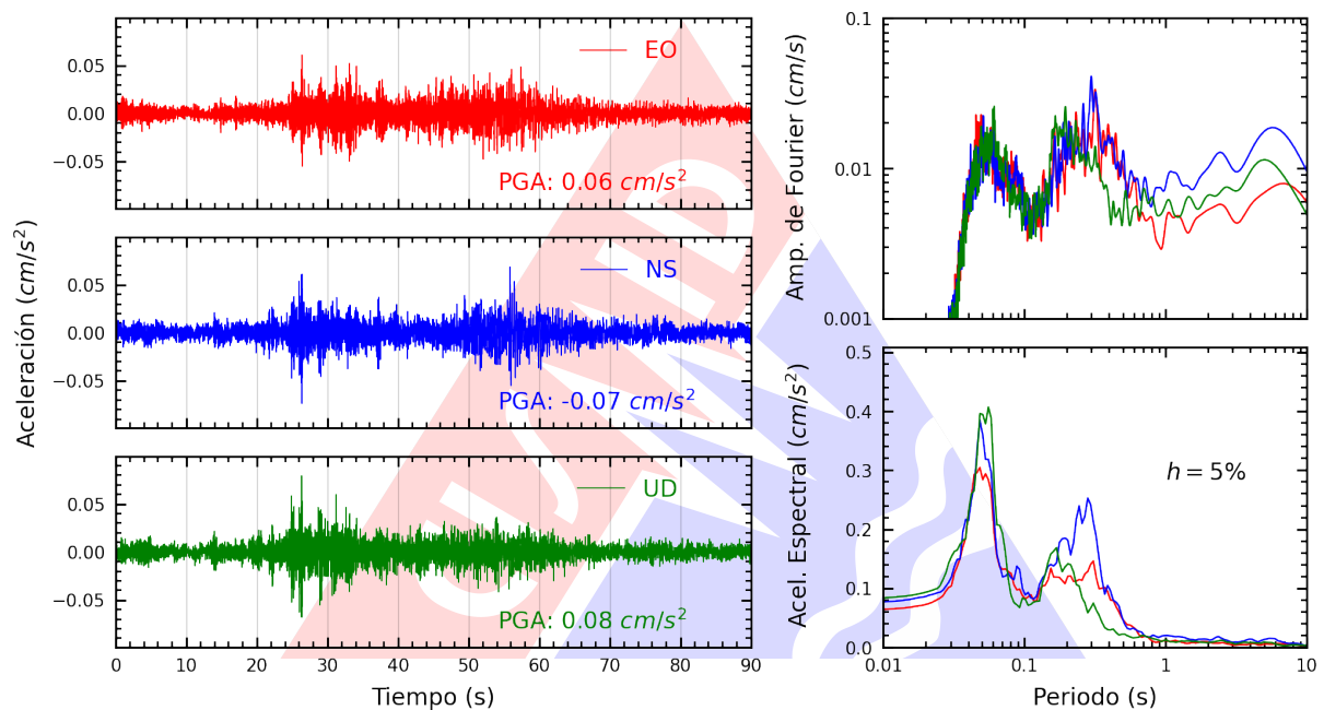
Figura A.3: Registros tiempo-historia, espectros de Fourier y de respuesta en las direcciones EO, NS y vertical de la estación CREY. Sismo de Mollendo, Islay - Arequipa del 2025-03-13, 04:54:26 (Hora local)
