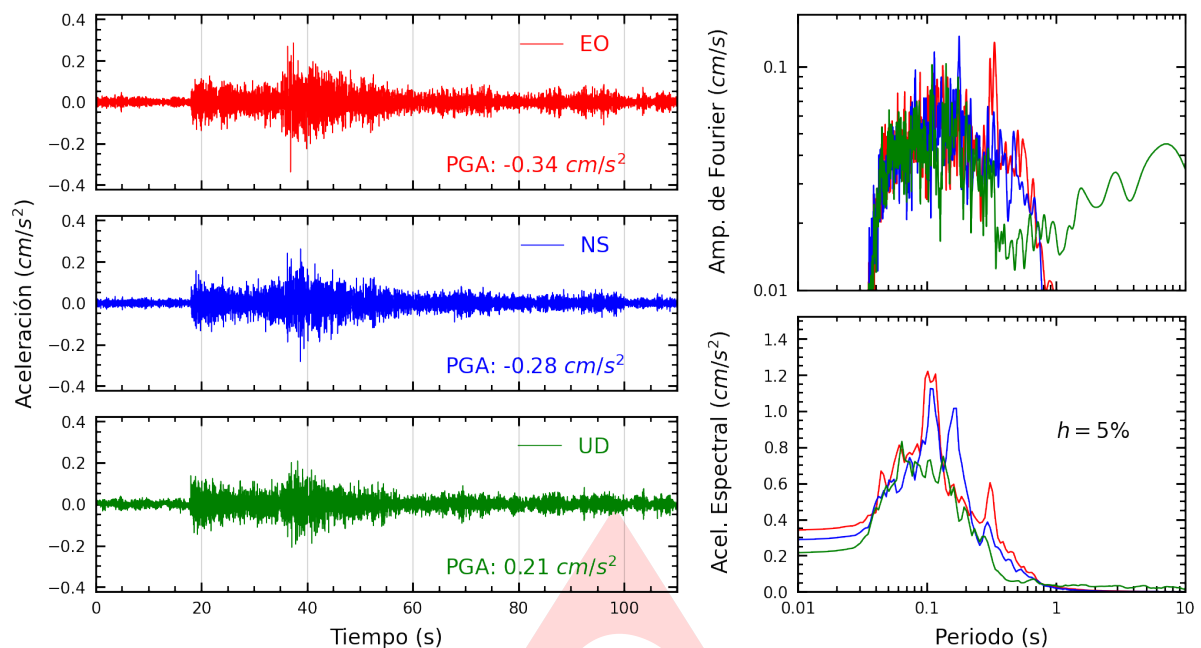
Figura A.1: Registros tiempo-historia, espectros de Fourier y de respuesta en las direcciones EO, NS y vertical de la estación SCARQ. Sismo de Mollendo, Islay - Arequipa del 2025-03-13, 04:54:26 (Hora local)
