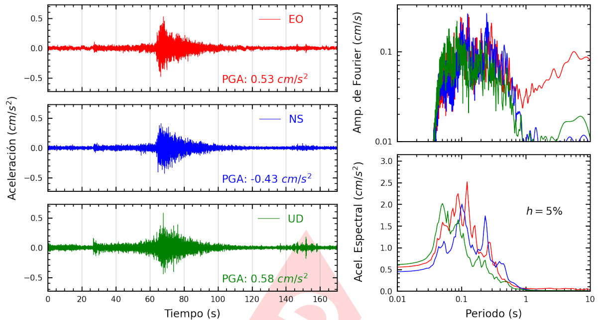
Figura A.5: Registros tiempo-historia, espectros de Fourier y de respuesta en las direcciones EO, NS y vertical de la estación UJBG3. Sismo de Caraveli, Caraveli - Arequipa del 2025-03-15, 21:20:53 (Hora local)
