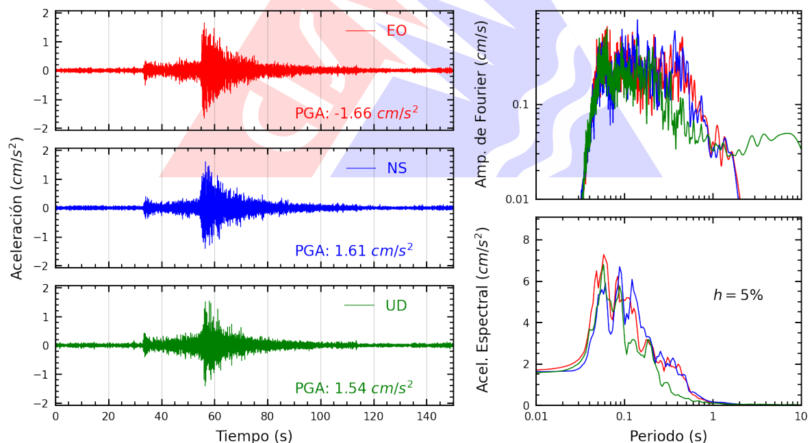
Figura A.2: Registros tiempo-historia, espectros de Fourier y de respuesta en las direcciones EO, NS y vertical de la estación SCARQ. Sismo de Caraveli, Caraveli - Arequipa del 2025-03-15, 21:20:53 (Hora local)
