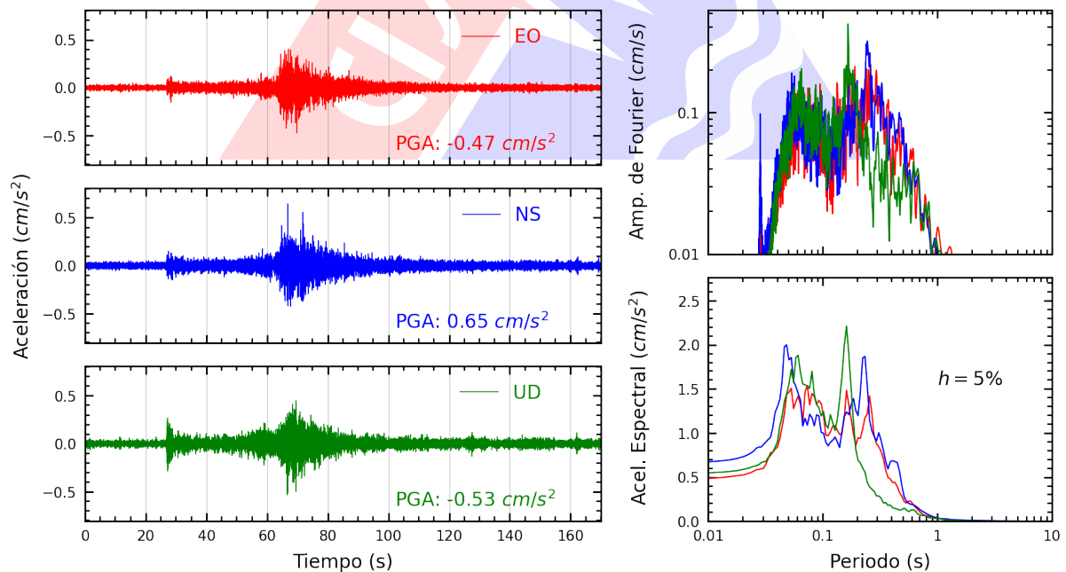
Figura A.4: Registros tiempo-historia, espectros de Fourier y de respuesta en las direcciones EO, NS y vertical de la estación UJB4. Sismo de Caraveli, Caraveli - Arequipa del 2025-03-15, 21:20:53 (Hora local)
