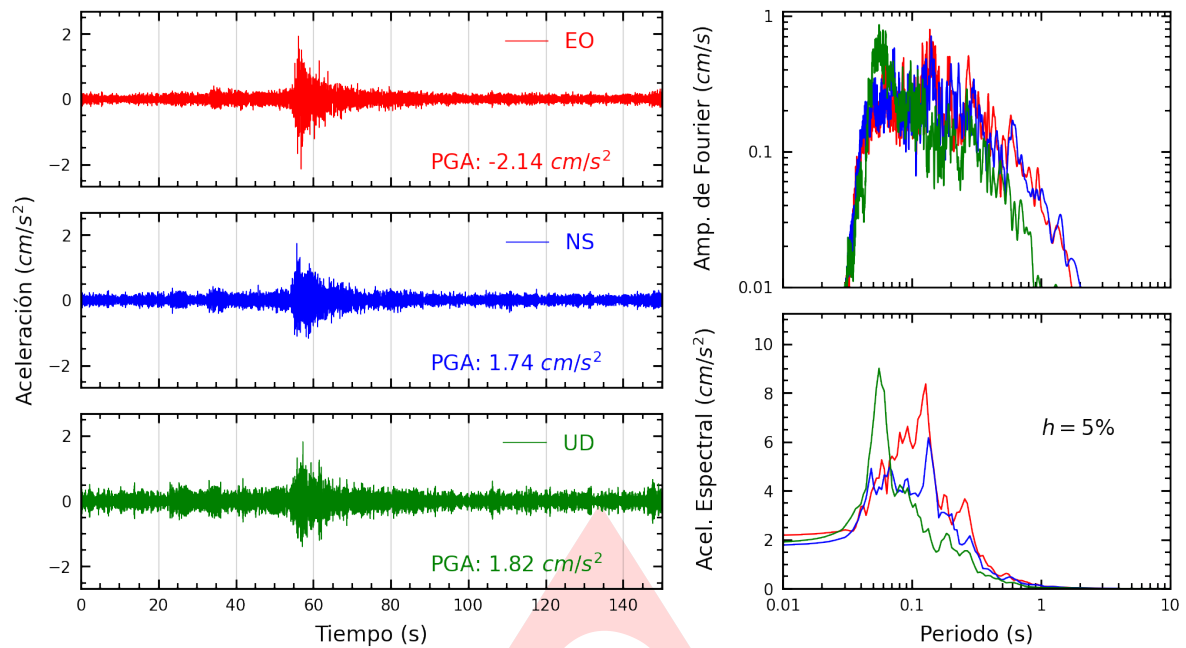
Figura A.1: Registros tiempo-historia, espectros de Fourier y de respuesta en las direcciones EO, NS y vertical de la estación SCAR2. Sismo de Caraveli, Caraveli - Arequipa del 2025-03-15, 21:20:53 (Hora local)
