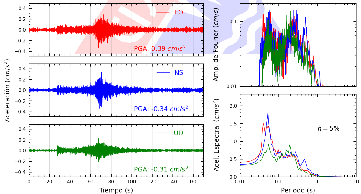
Figura A.6: Registros tiempo-historia, espectros de Fourier y de respuesta en las direcciones EO, NS y vertical de la estación UPTAC. Sismo de Caraveli, Caraveli - Arequipa del 2025-03-15, 21:20:53 (Hora local)
