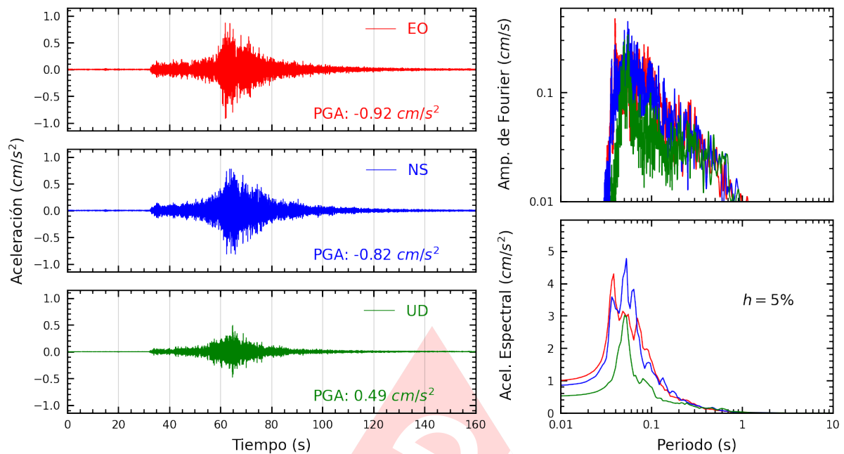
Figura A.3: Registros tiempo-historia, espectros de Fourier y de respuesta en las direcciones EO, NS y vertical de la estación UNAM. Sismo de Caraveli, Caraveli - Arequipa del 2025-03-15, 21:20:53 (Hora local)
