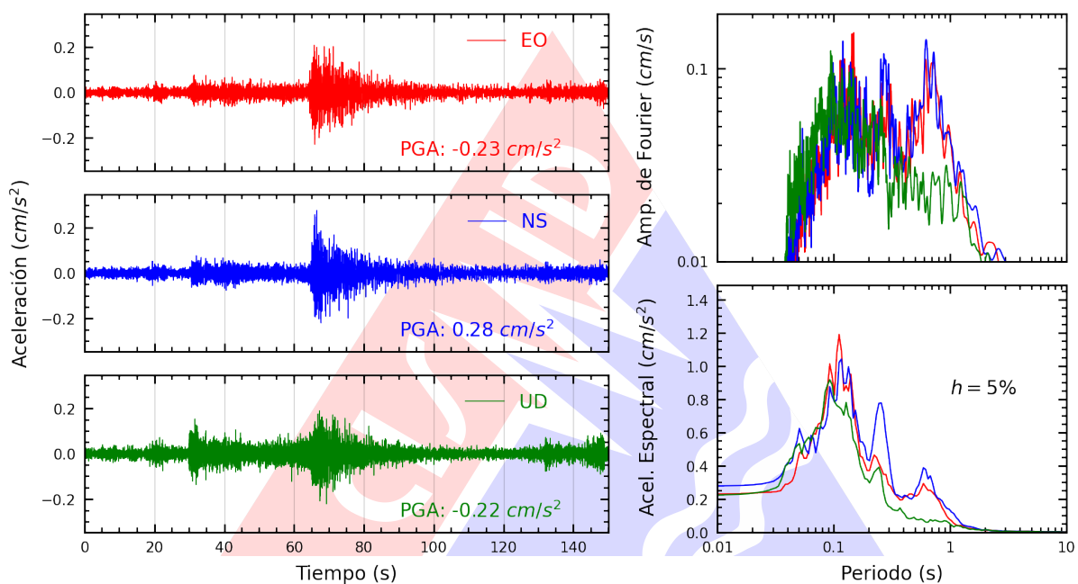
Figura A.7: Registros tiempo-historia, espectros de Fourier y de respuesta en las direcciones EO, NS y vertical de la estación UNICA. Sismo de Caraveli, Caraveli - Arequipa del 2025-03-15, 21:20:53 (Hora local)
