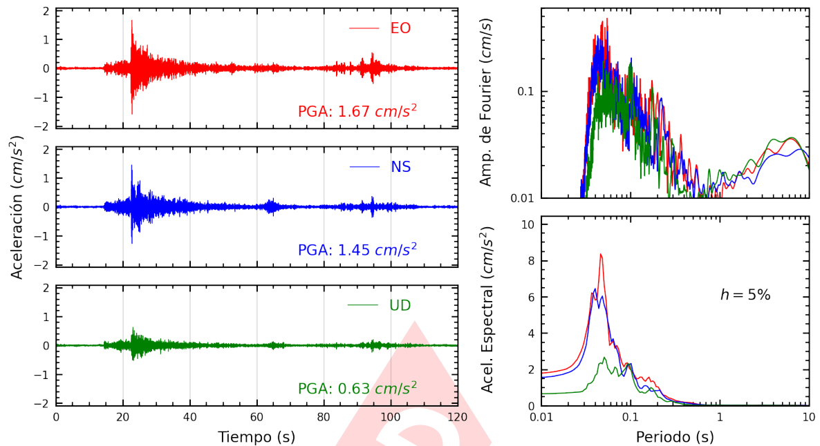
Figura A.7: Registros tiempo-historia, espectros de Fourier y de respuesta en las direcciones EO, NS y vertical de la estación OLIVO. Sismo de Provincia Constitucional del Callao , Callao - Lima del 2025-03-17, 02:35:03 (Hora local)
