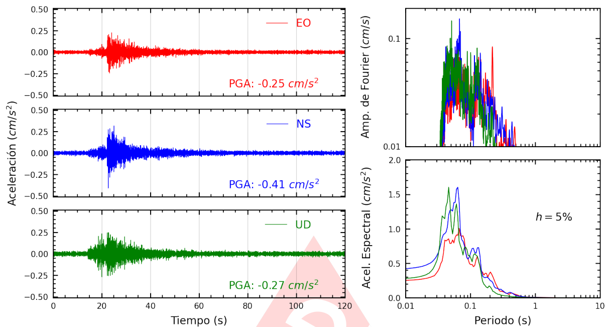
Figura A.33: Registros tiempo-historia, espectros de Fourier y de respuesta en las direcciones EO, NS y vertical de la estación VHAY2. Sismo de Provincia Constitucional del Callao , Callao - Lima del 2025-03-17, 02:35:03 (Hora local)
