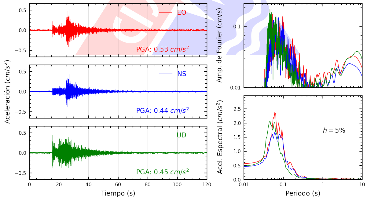
Figura A.30: Registros tiempo-historia, espectros de Fourier y de respuesta en las direcciones EO, NS y vertical de la estación USILP. Sismo de Provincia Constitucional del Callao , Callao - Lima del 2025-03-17, 02:35:03 (Hora local)
