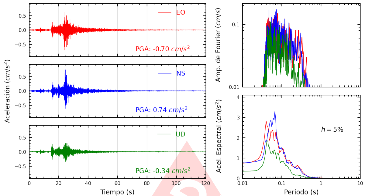
Figura A.25: Registros tiempo-historia, espectros de Fourier y de respuesta en las direcciones EO, NS y vertical de la estación BRISA. Sismo de Provincia Constitucional del Callao , Callao - Lima del 2025-03-17, 02:35:03 (Hora local)
