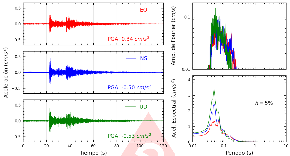
Figura A.29: Registros tiempo-historia, espectros de Fourier y de respuesta en las direcciones EO, NS y vertical de la estación ASIA. Sismo de Provincia Constitucional del Callao , Callao - Lima del 2025-03-17, 02:35:03 (Hora local)
