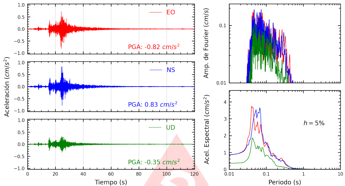
Figura A.17: Registros tiempo-historia, espectros de Fourier y de respuesta en las direcciones EO, NS y vertical de la estación BRIS2. Sismo de Provincia Constitucional del Callao , Callao - Lima del 2025-03-17, 02:35:03 (Hora local)
