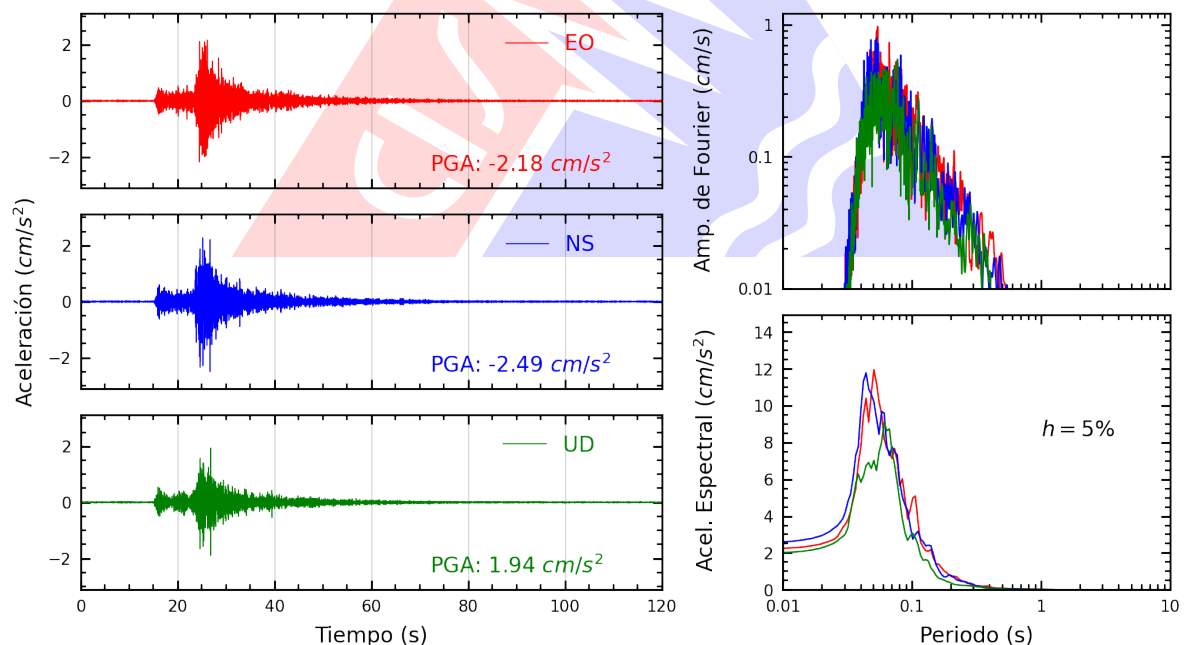
Figura A.2: Registros tiempo-historia, espectros de Fourier y de respuesta en las direcciones EO, NS y vertical de la estación UNTEL. Sismo de Provincia Constitucional del Callao , Callao - Lima del 2025-03-17, 02:35:03 (Hora local)
