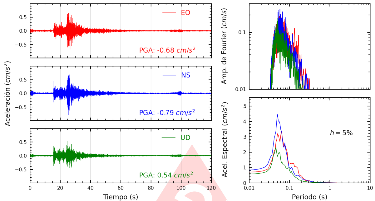
Figura A.19: Registros tiempo-historia, espectros de Fourier y de respuesta en las direcciones EO, NS y vertical de la estación PACHA. Sismo de Provincia Constitucional del Callao , Callao - Lima del 2025-03-17, 02:35:03 (Hora local)
