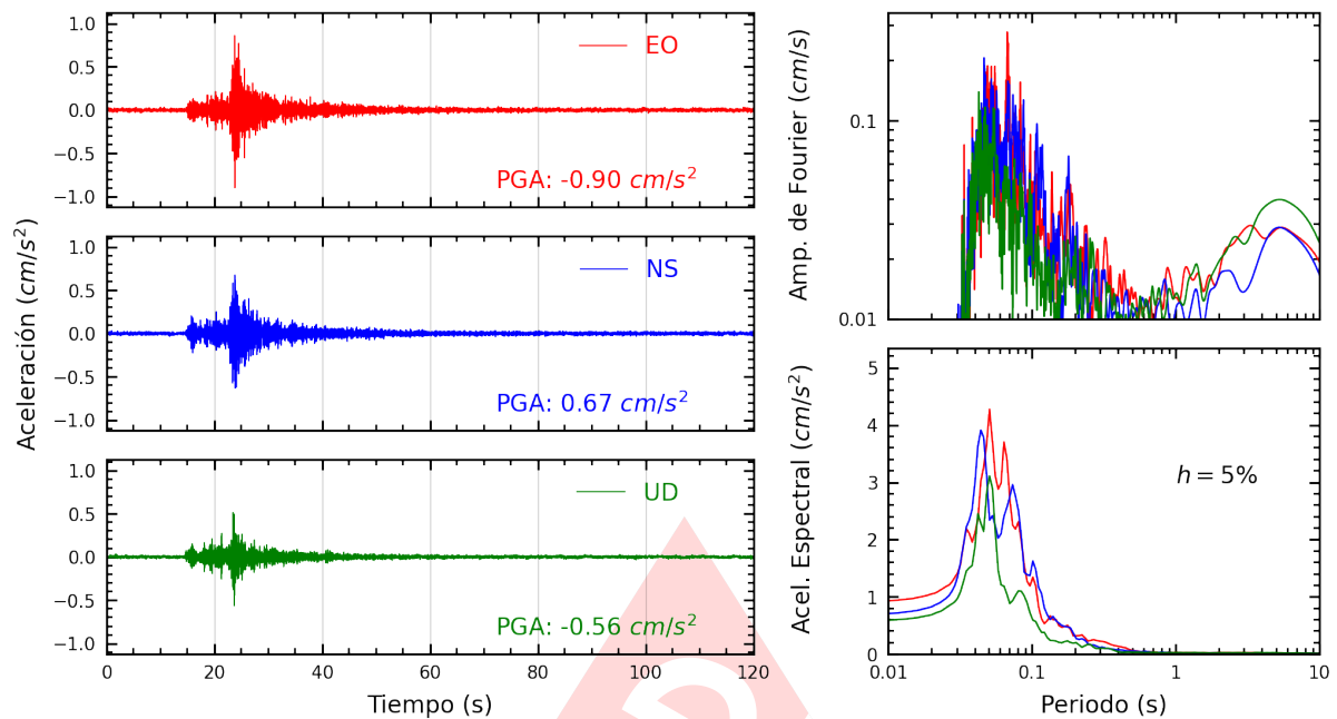
Figura A.15: Registros tiempo-historia, espectros de Fourier y de respuesta en las direcciones EO, NS y vertical de la estación UPCVI. Sismo de Provincia Constitucional del Callao , Callao - Lima del 2025-03-17, 02:35:03 (Hora local)
