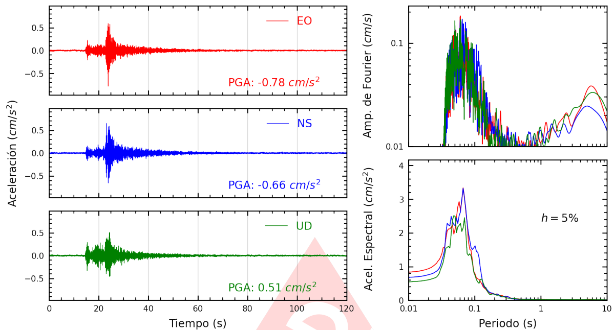
Figura A.21: Registros tiempo-historia, espectros de Fourier y de respuesta en las direcciones EO, NS y vertical de la estación SERVI. Sismo de Provincia Constitucional del Callao , Callao - Lima del 2025-03-17, 02:35:03 (Hora local)
