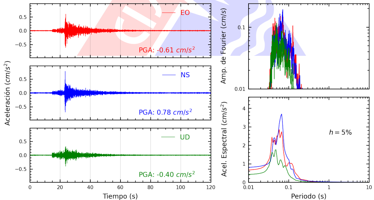
Figura A.20: Registros tiempo-historia, espectros de Fourier y de respuesta en las direcciones EO, NS y vertical de la estación ATARJ. Sismo de Provincia Constitucional del Callao , Callao - Lima del 2025-03-17, 02:35:03 (Hora local)
