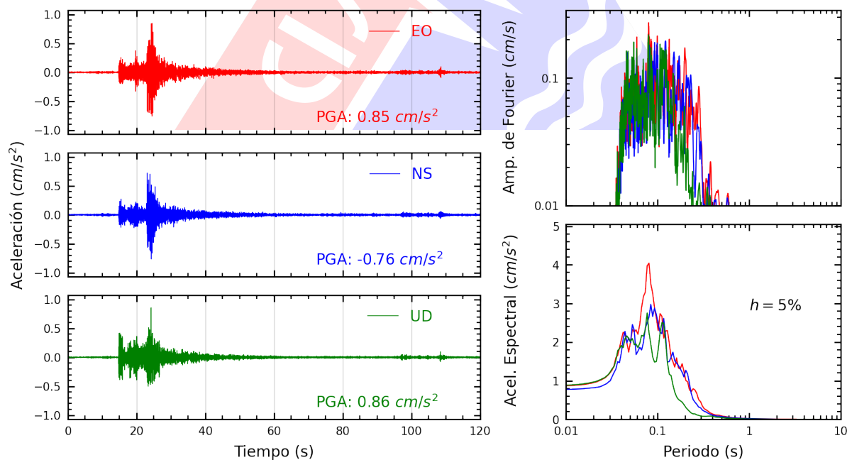
Figura A.16: Registros tiempo-historia, espectros de Fourier y de respuesta en las direcciones EO, NS y vertical de la estación SCCHO. Sismo de Provincia Constitucional del Callao , Callao - Lima del 2025-03-17, 02:35:03 (Hora local)
