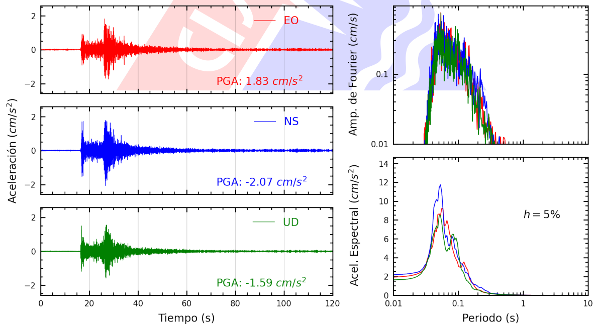
Figura A.4: Registros tiempo-historia, espectros de Fourier y de respuesta en las direcciones EO, NS y vertical de la estación PHER2. Sismo de Provincia Constitucional del Callao , Callao - Lima del 2025-03-17, 02:35:03 (Hora local)
