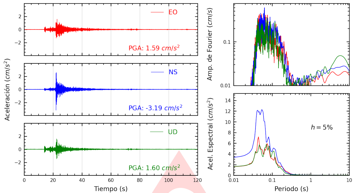
Figura A.1: Registros tiempo-historia, espectros de Fourier y de respuesta en las direcciones EO, NS y vertical de la estación INDEP. Sismo de Provincia Constitucional del Callao , Callao - Lima del 2025-03-17, 02:35:03 (Hora local)
