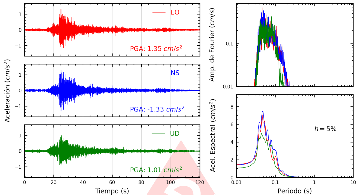
Figura A.9: Registros tiempo-historia, espectros de Fourier y de respuesta en las direcciones EO, NS y vertical de la estación SROS2. Sismo de Provincia Constitucional del Callao , Callao - Lima del 2025-03-17, 02:35:03 (Hora local)
