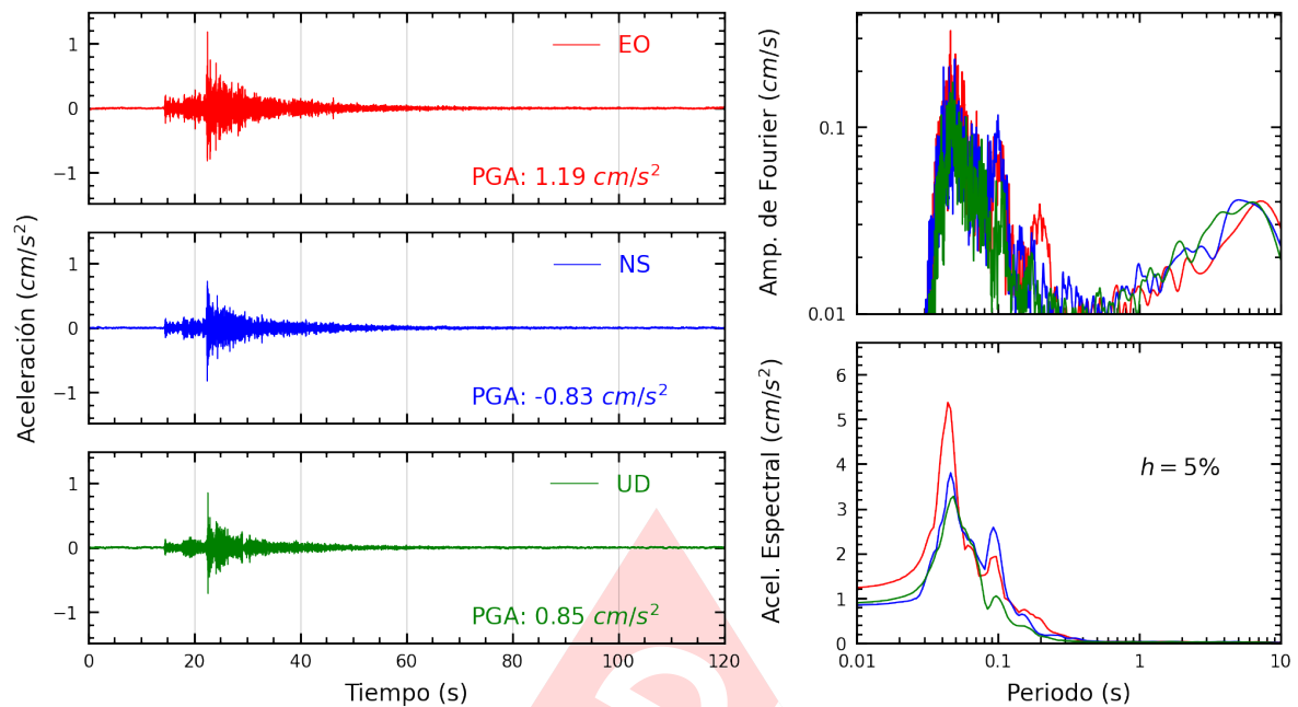
Figura A.13: Registros tiempo-historia, espectros de Fourier y de respuesta en las direcciones EO, NS y vertical de la estación UCSS. Sismo de Provincia Constitucional del Callao , Callao - Lima del 2025-03-17, 02:35:03 (Hora local)
