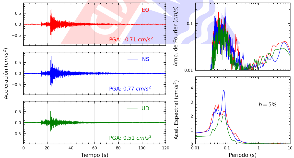
Figura A.22: Registros tiempo-historia, espectros de Fourier y de respuesta en las direcciones EO, NS y vertical de la estación COMAS. Sismo de Provincia Constitucional del Callao , Callao - Lima del 2025-03-17, 02:35:03 (Hora local)
