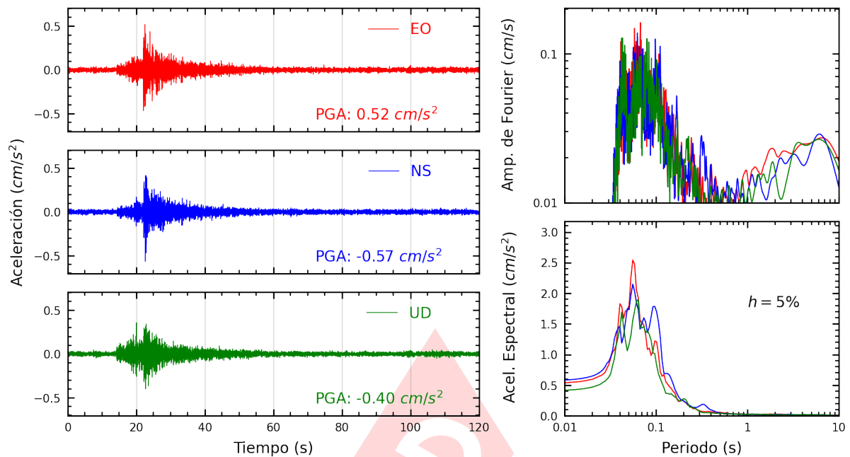
Figura A.27: Registros tiempo-historia, espectros de Fourier y de respuesta en las direcciones EO, NS y vertical de la estación MADRE. Sismo de Provincia Constitucional del Callao , Callao - Lima del 2025-03-17, 02:35:03 (Hora local)
