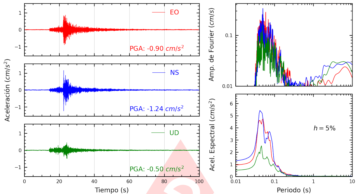
Figura A.11: Registros tiempo-historia, espectros de Fourier y de respuesta en las direcciones EO, NS y vertical de la estación CEPRE. Sismo de Provincia Constitucional del Callao , Callao - Lima del 2025-03-17, 02:35:03 (Hora local)
