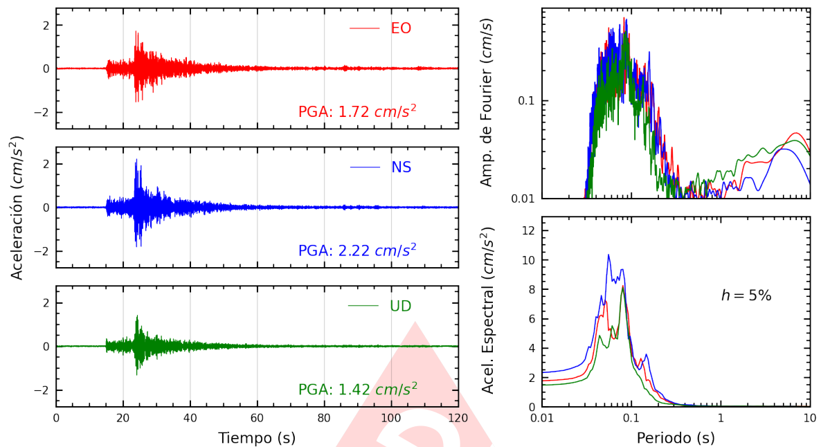
Figura A.3: Registros tiempo-historia, espectros de Fourier y de respuesta en las direcciones EO, NS y vertical de la estación USILM. Sismo de Provincia Constitucional del Callao , Callao - Lima del 2025-03-17, 02:35:03 (Hora local)
