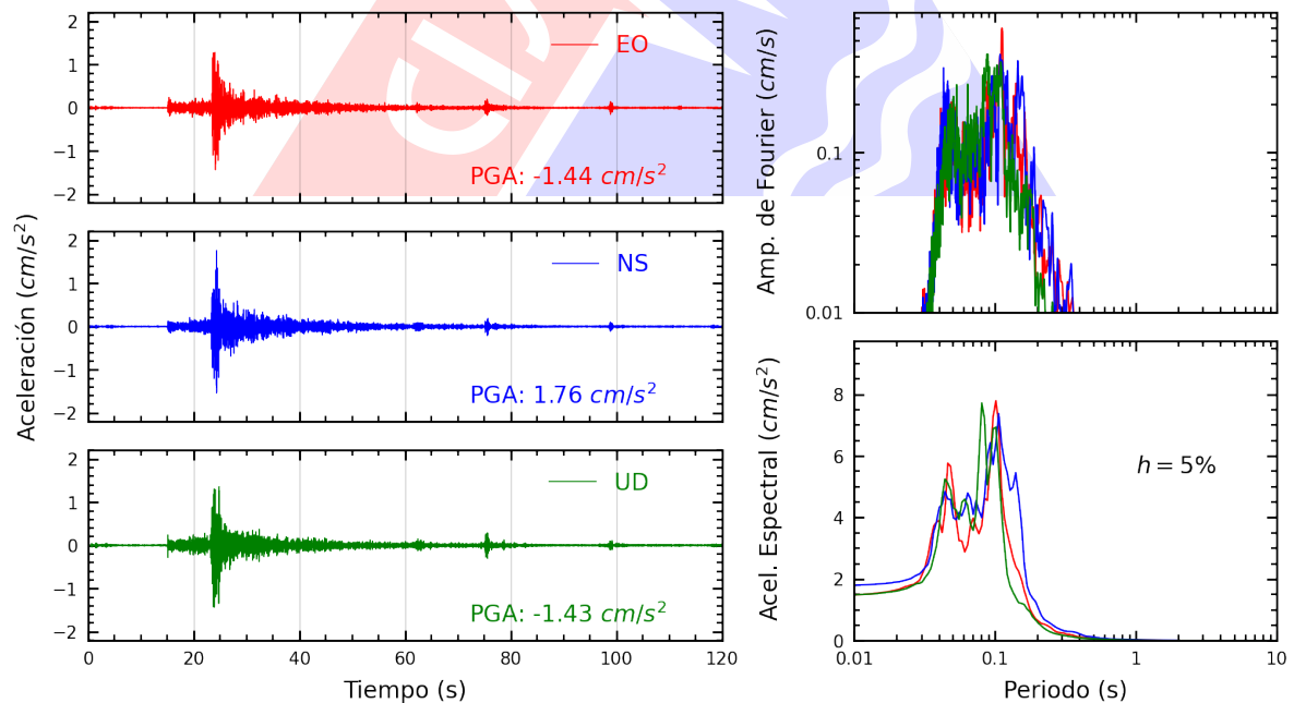
Figura A.6: Registros tiempo-historia, espectros de Fourier y de respuesta en las direcciones EO, NS y vertical de la estación CARA2. Sismo de Provincia Constitucional del Callao , Callao - Lima del 2025-03-17, 02:35:03 (Hora local)
