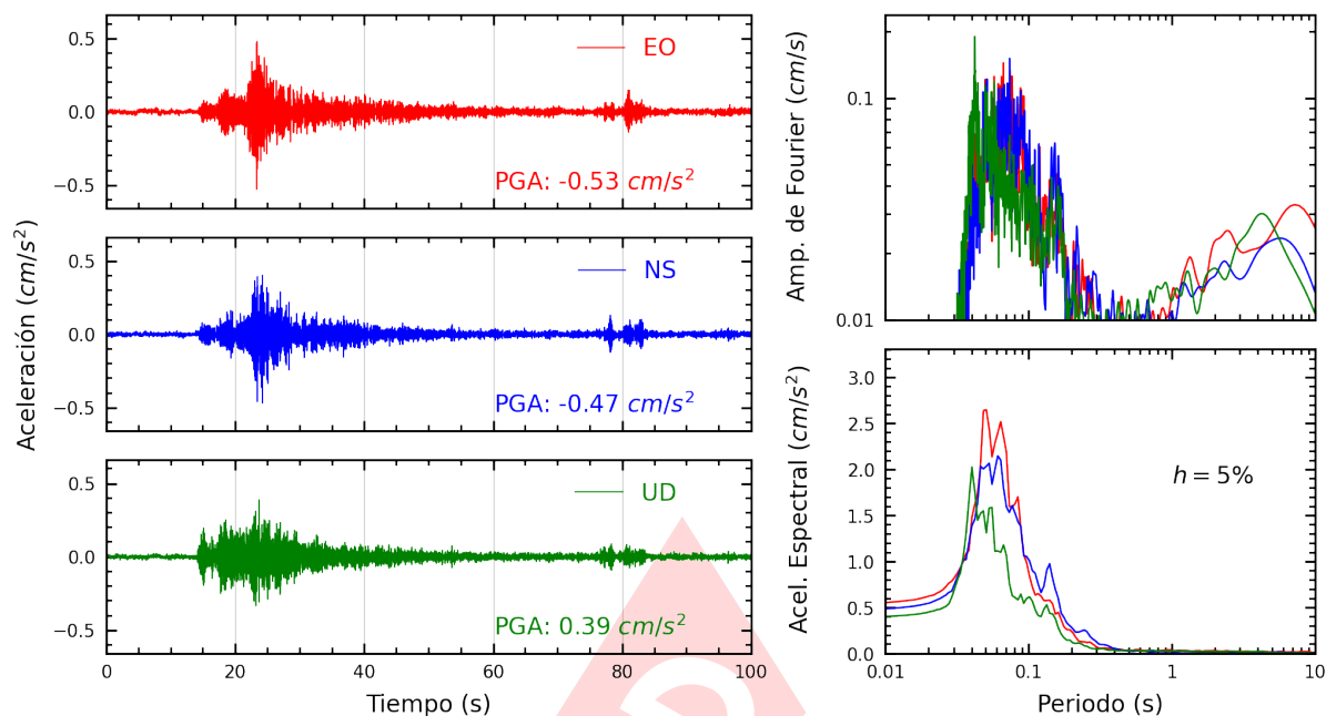
Figura A.31: Registros tiempo-historia, espectros de Fourier y de respuesta en las direcciones EO, NS y vertical de la estación UPCSM. Sismo de Provincia Constitucional del Callao , Callao - Lima del 2025-03-17, 02:35:03 (Hora local)
