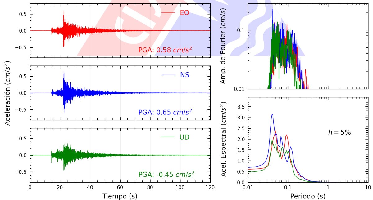
Figura A.26: Registros tiempo-historia, espectros de Fourier y de respuesta en las direcciones EO, NS y vertical de la estación JALV2. Sismo de Provincia Constitucional del Callao , Callao - Lima del 2025-03-17, 02:35:03 (Hora local)
