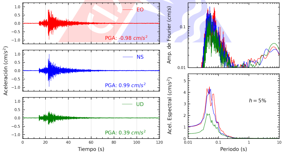
Figura A.14: Registros tiempo-historia, espectros de Fourier y de respuesta en las direcciones EO, NS y vertical de la estación FICPE. Sismo de Provincia Constitucional del Callao , Callao - Lima del 2025-03-17, 02:35:03 (Hora local)
