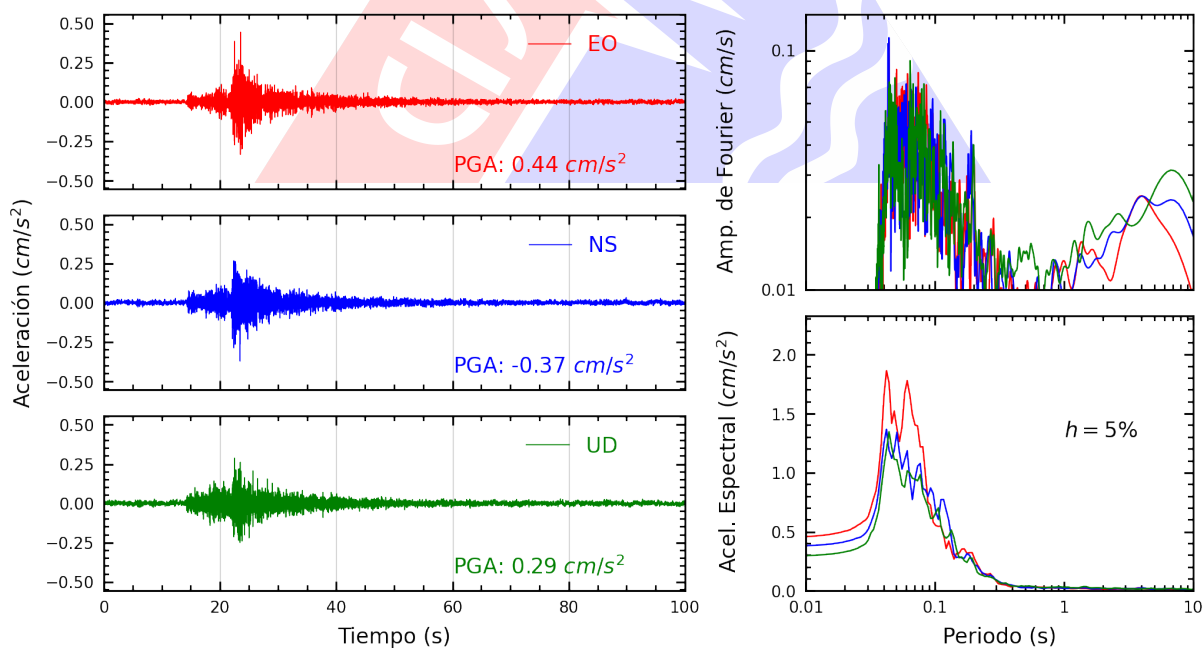
Figura A.32: Registros tiempo-historia, espectros de Fourier y de respuesta en las direcciones EO, NS y vertical de la estación UNFV. Sismo de Provincia Constitucional del Callao , Callao - Lima del 2025-03-17, 02:35:03 (Hora local)
