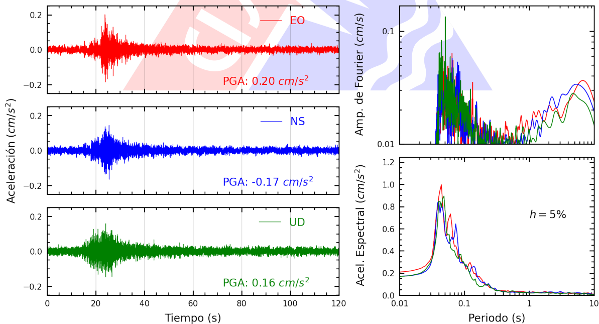
Figura A.36: Registros tiempo-historia, espectros de Fourier y de respuesta en las direcciones EO, NS y vertical de la estación BONDY. Sismo de Provincia Constitucional del Callao , Callao - Lima del 2025-03-17, 02:35:03 (Hora local)
