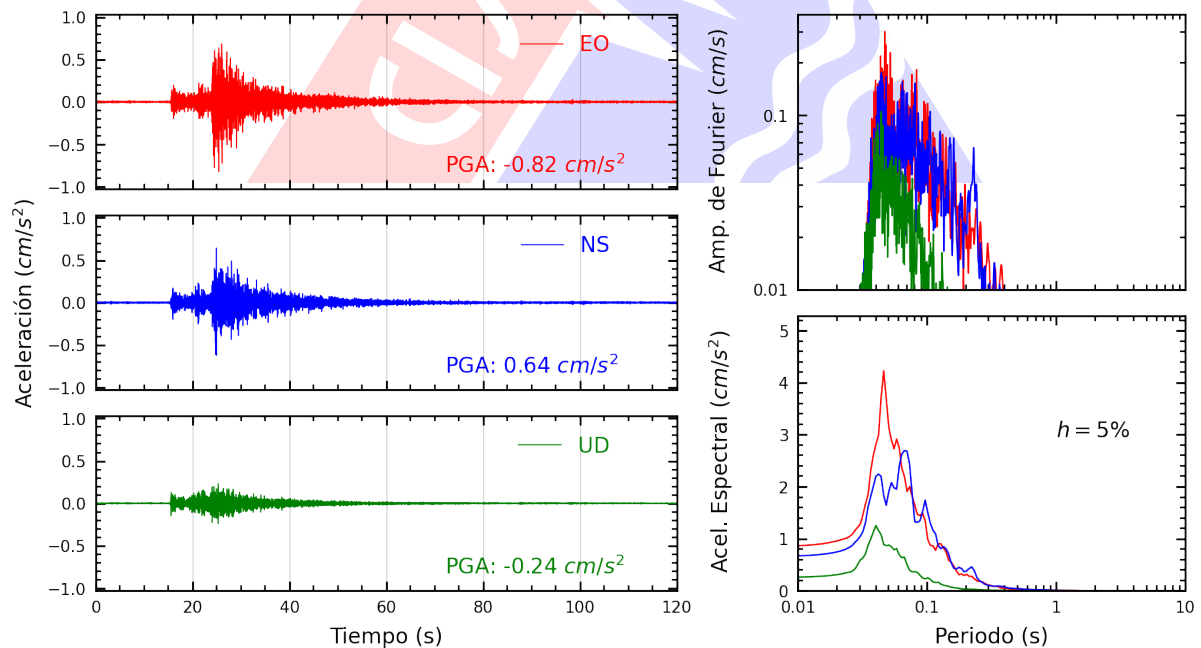
Figura A.18: Registros tiempo-historia, espectros de Fourier y de respuesta en las direcciones EO, NS y vertical de la estación UCVA2. Sismo de Provincia Constitucional del Callao , Callao - Lima del 2025-03-17, 02:35:03 (Hora local)
