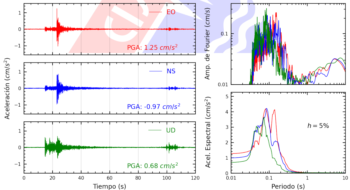
Figura A.10: Registros tiempo-historia, espectros de Fourier y de respuesta en las direcciones EO, NS y vertical de la estación SOCHO. Sismo de Provincia Constitucional del Callao , Callao - Lima del 2025-03-17, 02:35:03 (Hora local)
