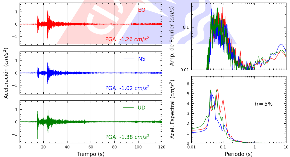
Figura A.8: Registros tiempo-historia, espectros de Fourier y de respuesta en las direcciones EO, NS y vertical de la estación URPE. Sismo de Provincia Constitucional del Callao , Callao - Lima del 2025-03-17, 02:35:03 (Hora local)
