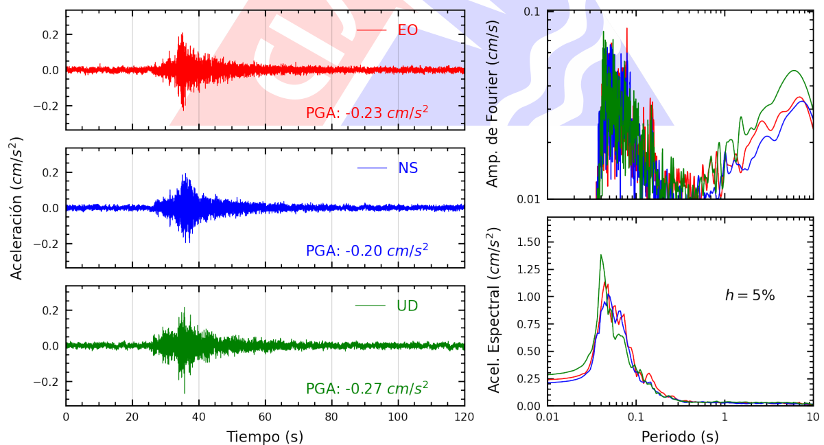
Figura A.34: Registros tiempo-historia, espectros de Fourier y de respuesta en las direcciones EO, NS y vertical de la estación UNMSM. Sismo de Provincia Constitucional del Callao , Callao - Lima del 2025-03-17, 02:35:03 (Hora local)
