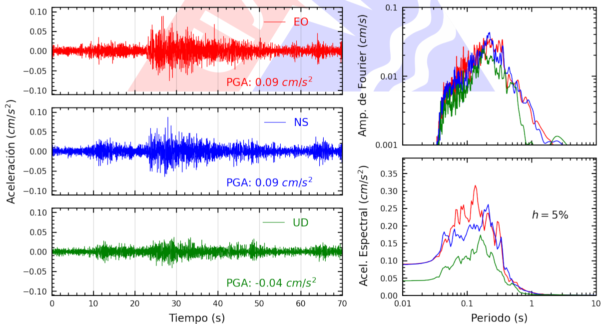
Figura A.18: Registros tiempo-historia, espectros de Fourier y de respuesta en las direcciones EO, NS y vertical de la estación BRISA. Sismo de Curimana, Padre Abad - Ucayali del 2025-03-18, 03:18:55 (Hora local)
