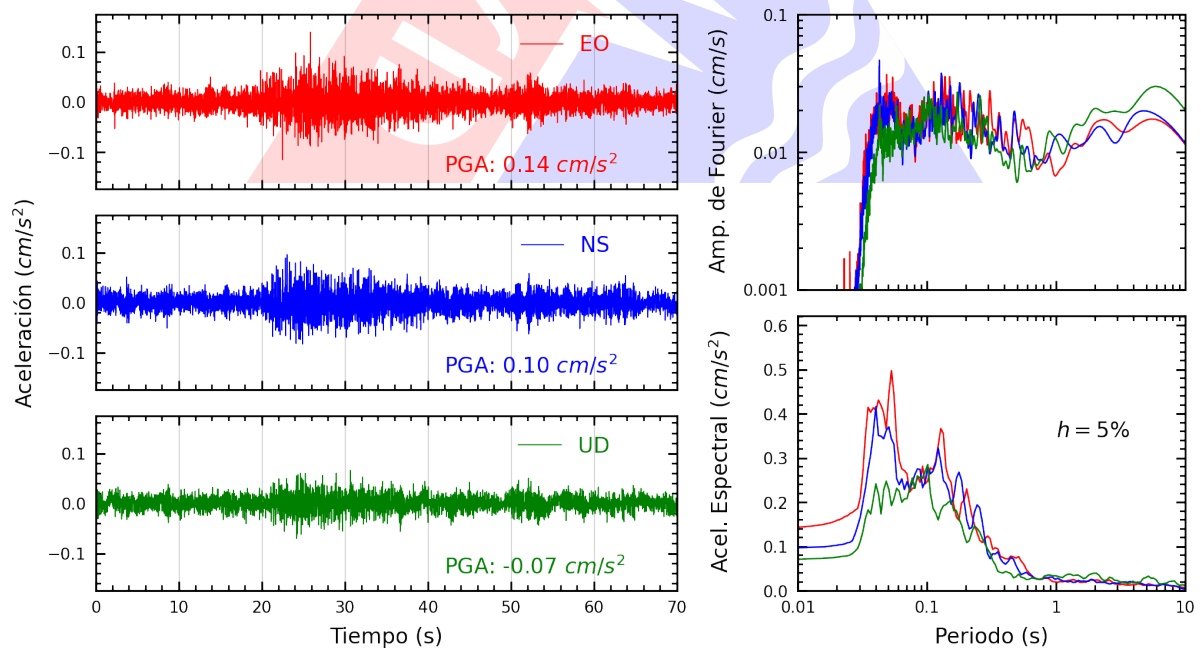
Figura A.10: Registros tiempo-historia, espectros de Fourier y de respuesta en las direcciones EO, NS y vertical de la estación OLIVO. Sismo de Curimana, Padre Abad - Ucayali del 2025-03-18, 03:18:55 (Hora local)
