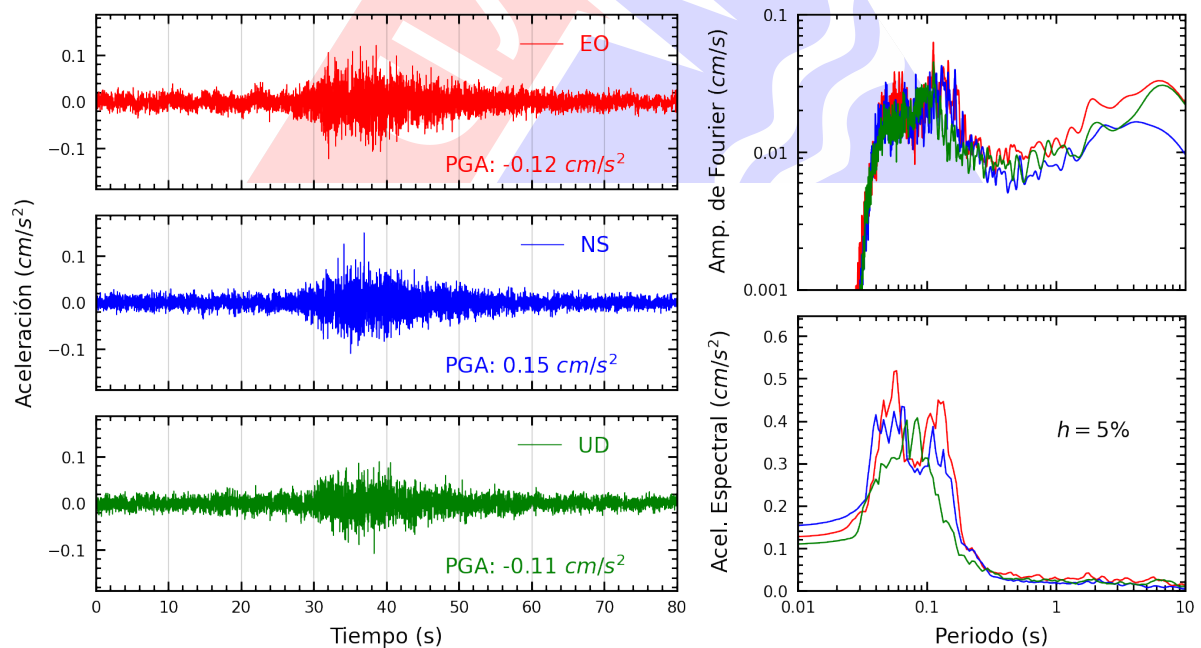
Figura A.8: Registros tiempo-historia, espectros de Fourier y de respuesta en las direcciones EO, NS y vertical de la estación AMORE. Sismo de Curimana, Padre Abad - Ucayali del 2025-03-18, 03:18:55 (Hora local)
