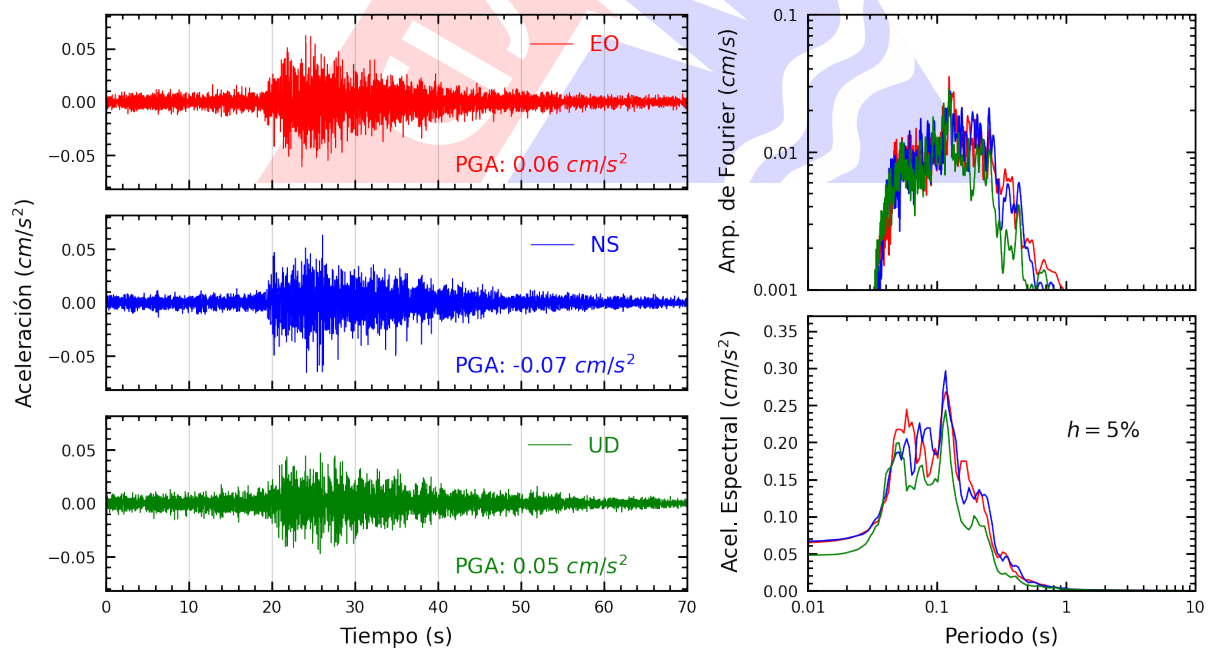
Figura A.20: Registros tiempo-historia, espectros de Fourier y de respuesta en las direcciones EO, NS y vertical de la estación JALV2. Sismo de Curimana, Padre Abad - Ucayali del 2025-03-18, 03:18:55 (Hora local)
