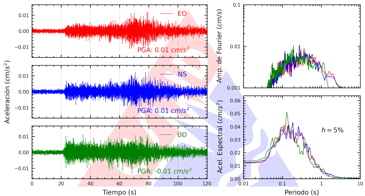
Figura A.21: Registros tiempo-historia, espectros de Fourier y de respuesta en las direcciones EO, NS y vertical de la estación UNCP. Sismo de Curimana, Padre Abad - Ucayali del 2025-03-18, 03:18:55 (Hora local)
