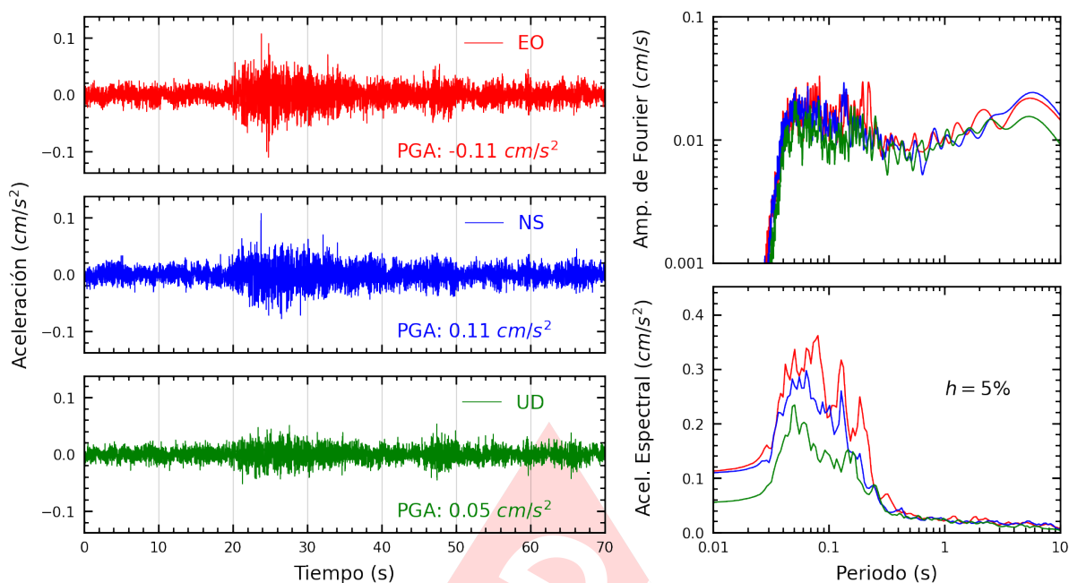
Figura A.13: Registros tiempo-historia, espectros de Fourier y de respuesta en las direcciones EO, NS y vertical de la estación FICPE. Sismo de Curimana, Padre Abad - Ucayali del 2025-03-18, 03:18:55 (Hora local)
