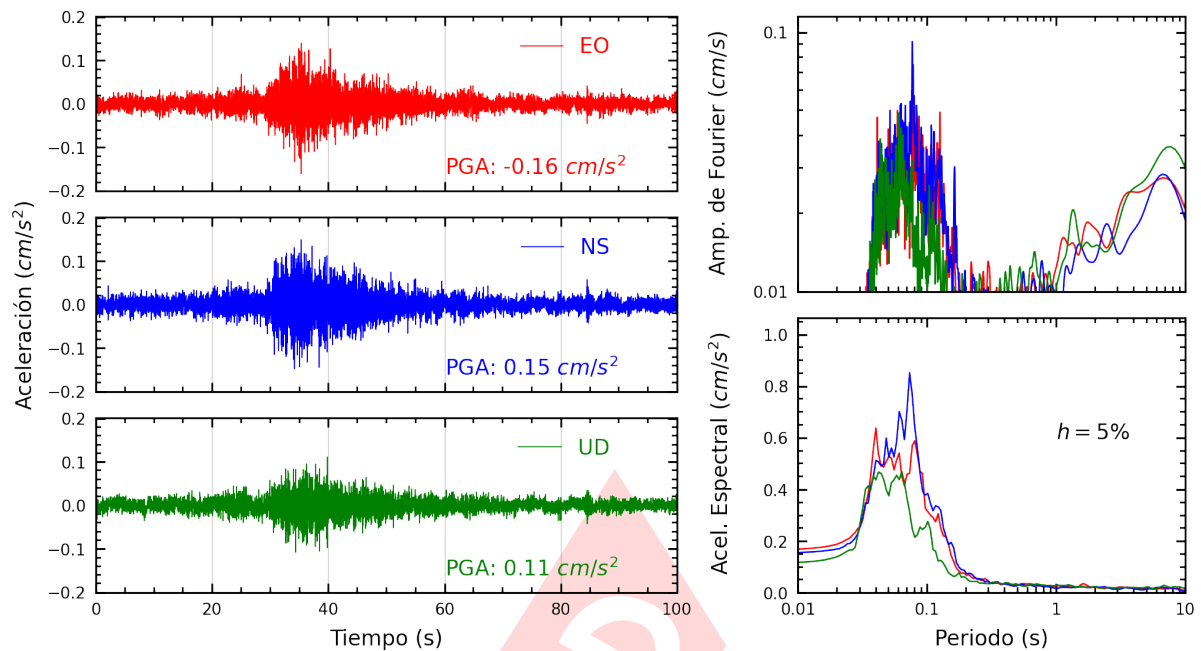
Figura A.7: Registros tiempo-historia, espectros de Fourier y de respuesta en las direcciones EO, NS y vertical de la estación JOSEO. Sismo de Curimana, Padre Abad - Ucayali del 2025-03-18, 03:18:55 (Hora local)
