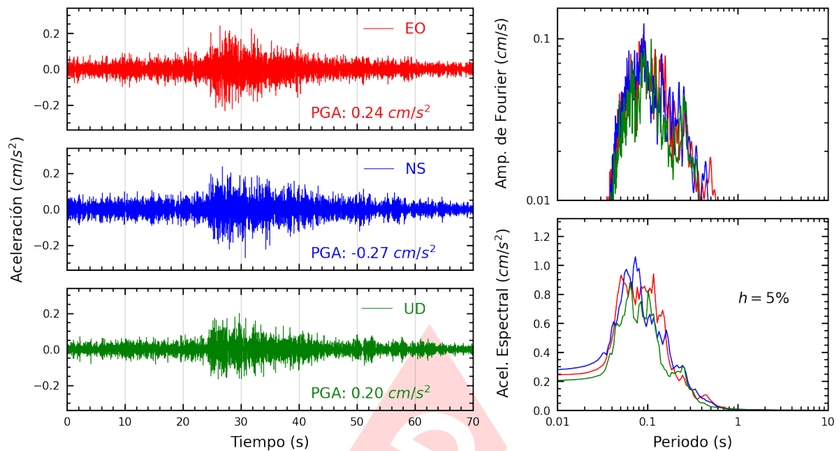
Figura A.5: Registros tiempo-historia, espectros de Fourier y de respuesta en las direcciones EO, NS y vertical de la estación PHER2. Sismo de Curimana, Padre Abad - Ucayali del 2025-03-18, 03:18:55 (Hora local)
