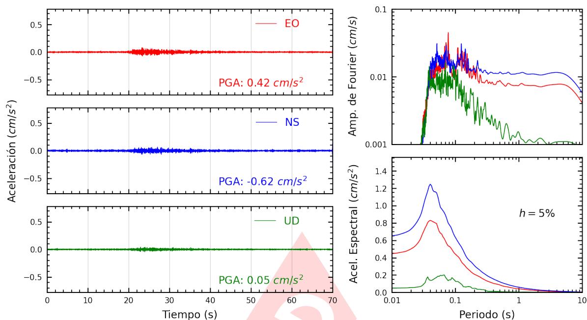
Figura A.3: Registros tiempo-historia, espectros de Fourier y de respuesta en las direcciones EO, NS y vertical de la estación ATARJ. Sismo de Curimana, Padre Abad - Ucayali del 2025-03-18, 03:18:55 (Hora local)
