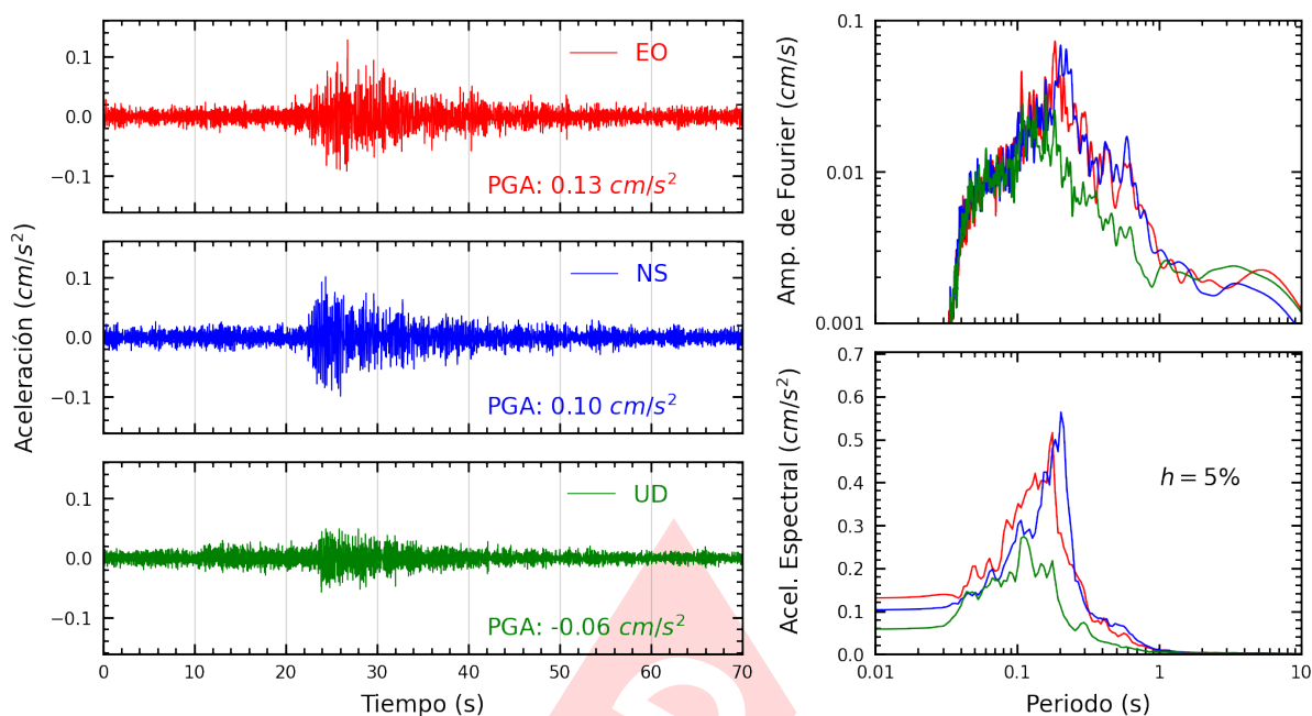
Figura A.11: Registros tiempo-historia, espectros de Fourier y de respuesta en las direcciones EO, NS y vertical de la estación SCCHO. Sismo de Curimana, Padre Abad - Ucayali del 2025-03-18, 03:18:55 (Hora local)
