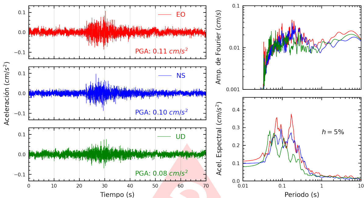
Figura A.15: Registros tiempo-historia, espectros de Fourier y de respuesta en las direcciones EO, NS y vertical de la estación USILP. Sismo de Curimana, Padre Abad - Ucayali del 2025-03-18, 03:18:55 (Hora local)
