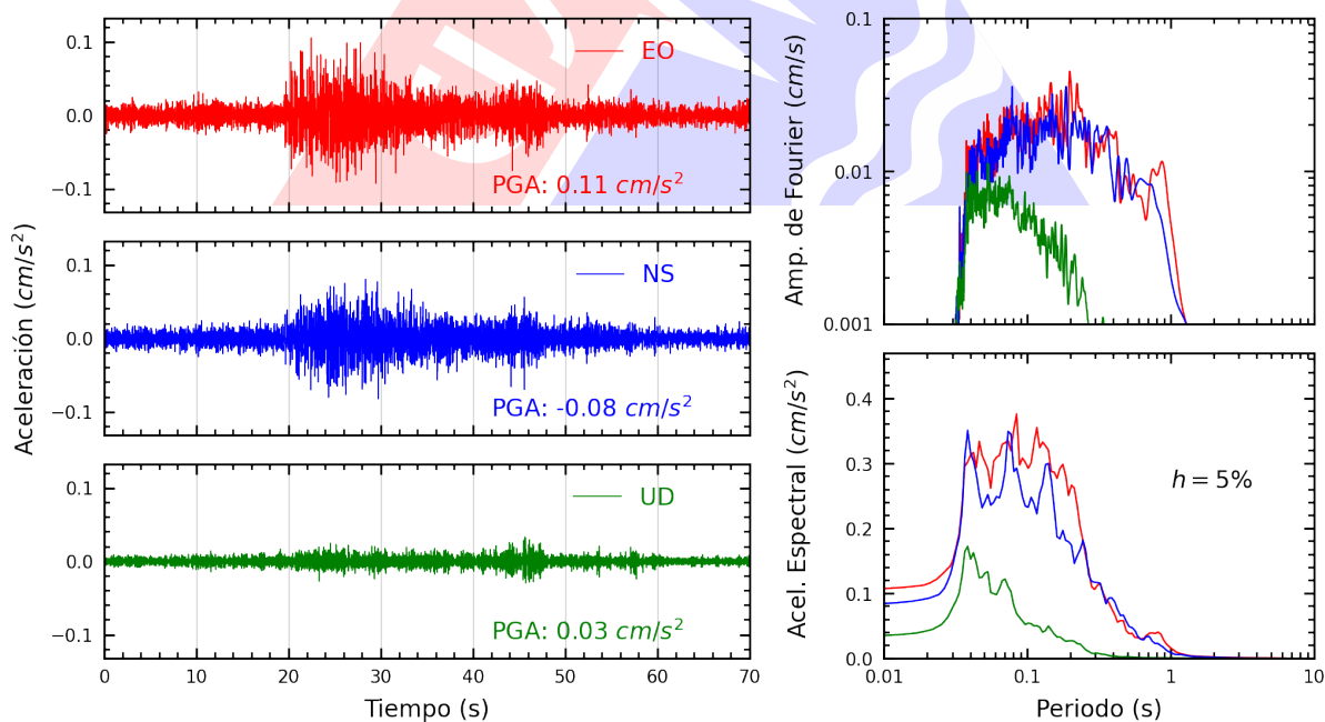
Figura A.16: Registros tiempo-historia, espectros de Fourier y de respuesta en las direcciones EO, NS y vertical de la estación UCVA2. Sismo de Curimana, Padre Abad - Ucayali del 2025-03-18, 03:18:55 (Hora local)
