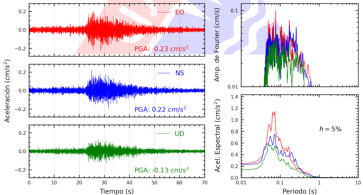
Figura A.6: Registros tiempo-historia, espectros de Fourier y de respuesta en las direcciones EO, NS y vertical de la estación UNTEL. Sismo de Curimana, Padre Abad - Ucayali del 2025-03-18, 03:18:55 (Hora local)
