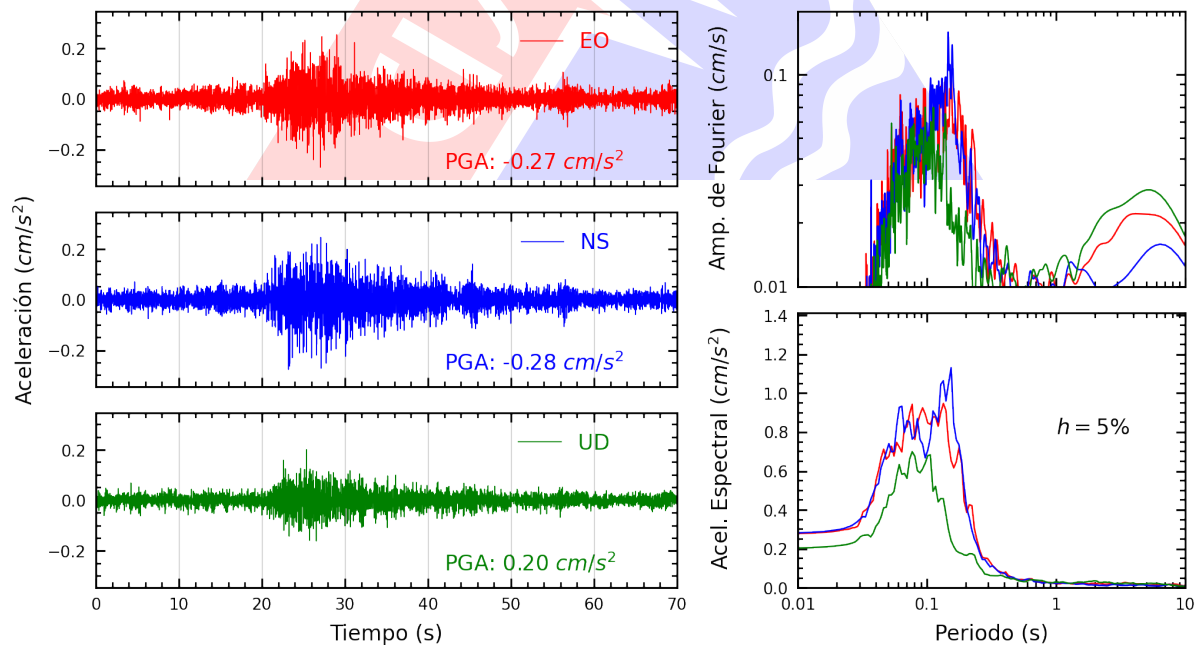
Figura A.4: Registros tiempo-historia, espectros de Fourier y de respuesta en las direcciones EO, NS y vertical de la estación USILM. Sismo de Curimana, Padre Abad - Ucayali del 2025-03-18, 03:18:55 (Hora local)
