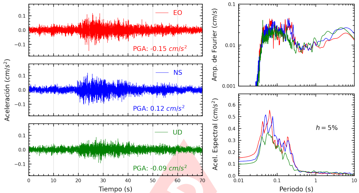
Figura A.9: Registros tiempo-historia, espectros de Fourier y de respuesta en las direcciones EO, NS y vertical de la estación INDEP. Sismo de Curimana, Padre Abad - Ucayali del 2025-03-18, 03:18:55 (Hora local)
