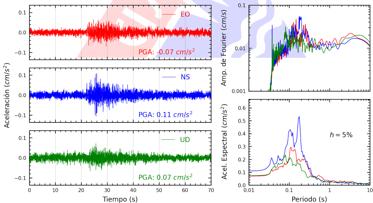
Figura A.14: Registros tiempo-historia, espectros de Fourier y de respuesta en las direcciones EO, NS y vertical de la estación SOCHO. Sismo de Curimana, Padre Abad - Ucayali del 2025-03-18, 03:18:55 (Hora local)
