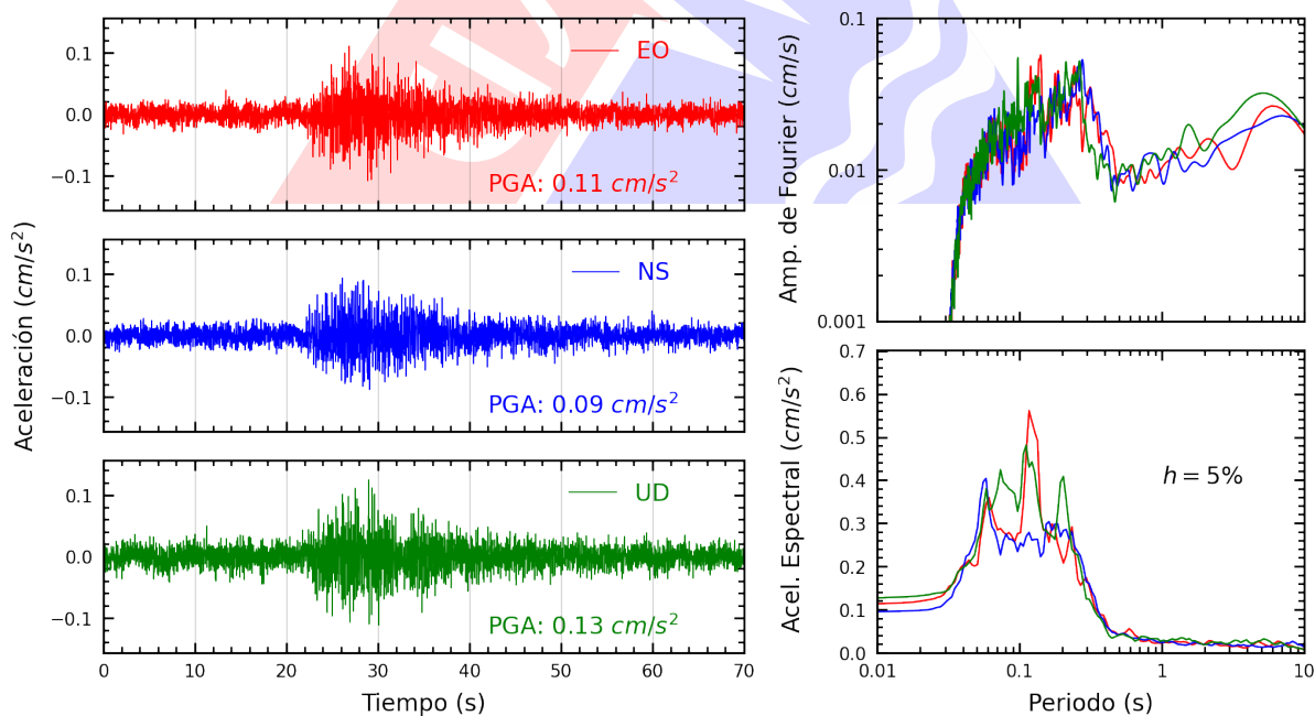
Figura A.12: Registros tiempo-historia, espectros de Fourier y de respuesta en las direcciones EO, NS y vertical de la estación SOVES. Sismo de Curimana, Padre Abad - Ucayali del 2025-03-18, 03:18:55 (Hora local)
