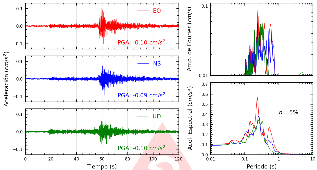
Figura A.17: Registros tiempo-historia, espectros de Fourier y de respuesta en las direcciones EO, NS y vertical de la estación CARAL. Sismo de Curimana, Padre Abad - Ucayali del 2025-03-18, 03:18:55 (Hora local)
