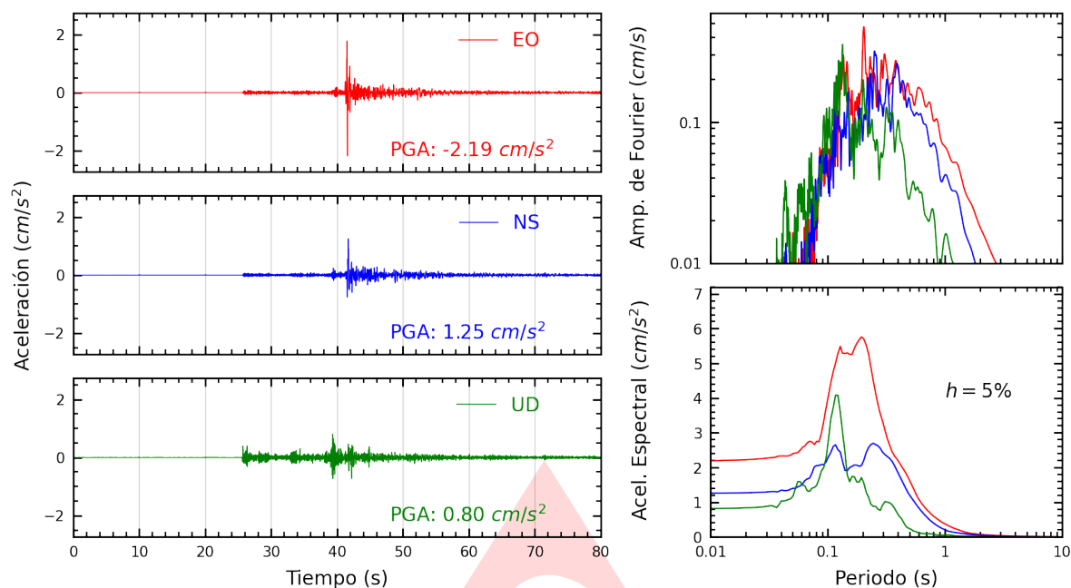
Figura A.1: Registros tiempo-historia, espectros de Fourier y de respuesta en las direcciones EO, NS y vertical de la estación UNIA. Sismo de Curimana, Padre Abad - Ucayali del 2025-03-18, 03:18:55 (Hora local)
