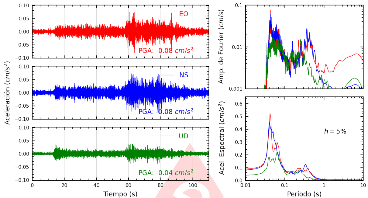
Figura A.19: Registros tiempo-historia, espectros de Fourier y de respuesta en las direcciones EO, NS y vertical de la estación SCTRU. Sismo de Curimana, Padre Abad - Ucayali del 2025-03-18, 03:18:55 (Hora local)
