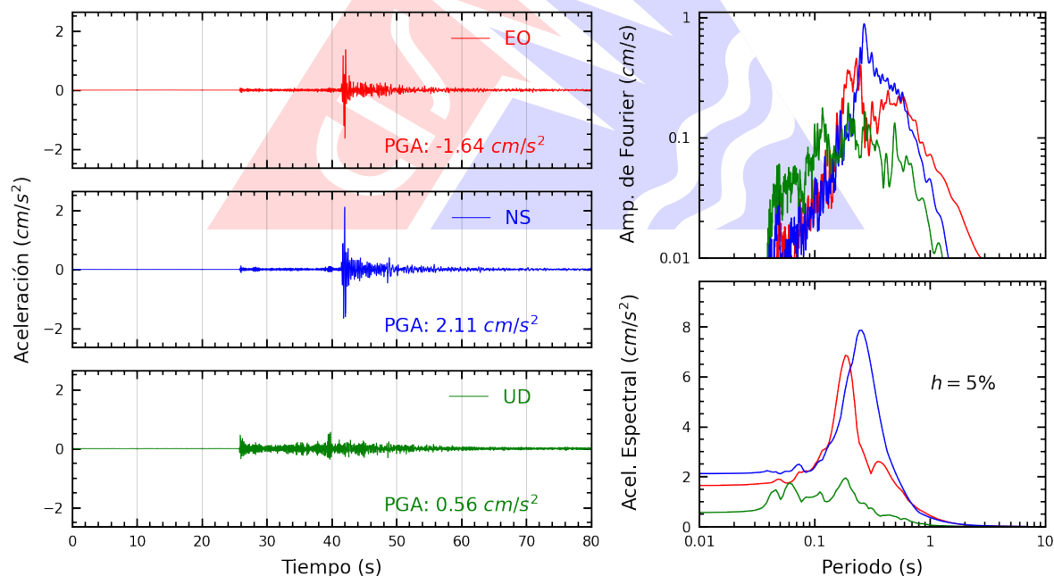
Figura A.2: Registros tiempo-historia, espectros de Fourier y de respuesta en las direcciones EO, NS y vertical de la estación SCPUC. Sismo de Curimana, Padre Abad - Ucayali del 2025-03-18, 03:18:55 (Hora local)
