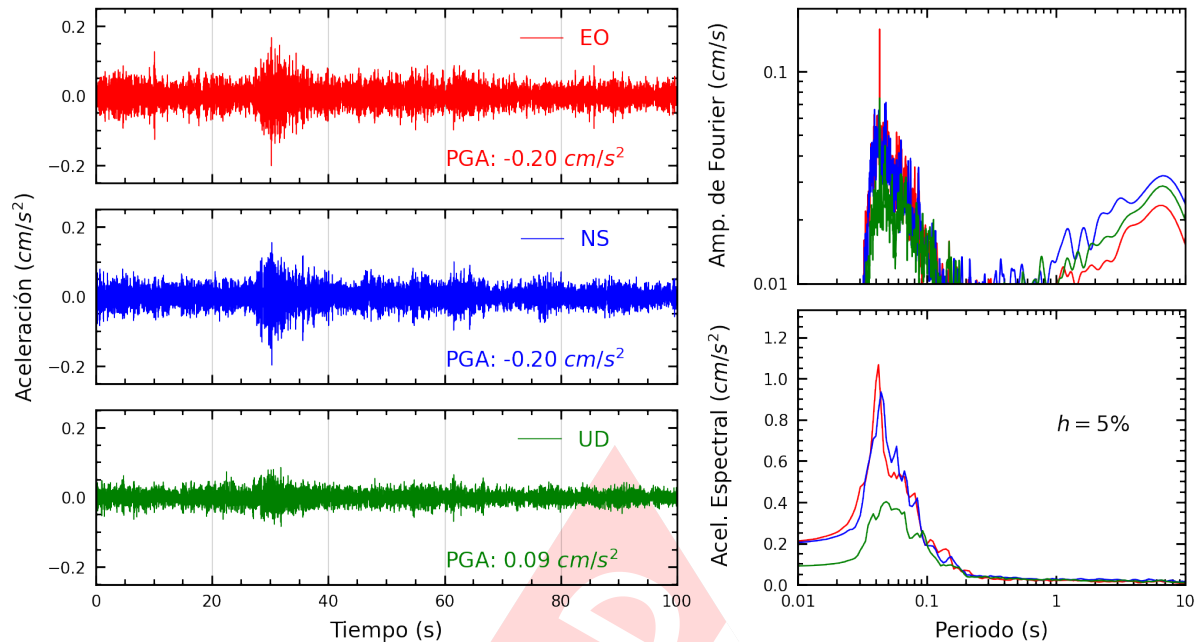
Figura A.9: Registros tiempo-historia, espectros de Fourier y de respuesta en las direcciones EO, NS y vertical de la estación CEPRE. Sismo de Ancon, Lima - Lima del 2025-03-20, 09:04:23 (Hora local)
