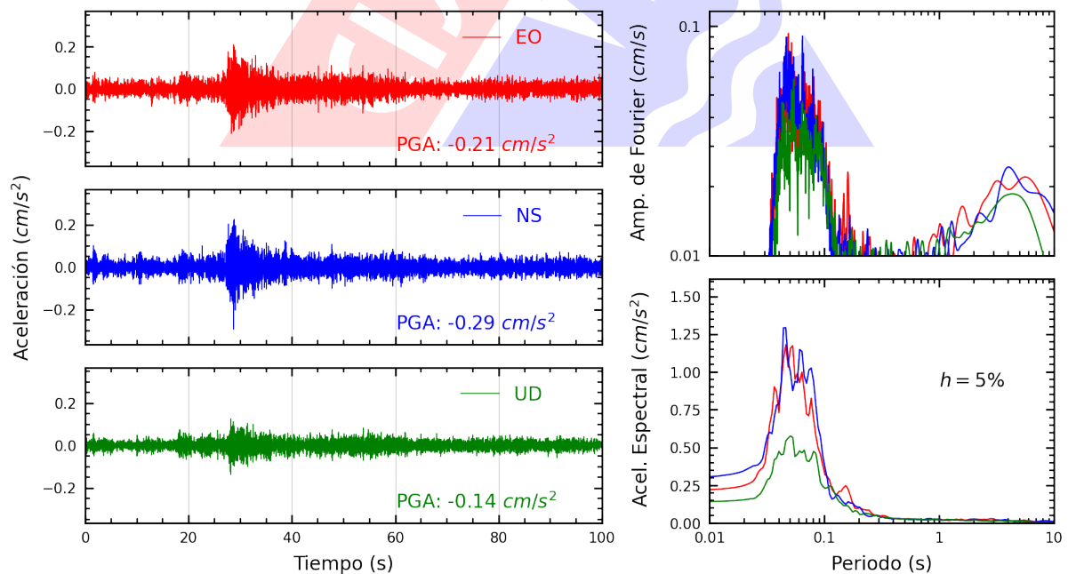
Figura A.6: Registros tiempo-historia, espectros de Fourier y de respuesta en las direcciones EO, NS y vertical de la estación FICPE. Sismo de Ancon, Lima - Lima del 2025-03-20, 09:04:23 (Hora local)
