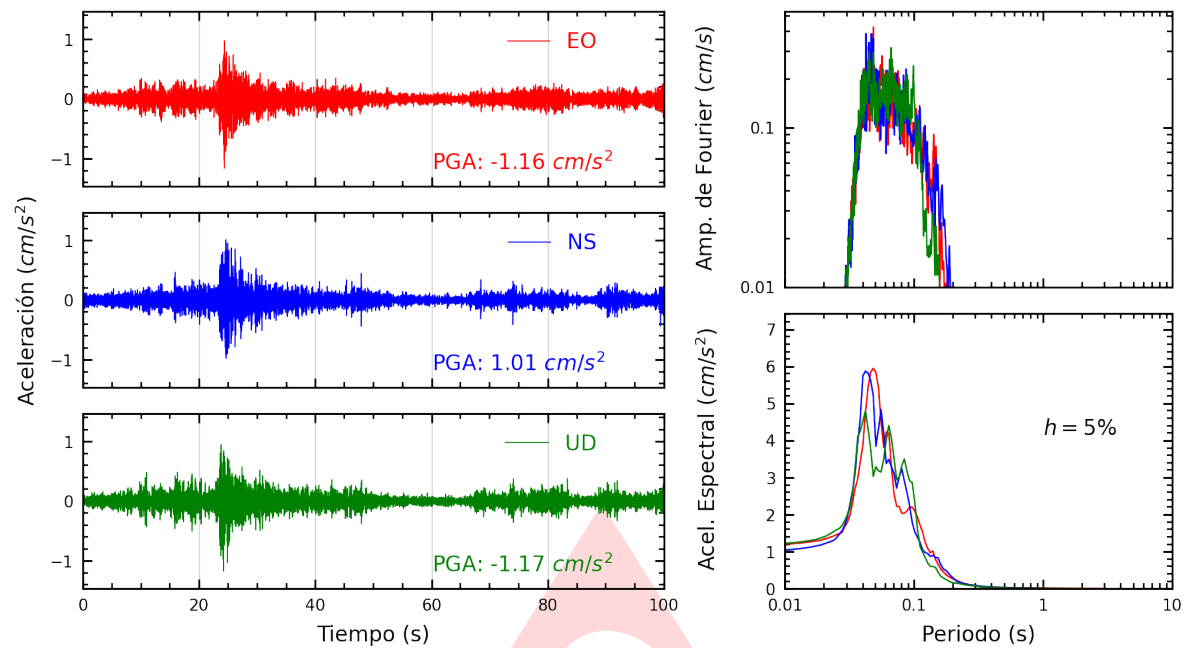
Figura A.1: Registros tiempo-historia, espectros de Fourier y de respuesta en las direcciones EO, NS y vertical de la estación SROS2. Sismo de Ancon, Lima - Lima del 2025-03-20, 09:04:23 (Hora local)
