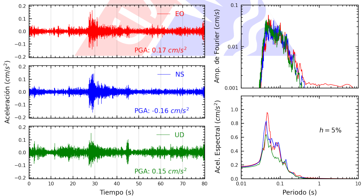
Figura A.12: Registros tiempo-historia, espectros de Fourier y de respuesta en las direcciones EO, NS y vertical de la estación JALV2. Sismo de Ancon, Lima - Lima del 2025-03-20, 09:04:23 (Hora local)
