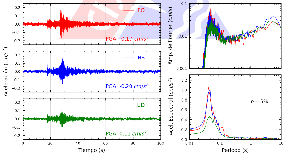
Figura A.10: Registros tiempo-historia, espectros de Fourier y de respuesta en las direcciones EO, NS y vertical de la estación UCSS. Sismo de Ancon, Lima - Lima del 2025-03-20, 09:04:23 (Hora local)
