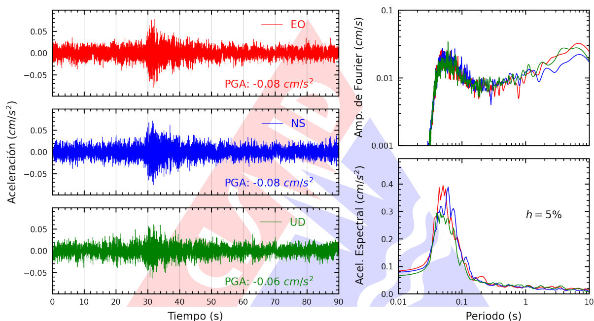
Figura A.17: Registros tiempo-historia, espectros de Fourier y de respuesta en las direcciones EO, NS y vertical de la estación SERVI. Sismo de Ancon, Lima - Lima del 2025-03-20, 09:04:23 (Hora local)
