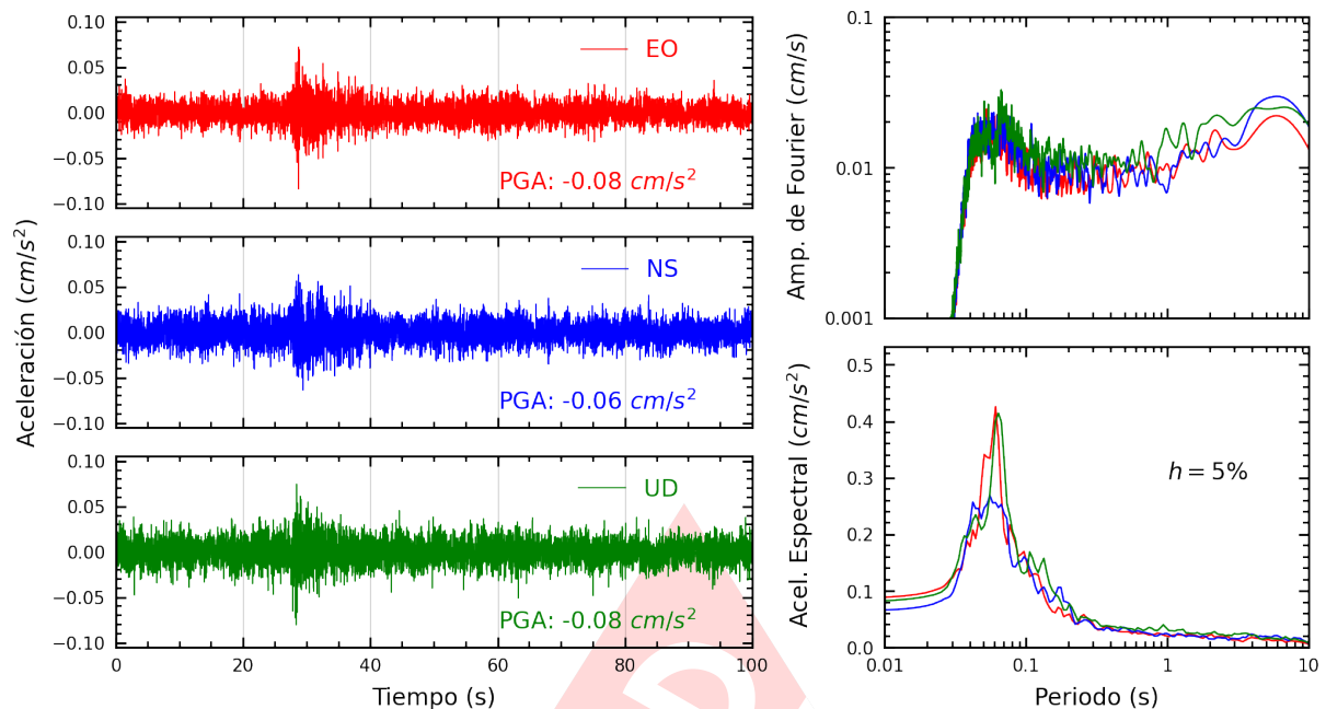
Figura A.15: Registros tiempo-historia, espectros de Fourier y de respuesta en las direcciones EO, NS y vertical de la estación UNFV. Sismo de Ancon, Lima - Lima del 2025-03-20, 09:04:23 (Hora local)
