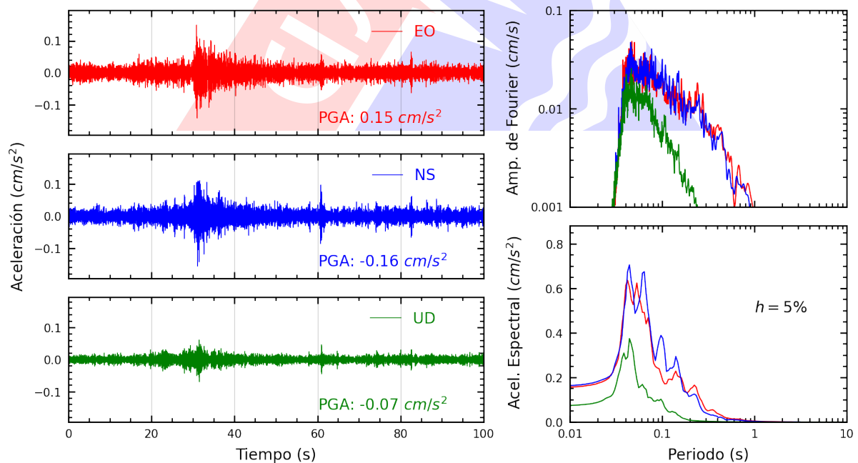
Figura A.14: Registros tiempo-historia, espectros de Fourier y de respuesta en las direcciones EO, NS y vertical de la estación UCVA2. Sismo de Ancon, Lima - Lima del 2025-03-20, 09:04:23 (Hora local)
