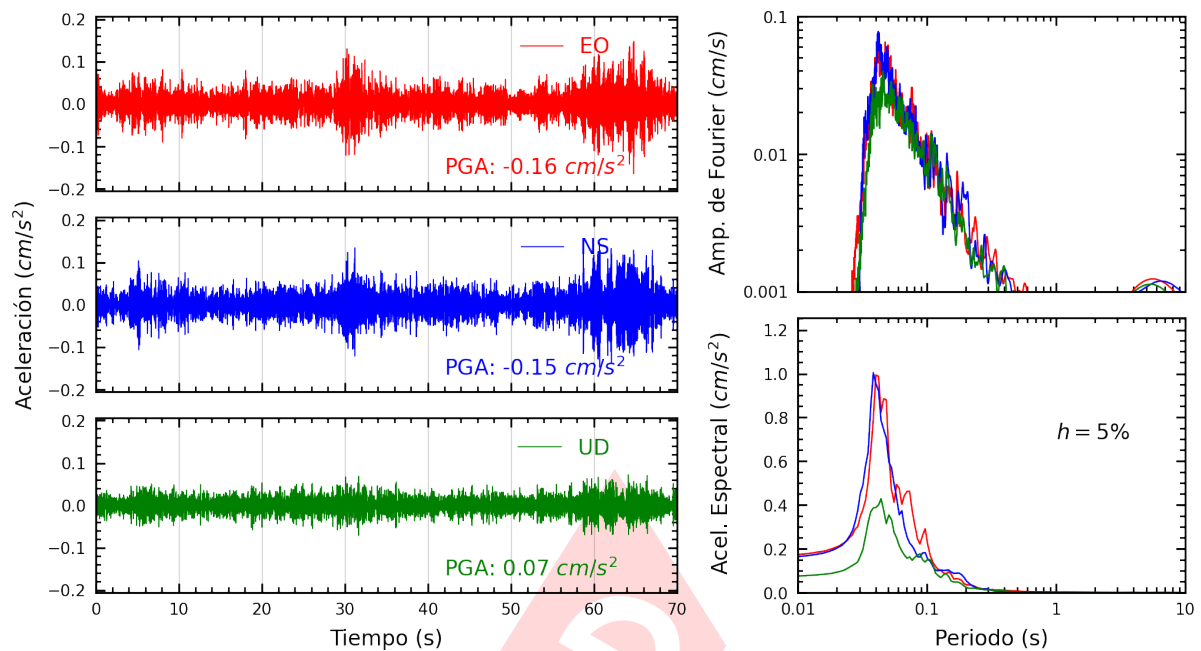
Figura A.13: Registros tiempo-historia, espectros de Fourier y de respuesta en las direcciones EO, NS y vertical de la estación BORJA. Sismo de Ancon, Lima - Lima del 2025-03-20, 09:04:23 (Hora local)
