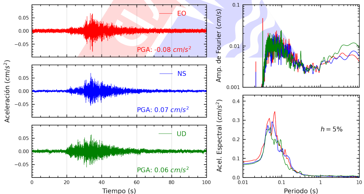
Figura A.16: Registros tiempo-historia, espectros de Fourier y de respuesta en las direcciones EO, NS y vertical de la estación CARAL. Sismo de Ancon, Lima - Lima del 2025-03-20, 09:04:23 (Hora local)
