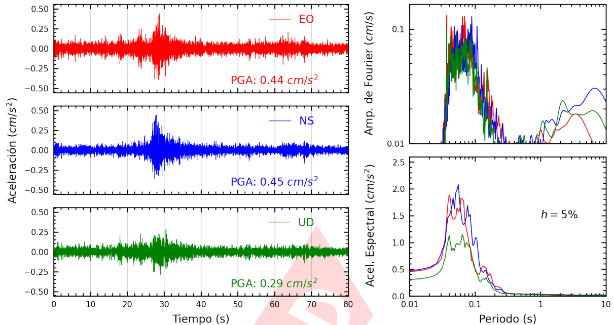
Figura A.5: Registros tiempo-historia, espectros de Fourier y de respuesta en las direcciones EO, NS y vertical de la estación INDEP. Sismo de Ancon, Lima - Lima del 2025-03-20, 09:04:23 (Hora local)
