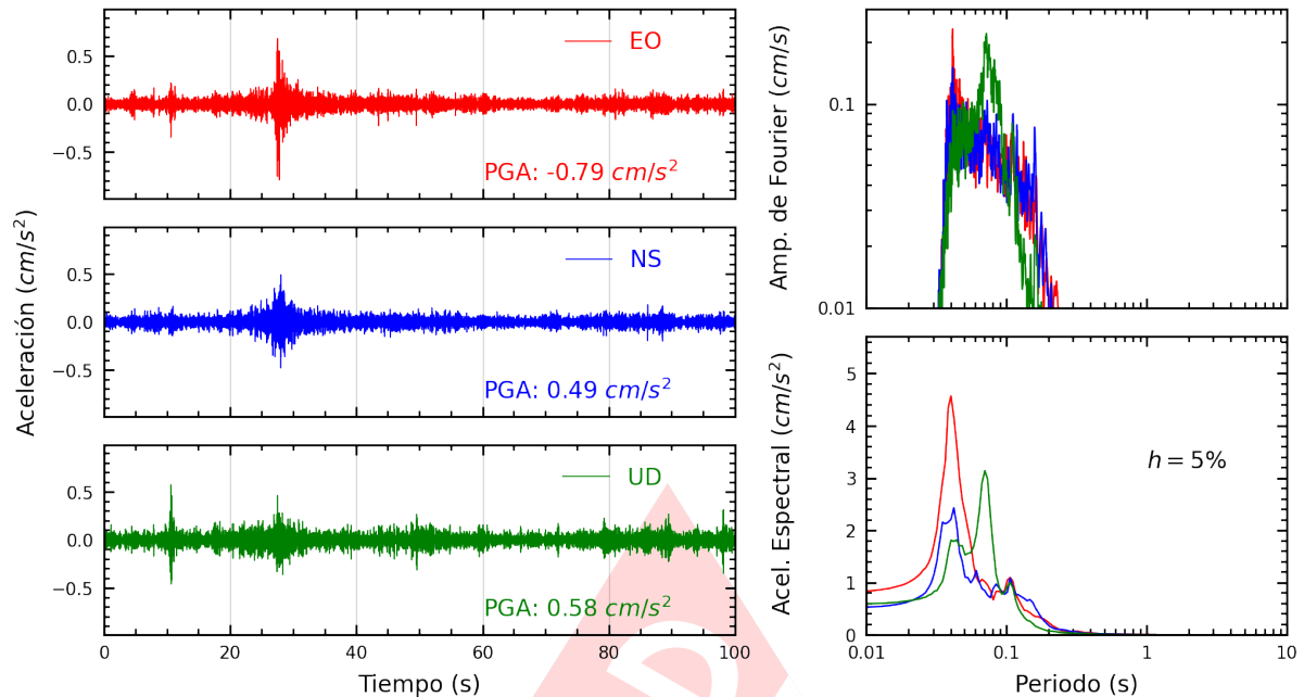
Figura A.3: Registros tiempo-historia, espectros de Fourier y de respuesta en las direcciones EO, NS y vertical de la estación CARA2. Sismo de Ancon, Lima - Lima del 2025-03-20, 09:04:23 (Hora local)
