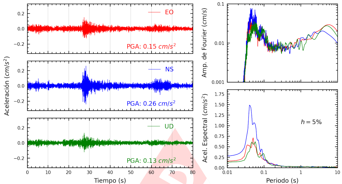
Figura A.7: Registros tiempo-historia, espectros de Fourier y de respuesta en las direcciones EO, NS y vertical de la estación COMAS. Sismo de Ancon, Lima - Lima del 2025-03-20, 09:04:23 (Hora local)
