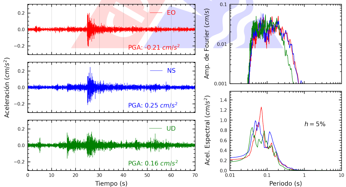
Figura A.8: Registros tiempo-historia, espectros de Fourier y de respuesta en las direcciones EO, NS y vertical de la estación VHAY2. Sismo de Ancon, Lima - Lima del 2025-03-20, 09:04:23 (Hora local)
