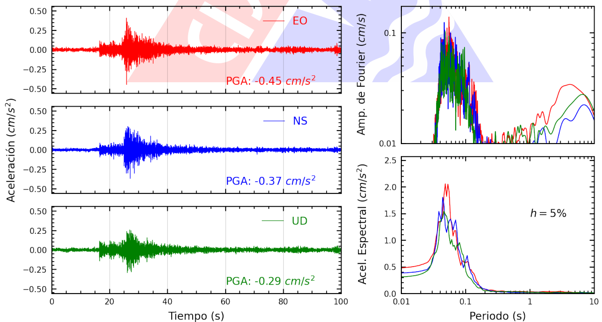
Figura A.4: Registros tiempo-historia, espectros de Fourier y de respuesta en las direcciones EO, NS y vertical de la estación AMORE. Sismo de Ancon, Lima - Lima del 2025-03-20, 09:04:23 (Hora local)
