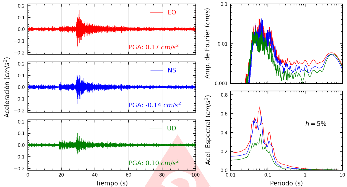
Figura A.11: Registros tiempo-historia, espectros de Fourier y de respuesta en las direcciones EO, NS y vertical de la estación ATARJ. Sismo de Ancon, Lima - Lima del 2025-03-20, 09:04:23 (Hora local)
