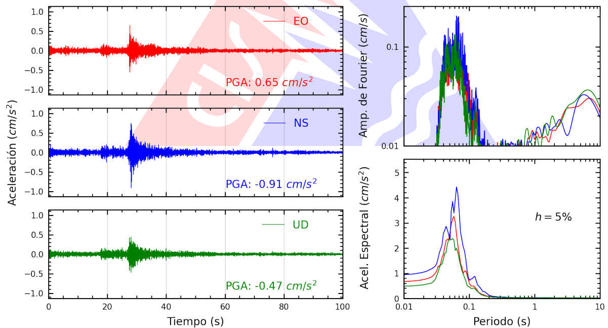
Figura A.2: Registros tiempo-historia, espectros de Fourier y de respuesta en las direcciones EO, NS y vertical de la estación JOSEO. Sismo de Ancon, Lima - Lima del 2025-03-20, 09:04:23 (Hora local)
