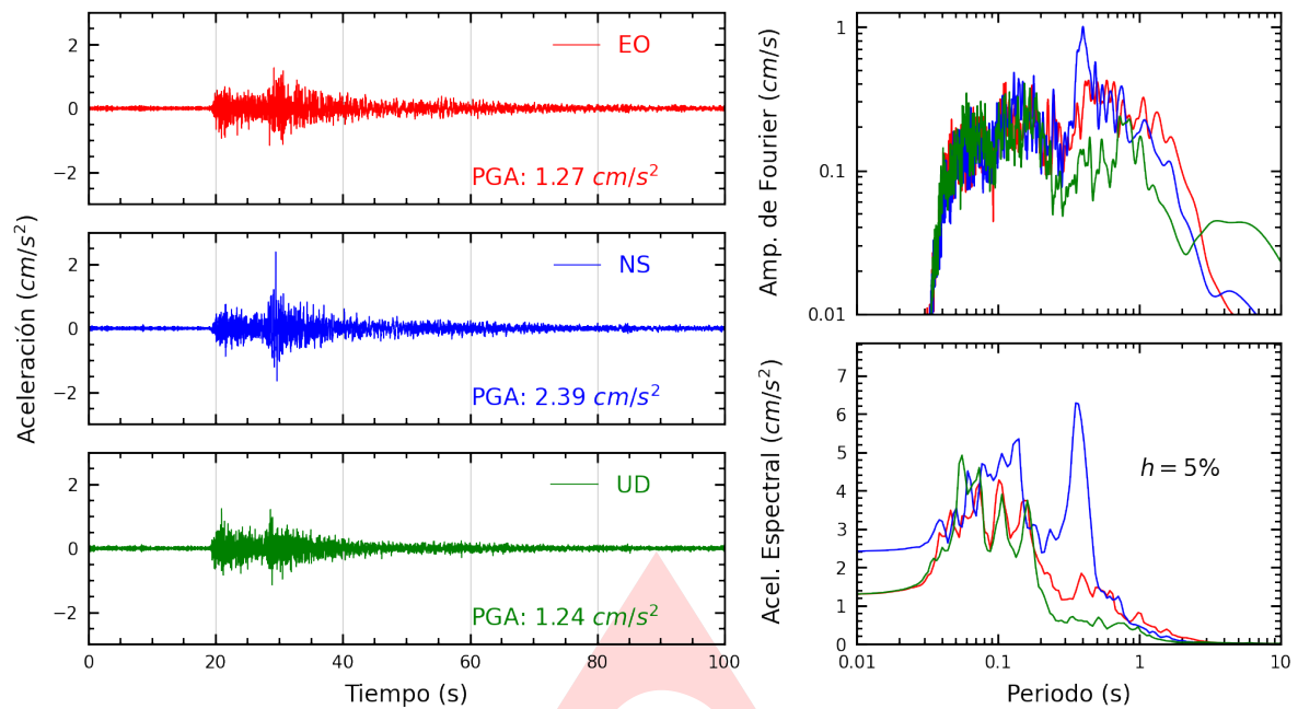
Figura A.1: Registros tiempo-historia, espectros de Fourier y de respuesta en las direcciones EO, NS y vertical de la estación SCARQ. Sismo de Maca, Caylloma - Arequipa del 2025-03-20, 20:04:16 (Hora local)
