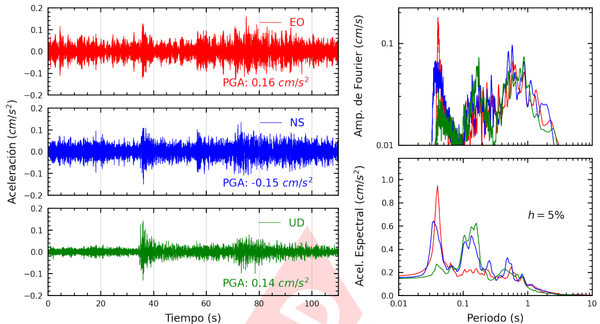
Figura A.5: Registros tiempo-historia, espectros de Fourier y de respuesta en las direcciones EO, NS y vertical de la estación UPTAC. Sismo de Maca, Caylloma - Arequipa del 2025-03-20, 20:04:16 (Hora local)
