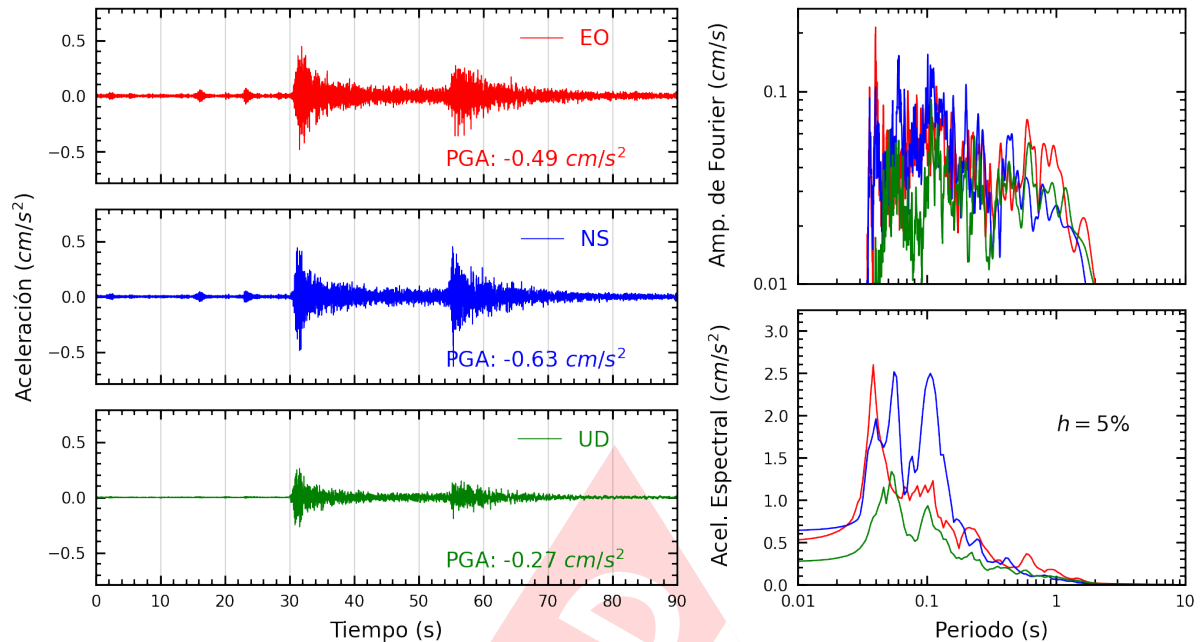
Figura A.3: Registros tiempo-historia, espectros de Fourier y de respuesta en las direcciones EO, NS y vertical de la estación UNAM. Sismo de Maca, Caylloma - Arequipa del 2025-03-20, 20:04:16 (Hora local)
