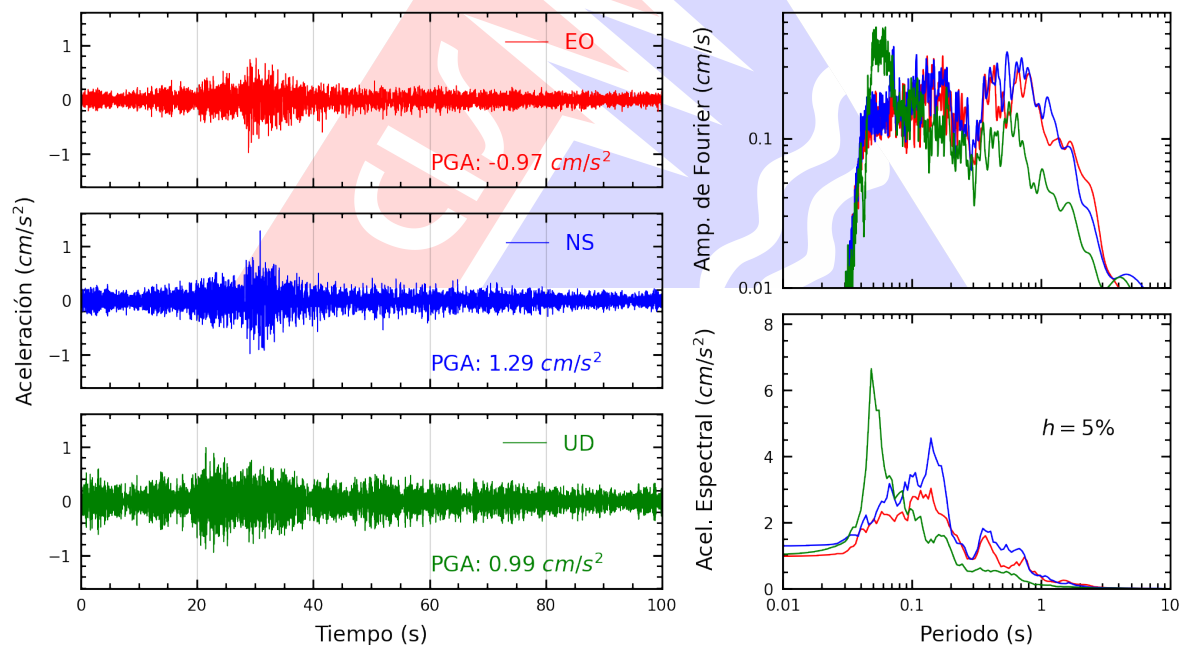
Figura A.2: Registros tiempo-historia, espectros de Fourier y de respuesta en las direcciones EO, NS y vertical de la estación SCAR2. Sismo de Maca, Caylloma - Arequipa del 2025-03-20, 20:04:16 (Hora local)
