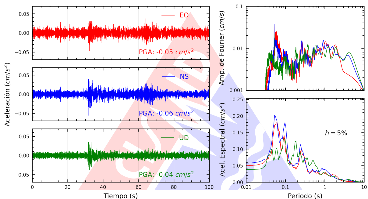
Figura A.7: Registros tiempo-historia, espectros de Fourier y de respuesta en las direcciones EO, NS y vertical de la estación UNMBA. Sismo de Maca, Caylloma - Arequipa del 2025-03-20, 20:04:16 (Hora local)
