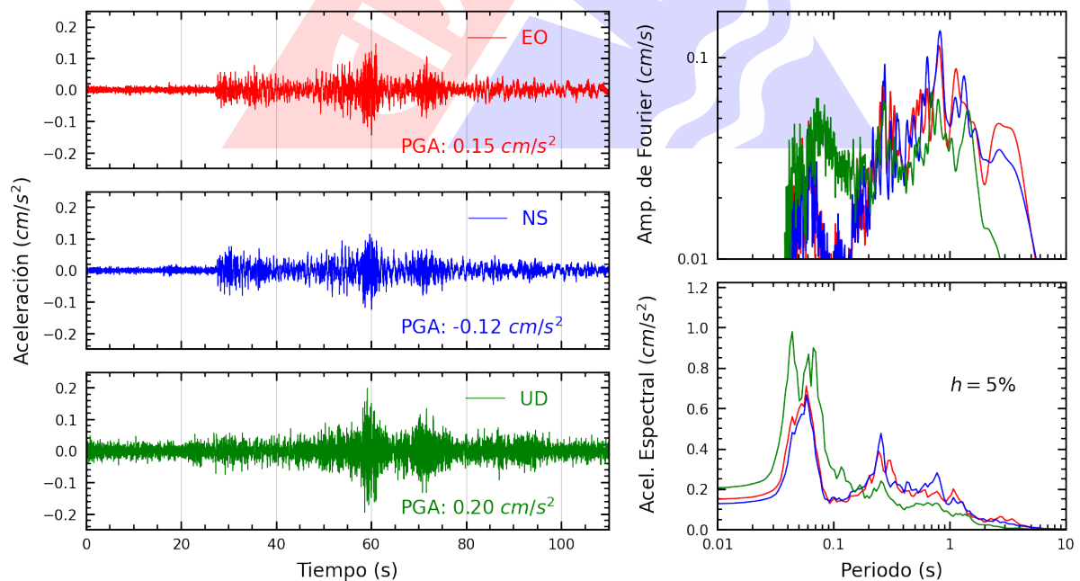
Figura A.4: Registros tiempo-historia, espectros de Fourier y de respuesta en las direcciones EO, NS y vertical de la estación UNAJ. Sismo de Maca, Caylloma - Arequipa del 2025-03-20, 20:04:16 (Hora local)
