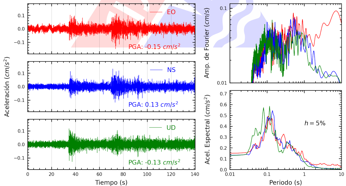
Figura A.6: Registros tiempo-historia, espectros de Fourier y de respuesta en las direcciones EO, NS y vertical de la estación UJBG3. Sismo de Maca, Caylloma - Arequipa del 2025-03-20, 20:04:16 (Hora local)
