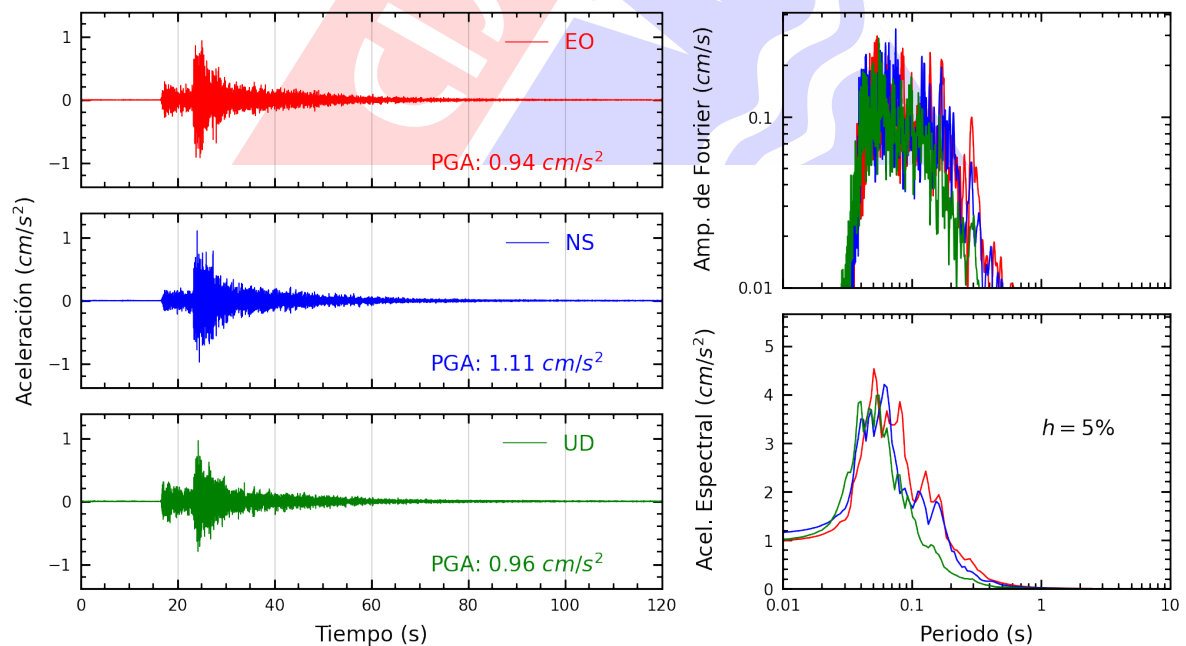
Figura A.26: Registros tiempo-historia, espectros de Fourier y de respuesta en las direcciones EO, NS y vertical de la estación JALV2. Sismo de Lima, Lima - Lima del 2025-03-22, 00:14:18 (Hora local)
