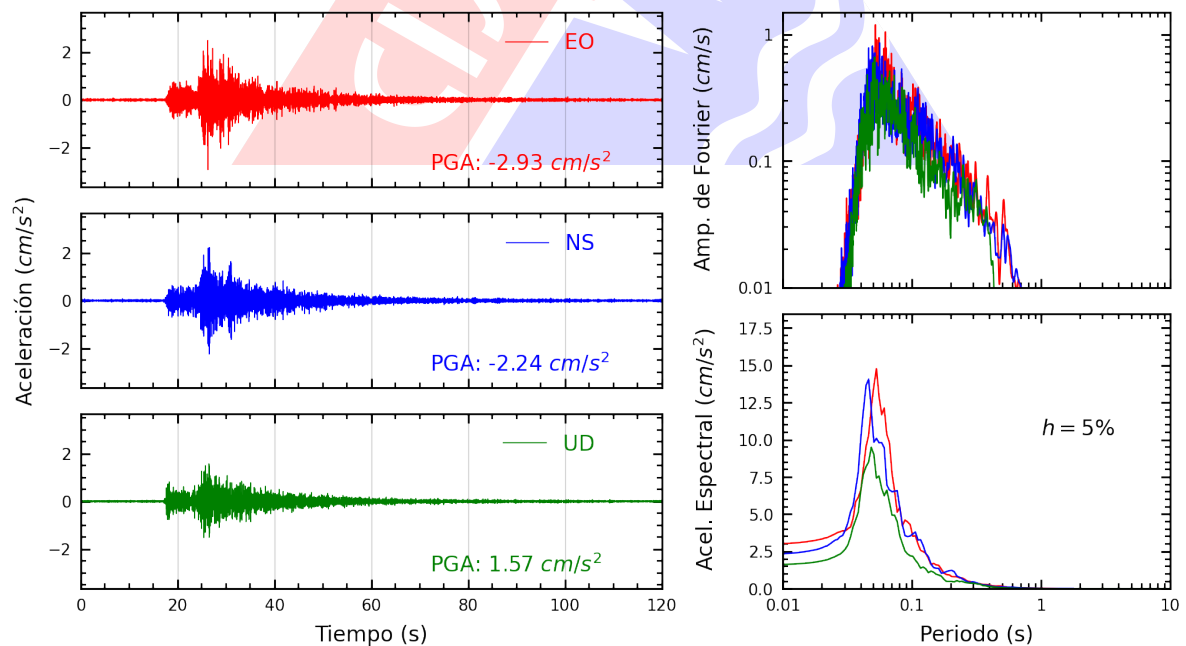
Figura A.8: Registros tiempo-historia, espectros de Fourier y de respuesta en las direcciones EO, NS y vertical de la estación UNTEL. Sismo de Lima, Lima - Lima del 2025-03-22, 00:14:18 (Hora local)
