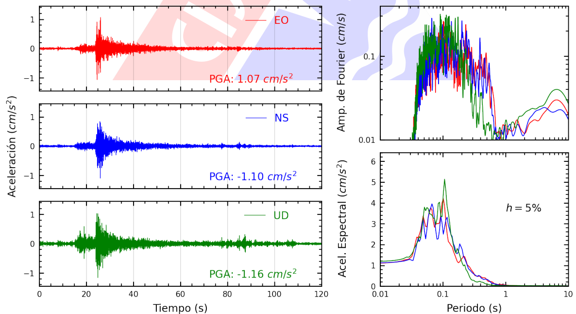
Figura A.22: Registros tiempo-historia, espectros de Fourier y de respuesta en las direcciones EO, NS y vertical de la estación MDPP. Sismo de Lima, Lima - Lima del 2025-03-22, 00:14:18 (Hora local)
