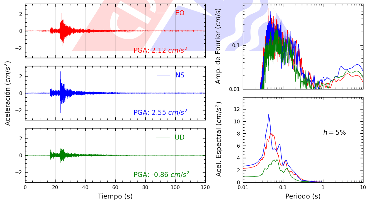
Figura A.10: Registros tiempo-historia, espectros de Fourier y de respuesta en las direcciones EO, NS y vertical de la estación CEPRE. Sismo de Lima, Lima - Lima del 2025-03-22, 00:14:18 (Hora local)
