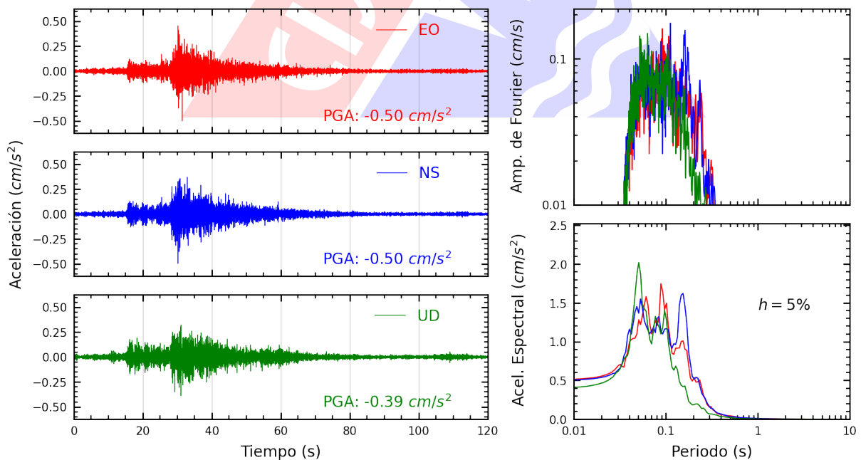
Figura A.36: Registros tiempo-historia, espectros de Fourier y de respuesta en las direcciones EO, NS y vertical de la estación ASIA. Sismo de Lima, Lima - Lima del 2025-03-22, 00:14:18 (Hora local)
