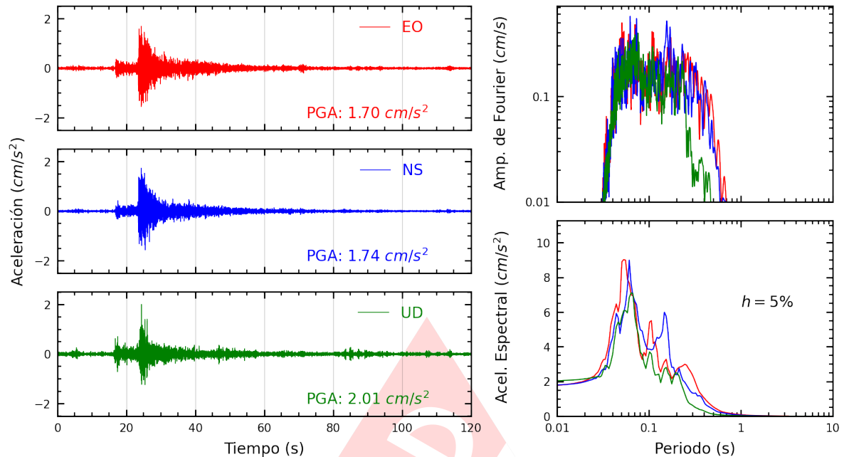
Figura A.15: Registros tiempo-historia, espectros de Fourier y de respuesta en las direcciones EO, NS y vertical de la estación SCOLI. Sismo de Lima, Lima - Lima del 2025-03-22, 00:14:18 (Hora local)
