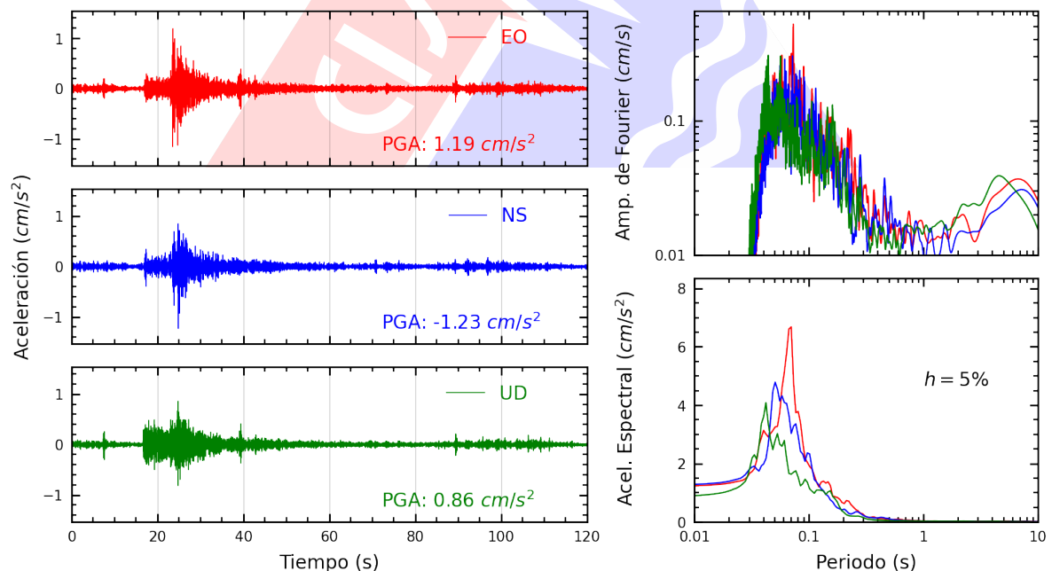
Figura A.20: Registros tiempo-historia, espectros de Fourier y de respuesta en las direcciones EO, NS y vertical de la estación UPCSM. Sismo de Lima, Lima - Lima del 2025-03-22, 00:14:18 (Hora local)
