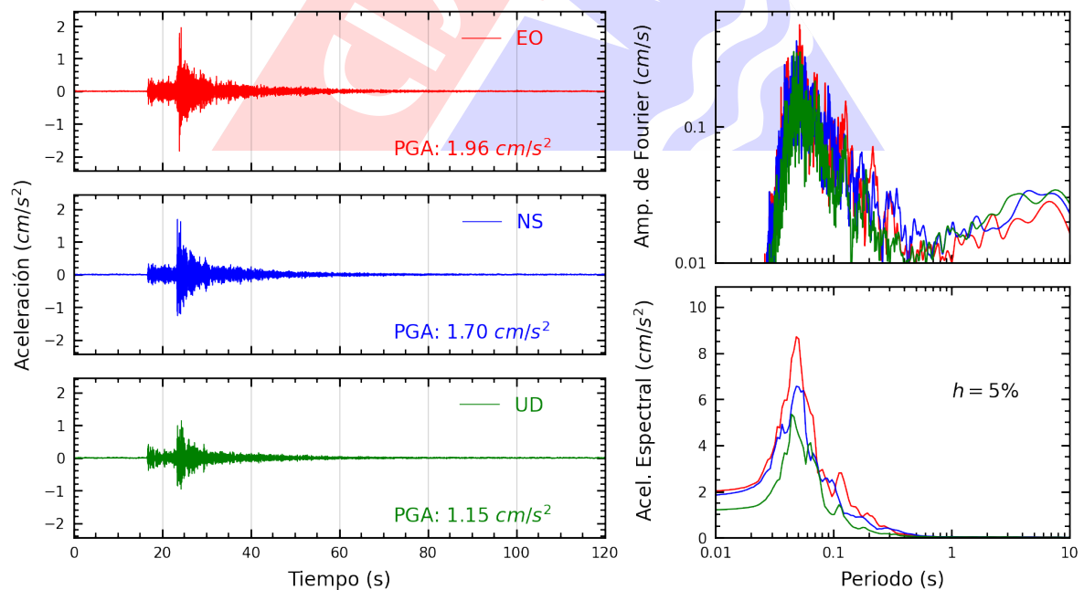
Figura A.16: Registros tiempo-historia, espectros de Fourier y de respuesta en las direcciones EO, NS y vertical de la estación UCSS. Sismo de Lima, Lima - Lima del 2025-03-22, 00:14:18 (Hora local)
