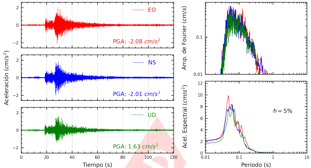
Figura A.13: Registros tiempo-historia, espectros de Fourier y de respuesta en las direcciones EO, NS y vertical de la estación PHER2. Sismo de Lima, Lima - Lima del 2025-03-22, 00:14:18 (Hora local)
