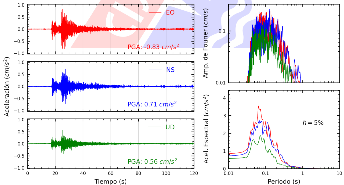
Figura A.32: Registros tiempo-historia, espectros de Fourier y de respuesta en las direcciones EO, NS y vertical de la estación BRISA. Sismo de Lima, Lima - Lima del 2025-03-22, 00:14:18 (Hora local)
