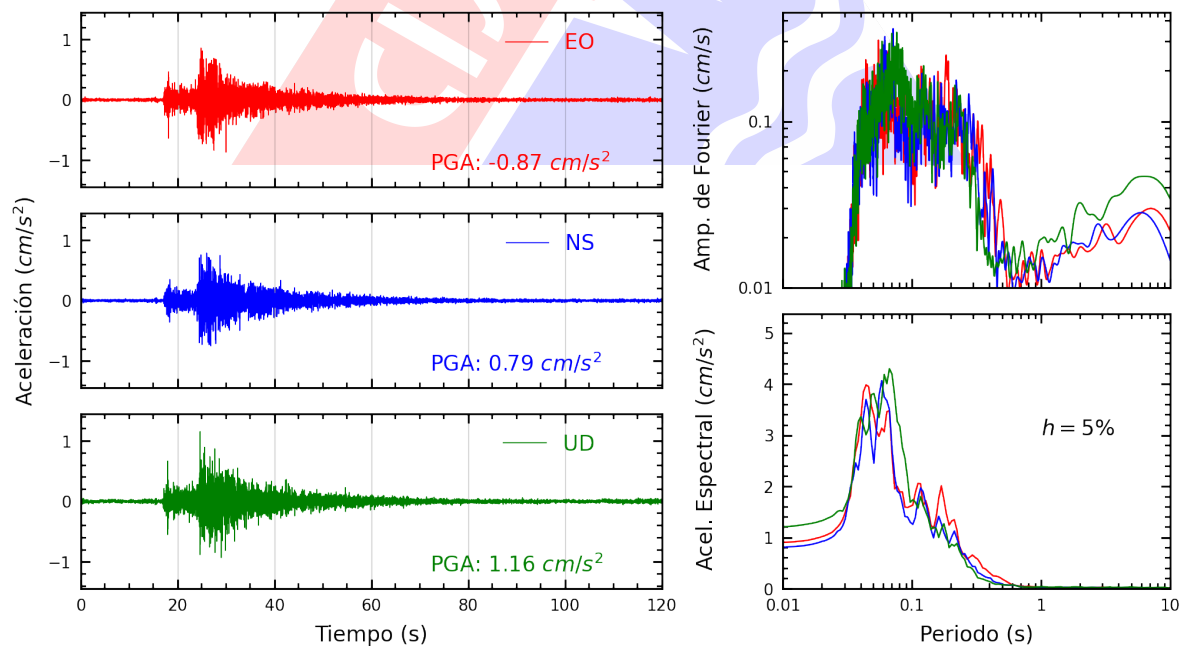
Figura A.24: Registros tiempo-historia, espectros de Fourier y de respuesta en las direcciones EO, NS y vertical de la estación SOVES. Sismo de Lima, Lima - Lima del 2025-03-22, 00:14:18 (Hora local)
