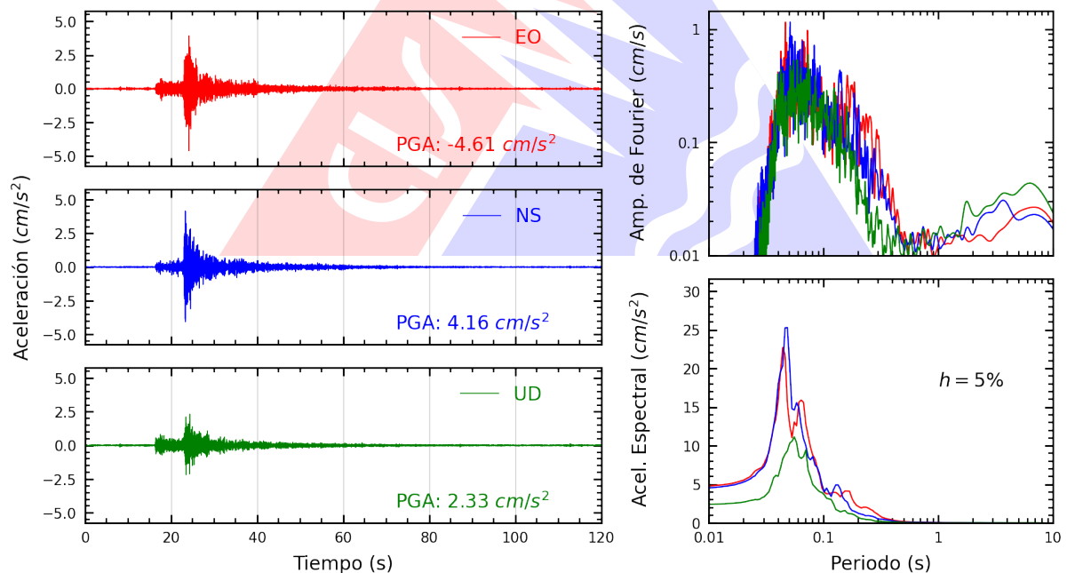
Figura A.2: Registros tiempo-historia, espectros de Fourier y de respuesta en las direcciones EO, NS y vertical de la estación INDEP. Sismo de Lima, Lima - Lima del 2025-03-22, 00:14:18 (Hora local)
