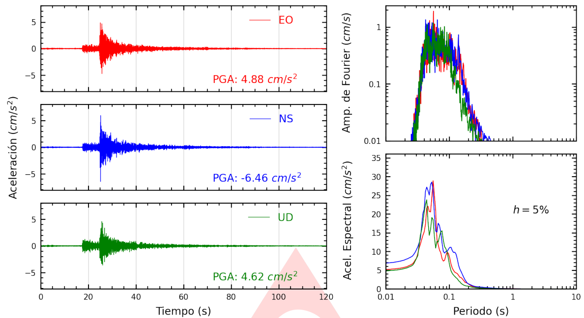
Figura A.1: Registros tiempo-historia, espectros de Fourier y de respuesta en las direcciones EO, NS y vertical de la estación SROS2. Sismo de Lima, Lima - Lima del 2025-03-22, 00:14:18 (Hora local)
