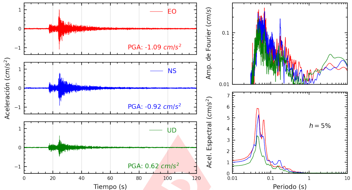
Figura A.27: Registros tiempo-historia, espectros de Fourier y de respuesta en las direcciones EO, NS y vertical de la estación UPCVI. Sismo de Lima, Lima - Lima del 2025-03-22, 00:14:18 (Hora local)
