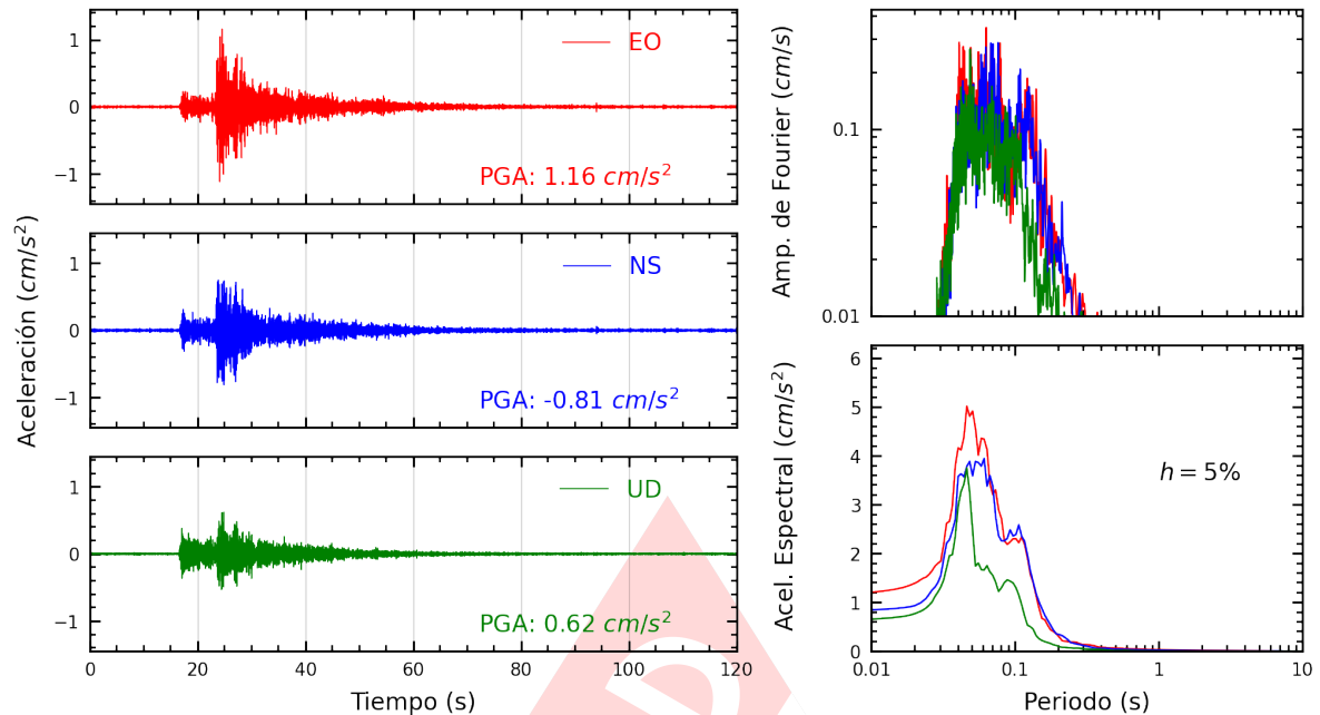
Figura A.23: Registros tiempo-historia, espectros de Fourier y de respuesta en las direcciones EO, NS y vertical de la estación ATARJ. Sismo de Lima, Lima - Lima del 2025-03-22, 00:14:18 (Hora local)
