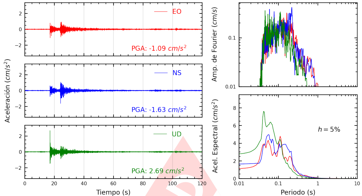
Figura A.9: Registros tiempo-historia, espectros de Fourier y de respuesta en las direcciones EO, NS y vertical de la estación SCCHO. Sismo de Lima, Lima - Lima del 2025-03-22, 00:14:18 (Hora local)
