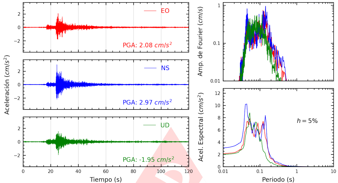
Figura A.7: Registros tiempo-historia, espectros de Fourier y de respuesta en las direcciones EO, NS y vertical de la estación CARA2. Sismo de Lima, Lima - Lima del 2025-03-22, 00:14:18 (Hora local)
