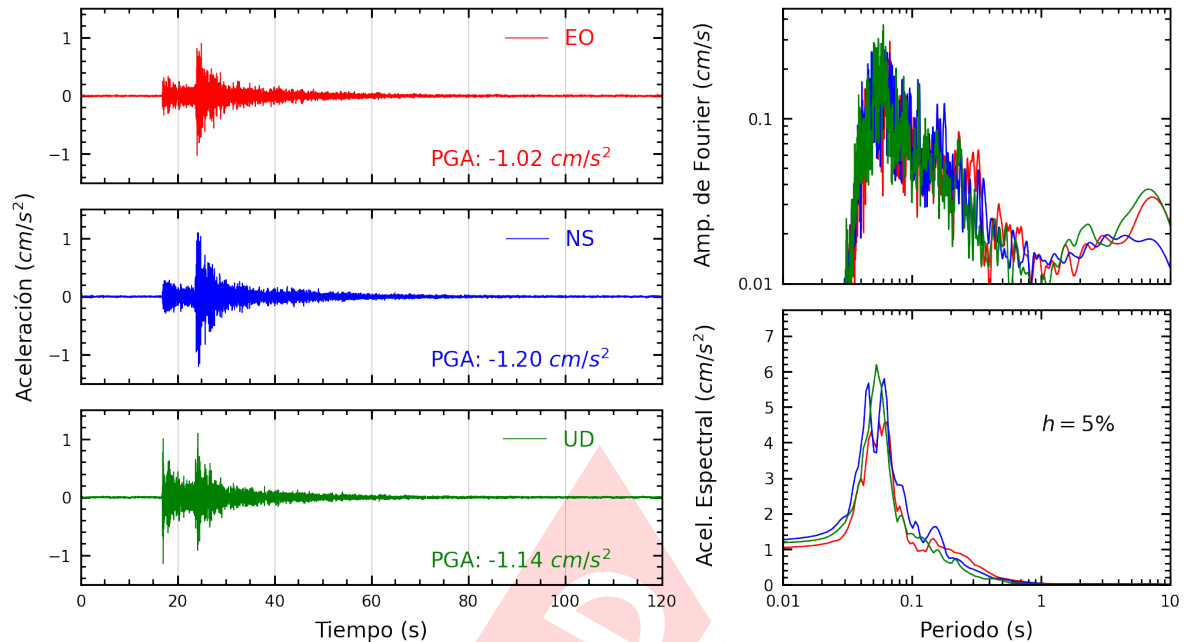
Figura A.21: Registros tiempo-historia, espectros de Fourier y de respuesta en las direcciones EO, NS y vertical de la estación SERVI. Sismo de Lima, Lima - Lima del 2025-03-22, 00:14:18 (Hora local)
