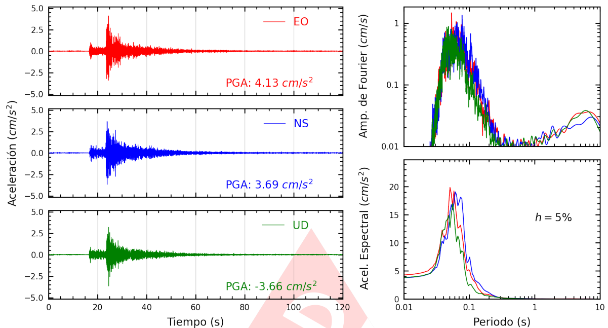
Figura A.3: Registros tiempo-historia, espectros de Fourier y de respuesta en las direcciones EO, NS y vertical de la estación JOSEO. Sismo de Lima, Lima - Lima del 2025-03-22, 00:14:18 (Hora local)
