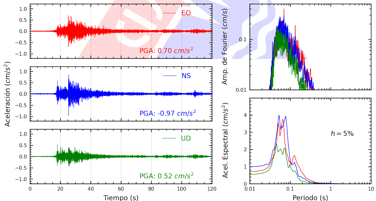
Figura A.28: Registros tiempo-historia, espectros de Fourier y de respuesta en las direcciones EO, NS y vertical de la estación PACHA. Sismo de Lima, Lima - Lima del 2025-03-22, 00:14:18 (Hora local)
