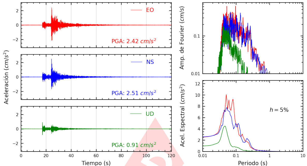
Figura A.11: Registros tiempo-historia, espectros de Fourier y de respuesta en las direcciones EO, NS y vertical de la estación UCVA2. Sismo de Lima, Lima - Lima del 2025-03-22, 00:14:18 (Hora local)
