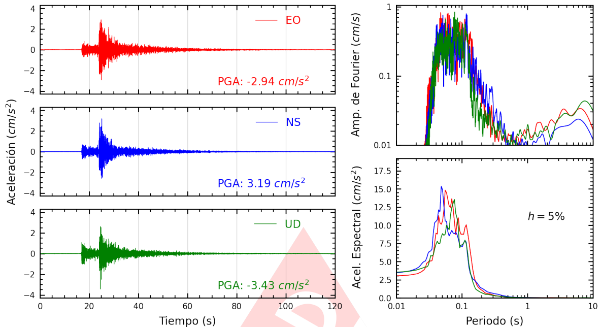
Figura A.5: Registros tiempo-historia, espectros de Fourier y de respuesta en las direcciones EO, NS y vertical de la estación AMORE. Sismo de Lima, Lima - Lima del 2025-03-22, 00:14:18 (Hora local)
