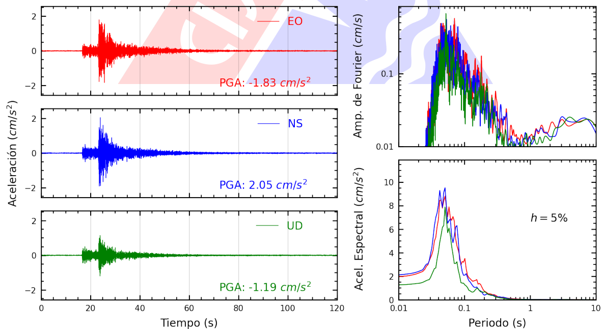
Figura A.14: Registros tiempo-historia, espectros de Fourier y de respuesta en las direcciones EO, NS y vertical de la estación FICPE. Sismo de Lima, Lima - Lima del 2025-03-22, 00:14:18 (Hora local)
