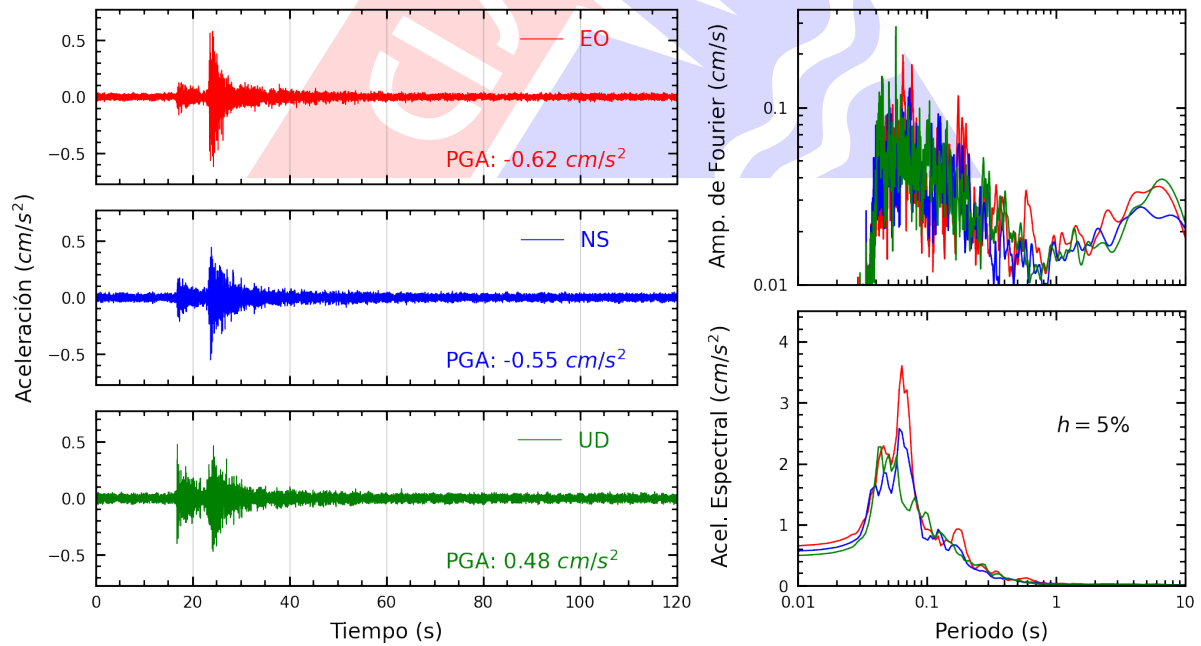
Figura A.34: Registros tiempo-historia, espectros de Fourier y de respuesta en las direcciones EO, NS y vertical de la estación BONDY. Sismo de Lima, Lima - Lima del 2025-03-22, 00:14:18 (Hora local)
