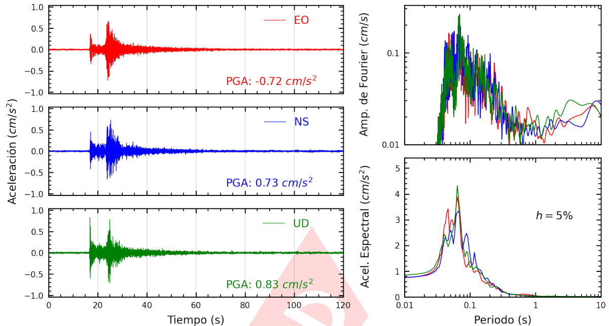
Figura A.31: Registros tiempo-historia, espectros de Fourier y de respuesta en las direcciones EO, NS y vertical de la estación UNFV. Sismo de Lima, Lima - Lima del 2025-03-22, 00:14:18 (Hora local)
