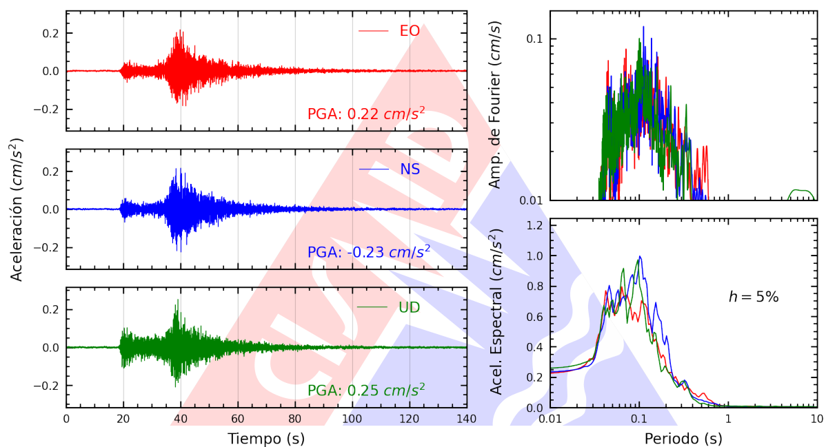
Figura A.37: Registros tiempo-historia, espectros de Fourier y de respuesta en las direcciones EO, NS y vertical de la estación CARAL. Sismo de Lima, Lima - Lima del 2025-03-22, 00:14:18 (Hora local)
