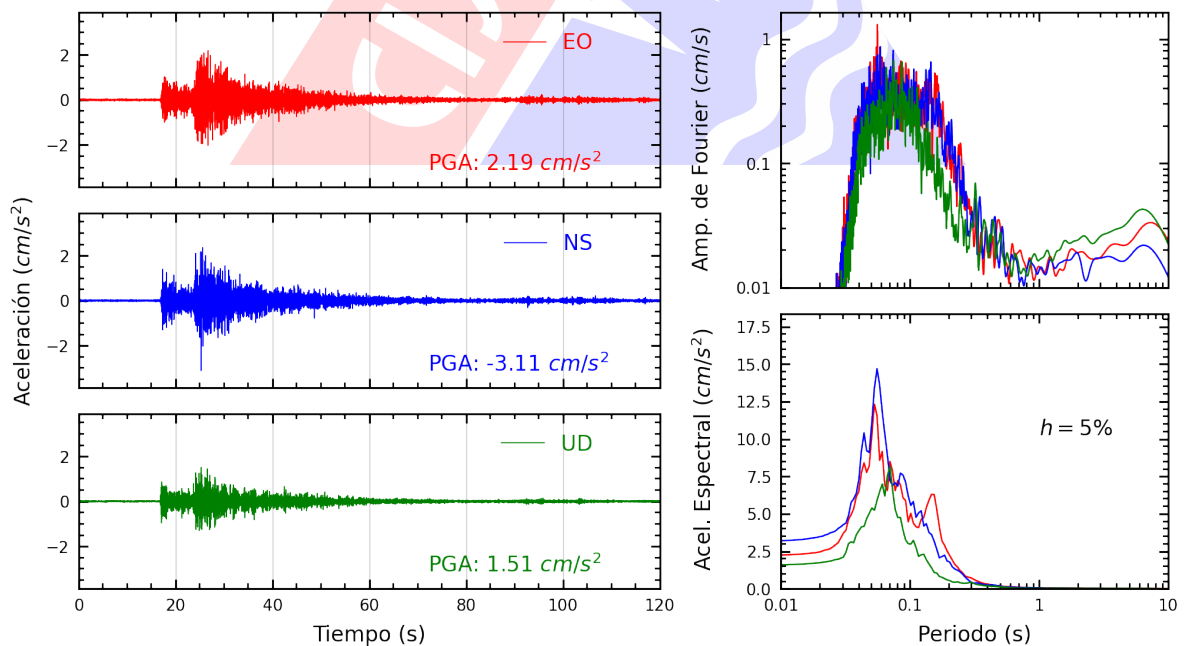
Figura A.6: Registros tiempo-historia, espectros de Fourier y de respuesta en las direcciones EO, NS y vertical de la estación USILM. Sismo de Lima, Lima - Lima del 2025-03-22, 00:14:18 (Hora local)
