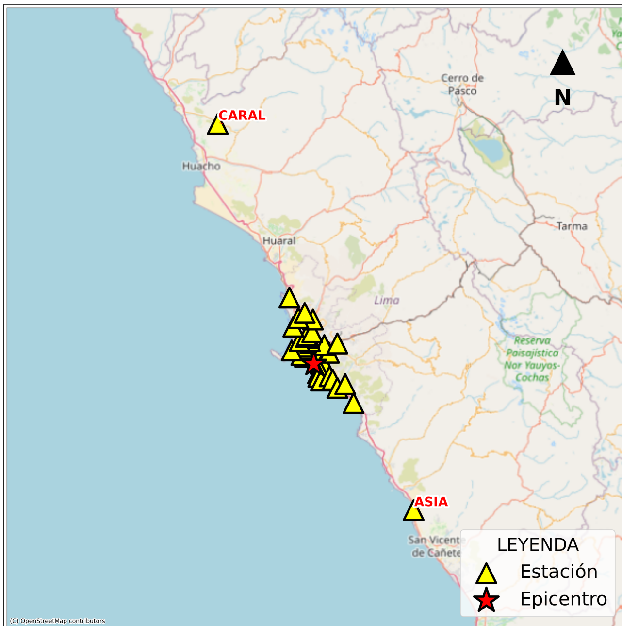
Figura 2: Mapa de ubicación de la(s) estación(es) acelerográfica(s) a nivel nacional correspondiente(s) al Sismo de Lima, Lima - Lima del 22 de marzo de 2025 a las 00:14:18 (hora local)
