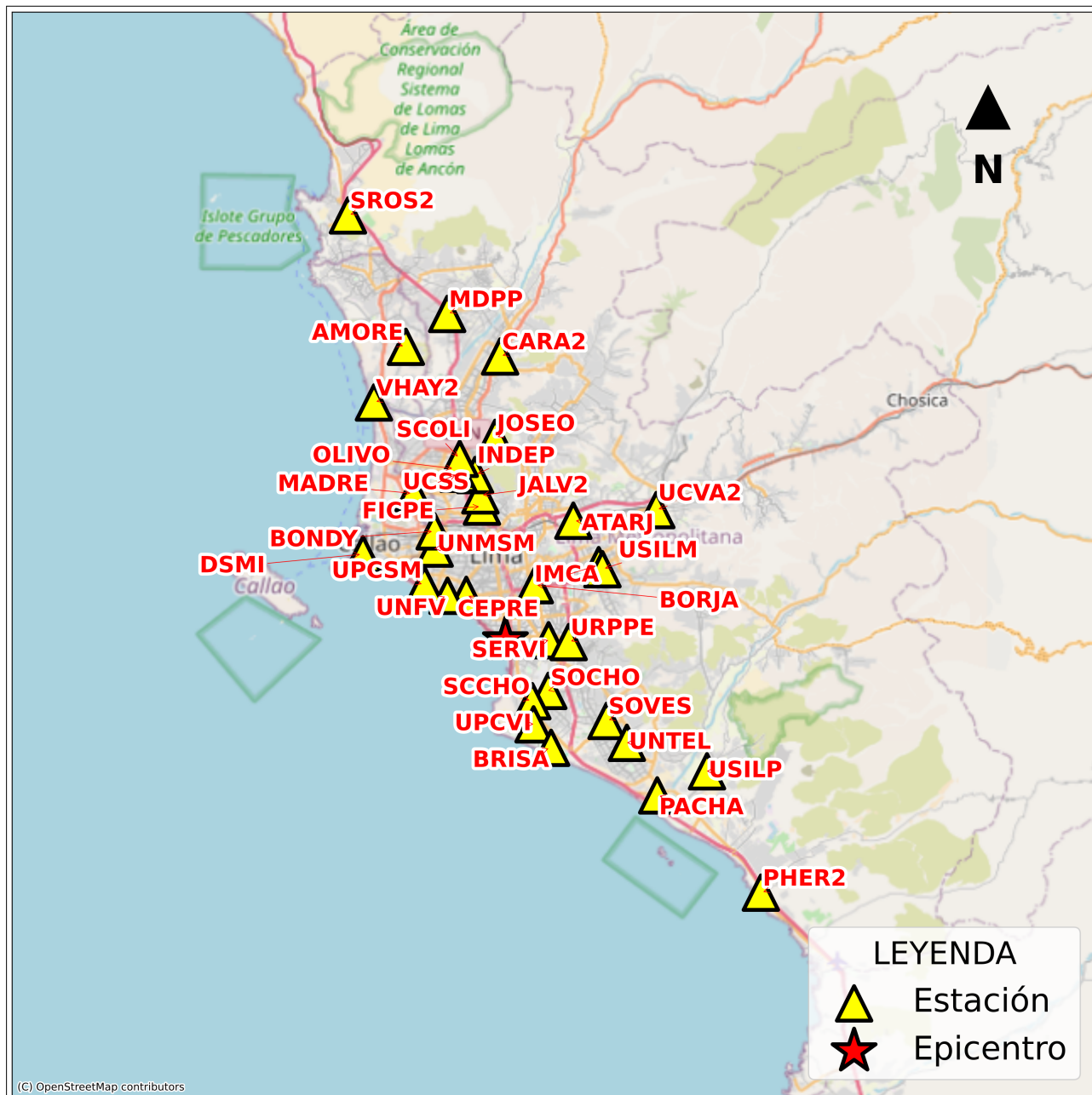
Figura 3: Mapa de ubicación de la(s) estación(es) acelerográfica(s) en Lima Metropolitana correspondiente(s) al Sismo de Lima, Lima - Lima del 22 de marzo de 2025 a las 00:14:18 (hora local)
