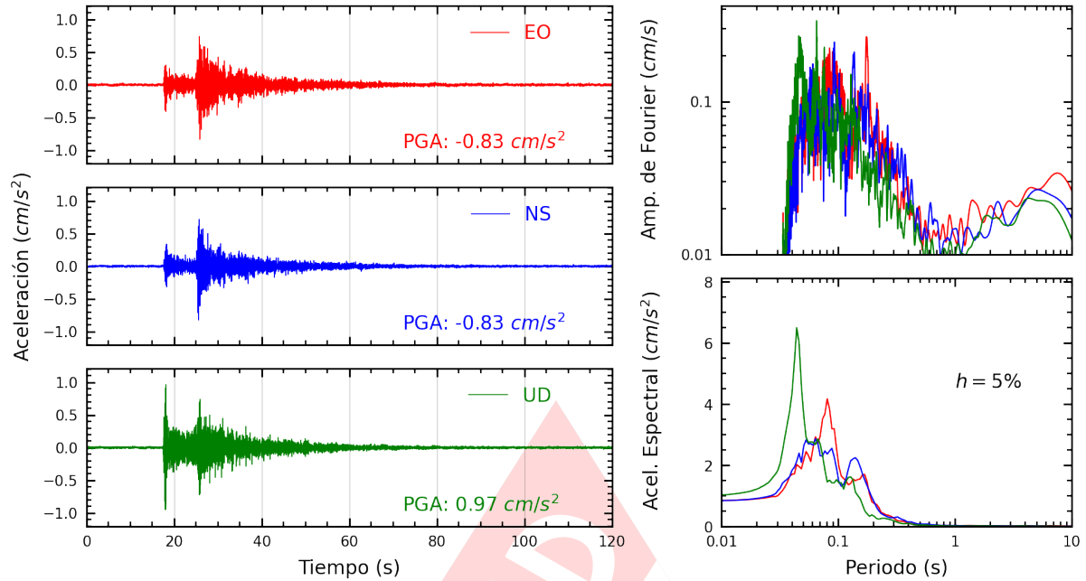
Figura A.29: Registros tiempo-historia, espectros de Fourier y de respuesta en las direcciones EO, NS y vertical de la estación USILP. Sismo de Lima, Lima - Lima del 2025-03-22, 00:14:18 (Hora local)
