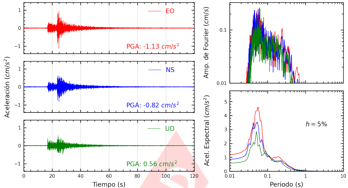
Figura A.25: Registros tiempo-historia, espectros de Fourier y de respuesta en las direcciones EO, NS y vertical de la estación BORJA. Sismo de Lima, Lima - Lima del 2025-03-22, 00:14:18 (Hora local)
