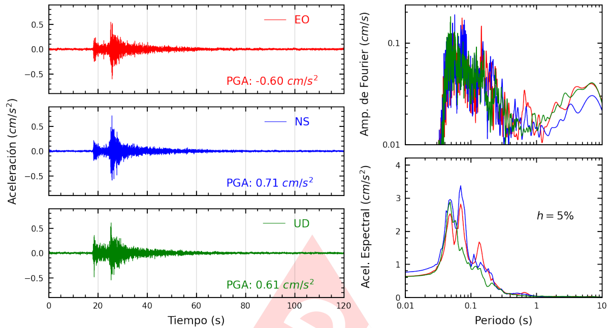
Figura A.33: Registros tiempo-historia, espectros de Fourier y de respuesta en las direcciones EO, NS y vertical de la estación UNMSM. Sismo de Lima, Lima - Lima del 2025-03-22, 00:14:18 (Hora local)
