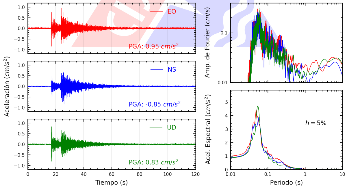
Figura A.30: Registros tiempo-historia, espectros de Fourier y de respuesta en las direcciones EO, NS y vertical de la estación IMCA. Sismo de Lima, Lima - Lima del 2025-03-22, 00:14:18 (Hora local)
