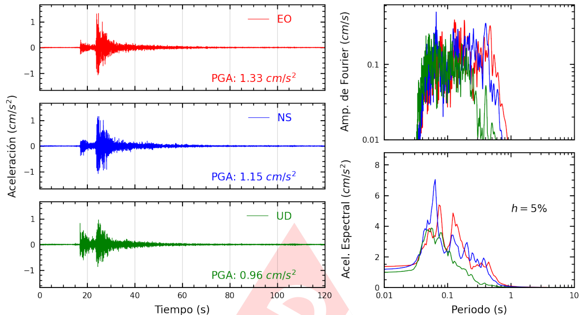
Figura A.19: Registros tiempo-historia, espectros de Fourier y de respuesta en las direcciones EO, NS y vertical de la estación VHAY2. Sismo de Lima, Lima - Lima del 2025-03-22, 00:14:18 (Hora local)
