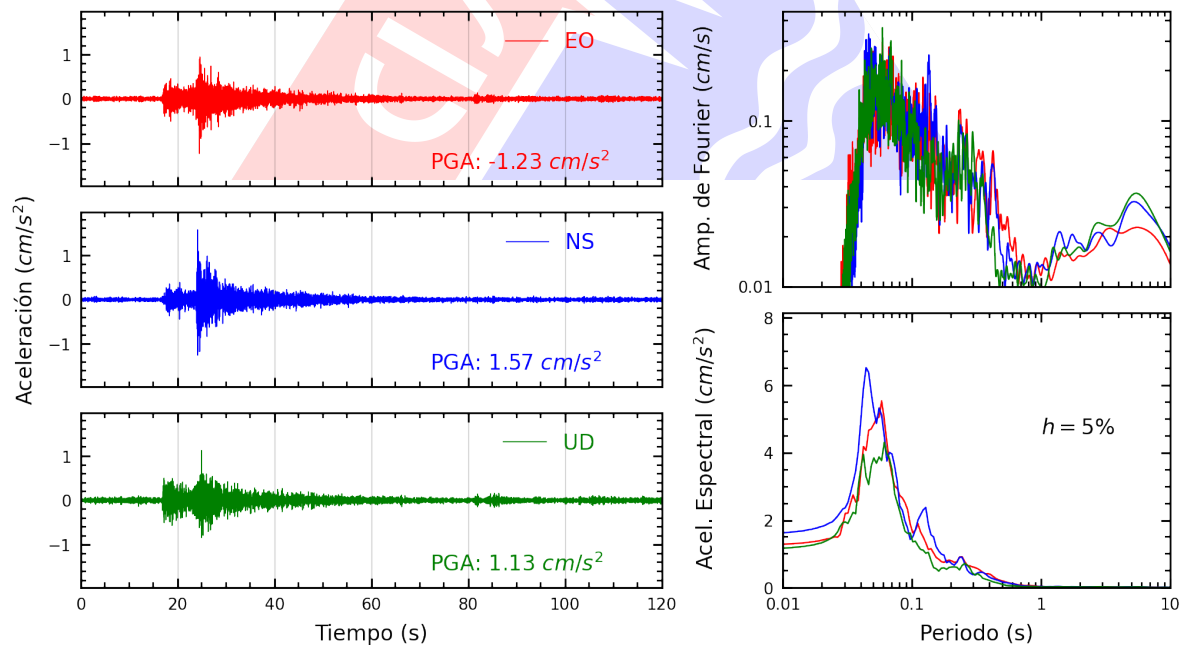
Figura A.18: Registros tiempo-historia, espectros de Fourier y de respuesta en las direcciones EO, NS y vertical de la estación URPE. Sismo de Lima, Lima - Lima del 2025-03-22, 00:14:18 (Hora local)
