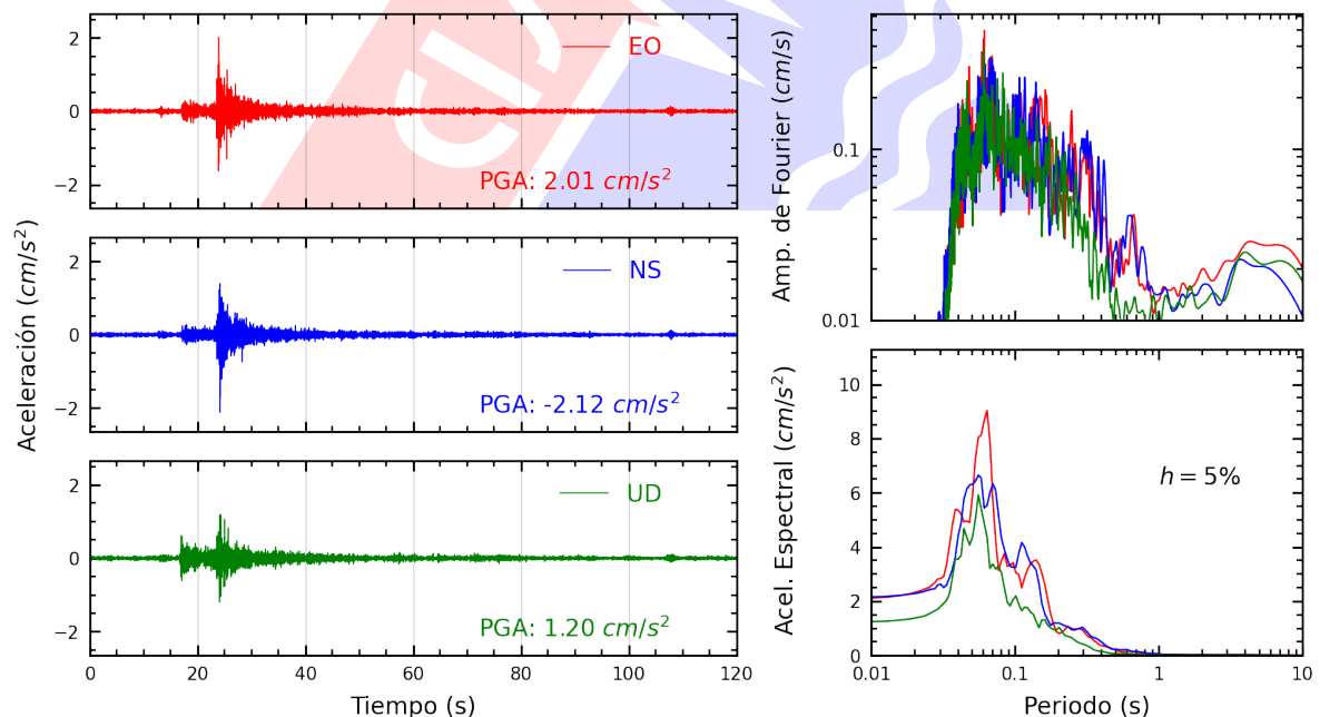
Figura A.12: Registros tiempo-historia, espectros de Fourier y de respuesta en las direcciones EO, NS y vertical de la estación MADRE. Sismo de Lima, Lima - Lima del 2025-03-22, 00:14:18 (Hora local)
