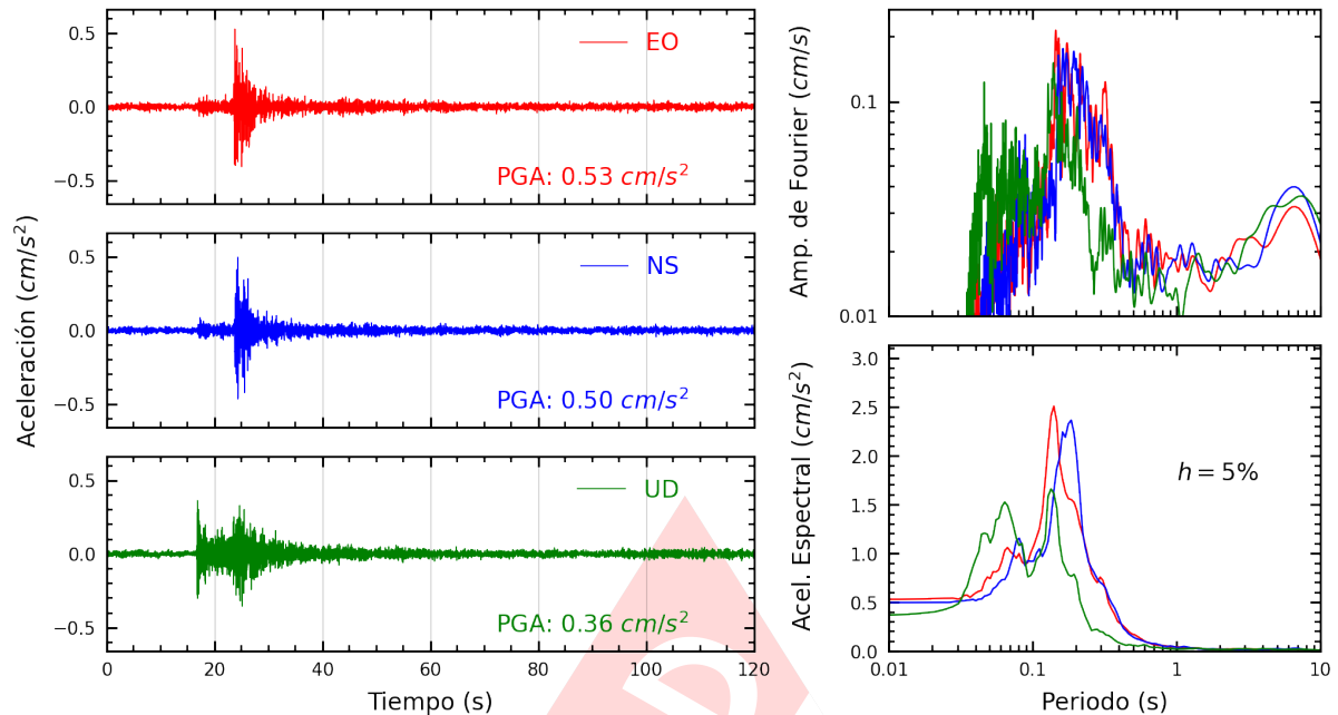
Figura A.35: Registros tiempo-historia, espectros de Fourier y de respuesta en las direcciones EO, NS y vertical de la estación DSML. Sismo de Lima, Lima - Lima del 2025-03-22, 00:14:18 (Hora local)
