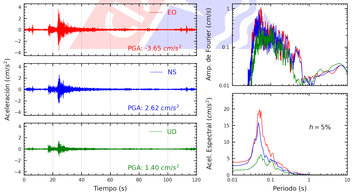
Figura A.4: Registros tiempo-historia, espectros de Fourier y de respuesta en las direcciones EO, NS y vertical de la estación OLIVO. Sismo de Lima, Lima - Lima del 2025-03-22, 00:14:18 (Hora local)
