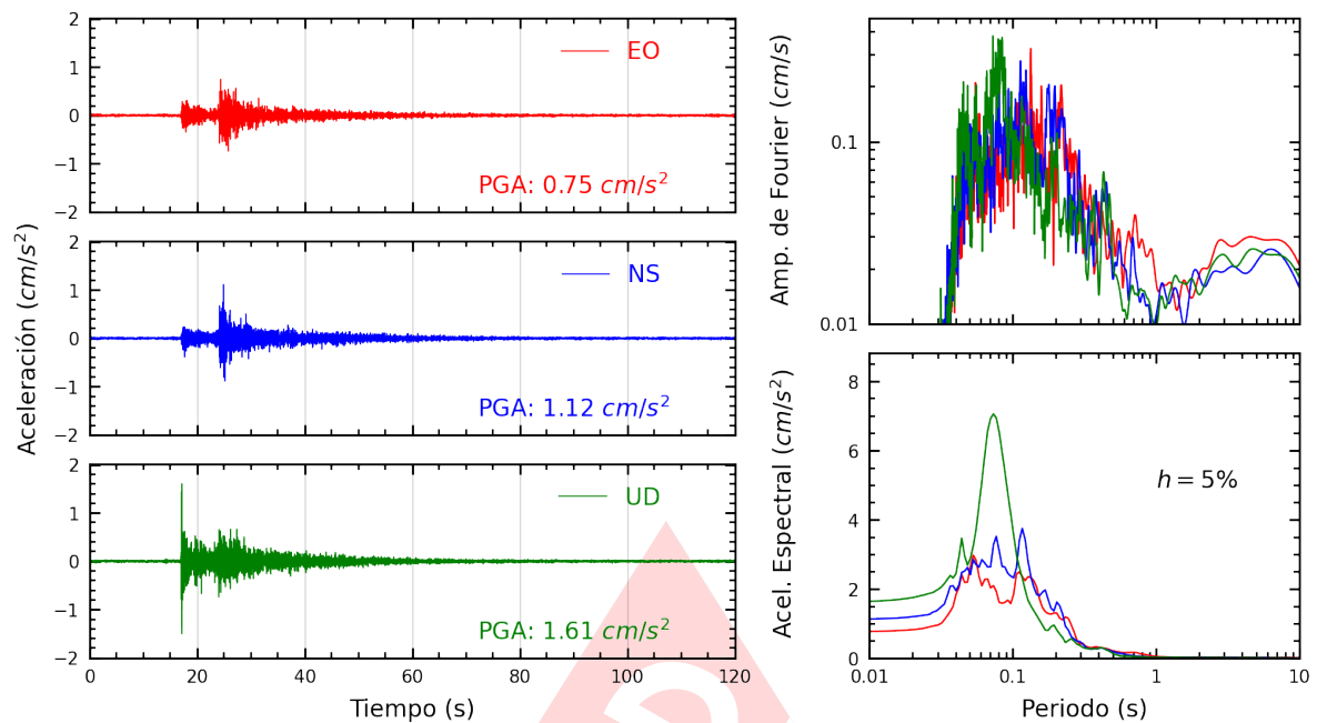
Figura A.17: Registros tiempo-historia, espectros de Fourier y de respuesta en las direcciones EO, NS y vertical de la estación SOCHO. Sismo de Lima, Lima - Lima del 2025-03-22, 00:14:18 (Hora local)
