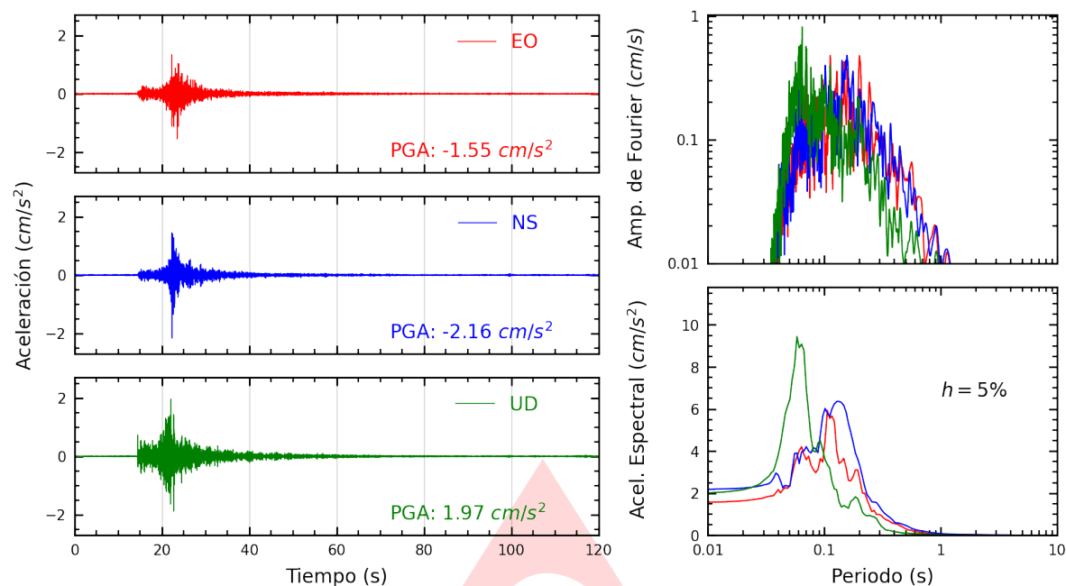
Figura A.1: Registros tiempo-historia, espectros de Fourier y de respuesta en las direcciones EO, NS y vertical de la estación UNAAA. Sismo de Moyobamba, Moyobamba - San Martín del 2025-03-23, 10:32:35 (Hora local)
