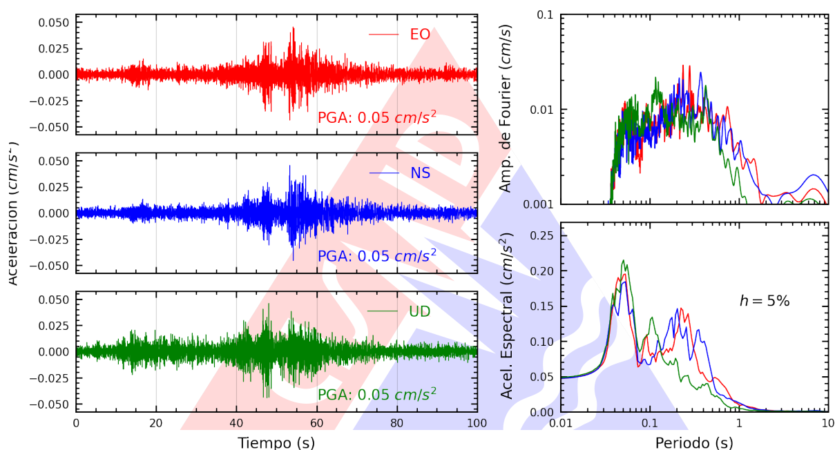
Figura A.3: Registros tiempo-historia, espectros de Fourier y de respuesta en las direcciones EO, NS y vertical de la estación UNIA. Sismo de Moyobamba, Moyobamba - San Martín del 2025-03-23, 10:32:35 (Hora local)
