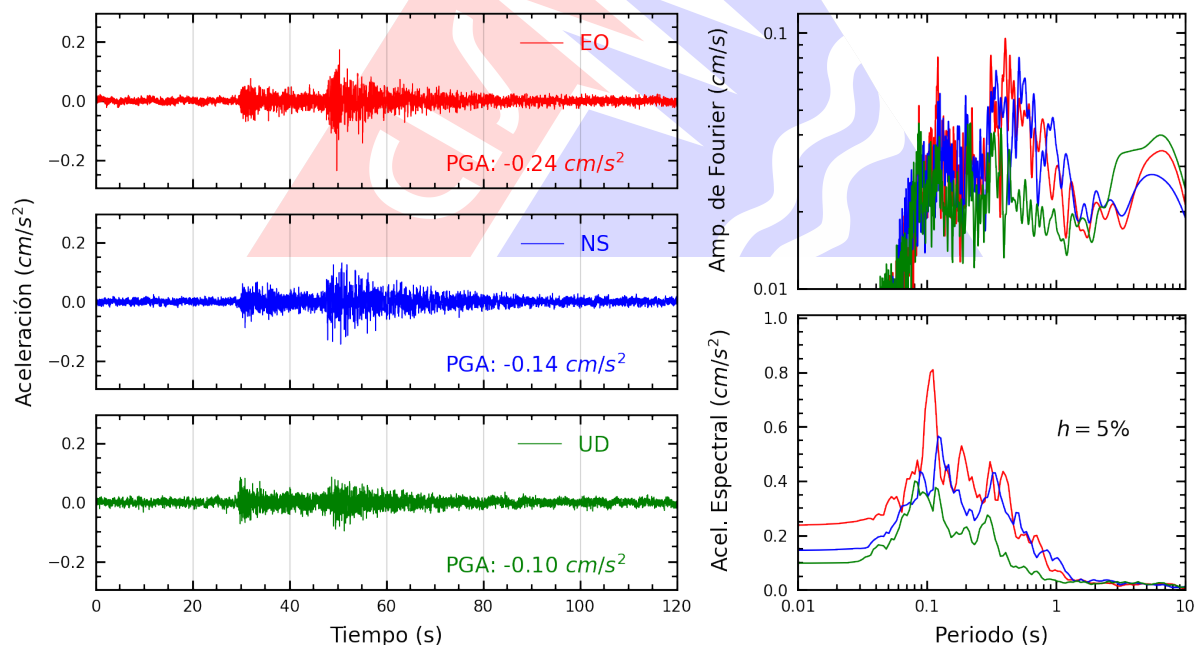
Figura A.2: Registros tiempo-historia, espectros de Fourier y de respuesta en las direcciones EO, NS y vertical de la estación UNTRM. Sismo de Moyobamba, Moyobamba - San Martín del 2025-03-23, 10:32:35 (Hora local)
