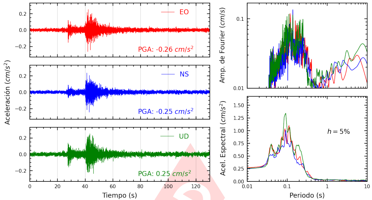
Figura A.19: Registros tiempo-historia, espectros de Fourier y de respuesta en las direcciones EO, NS y vertical de la estación SOVES. Sismo de Matucana, Huarochiri - Lima del 2025-03-23, 22:59:59 (Hora local)
