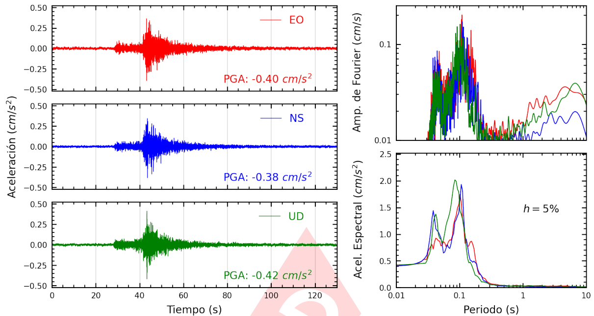
Figura A.13: Registros tiempo-historia, espectros de Fourier y de respuesta en las direcciones EO, NS y vertical de la estación AMORE. Sismo de Matucana, Huarochiri - Lima del 2025-03-23, 22:59:59 (Hora local)
