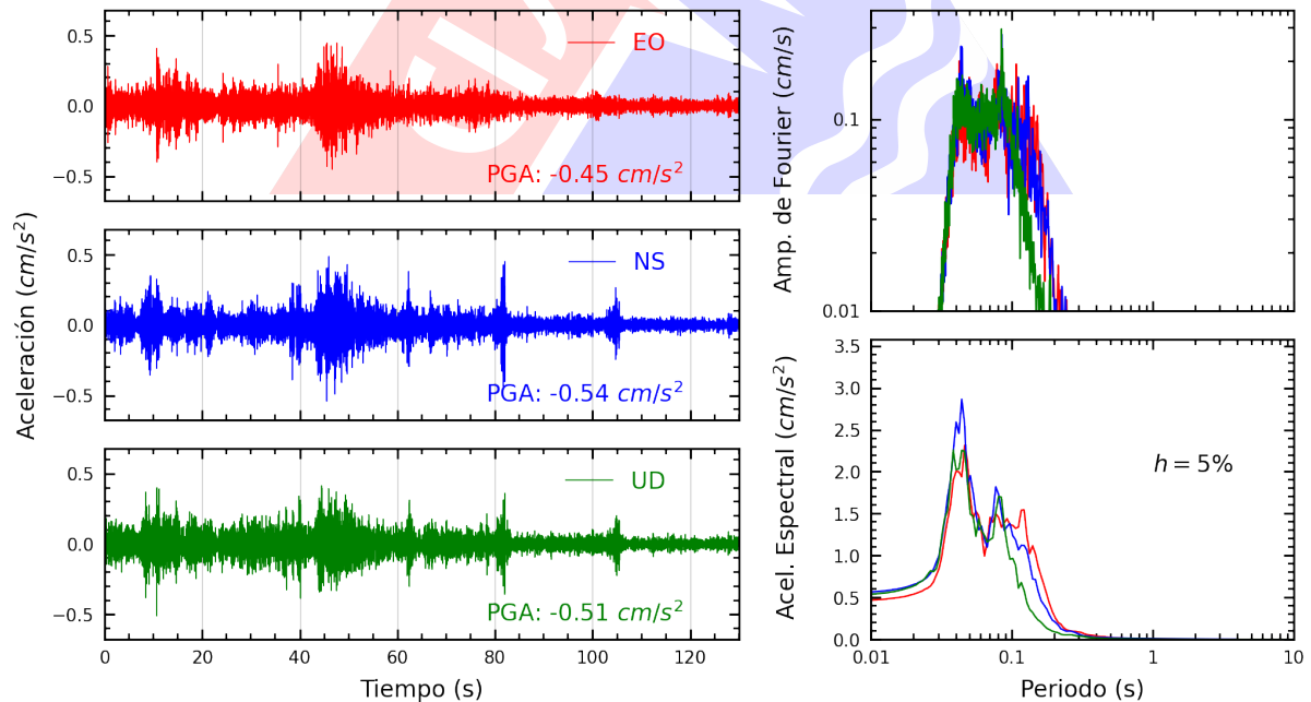
Figura A.8: Registros tiempo-historia, espectros de Fourier y de respuesta en las direcciones EO, NS y vertical de la estación SROS2. Sismo de Matucana, Huarochiri - Lima del 2025-03-23, 22:59:59 (Hora local)
