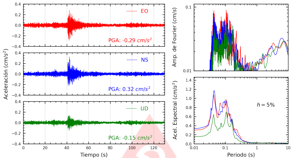
Figura A.17: Registros tiempo-historia, espectros de Fourier y de respuesta en las direcciones EO, NS y vertical de la estación FICPE. Sismo de Matucana, Huarochiri - Lima del 2025-03-23, 22:59:59 (Hora local)
