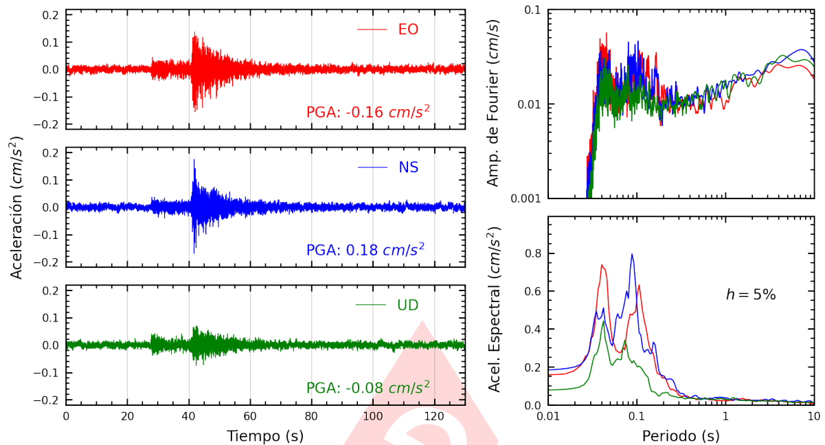
Figura A.27: Registros tiempo-historia, espectros de Fourier y de respuesta en las direcciones EO, NS y vertical de la estación UCSS. Sismo de Matucana, Huarochiri - Lima del 2025-03-23, 22:59:59 (Hora local)
