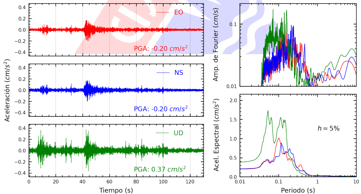
Figura A.14: Registros tiempo-historia, espectros de Fourier y de respuesta en las direcciones EO, NS y vertical de la estación MDPP. Sismo de Matucana, Huarochiri - Lima del 2025-03-23, 22:59:59 (Hora local)
