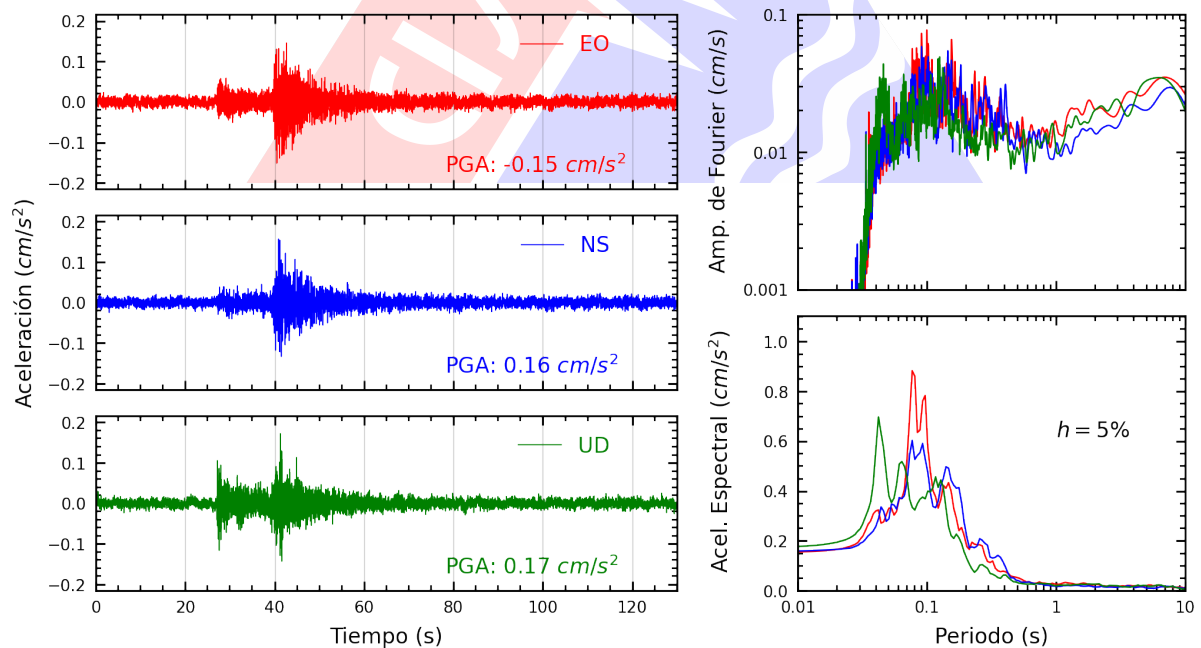
Figura A.28: Registros tiempo-historia, espectros de Fourier y de respuesta en las direcciones EO, NS y vertical de la estación USILP. Sismo de Matucana, Huarochiri - Lima del 2025-03-23, 22:59:59 (Hora local)
