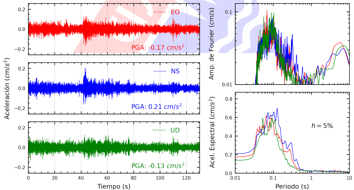
Figura A.24: Registros tiempo-historia, espectros de Fourier y de respuesta en las direcciones EO, NS y vertical de la estación MADRE. Sismo de Matucana, Huarochiri - Lima del 2025-03-23, 22:59:59 (Hora local)
