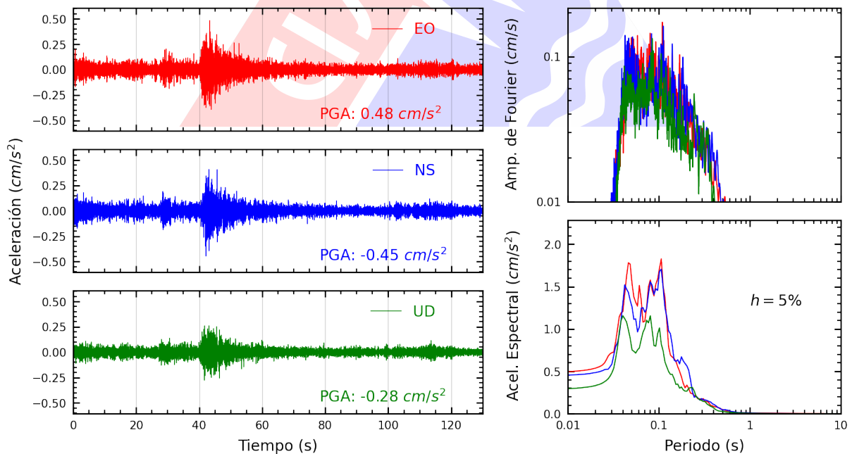
Figura A.10: Registros tiempo-historia, espectros de Fourier y de respuesta en las direcciones EO, NS y vertical de la estación UNTEL. Sismo de Matucana, Huarochiri - Lima del 2025-03-23, 22:59:59 (Hora local)
