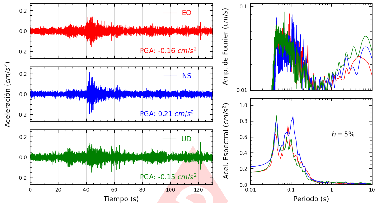
Figura A.21: Registros tiempo-historia, espectros de Fourier y de respuesta en las direcciones EO, NS y vertical de la estación URPE. Sismo de Matucana, Huarochiri - Lima del 2025-03-23, 22:59:59 (Hora local)
