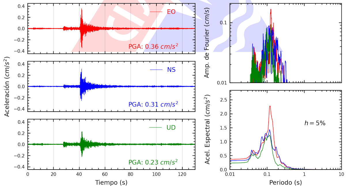
Figura A.16: Registros tiempo-historia, espectros de Fourier y de respuesta en las direcciones EO, NS y vertical de la estación JALV2. Sismo de Matucana, Huarochiri - Lima del 2025-03-23, 22:59:59 (Hora local)
