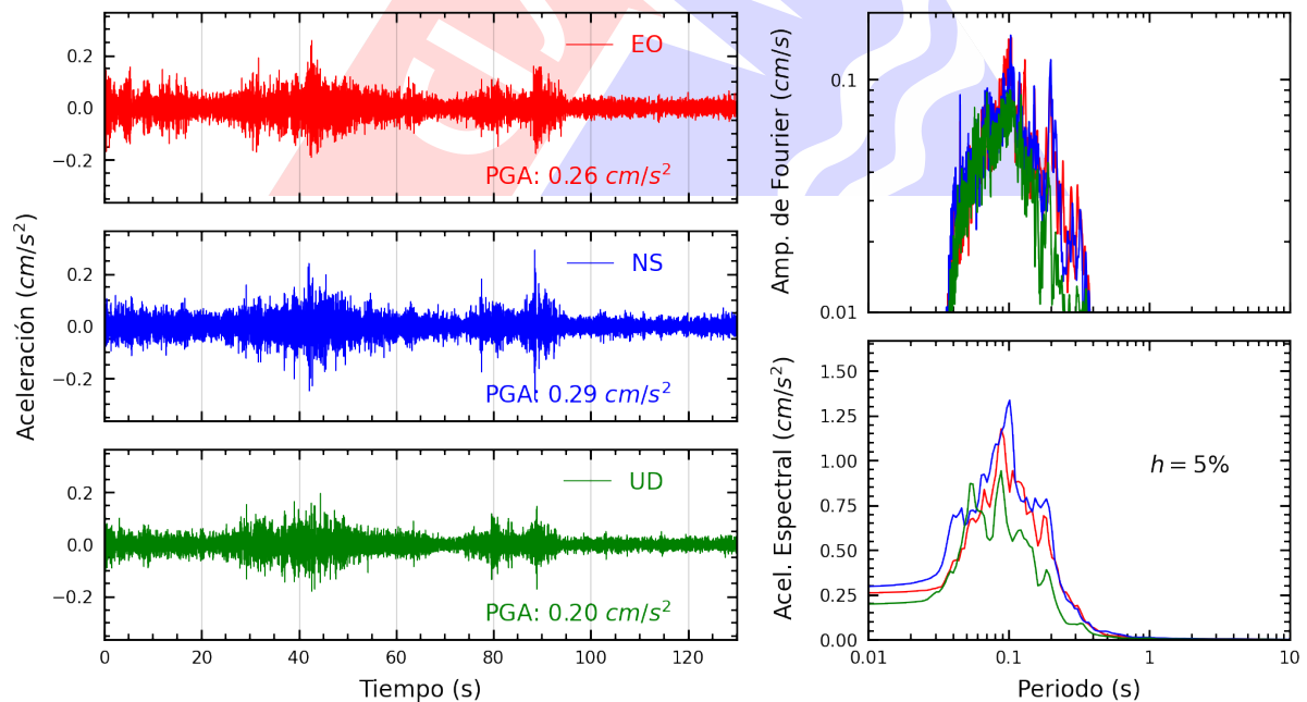
Figura A.18: Registros tiempo-historia, espectros de Fourier y de respuesta en las direcciones EO, NS y vertical de la estación SCCHO. Sismo de Matucana, Huarochiri - Lima del 2025-03-23, 22:59:59 (Hora local)
