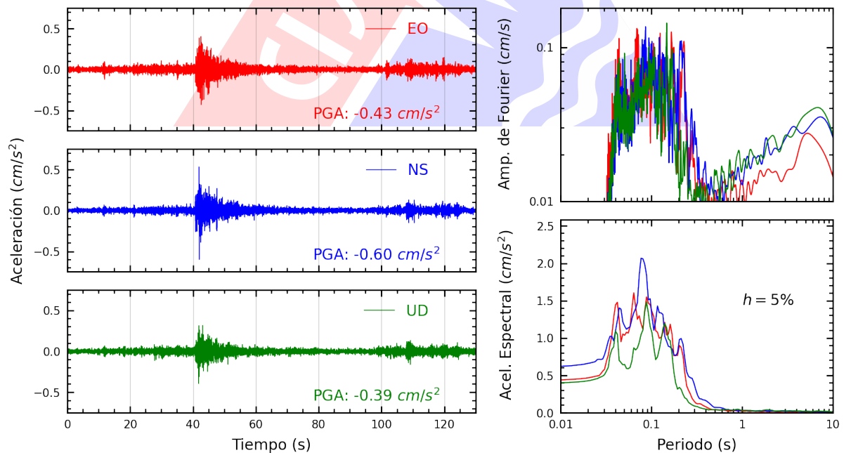
Figura A.6: Registros tiempo-historia, espectros de Fourier y de respuesta en las direcciones EO, NS y vertical de la estación INDEP. Sismo de Matucana, Huarochiri - Lima del 2025-03-23, 22:59:59 (Hora local)
