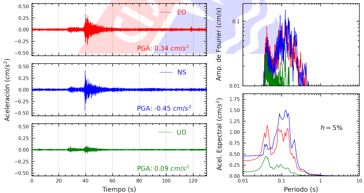
Figura A.12: Registros tiempo-historia, espectros de Fourier y de respuesta en las direcciones EO, NS y vertical de la estación UCVA2. Sismo de Matucana, Huarochiri - Lima del 2025-03-23, 22:59:59 (Hora local)
