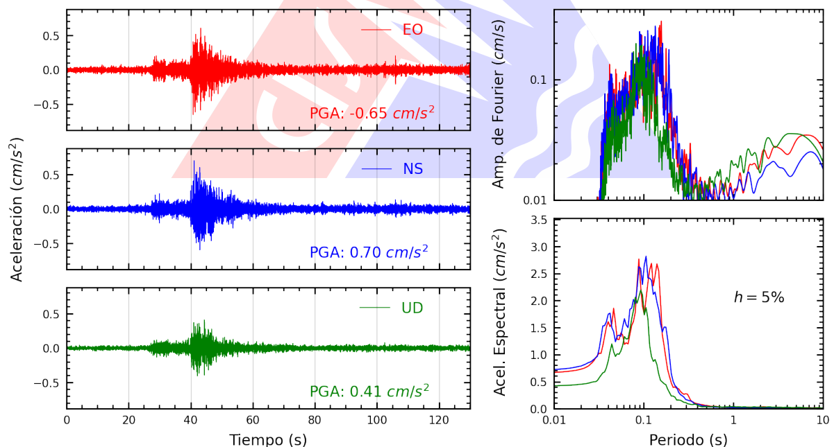
Figura A.2: Registros tiempo-historia, espectros de Fourier y de respuesta en las direcciones EO, NS y vertical de la estación USILM. Sismo de Matucana, Huarochiri - Lima del 2025-03-23, 22:59:59 (Hora local)
