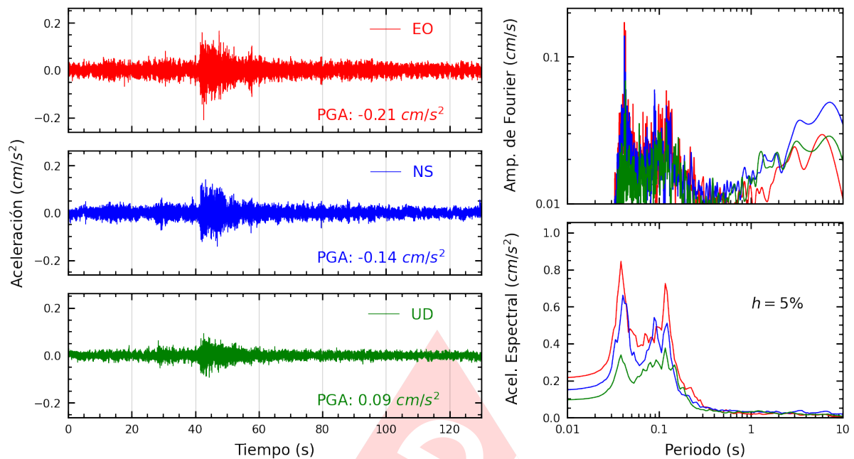
Figura A.23: Registros tiempo-historia, espectros de Fourier y de respuesta en las direcciones EO, NS y vertical de la estación CEPRE. Sismo de Matucana, Huarochiri - Lima del 2025-03-23, 22:59:59 (Hora local)
