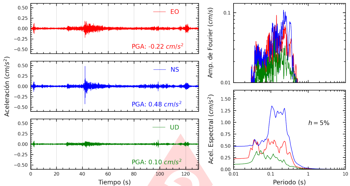
Figura A.11: Registros tiempo-historia, espectros de Fourier y de respuesta en las direcciones EO, NS y vertical de la estación BRIS2. Sismo de Matucana, Huarochiri - Lima del 2025-03-23, 22:59:59 (Hora local)
