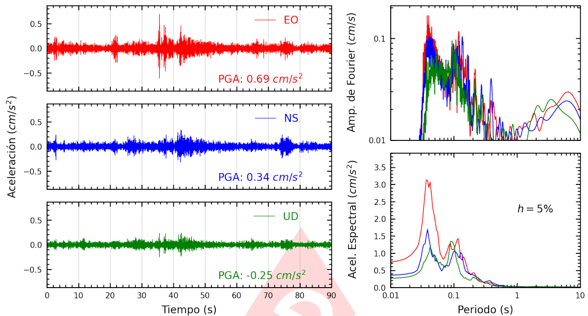
Figura A.3: Registros tiempo-historia, espectros de Fourier y de respuesta en las direcciones EO, NS y vertical de la estación OLIVO. Sismo de Matucana, Huarochiri - Lima del 2025-03-23, 22:59:59 (Hora local)
