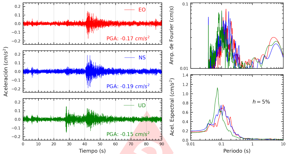
Figura A.25: Registros tiempo-historia, espectros de Fourier y de respuesta en las direcciones EO, NS y vertical de la estación SOCHO. Sismo de Matucana, Huarochiri - Lima del 2025-03-23, 22:59:59 (Hora local)
