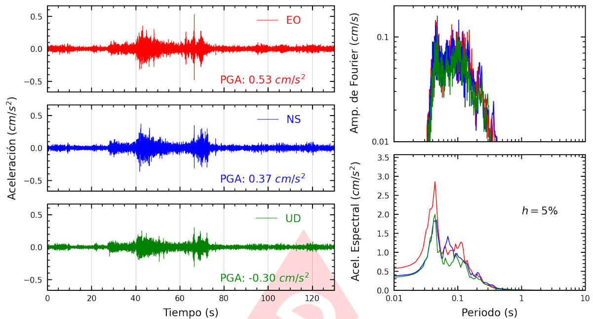
Figura A.9: Registros tiempo-historia, espectros de Fourier y de respuesta en las direcciones EO, NS y vertical de la estación PHER2. Sismo de Matucana, Huarochiri - Lima del 2025-03-23, 22:59:59 (Hora local)
