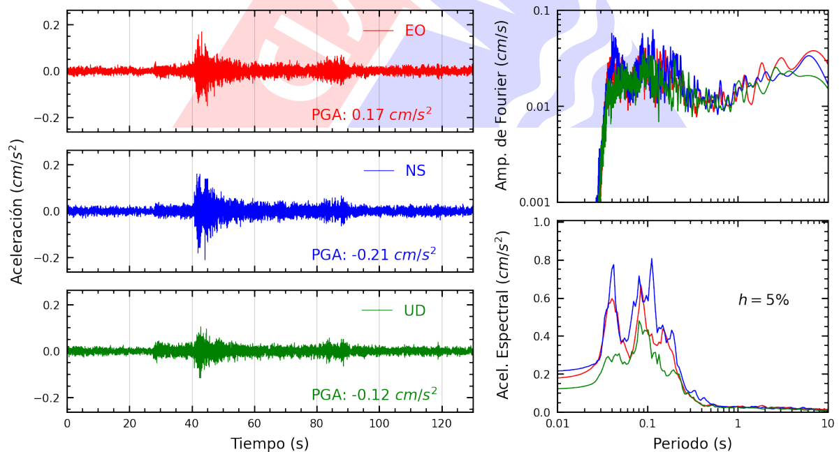
Figura A.22: Registros tiempo-historia, espectros de Fourier y de respuesta en las direcciones EO, NS y vertical de la estación COMAS. Sismo de Matucana, Huarochiri - Lima del 2025-03-23, 22:59:59 (Hora local)
