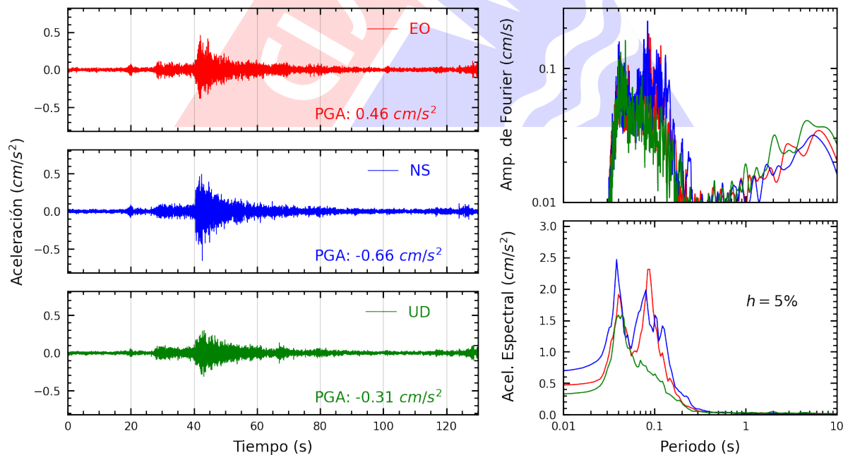
Figura A.4: Registros tiempo-historia, espectros de Fourier y de respuesta en las direcciones EO, NS y vertical de la estación JOSEO. Sismo de Matucana, Huarochiri - Lima del 2025-03-23, 22:59:59 (Hora local)
