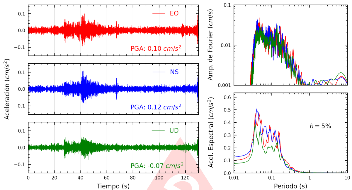
Figura A.33: Registros tiempo-historia, espectros de Fourier y de respuesta en las direcciones EO, NS y vertical de la estación BORJA. Sismo de Matucana, Huarochiri - Lima del 2025-03-23, 22:59:59 (Hora local)
