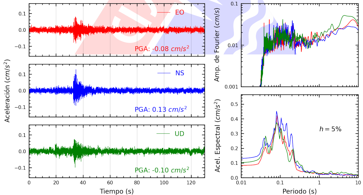
Figura A.30: Registros tiempo-historia, espectros de Fourier y de respuesta en las direcciones EO, NS y vertical de la estación UNMSM. Sismo de Matucana, Huarochiri - Lima del 2025-03-23, 22:59:59 (Hora local)
