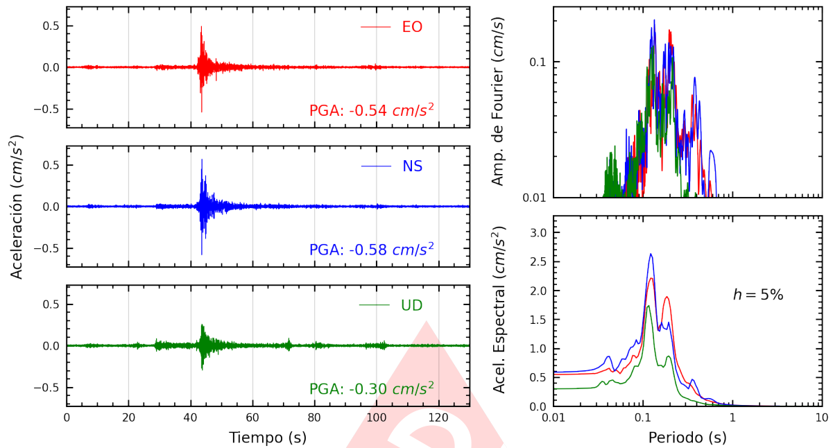
Figura A.7: Registros tiempo-historia, espectros de Fourier y de respuesta en las direcciones EO, NS y vertical de la estación VHAY2. Sismo de Matucana, Huarochiri - Lima del 2025-03-23, 22:59:59 (Hora local)
