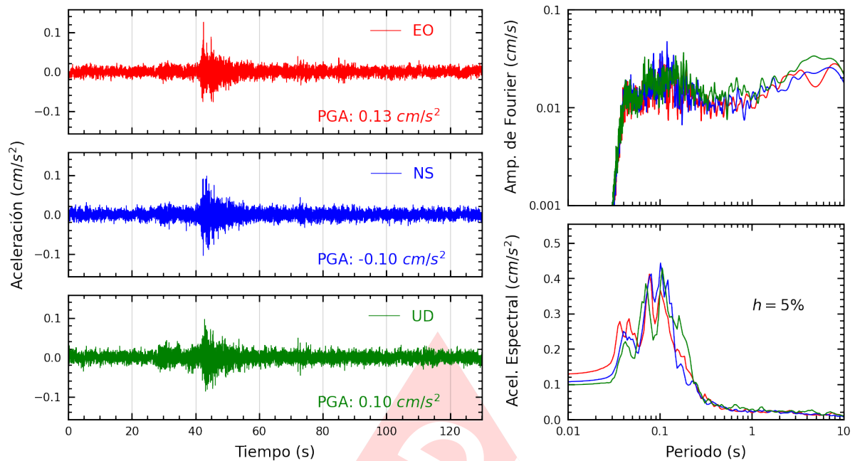
Figura A.31: Registros tiempo-historia, espectros de Fourier y de respuesta en las direcciones EO, NS y vertical de la estación UNFV. Sismo de Matucana, Huarochiri - Lima del 2025-03-23, 22:59:59 (Hora local)
