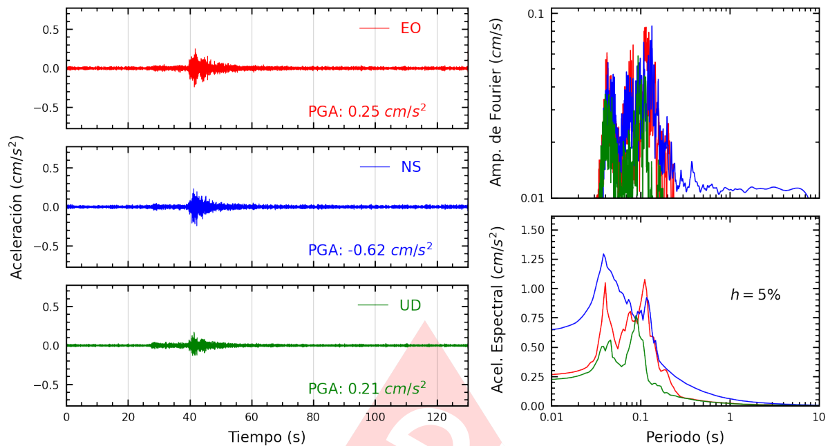
Figura A.5: Registros tiempo-historia, espectros de Fourier y de respuesta en las direcciones EO, NS y vertical de la estación ATARJ. Sismo de Matucana, Huarochiri - Lima del 2025-03-23, 22:59:59 (Hora local)
