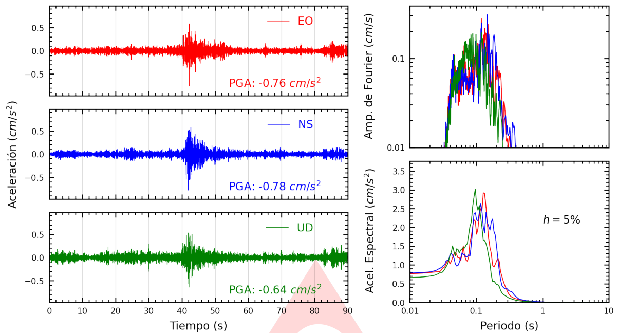
Figura A.1: Registros tiempo-historia, espectros de Fourier y de respuesta en las direcciones EO, NS y vertical de la estación CARA2. Sismo de Matucana, Huarochiri - Lima del 2025-03-23, 22:59:59 (Hora local)
