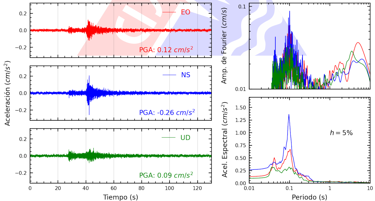
Figura A.20: Registros tiempo-historia, espectros de Fourier y de respuesta en las direcciones EO, NS y vertical de la estación SERVI. Sismo de Matucana, Huarochiri - Lima del 2025-03-23, 22:59:59 (Hora local)
