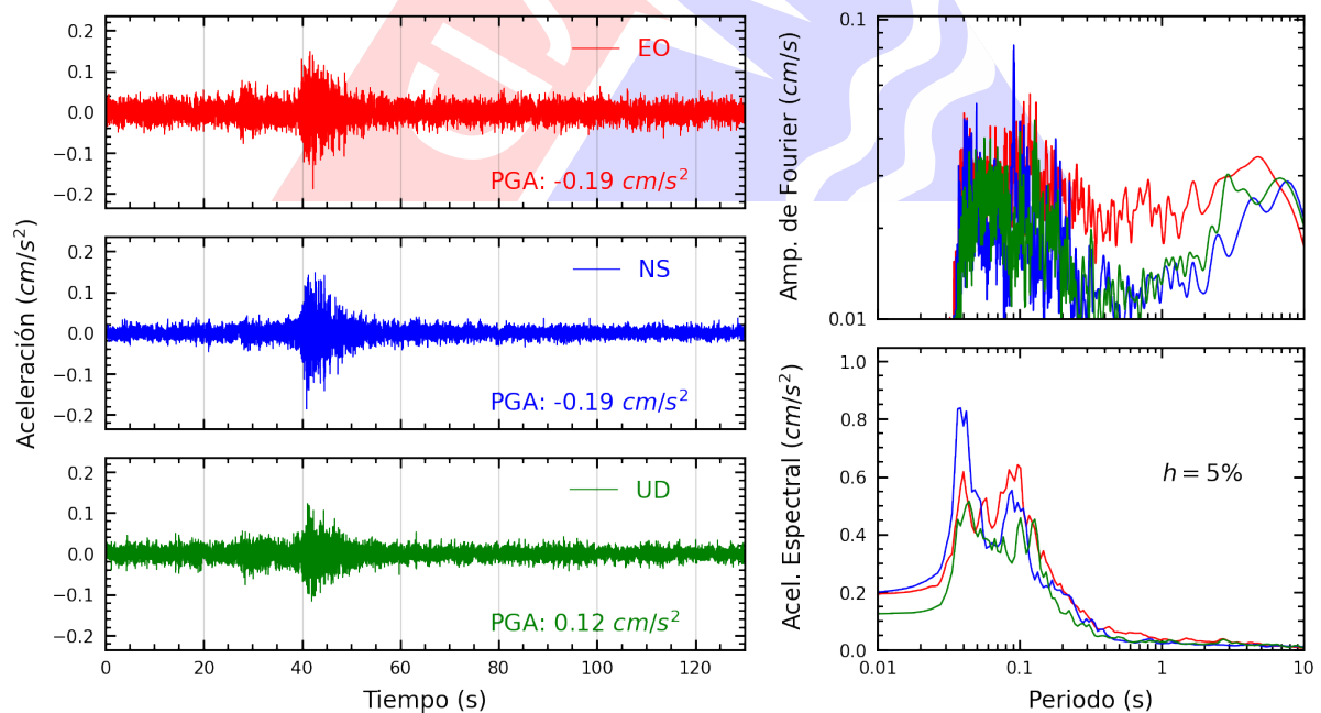
Figura A.26: Registros tiempo-historia, espectros de Fourier y de respuesta en las direcciones EO, NS y vertical de la estación IMCA. Sismo de Matucana, Huarochiri - Lima del 2025-03-23, 22:59:59 (Hora local)
