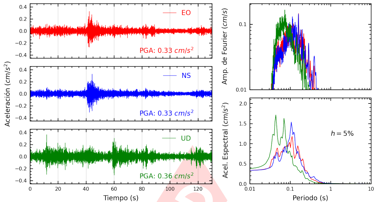
Figura A.15: Registros tiempo-historia, espectros de Fourier y de respuesta en las direcciones EO, NS y vertical de la estación SCOLI. Sismo de Matucana, Huarochiri - Lima del 2025-03-23, 22:59:59 (Hora local)
