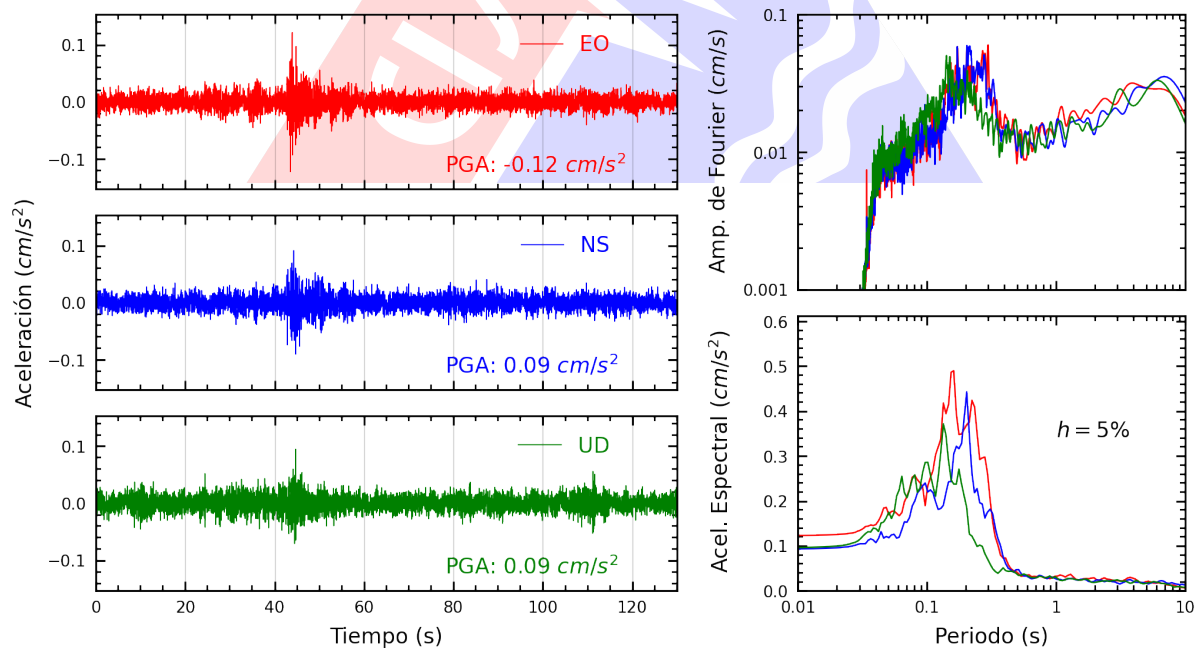
Figura A.32: Registros tiempo-historia, espectros de Fourier y de respuesta en las direcciones EO, NS y vertical de la estación DSMI. Sismo de Matucana, Huarochiri - Lima del 2025-03-23, 22:59:59 (Hora local)
