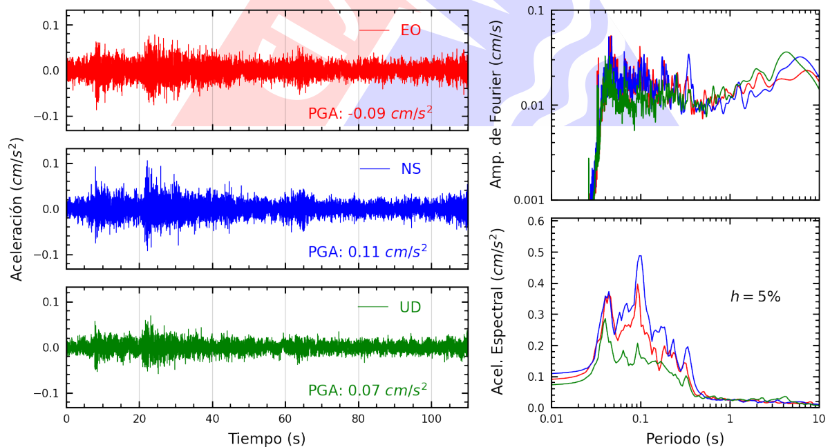
Figura A.34: Registros tiempo-historia, espectros de Fourier y de respuesta en las direcciones EO, NS y vertical de la estación UPCVI. Sismo de Matucana, Huarochiri - Lima del 2025-03-23, 22:59:59 (Hora local)
