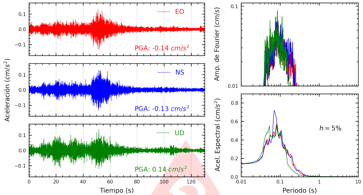
Figura A.29: Registros tiempo-historia, espectros de Fourier y de respuesta en las direcciones EO, NS y vertical de la estación ASIA. Sismo de Matucana, Huarochiri - Lima del 2025-03-23, 22:59:59 (Hora local)
