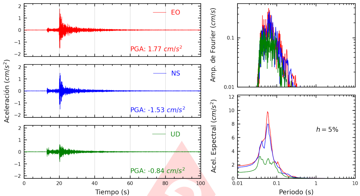
Figura A.13: Registros tiempo-historia, espectros de Fourier y de respuesta en las direcciones EO, NS y vertical de la estación ATARJ. Sismo de Provincia Constitucional del Callao , Callao - Lima del 2025-03-28, 05:45:11 (Hora local)
