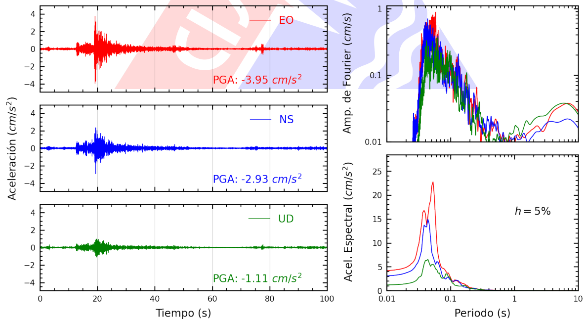
Figura A.6: Registros tiempo-historia, espectros de Fourier y de respuesta en las direcciones EO, NS y vertical de la estación OLIVO. Sismo de Provincia Constitucional del Callao , Callao - Lima del 2025-03-28, 05:45:11 (Hora local)
