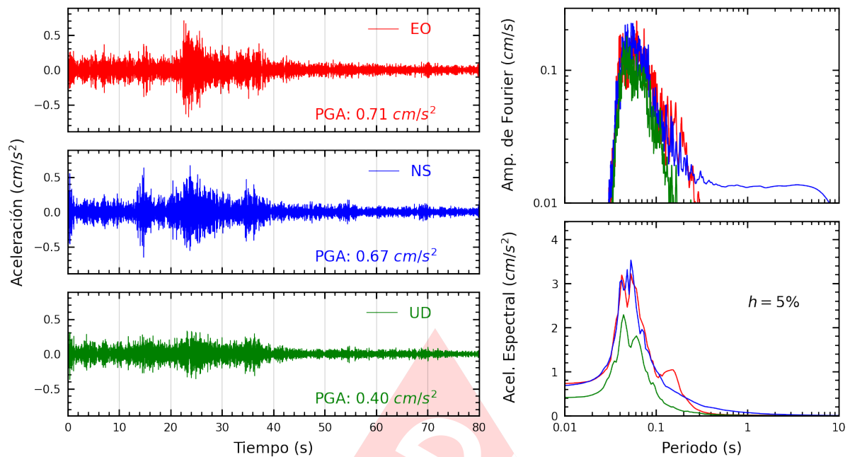
Figura A.29: Registros tiempo-historia, espectros de Fourier y de respuesta en las direcciones EO, NS y vertical de la estación PACHA. Sismo de Provincia Constitucional del Callao , Callao - Lima del 2025-03-28, 05:45:11 (Hora local)
