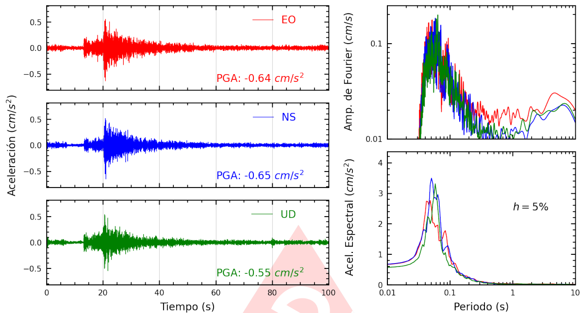
Figura A.31: Registros tiempo-historia, espectros de Fourier y de respuesta en las direcciones EO, NS y vertical de la estación IMCA. Sismo de Provincia Constitucional del Callao , Callao - Lima del 2025-03-28, 05:45:11 (Hora local)
