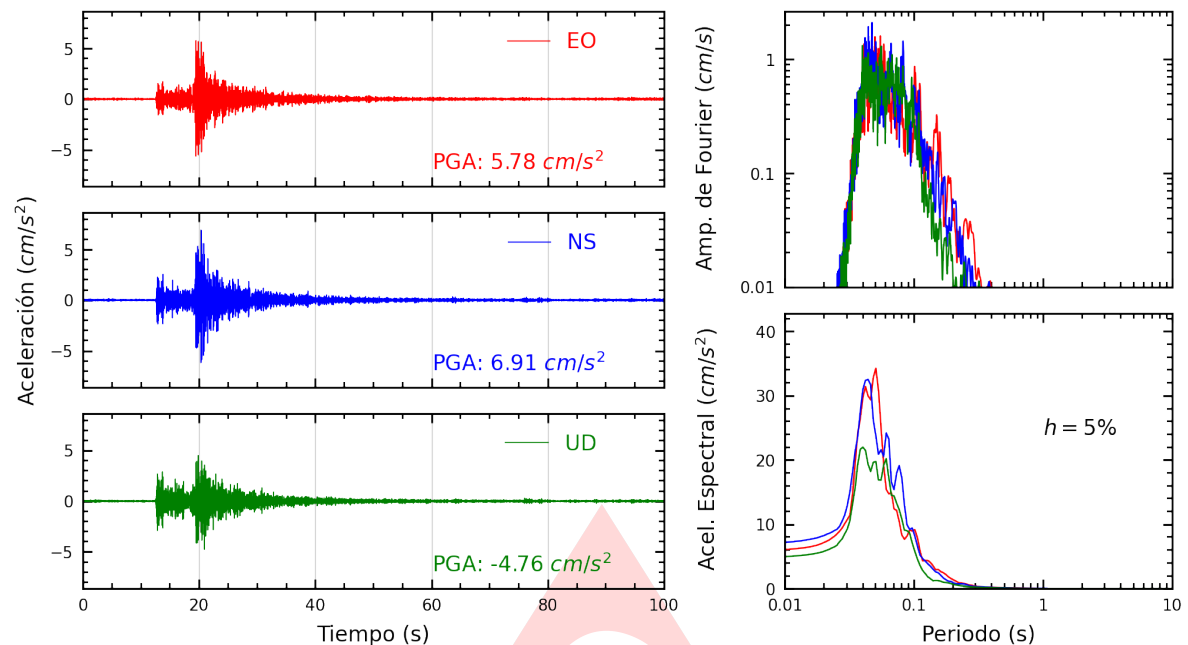
Figura A.1: Registros tiempo-historia, espectros de Fourier y de respuesta en las direcciones EO, NS y vertical de la estación SROS2. Sismo de Provincia Constitucional del Callao , Callao - Lima del 2025-03-28, 05:45:11 (Hora local)
