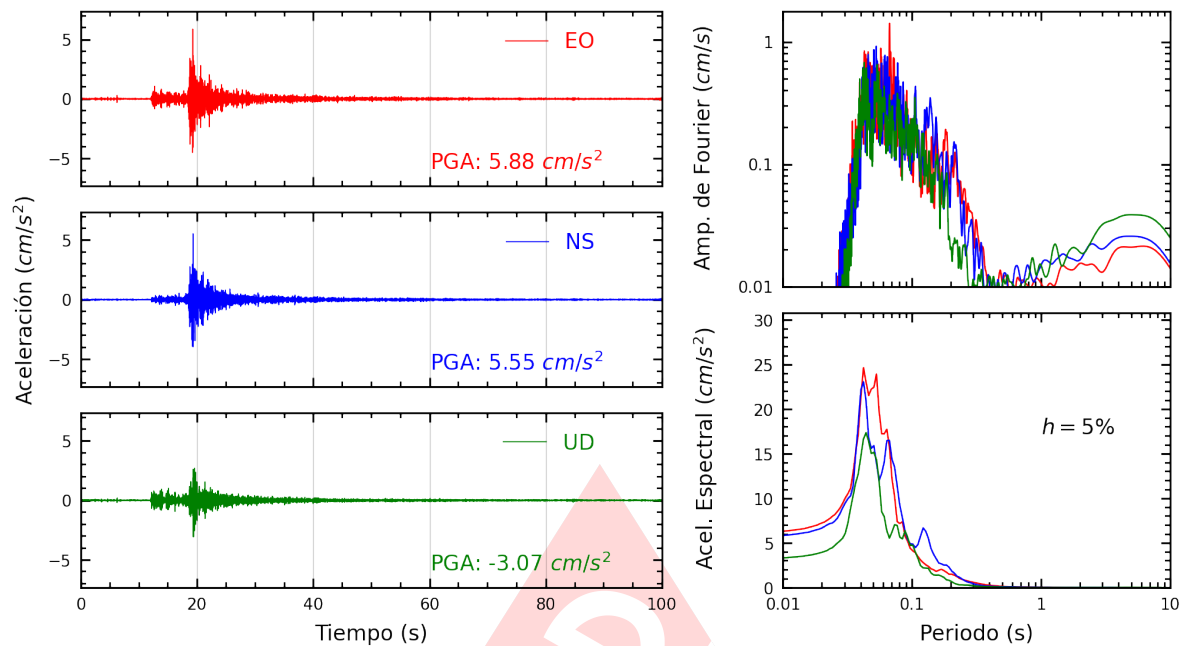
Figura A.3: Registros tiempo-historia, espectros de Fourier y de respuesta en las direcciones EO, NS y vertical de la estación INDEP. Sismo de Provincia Constitucional del Callao , Callao - Lima del 2025-03-28, 05:45:11 (Hora local)
