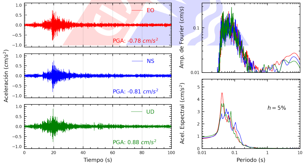
Figura A.24: Registros tiempo-historia, espectros de Fourier y de respuesta en las direcciones EO, NS y vertical de la estación MADRE. Sismo de Provincia Constitucional del Callao , Callao - Lima del 2025-03-28, 05:45:11 (Hora local)
