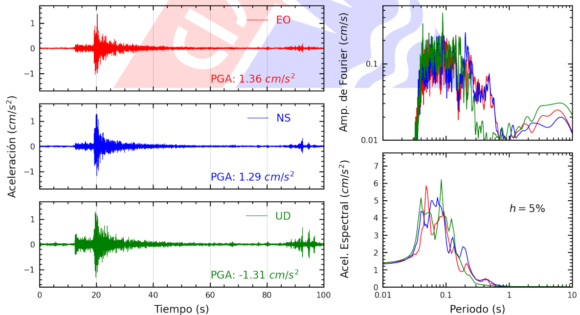
Figura A.18: Registros tiempo-historia, espectros de Fourier y de respuesta en las direcciones EO, NS y vertical de la estación MDPP. Sismo de Provincia Constitucional del Callao , Callao - Lima del 2025-03-28, 05:45:11 (Hora local)
