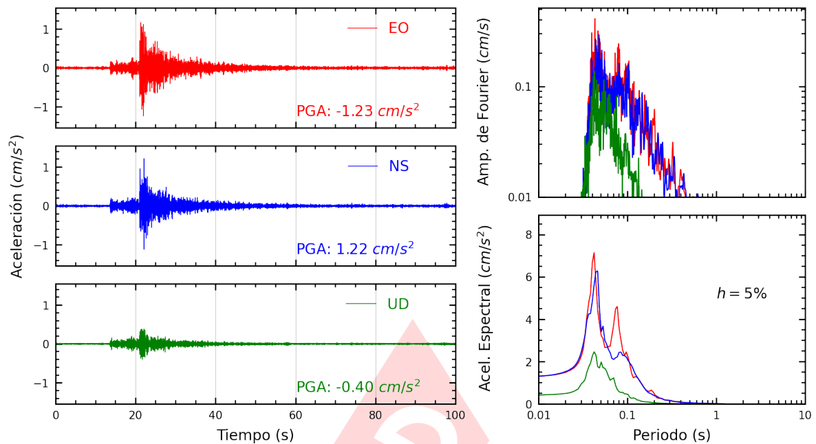
Figura A.19: Registros tiempo-historia, espectros de Fourier y de respuesta en las direcciones EO, NS y vertical de la estación UCVA2. Sismo de Provincia Constitucional del Callao , Callao - Lima del 2025-03-28, 05:45:11 (Hora local)
