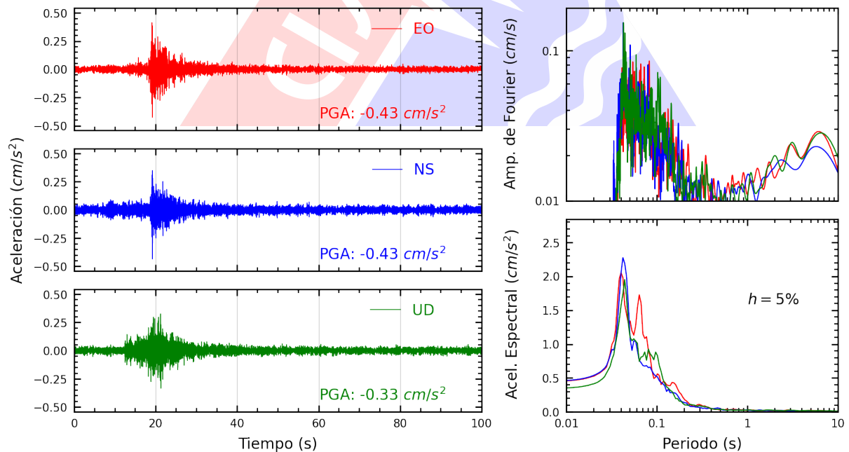
Figura A.34: Registros tiempo-historia, espectros de Fourier y de respuesta en las direcciones EO, NS y vertical de la estación BONDY. Sismo de Provincia Constitucional del Callao , Callao - Lima del 2025-03-28, 05:45:11 (Hora local)
