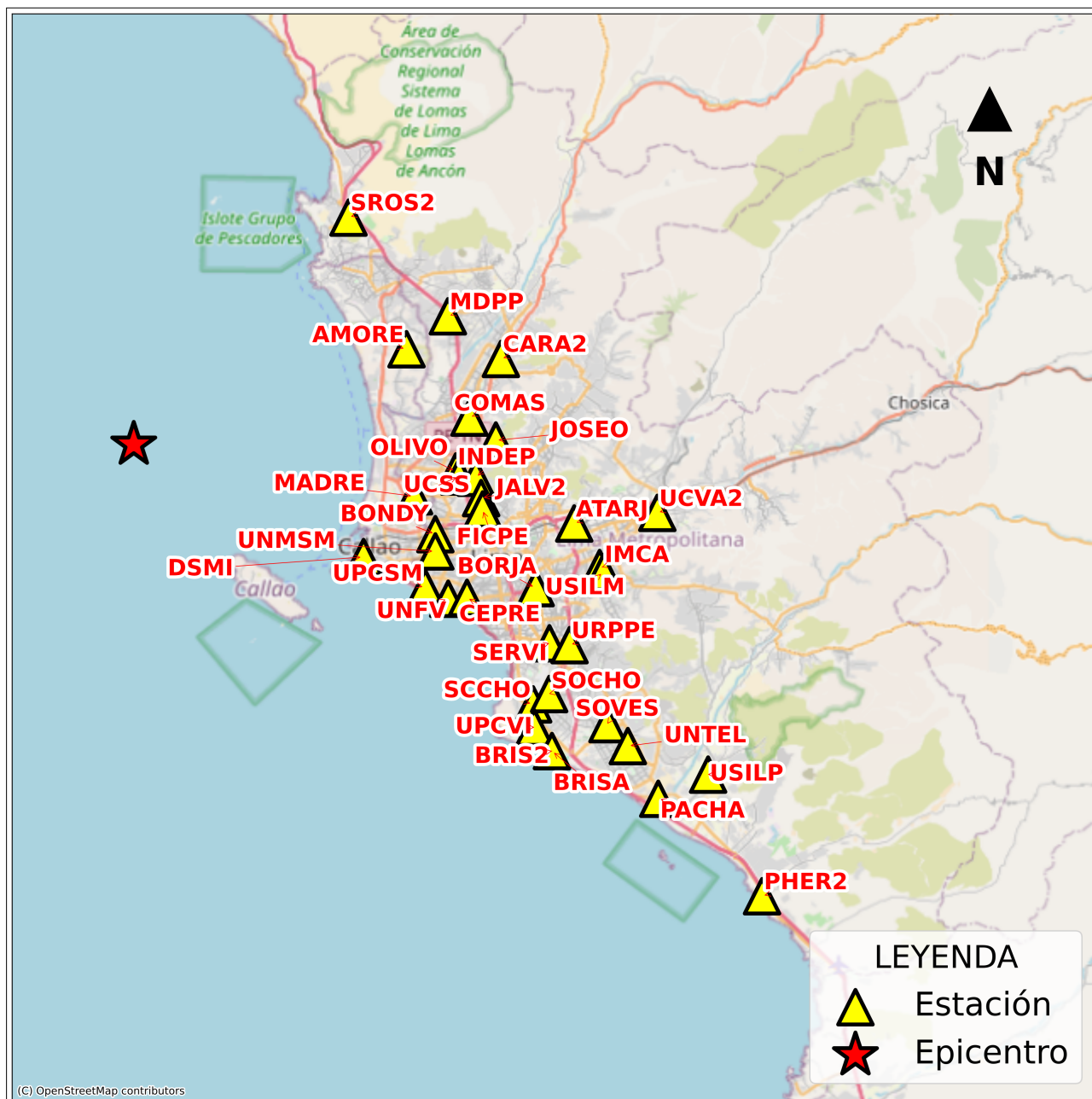
Figura 3: Mapa de ubicación de la(s) estación(es) acelerográfica(s) en Lima Metropolitana correspondiente(s) al Sismo de Provincia Constitucional del Callao , Callao - Lima del 28 de marzo de 2025 a las 05:45:11 (hora local)
