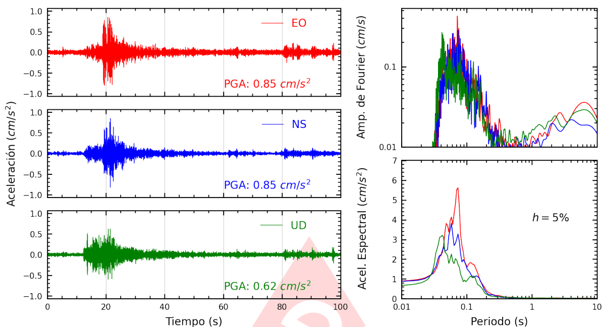
Figura A.27: Registros tiempo-historia, espectros de Fourier y de respuesta en las direcciones EO, NS y vertical de la estación UPCSM. Sismo de Provincia Constitucional del Callao , Callao - Lima del 2025-03-28, 05:45:11 (Hora local)
