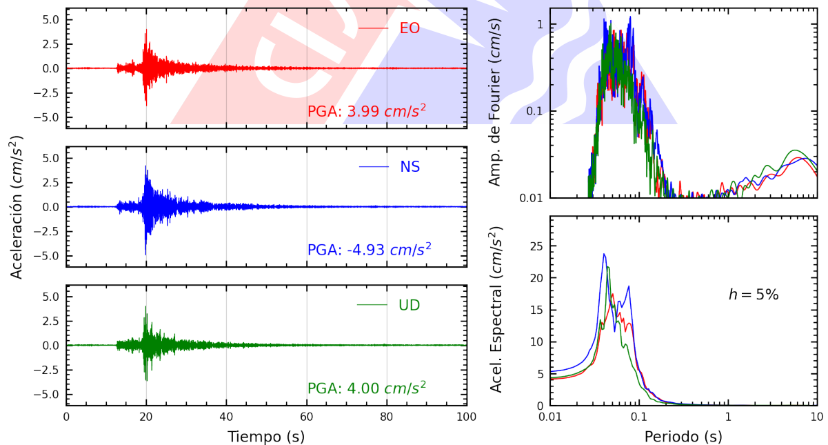
Figura A.4: Registros tiempo-historia, espectros de Fourier y de respuesta en las direcciones EO, NS y vertical de la estación JOSEO. Sismo de Provincia Constitucional del Callao , Callao - Lima del 2025-03-28, 05:45:11 (Hora local)
