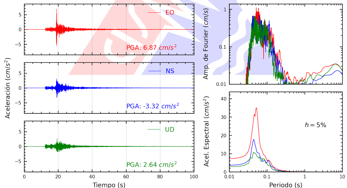
Figura A.2: Registros tiempo-historia, espectros de Fourier y de respuesta en las direcciones EO, NS y vertical de la estación AMORE. Sismo de Provincia Constitucional del Callao , Callao - Lima del 2025-03-28, 05:45:11 (Hora local)
