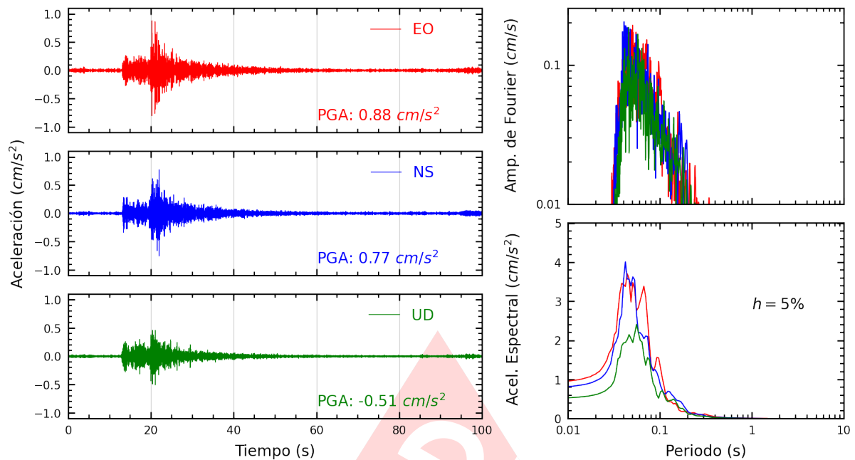
Figura A.25: Registros tiempo-historia, espectros de Fourier y de respuesta en las direcciones EO, NS y vertical de la estación BORJA. Sismo de Provincia Constitucional del Callao , Callao - Lima del 2025-03-28, 05:45:11 (Hora local)
