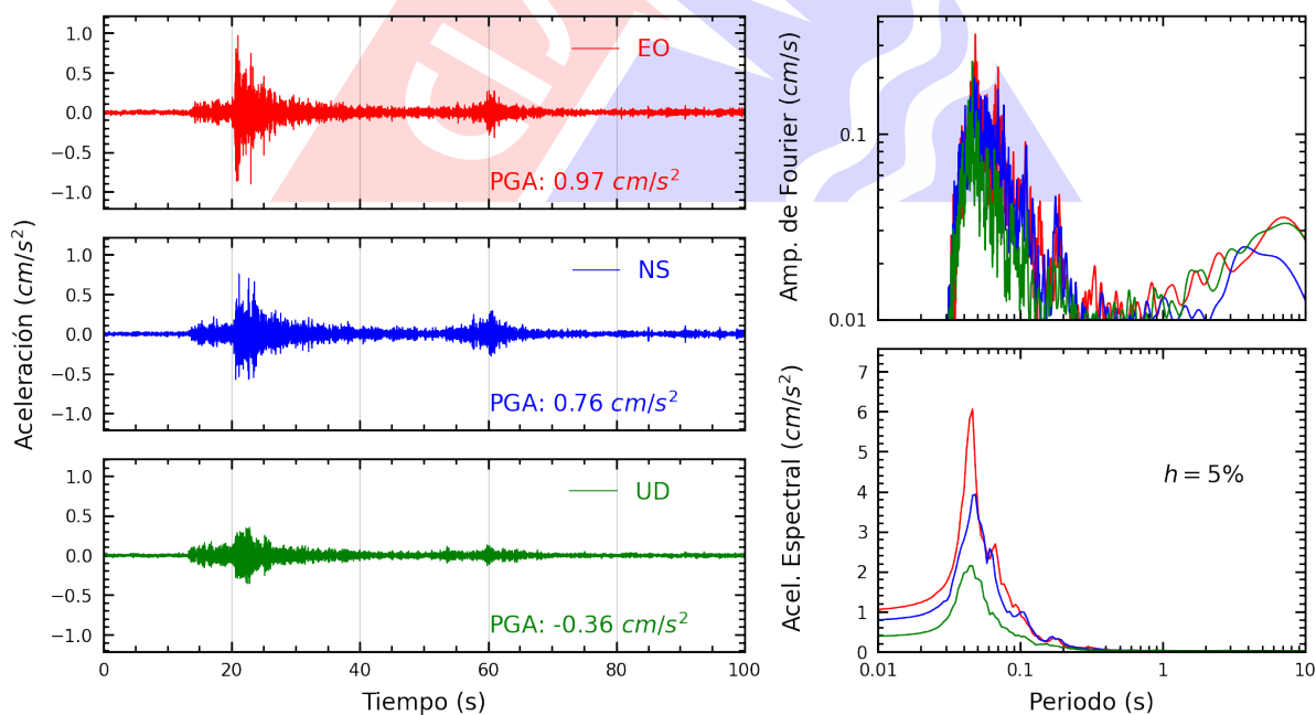
Figura A.22: Registros tiempo-historia, espectros de Fourier y de respuesta en las direcciones EO, NS y vertical de la estación UPCVI. Sismo de Provincia Constitucional del Callao , Callao - Lima del 2025-03-28, 05:45:11 (Hora local)
