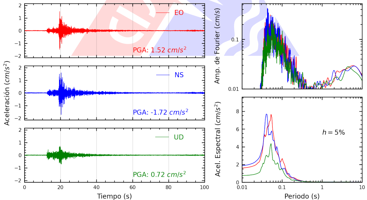
Figura A.14: Registros tiempo-historia, espectros de Fourier y de respuesta en las direcciones EO, NS y vertical de la estación COMAS. Sismo de Provincia Constitucional del Callao , Callao - Lima del 2025-03-28, 05:45:11 (Hora local)
