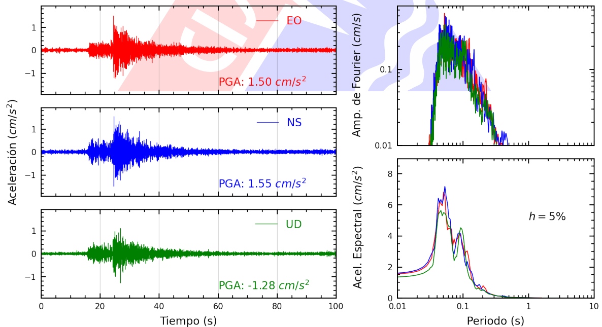
Figura A.16: Registros tiempo-historia, espectros de Fourier y de respuesta en las direcciones EO, NS y vertical de la estación PHER2. Sismo de Provincia Constitucional del Callao , Callao - Lima del 2025-03-28, 05:45:11 (Hora local)
