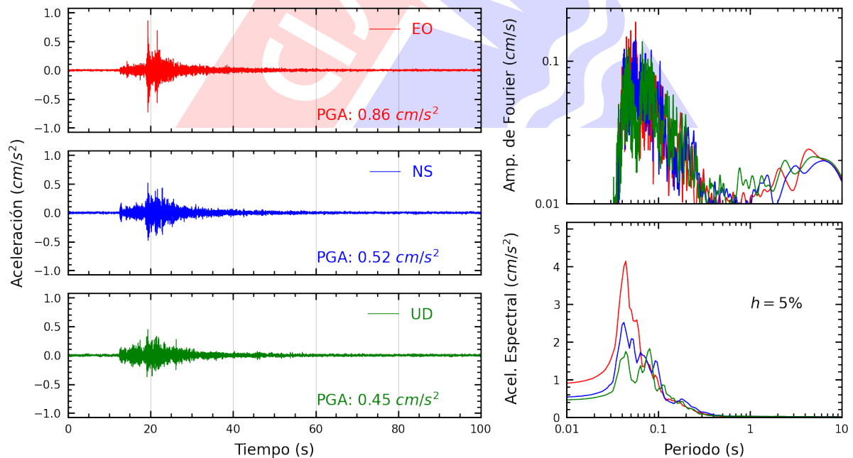
Figura A.26: Registros tiempo-historia, espectros de Fourier y de respuesta en las direcciones EO, NS y vertical de la estación UNFV. Sismo de Provincia Constitucional del Callao , Callao - Lima del 2025-03-28, 05:45:11 (Hora local)
