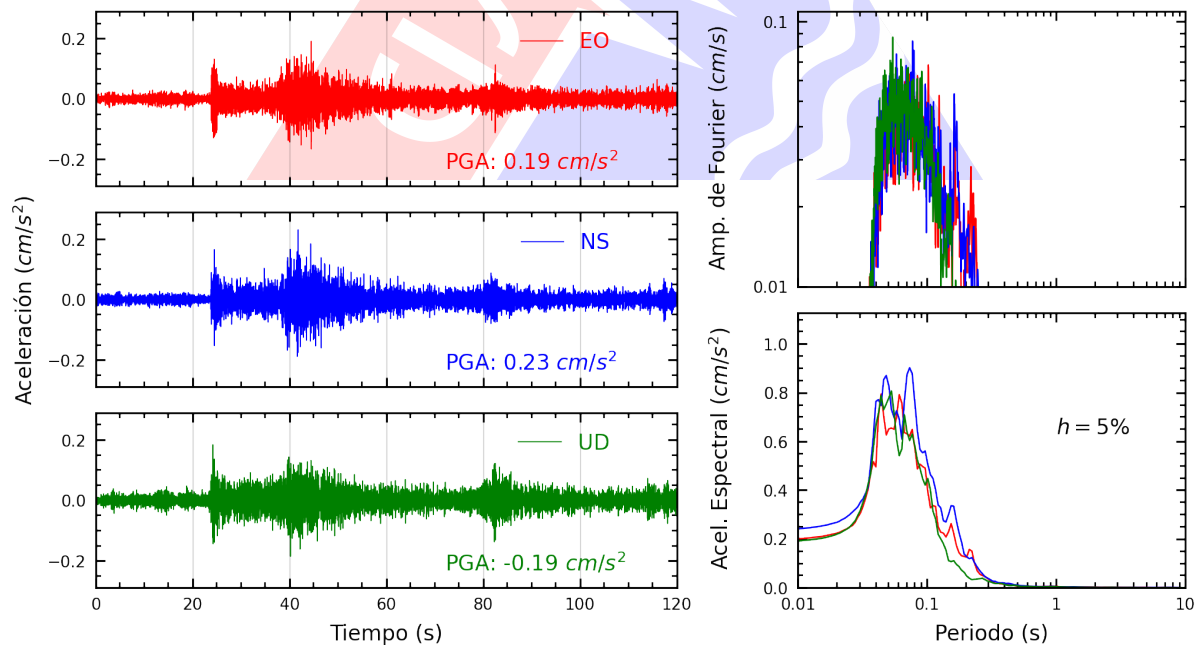
Figura A.36: Registros tiempo-historia, espectros de Fourier y de respuesta en las direcciones EO, NS y vertical de la estación ASIA. Sismo de Provincia Constitucional del Callao , Callao - Lima del 2025-03-28, 05:45:11 (Hora local)
