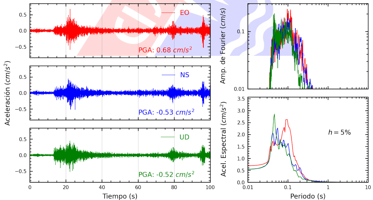
Figura A.30: Registros tiempo-historia, espectros de Fourier y de respuesta en las direcciones EO, NS y vertical de la estación SCCHO. Sismo de Provincia Constitucional del Callao , Callao - Lima del 2025-03-28, 05:45:11 (Hora local)
