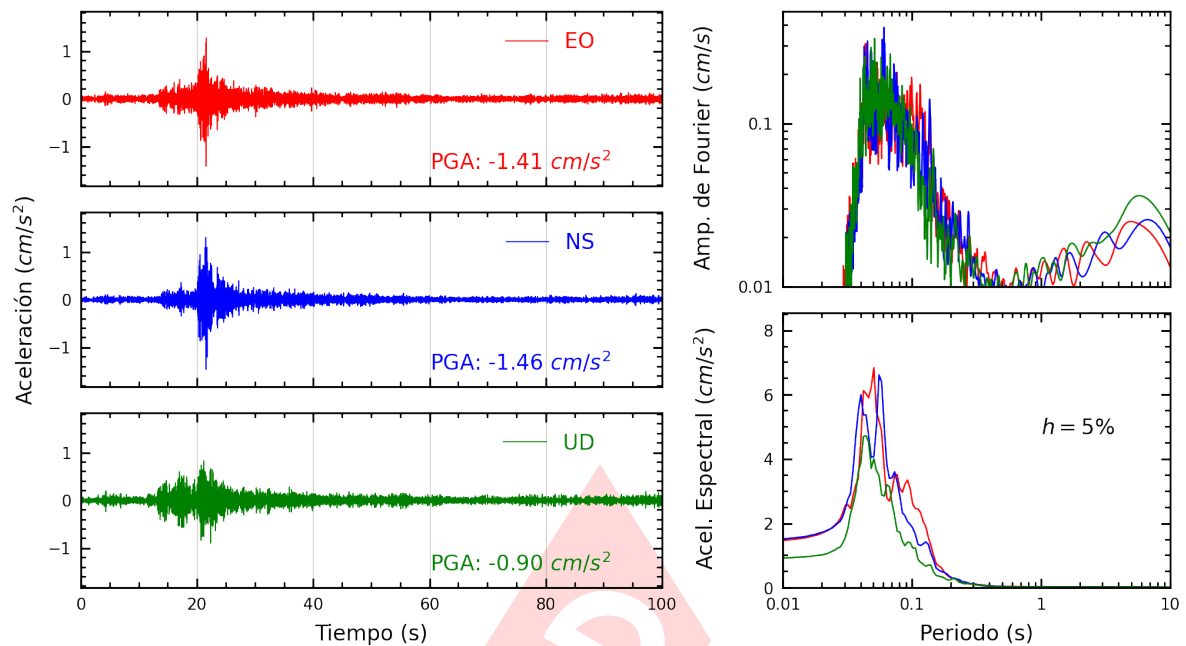
Figura A.17: Registros tiempo-historia, espectros de Fourier y de respuesta en las direcciones EO, NS y vertical de la estación URPE. Sismo de Provincia Constitucional del Callao , Callao - Lima del 2025-03-28, 05:45:11 (Hora local)
