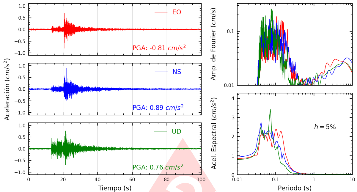
Figura A.23: Registros tiempo-historia, espectros de Fourier y de respuesta en las direcciones EO, NS y vertical de la estación SOCHO. Sismo de Provincia Constitucional del Callao , Callao - Lima del 2025-03-28, 05:45:11 (Hora local)
