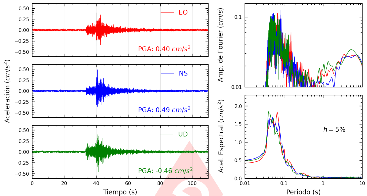
Figura A.33: Registros tiempo-historia, espectros de Fourier y de respuesta en las direcciones EO, NS y vertical de la estación UNMSM. Sismo de Provincia Constitucional del Callao , Callao - Lima del 2025-03-28, 05:45:11 (Hora local)
