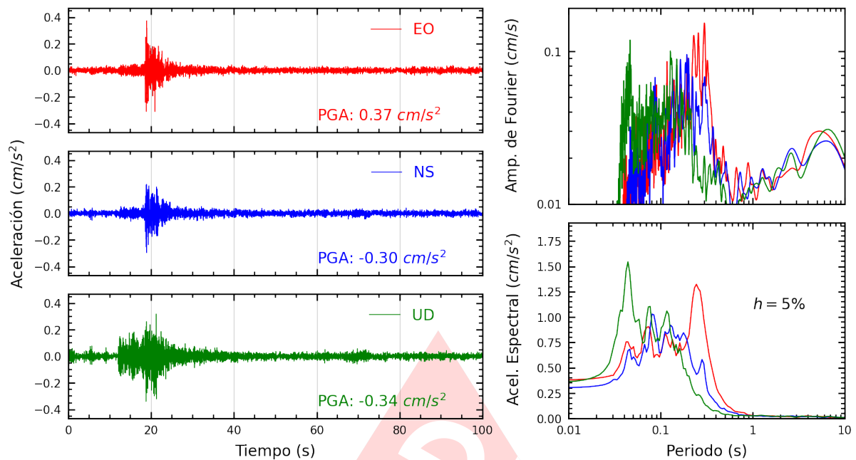
Figura A.35: Registros tiempo-historia, espectros de Fourier y de respuesta en las direcciones EO, NS y vertical de la estación DSML. Sismo de Provincia Constitucional del Callao , Callao - Lima del 2025-03-28, 05:45:11 (Hora local)
