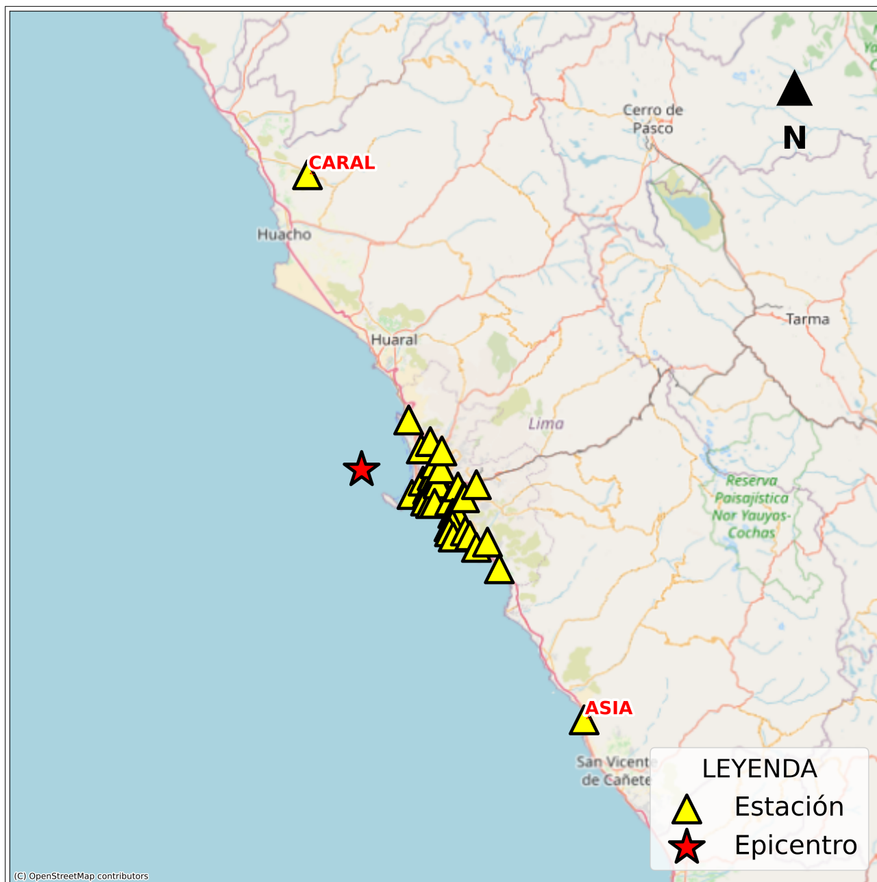
Figura 2: Mapa de ubicación de la(s) estación(es) acelerográfica(s) a nivel nacional correspondiente(s) al Sismo de Provincia Constitucional del Callao , Callao - Lima del 28 de marzo de 2025 a las 05:45:11 (hora local)
