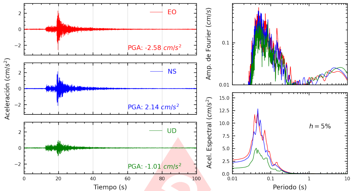
Figura A.9: Registros tiempo-historia, espectros de Fourier y de respuesta en las direcciones EO, NS y vertical de la estación FICPE. Sismo de Provincia Constitucional del Callao , Callao - Lima del 2025-03-28, 05:45:11 (Hora local)
