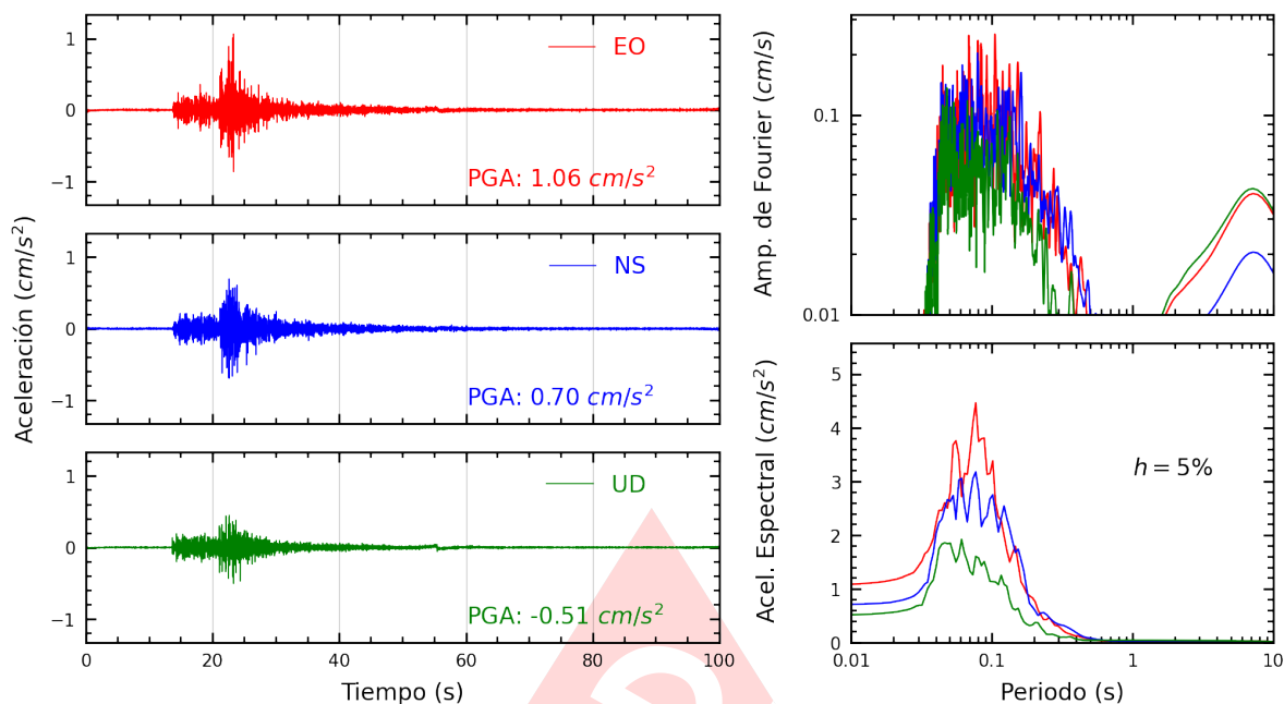
Figura A.21: Registros tiempo-historia, espectros de Fourier y de respuesta en las direcciones EO, NS y vertical de la estación BRISA. Sismo de Provincia Constitucional del Callao , Callao - Lima del 2025-03-28, 05:45:11 (Hora local)
