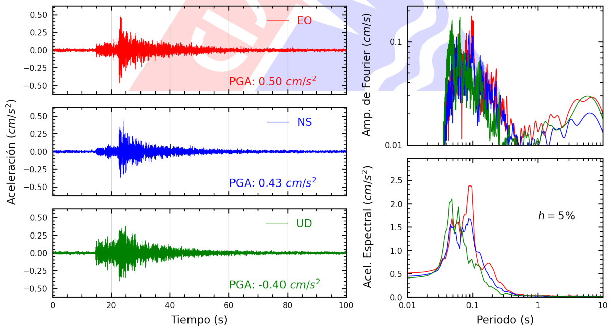
Figura A.32: Registros tiempo-historia, espectros de Fourier y de respuesta en las direcciones EO, NS y vertical de la estación USILP. Sismo de Provincia Constitucional del Callao , Callao - Lima del 2025-03-28, 05:45:11 (Hora local)
