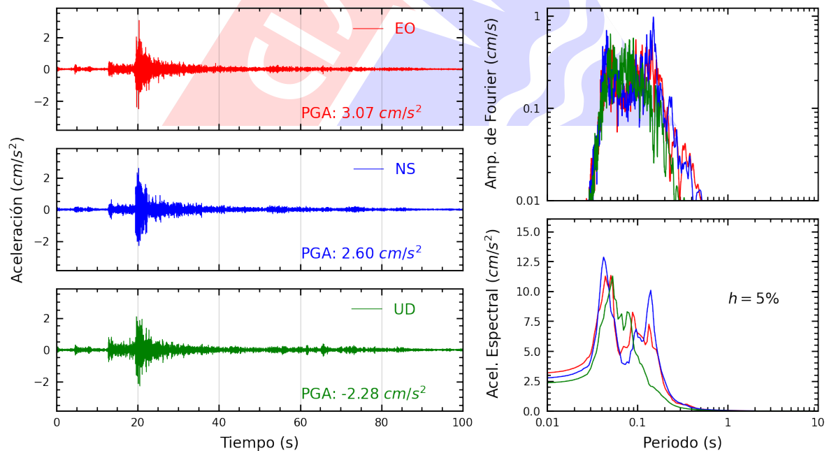
Figura A.8: Registros tiempo-historia, espectros de Fourier y de respuesta en las direcciones EO, NS y vertical de la estación CARA2. Sismo de Provincia Constitucional del Callao , Callao - Lima del 2025-03-28, 05:45:11 (Hora local)
