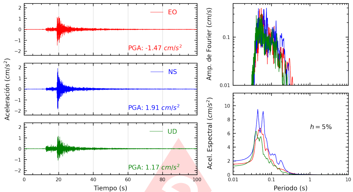
Figura A.11: Registros tiempo-historia, espectros de Fourier y de respuesta en las direcciones EO, NS y vertical de la estación JALV2. Sismo de Provincia Constitucional del Callao , Callao - Lima del 2025-03-28, 05:45:11 (Hora local)
