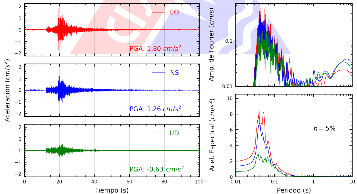
Figura A.12: Registros tiempo-historia, espectros de Fourier y de respuesta en las direcciones EO, NS y vertical de la estación CEPRE. Sismo de Provincia Constitucional del Callao , Callao - Lima del 2025-03-28, 05:45:11 (Hora local)
