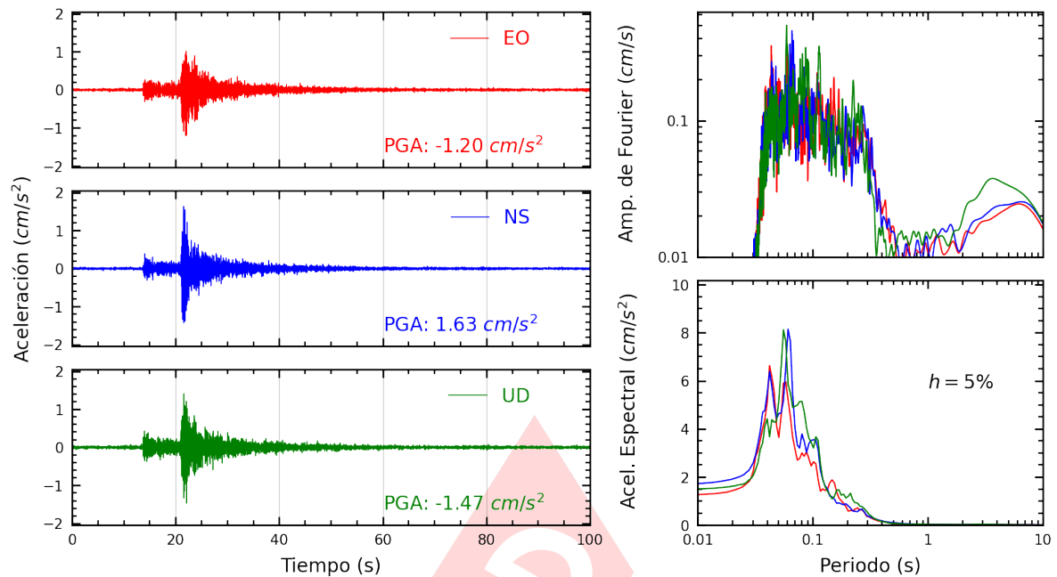
Figura A.15: Registros tiempo-historia, espectros de Fourier y de respuesta en las direcciones EO, NS y vertical de la estación SOVES. Sismo de Provincia Constitucional del Callao , Callao - Lima del 2025-03-28, 05:45:11 (Hora local)
