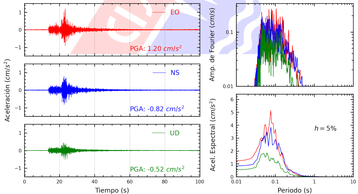
Figura A.20: Registros tiempo-historia, espectros de Fourier y de respuesta en las direcciones EO, NS y vertical de la estación BRIS2. Sismo de Provincia Constitucional del Callao , Callao - Lima del 2025-03-28, 05:45:11 (Hora local)
