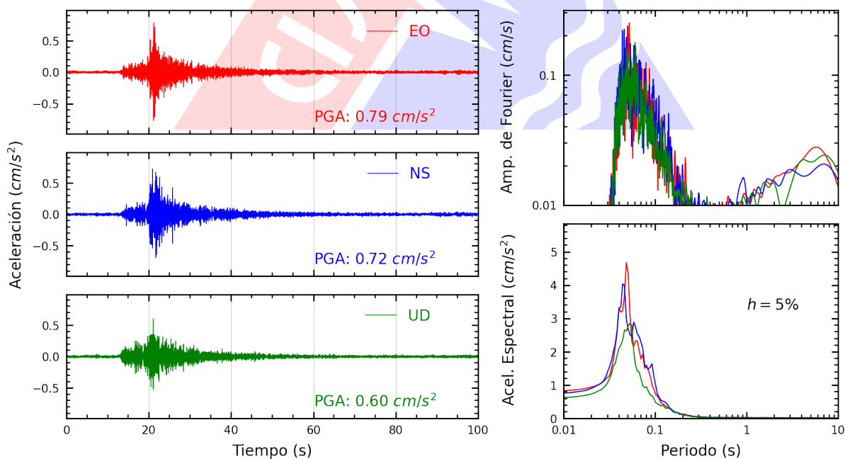
Figura A.28: Registros tiempo-historia, espectros de Fourier y de respuesta en las direcciones EO, NS y vertical de la estación SERVI. Sismo de Provincia Constitucional del Callao , Callao - Lima del 2025-03-28, 05:45:11 (Hora local)
