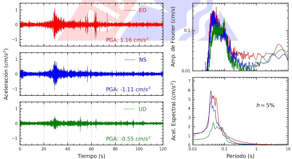
Figura A.10: Registros tiempo-historia, espectros de Fourier y de respuesta en las direcciones EO, NS y vertical de la estación OLIVO. Sismo de Lima, Lima - Lima del 2025-03-28, 06:24:27 (Hora local)
