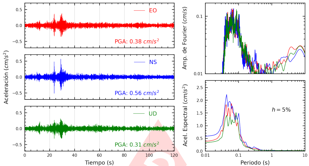
Figura A.17: Registros tiempo-historia, espectros de Fourier y de respuesta en las direcciones EO, NS y vertical de la estación MADRE. Sismo de Lima, Lima - Lima del 2025-03-28, 06:24:27 (Hora local)
