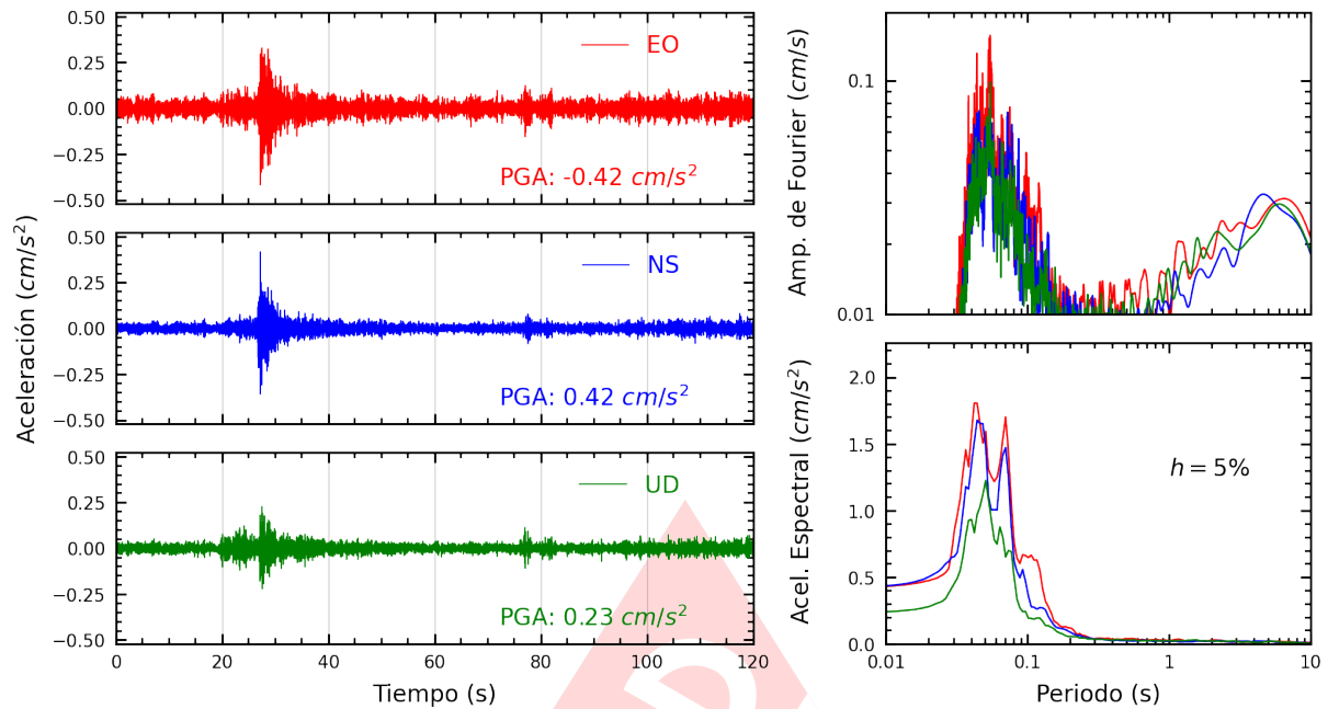
Figura A.25: Registros tiempo-historia, espectros de Fourier y de respuesta en las direcciones EO, NS y vertical de la estación INICT. Sismo de Lima, Lima - Lima del 2025-03-28, 06:24:27 (Hora local)
