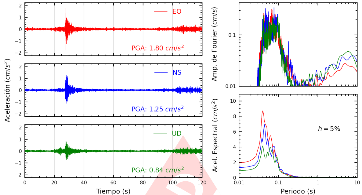
Figura A.5: Registros tiempo-historia, espectros de Fourier y de respuesta en las direcciones EO, NS y vertical de la estación INDEP. Sismo de Lima, Lima - Lima del 2025-03-28, 06:24:27 (Hora local)
