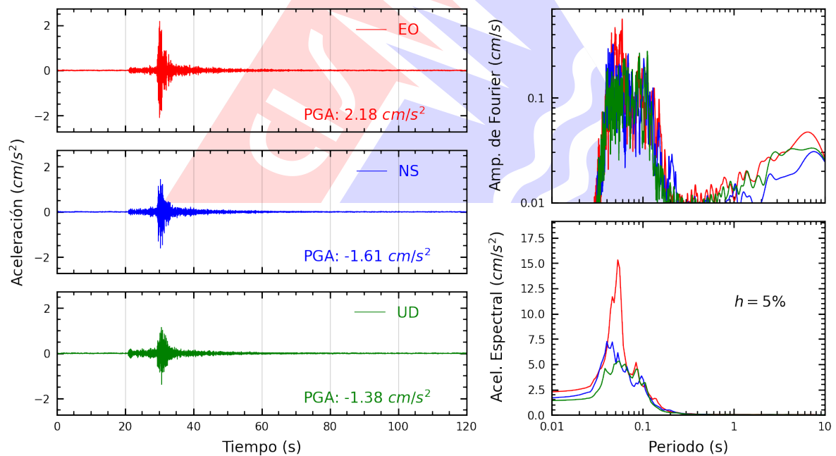
Figura A.2: Registros tiempo-historia, espectros de Fourier y de respuesta en las direcciones EO, NS y vertical de la estación AMORE. Sismo de Lima, Lima - Lima del 2025-03-28, 06:24:27 (Hora local)
