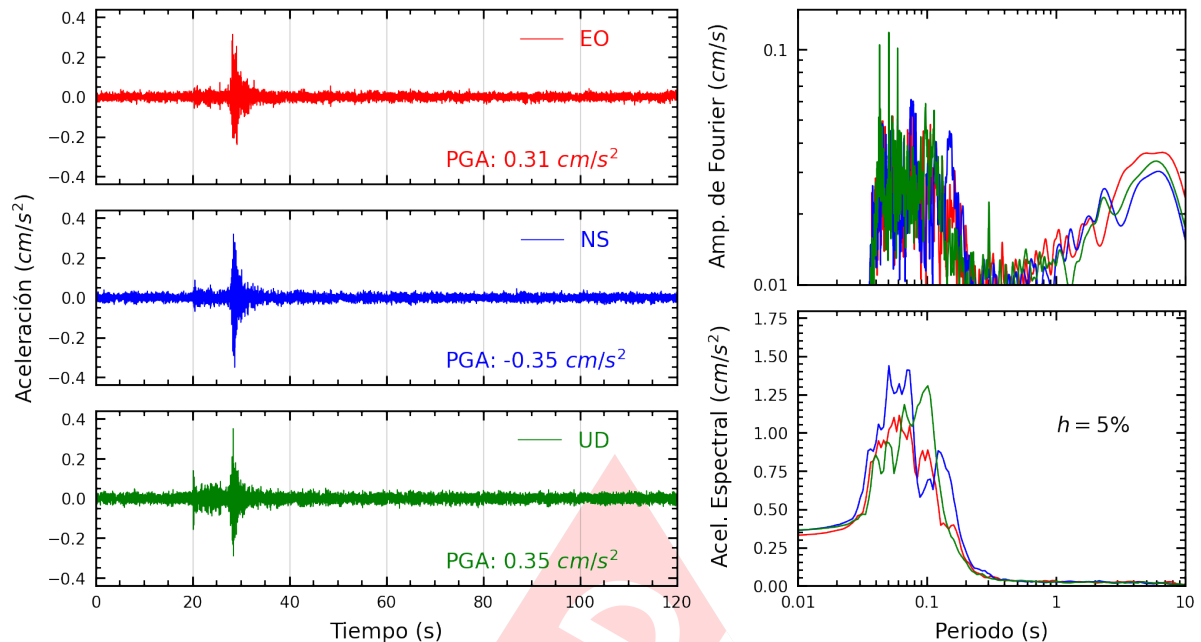
Figura A.31: Registros tiempo-historia, espectros de Fourier y de respuesta en las direcciones EO, NS y vertical de la estación BONDY. Sismo de Lima, Lima - Lima del 2025-03-28, 06:24:27 (Hora local)
