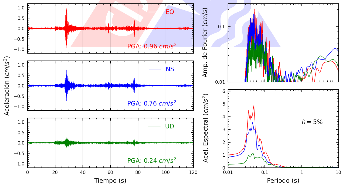
Figura A.12: Registros tiempo-historia, espectros de Fourier y de respuesta en las direcciones EO, NS y vertical de la estación CEPRE. Sismo de Lima, Lima - Lima del 2025-03-28, 06:24:27 (Hora local)
