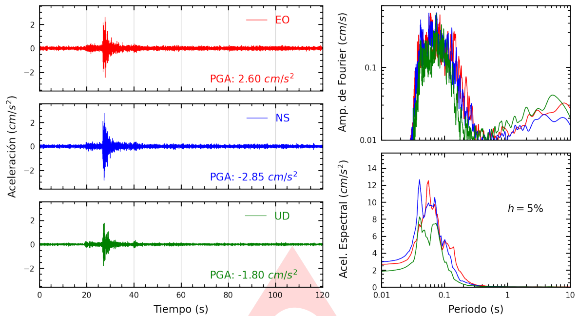
Figura A.1: Registros tiempo-historia, espectros de Fourier y de respuesta en las direcciones EO, NS y vertical de la estación USILM. Sismo de Lima, Lima - Lima del 2025-03-28, 06:24:27 (Hora local)
