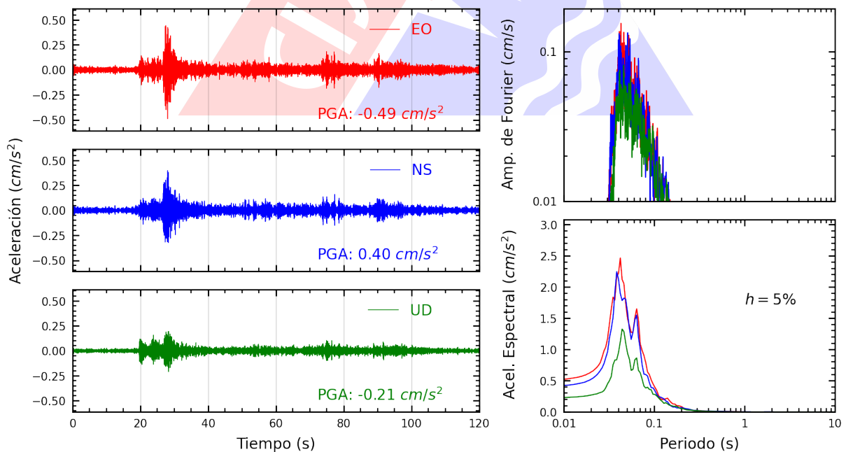
Figura A.22: Registros tiempo-historia, espectros de Fourier y de respuesta en las direcciones EO, NS y vertical de la estación BORJA. Sismo de Lima, Lima - Lima del 2025-03-28, 06:24:27 (Hora local)
