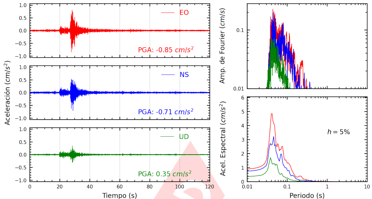
Figura A.13: Registros tiempo-historia, espectros de Fourier y de respuesta en las direcciones EO, NS y vertical de la estación UCVA2. Sismo de Lima, Lima - Lima del 2025-03-28, 06:24:27 (Hora local)
