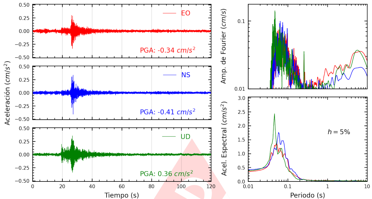
Figura A.27: Registros tiempo-historia, espectros de Fourier y de respuesta en las direcciones EO, NS y vertical de la estación USILP. Sismo de Lima, Lima - Lima del 2025-03-28, 06:24:27 (Hora local)
