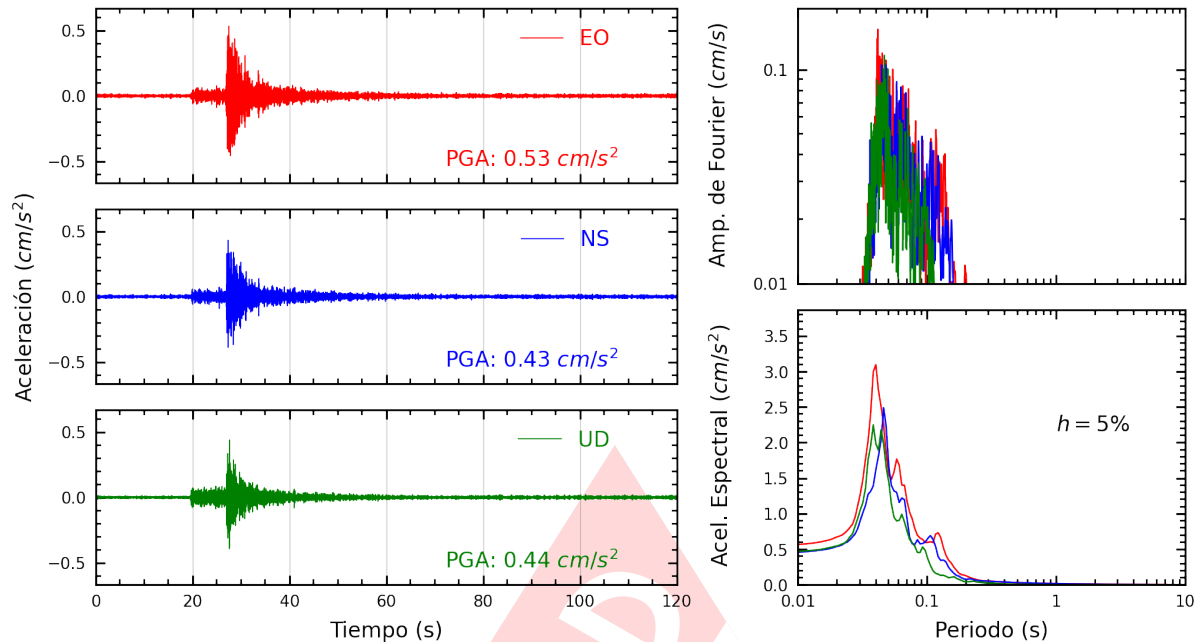
Figura A.19: Registros tiempo-historia, espectros de Fourier y de respuesta en las direcciones EO, NS y vertical de la estación ATARJ. Sismo de Lima, Lima - Lima del 2025-03-28, 06:24:27 (Hora local)
