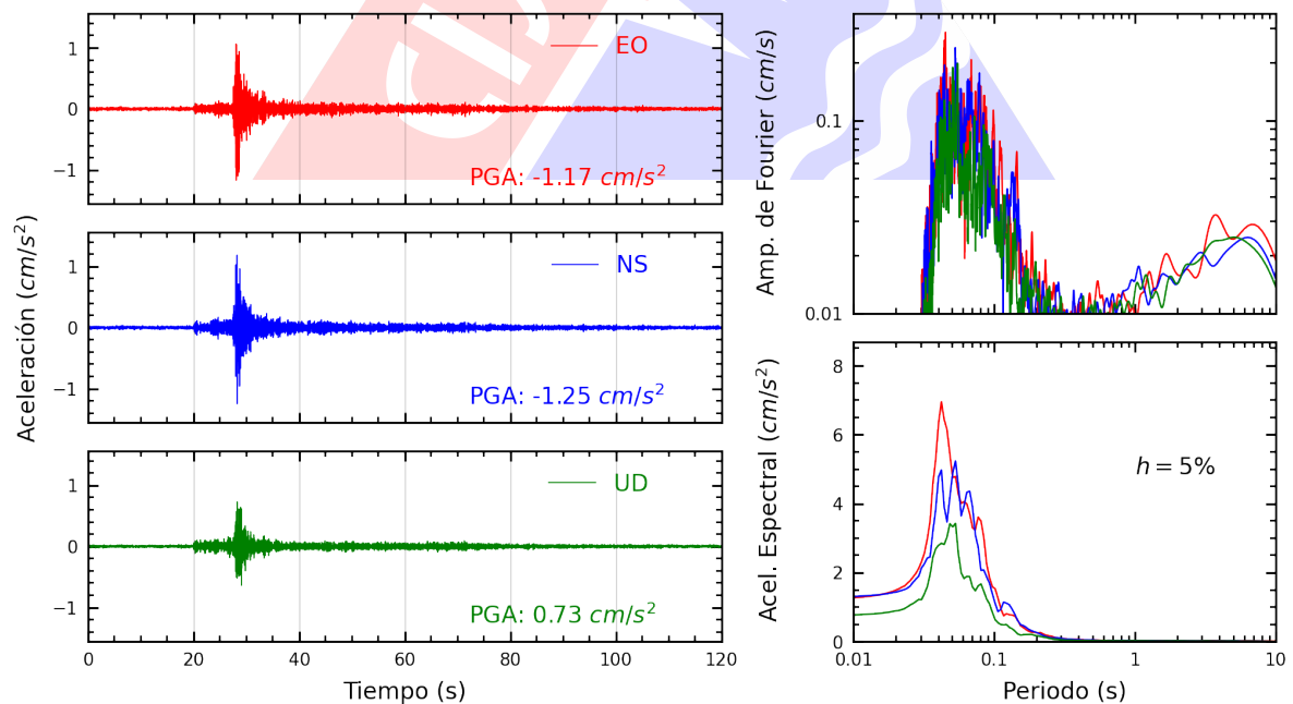
Figura A.8: Registros tiempo-historia, espectros de Fourier y de respuesta en las direcciones EO, NS y vertical de la estación FICPE. Sismo de Lima, Lima - Lima del 2025-03-28, 06:24:27 (Hora local)
