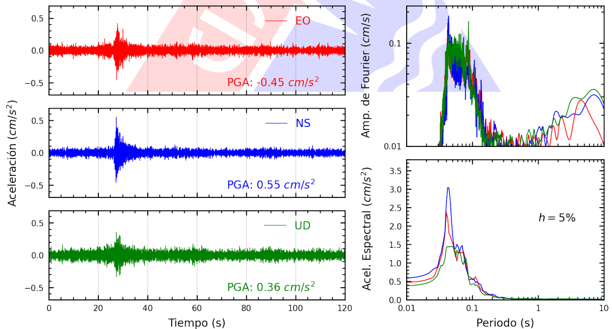
Figura A.18: Registros tiempo-historia, espectros de Fourier y de respuesta en las direcciones EO, NS y vertical de la estación URPE. Sismo de Lima, Lima - Lima del 2025-03-28, 06:24:27 (Hora local)
