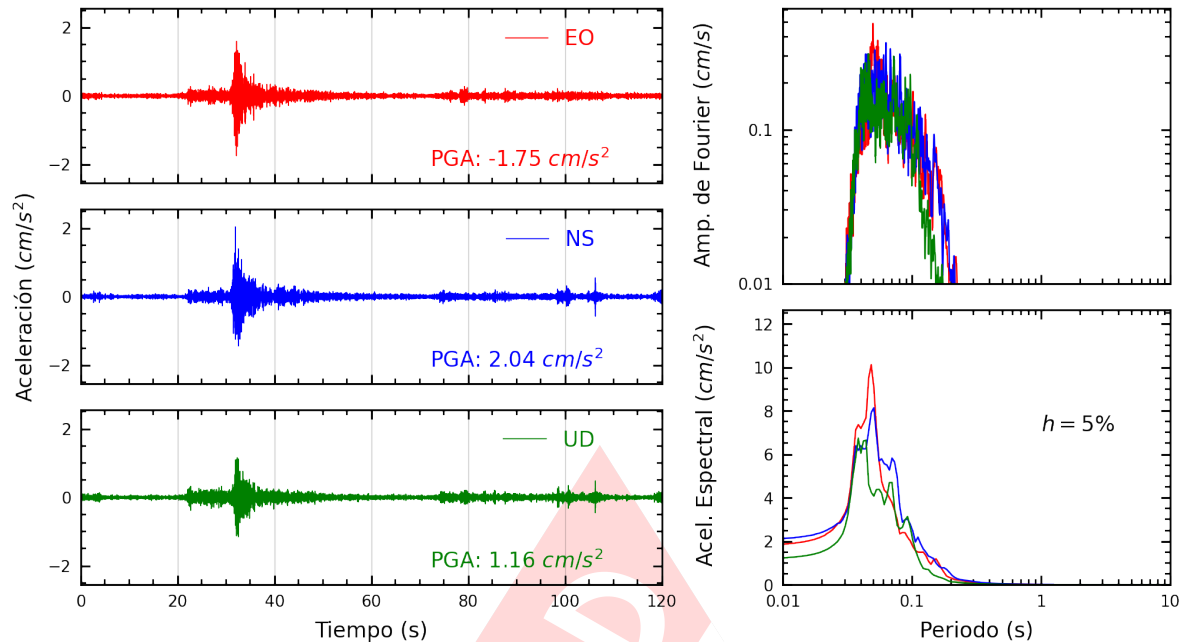
Figura A.3: Registros tiempo-historia, espectros de Fourier y de respuesta en las direcciones EO, NS y vertical de la estación SROS2. Sismo de Lima, Lima - Lima del 2025-03-28, 06:24:27 (Hora local)
