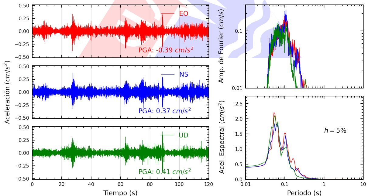
Figura A.26: Registros tiempo-historia, espectros de Fourier y de respuesta en las direcciones EO, NS y vertical de la estación SCCHO. Sismo de Lima, Lima - Lima del 2025-03-28, 06:24:27 (Hora local)
