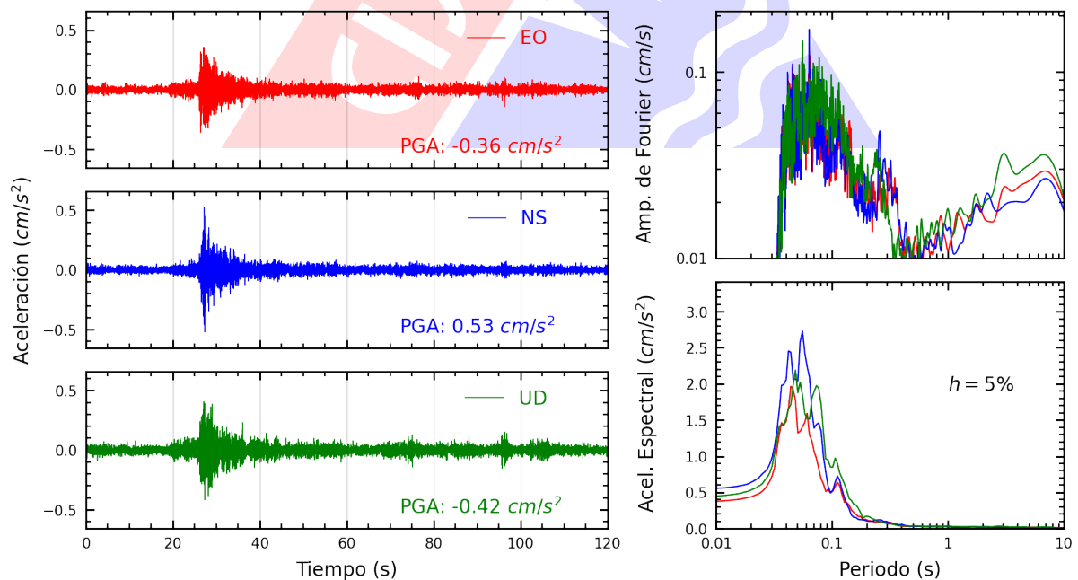
Figura A.20: Registros tiempo-historia, espectros de Fourier y de respuesta en las direcciones EO, NS y vertical de la estación SOVES. Sismo de Lima, Lima - Lima del 2025-03-28, 06:24:27 (Hora local)
