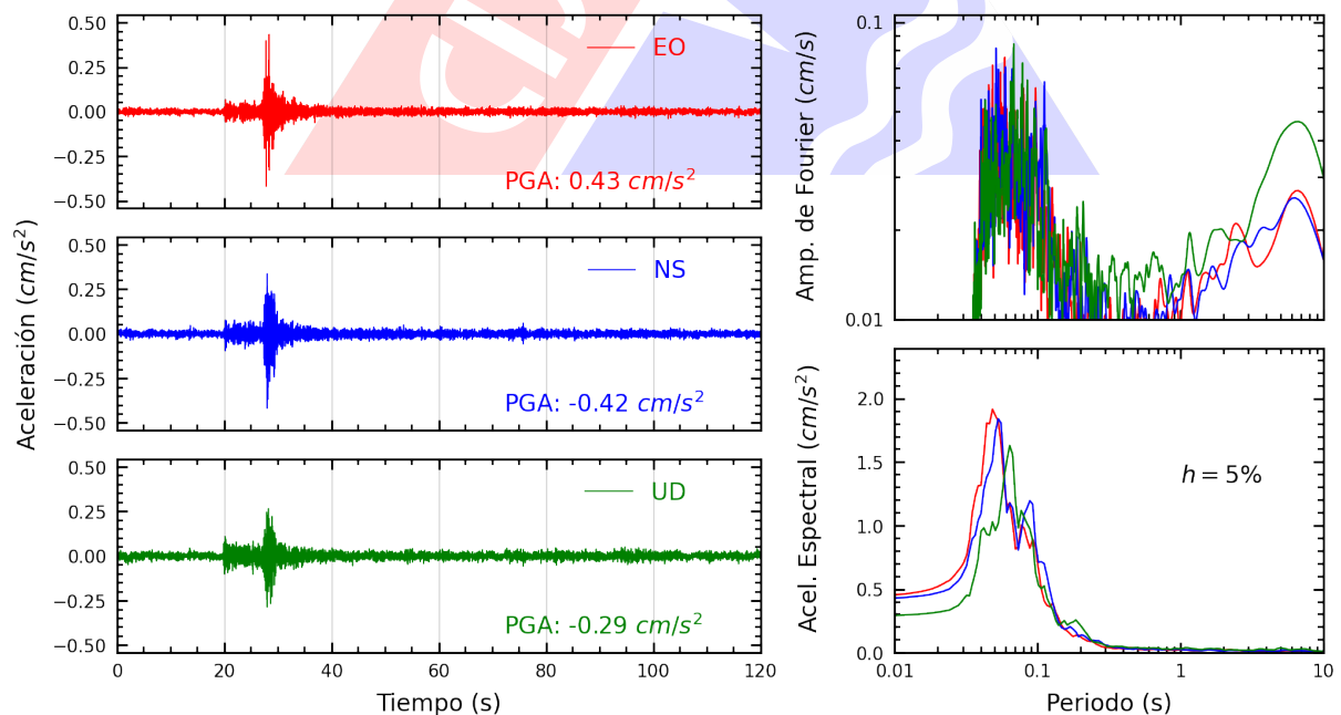
Figura A.24: Registros tiempo-historia, espectros de Fourier y de respuesta en las direcciones EO, NS y vertical de la estación UNFV. Sismo de Lima, Lima - Lima del 2025-03-28, 06:24:27 (Hora local)
