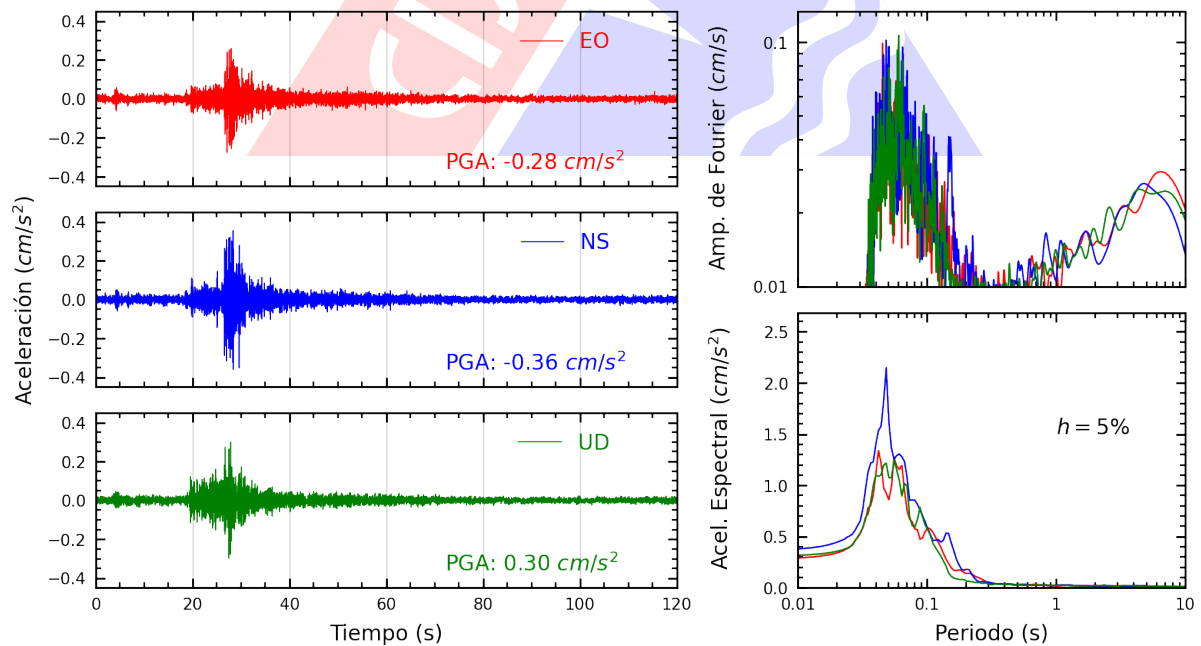
Figura A.30: Registros tiempo-historia, espectros de Fourier y de respuesta en las direcciones EO, NS y vertical de la estación SERVI. Sismo de Lima, Lima - Lima del 2025-03-28, 06:24:27 (Hora local)
