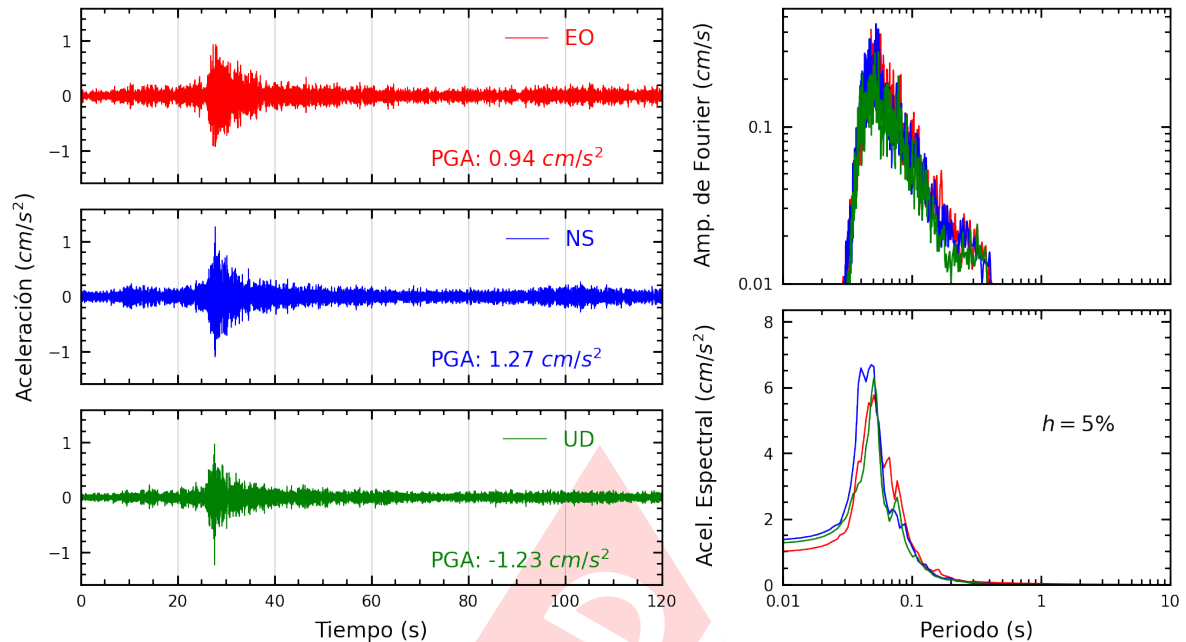
Figura A.7: Registros tiempo-historia, espectros de Fourier y de respuesta en las direcciones EO, NS y vertical de la estación UNTEL. Sismo de Lima, Lima - Lima del 2025-03-28, 06:24:27 (Hora local)
