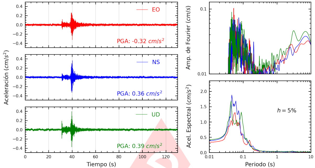
Figura A.29: Registros tiempo-historia, espectros de Fourier y de respuesta en las direcciones EO, NS y vertical de la estación UNMSM. Sismo de Lima, Lima - Lima del 2025-03-28, 06:24:27 (Hora local)
