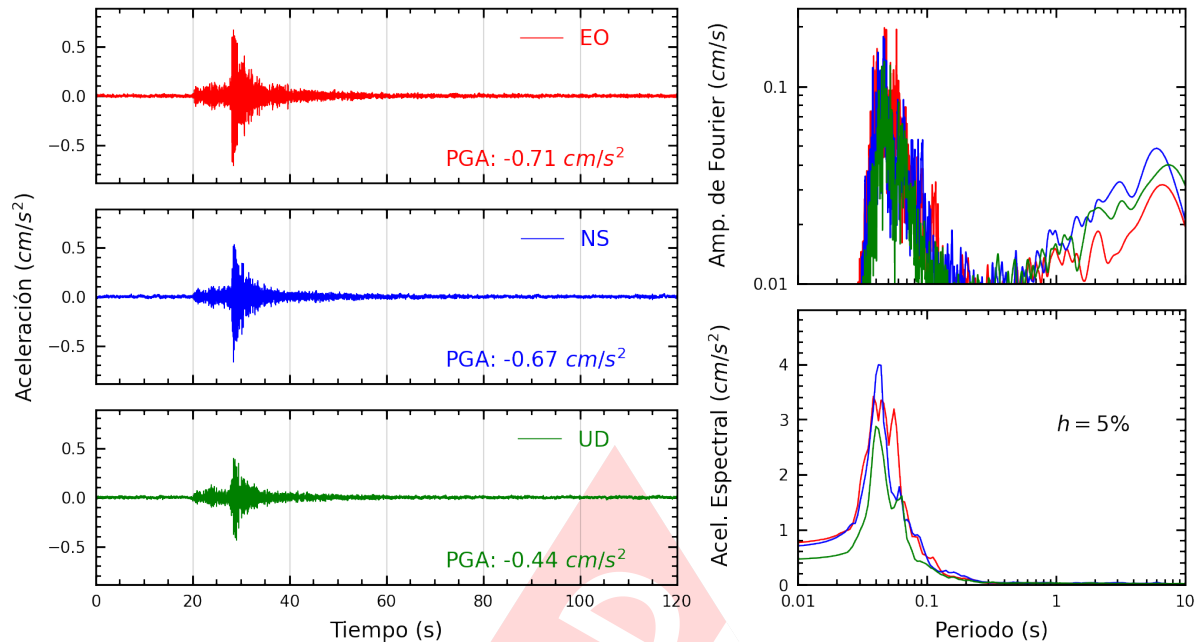
Figura A.15: Registros tiempo-historia, espectros de Fourier y de respuesta en las direcciones EO, NS y vertical de la estación UCSS. Sismo de Lima, Lima - Lima del 2025-03-28, 06:24:27 (Hora local)
