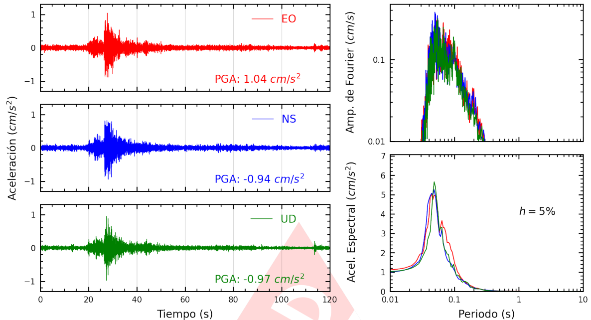
Figura A.11: Registros tiempo-historia, espectros de Fourier y de respuesta en las direcciones EO, NS y vertical de la estación PHER2. Sismo de Lima, Lima - Lima del 2025-03-28, 06:24:27 (Hora local)
