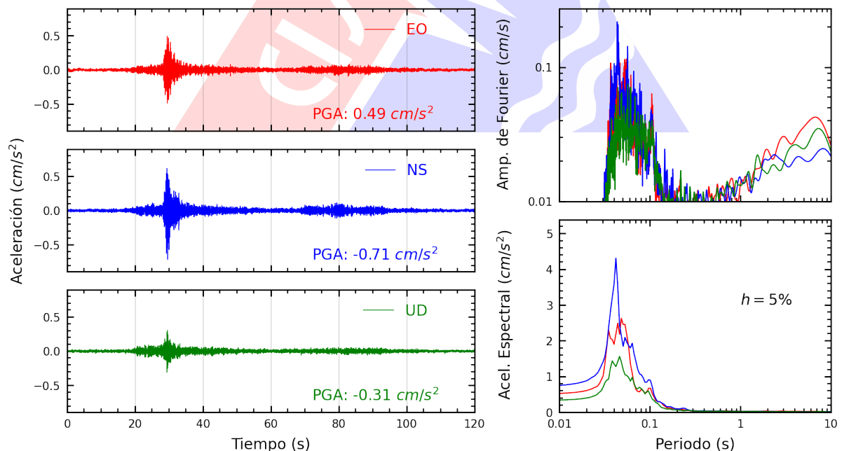
Figura A.14: Registros tiempo-historia, espectros de Fourier y de respuesta en las direcciones EO, NS y vertical de la estación COMAS. Sismo de Lima, Lima - Lima del 2025-03-28, 06:24:27 (Hora local)
