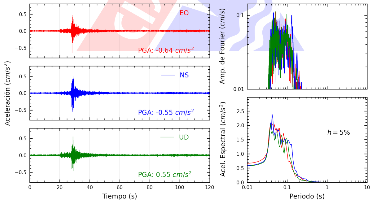
Figura A.16: Registros tiempo-historia, espectros de Fourier y de respuesta en las direcciones EO, NS y vertical de la estación JALV2. Sismo de Lima, Lima - Lima del 2025-03-28, 06:24:27 (Hora local)
