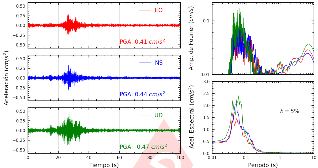
Figura A.23: Registros tiempo-historia, espectros de Fourier y de respuesta en las direcciones EO, NS y vertical de la estación SOCHO. Sismo de Lima, Lima - Lima del 2025-03-28, 06:24:27 (Hora local)
