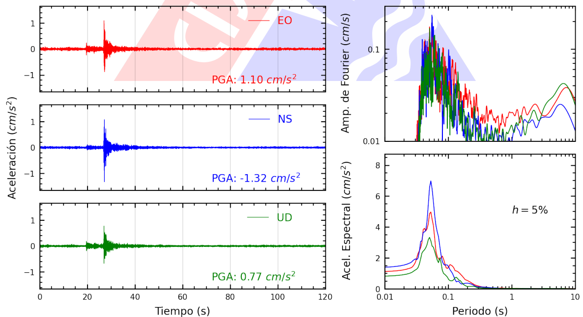
Figura A.6: Registros tiempo-historia, espectros de Fourier y de respuesta en las direcciones EO, NS y vertical de la estación IMCA. Sismo de Lima, Lima - Lima del 2025-03-28, 06:24:27 (Hora local)
