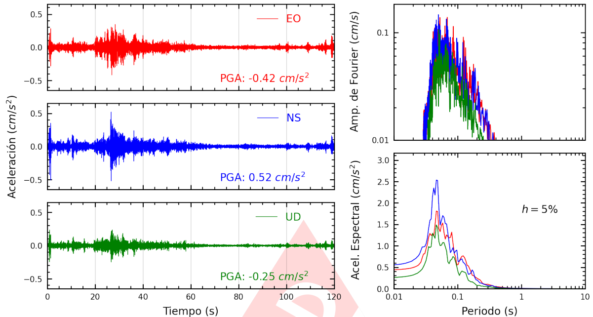
Figura A.21: Registros tiempo-historia, espectros de Fourier y de respuesta en las direcciones EO, NS y vertical de la estación BRIS2. Sismo de Lima, Lima - Lima del 2025-03-28, 06:24:27 (Hora local)
