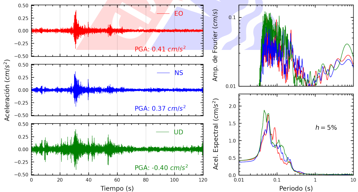
Figura A.28: Registros tiempo-historia, espectros de Fourier y de respuesta en las direcciones EO, NS y vertical de la estación MDPP. Sismo de Lima, Lima - Lima del 2025-03-28, 06:24:27 (Hora local)
