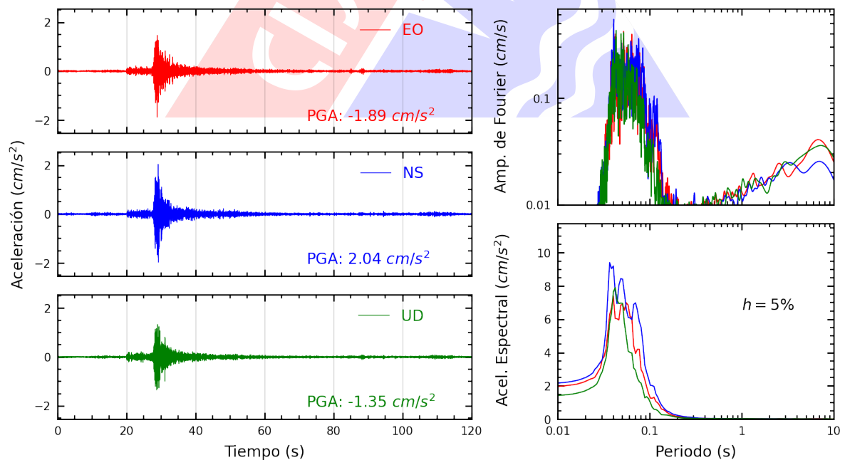
Figura A.4: Registros tiempo-historia, espectros de Fourier y de respuesta en las direcciones EO, NS y vertical de la estación JOSEO. Sismo de Lima, Lima - Lima del 2025-03-28, 06:24:27 (Hora local)
