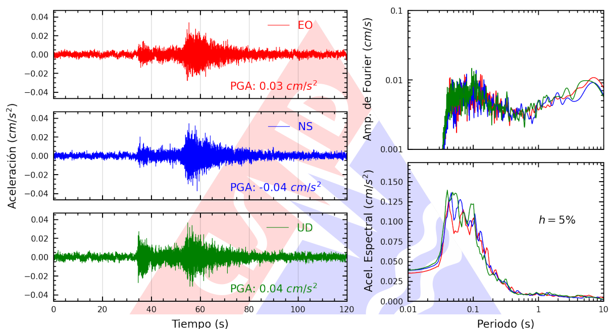
Figura A.33: Registros tiempo-historia, espectros de Fourier y de respuesta en las direcciones EO, NS y vertical de la estación CARAL. Sismo de Lima, Lima - Lima del 2025-03-28, 06:24:27 (Hora local)
