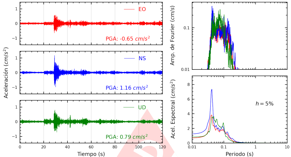
Figura A.9: Registros tiempo-historia, espectros de Fourier y de respuesta en las direcciones EO, NS y vertical de la estación CARA2. Sismo de Lima, Lima - Lima del 2025-03-28, 06:24:27 (Hora local)
