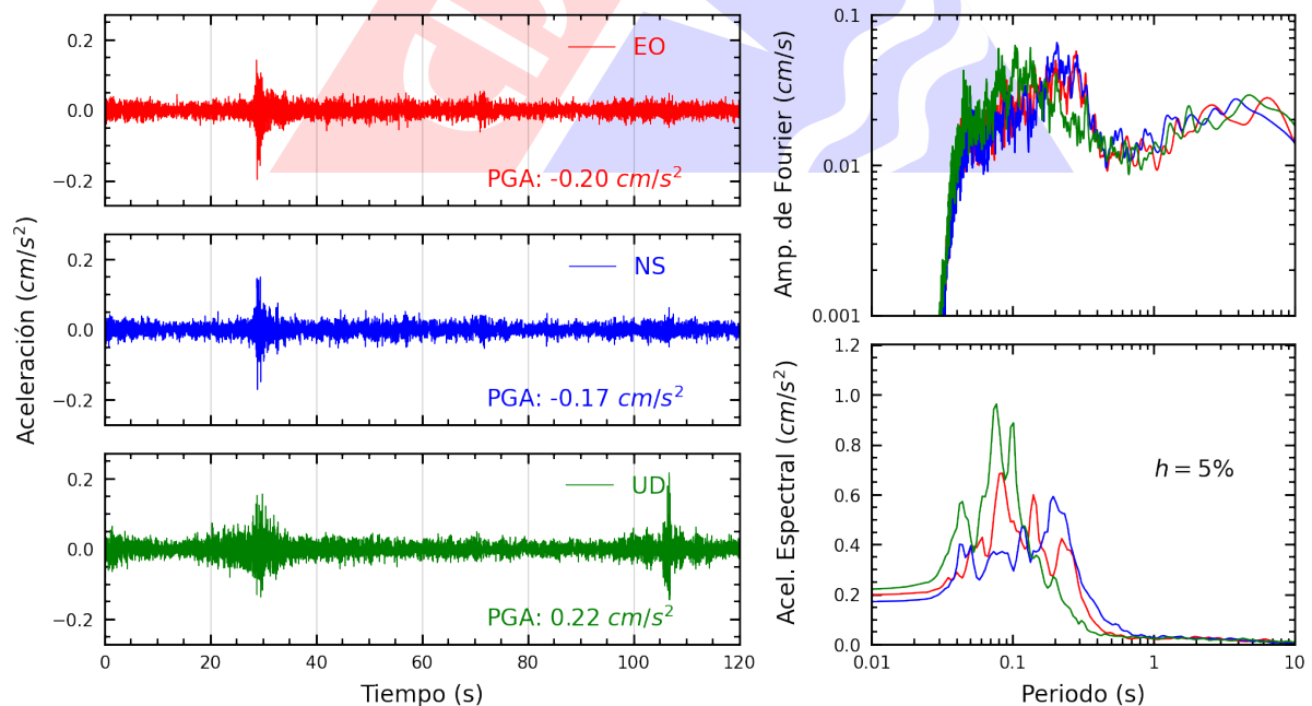
Figura A.32: Registros tiempo-historia, espectros de Fourier y de respuesta en las direcciones EO, NS y vertical de la estación DSMI. Sismo de Lima, Lima - Lima del 2025-03-28, 06:24:27 (Hora local)
