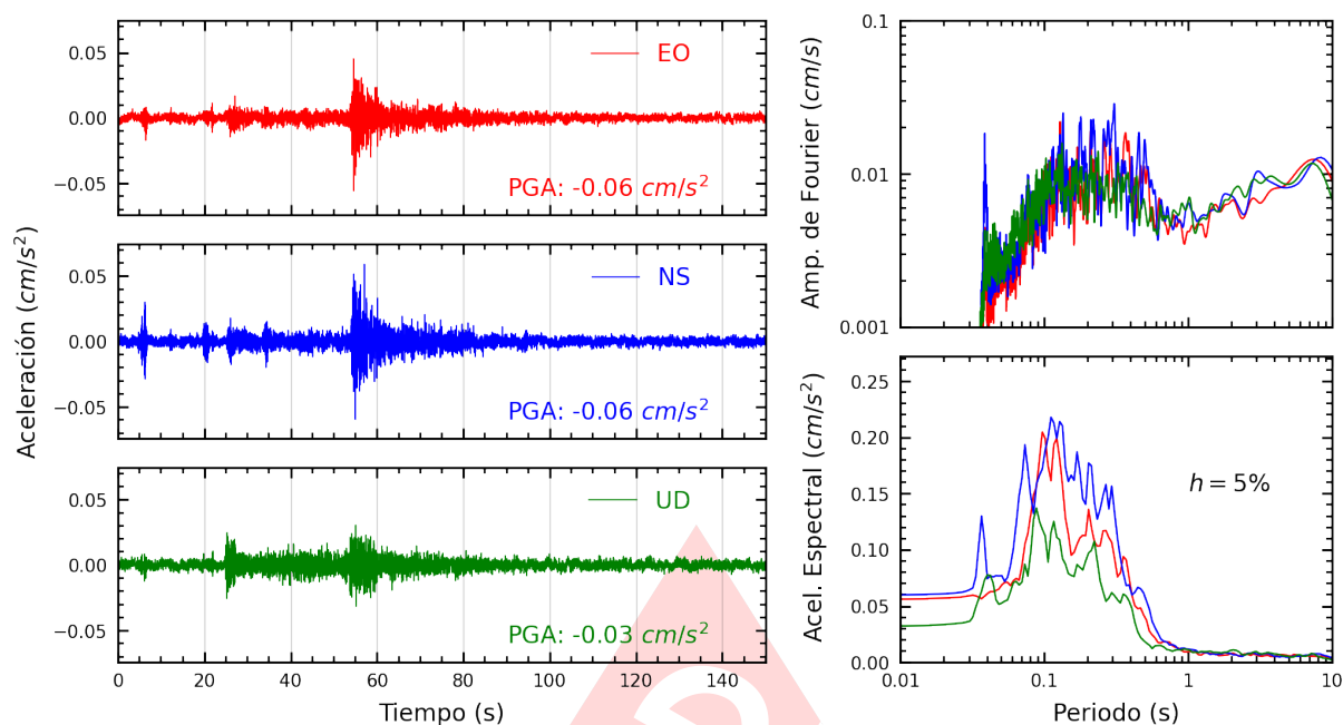
Figura A.7: Registros tiempo-historia, espectros de Fourier y de respuesta en las direcciones EO, NS y vertical de la estación UNJ. Sismo de Barranca, Datem del Marañón - Loreto del 2025-03-29, 03:36:13 (Hora local)
