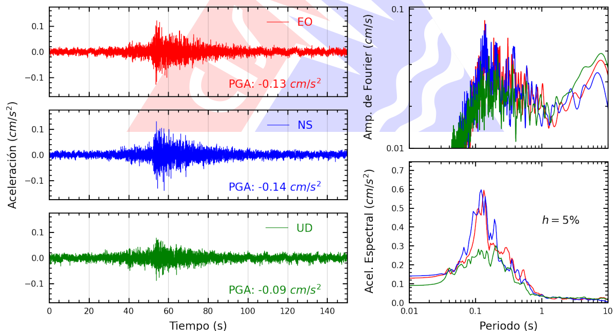
Figura A.2: Registros tiempo-historia, espectros de Fourier y de respuesta en las direcciones EO, NS y vertical de la estación UNTRM. Sismo de Barranca, Datem del Marañón - Loreto del 2025-03-29, 03:36:13 (Hora local)
