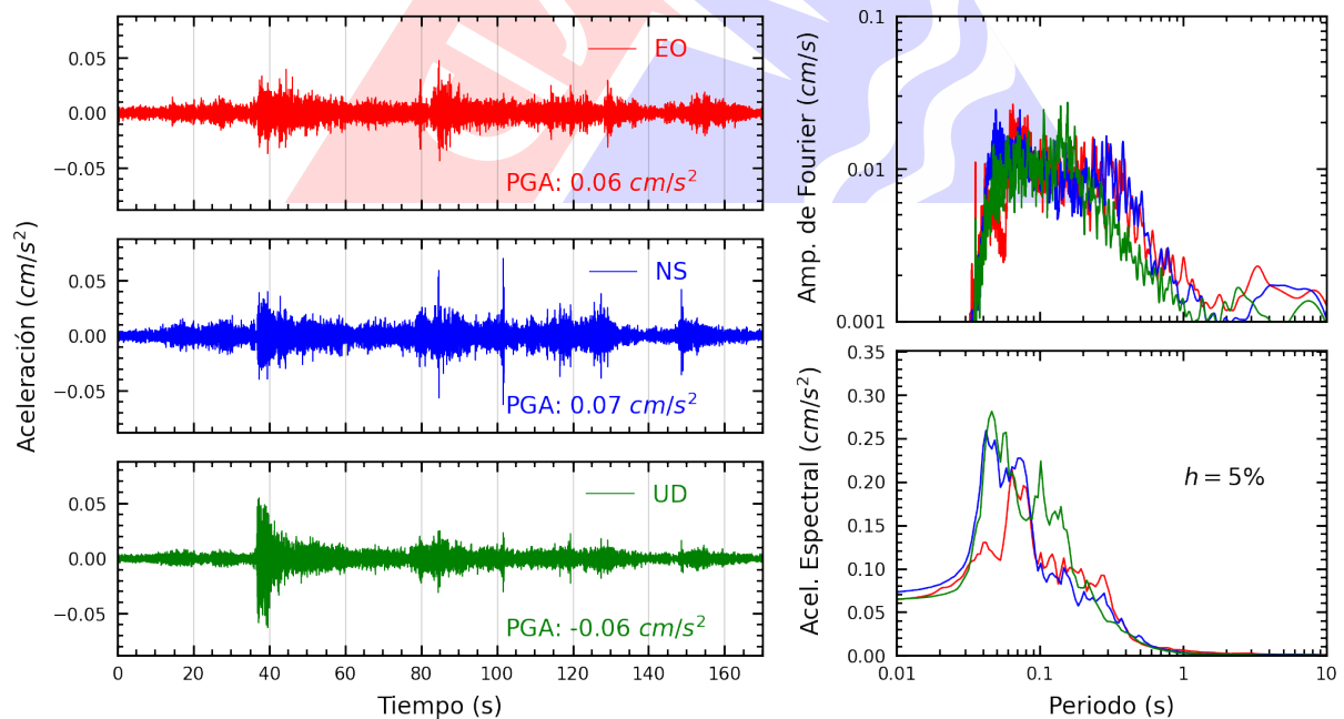
Figura A.4: Registros tiempo-historia, espectros de Fourier y de respuesta en las direcciones EO, NS y vertical de la estación UPAOP. Sismo de Barranca, Datem del Marañón - Loreto del 2025-03-29, 03:36:13 (Hora local)
