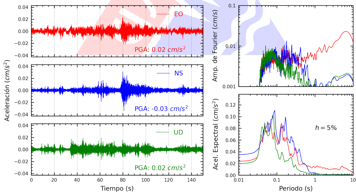
Figura A.8: Registros tiempo-historia, espectros de Fourier y de respuesta en las direcciones EO, NS y vertical de la estación SCCHI. Sismo de Barranca, Datem del Marañón - Loreto del 2025-03-29, 03:36:13 (Hora local)
