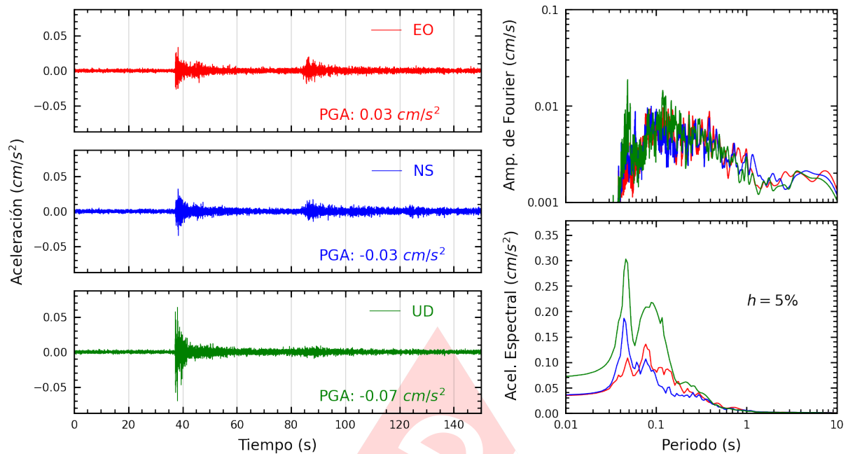
Figura A.5: Registros tiempo-historia, espectros de Fourier y de respuesta en las direcciones EO, NS y vertical de la estación UNF. Sismo de Barranca, Datem del Marañón - Loreto del 2025-03-29, 03:36:13 (Hora local)
