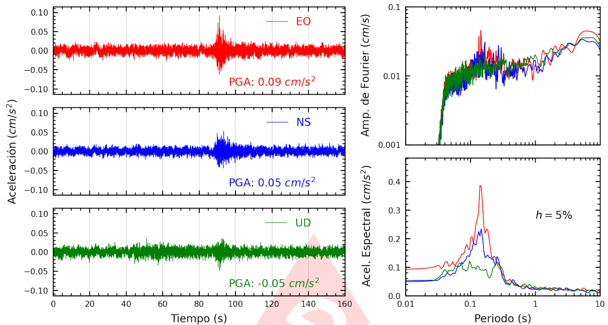
Figura A.3: Registros tiempo-historia, espectros de Fourier y de respuesta en las direcciones EO, NS y vertical de la estación UCVCH. Sismo de Barranca, Datem del Marañón - Loreto del 2025-03-29, 03:36:13 (Hora local)
