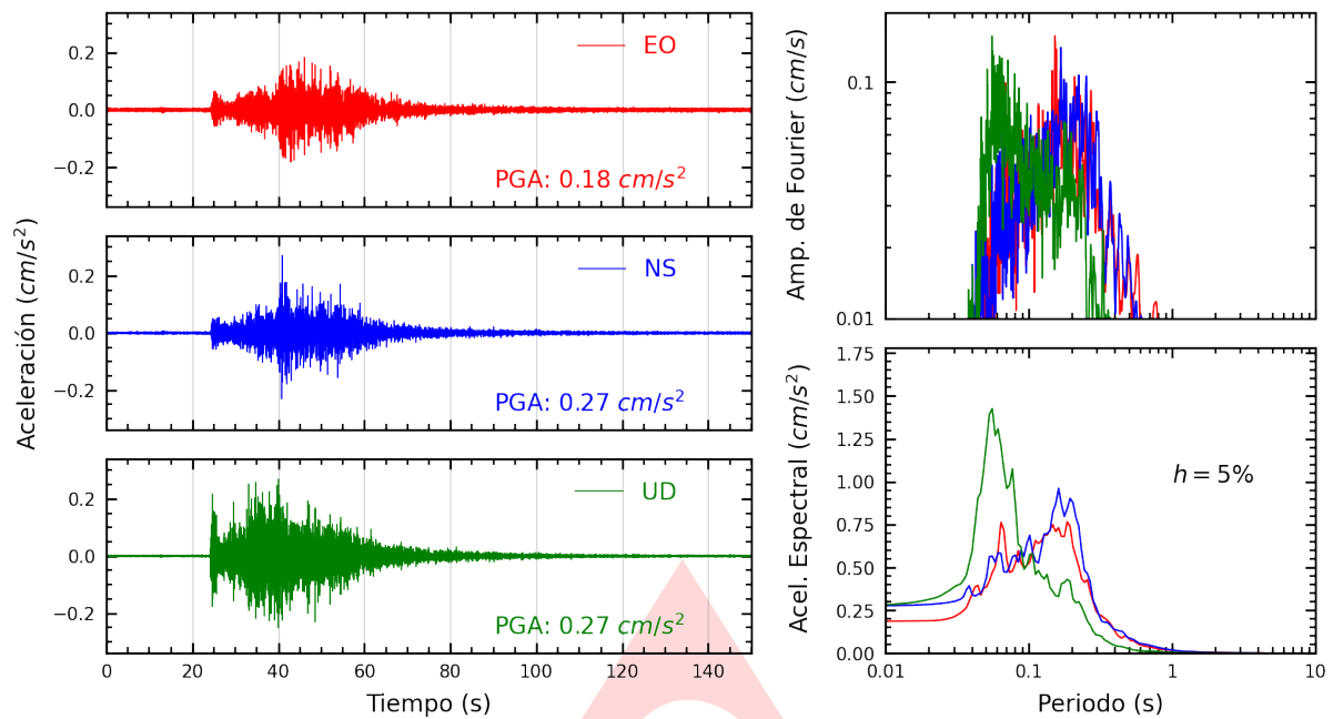
Figura A.1: Registros tiempo-historia, espectros de Fourier y de respuesta en las direcciones EO, NS y vertical de la estación UNAAA. Sismo de Barranca, Datem del Marañón - Loreto del 2025-03-29, 03:36:13 (Hora local)
