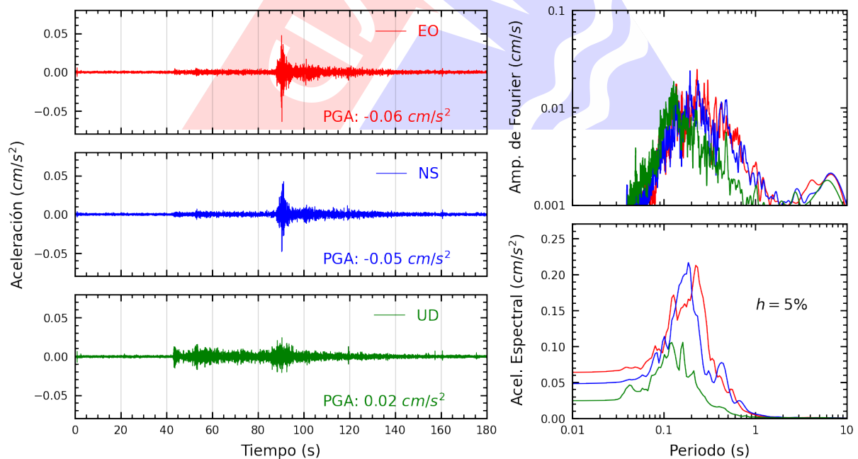
Figura A.6: Registros tiempo-historia, espectros de Fourier y de respuesta en las direcciones EO, NS y vertical de la estación UNIA. Sismo de Barranca, Datem del Marañón - Loreto del 2025-03-29, 03:36:13 (Hora local)
