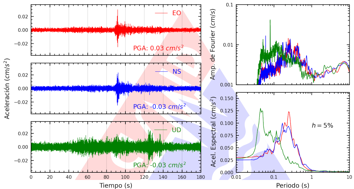
Figura A.9: Registros tiempo-historia, espectros de Fourier y de respuesta en las direcciones EO, NS y vertical de la estación SCPUC. Sismo de Barranca, Datem del Marañón - Loreto del 2025-03-29, 03:36:13 (Hora local)
