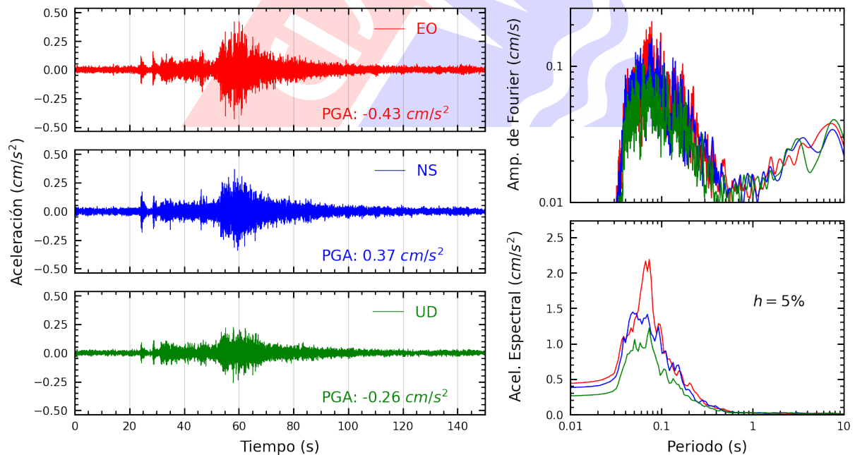
Figura A.22: Registros tiempo-historia, espectros de Fourier y de respuesta en las direcciones EO, NS y vertical de la estación FICPE. Sismo de Lunahuana, Cañete - Lima del 2025-03-29, 14:53:31 (Hora local)
