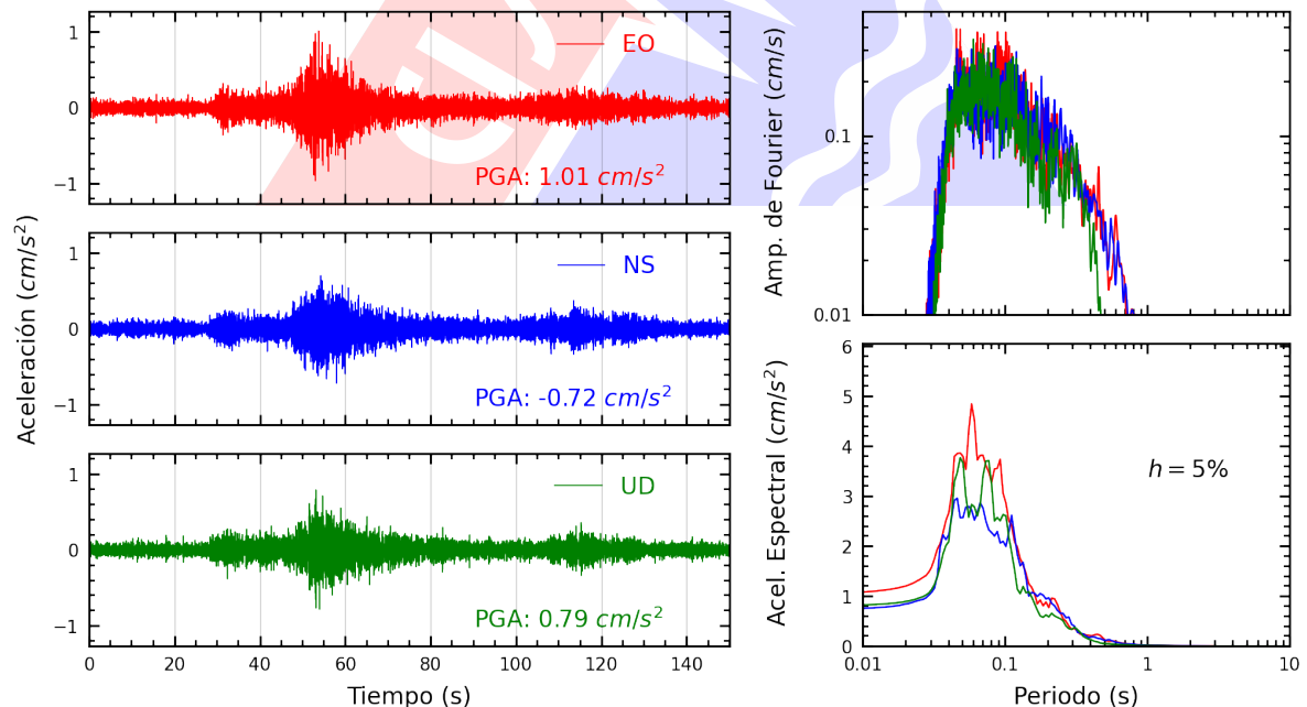
Figura A.10: Registros tiempo-historia, espectros de Fourier y de respuesta en las direcciones EO, NS y vertical de la estación UNTEL. Sismo de Lunahuana, Cañete - Lima del 2025-03-29, 14:53:31 (Hora local)
