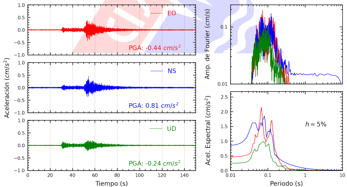
Figura A.12: Registros tiempo-historia, espectros de Fourier y de respuesta en las direcciones EO, NS y vertical de la estación ATARJ. Sismo de Lunahuana, Cañete - Lima del 2025-03-29, 14:53:31 (Hora local)
