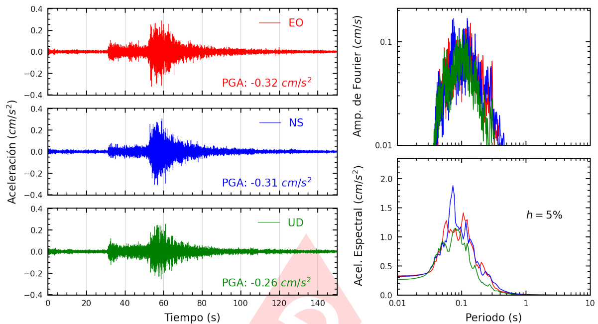
Figura A.29: Registros tiempo-historia, espectros de Fourier y de respuesta en las direcciones EO, NS y vertical de la estación JALV2. Sismo de Lunahuana, Cañete - Lima del 2025-03-29, 14:53:31 (Hora local)
