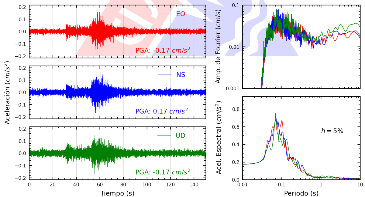
Figura A.36: Registros tiempo-historia, espectros de Fourier y de respuesta en las direcciones EO, NS y vertical de la estación UNFV. Sismo de Lunahuana, Cañete - Lima del 2025-03-29, 14:53:31 (Hora local)
