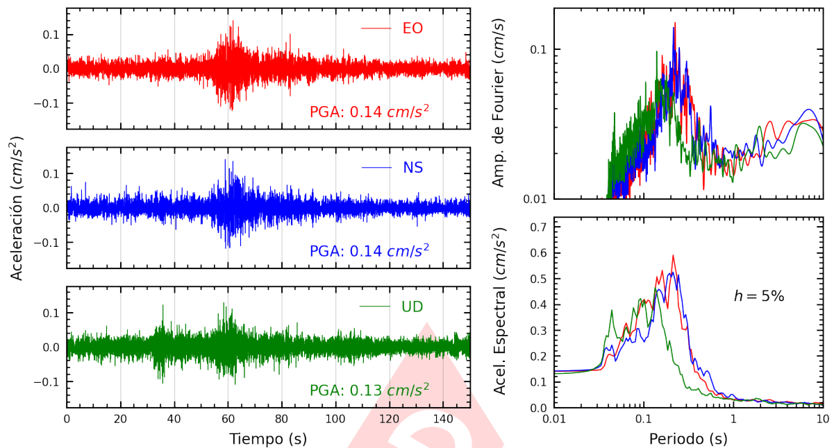
Figura A.39: Registros tiempo-historia, espectros de Fourier y de respuesta en las direcciones EO, NS y vertical de la estación DSMI. Sismo de Lunahuana, Cañete - Lima del 2025-03-29, 14:53:31 (Hora local)
