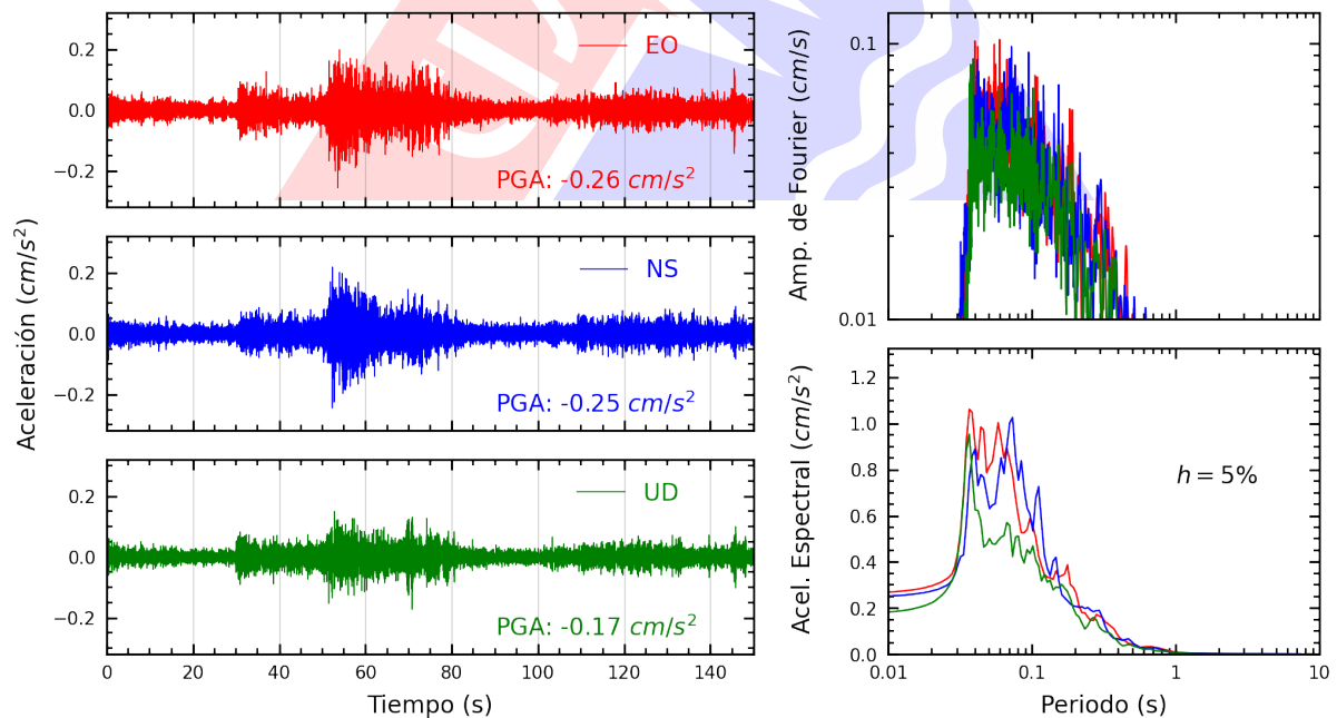
Figura A.34: Registros tiempo-historia, espectros de Fourier y de respuesta en las direcciones EO, NS y vertical de la estación BORJA. Sismo de Lunahuana, Cañete - Lima del 2025-03-29, 14:53:31 (Hora local)
