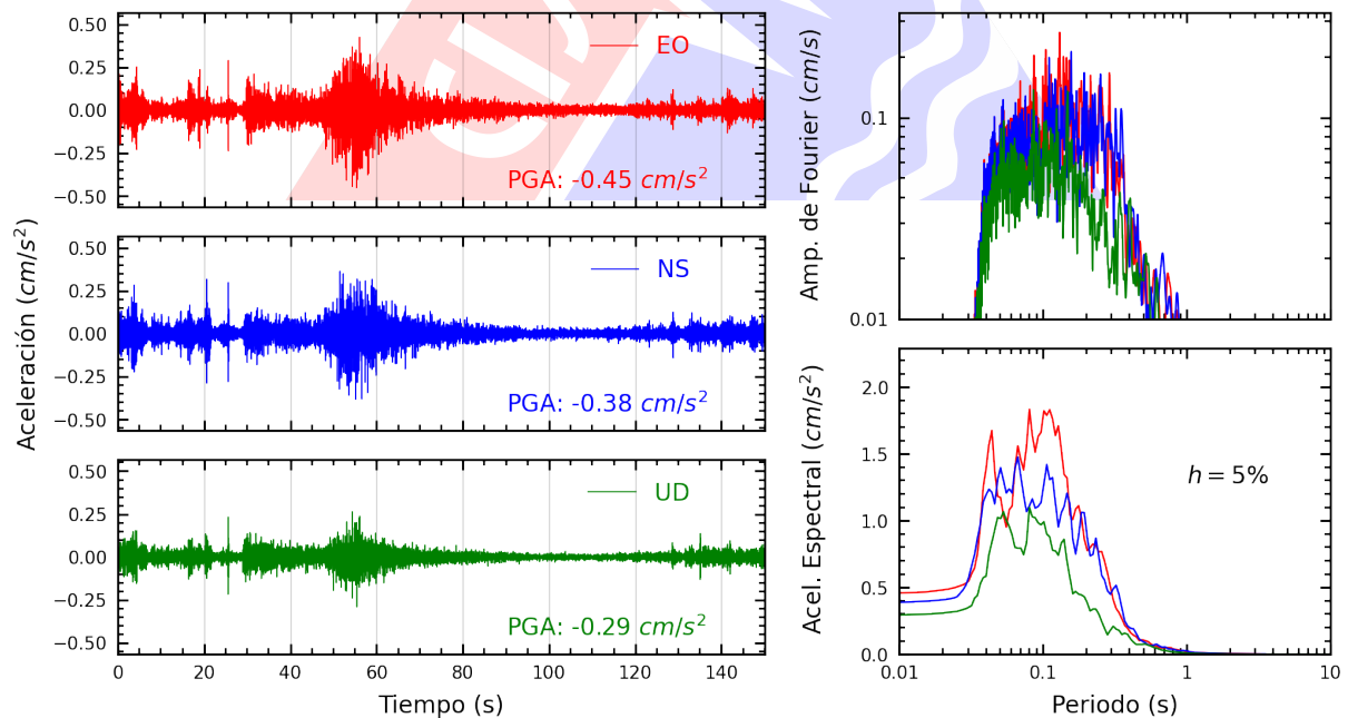
Figura A.20: Registros tiempo-historia, espectros de Fourier y de respuesta en las direcciones EO, NS y vertical de la estación BRISA. Sismo de Lunahuana, Cañete - Lima del 2025-03-29, 14:53:31 (Hora local)
