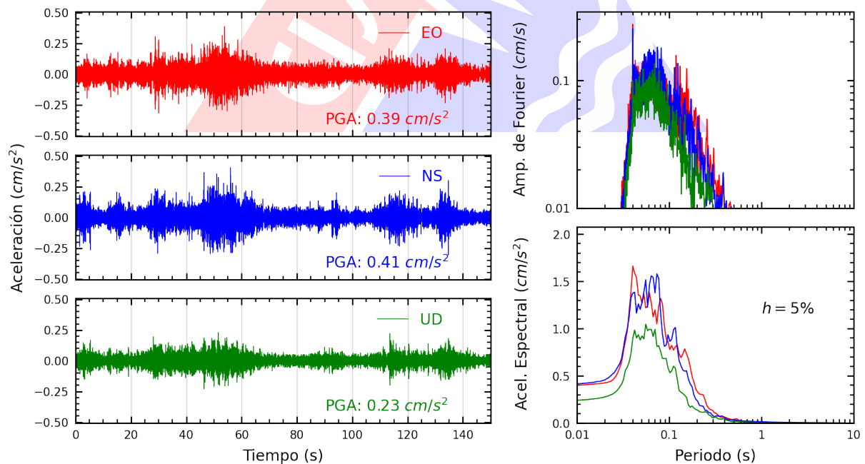
Figura A.24: Registros tiempo-historia, espectros de Fourier y de respuesta en las direcciones EO, NS y vertical de la estación PACHA. Sismo de Lunahuana, Cañete - Lima del 2025-03-29, 14:53:31 (Hora local)
