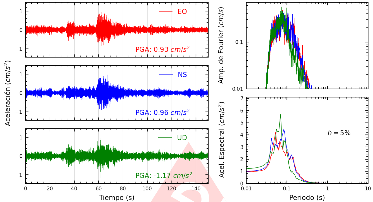
Figura A.9: Registros tiempo-historia, espectros de Fourier y de respuesta en las direcciones EO, NS y vertical de la estación SROS2. Sismo de Lunahuana, Cañete - Lima del 2025-03-29, 14:53:31 (Hora local)
