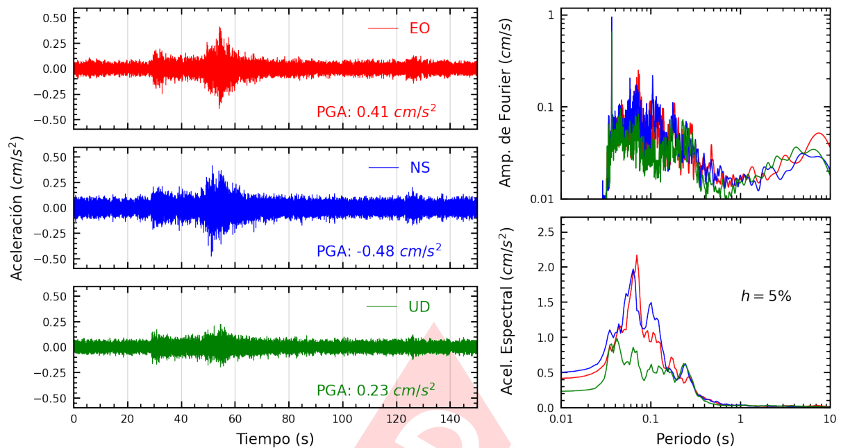
Figura A.19: Registros tiempo-historia, espectros de Fourier y de respuesta en las direcciones EO, NS y vertical de la estación UPCVI. Sismo de Lunahuana, Cañete - Lima del 2025-03-29, 14:53:31 (Hora local)
