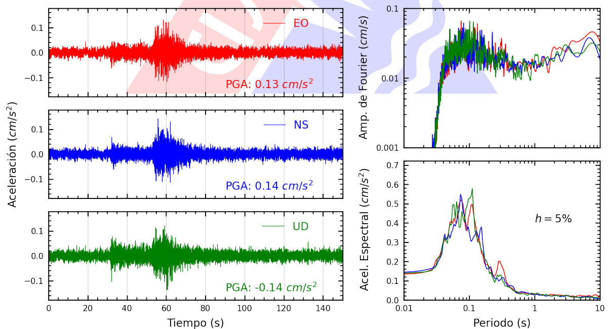
Figura A.38: Registros tiempo-historia, espectros de Fourier y de respuesta en las direcciones EO, NS y vertical de la estación BONDY. Sismo de Lunahuana, Cañete - Lima del 2025-03-29, 14:53:31 (Hora local)
