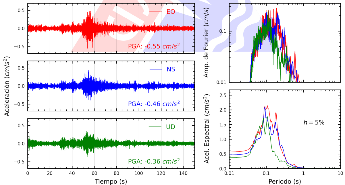
Figura A.16: Registros tiempo-historia, espectros de Fourier y de respuesta en las direcciones EO, NS y vertical de la estación SCCHO. Sismo de Lunahuana, Cañete - Lima del 2025-03-29, 14:53:31 (Hora local)
