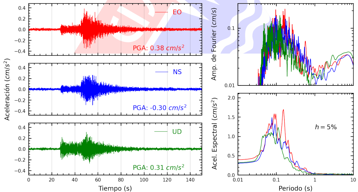
Figura A.26: Registros tiempo-historia, espectros de Fourier y de respuesta en las direcciones EO, NS y vertical de la estación USILP. Sismo de Lunahuana, Cañete - Lima del 2025-03-29, 14:53:31 (Hora local)
