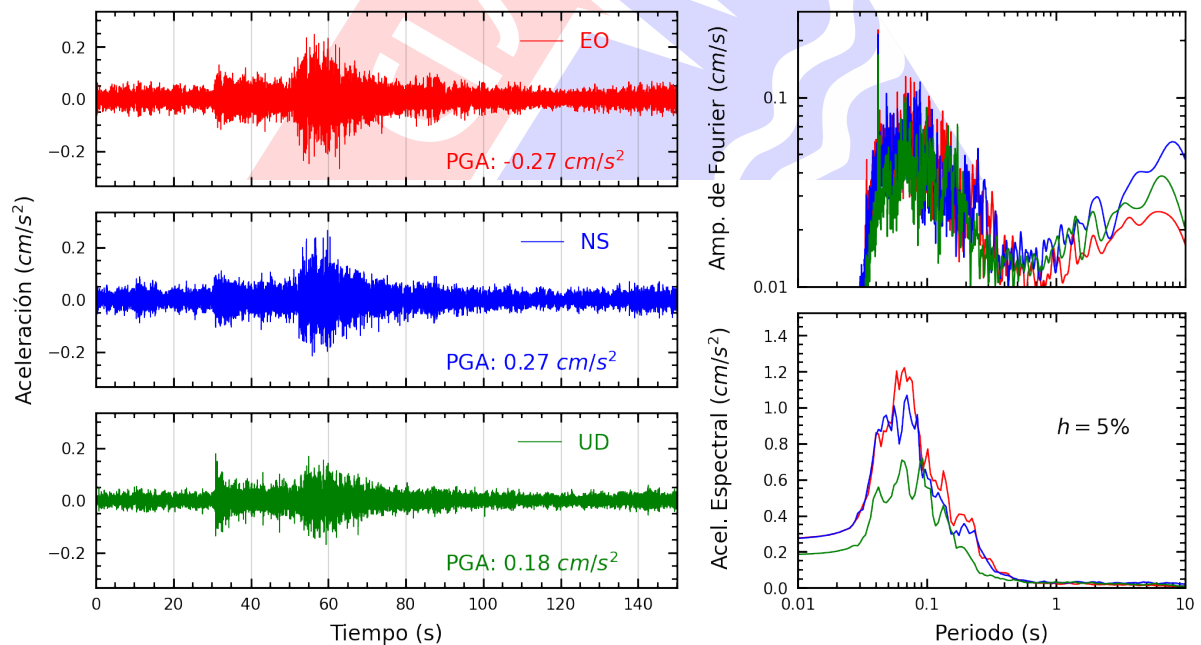
Figura A.32: Registros tiempo-historia, espectros de Fourier y de respuesta en las direcciones EO, NS y vertical de la estación CEPRE. Sismo de Lunahuana, Cañete - Lima del 2025-03-29, 14:53:31 (Hora local)
