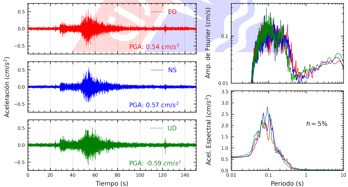
Figura A.14: Registros tiempo-historia, espectros de Fourier y de respuesta en las direcciones EO, NS y vertical de la estación SOVES. Sismo de Lunahuana, Cañete - Lima del 2025-03-29, 14:53:31 (Hora local)
