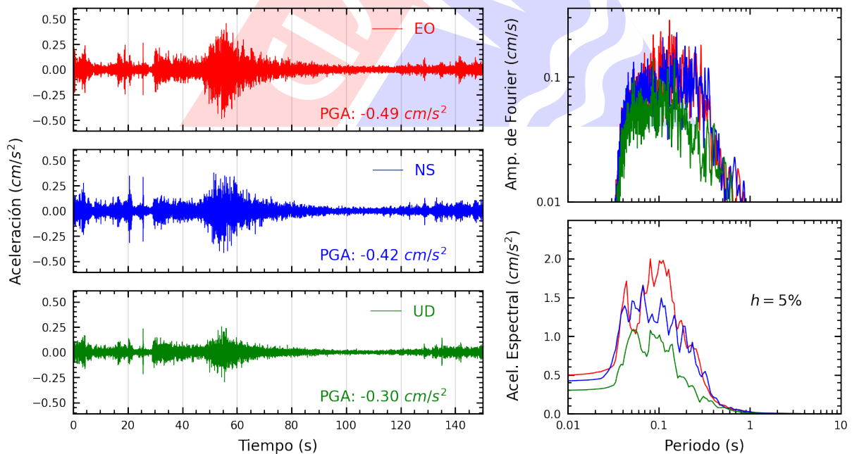
Figura A.18: Registros tiempo-historia, espectros de Fourier y de respuesta en las direcciones EO, NS y vertical de la estación BRIS2. Sismo de Lunahuana, Cañete - Lima del 2025-03-29, 14:53:31 (Hora local)
