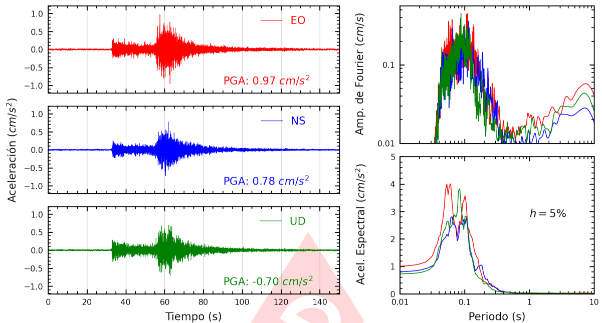
Figura A.11: Registros tiempo-historia, espectros de Fourier y de respuesta en las direcciones EO, NS y vertical de la estación AMORE. Sismo de Lunahuana, Cañete - Lima del 2025-03-29, 14:53:31 (Hora local)
