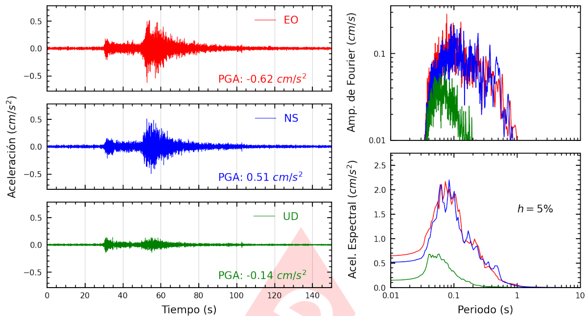
Figura A.13: Registros tiempo-historia, espectros de Fourier y de respuesta en las direcciones EO, NS y vertical de la estación UCVA2. Sismo de Lunahuana, Cañete - Lima del 2025-03-29, 14:53:31 (Hora local)
