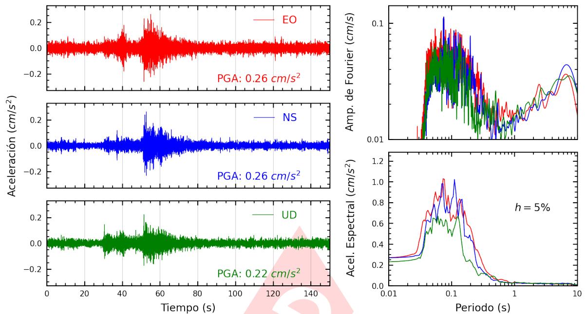
Figura A.33: Registros tiempo-historia, espectros de Fourier y de respuesta en las direcciones EO, NS y vertical de la estación INICT. Sismo de Lunahuana, Cañete - Lima del 2025-03-29, 14:53:31 (Hora local)
