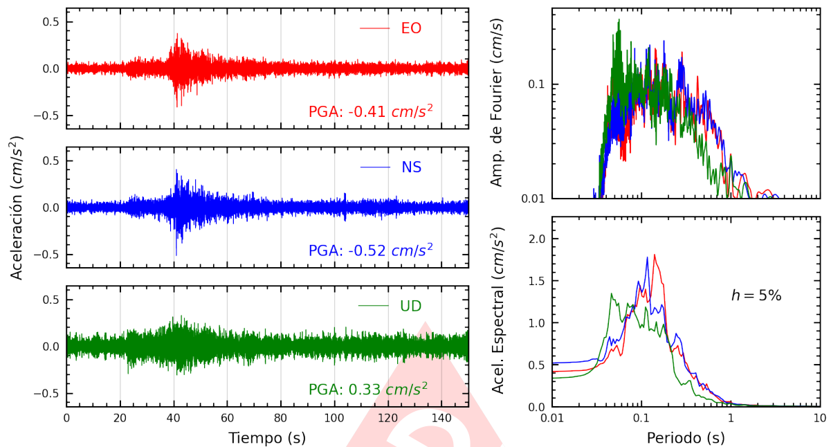
Figura A.17: Registros tiempo-historia, espectros de Fourier y de respuesta en las direcciones EO, NS y vertical de la estación UNICA. Sismo de Lunahuana, Cañete - Lima del 2025-03-29, 14:53:31 (Hora local)
