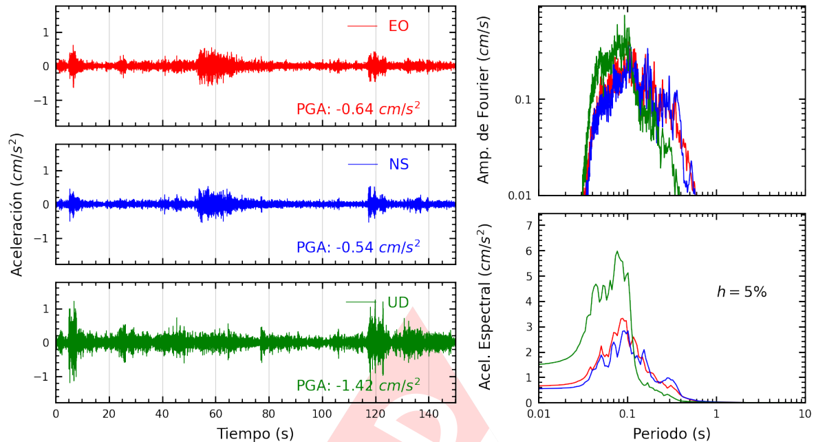
Figura A.5: Registros tiempo-historia, espectros de Fourier y de respuesta en las direcciones EO, NS y vertical de la estación SCOLI. Sismo de Lunahuana, Cañete - Lima del 2025-03-29, 14:53:31 (Hora local)
