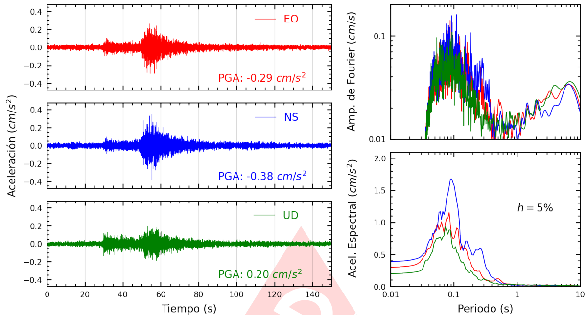
Figura A.27: Registros tiempo-historia, espectros de Fourier y de respuesta en las direcciones EO, NS y vertical de la estación SERVI. Sismo de Lunahuana, Cañete - Lima del 2025-03-29, 14:53:31 (Hora local)
