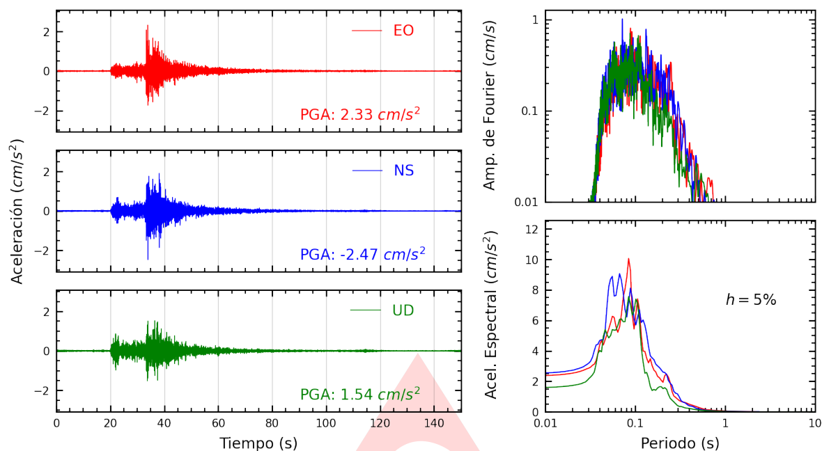
Figura A.1: Registros tiempo-historia, espectros de Fourier y de respuesta en las direcciones EO, NS y vertical de la estación ASIA. Sismo de Lunahuana, Cañete - Lima del 2025-03-29, 14:53:31 (Hora local)
