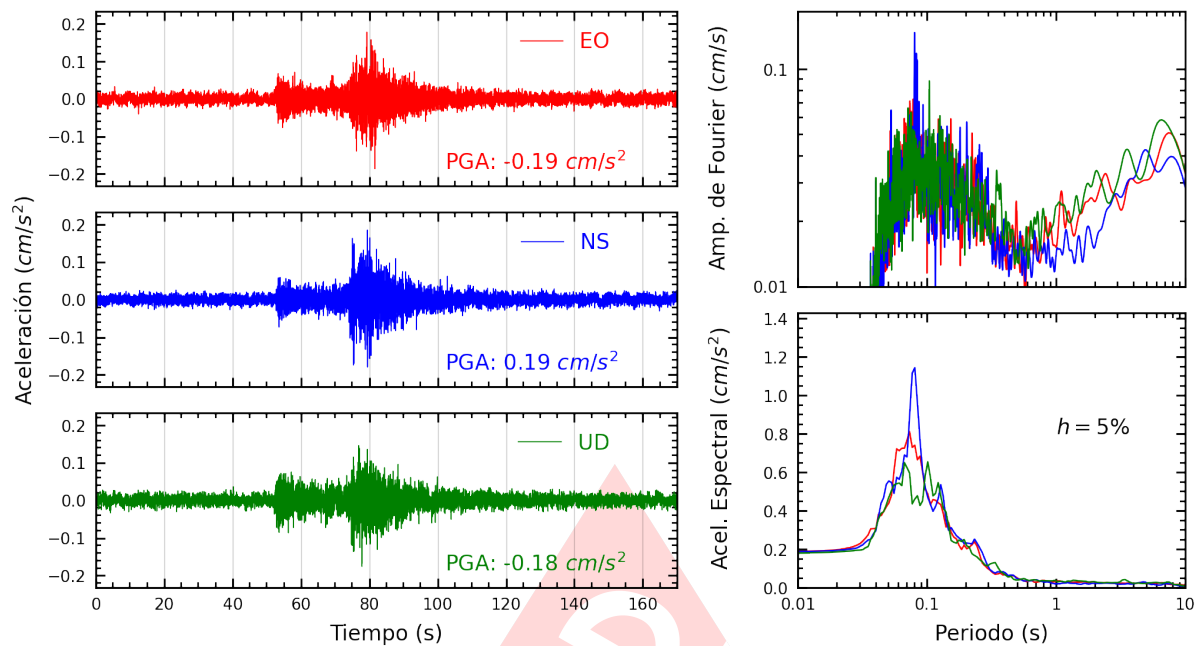
Figura A.35: Registros tiempo-historia, espectros de Fourier y de respuesta en las direcciones EO, NS y vertical de la estación UNMSM. Sismo de Lunahuana, Cañete - Lima del 2025-03-29, 14:53:31 (Hora local)
