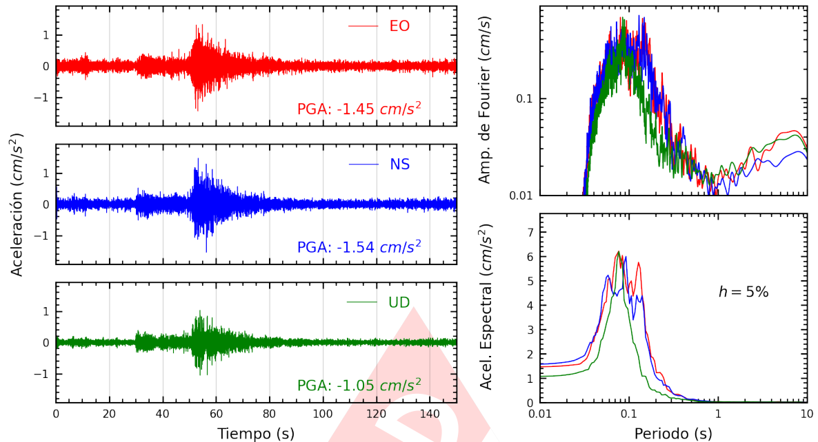
Figura A.3: Registros tiempo-historia, espectros de Fourier y de respuesta en las direcciones EO, NS y vertical de la estación USILM. Sismo de Lunahuana, Cañete - Lima del 2025-03-29, 14:53:31 (Hora local)
