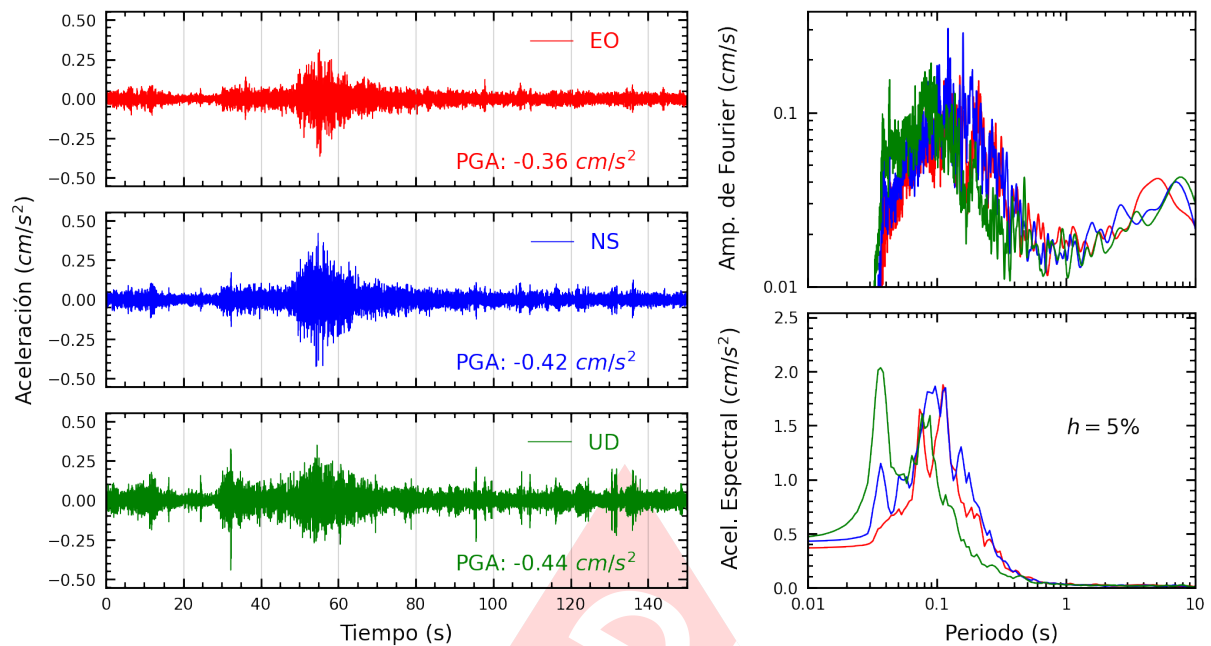
Figura A.21: Registros tiempo-historia, espectros de Fourier y de respuesta en las direcciones EO, NS y vertical de la estación SOCHO. Sismo de Lunahuana, Cañete - Lima del 2025-03-29, 14:53:31 (Hora local)
