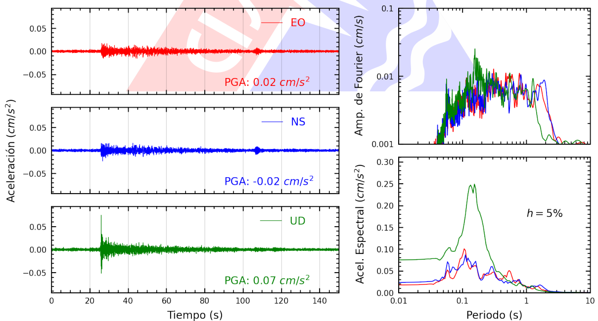
Figura A.40: Registros tiempo-historia, espectros de Fourier y de respuesta en las direcciones EO, NS y vertical de la estación UNCP. Sismo de Lunahuana, Cañete - Lima del 2025-03-29, 14:53:31 (Hora local)
