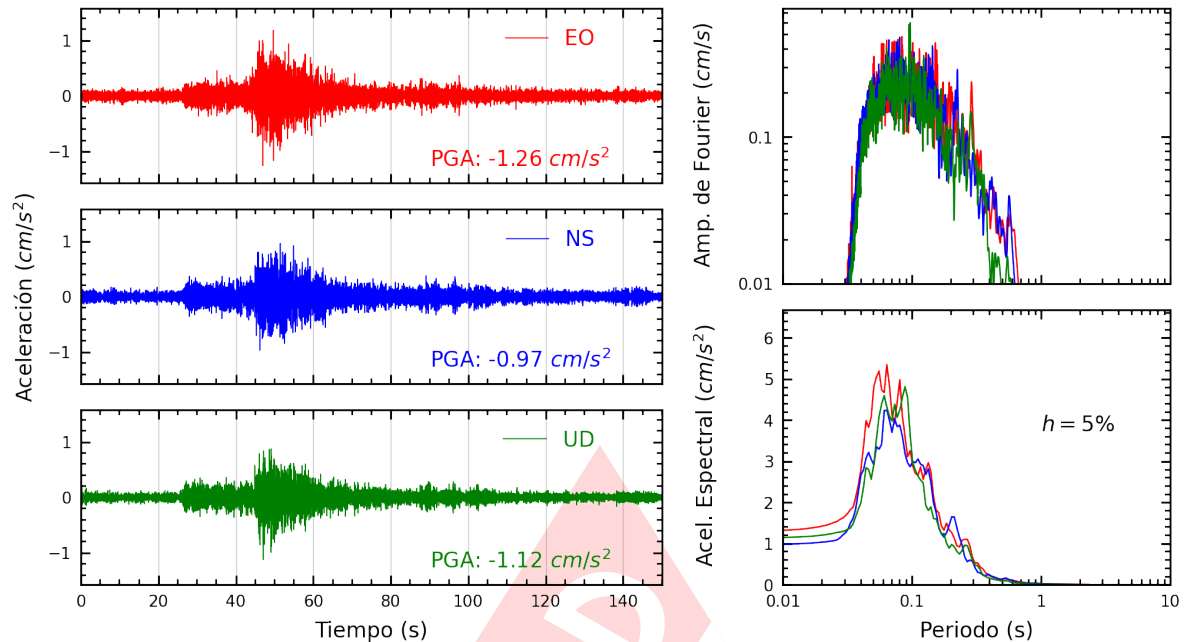
Figura A.7: Registros tiempo-historia, espectros de Fourier y de respuesta en las direcciones EO, NS y vertical de la estación PHER2. Sismo de Lunahuana, Cañete - Lima del 2025-03-29, 14:53:31 (Hora local)
