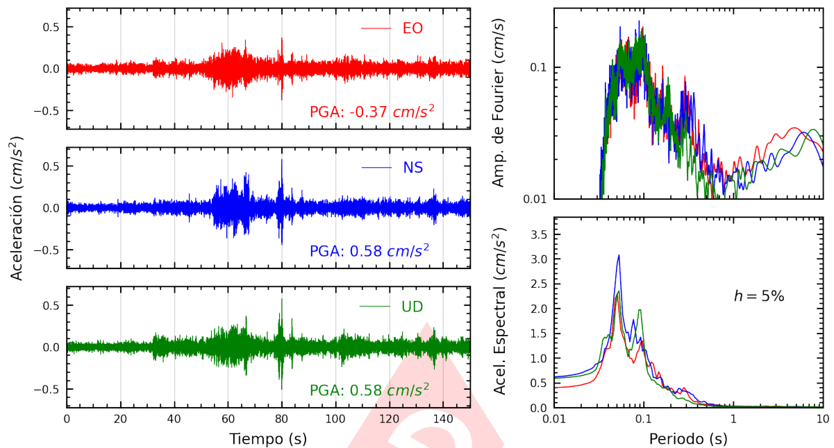
Figura A.15: Registros tiempo-historia, espectros de Fourier y de respuesta en las direcciones EO, NS y vertical de la estación MADRE. Sismo de Lunahuana, Cañete - Lima del 2025-03-29, 14:53:31 (Hora local)
