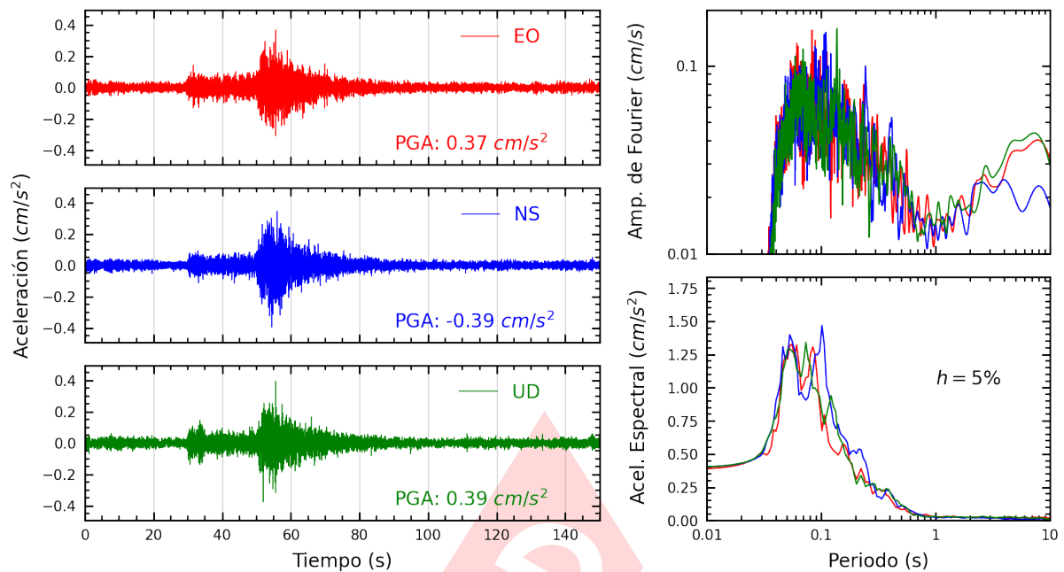
Figura A.25: Registros tiempo-historia, espectros de Fourier y de respuesta en las direcciones EO, NS y vertical de la estación IMCA. Sismo de Lunahuana, Cañete - Lima del 2025-03-29, 14:53:31 (Hora local)
