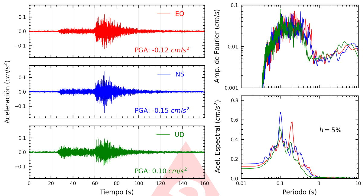
Figura A.37: Registros tiempo-historia, espectros de Fourier y de respuesta en las direcciones EO, NS y vertical de la estación CARAL. Sismo de Lunahuana, Cañete - Lima del 2025-03-29, 14:53:31 (Hora local)
