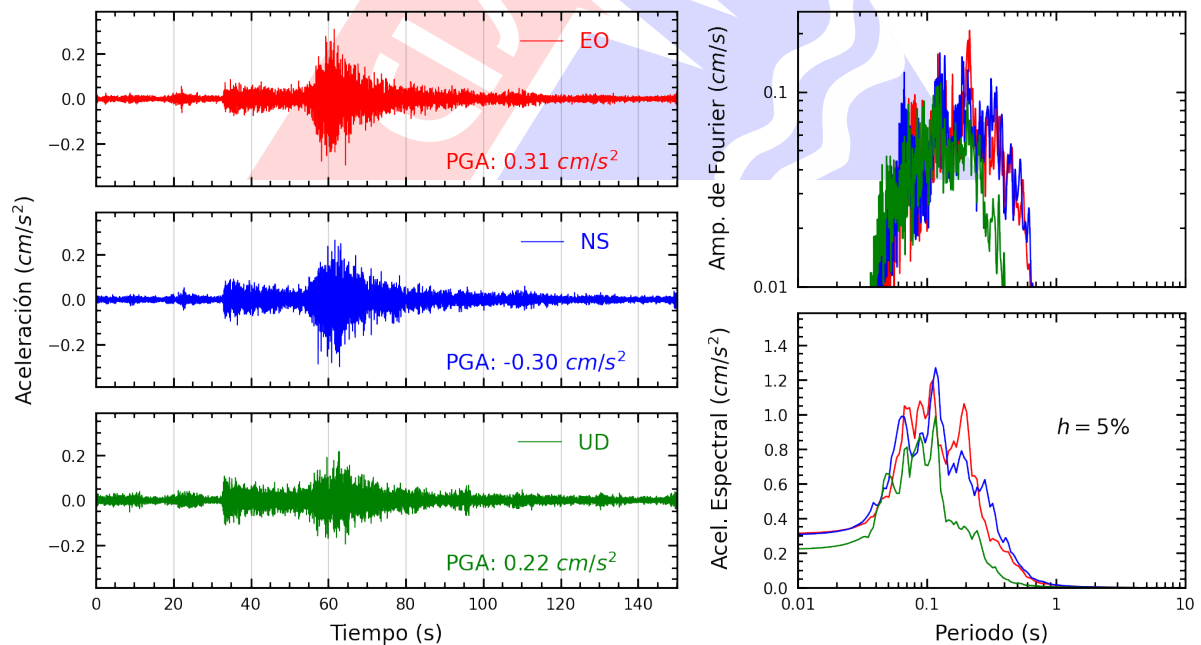
Figura A.30: Registros tiempo-historia, espectros de Fourier y de respuesta en las direcciones EO, NS y vertical de la estación VHAY2. Sismo de Lunahuana, Cañete - Lima del 2025-03-29, 14:53:31 (Hora local)
