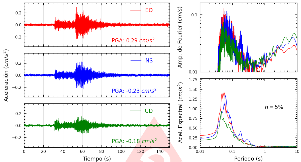
Figura A.31: Registros tiempo-historia, espectros de Fourier y de respuesta en las direcciones EO, NS y vertical de la estación UCSS. Sismo de Lunahuana, Cañete - Lima del 2025-03-29, 14:53:31 (Hora local)
