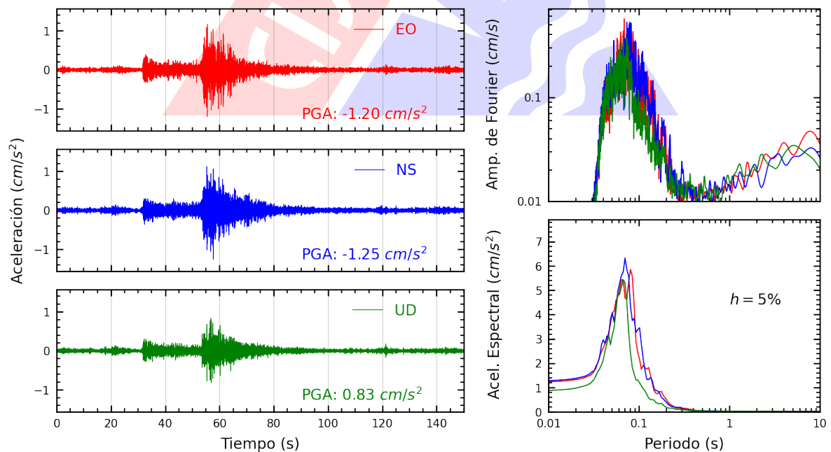
Figura A.8: Registros tiempo-historia, espectros de Fourier y de respuesta en las direcciones EO, NS y vertical de la estación JOSEO. Sismo de Lunahuana, Cañete - Lima del 2025-03-29, 14:53:31 (Hora local)
