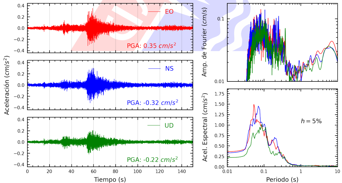
Figura A.28: Registros tiempo-historia, espectros de Fourier y de respuesta en las direcciones EO, NS y vertical de la estación COMAS. Sismo de Lunahuana, Cañete - Lima del 2025-03-29, 14:53:31 (Hora local)
