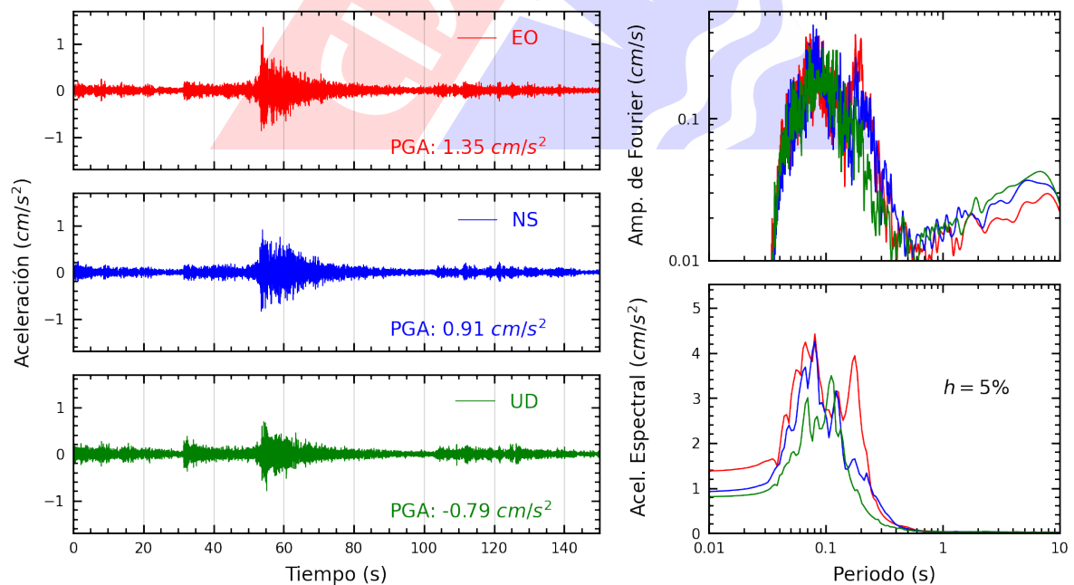
Figura A.6: Registros tiempo-historia, espectros de Fourier y de respuesta en las direcciones EO, NS y vertical de la estación INDEP. Sismo de Lunahuana, Cañete - Lima del 2025-03-29, 14:53:31 (Hora local)
