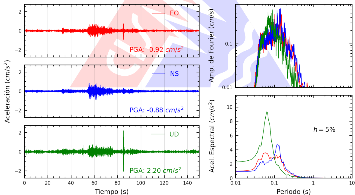
Figura A.2: Registros tiempo-historia, espectros de Fourier y de respuesta en las direcciones EO, NS y vertical de la estación CARA2. Sismo de Lunahuana, Cañete - Lima del 2025-03-29, 14:53:31 (Hora local)
