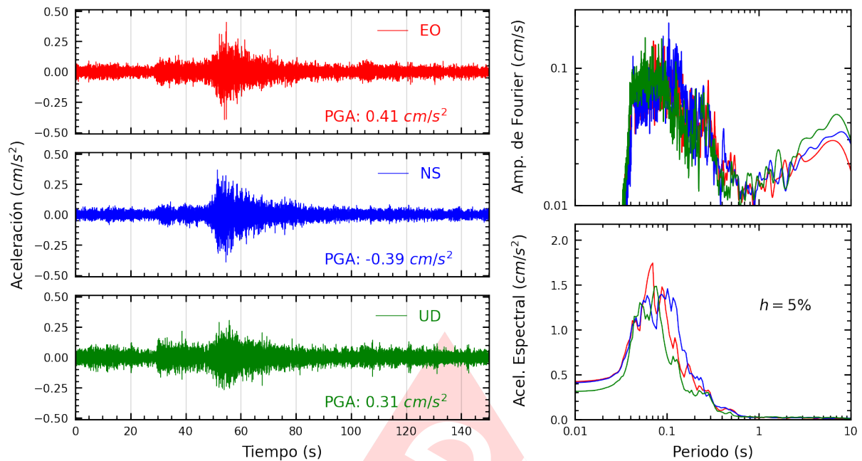
Figura A.23: Registros tiempo-historia, espectros de Fourier y de respuesta en las direcciones EO, NS y vertical de la estación URPPE. Sismo de Lunahuana, Cañete - Lima del 2025-03-29, 14:53:31 (Hora local)
