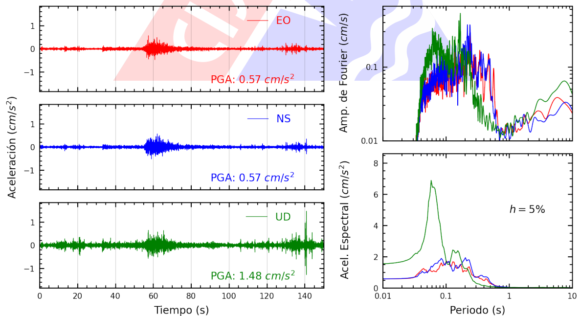
Figura A.4: Registros tiempo-historia, espectros de Fourier y de respuesta en las direcciones EO, NS y vertical de la estación MDPP. Sismo de Lunahuana, Cañete - Lima del 2025-03-29, 14:53:31 (Hora local)
