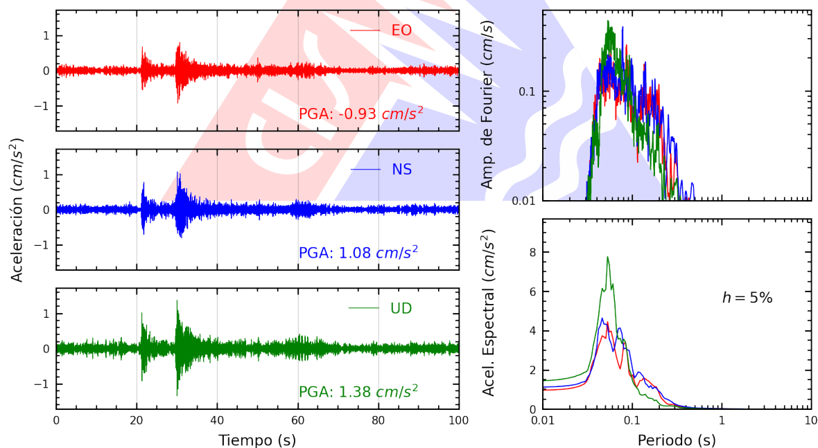
Figura A.2: Registros tiempo-historia, espectros de Fourier y de respuesta en las direcciones EO, NS y vertical de la estación SCAR2. Sismo de Quilca, Camana - Arequipa del 2025-03-30, 00:43:18 (Hora local)
