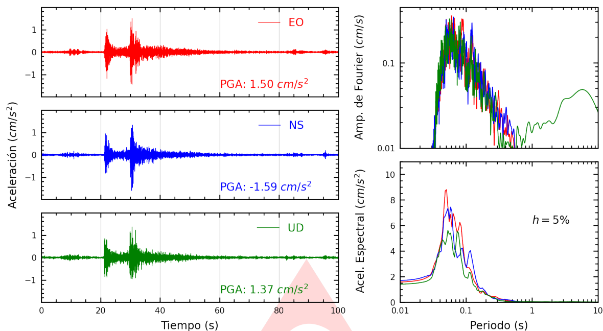
Figura A.1: Registros tiempo-historia, espectros de Fourier y de respuesta en las direcciones EO, NS y vertical de la estación SCARQ. Sismo de Quilca, Camana - Arequipa del 2025-03-30, 00:43:18 (Hora local)
