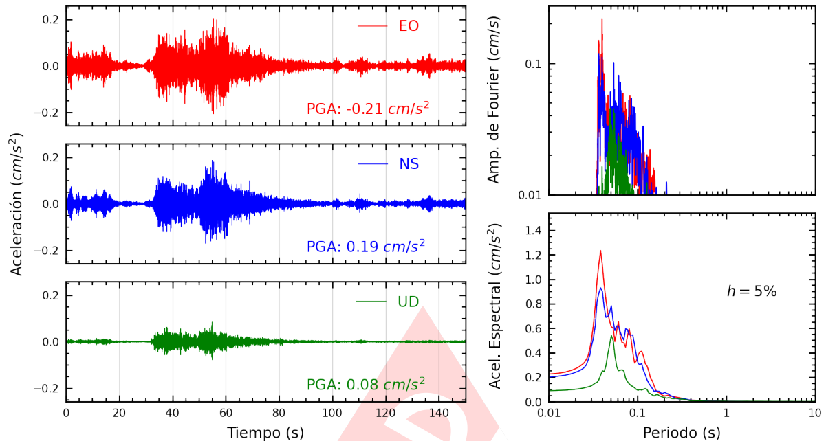
Figura A.3: Registros tiempo-historia, espectros de Fourier y de respuesta en las direcciones EO, NS y vertical de la estación UNAM. Sismo de Quilca, Camana - Arequipa del 2025-03-30, 00:43:18 (Hora local)
