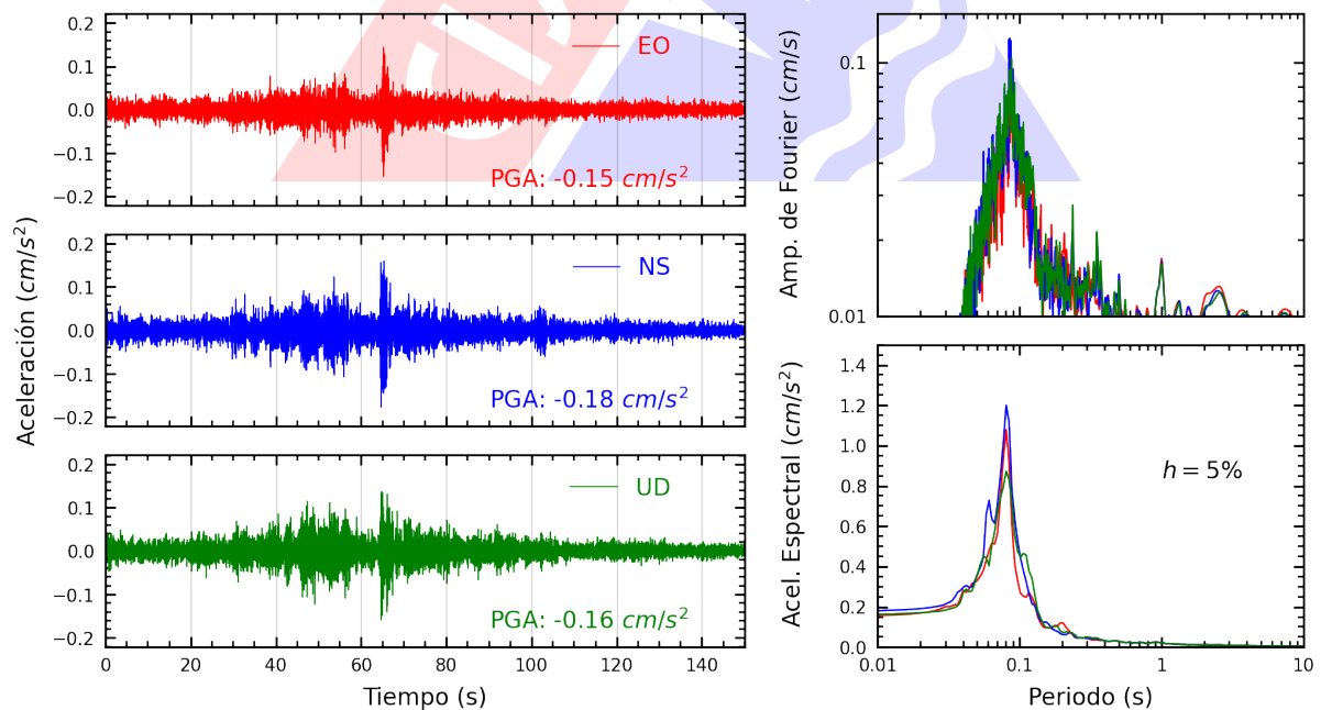
Figura A.4: Registros tiempo-historia, espectros de Fourier y de respuesta en las direcciones EO, NS y vertical de la estación UNICA. Sismo de Quilca, Camana - Arequipa del 2025-03-30, 00:43:18 (Hora local)
