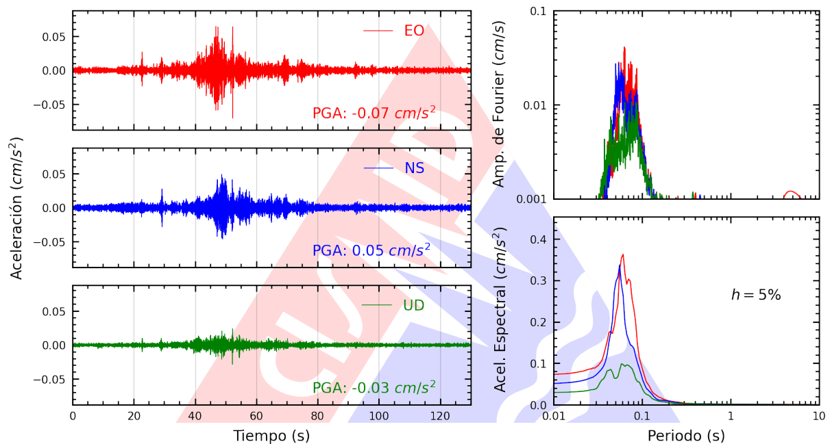
Figura A.5: Registros tiempo-historia, espectros de Fourier y de respuesta en las direcciones EO, NS y vertical de la estación UNMBA. Sismo de Quilca, Camana - Arequipa del 2025-03-30, 00:43:18 (Hora local)
