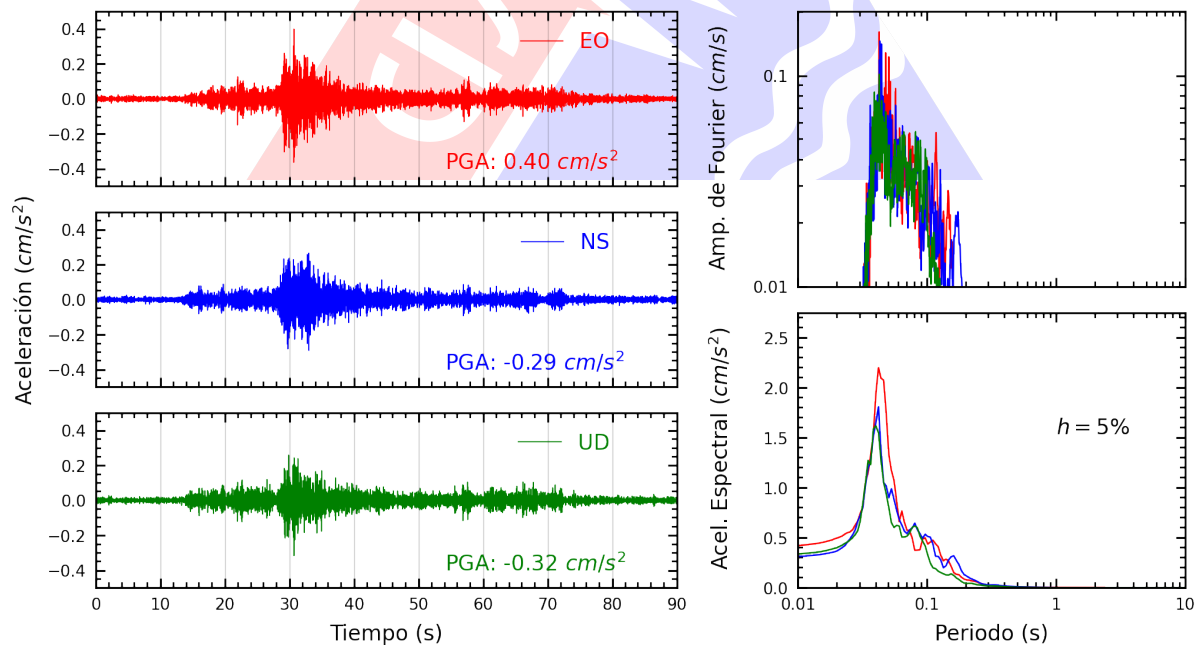
Figura A.18: Registros tiempo-historia, espectros de Fourier y de respuesta en las direcciones EO, NS y vertical de la estación SROS2. Sismo de Chilca, Cañete - Lima del 2025-03-30, 03:04:16 (Hora local)
