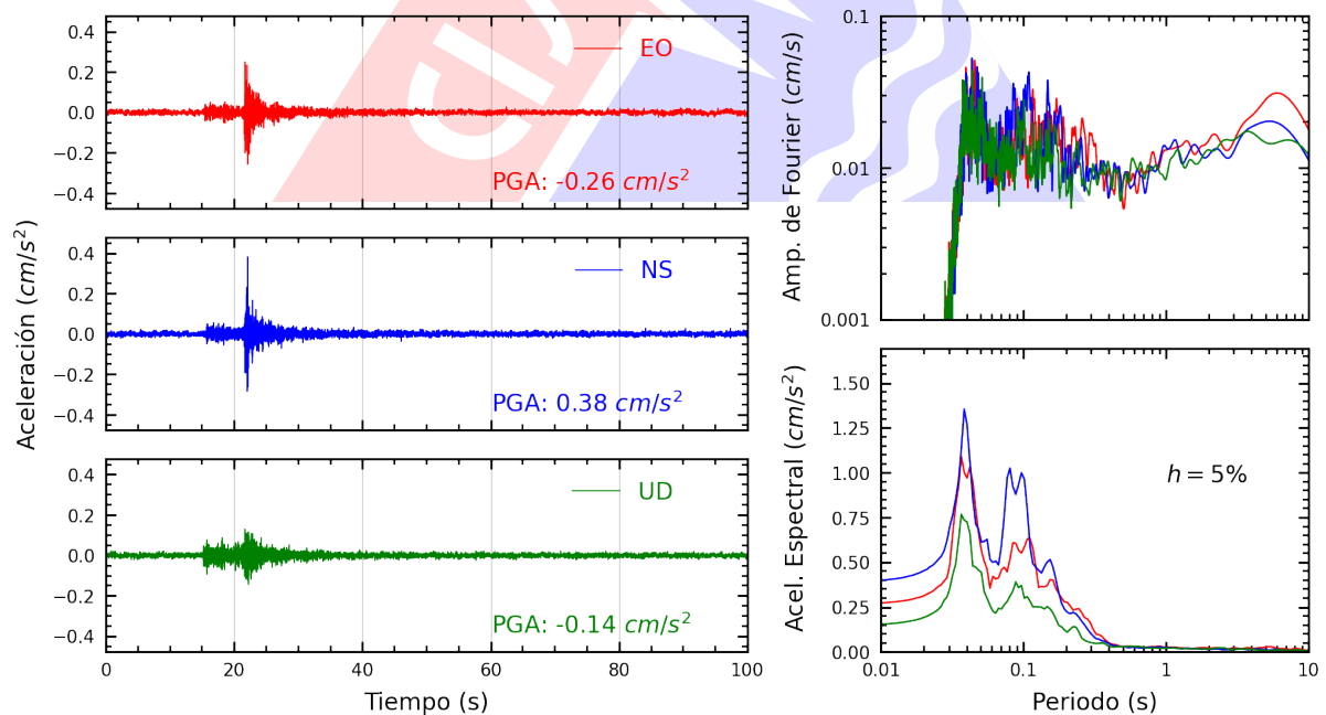
Figura A.20: Registros tiempo-historia, espectros de Fourier y de respuesta en las direcciones EO, NS y vertical de la estación SERVI. Sismo de Chilca, Cañete - Lima del 2025-03-30, 03:04:16 (Hora local)
