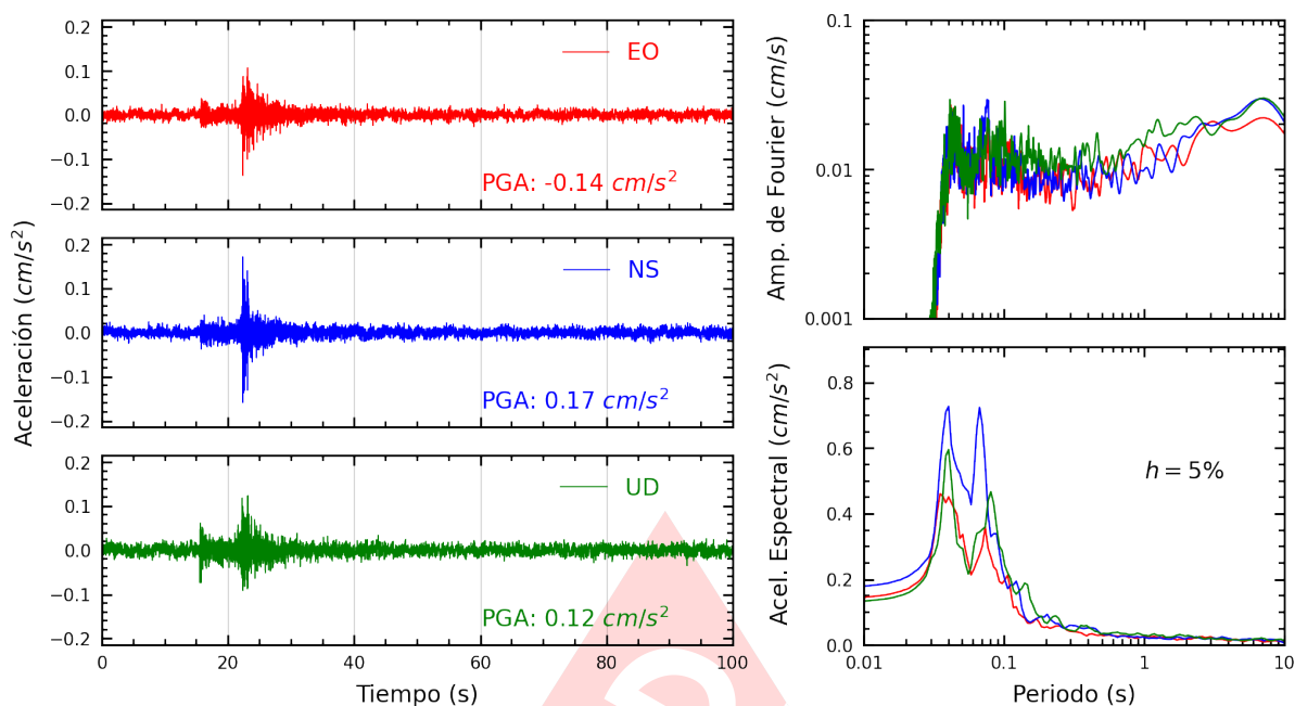
Figura A.29: Registros tiempo-historia, espectros de Fourier y de respuesta en las direcciones EO, NS y vertical de la estación UNFV. Sismo de Chilca, Cañete - Lima del 2025-03-30, 03:04:16 (Hora local)
