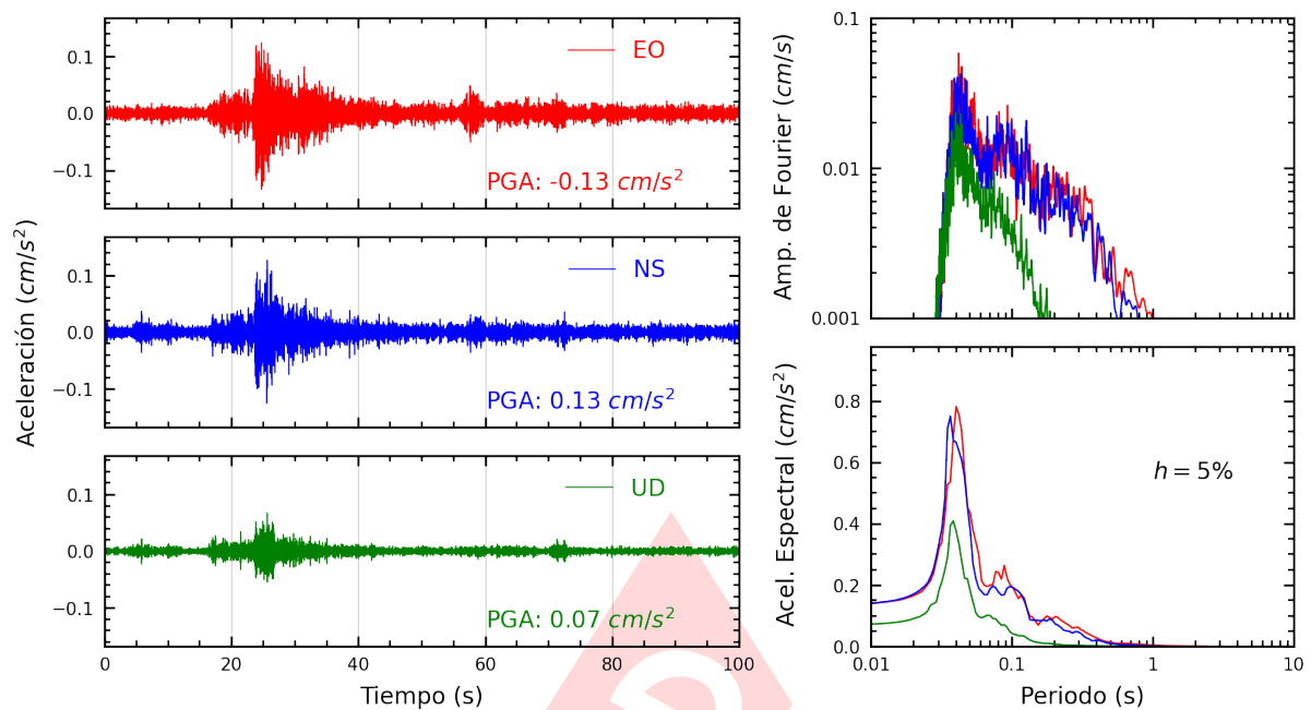
Figura A.33: Registros tiempo-historia, espectros de Fourier y de respuesta en las direcciones EO, NS y vertical de la estación UCVA2. Sismo de Chilca, Cañete - Lima del 2025-03-30, 03:04:16 (Hora local)
