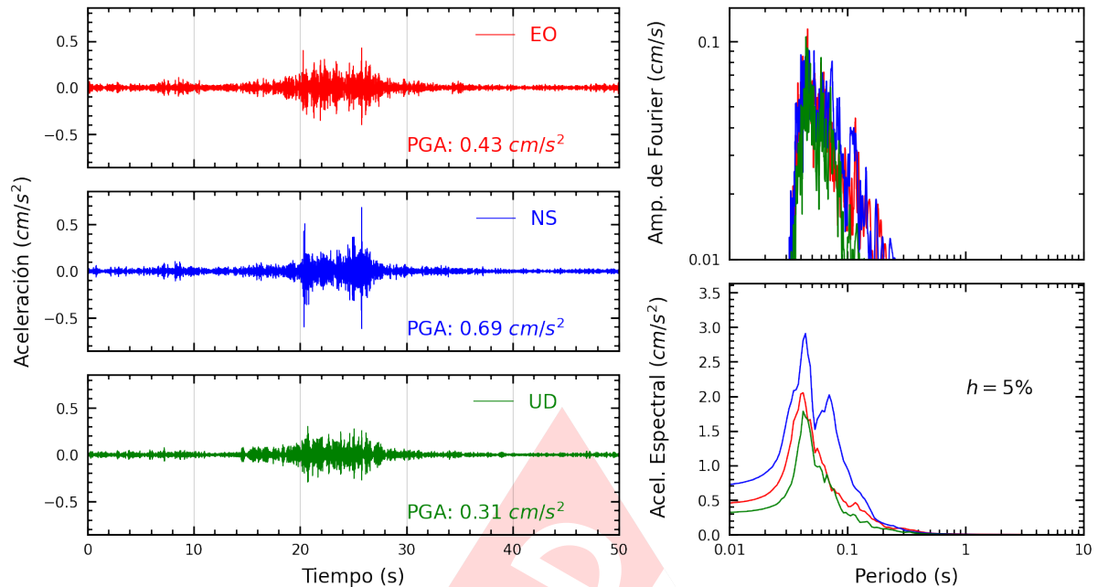
Figura A.7: Registros tiempo-historia, espectros de Fourier y de respuesta en las direcciones EO, NS y vertical de la estación PACHA. Sismo de Chilca, Cañete - Lima del 2025-03-30, 03:04:16 (Hora local)
