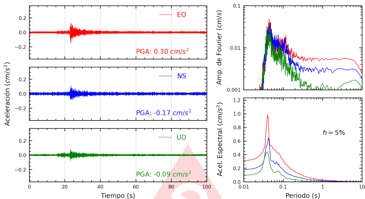
Figura A.21: Registros tiempo-historia, espectros de Fourier y de respuesta en las direcciones EO, NS y vertical de la estación ATARJ. Sismo de Chilca, Cañete - Lima del 2025-03-30, 03:04:16 (Hora local)
