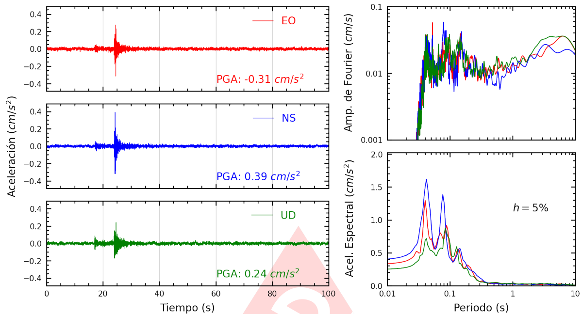
Figura A.19: Registros tiempo-historia, espectros de Fourier y de respuesta en las direcciones EO, NS y vertical de la estación UNMSM. Sismo de Chilca, Cañete - Lima del 2025-03-30, 03:04:16 (Hora local)
