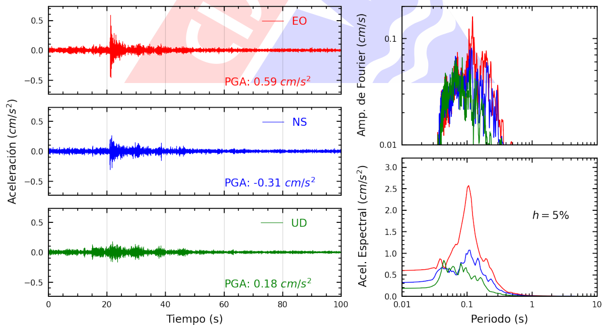
Figura A.8: Registros tiempo-historia, espectros de Fourier y de respuesta en las direcciones EO, NS y vertical de la estación SCCHO. Sismo de Chilca, Cañete - Lima del 2025-03-30, 03:04:16 (Hora local)
