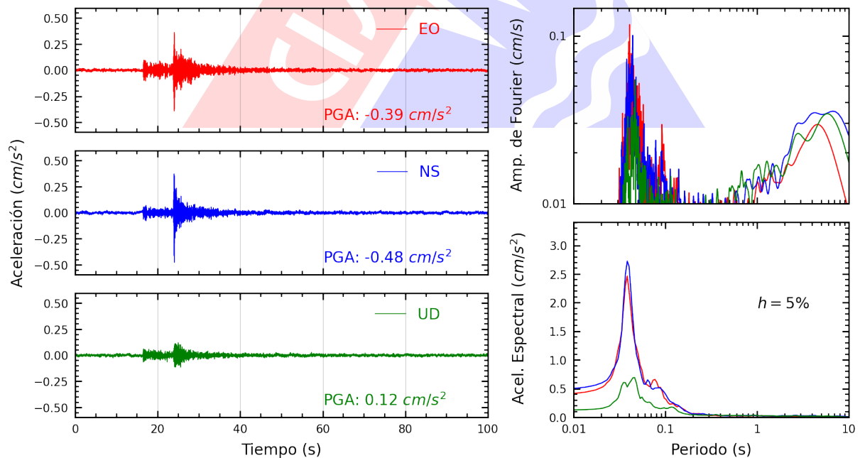
Figura A.12: Registros tiempo-historia, espectros de Fourier y de respuesta en las direcciones EO, NS y vertical de la estación UCSS. Sismo de Chilca, Cañete - Lima del 2025-03-30, 03:04:16 (Hora local)
