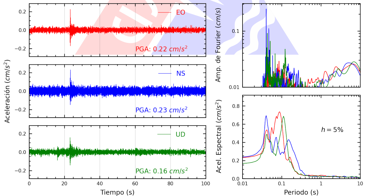
Figura A.26: Registros tiempo-historia, espectros de Fourier y de respuesta en las direcciones EO, NS y vertical de la estación BONDY. Sismo de Chilca, Cañete - Lima del 2025-03-30, 03:04:16 (Hora local)
