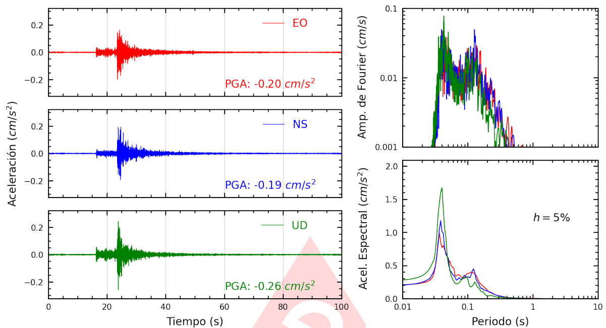
Figura A.23: Registros tiempo-historia, espectros de Fourier y de respuesta en las direcciones EO, NS y vertical de la estación JALV2. Sismo de Chilca, Cañete - Lima del 2025-03-30, 03:04:16 (Hora local)
