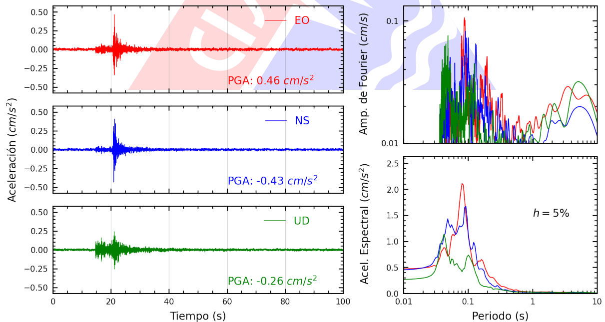
Figura A.14: Registros tiempo-historia, espectros de Fourier y de respuesta en las direcciones EO, NS y vertical de la estación USILP. Sismo de Chilca, Cañete - Lima del 2025-03-30, 03:04:16 (Hora local)
