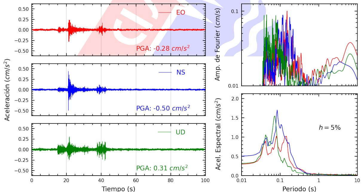
Figura A.10: Registros tiempo-historia, espectros de Fourier y de respuesta en las direcciones EO, NS y vertical de la estación SOCHO. Sismo de Chilca, Cañete - Lima del 2025-03-30, 03:04:16 (Hora local)
