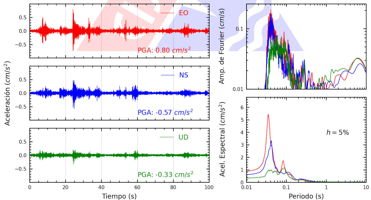
Figura A.4: Registros tiempo-historia, espectros de Fourier y de respuesta en las direcciones EO, NS y vertical de la estación OLIVO. Sismo de Chilca, Cañete - Lima del 2025-03-30, 03:04:16 (Hora local)
