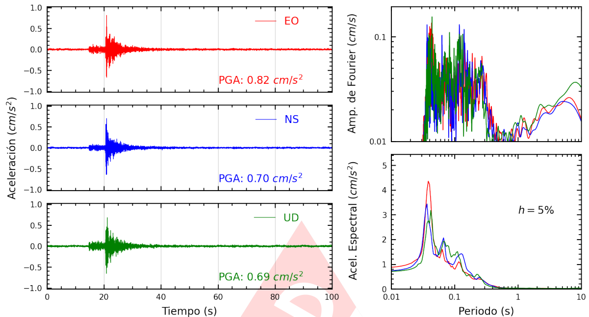
Figura A.3: Registros tiempo-historia, espectros de Fourier y de respuesta en las direcciones EO, NS y vertical de la estación SOVES. Sismo de Chilca, Cañete - Lima del 2025-03-30, 03:04:16 (Hora local)
