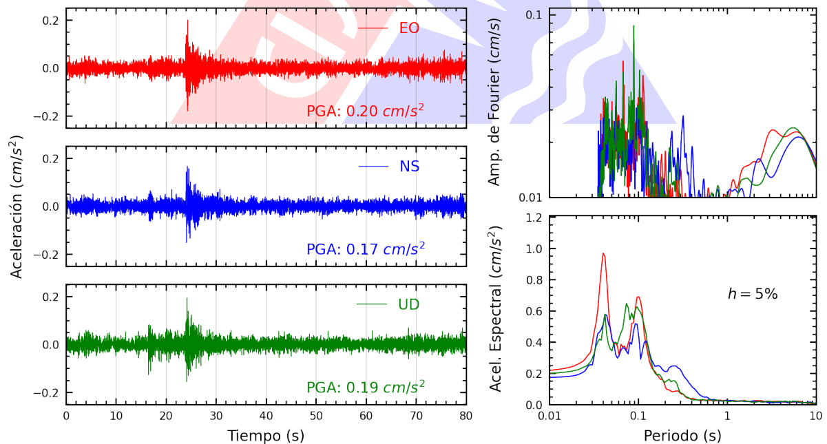
Figura A.28: Registros tiempo-historia, espectros de Fourier y de respuesta en las direcciones EO, NS y vertical de la estación MADRE. Sismo de Chilca, Cañete - Lima del 2025-03-30, 03:04:16 (Hora local)
