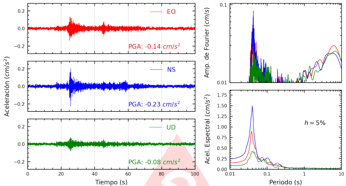
Figura A.27: Registros tiempo-historia, espectros de Fourier y de respuesta en las direcciones EO, NS y vertical de la estación COMAS. Sismo de Chilca, Cañete - Lima del 2025-03-30, 03:04:16 (Hora local)
