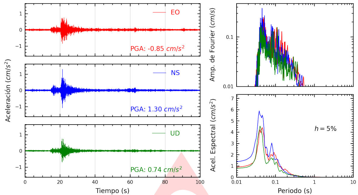
Figura A.1: Registros tiempo-historia, espectros de Fourier y de respuesta en las direcciones EO, NS y vertical de la estación UNTEL. Sismo de Chilca, Cañete - Lima del 2025-03-30, 03:04:16 (Hora local)
