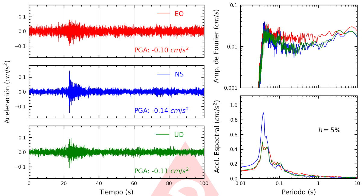
Figura A.31: Registros tiempo-historia, espectros de Fourier y de respuesta en las direcciones EO, NS y vertical de la estación IMCA. Sismo de Chilca, Cañete - Lima del 2025-03-30, 03:04:16 (Hora local)
