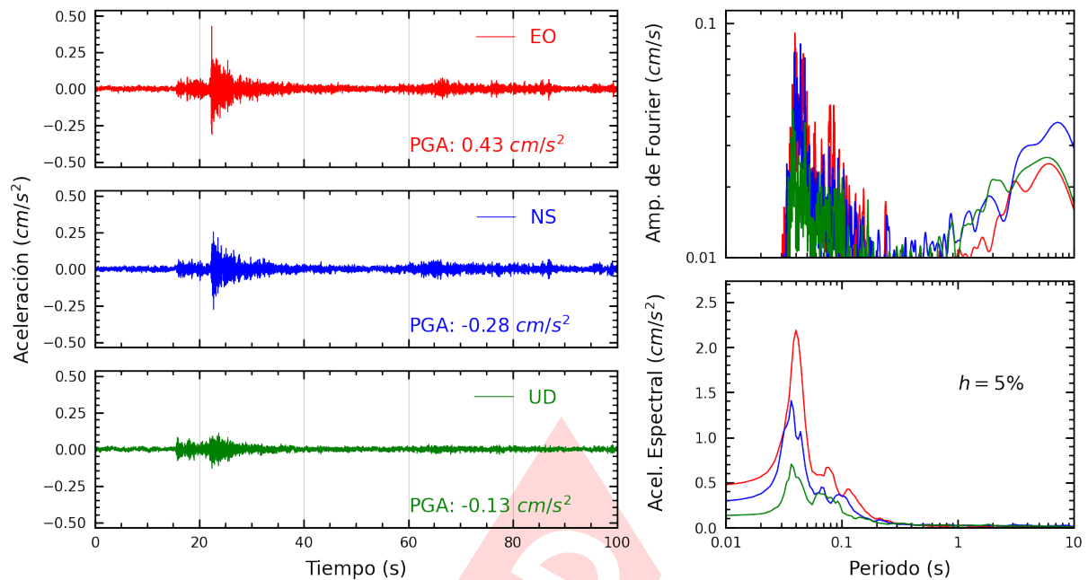
Figura A.15: Registros tiempo-historia, espectros de Fourier y de respuesta en las direcciones EO, NS y vertical de la estación CEPRE. Sismo de Chilca, Cañete - Lima del 2025-03-30, 03:04:16 (Hora local)
