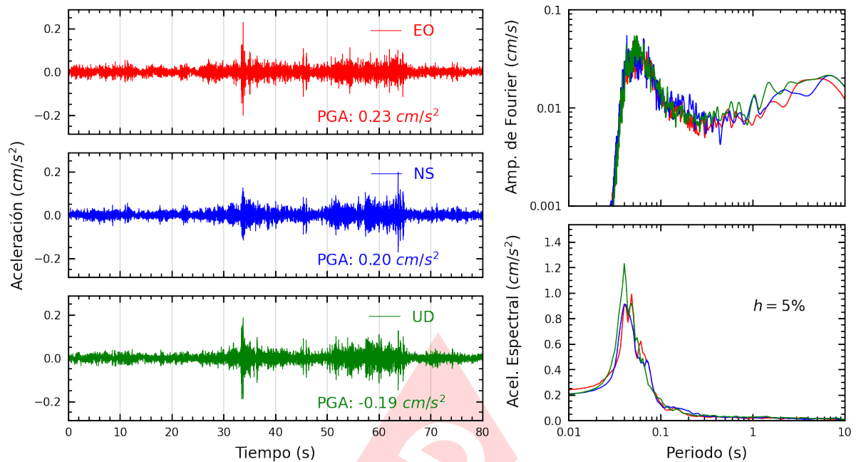
Figura A.25: Registros tiempo-historia, espectros de Fourier y de respuesta en las direcciones EO, NS y vertical de la estación PRADO. Sismo de Chilca, Cañete - Lima del 2025-03-30, 03:04:16 (Hora local)
