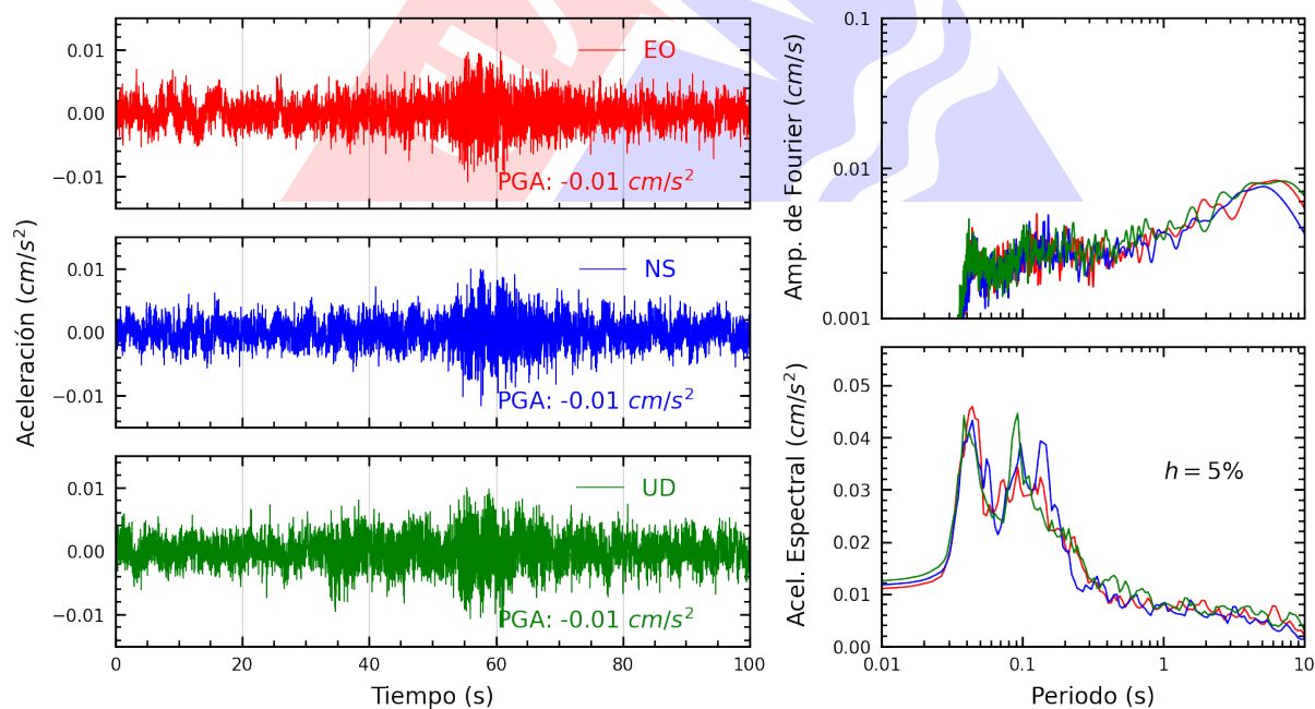
Figura A.36: Registros tiempo-historia, espectros de Fourier y de respuesta en las direcciones EO, NS y vertical de la estación CARAL. Sismo de Chilca, Cañete - Lima del 2025-03-30, 03:04:16 (Hora local)
