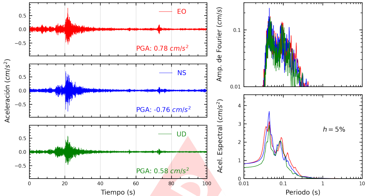
Figura A.5: Registros tiempo-historia, espectros de Fourier y de respuesta en las direcciones EO, NS y vertical de la estación PHER2. Sismo de Chilca, Cañete - Lima del 2025-03-30, 03:04:16 (Hora local)
