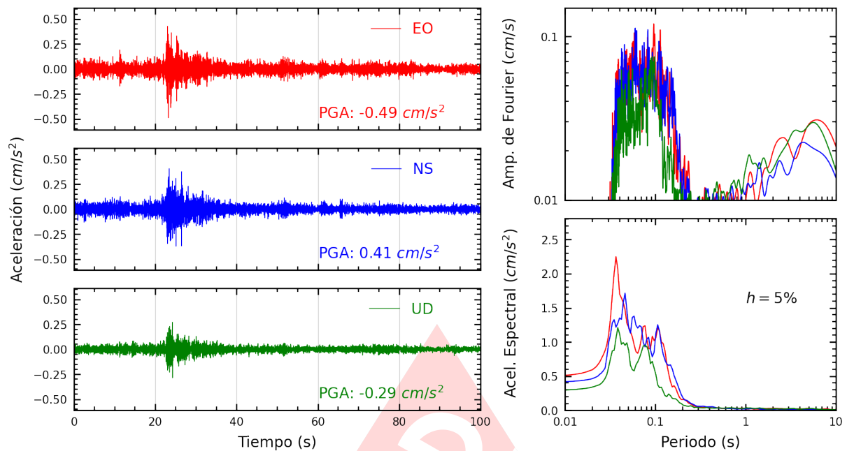
Figura A.11: Registros tiempo-historia, espectros de Fourier y de respuesta en las direcciones EO, NS y vertical de la estación USILM. Sismo de Chilca, Cañete - Lima del 2025-03-30, 03:04:16 (Hora local)
