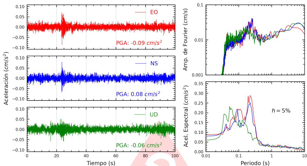
Figura A.35: Registros tiempo-historia, espectros de Fourier y de respuesta en las direcciones EO, NS y vertical de la estación DSMI. Sismo de Chilca, Cañete - Lima del 2025-03-30, 03:04:16 (Hora local)
