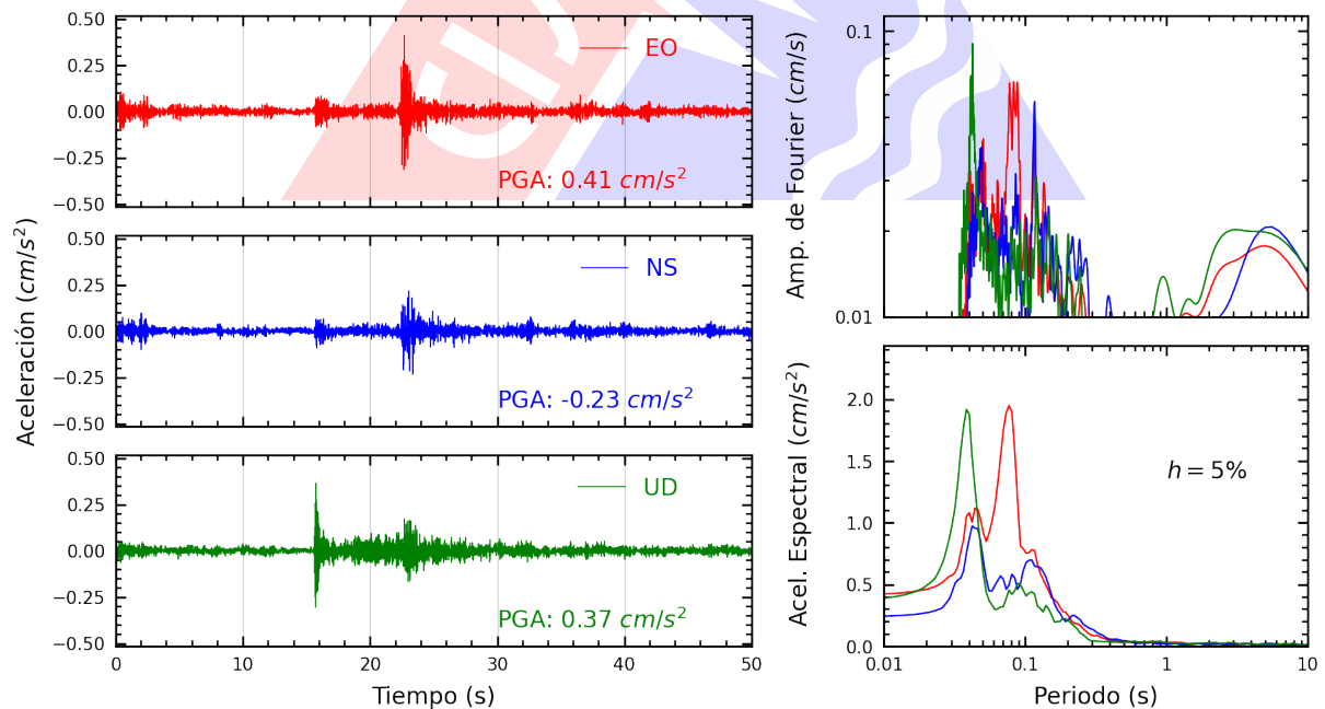
Figura A.16: Registros tiempo-historia, espectros de Fourier y de respuesta en las direcciones EO, NS y vertical de la estación UPCSM. Sismo de Chilca, Cañete - Lima del 2025-03-30, 03:04:16 (Hora local)
