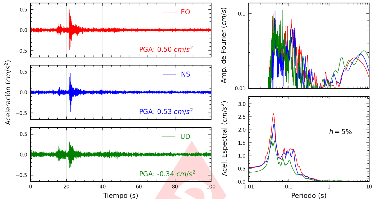
Figura A.9: Registros tiempo-historia, espectros de Fourier y de respuesta en las direcciones EO, NS y vertical de la estación URPE. Sismo de Chilca, Cañete - Lima del 2025-03-30, 03:04:16 (Hora local)
