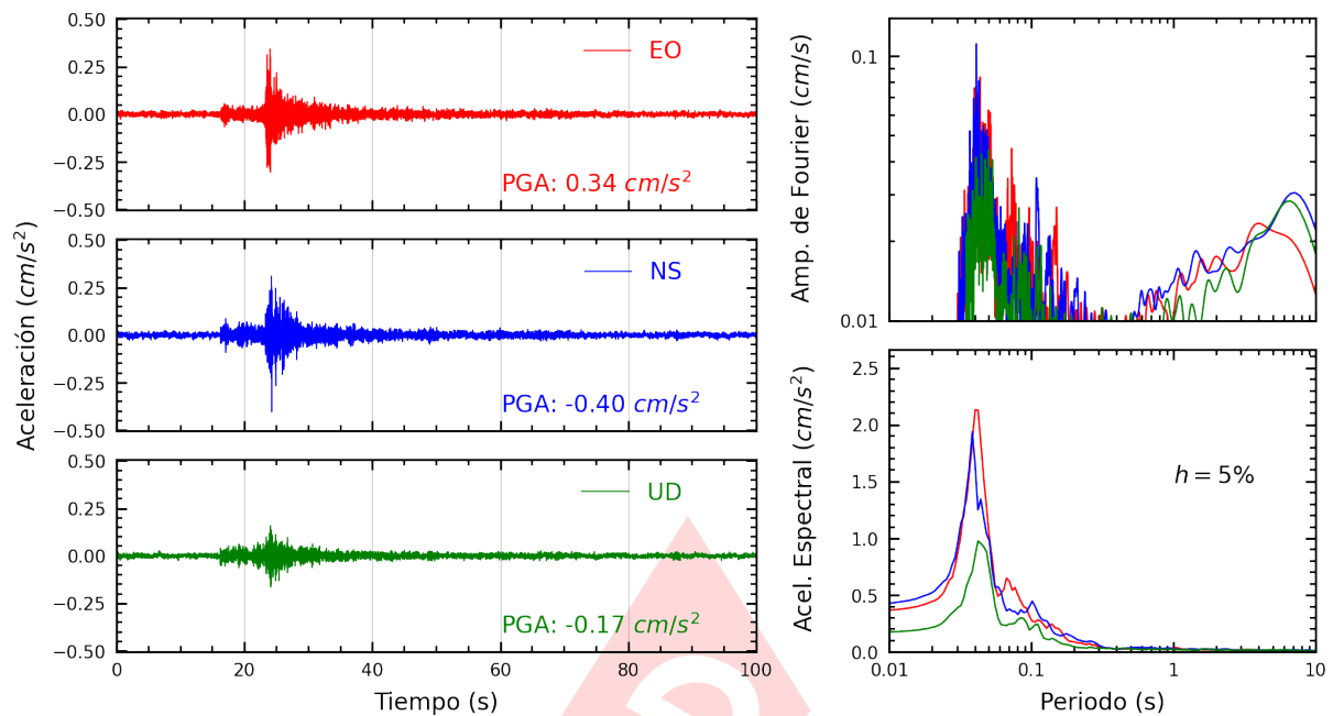
Figura A.17: Registros tiempo-historia, espectros de Fourier y de respuesta en las direcciones EO, NS y vertical de la estación FICPE. Sismo de Chilca, Cañete - Lima del 2025-03-30, 03:04:16 (Hora local)
