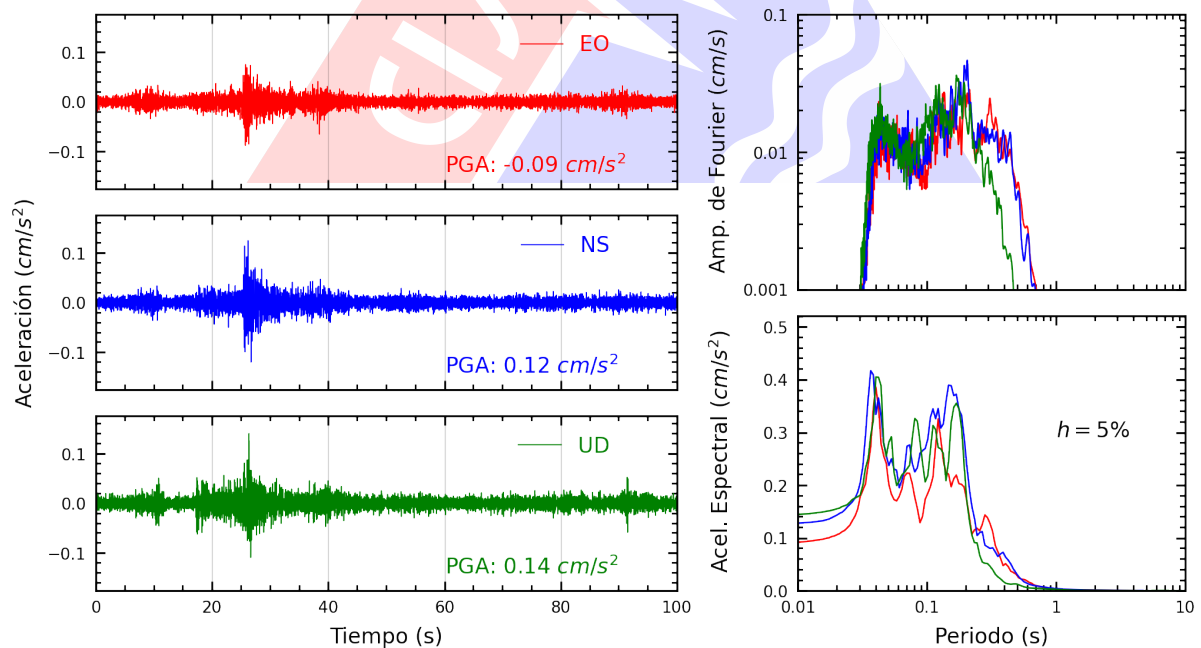
Figura A.32: Registros tiempo-historia, espectros de Fourier y de respuesta en las direcciones EO, NS y vertical de la estación VHAY2. Sismo de Chilca, Cañete - Lima del 2025-03-30, 03:04:16 (Hora local)
