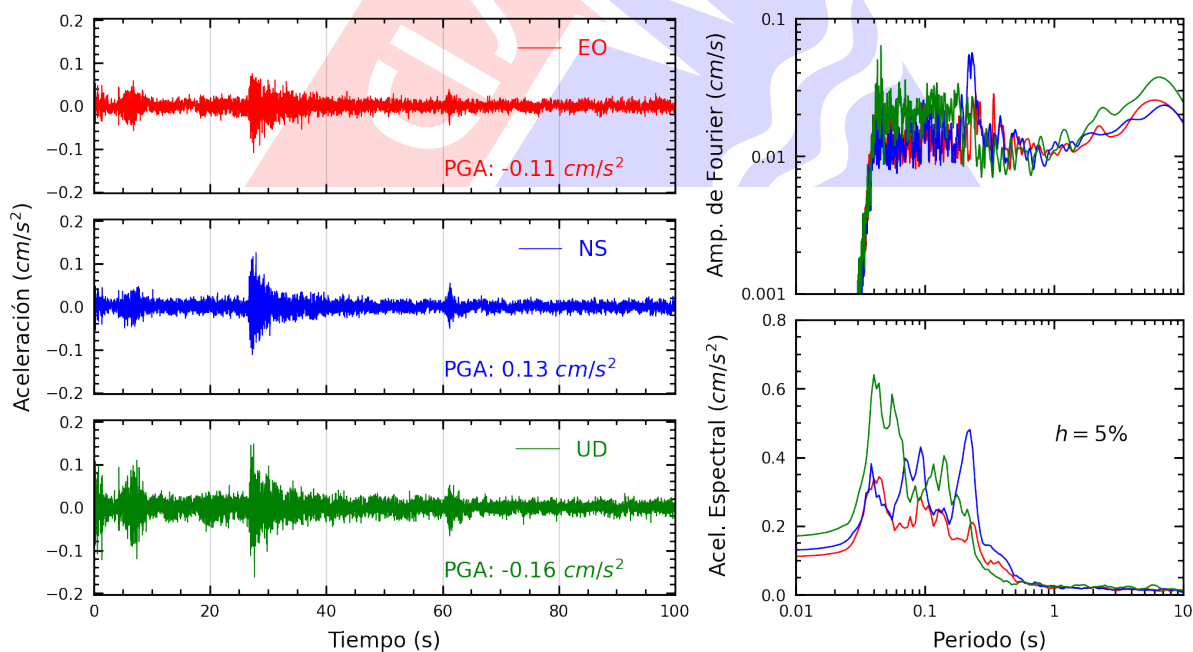
Figura A.30: Registros tiempo-historia, espectros de Fourier y de respuesta en las direcciones EO, NS y vertical de la estación MDPP. Sismo de Chilca, Cañete - Lima del 2025-03-30, 03:04:16 (Hora local)
