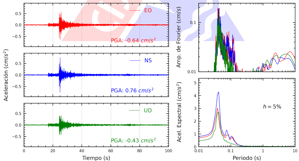
Figura A.6: Registros tiempo-historia, espectros de Fourier y de respuesta en las direcciones EO, NS y vertical de la estación JOSEO. Sismo de Chilca, Cañete - Lima del 2025-03-30, 03:04:16 (Hora local)
