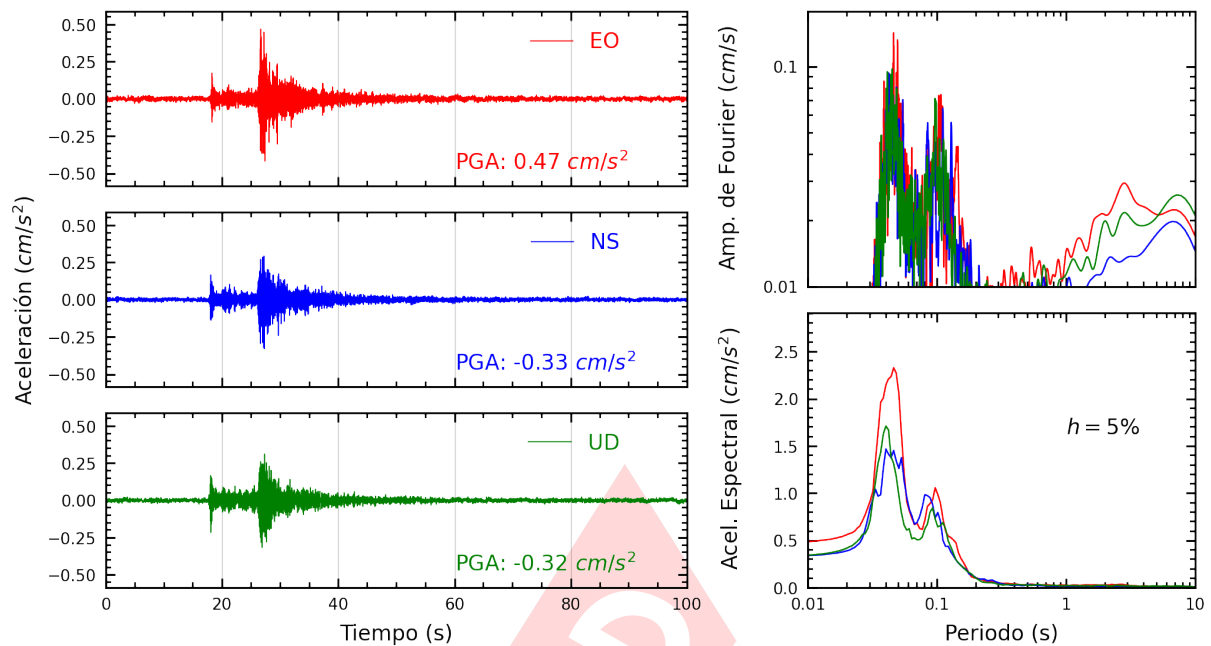
Figura A.13: Registros tiempo-historia, espectros de Fourier y de respuesta en las direcciones EO, NS y vertical de la estación AMORE. Sismo de Chilca, Cañete - Lima del 2025-03-30, 03:04:16 (Hora local)
