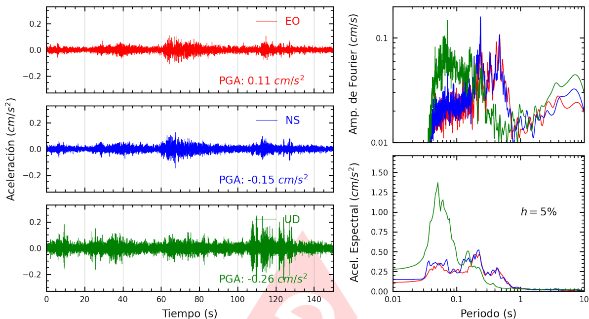
Figura A.3: Registros tiempo-historia, espectros de Fourier y de respuesta en las direcciones EO, NS y vertical de la estación MDPP. Sismo de San Martín De Pangoa, Satipo - Junín del 2025-03-30, 23:50:25 (Hora local)
