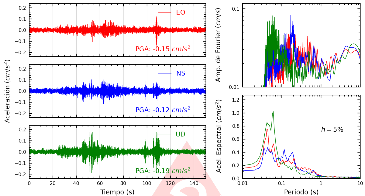
Figura A.5: Registros tiempo-historia, espectros de Fourier y de respuesta en las direcciones EO, NS y vertical de la estación SOCHO. Sismo de San Martín De Pangoa, Satipo - Junín del 2025-03-30, 23:50:25 (Hora local)
