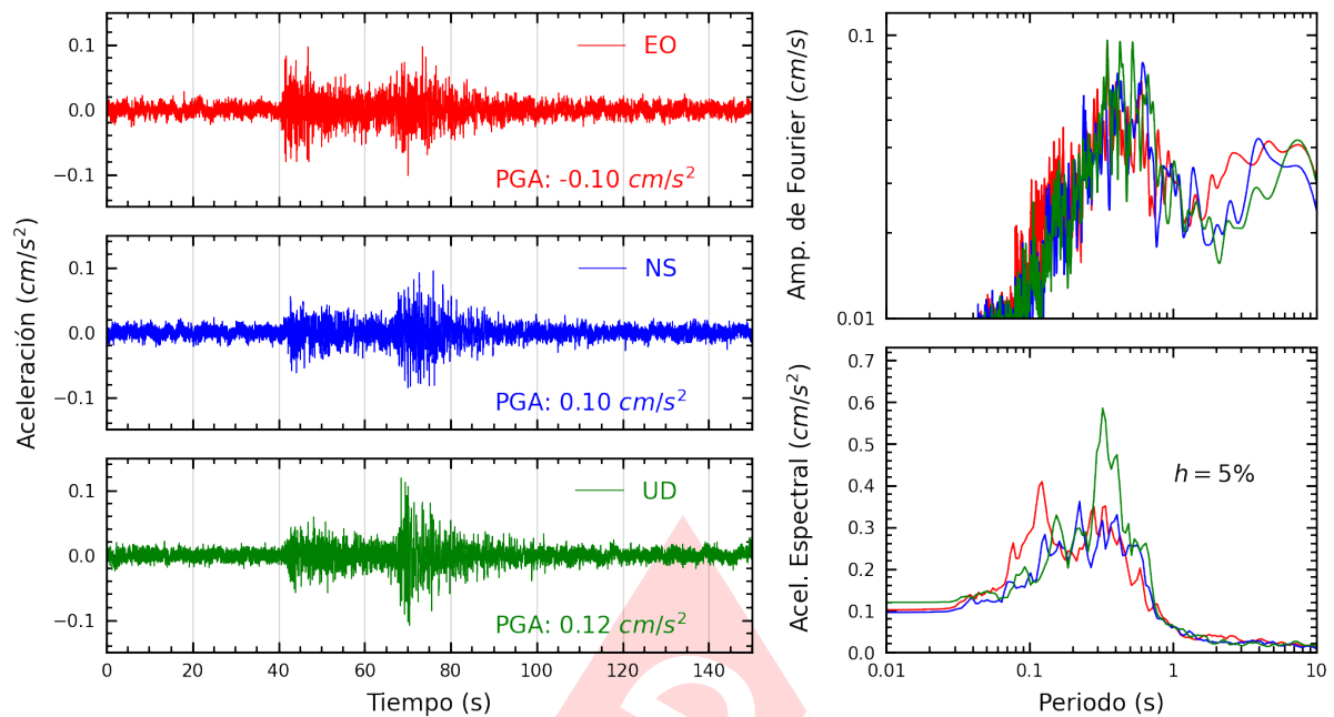
Figura A.13: Registros tiempo-historia, espectros de Fourier y de respuesta en las direcciones EO, NS y vertical de la estación UNSCH. Sismo de San Martín De Pangoa, Satipo - Junín del 2025-03-30, 23:50:25 (Hora local)
