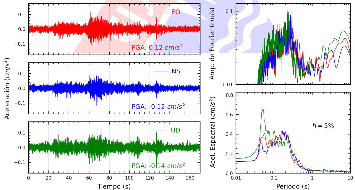
Figura A.10: Registros tiempo-historia, espectros de Fourier y de respuesta en las direcciones EO, NS y vertical de la estación SOVES. Sismo de San Martín De Pangoa, Satipo - Junín del 2025-03-30, 23:50:25 (Hora local)
