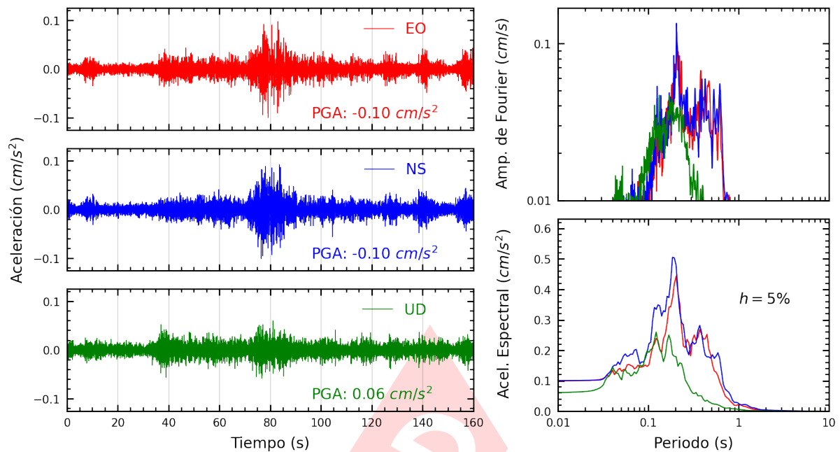
Figura A.17: Registros tiempo-historia, espectros de Fourier y de respuesta en las direcciones EO, NS y vertical de la estación VHAY2. Sismo de San Martín De Pangoa, Satipo - Junín del 2025-03-30, 23:50:25 (Hora local)
