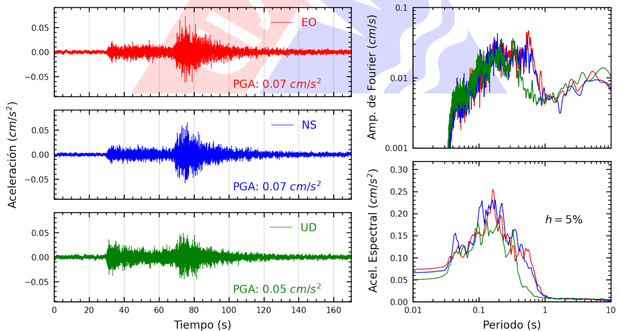
Figura A.20: Registros tiempo-historia, espectros de Fourier y de respuesta en las direcciones EO, NS y vertical de la estación CARAL. Sismo de San Martín De Pangoa, Satipo - Junín del 2025-03-30, 23:50:25 (Hora local)
