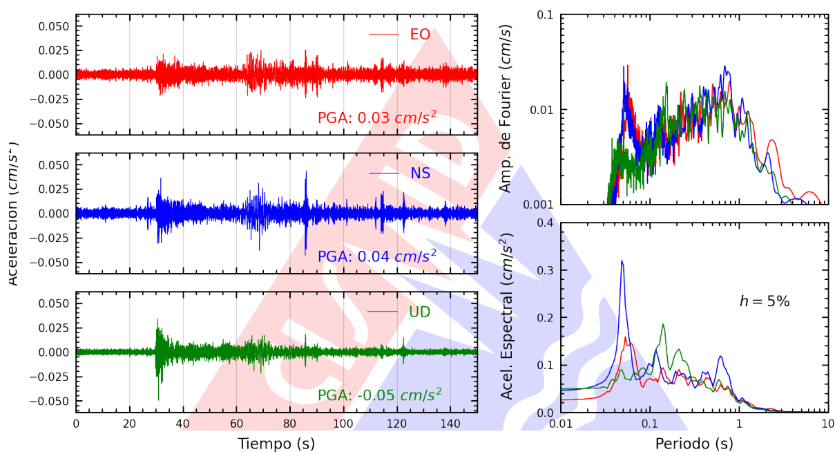
Figura A.23: Registros tiempo-historia, espectros de Fourier y de respuesta en las direcciones EO, NS y vertical de la estación UNMBA. Sismo de San Martín De Pangoa, Satipo - Junín del 2025-03-30, 23:50:25 (Hora local)
