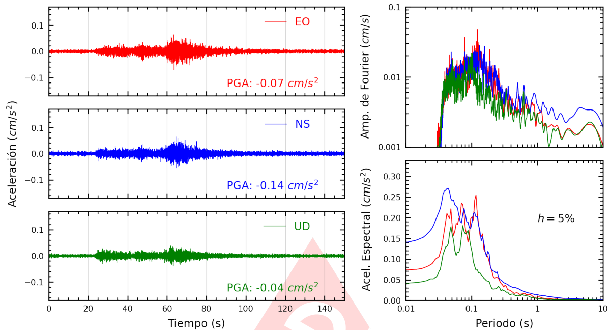
Figura A.11: Registros tiempo-historia, espectros de Fourier y de respuesta en las direcciones EO, NS y vertical de la estación ATARJ. Sismo de San Martín De Pangoa, Satipo - Junín del 2025-03-30, 23:50:25 (Hora local)
