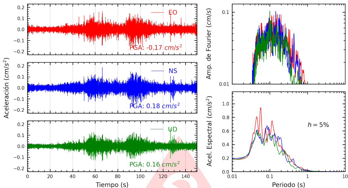
Figura A.7: Registros tiempo-historia, espectros de Fourier y de respuesta en las direcciones EO, NS y vertical de la estación PHER2. Sismo de San Martín De Pangoa, Satipo - Junín del 2025-03-30, 23:50:25 (Hora local)
