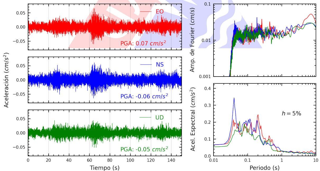
Figura A.22: Registros tiempo-historia, espectros de Fourier y de respuesta en las direcciones EO, NS y vertical de la estación COMAS. Sismo de San Martín De Pangoa, Satipo - Junín del 2025-03-30, 23:50:25 (Hora local)
