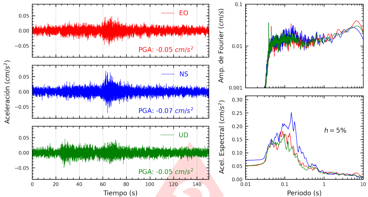
Figura A.21: Registros tiempo-historia, espectros de Fourier y de respuesta en las direcciones EO, NS y vertical de la estación SERVI. Sismo de San Martín De Pangoa, Satipo - Junín del 2025-03-30, 23:50:25 (Hora local)
