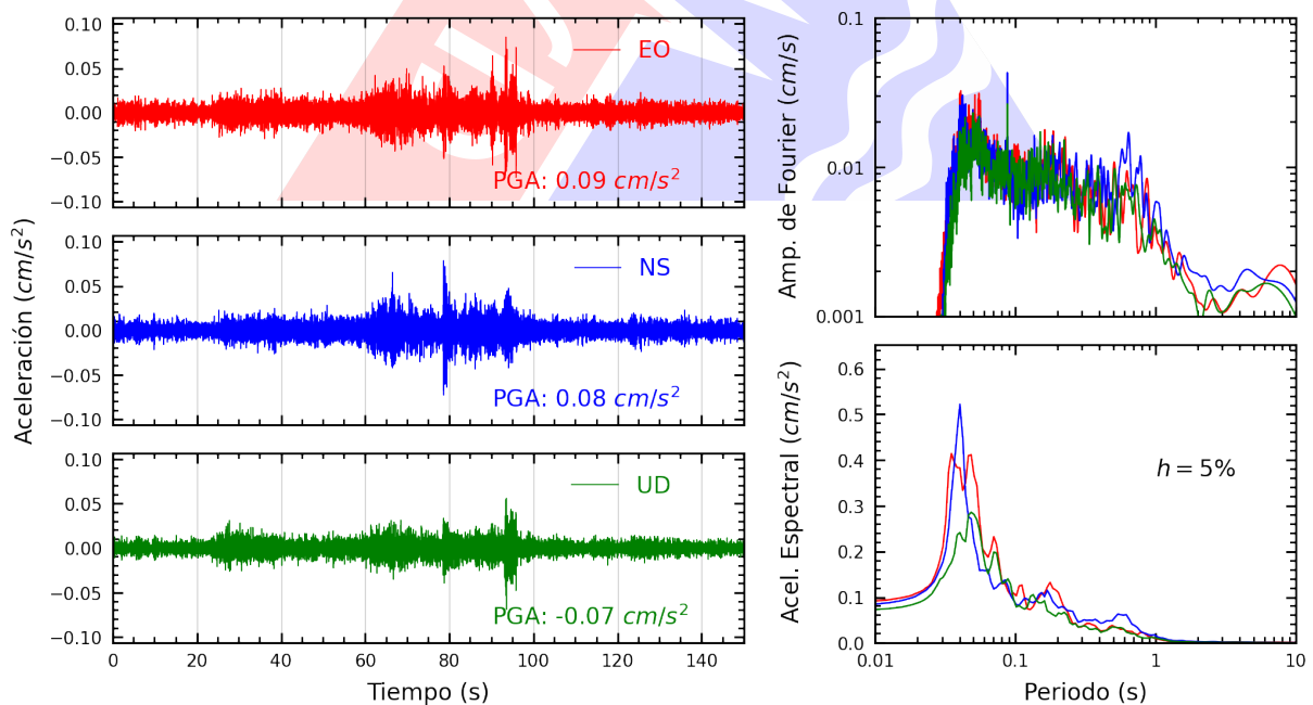
Figura A.18: Registros tiempo-historia, espectros de Fourier y de respuesta en las direcciones EO, NS y vertical de la estación BORJA. Sismo de San Martín De Pangoa, Satipo - Junín del 2025-03-30, 23:50:25 (Hora local)
