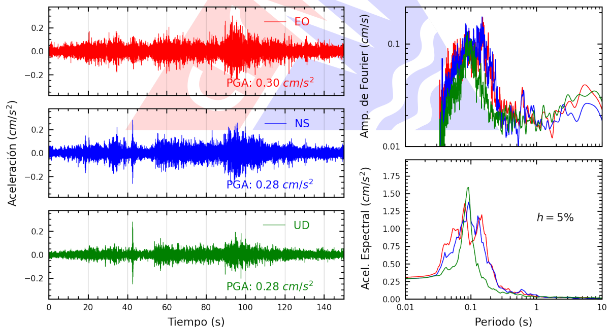
Figura A.2: Registros tiempo-historia, espectros de Fourier y de respuesta en las direcciones EO, NS y vertical de la estación USILM. Sismo de San Martín De Pangoa, Satipo - Junín del 2025-03-30, 23:50:25 (Hora local)
