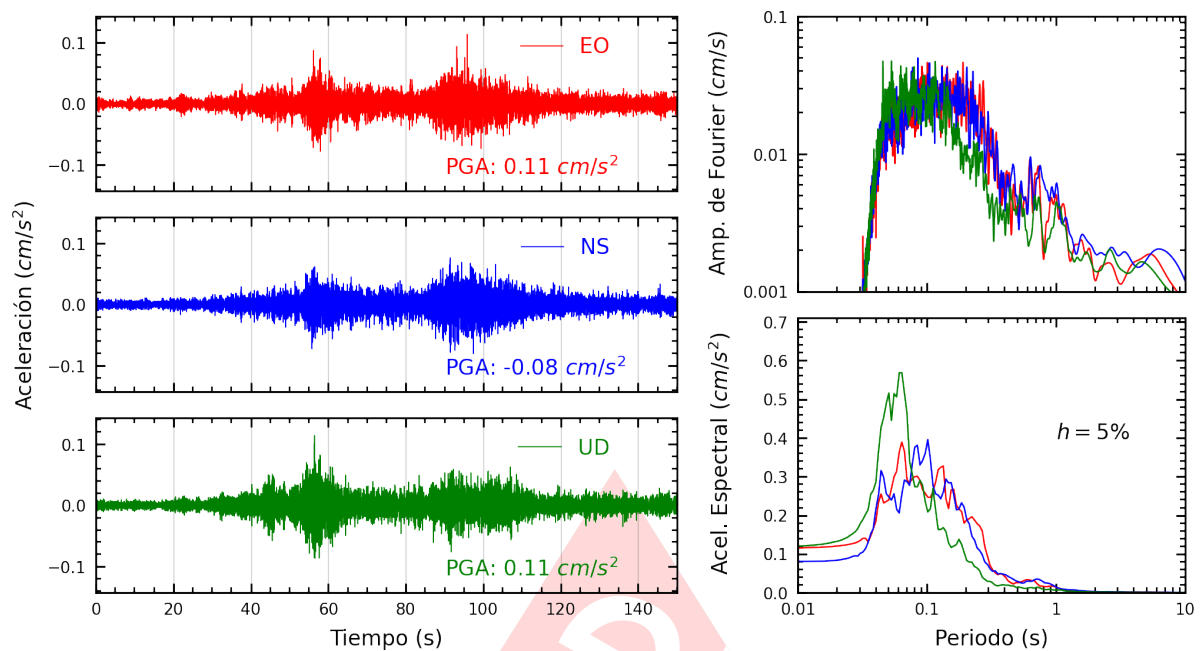
Figura A.15: Registros tiempo-historia, espectros de Fourier y de respuesta en las direcciones EO, NS y vertical de la estación ASIA. Sismo de San Martín De Pangoa, Satipo - Junín del 2025-03-30, 23:50:25 (Hora local)
