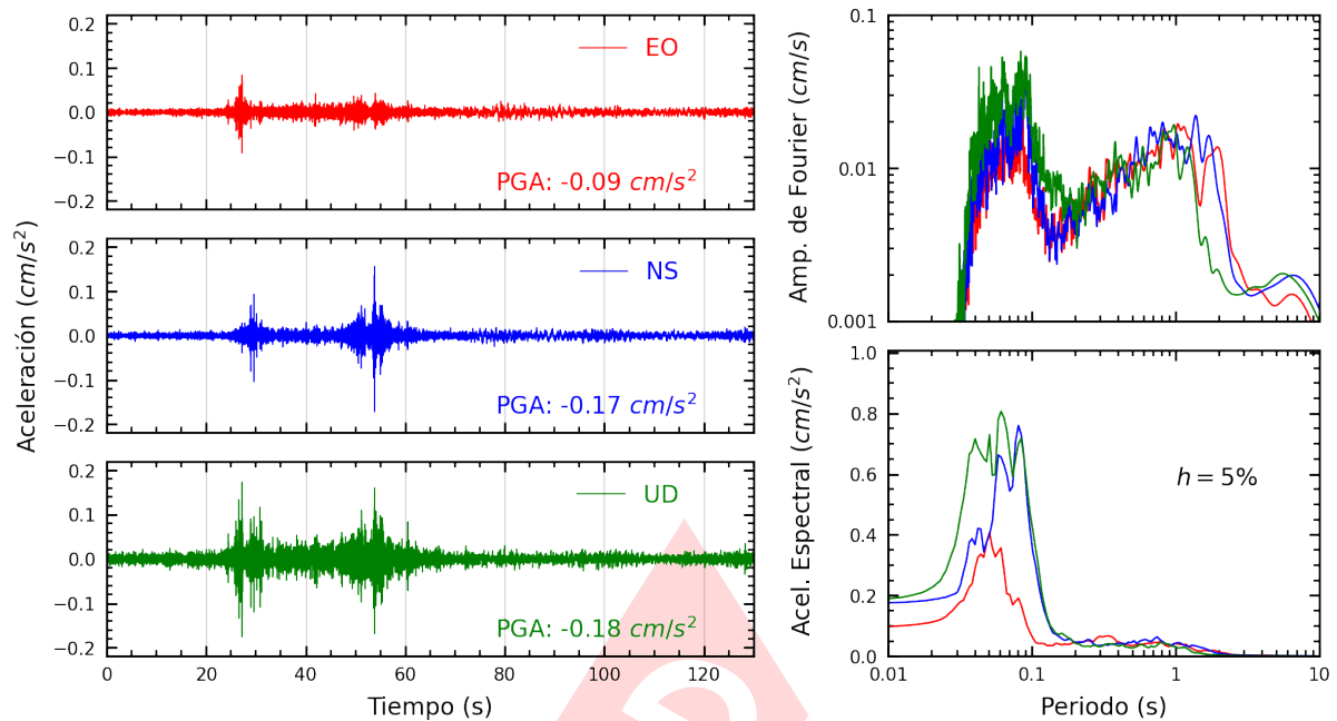
Figura A.9: Registros tiempo-historia, espectros de Fourier y de respuesta en las direcciones EO, NS y vertical de la estación SCCUS. Sismo de San Martín De Pangoa, Satipo - Junín del 2025-03-30, 23:50:25 (Hora local)
