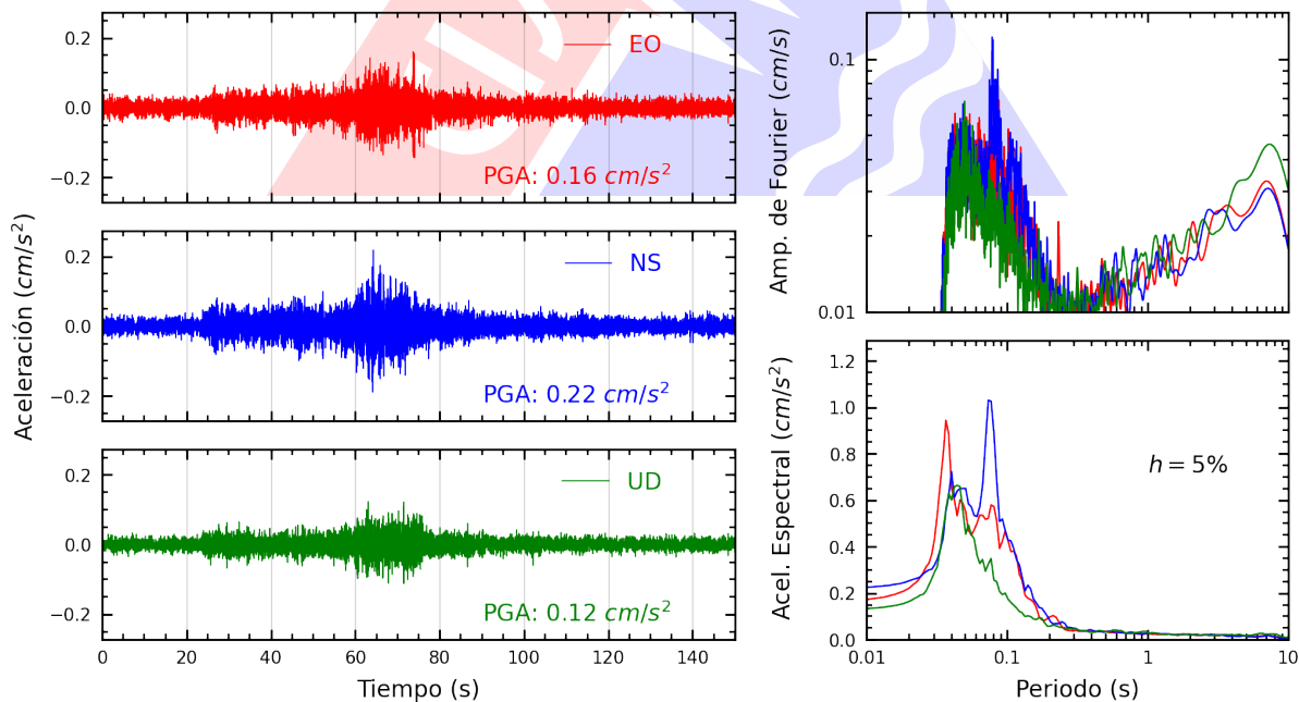
Figura A.4: Registros tiempo-historia, espectros de Fourier y de respuesta en las direcciones EO, NS y vertical de la estación JOSEO. Sismo de San Martín De Pangoa, Satipo - Junín del 2025-03-30, 23:50:25 (Hora local)
