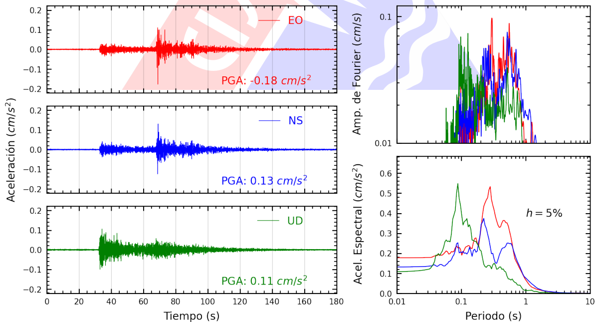
Figura A.8: Registros tiempo-historia, espectros de Fourier y de respuesta en las direcciones EO, NS y vertical de la estación UNIA. Sismo de San Martín De Pangoa, Satipo - Junín del 2025-03-30, 23:50:25 (Hora local)
