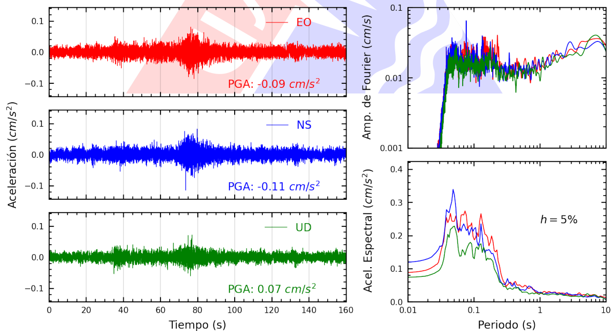
Figura A.14: Registros tiempo-historia, espectros de Fourier y de respuesta en las direcciones EO, NS y vertical de la estación FICPE. Sismo de San Martín De Pangoa, Satipo - Junín del 2025-03-30, 23:50:25 (Hora local)
