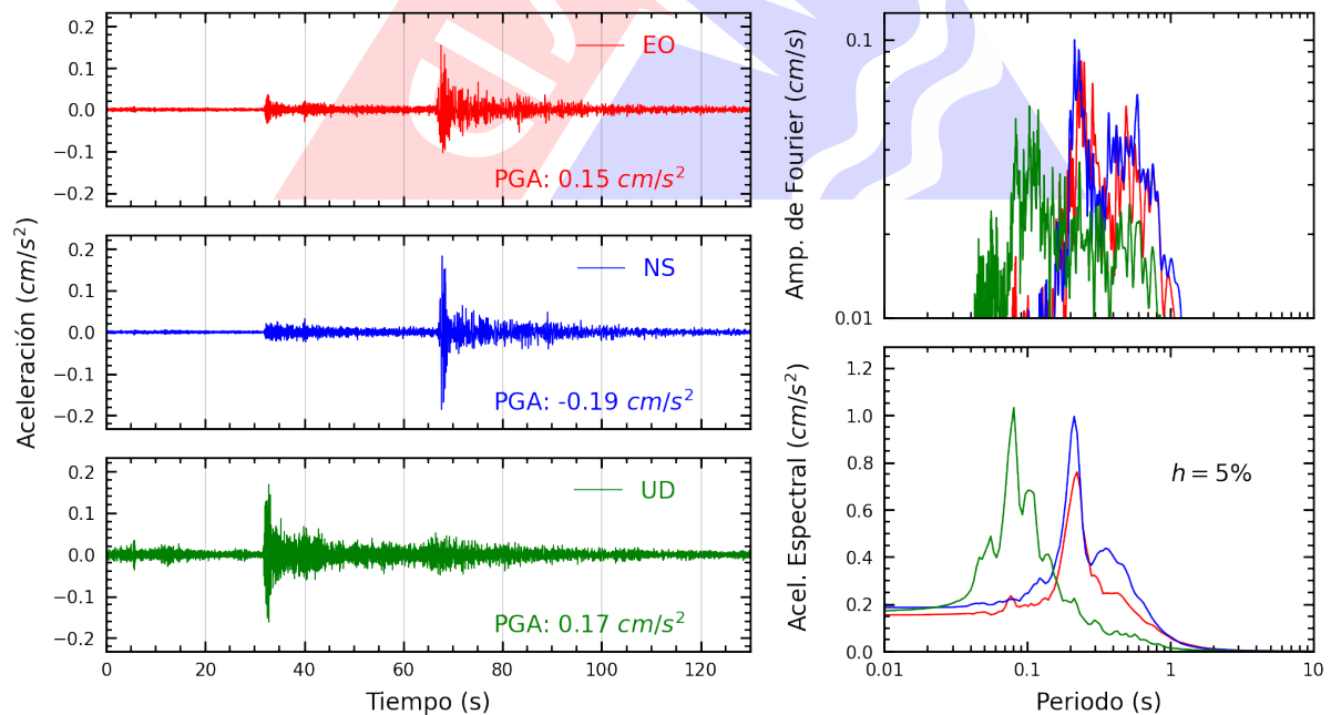
Figura A.6: Registros tiempo-historia, espectros de Fourier y de respuesta en las direcciones EO, NS y vertical de la estación SCPUC. Sismo de San Martín De Pangoa, Satipo - Junín del 2025-03-30, 23:50:25 (Hora local)
