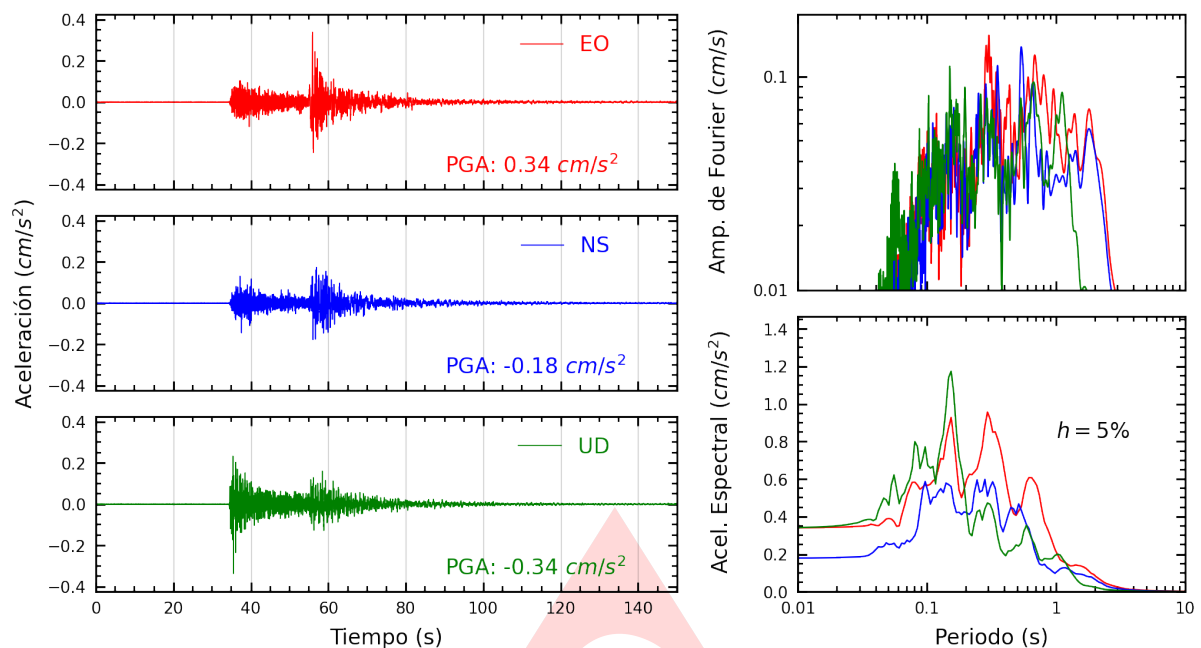
Figura A.1: Registros tiempo-historia, espectros de Fourier y de respuesta en las direcciones EO, NS y vertical de la estación UNCP. Sismo de San Martín De Pangoa, Satipo - Junín del 2025-03-30, 23:50:25 (Hora local)
