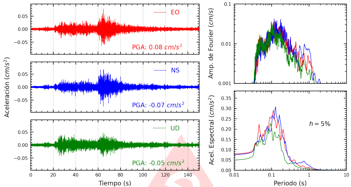
Figura A.19: Registros tiempo-historia, espectros de Fourier y de respuesta en las direcciones EO, NS y vertical de la estación JALV2. Sismo de San Martín De Pangoa, Satipo - Junín del 2025-03-30, 23:50:25 (Hora local)
