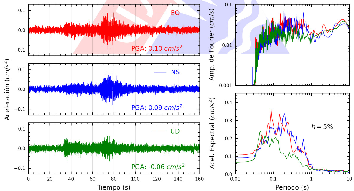
Figura A.16: Registros tiempo-historia, espectros de Fourier y de respuesta en las direcciones EO, NS y vertical de la estación USILP. Sismo de San Martín De Pangoa, Satipo - Junín del 2025-03-30, 23:50:25 (Hora local)
