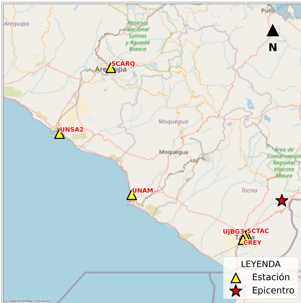
Figura 2: Mapa de ubicación de la(s) estación(es) acelerográfica(s) correspondiente(s) al Sismo de Tarata, Tarata - Tacna del 12 de julio de 2024 a las 13:19:03 (hora local)
