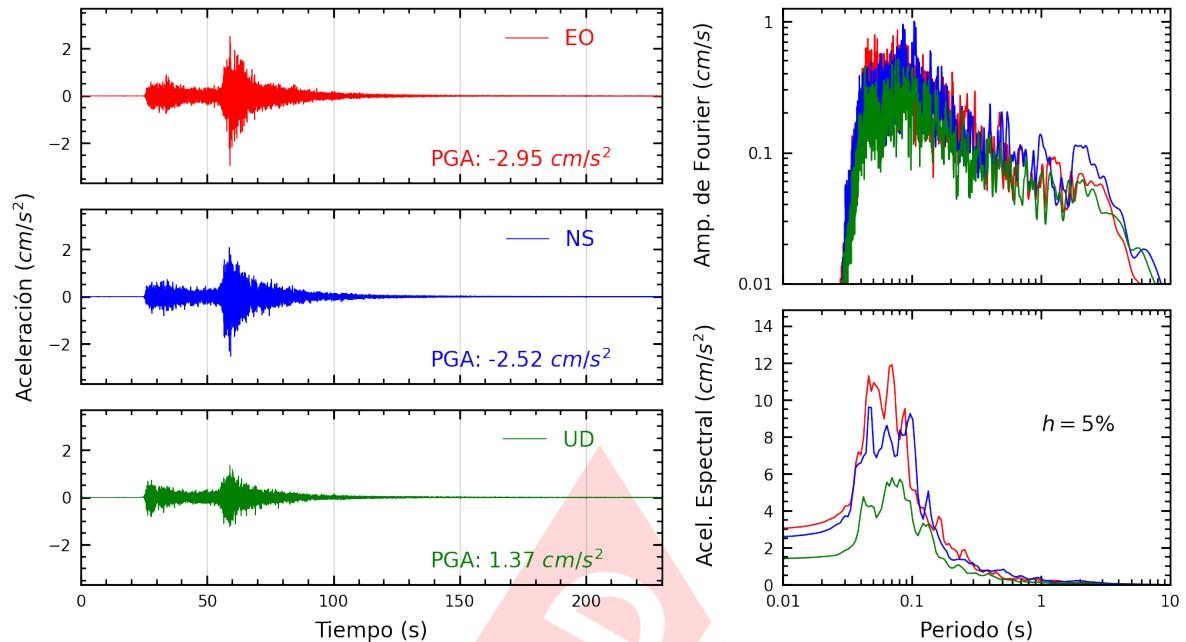
Figura A.5: Registros tiempo-historia, espectros de Fourier y de respuesta en las direcciones EO, NS y vertical de la estación UNSA2. Sismo de Tarata, Tarata - Tacna del 2024-07-12, 13:19:03 (Hora local)
