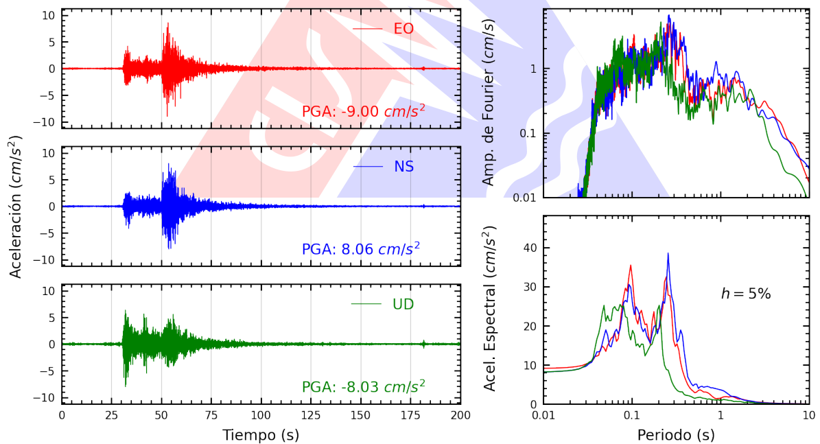
Figura A.2: Registros tiempo-historia, espectros de Fourier y de respuesta en las direcciones EO, NS y vertical de la estación SCTAC. Sismo de Tarata, Tarata - Tacna del 2024-07-12, 13:19:03 (Hora local)
