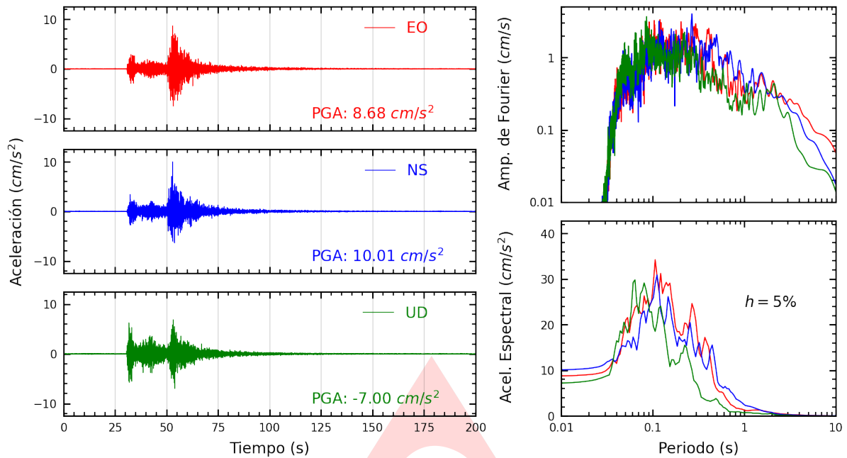
Figura A.1: Registros tiempo-historia, espectros de Fourier y de respuesta en las direcciones EO, NS y vertical de la estación UJBG3. Sismo de Tarata, Tarata - Tacna del 2024-07-12, 13:19:03 (Hora local)
