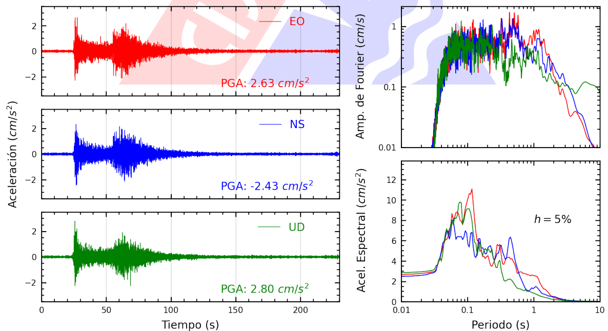
Figura A.6: Registros tiempo-historia, espectros de Fourier y de respuesta en las direcciones EO, NS y vertical de la estación SCARQ. Sismo de Tarata, Tarata - Tacna del 2024-07-12, 13:19:03 (Hora local)
