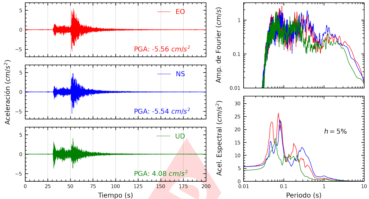
Figura A.3: Registros tiempo-historia, espectros de Fourier y de respuesta en las direcciones EO, NS y vertical de la estación CREY. Sismo de Tarata, Tarata - Tacna del 2024-07-12, 13:19:03 (Hora local)
