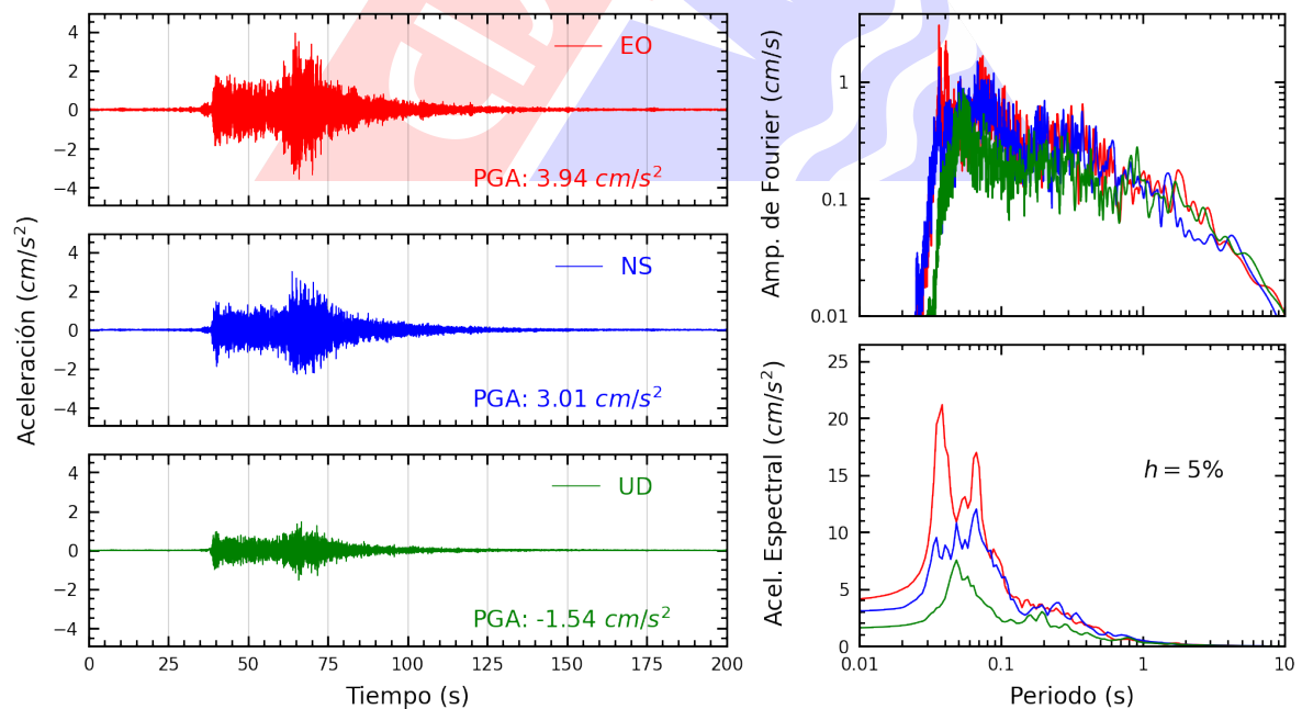
Figura A.4: Registros tiempo-historia, espectros de Fourier y de respuesta en las direcciones EO, NS y vertical de la estación UNAM. Sismo de Tarata, Tarata - Tacna del 2024-07-12, 13:19:03 (Hora local)
